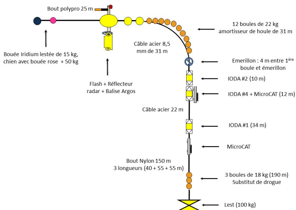
Figure 20 : schéma du mouillage "IODA"
