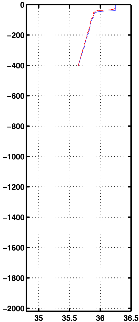
Sali 3092
