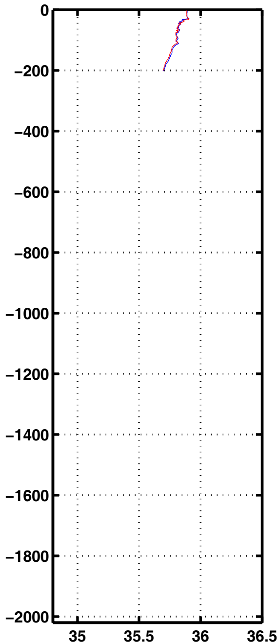
Sali 3246
