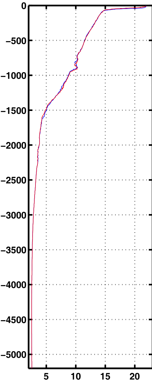
Tempe 3031
