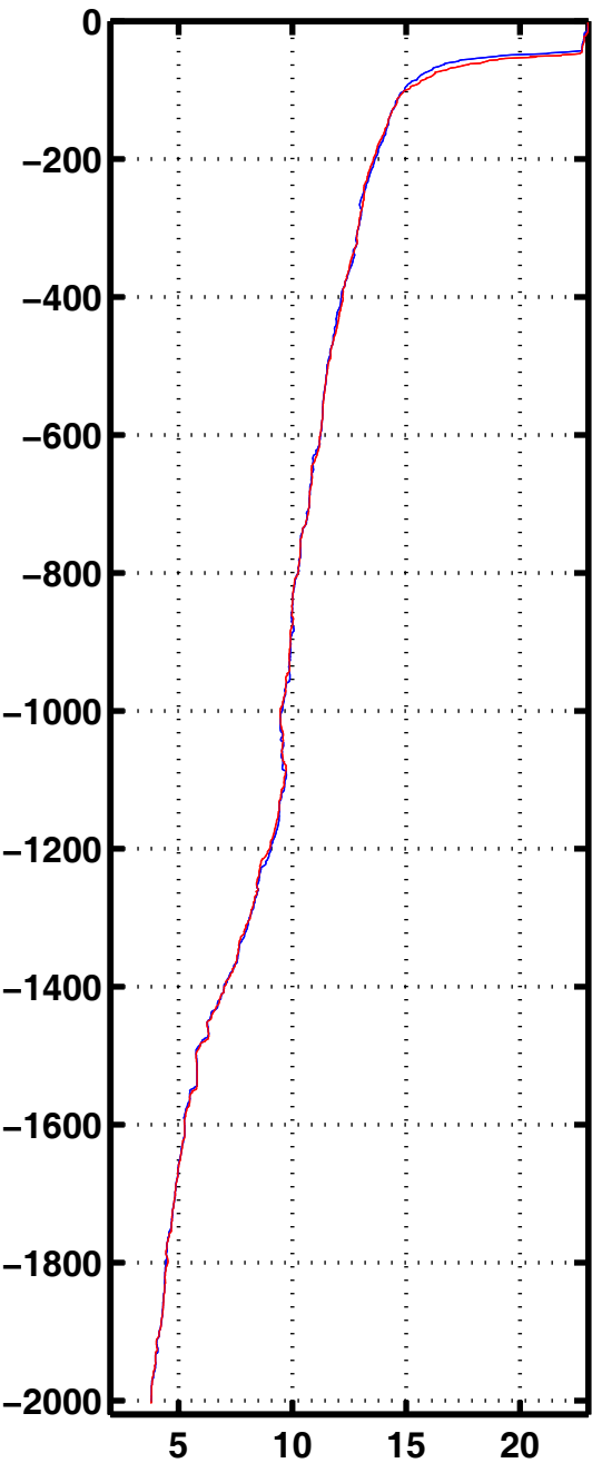
Tempe 3081
