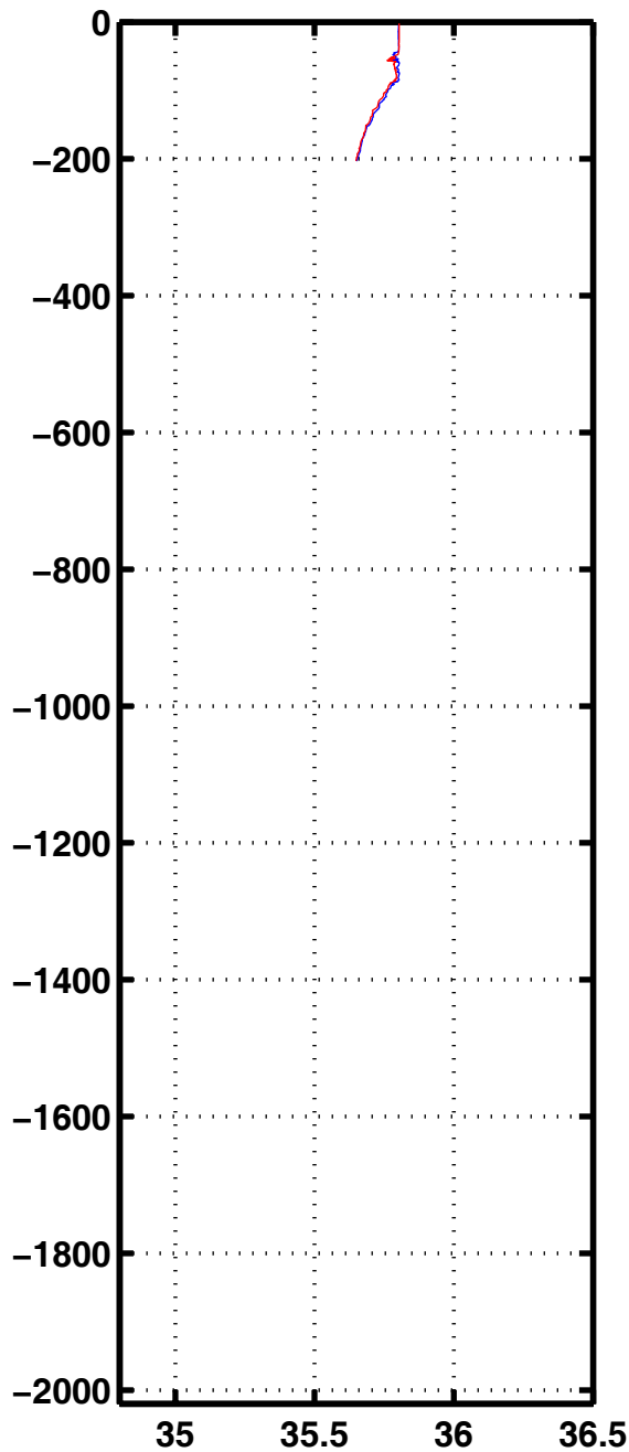
Sali 3331
