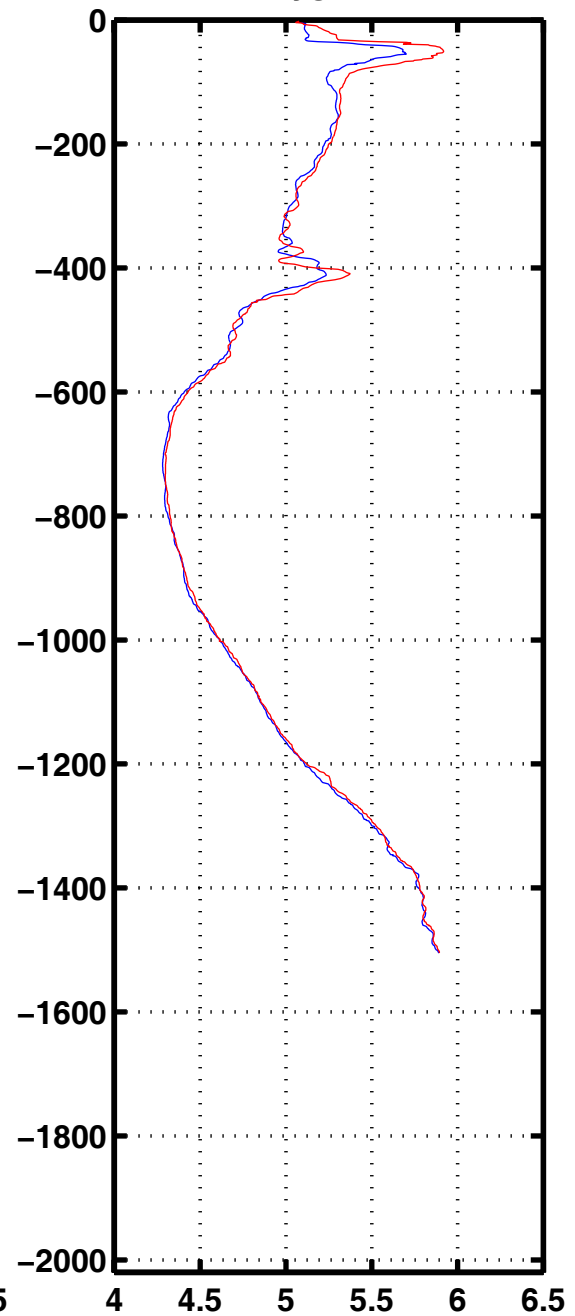
Oxyg 3251
