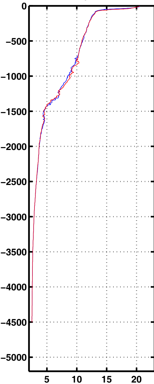
Tempe 3004
