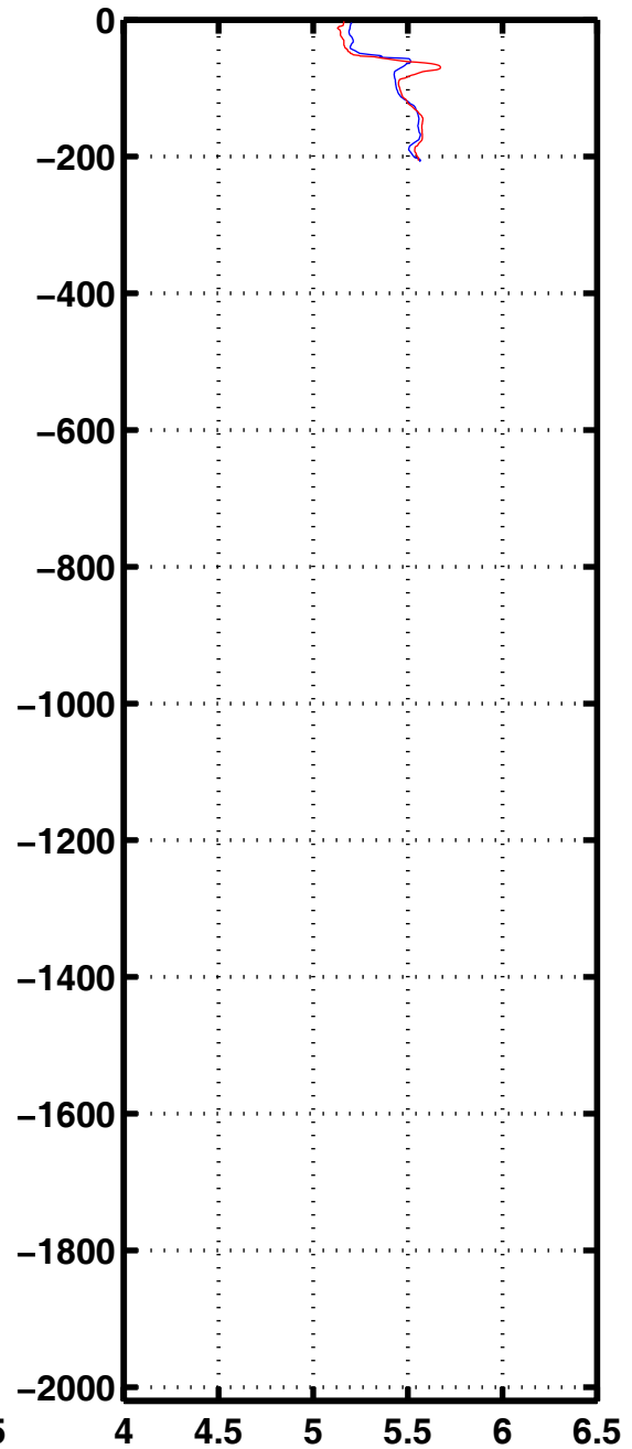
Oxyg 3333
