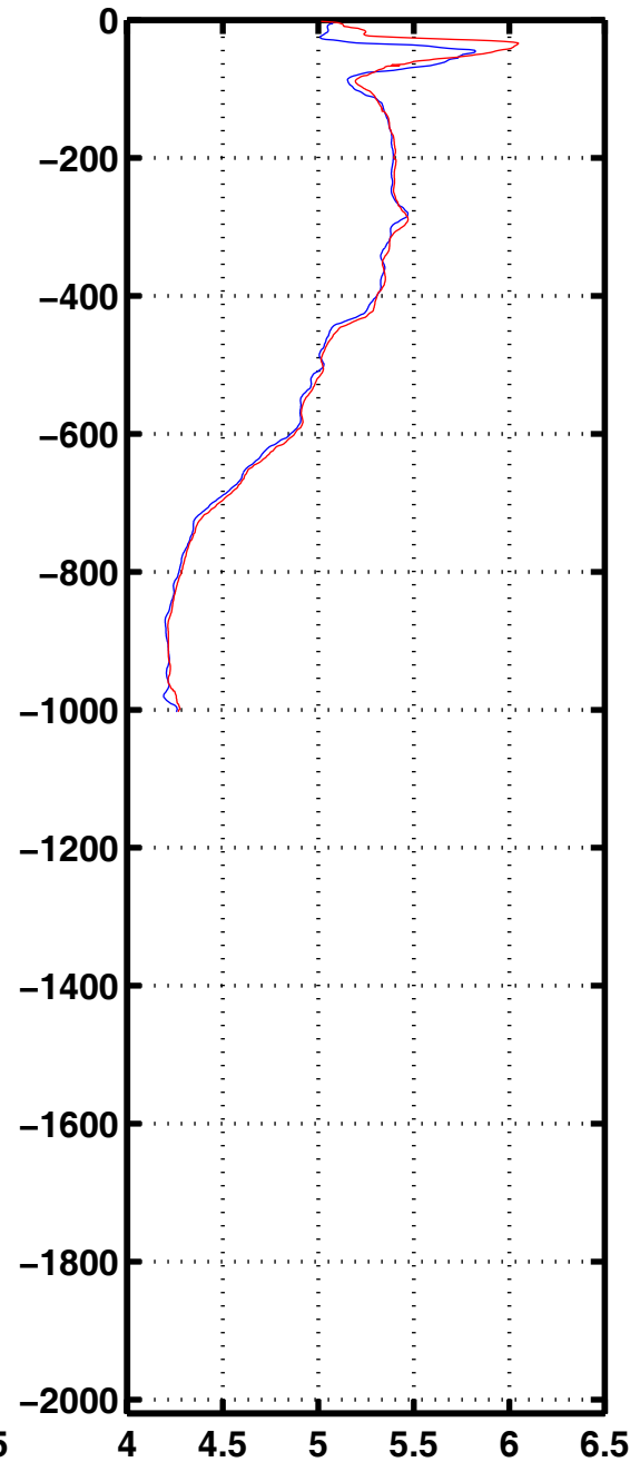
Oxyg 3088
