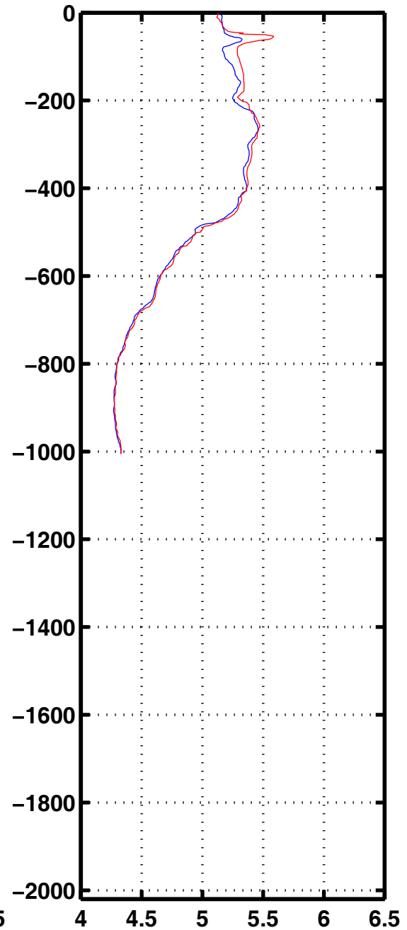
Oxyg 3328
