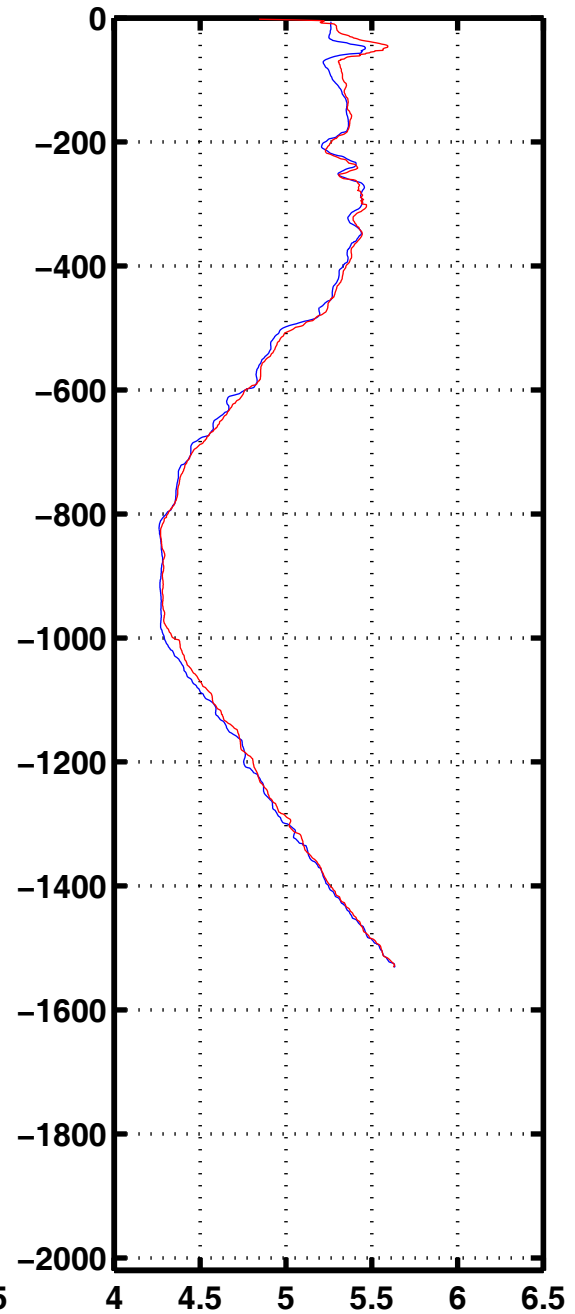
Oxyg 3335
