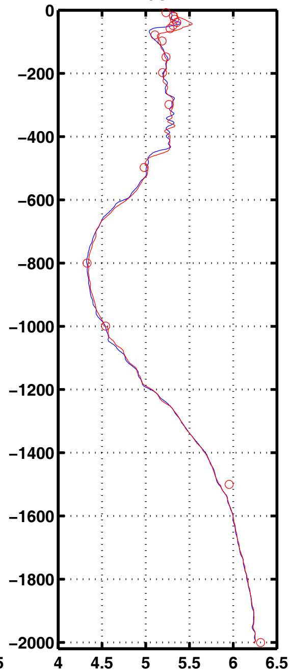
Oxyg 3062
