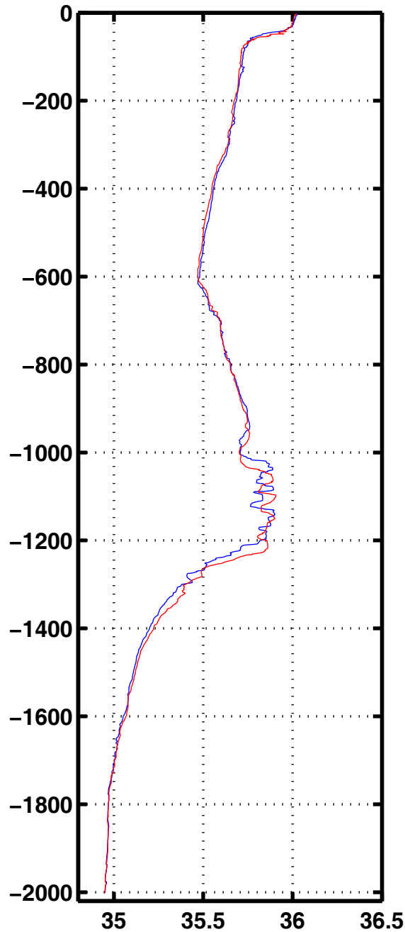
Sali 3016
