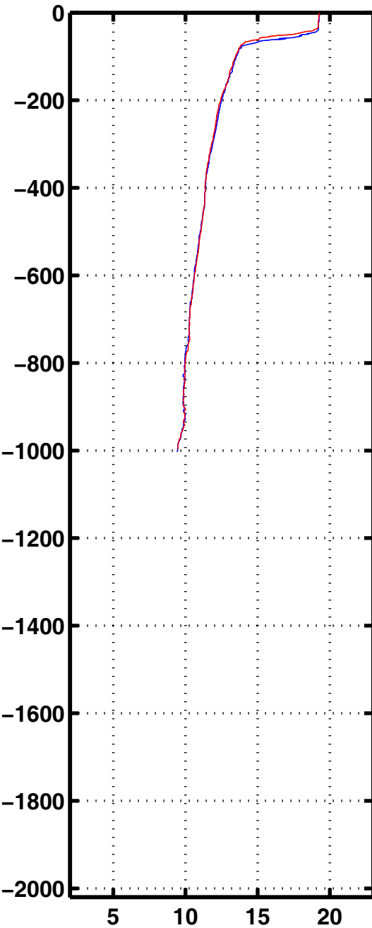
Tempe 3326
