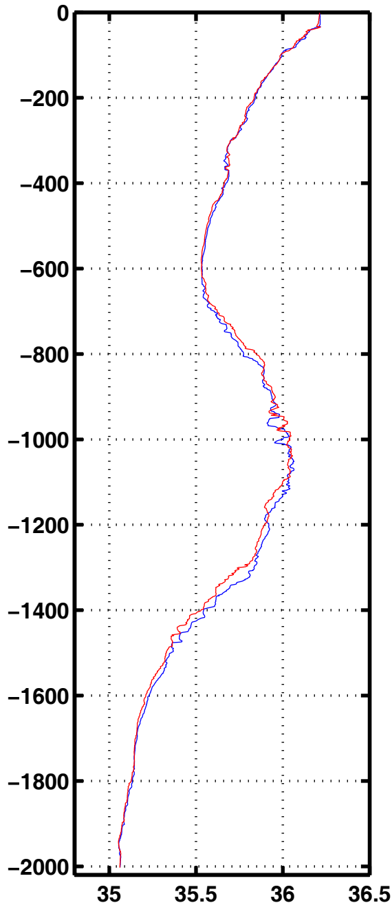
Sali 3044
