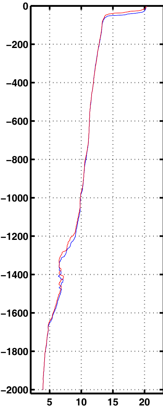
Tempe 3026
