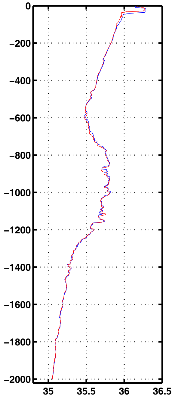
Sali 3083
