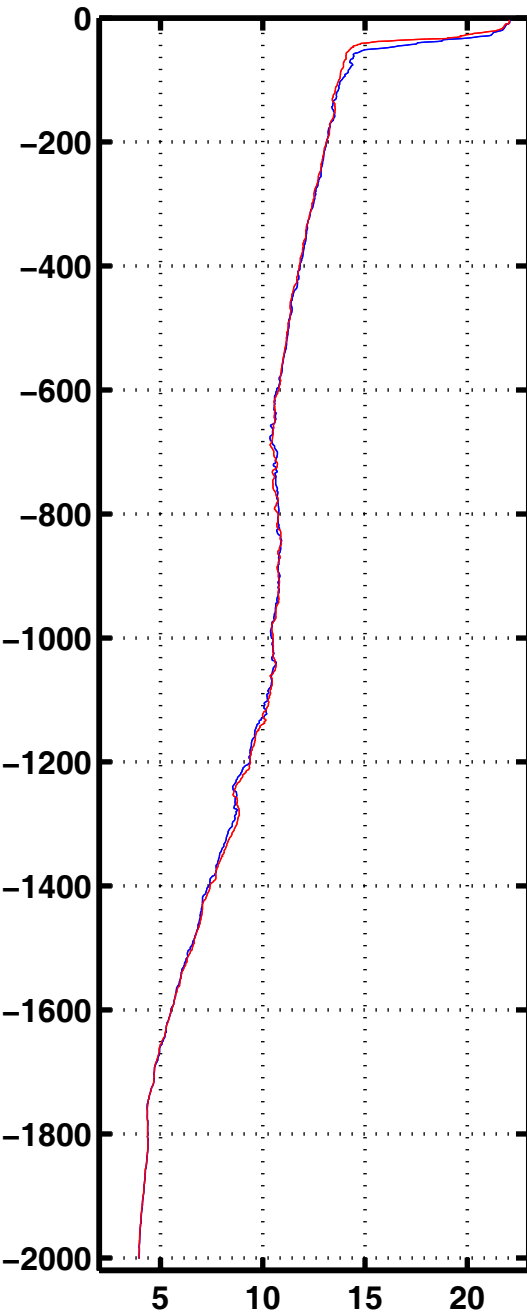
Tempe 3007
