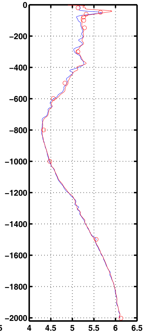
Oxyg 3052
