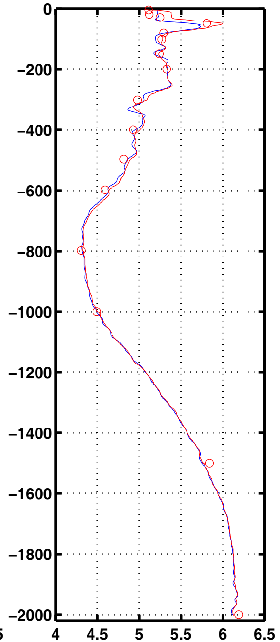
Oxyg 3075
