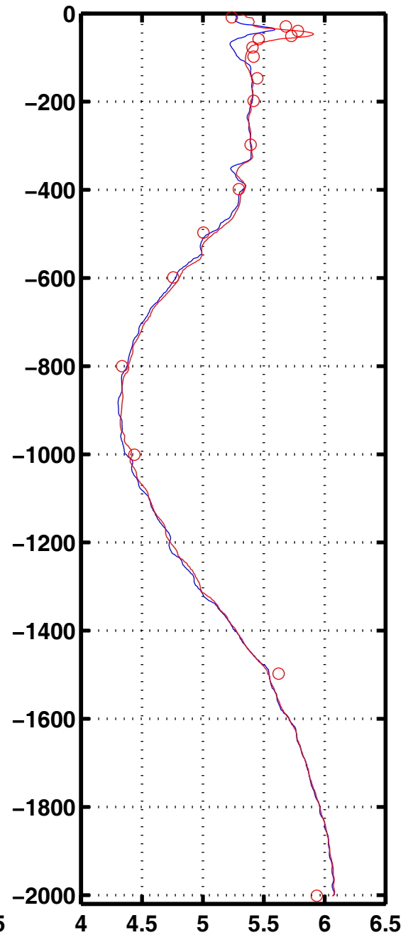
Oxyg 3049
