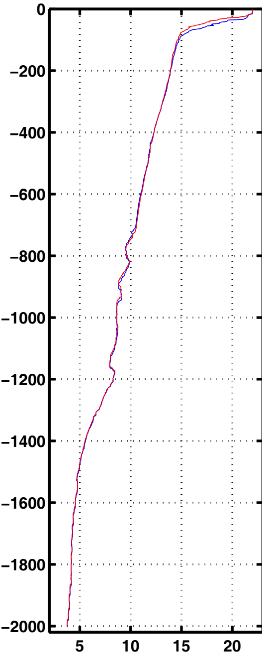
Tempe 3077
