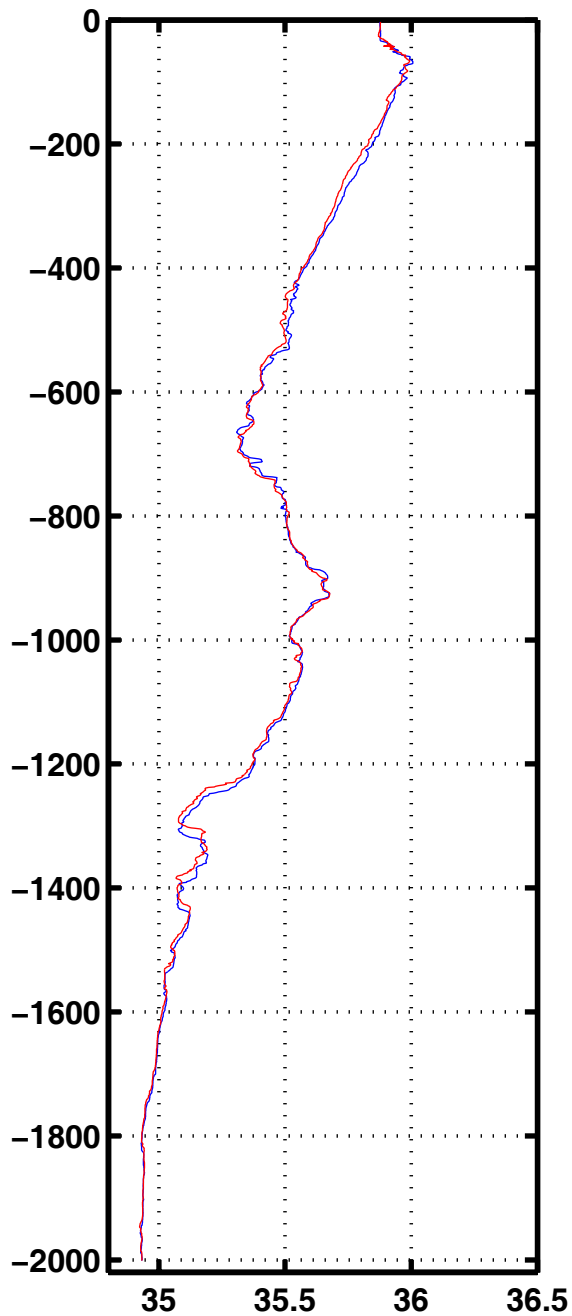
Sali 3070
