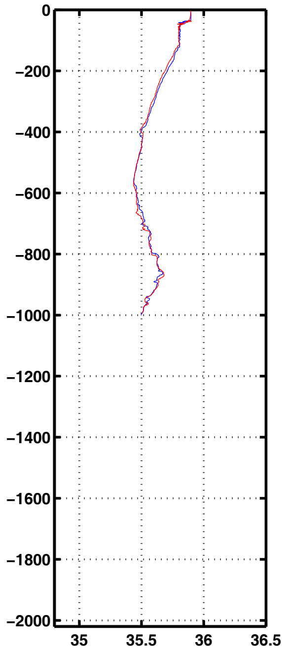
Sali 3244
