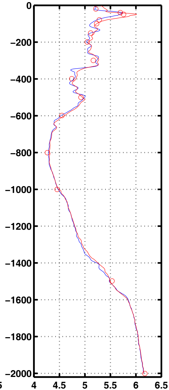
Oxyg 3058
