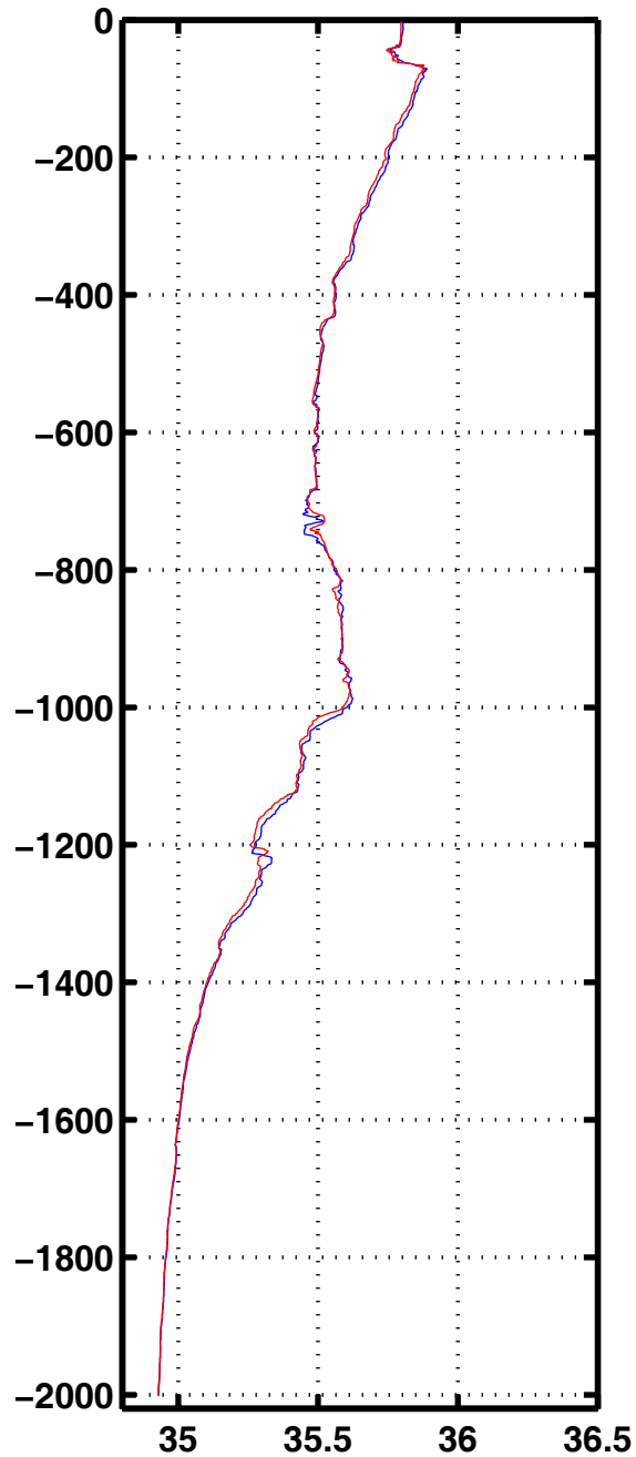
Sali 3064
