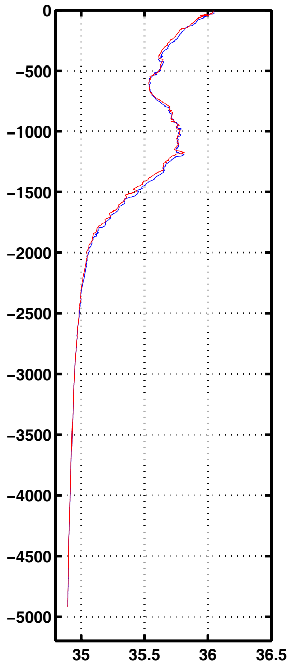
Sali 3036
