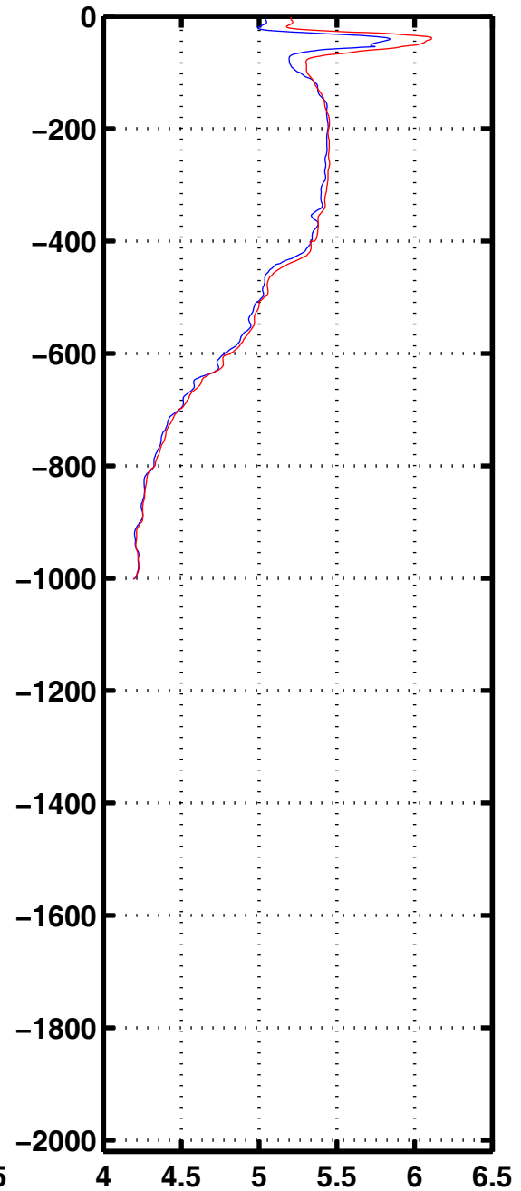
Oxyg 3091
