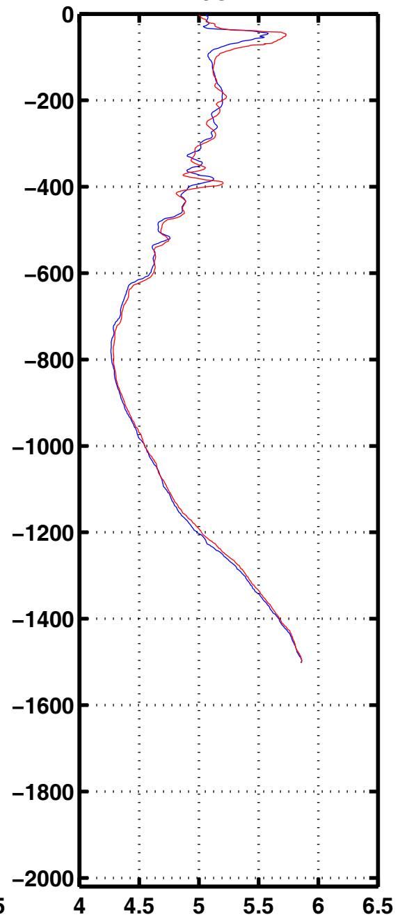
Oxyg 3155
