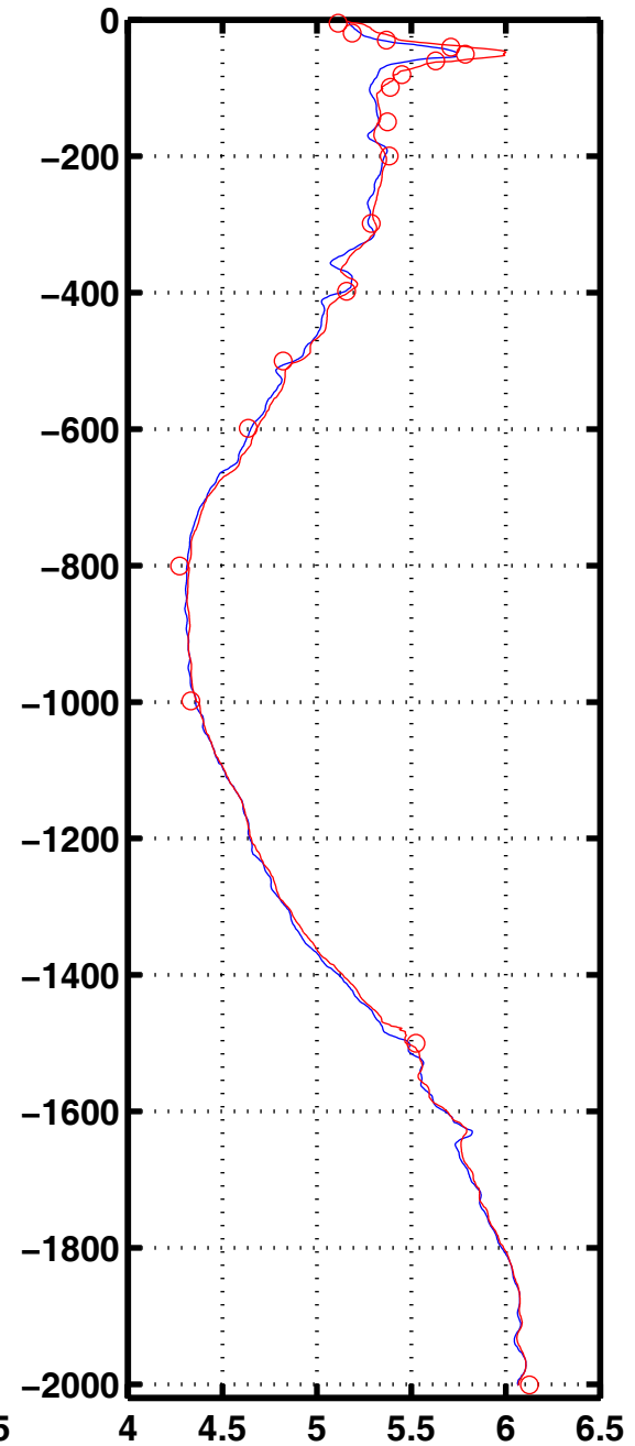
Oxyg 3017
