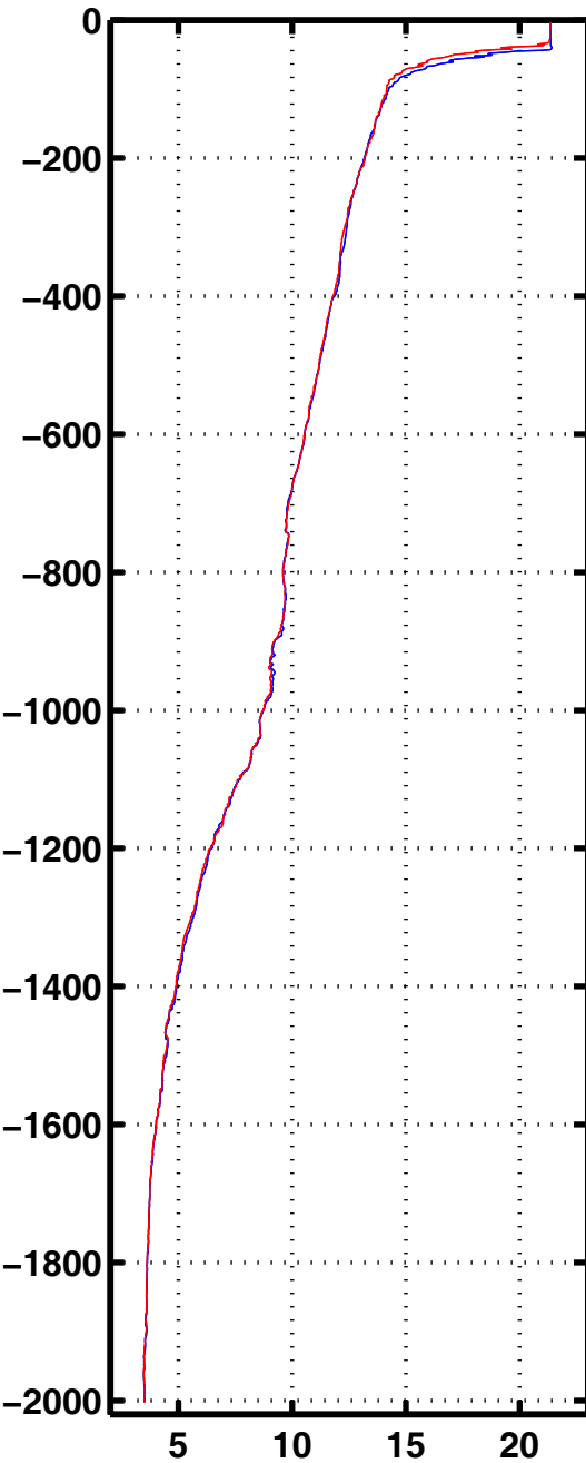
Tempe 3075
