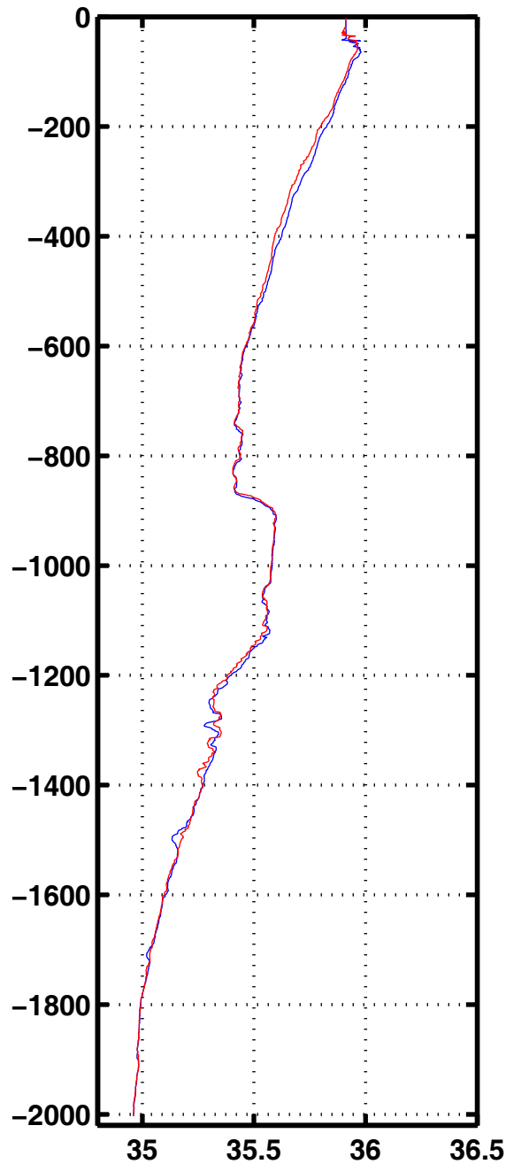
Sali 3052
