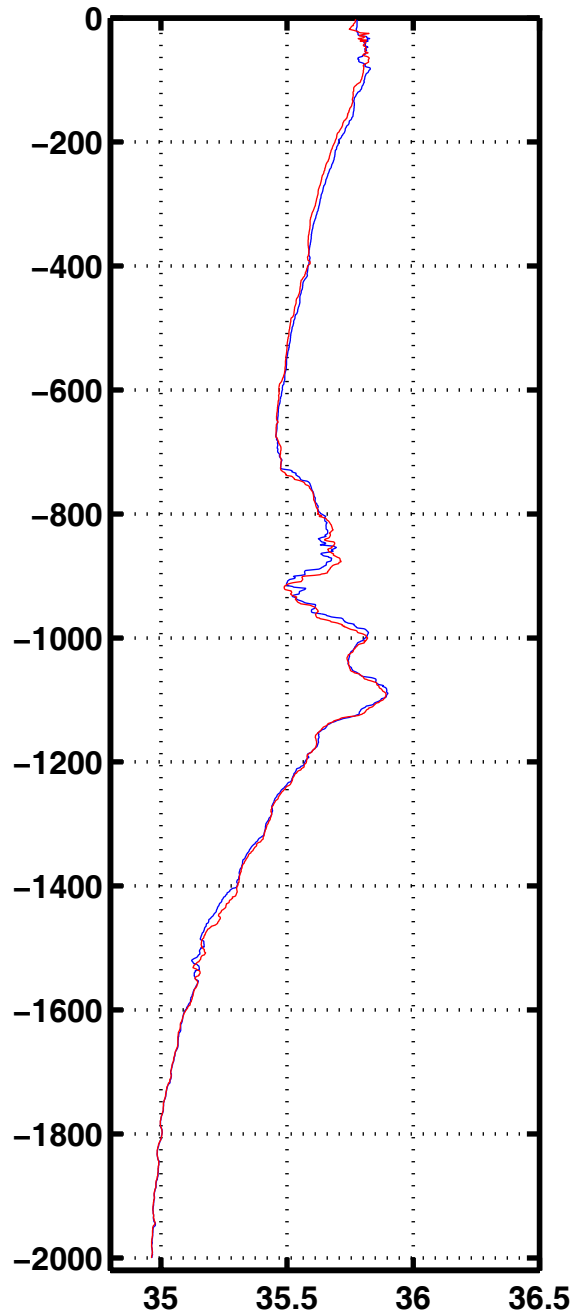
Sali 3022
