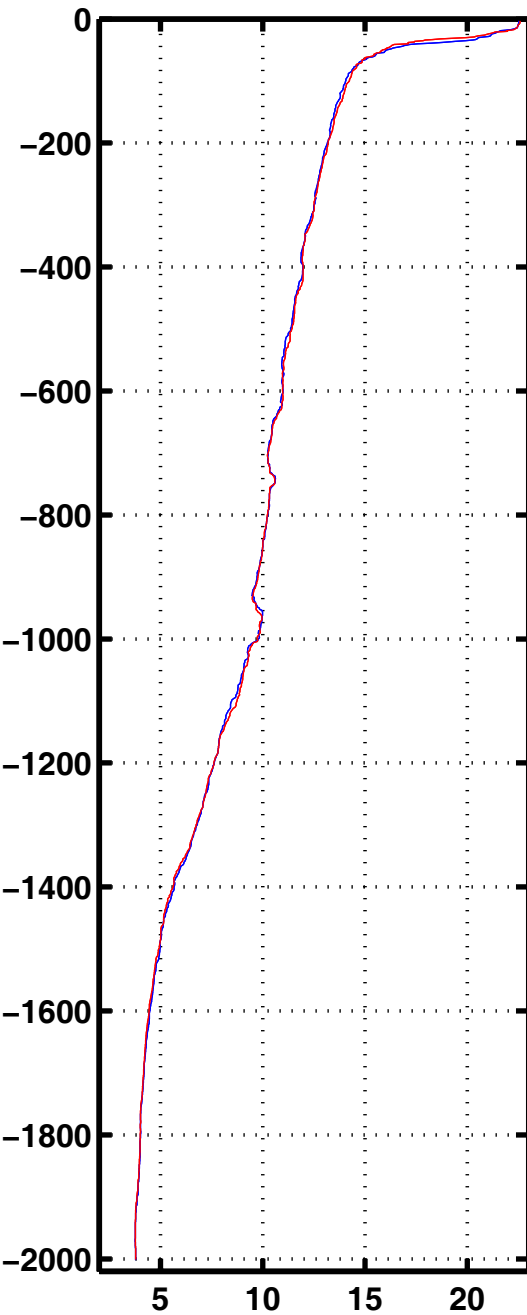
Tempe 3010
