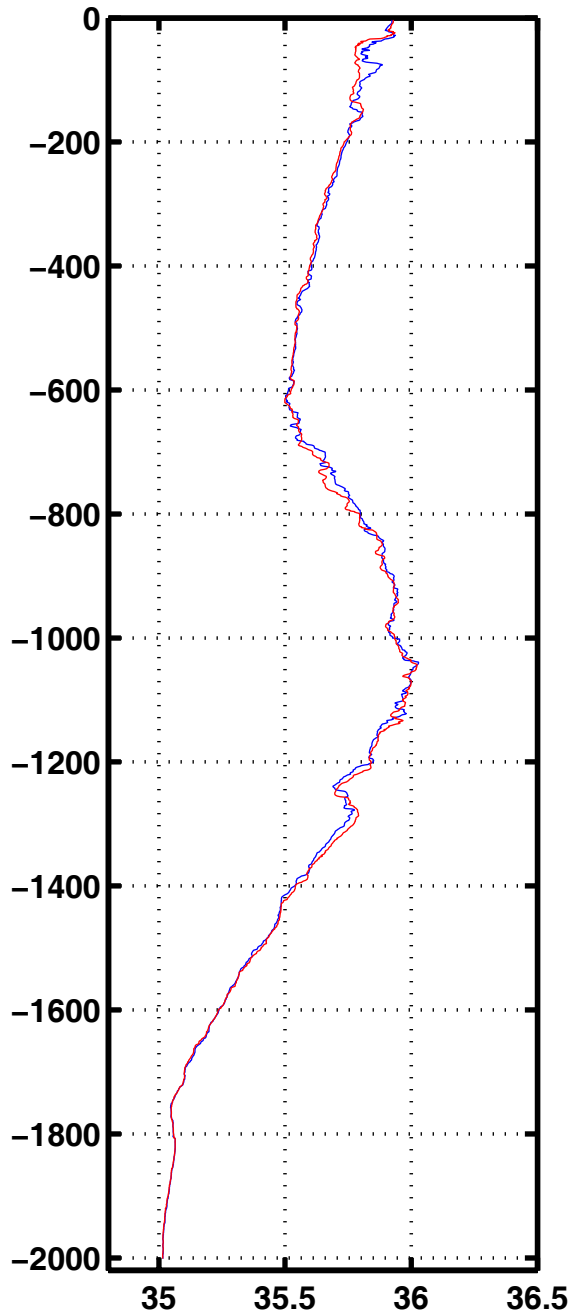
Sali 3007
