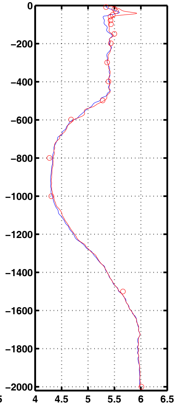
Oxyg 3028
