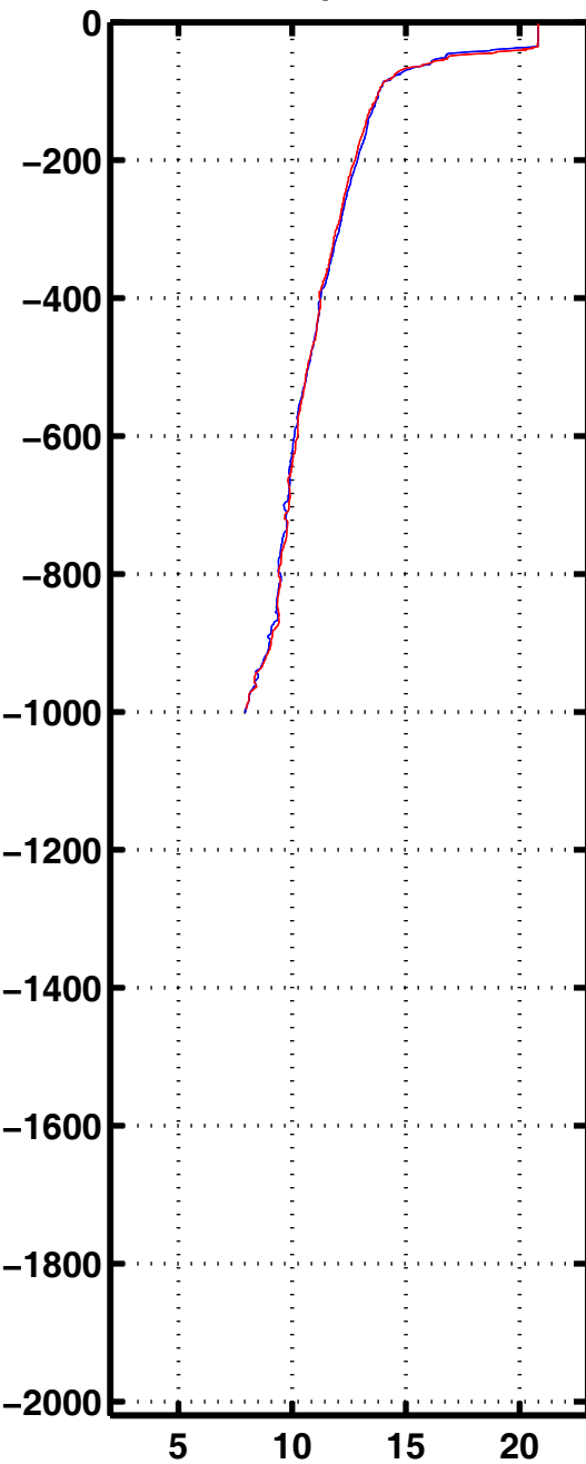
Tempe 3244
