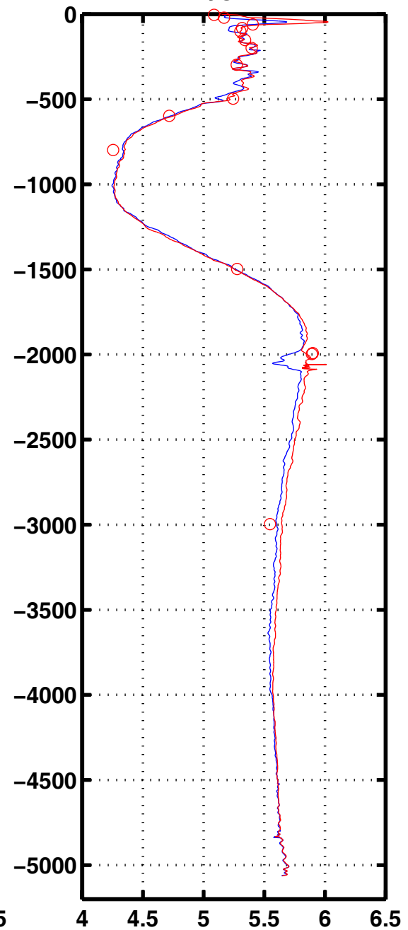
Oxyg 3006
