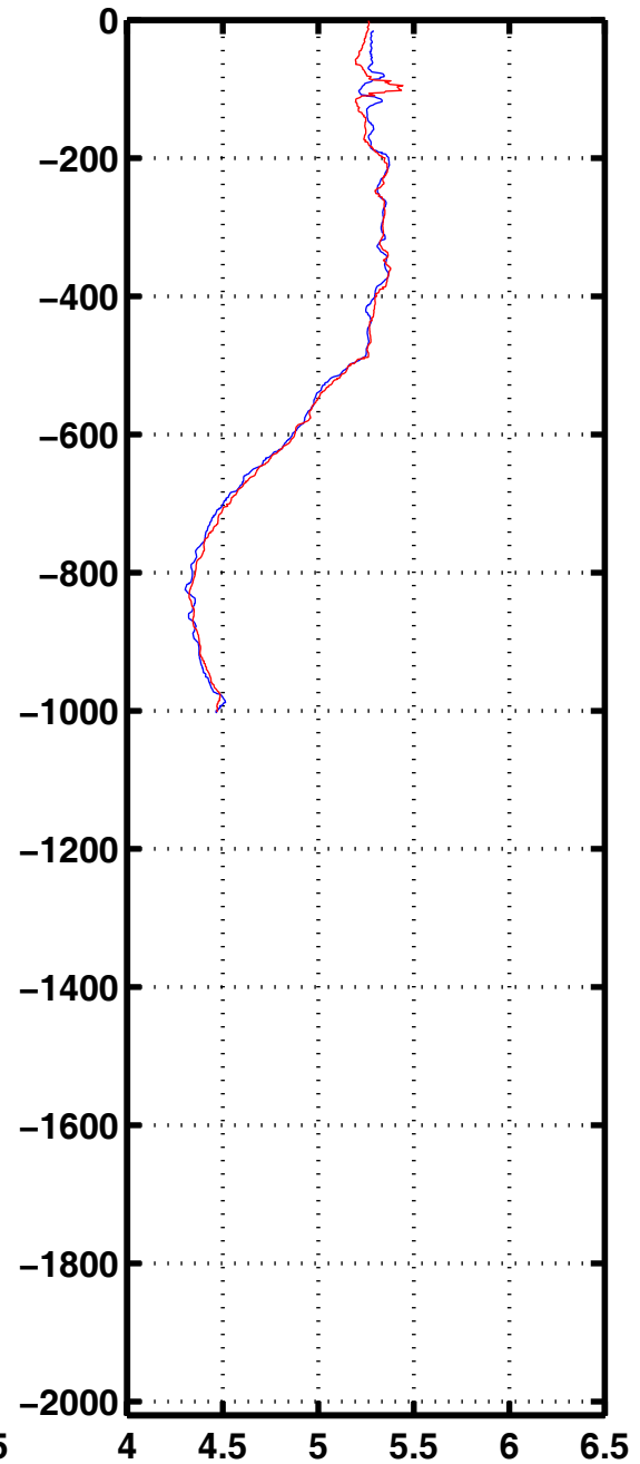
Oxyg 3338
