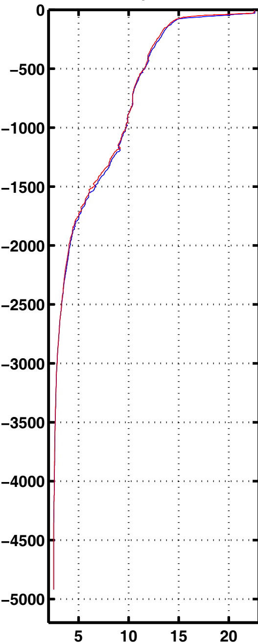
Tempe 3036
