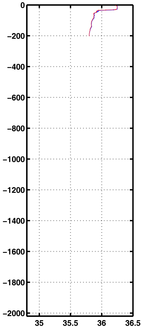
Sali 3094
