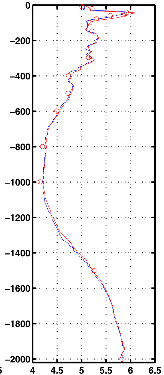
Oxyg 3044
