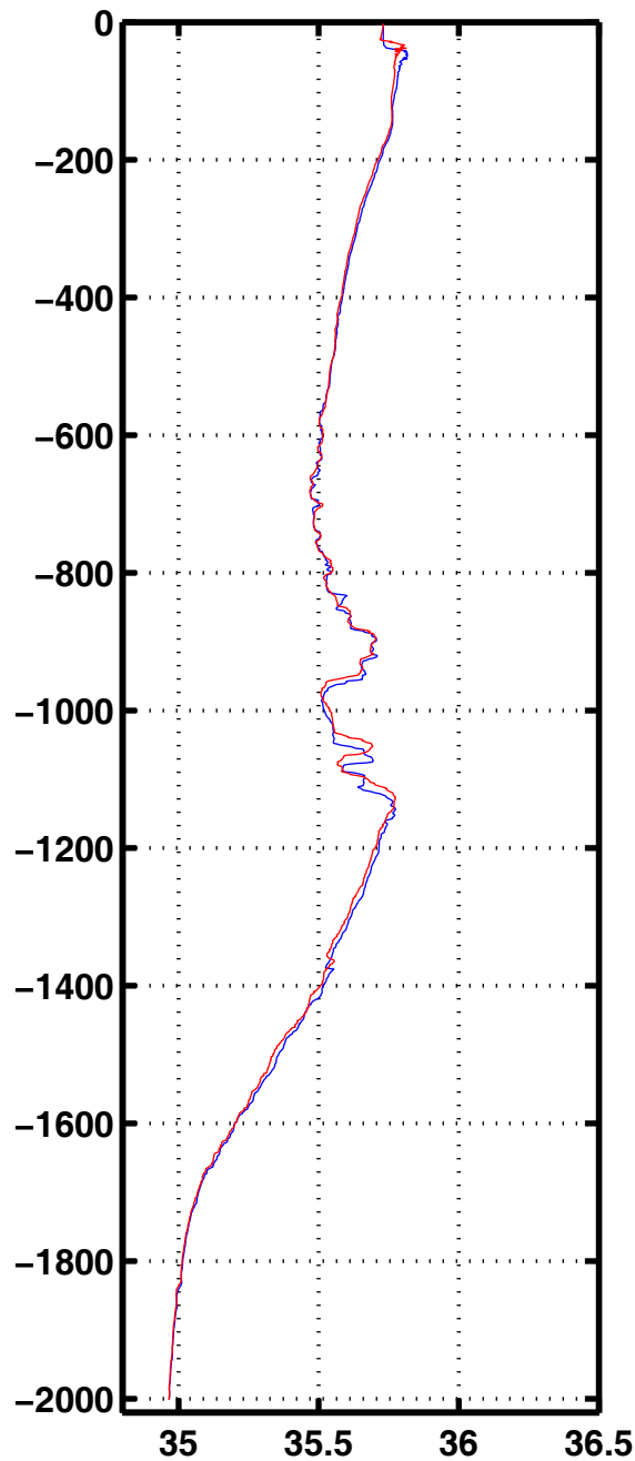
Sali 3065
