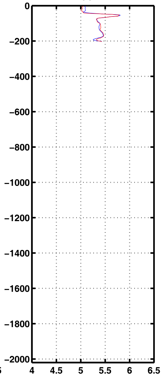
Oxyg 3163
