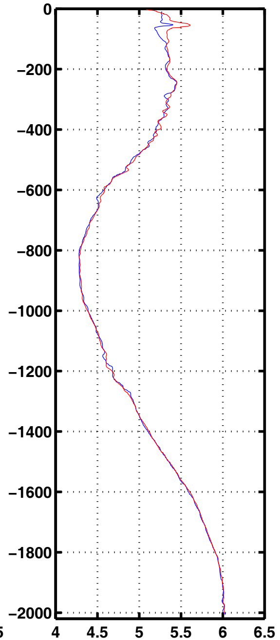
Oxyg 3336
