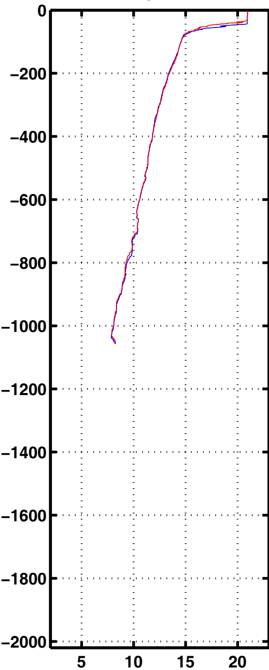
Tempe 3158
