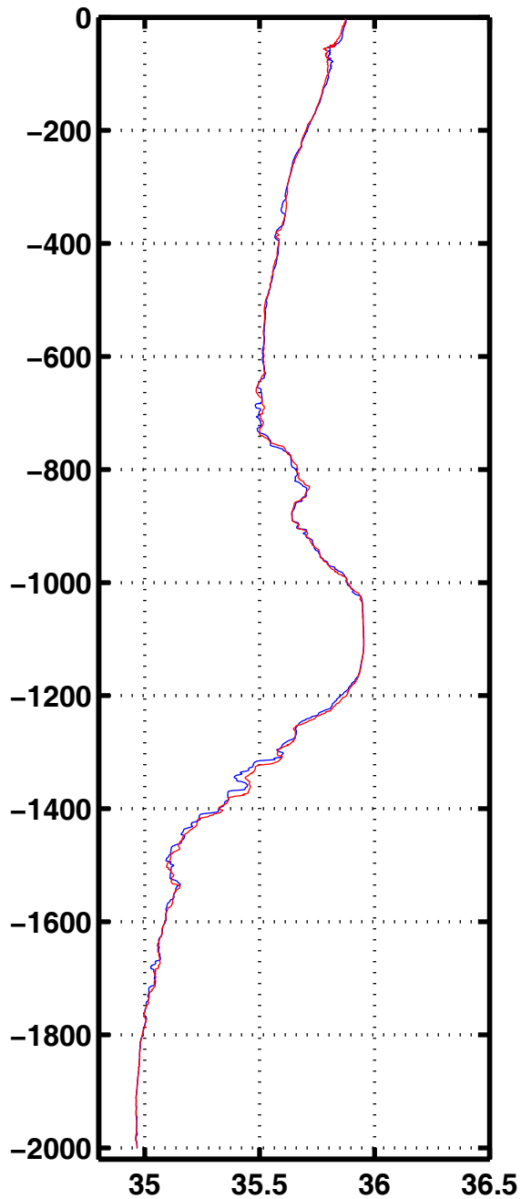
Sali 3024
