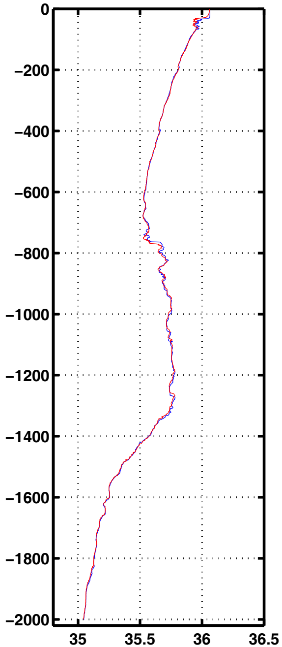
Sali 3042
