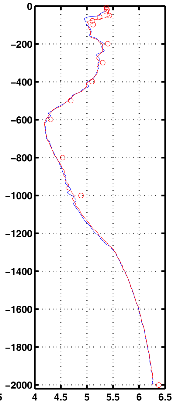
Oxyg 3067
