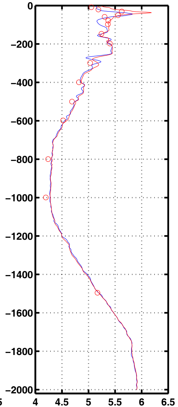
Oxyg 3007
