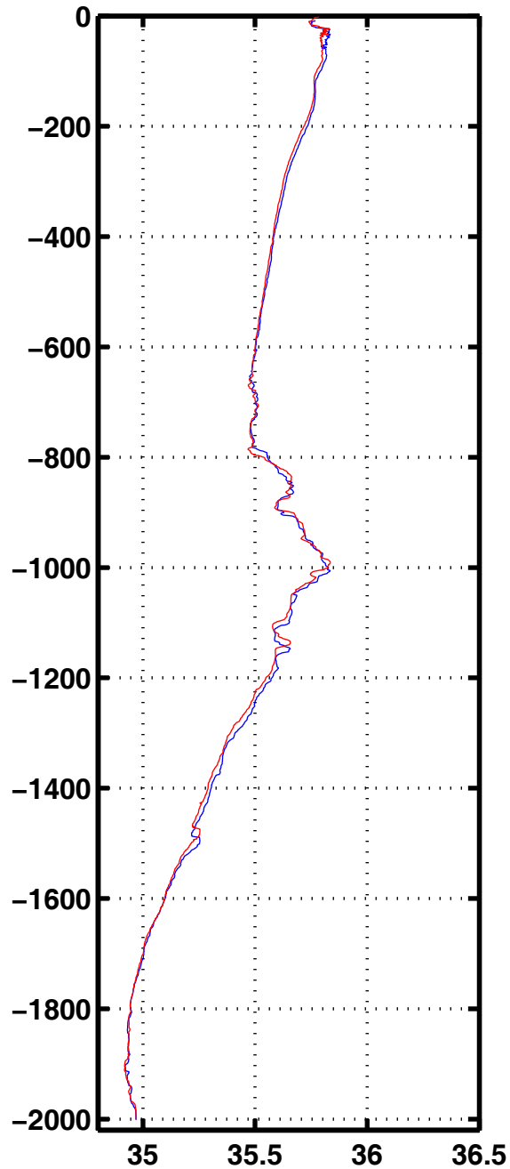
Sali 3027
