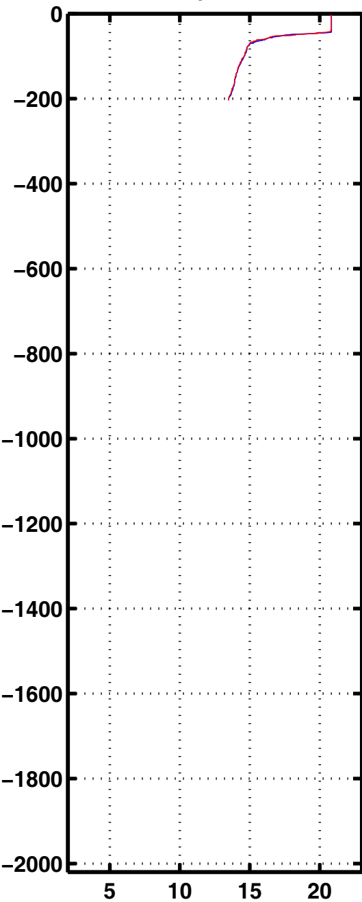
Tempe 3163
