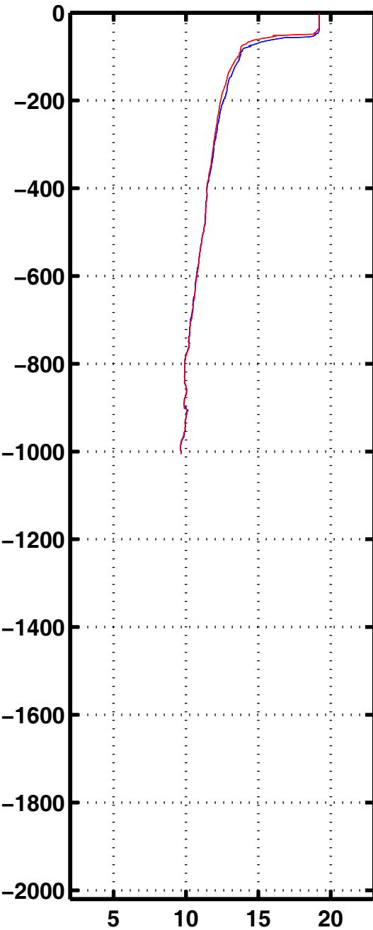
Tempe 3328
