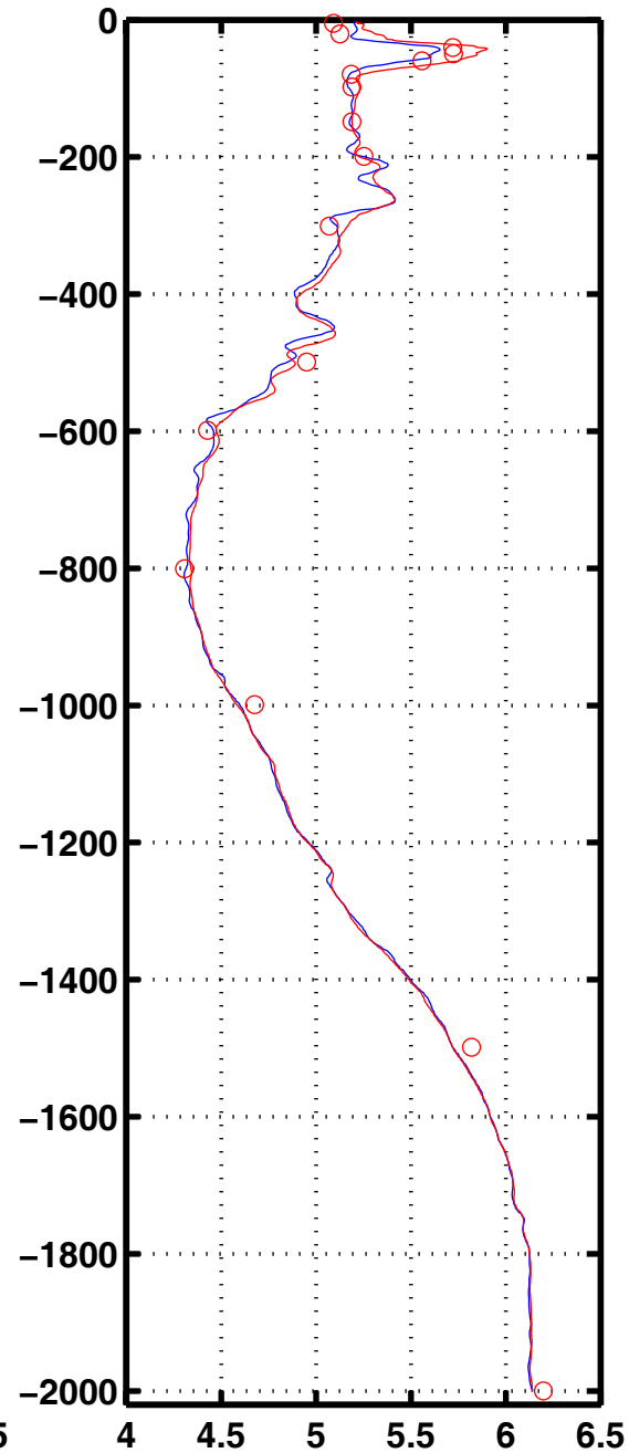
Oxyg 3076
