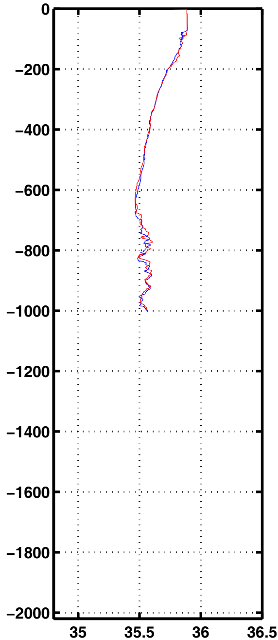
Sali 3338
