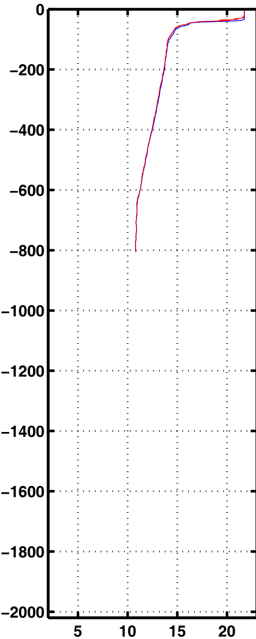
Tempe 3095
