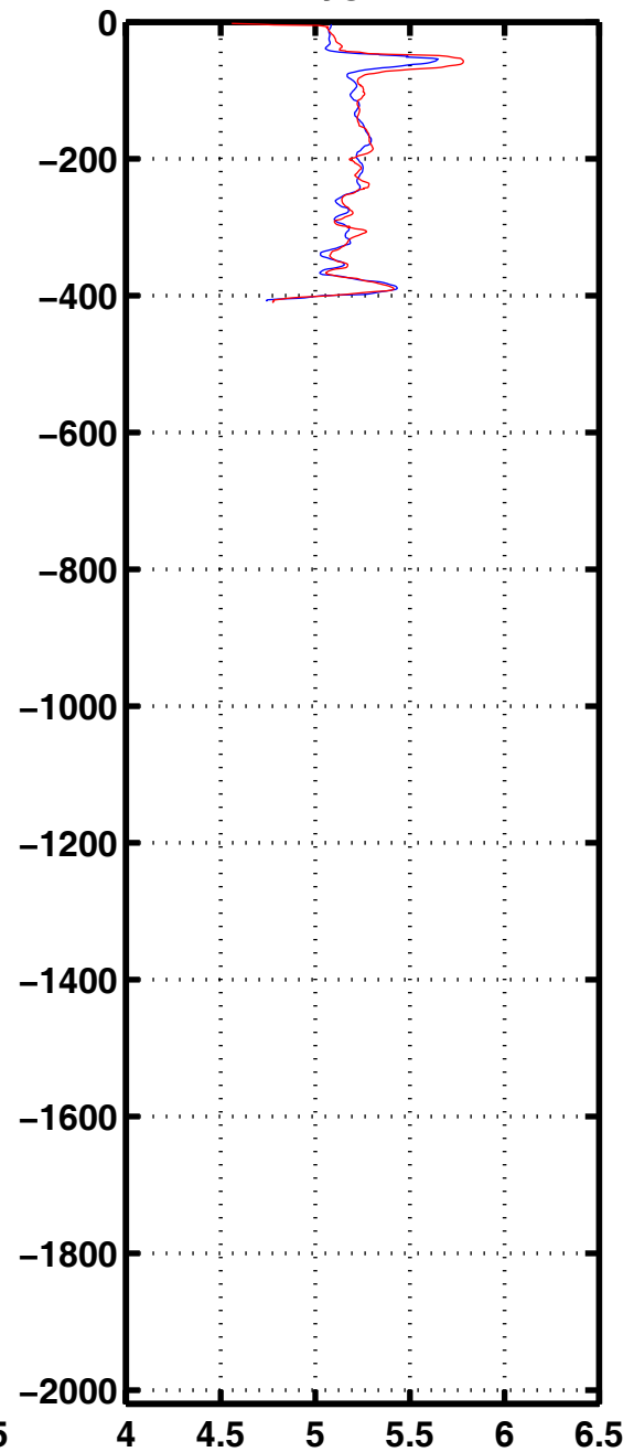
Oxyg 3161
