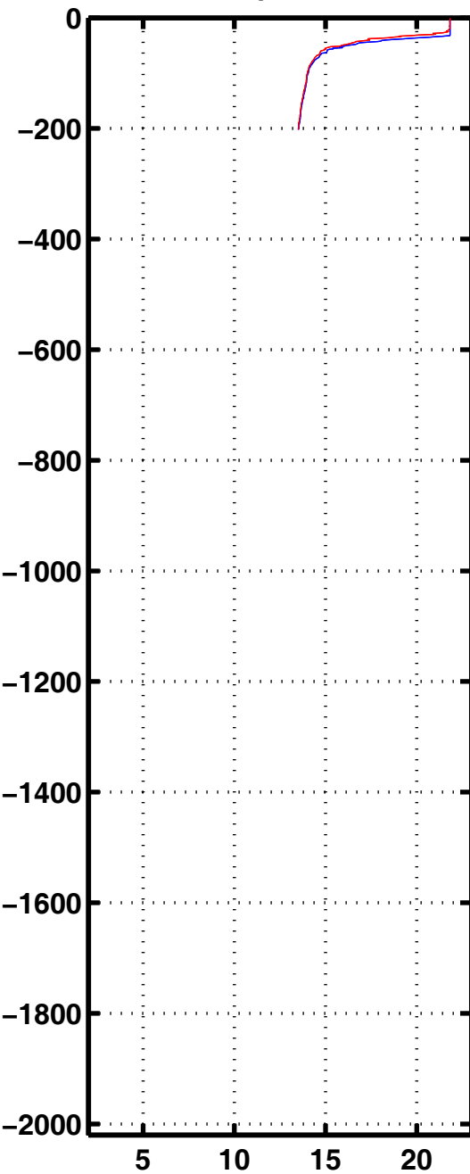
Tempe 3086
