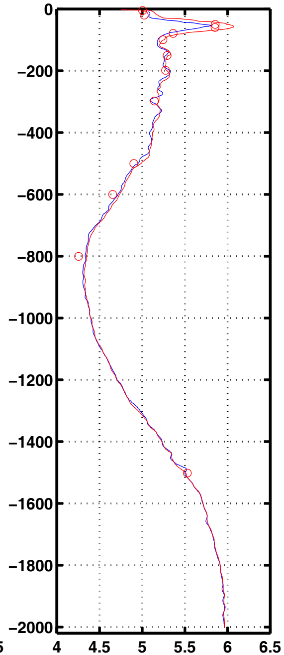
Oxyg 3035
