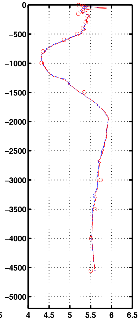
Oxyg 3025
