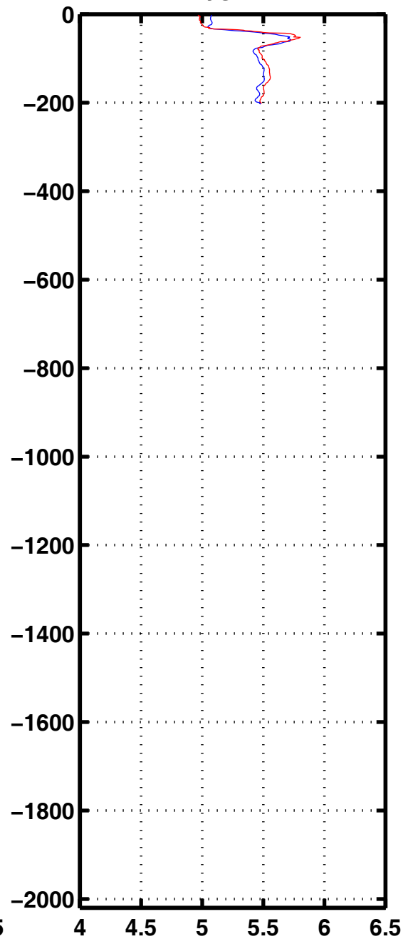
Oxyg 3247
