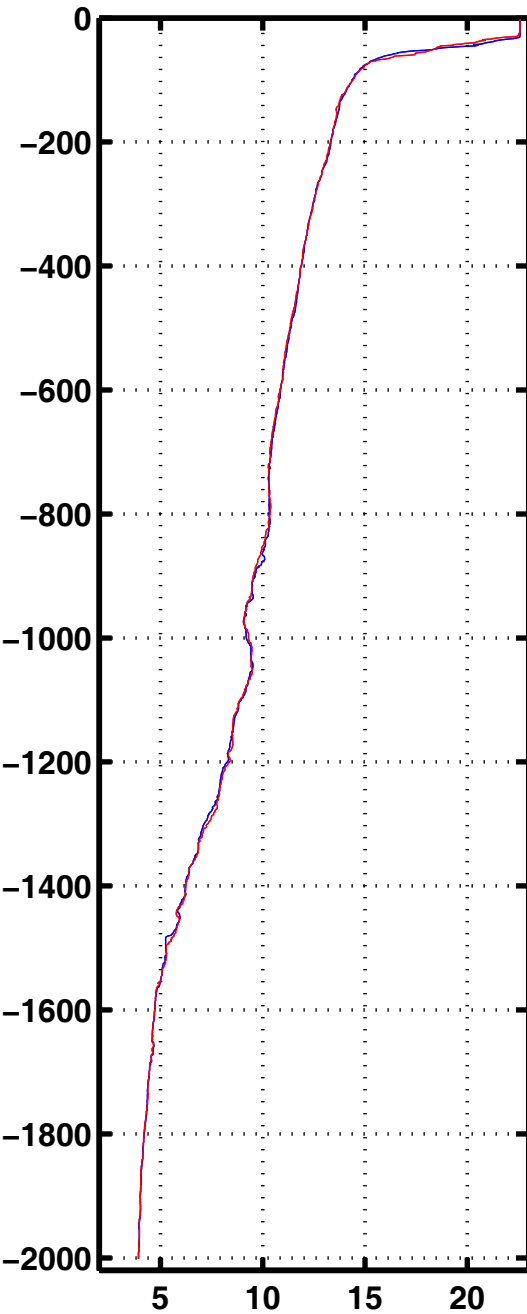
Tempe 3035
