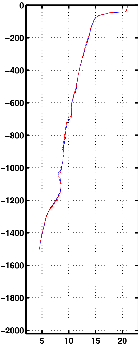
Tempe 3167
