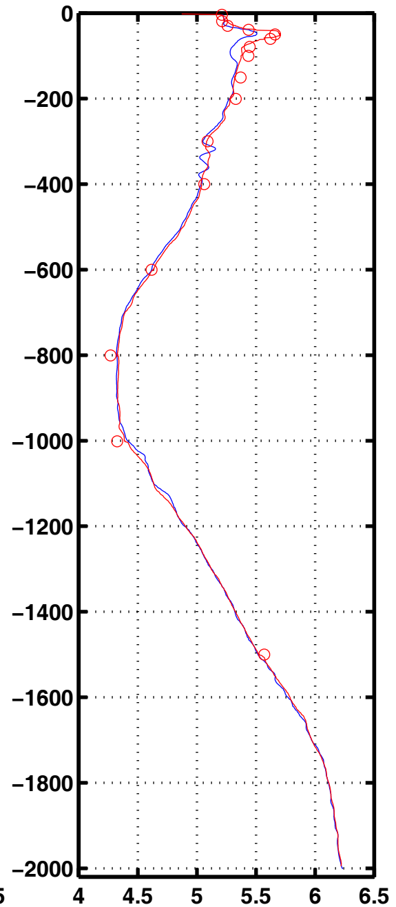
Oxyg 3001
