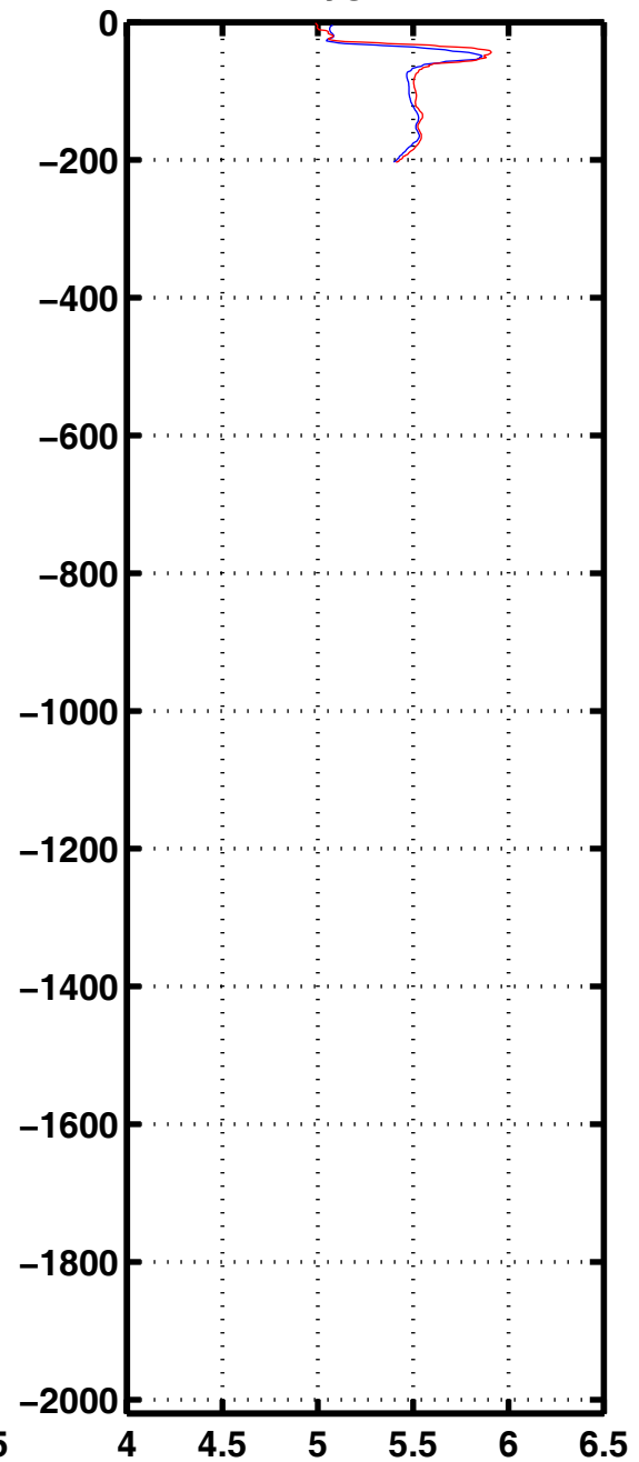
Oxyg 3249
