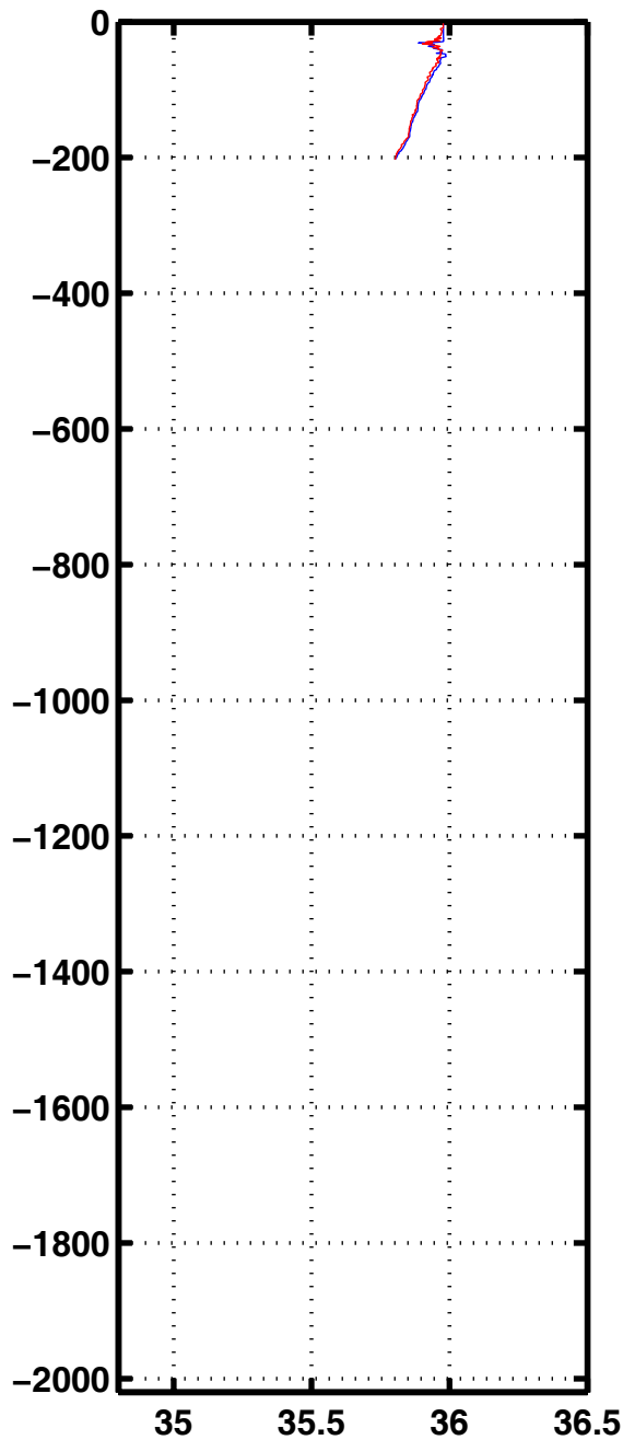
Sali 3156
