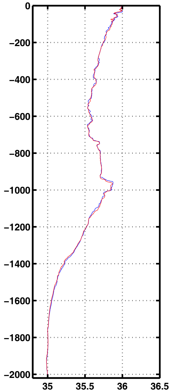
Sali 3010
