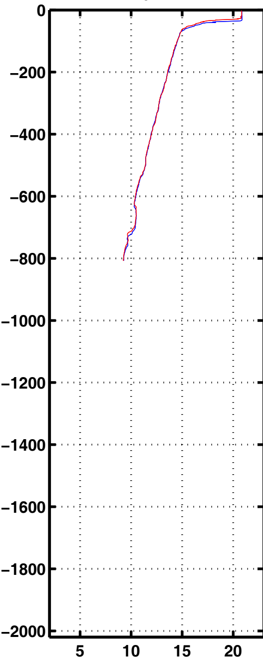
Tempe 3164
