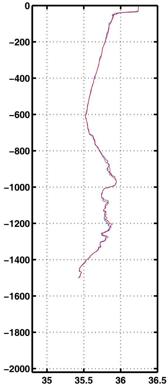
Sali 3087
