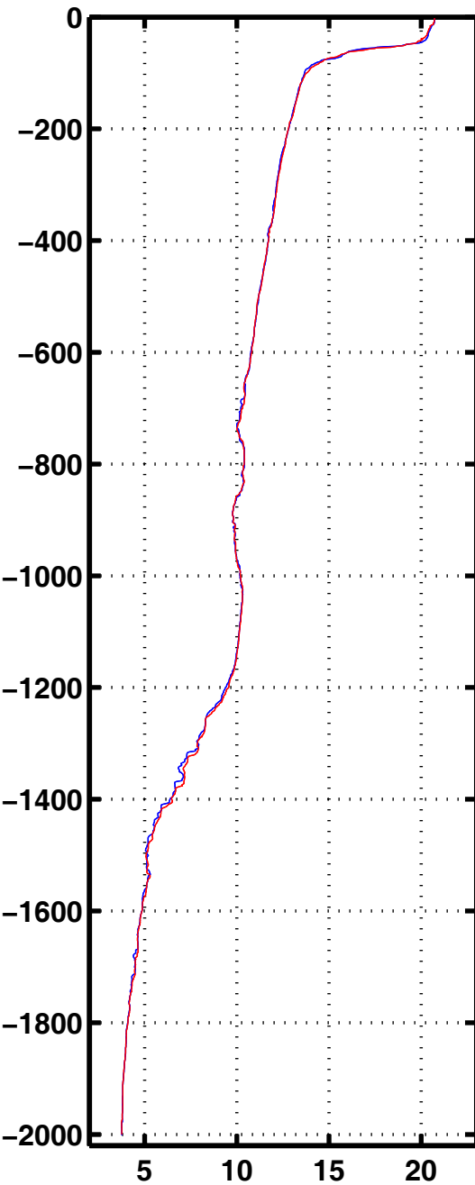
Tempe 3024
