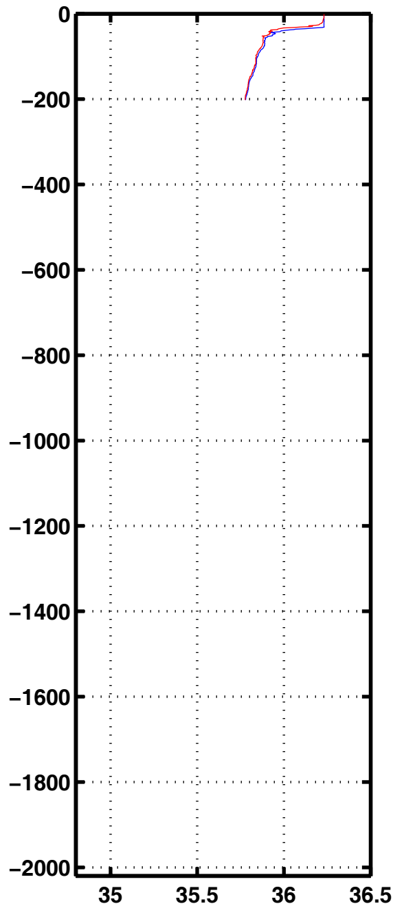
Sali 3086
