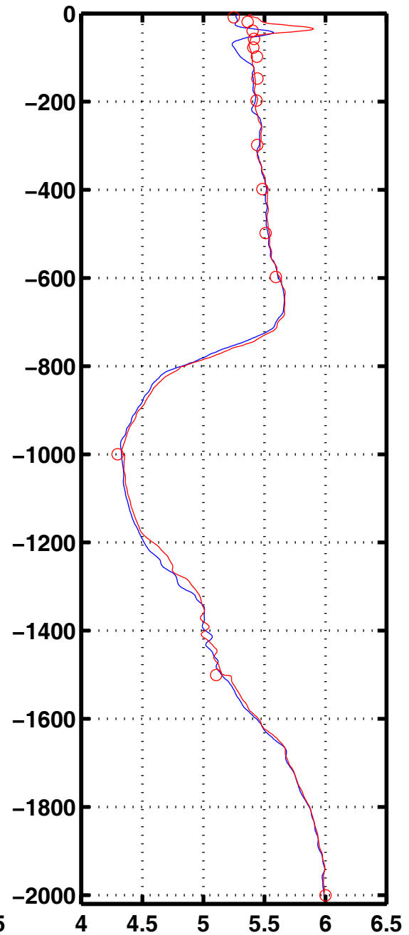
Oxyg 3026
