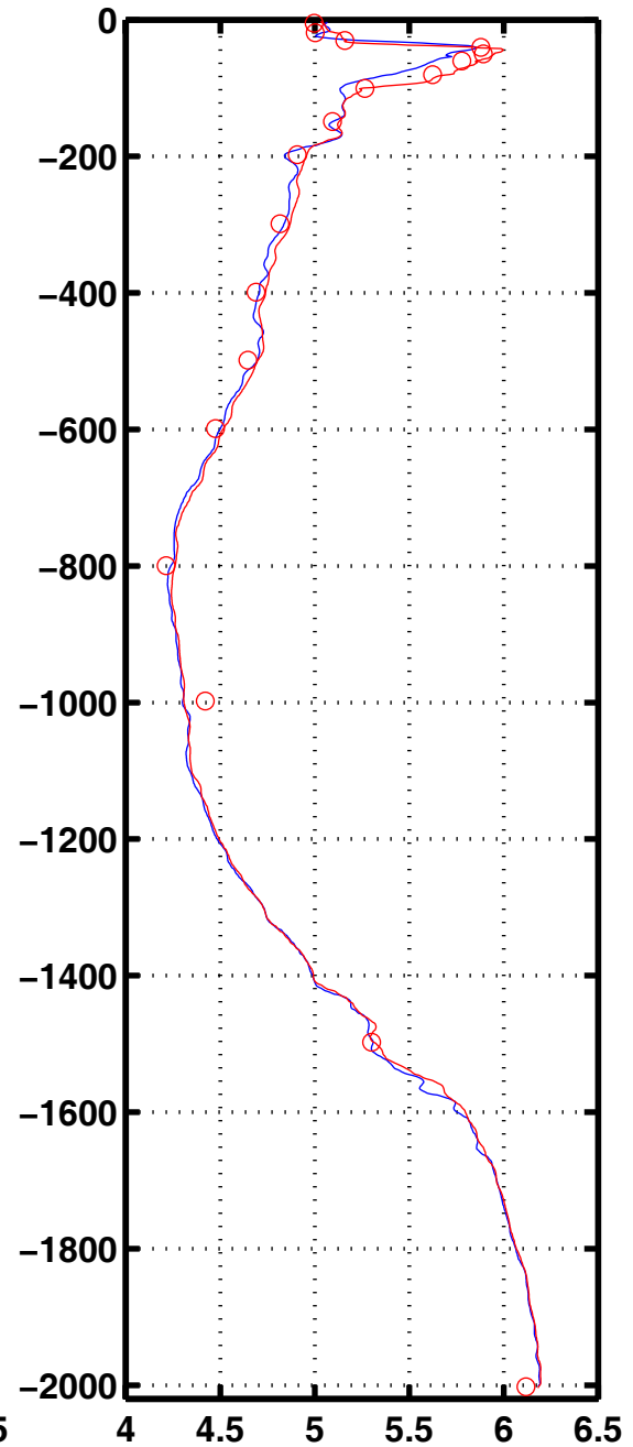
Oxyg 3043
