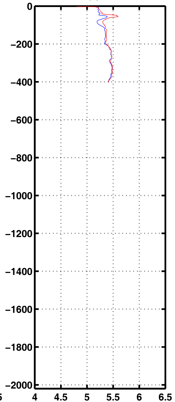
Oxyg 3329
