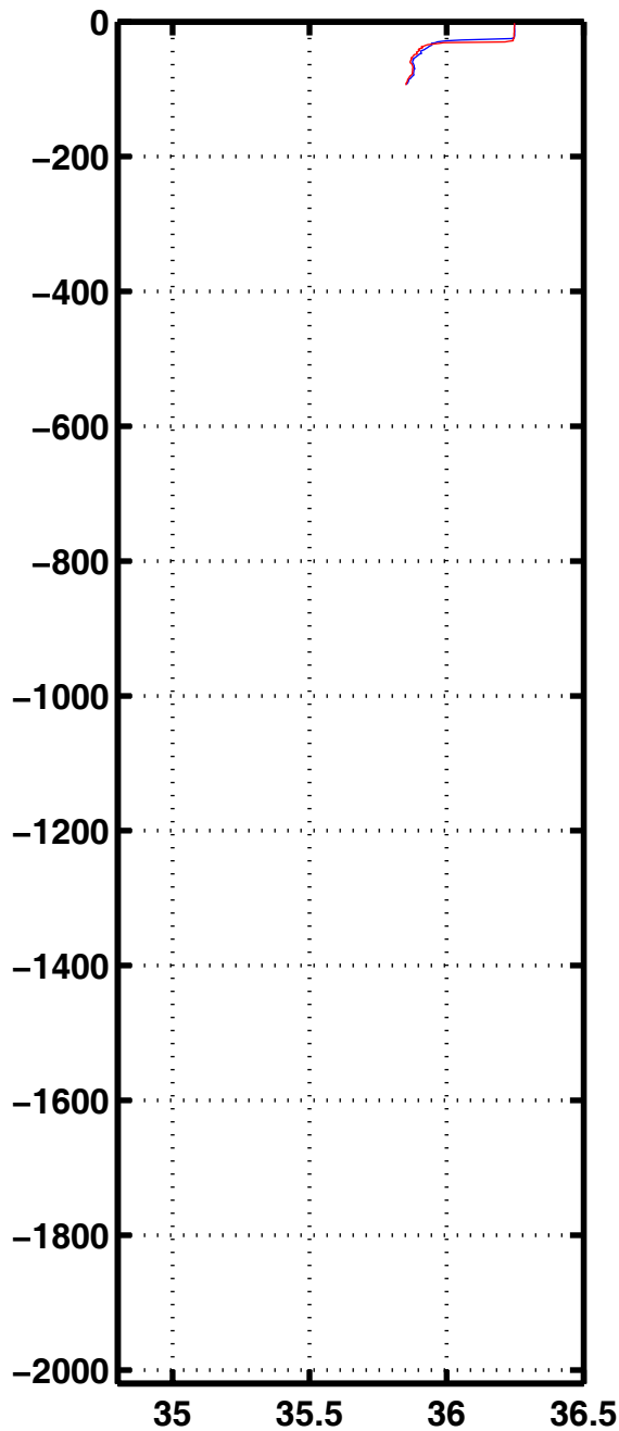
Sali 3090
