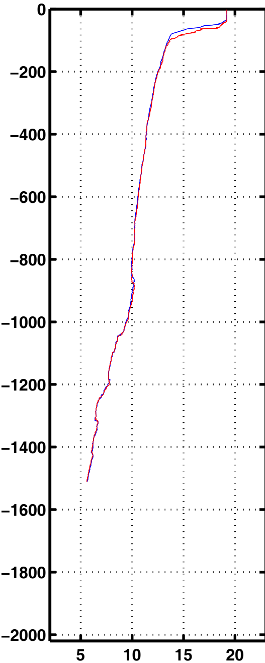
Tempe 3327
