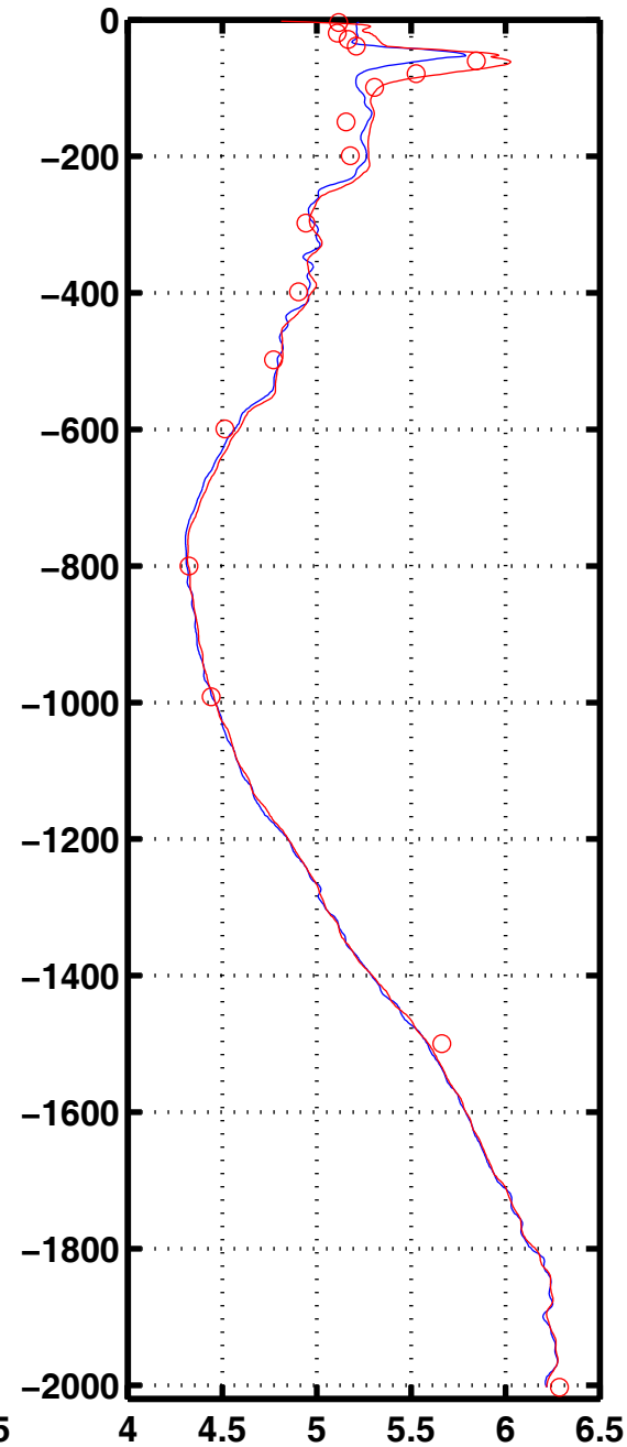
Oxyg 3060
