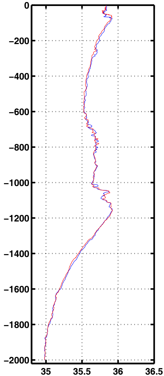
Sali 3008
