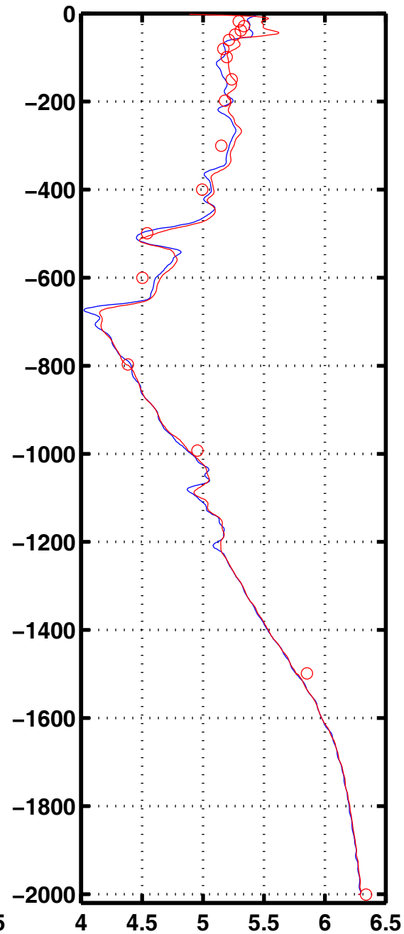
Oxyg 3068
