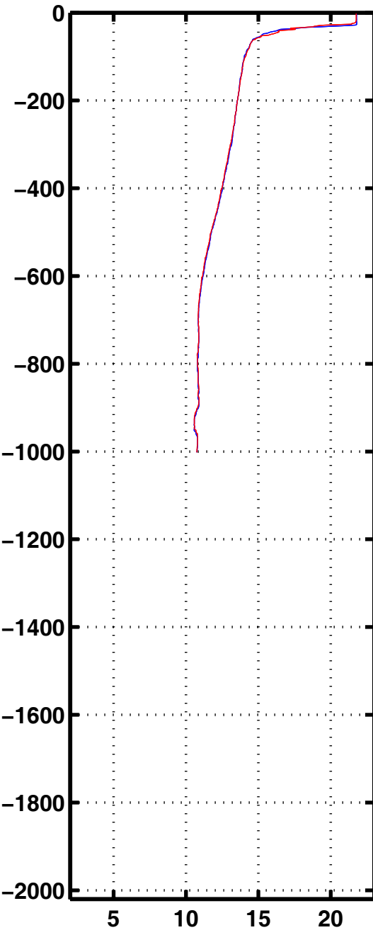
Tempe 3091
