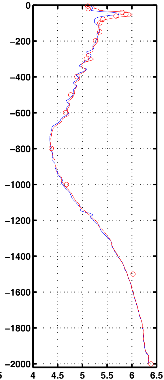
Oxyg 3071
