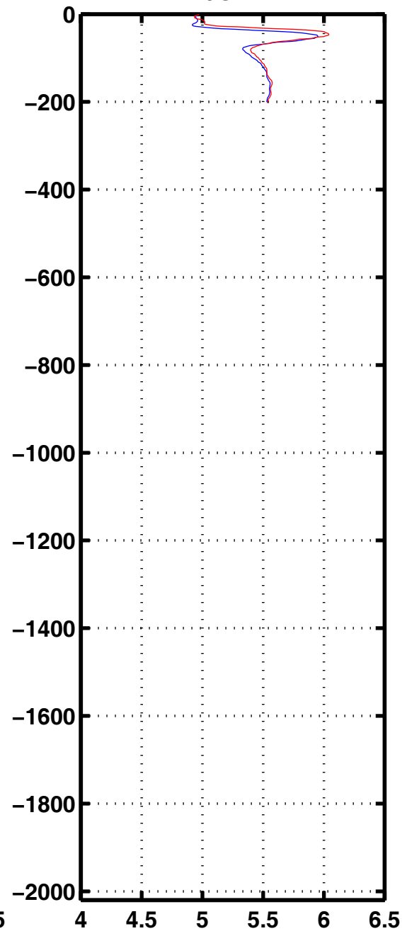
Oxyg 3086
