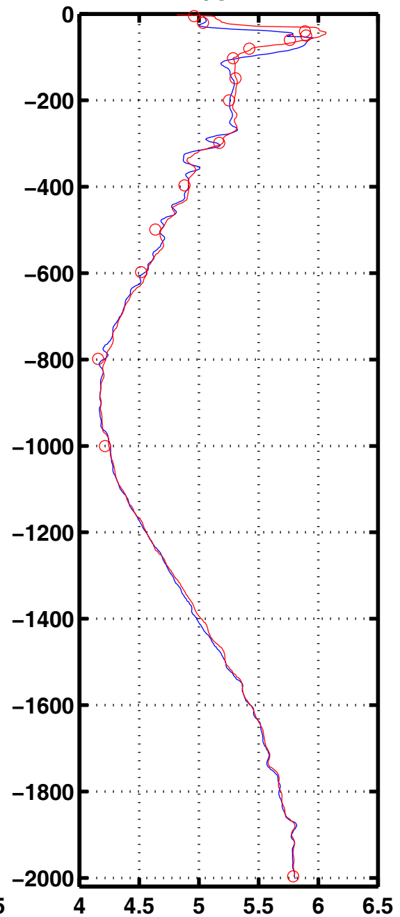
Oxyg 3039
