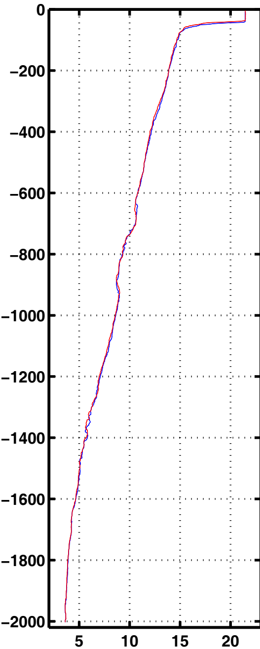
Tempe 3053
