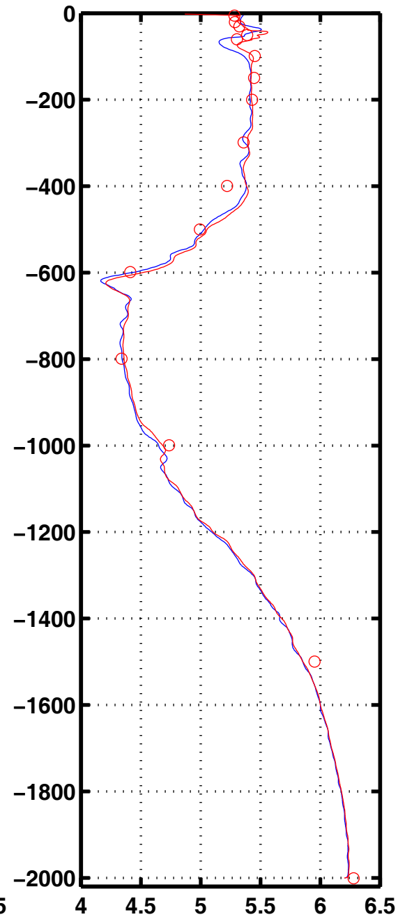
Oxyg 3066
