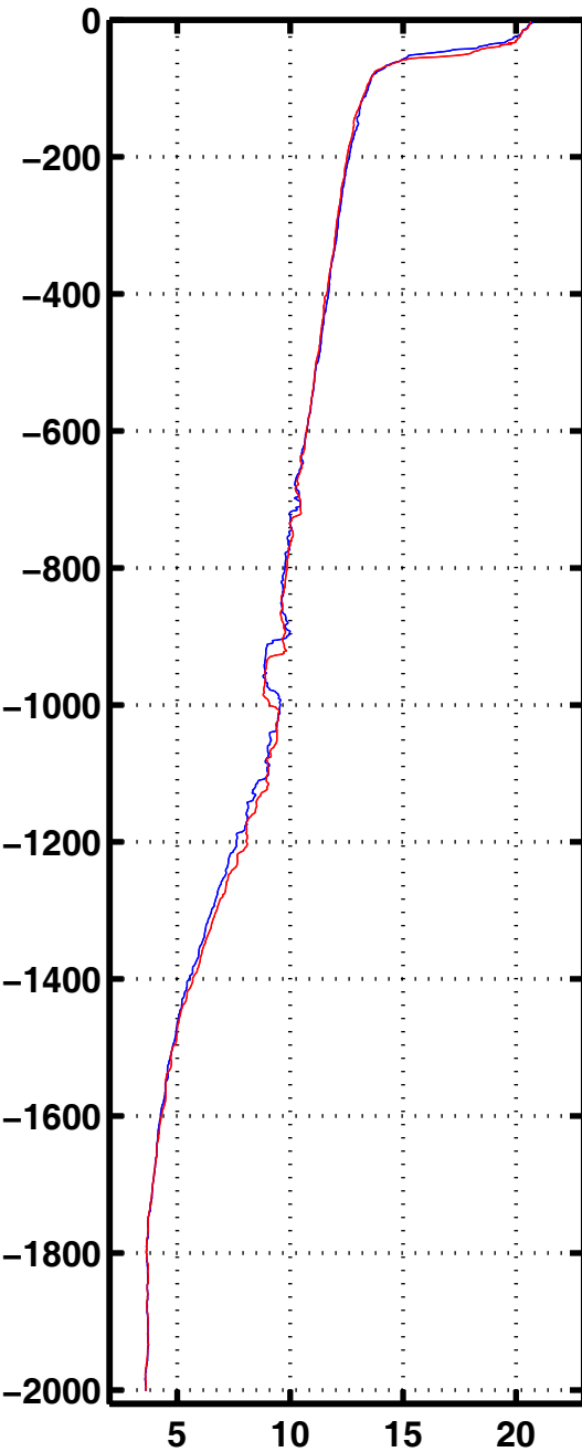
Tempe 3029
