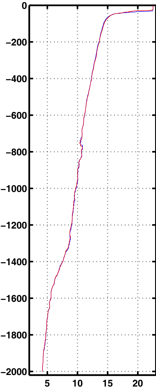
Tempe 3042
