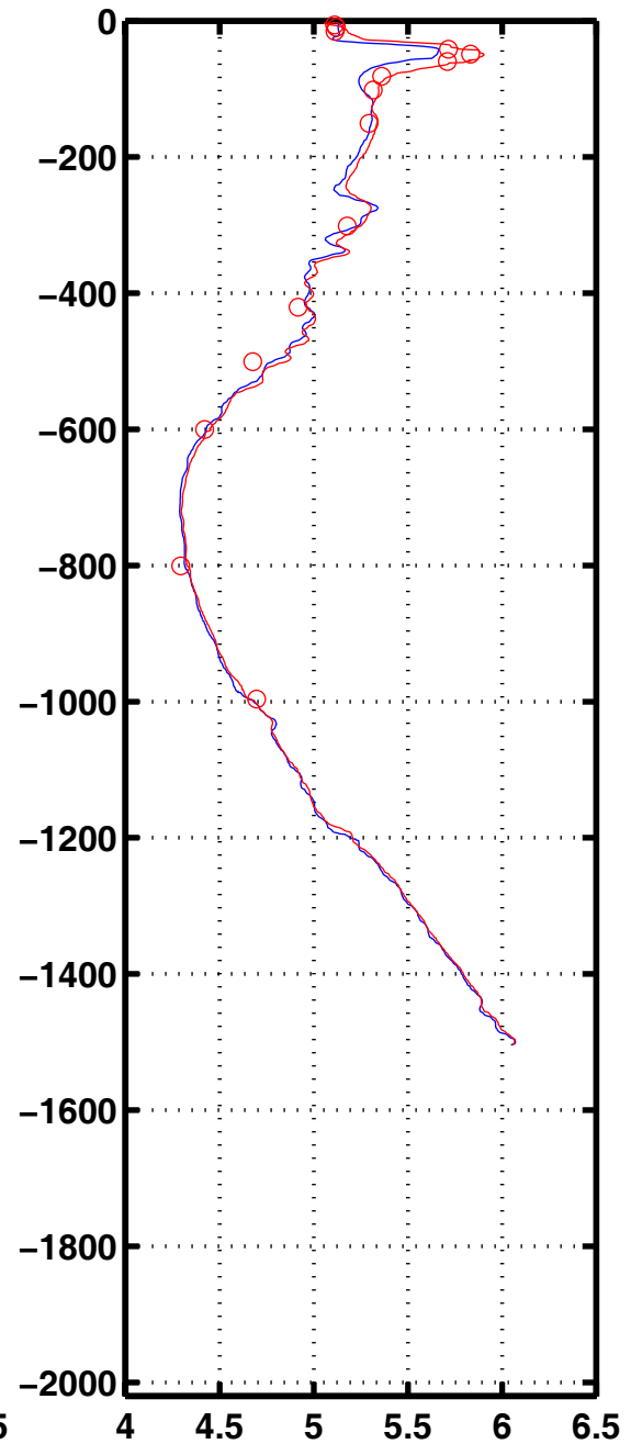
Oxyg 3241
