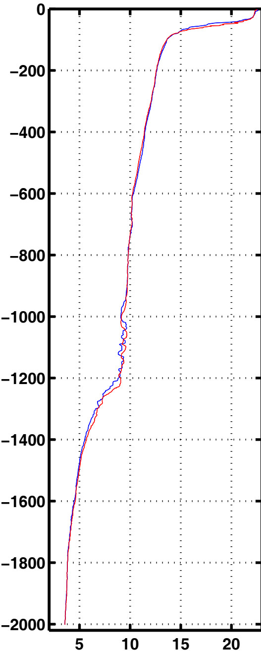
Tempe 3016
