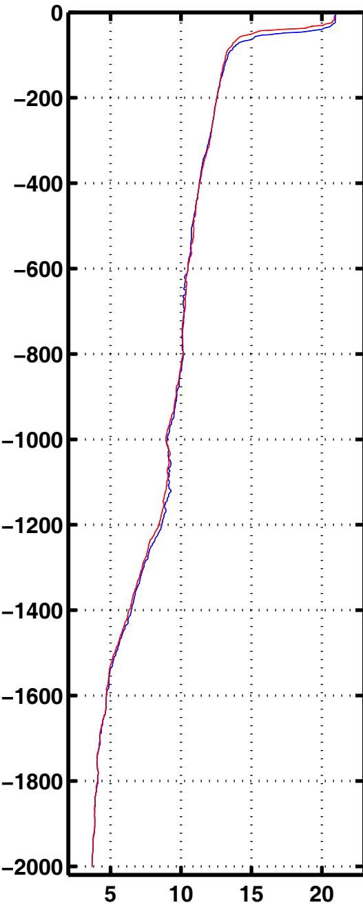
Tempe 3005
