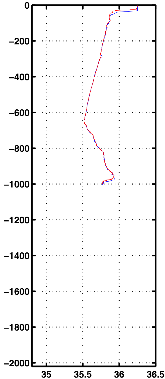
Sali 3088
