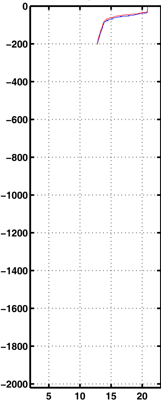
Tempe 3247
