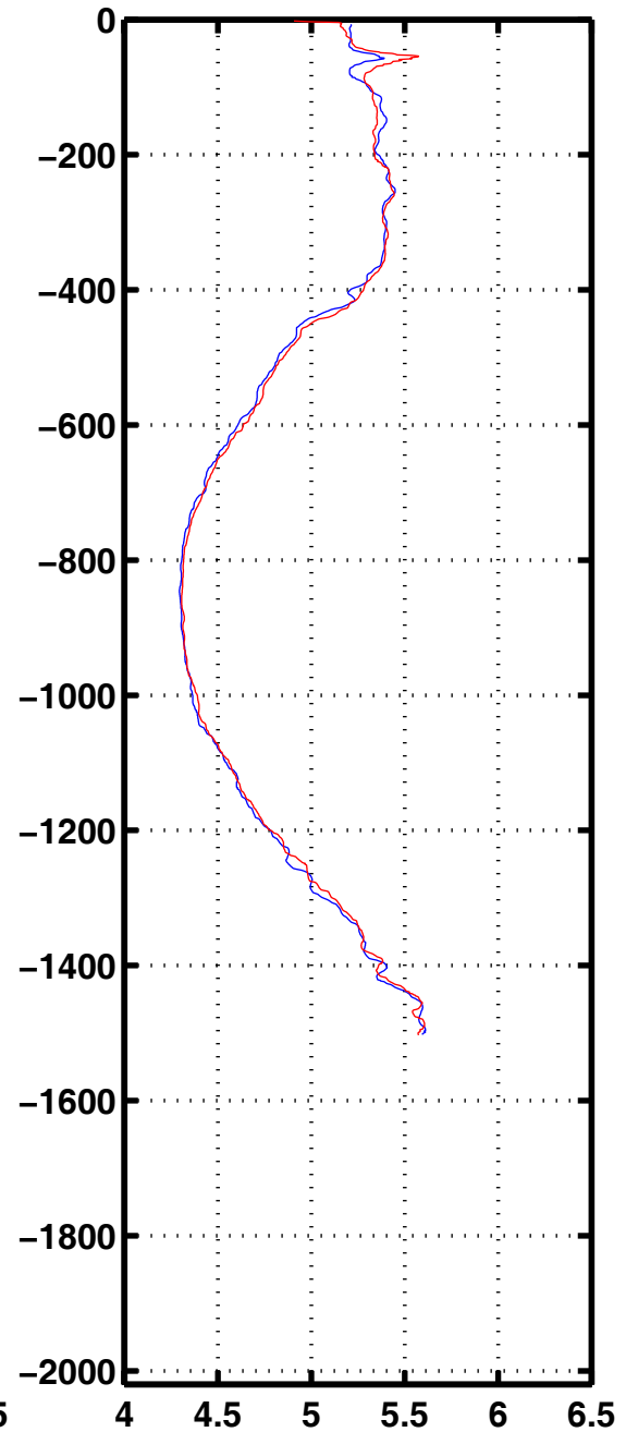
Oxyg 3323
