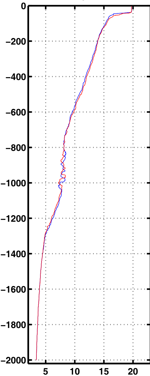
Tempe 3067
