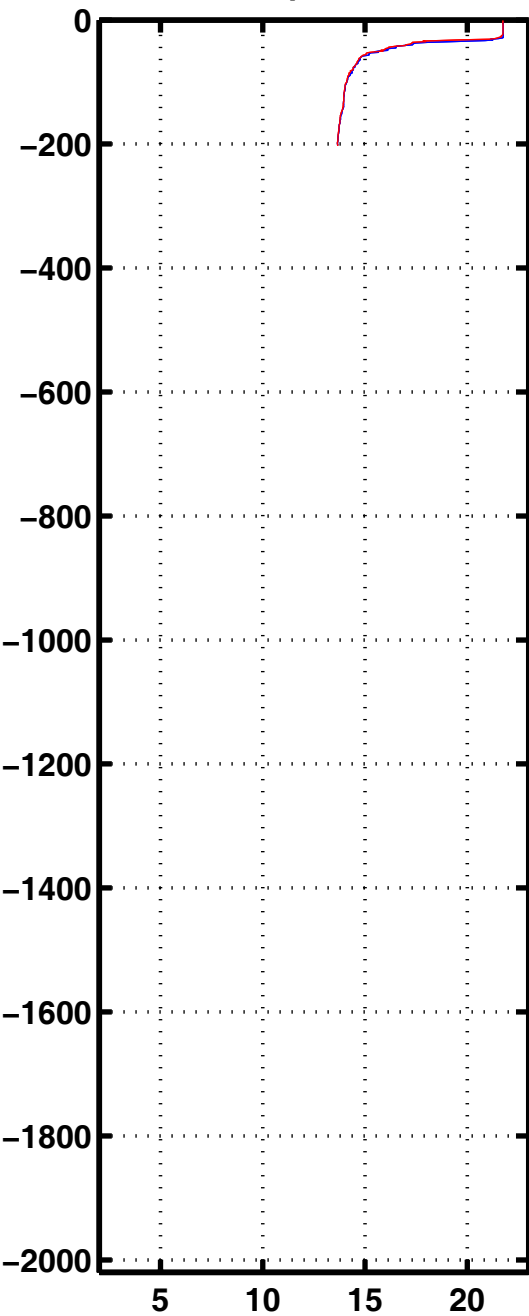
Tempe 3094
