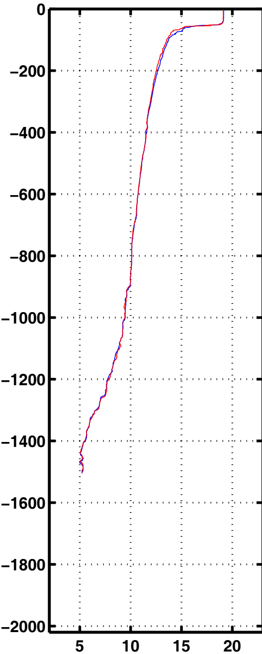
Tempe 3325
