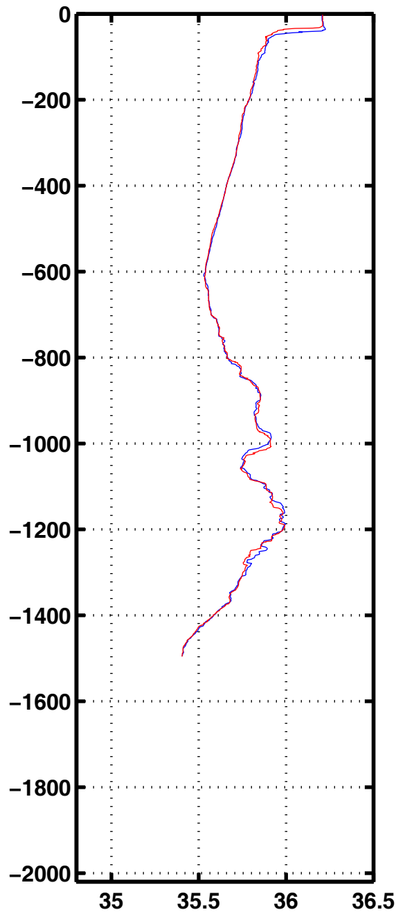
Sali 3097
