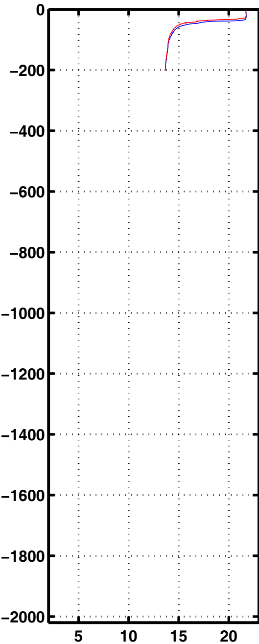
Tempe 3096
