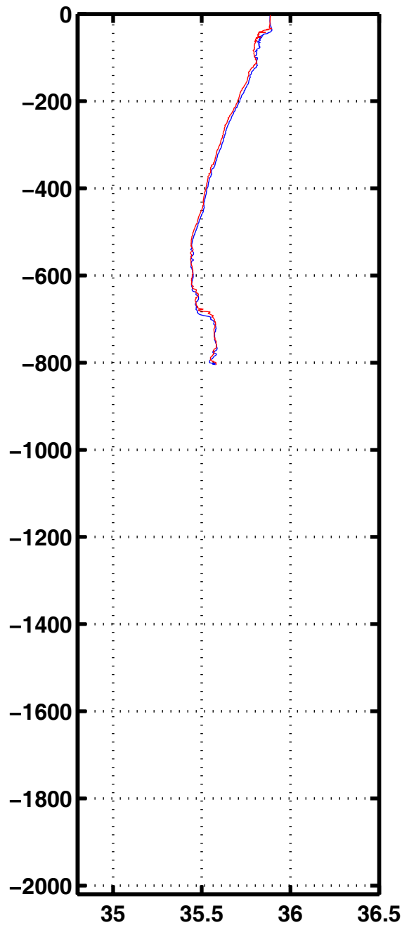
Sali 3248
