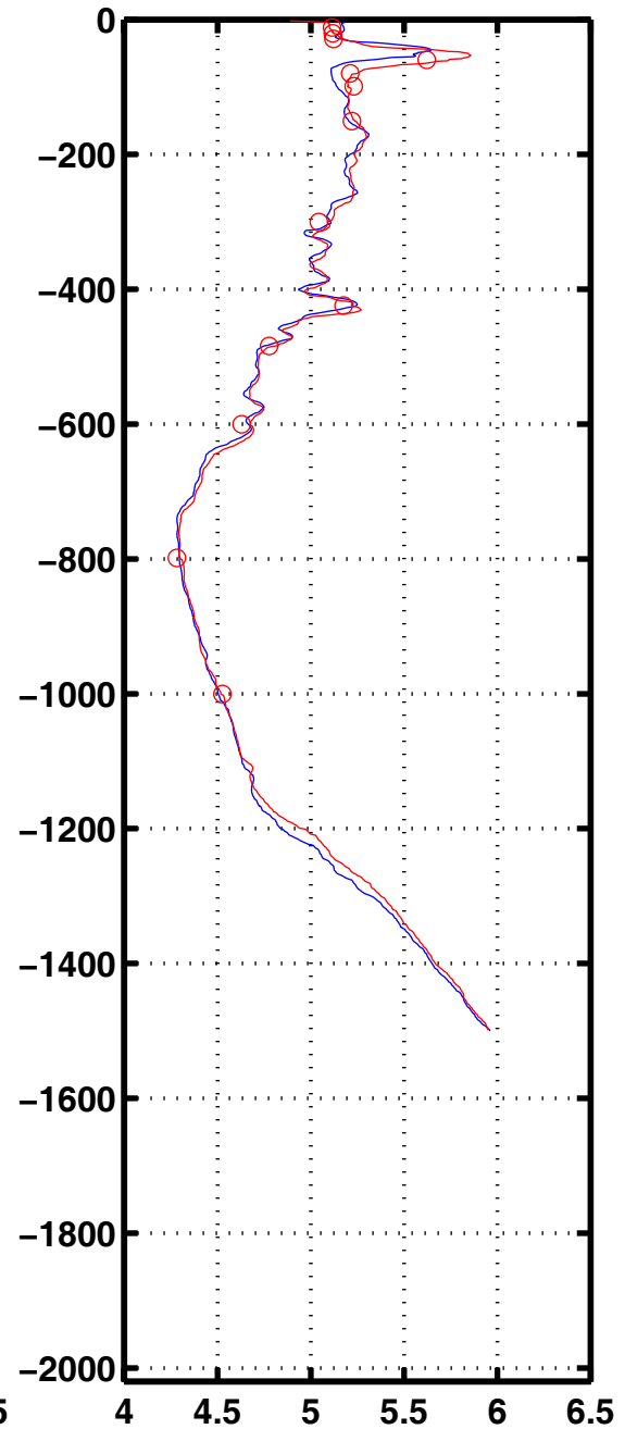
Oxyg 3166
