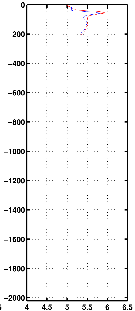
Oxyg 3240
