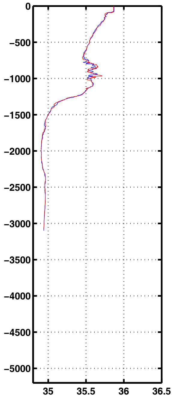
Sali 3339
