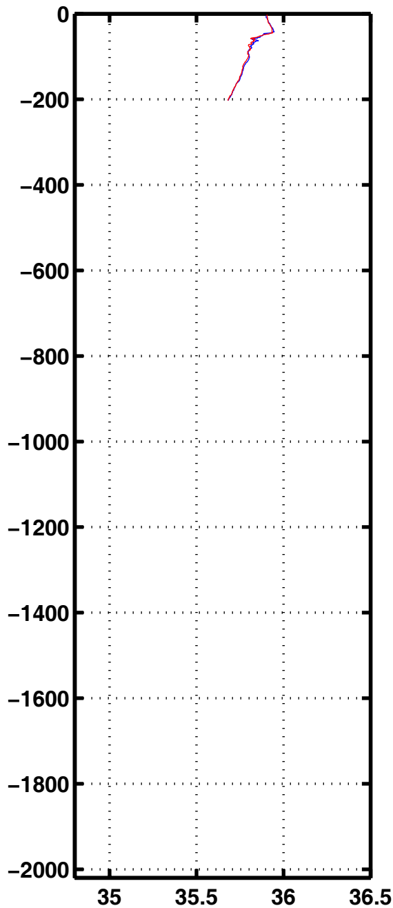
Sali 3238
