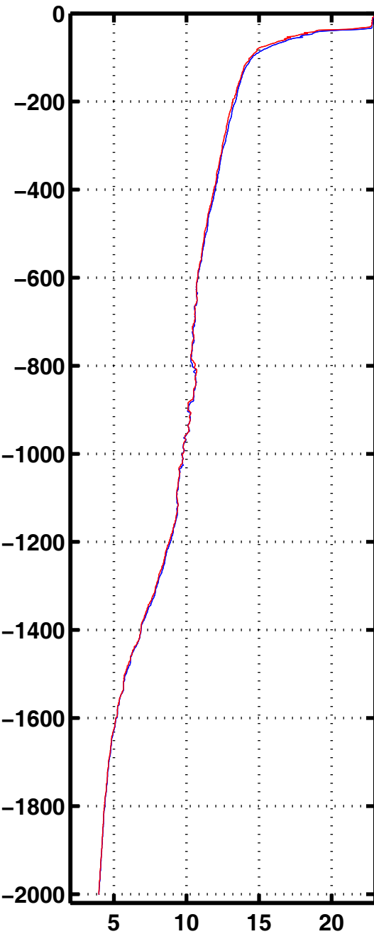
Tempe 3082
