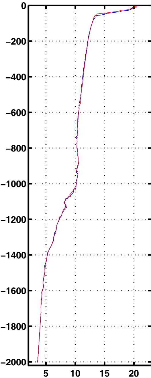
Tempe 3021
