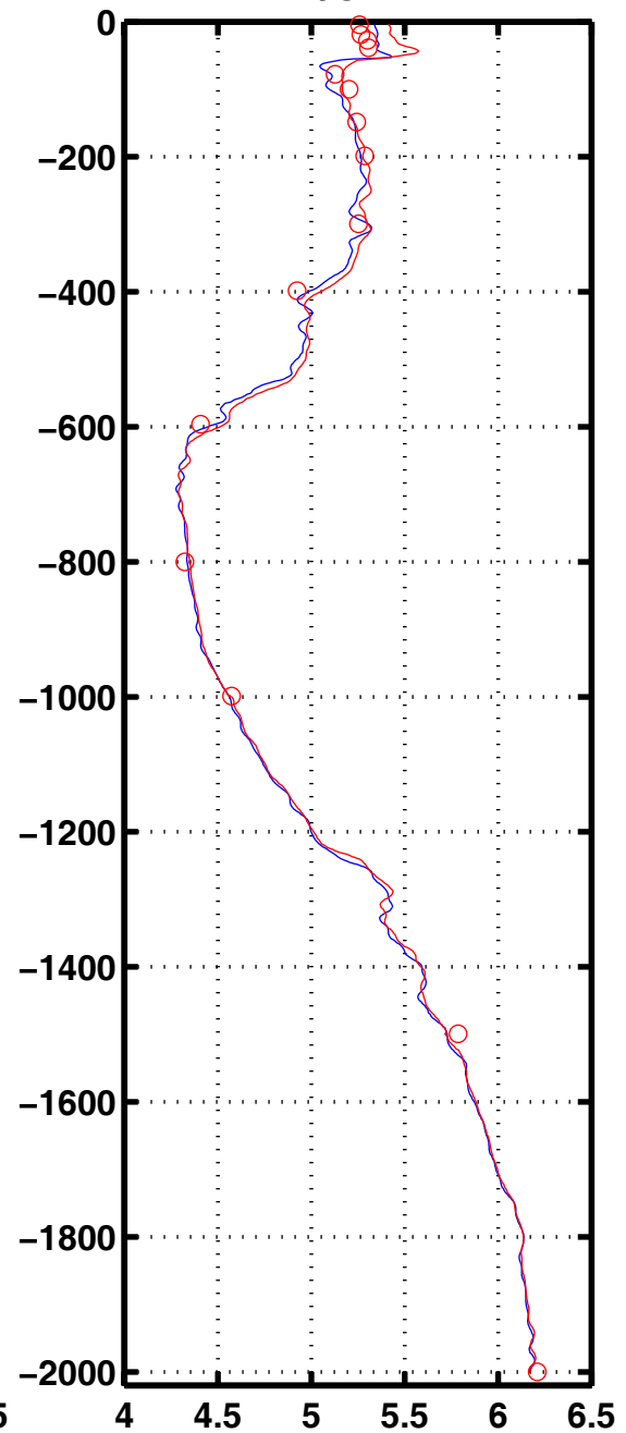
Oxyg 3070
