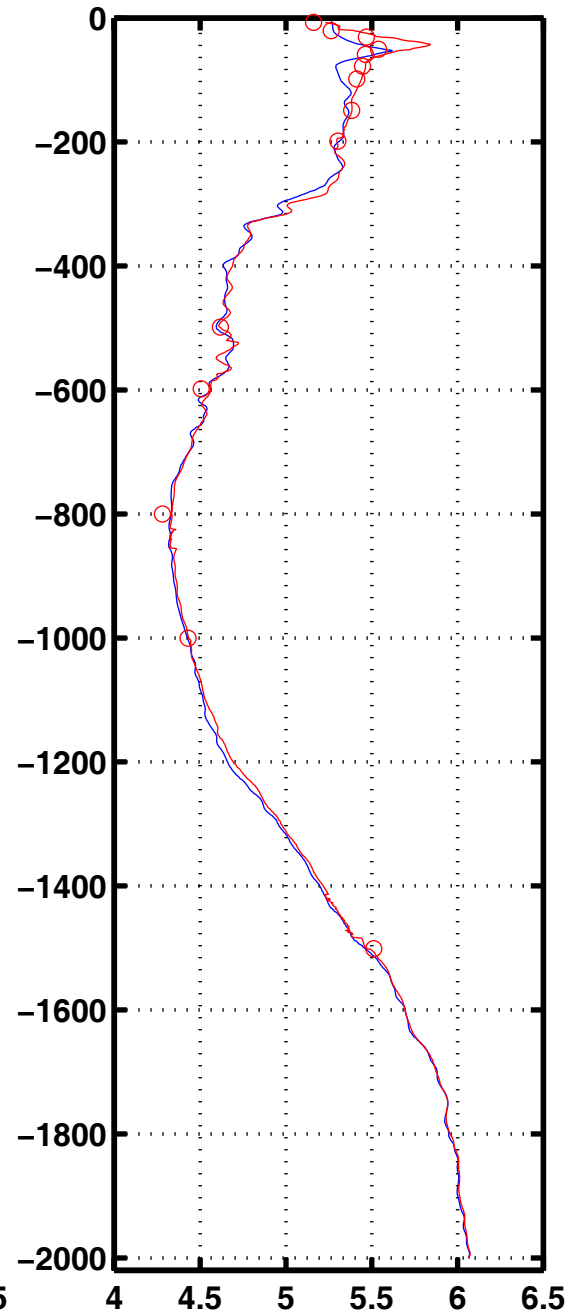
Oxyg 3005
