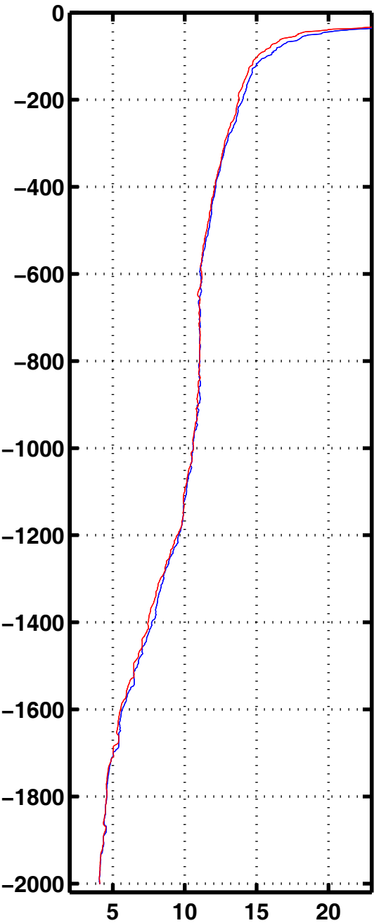
Tempe 3014
