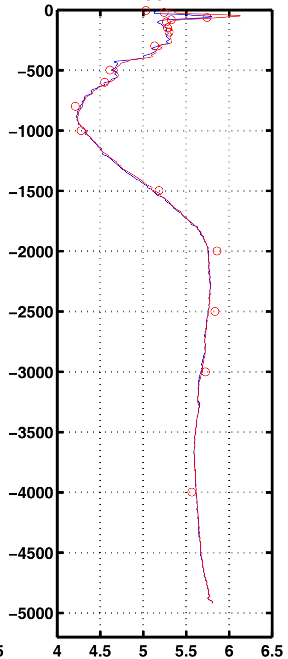
Oxyg 3036
