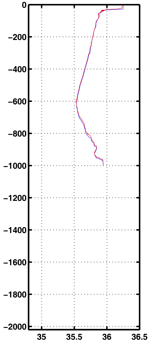
Sali 3091
