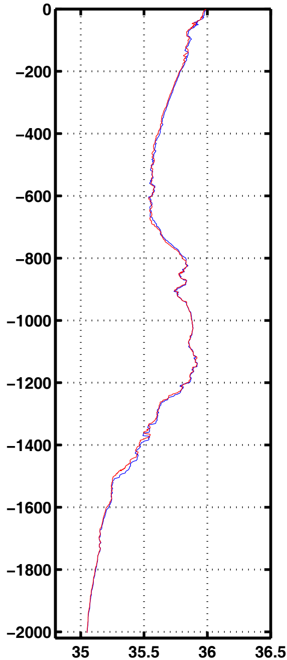
Sali 3018
