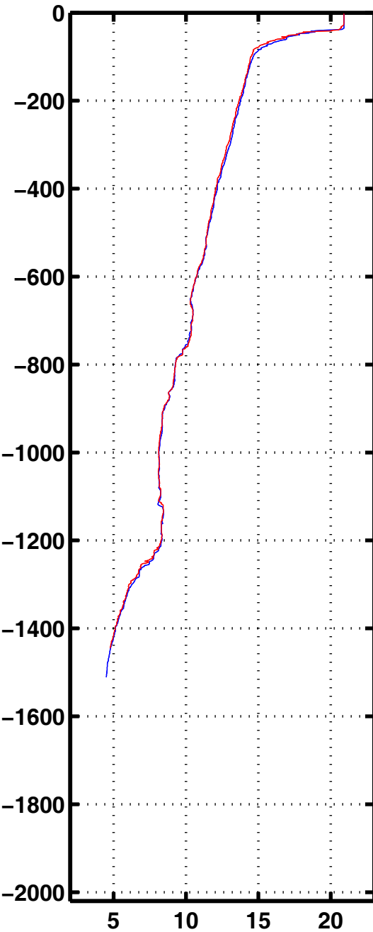
Tempe 3157
