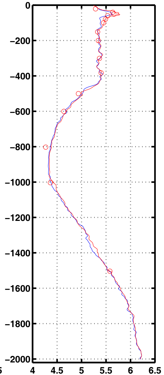
Oxyg 3003
