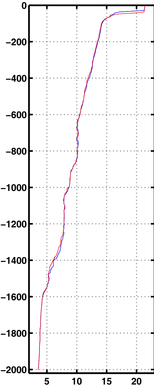
Tempe 3058
