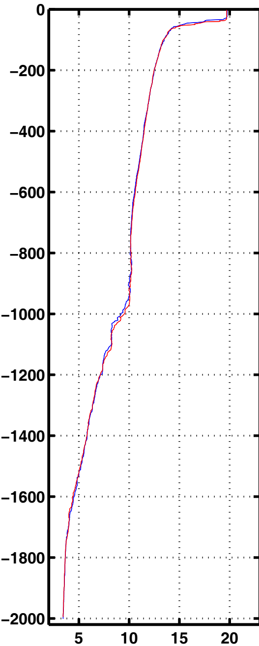
Tempe 3001
