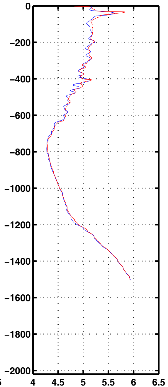
Oxyg 3159
