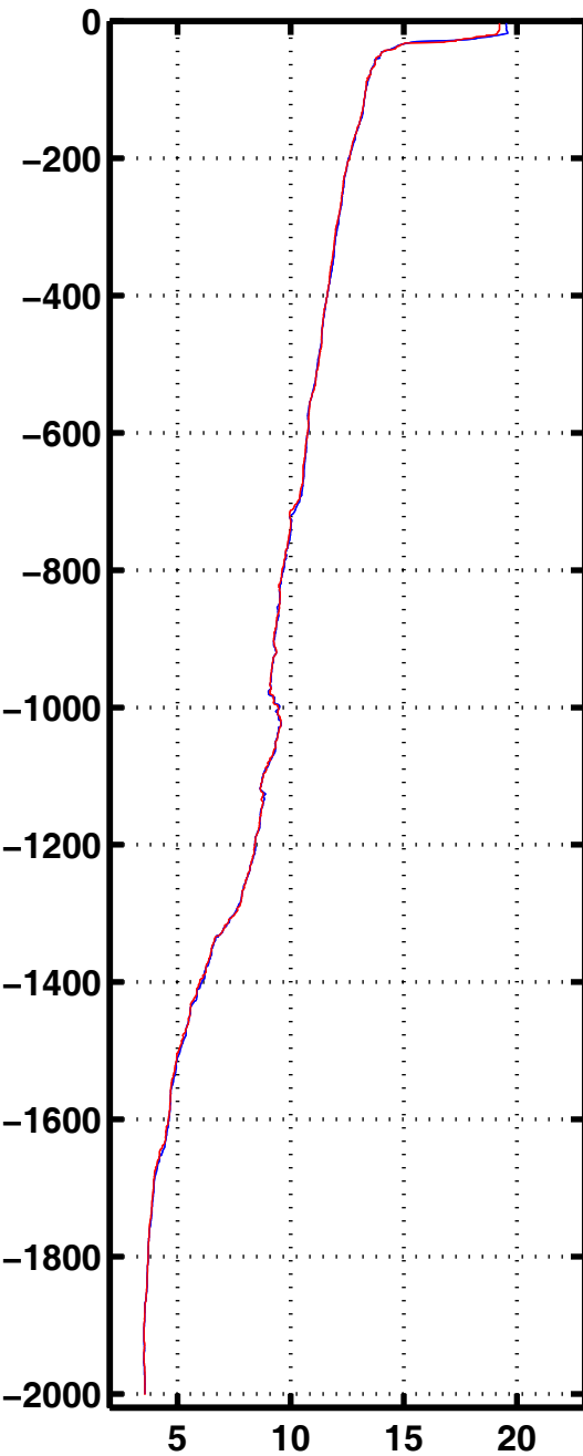
Tempe 3002
