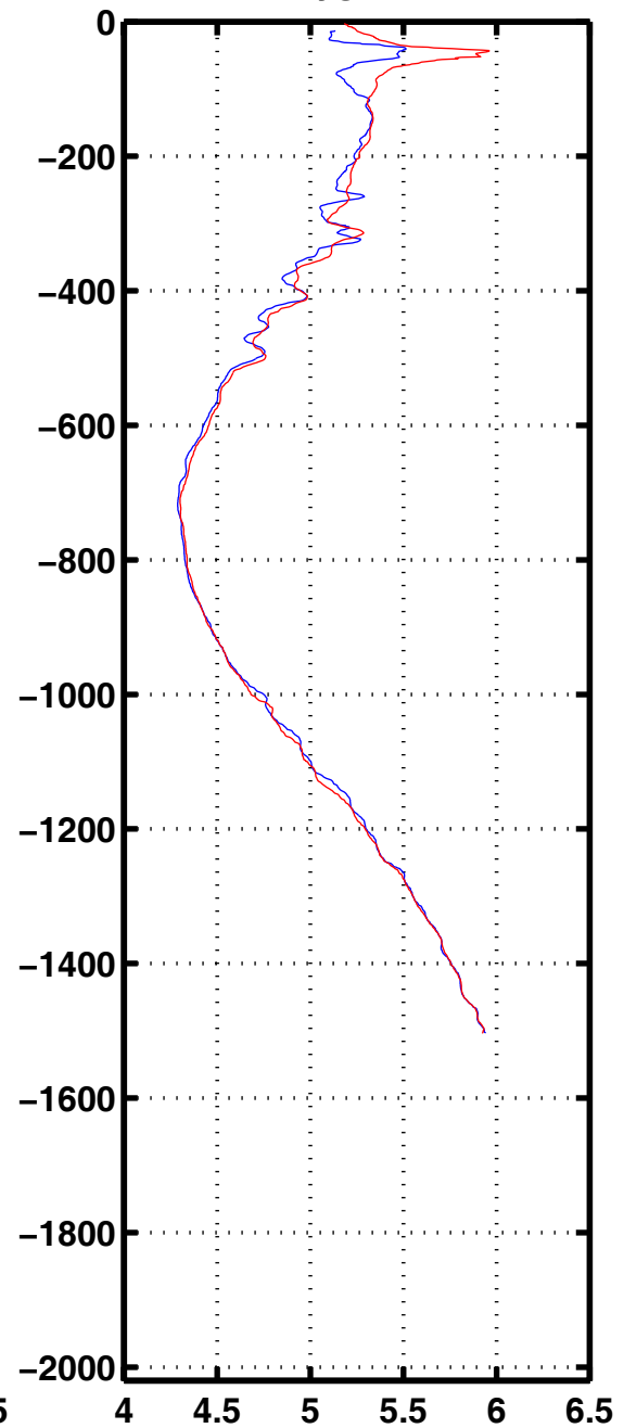
Oxyg 3239
