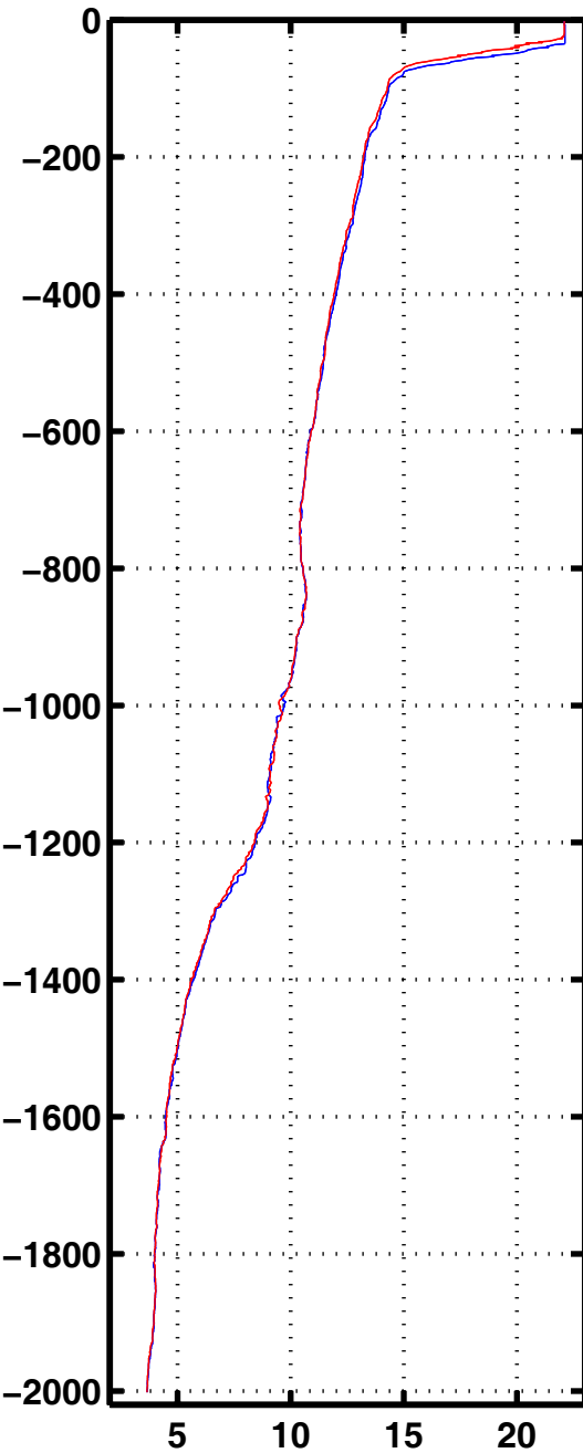
Tempe 3033
