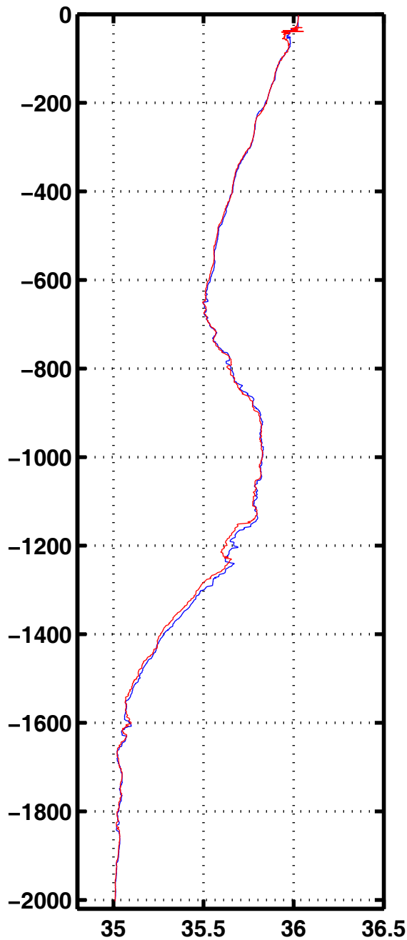
Sali 3046
