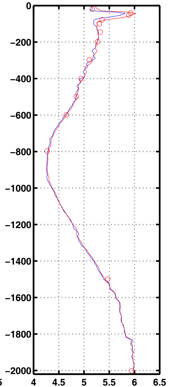
Oxyg 3047
