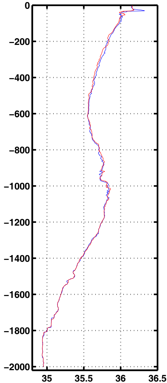
Sali 3079
