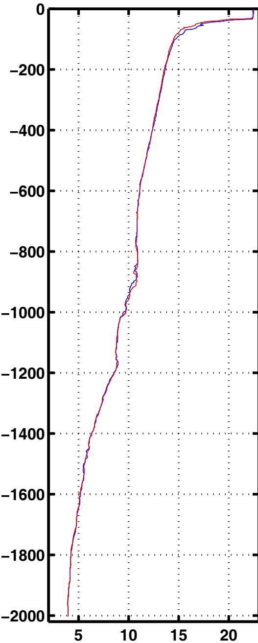
Tempe 3040
