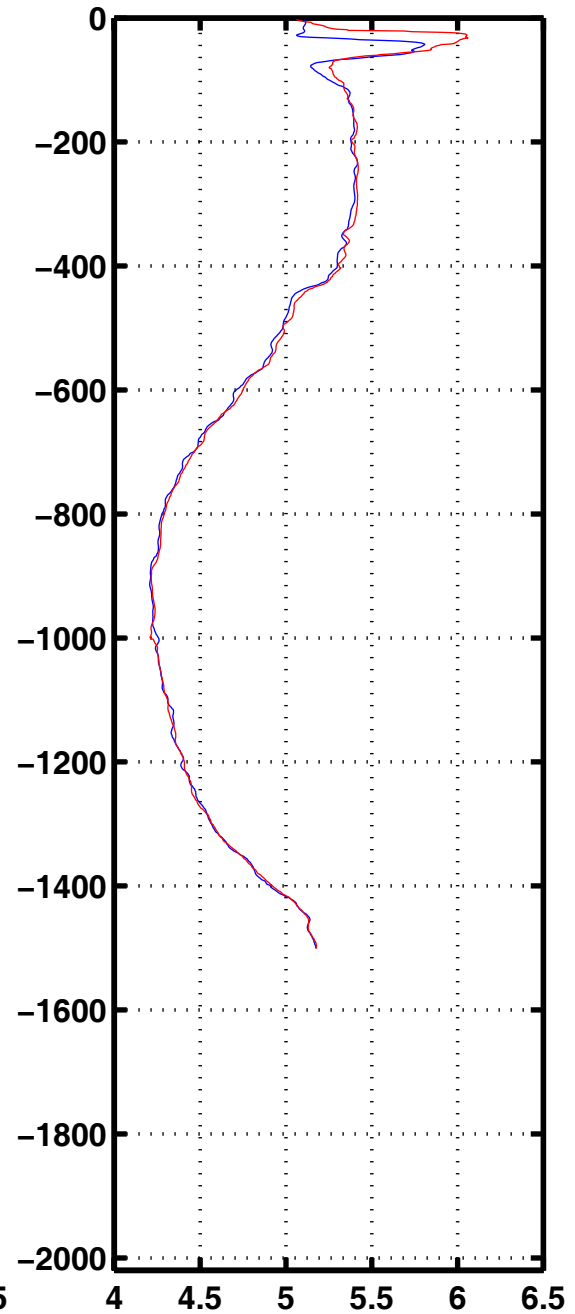
Oxyg 3089
