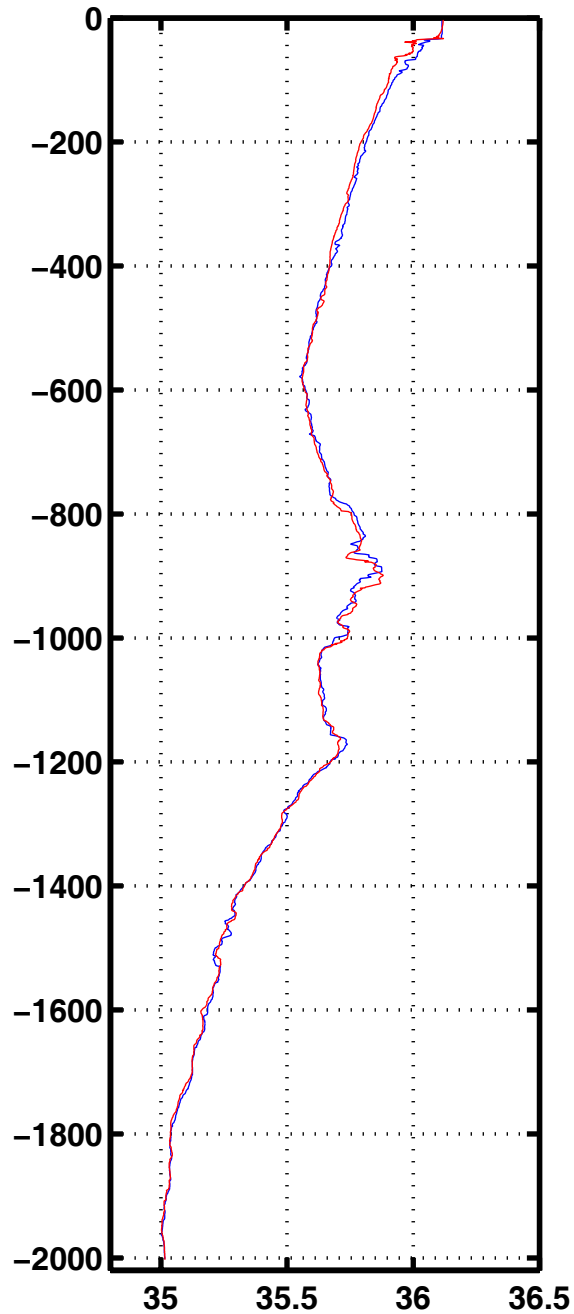
Sali 3040
