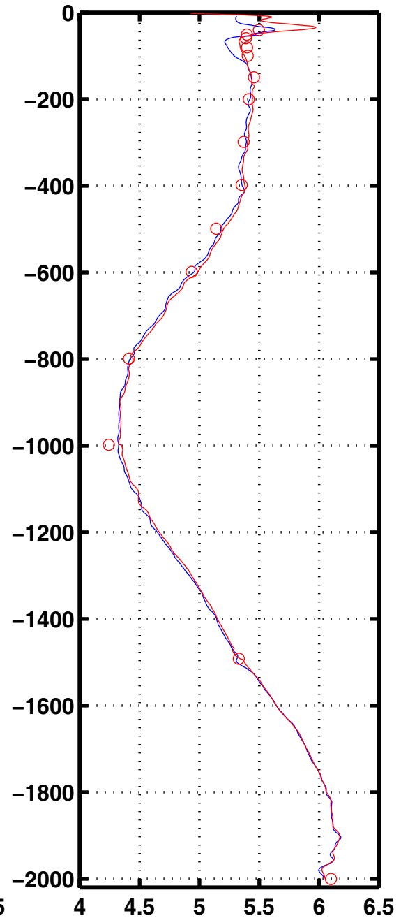
Oxyg 3027
