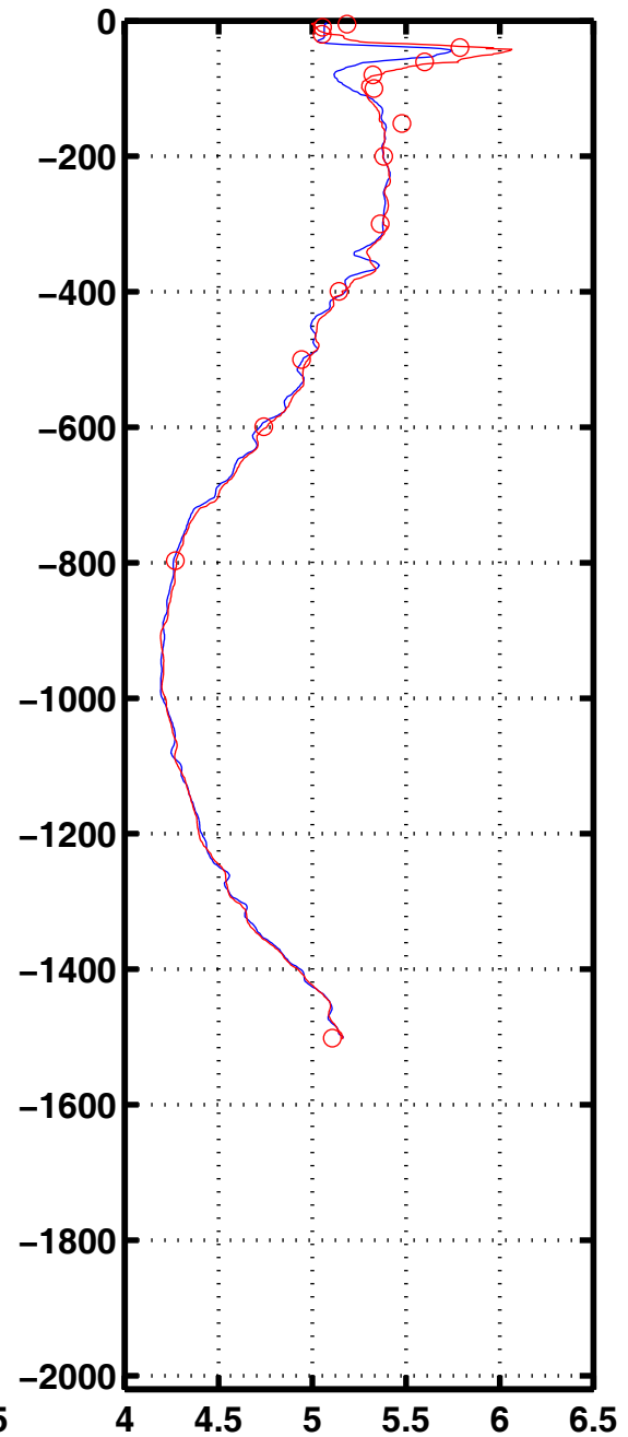
Oxyg 3087
