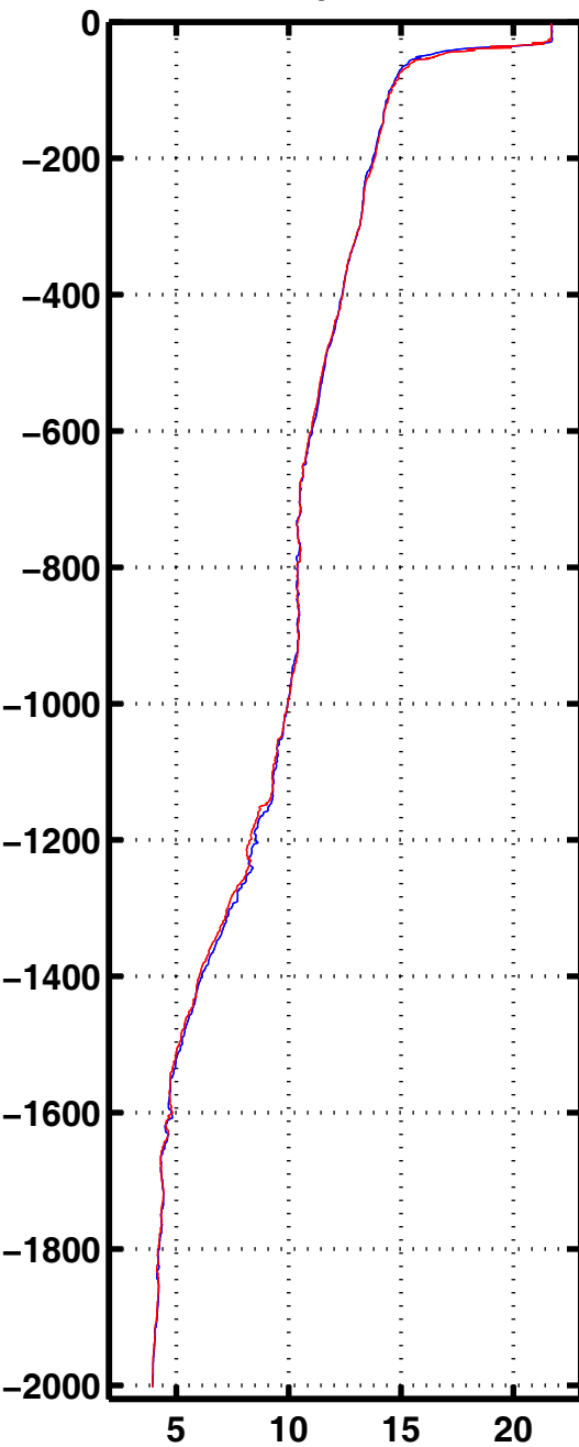
Tempe 3046
