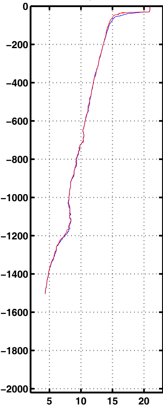
Tempe 3159
