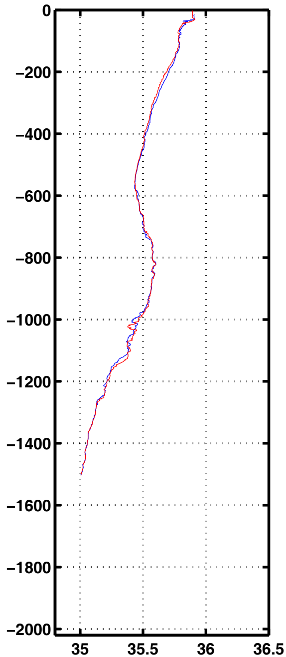
Sali 3239
