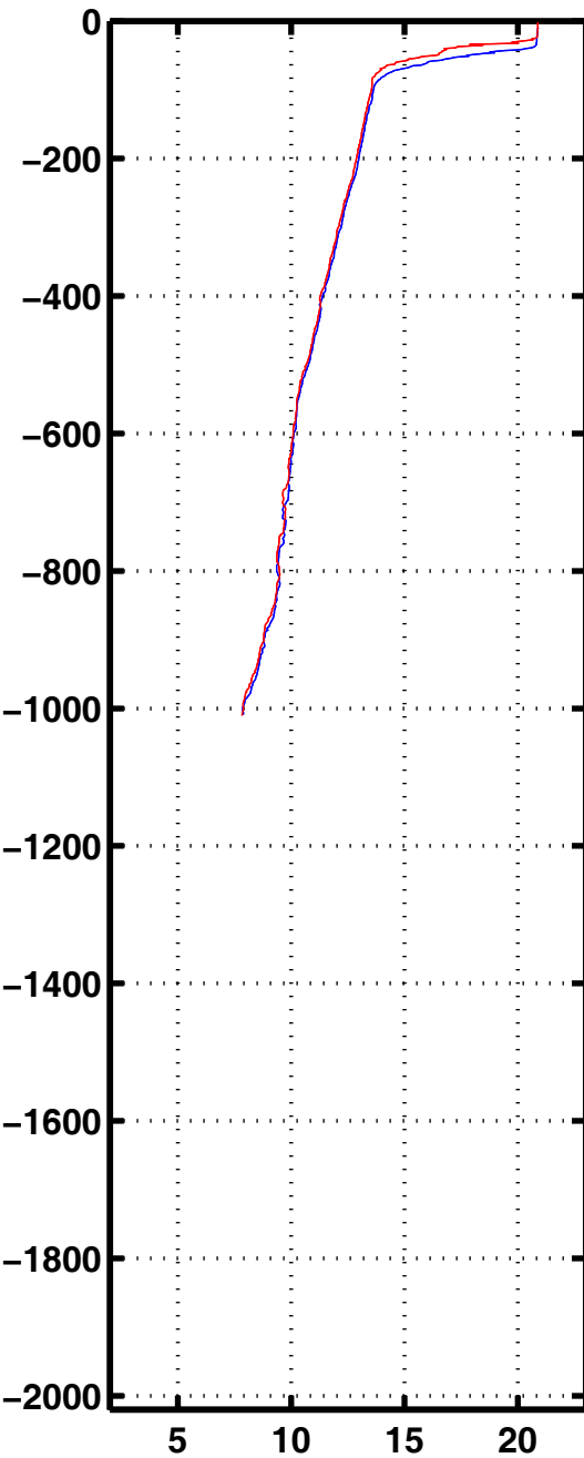
Tempe 3242
