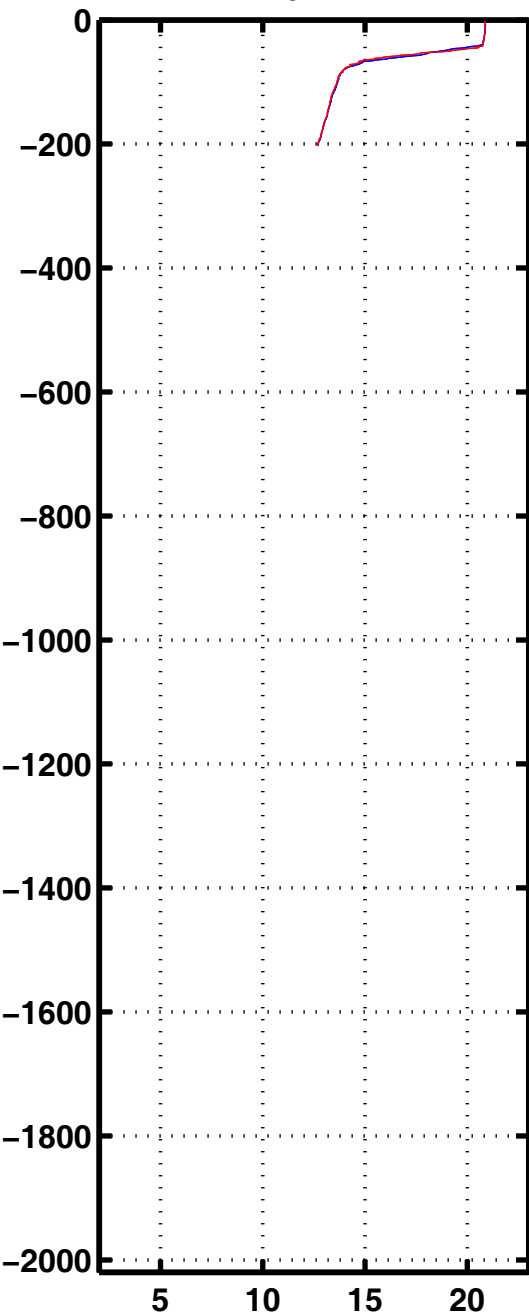
Tempe 3238
