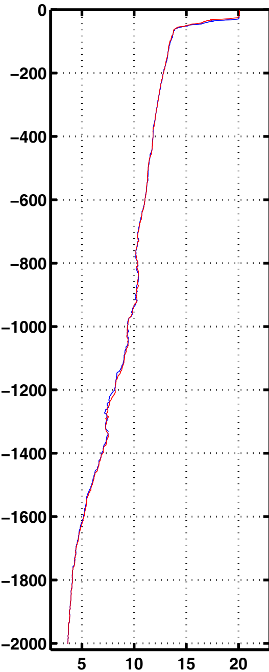
Tempe 3050
