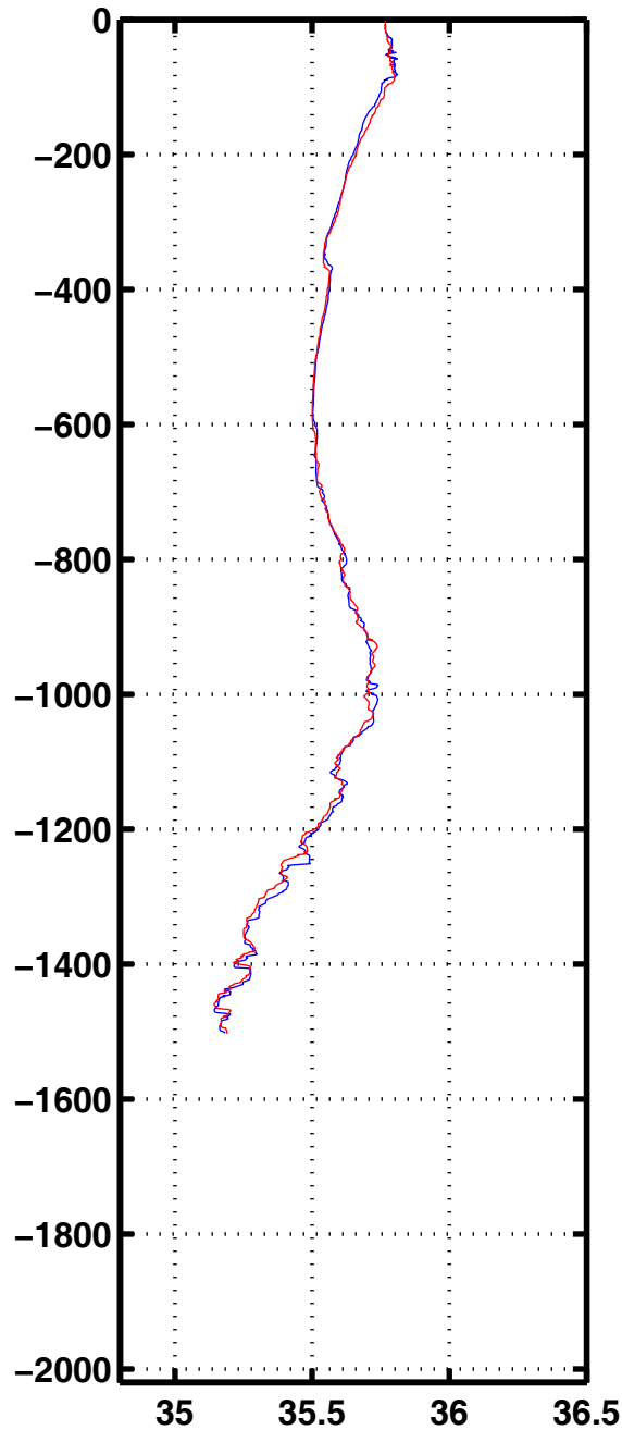
Sali 3323
