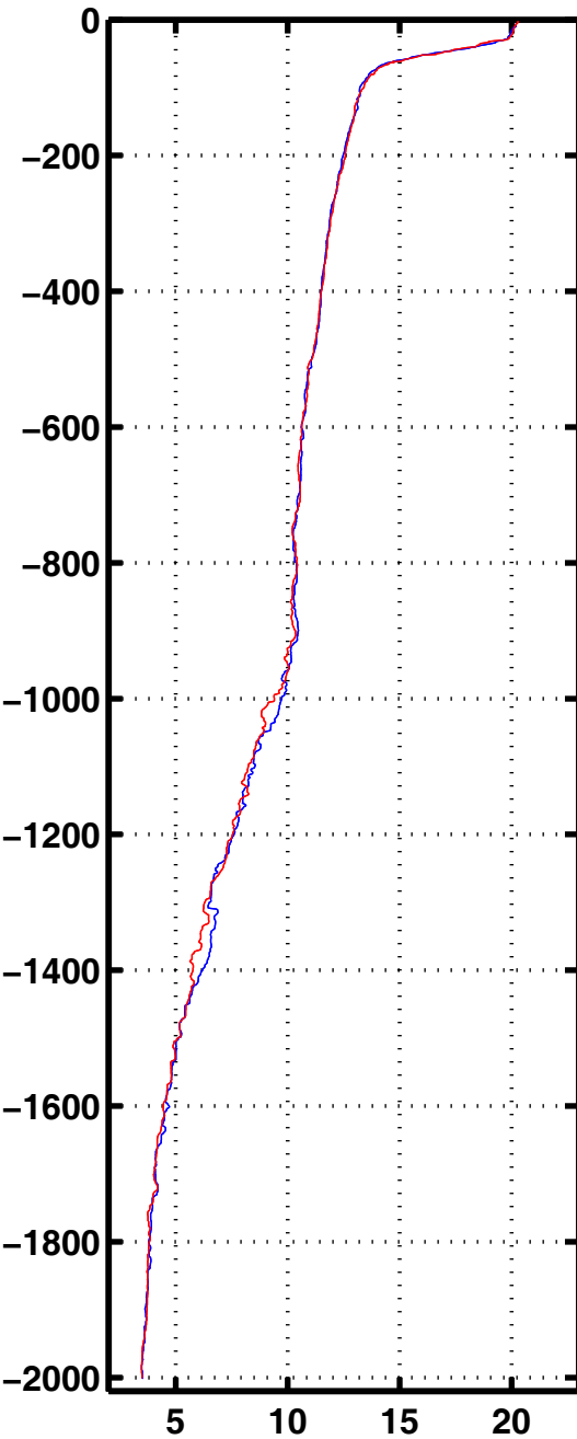
Tempe 3003
