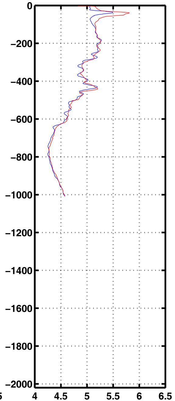
Oxyg 3160
