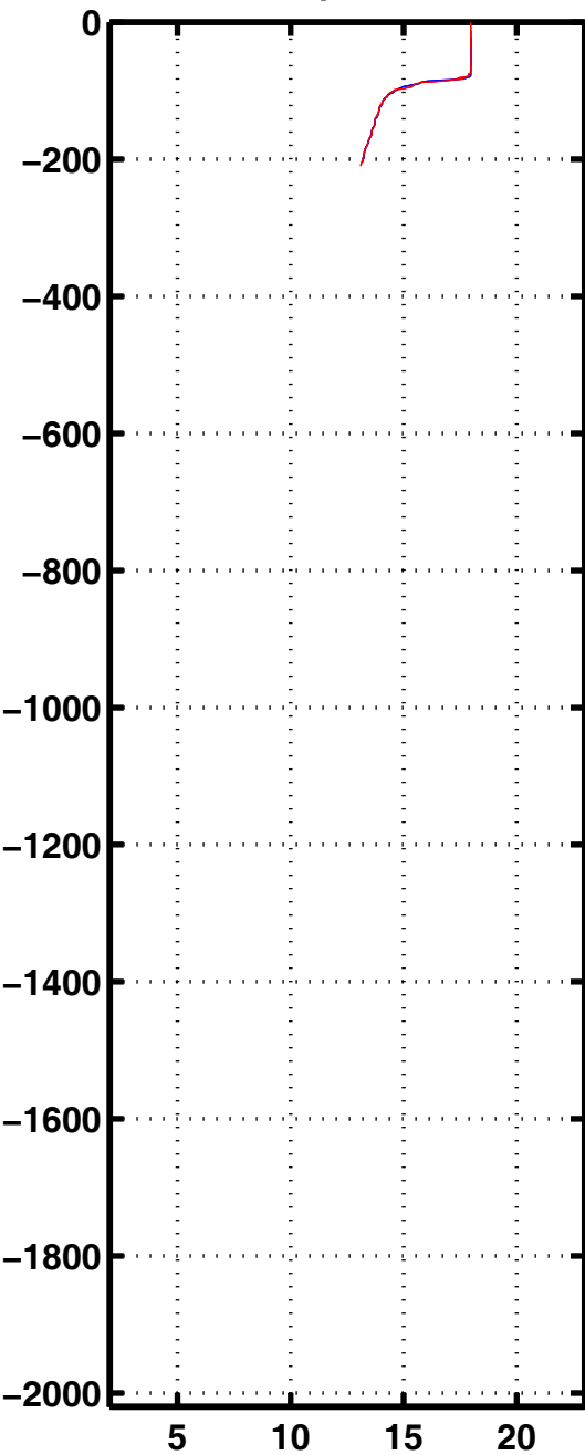
Tempe 3337
