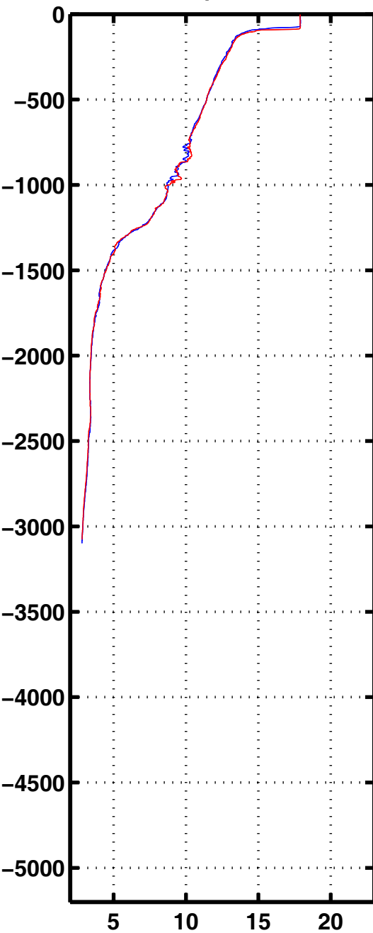
Tempe 3339
