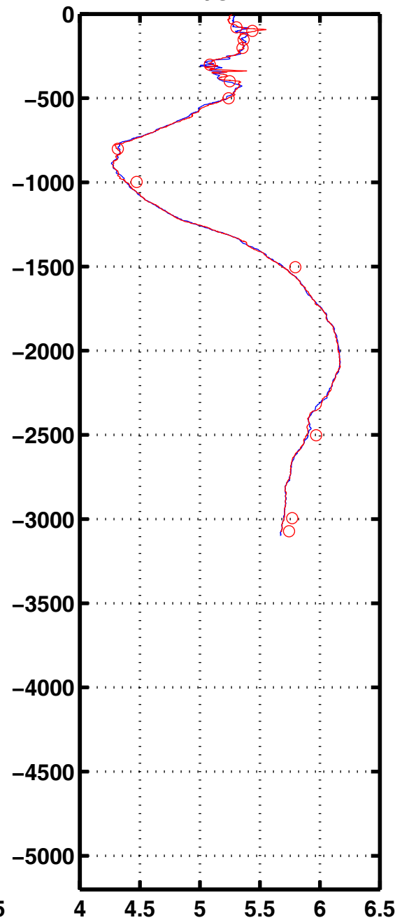
Oxyg 3339
