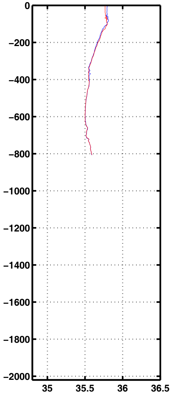
Sali 3332
