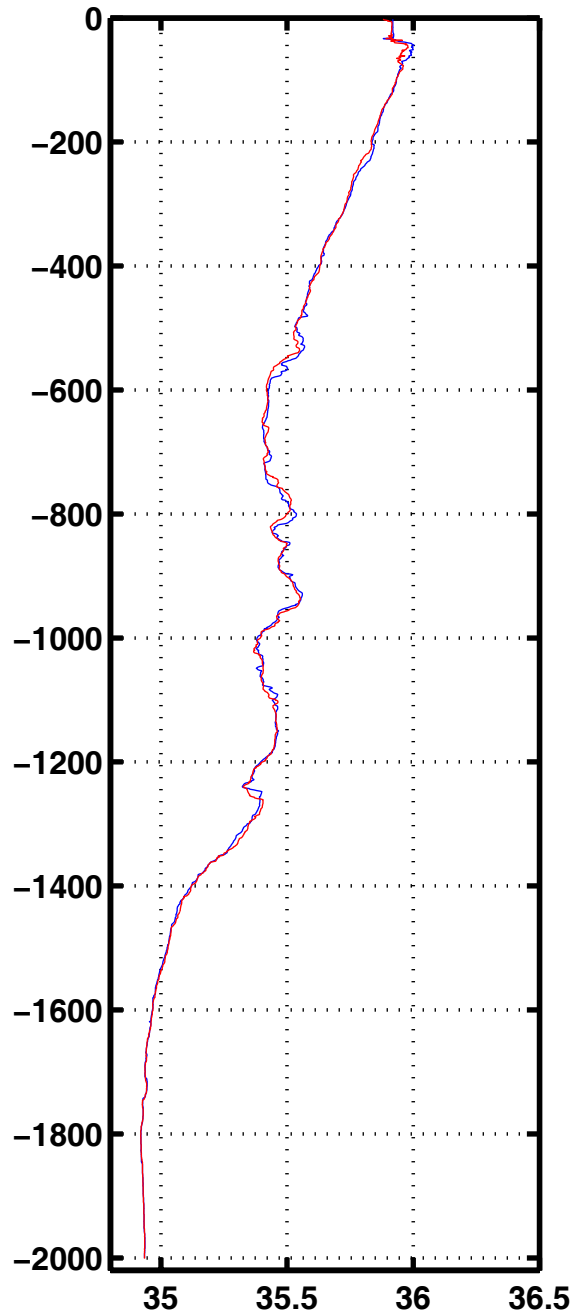
Sali 3076
