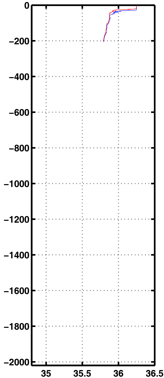
Sali 3093
