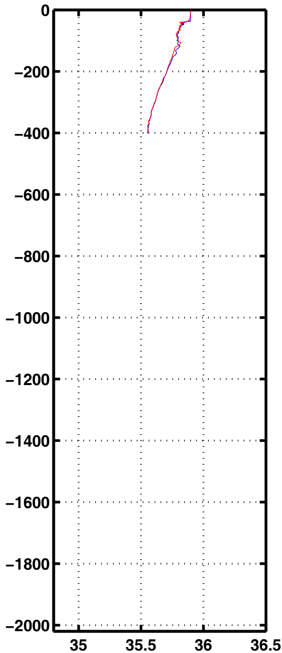
Sali 3245
