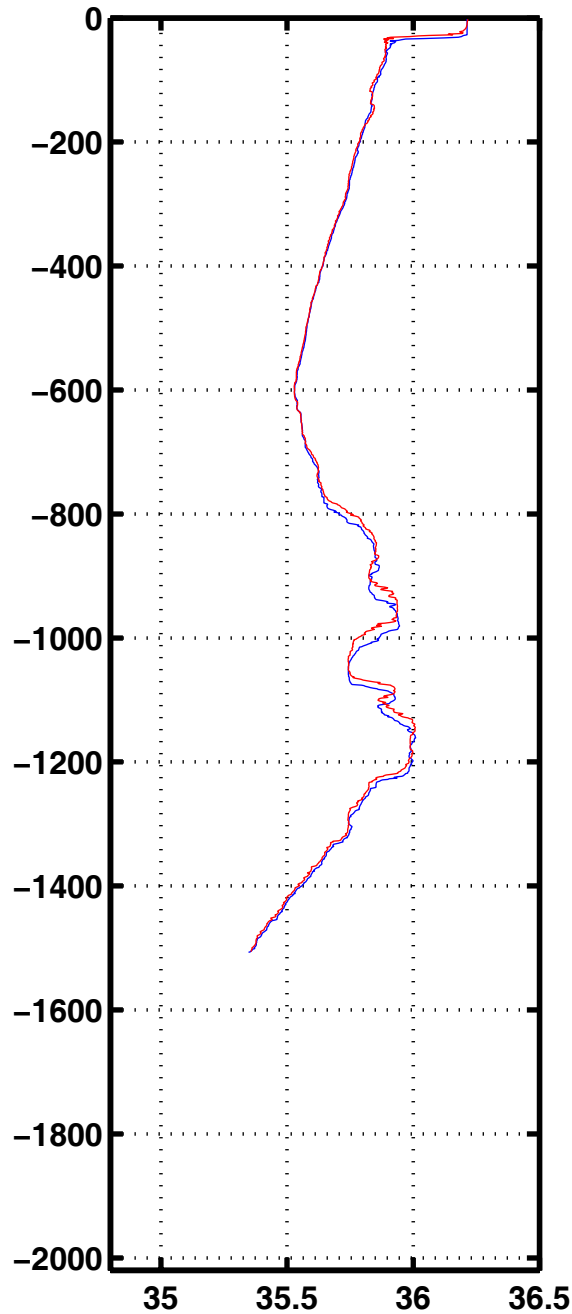
Sali 3098
