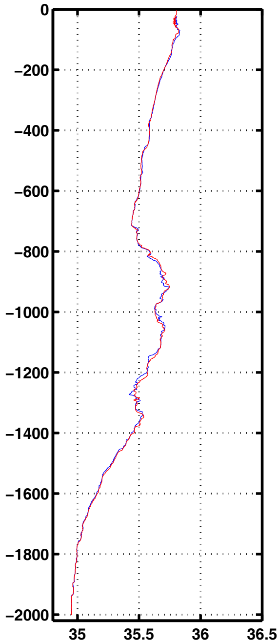
Sali 3050
