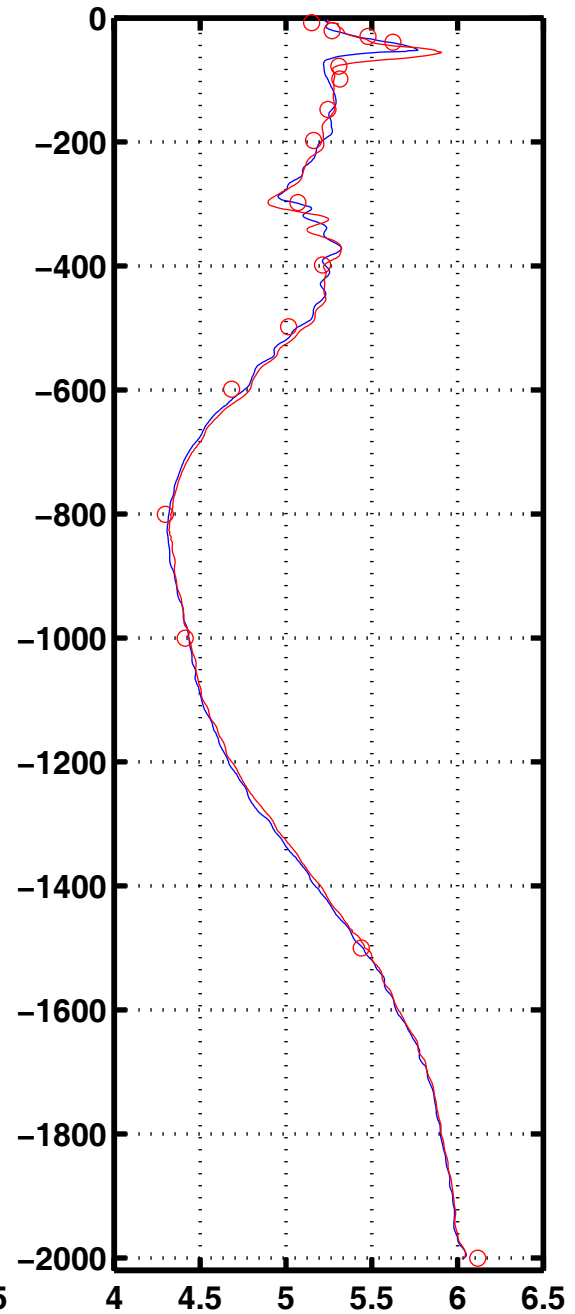
Oxyg 3020
