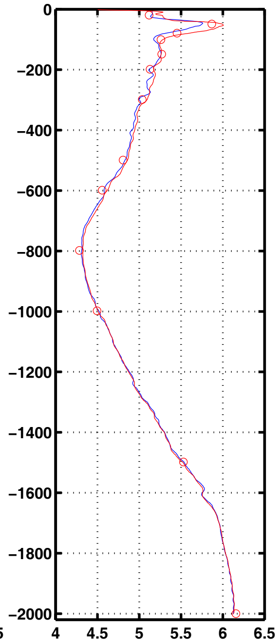
Oxyg 3055
