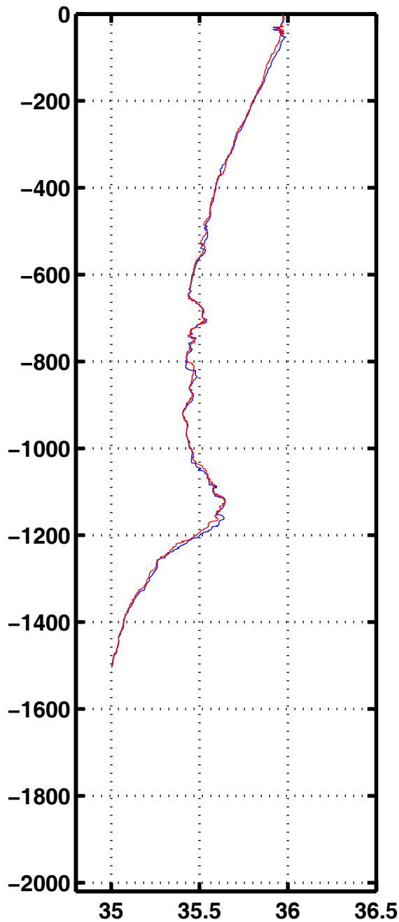
Sali 3159
