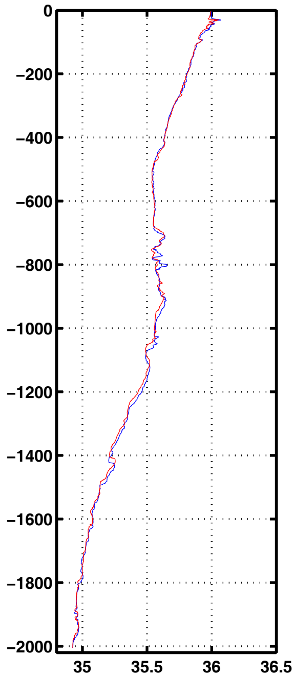
Sali 3045
