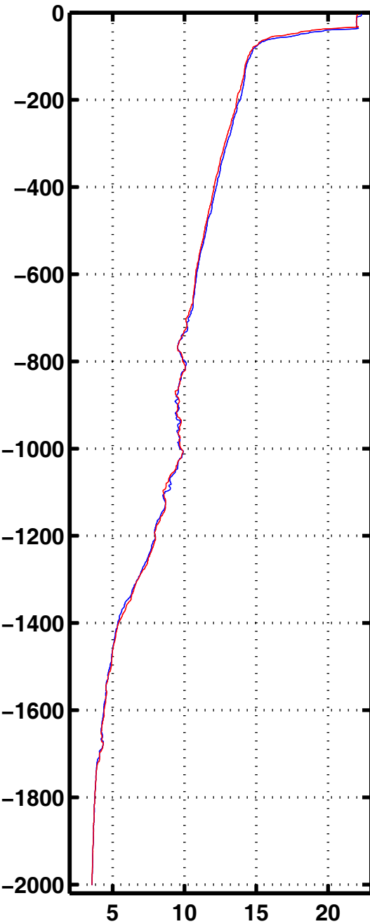
Tempe 3080
