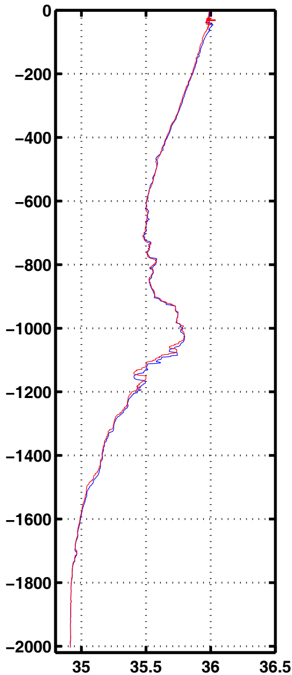
Sali 3057
