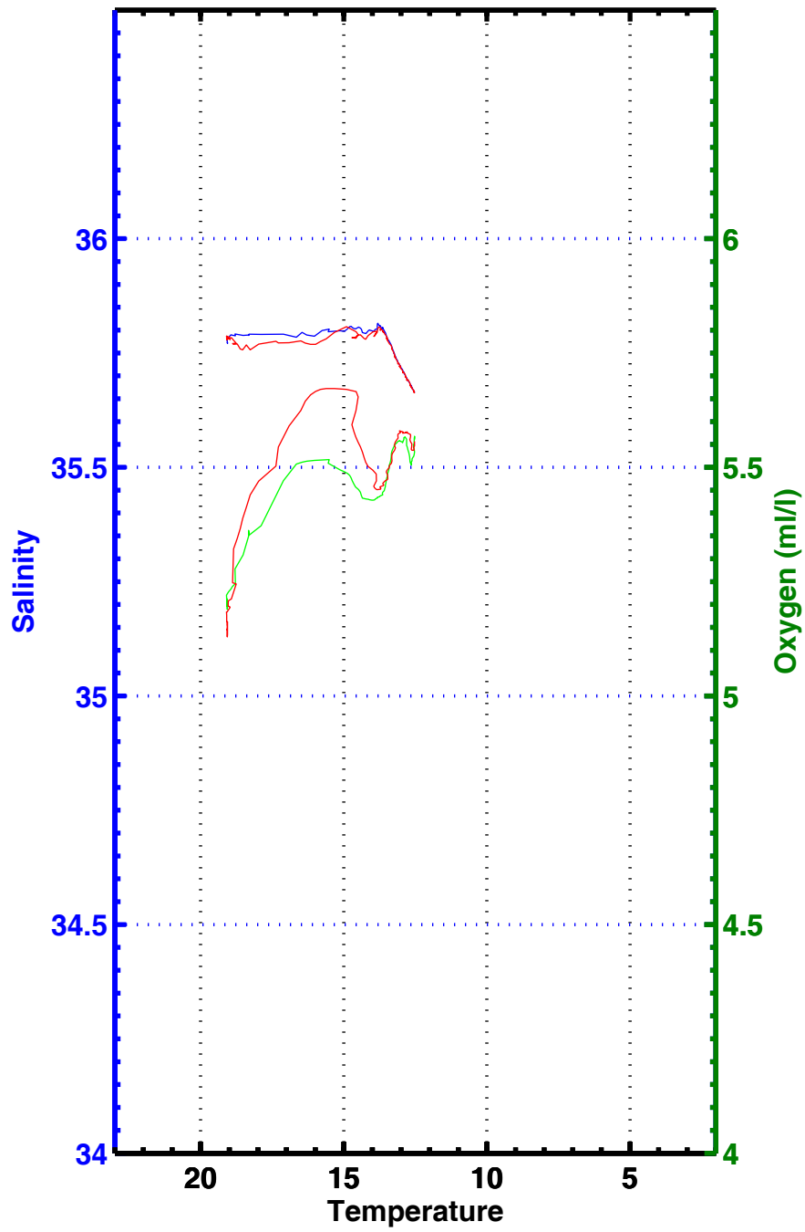
T-S , T-02 , station 3333
