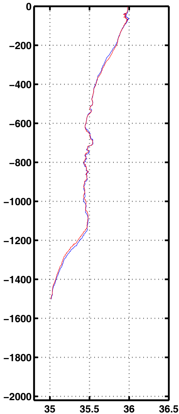
Sali 3155
