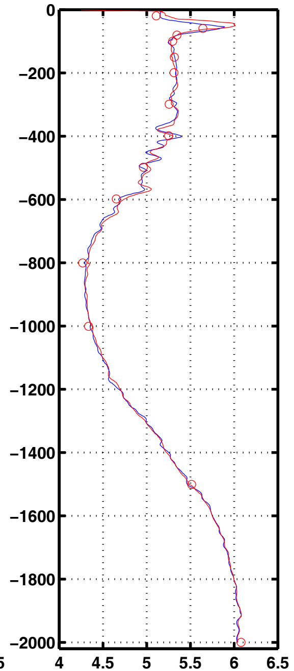
Oxyg 3032
