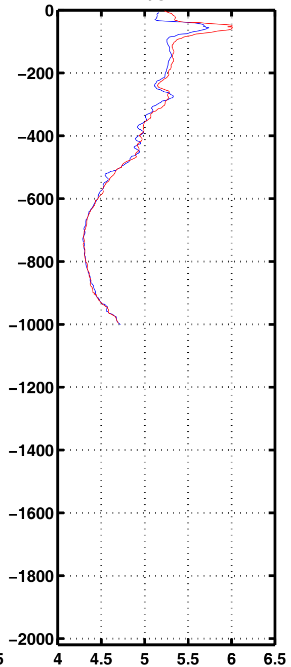
Oxyg 3244
