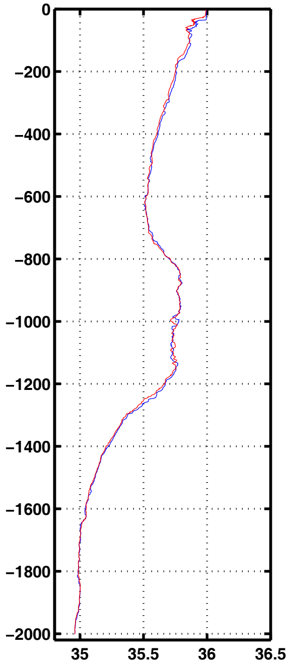
Sali 3033
