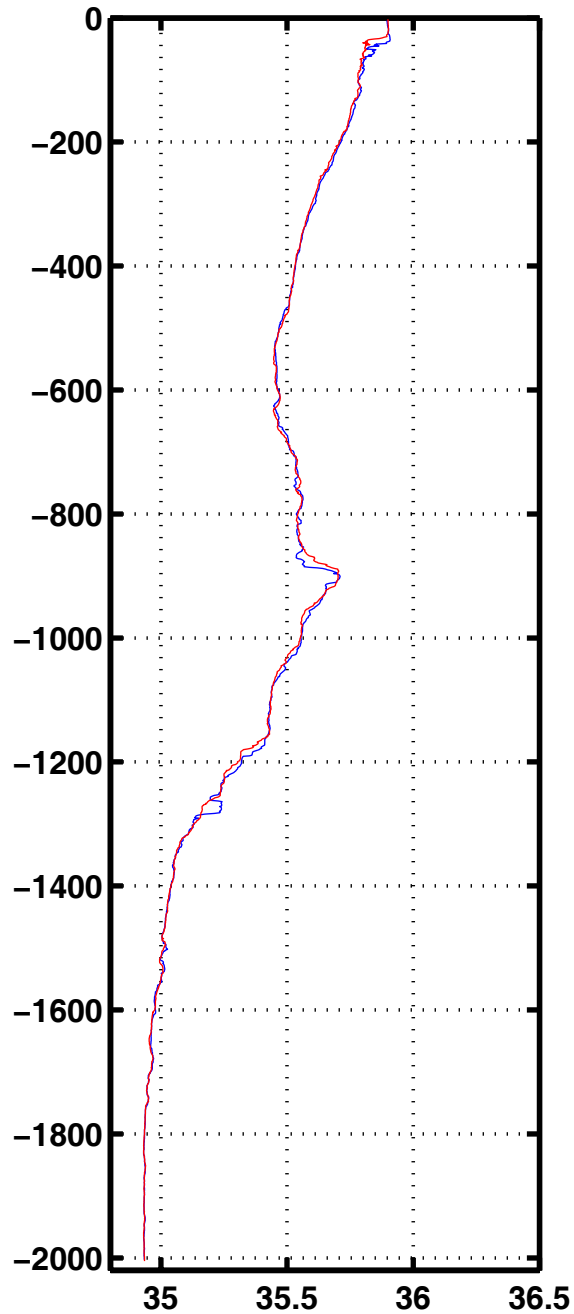
Sali 3252
