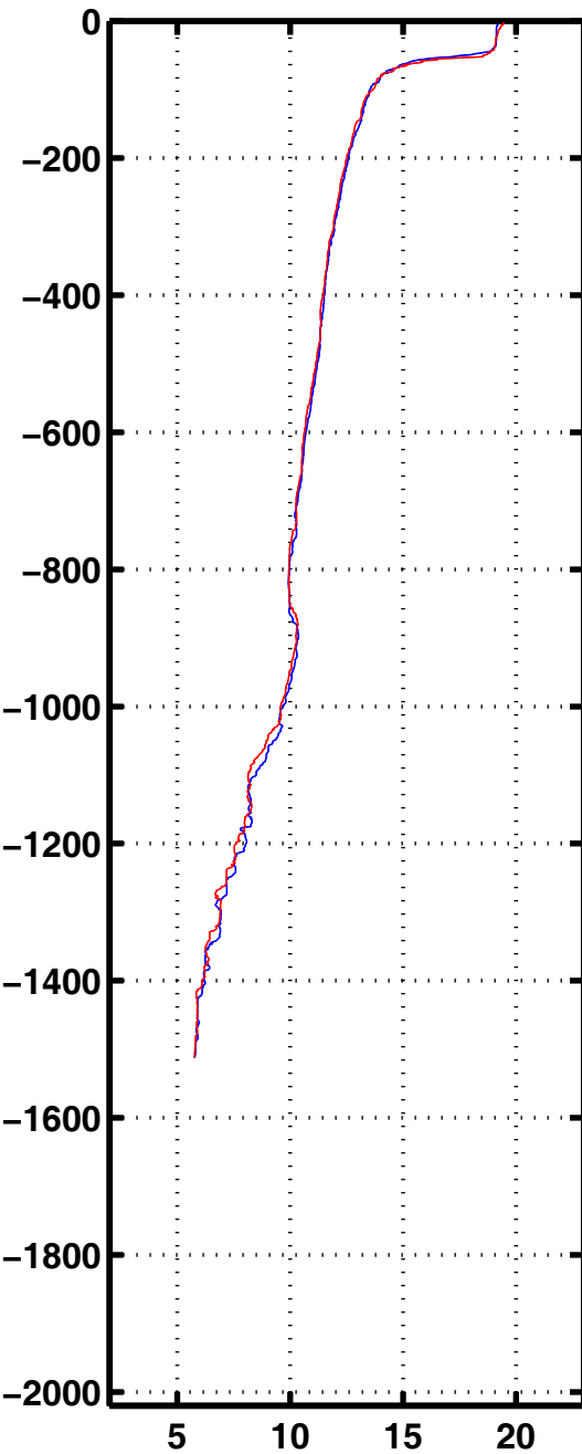
Tempe 3334
