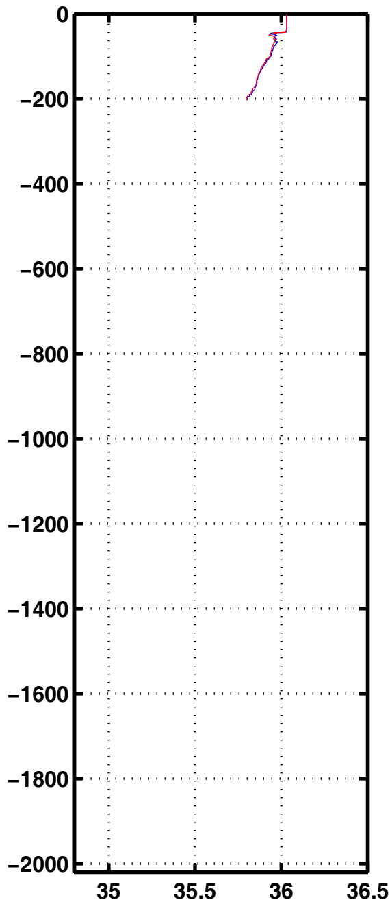
Sali 3163
