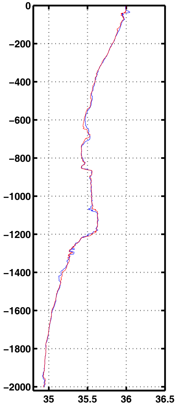
Sali 3168
