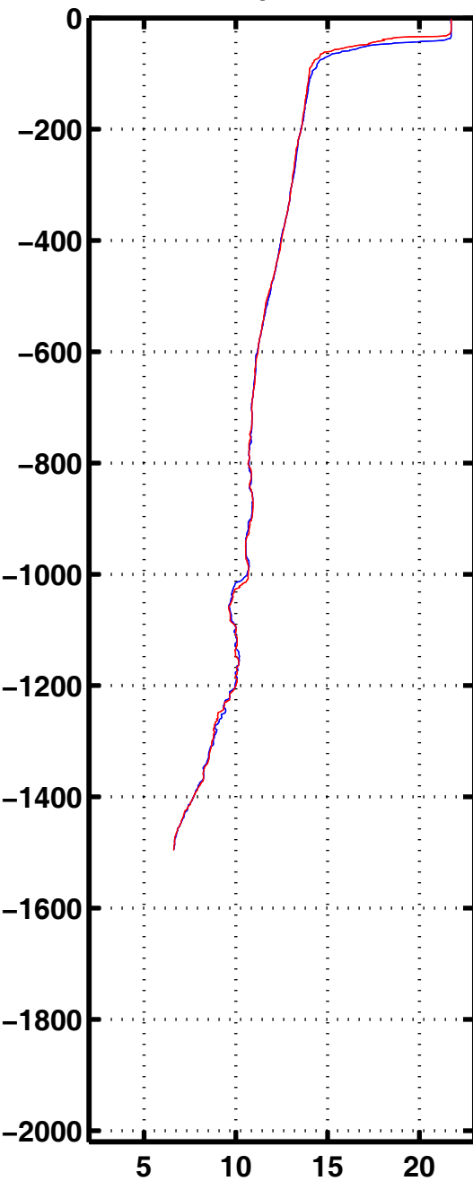
Tempe 3097
