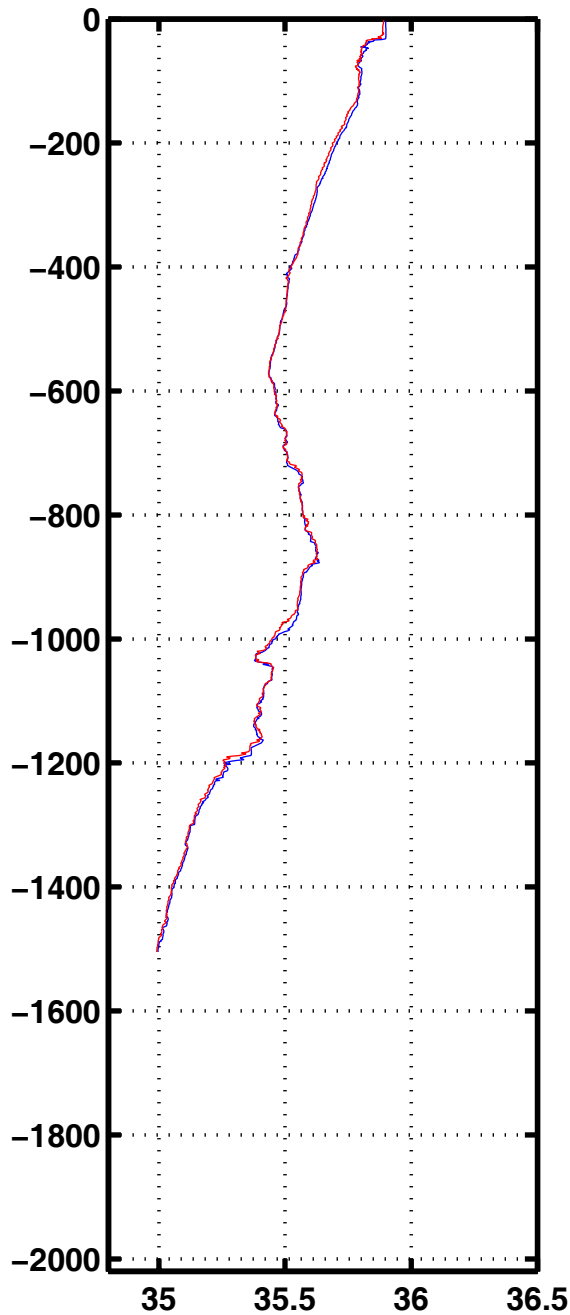
Sali 3241
