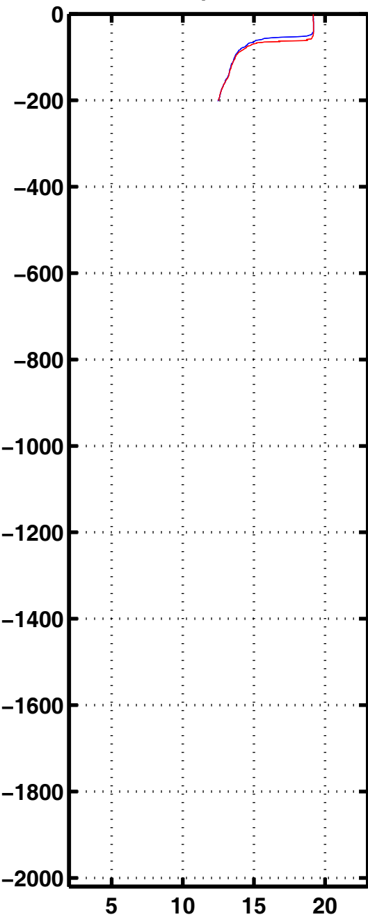
Tempe 3324
