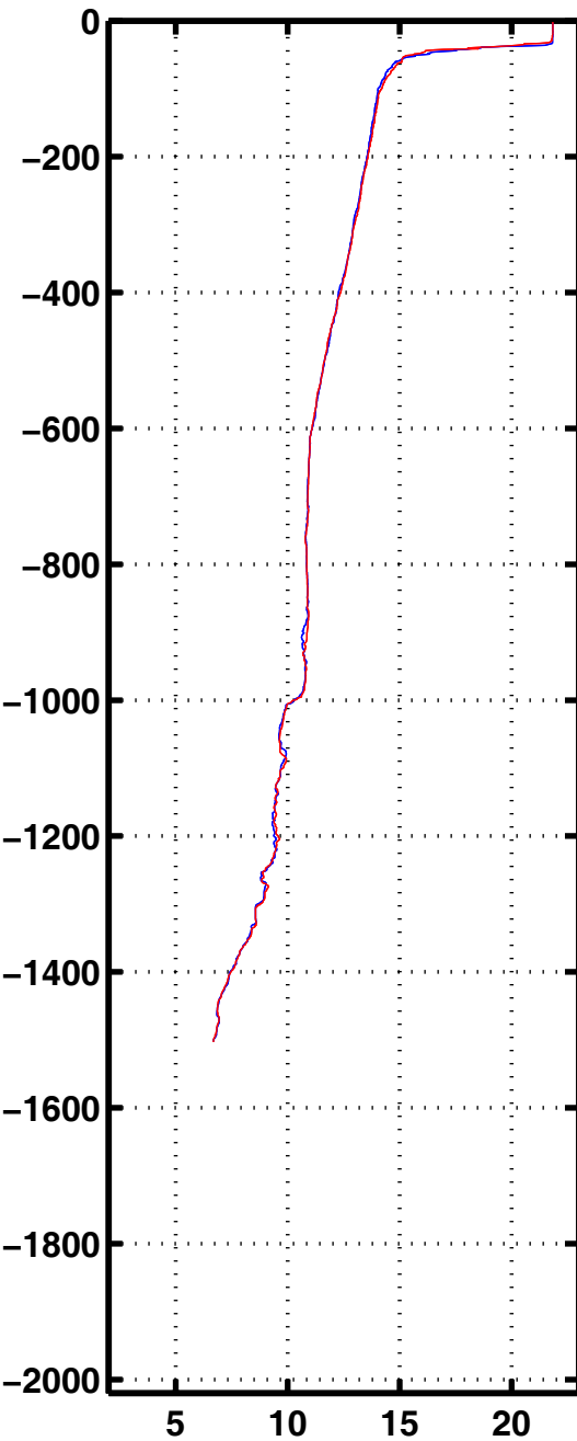
Tempe 3087
