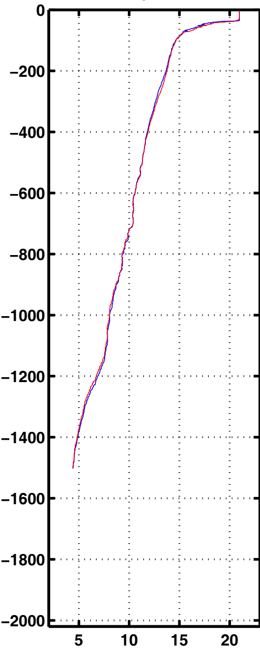
Tempe 3155
