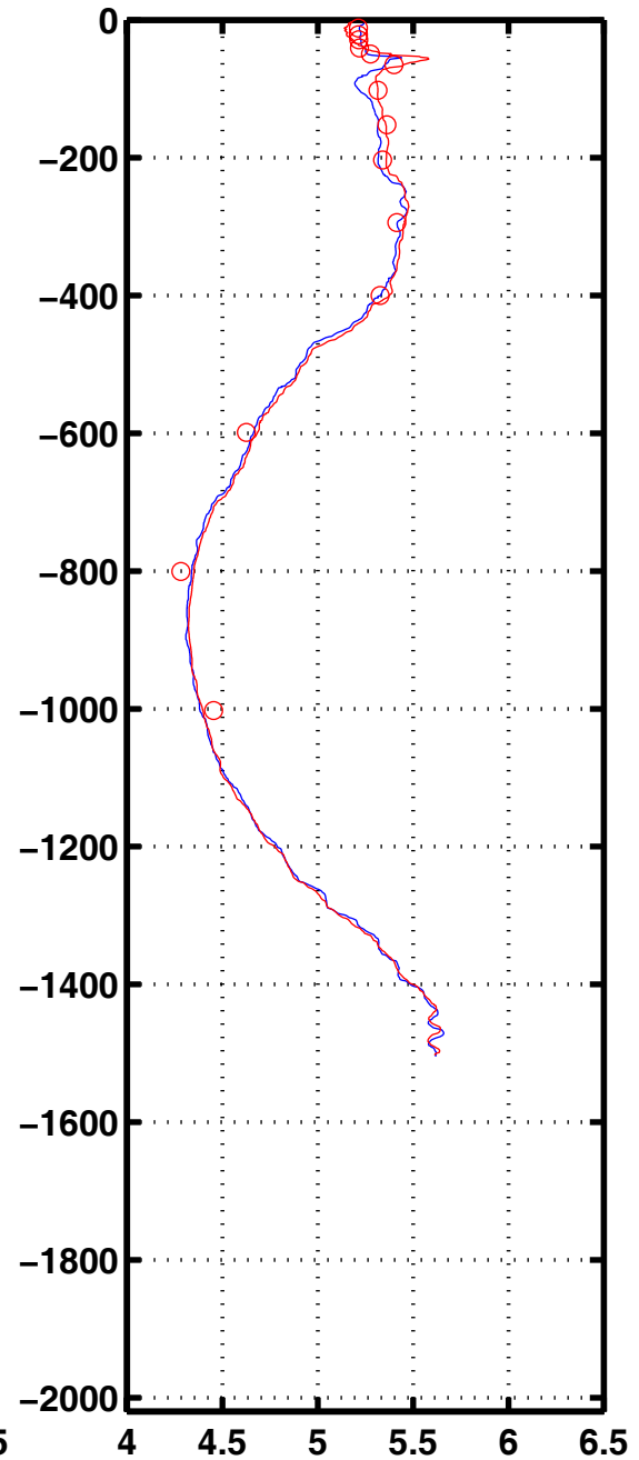
Oxyg 3325
