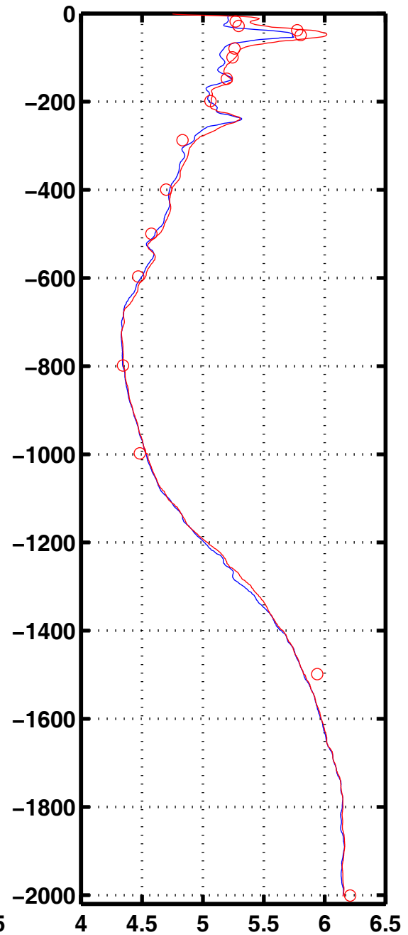
Oxyg 3073
