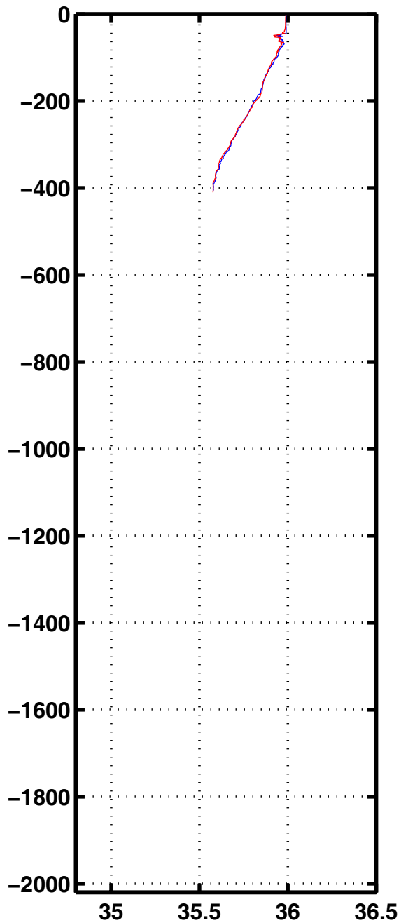
Sali 3161
