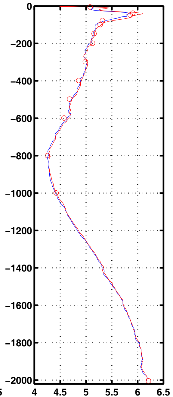
Oxyg 3045
