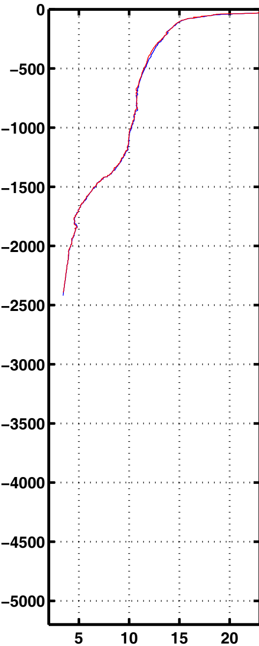
Tempe 3013
