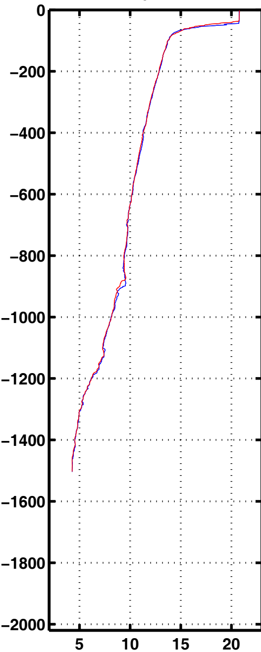
Tempe 3250
