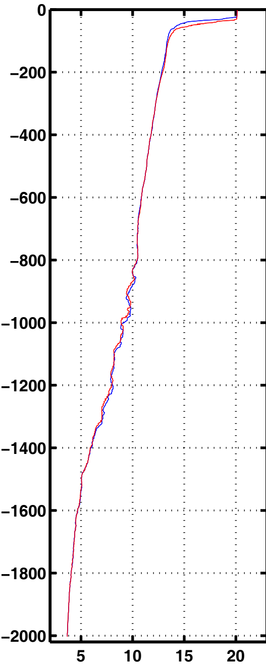
Tempe 3049
