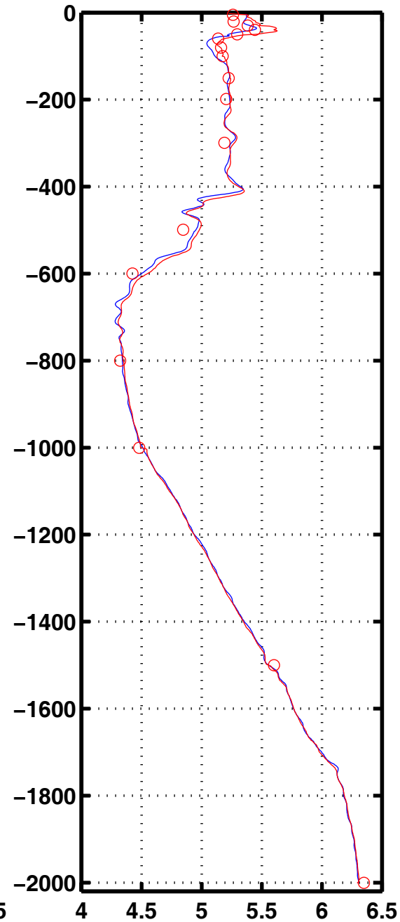
Oxyg 3069
