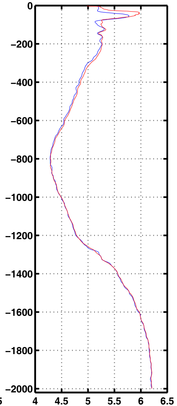
Oxyg 3059
