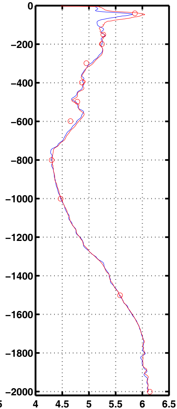
Oxyg 3019
