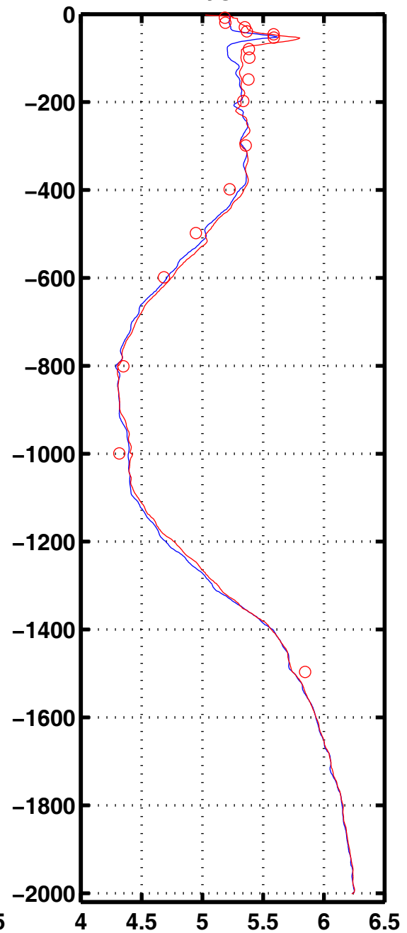
Oxyg 3051
