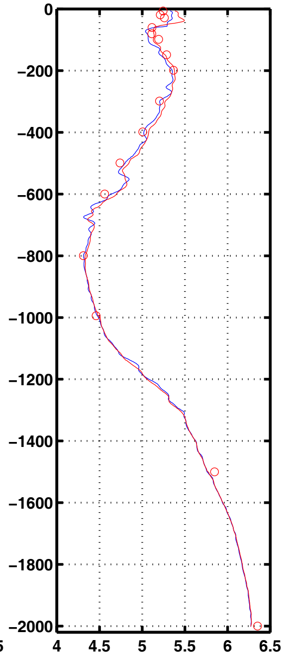
Oxyg 3063
