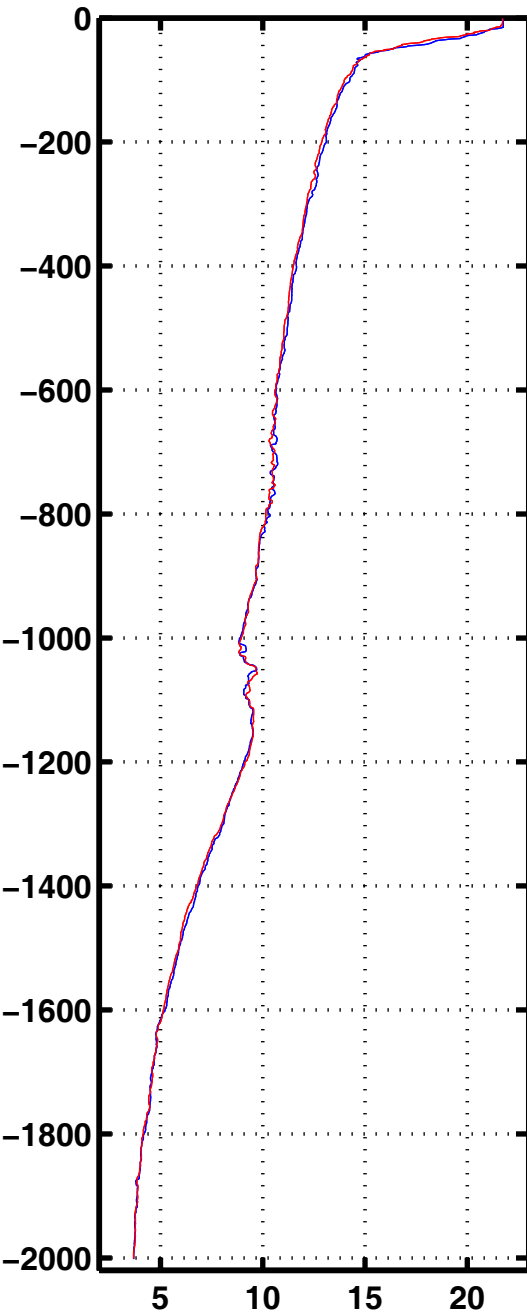
Tempe 3008
