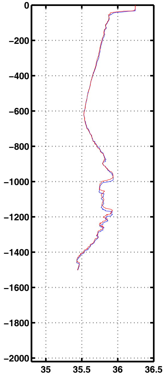
Sali 3085
