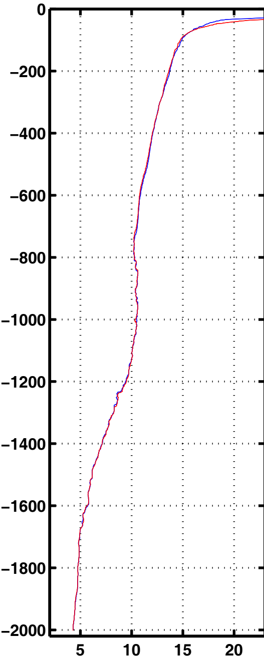
Tempe 3038
