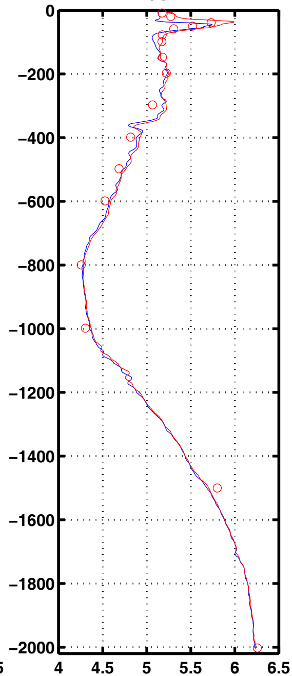
Oxyg 3057
