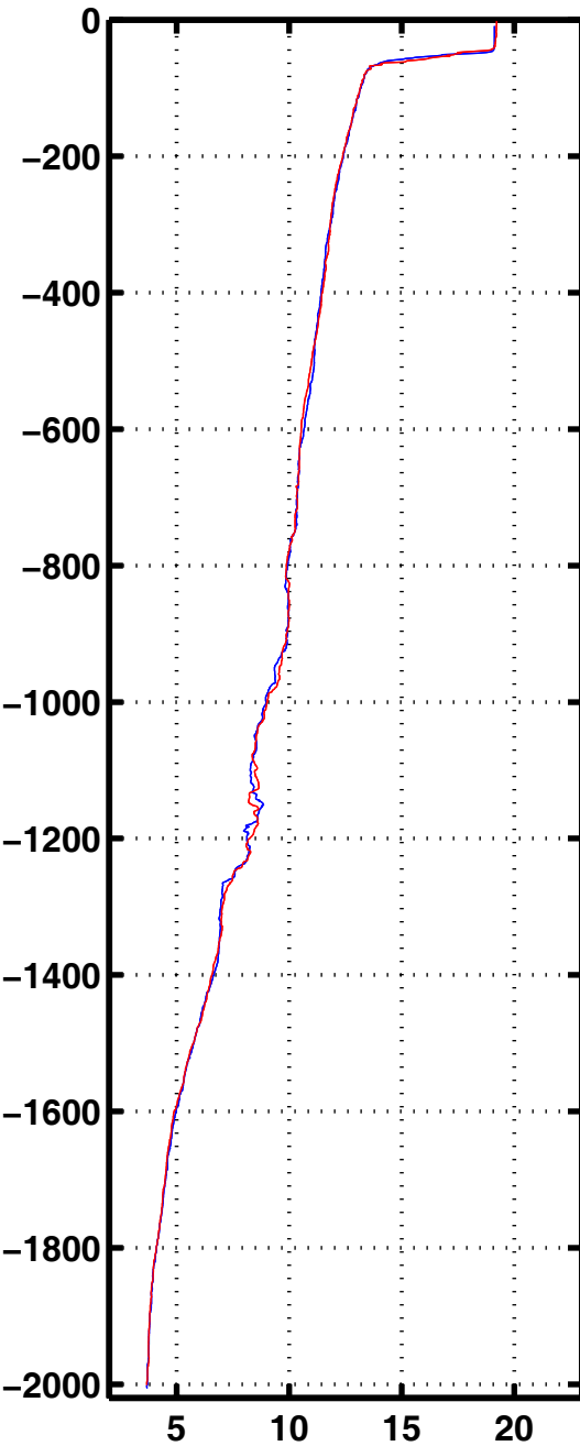
Tempe 3336
