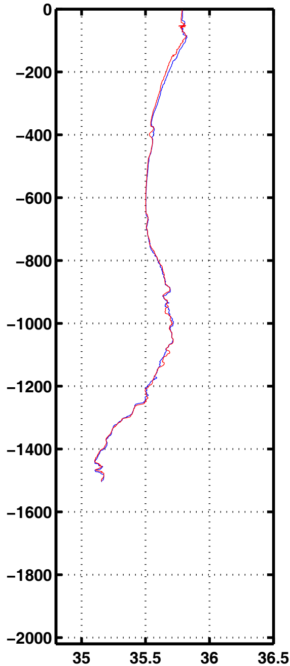
Sali 3325
