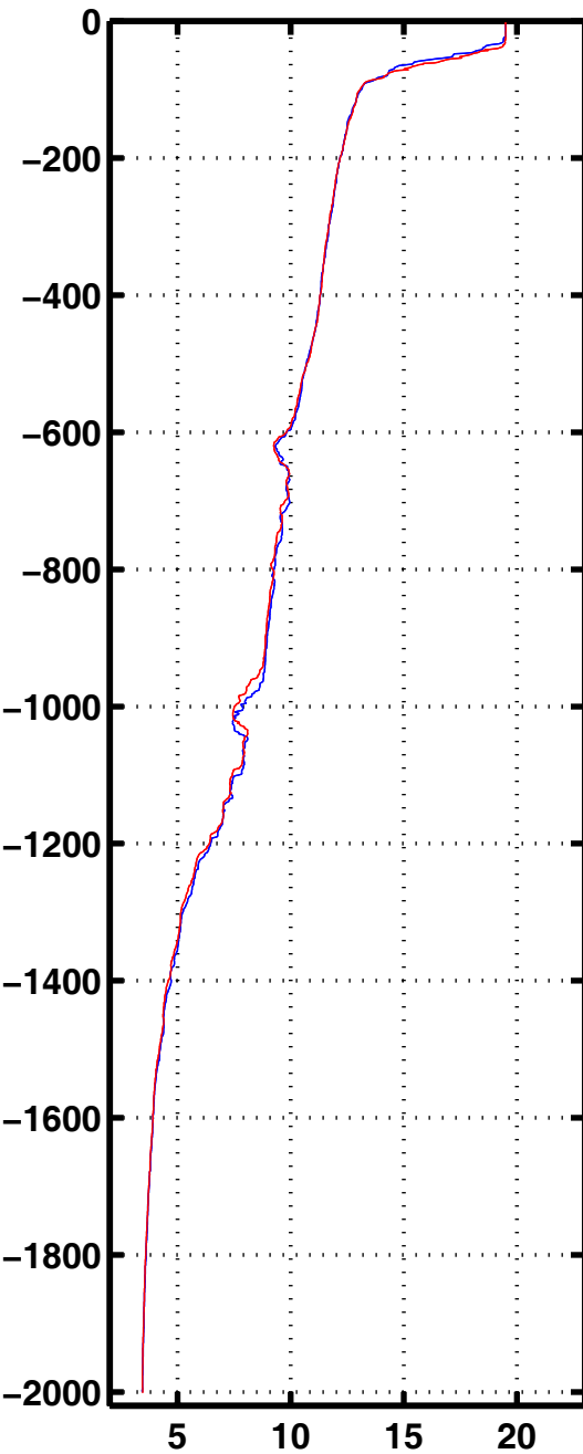
Tempe 3066
