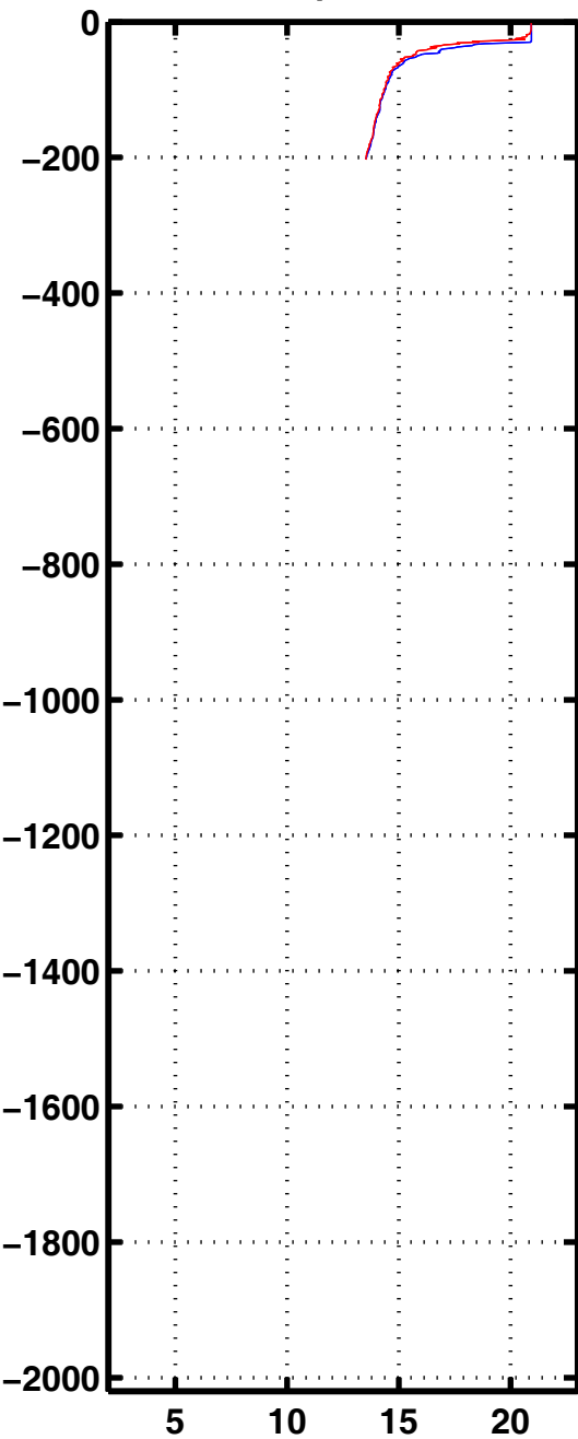
Tempe 3156
