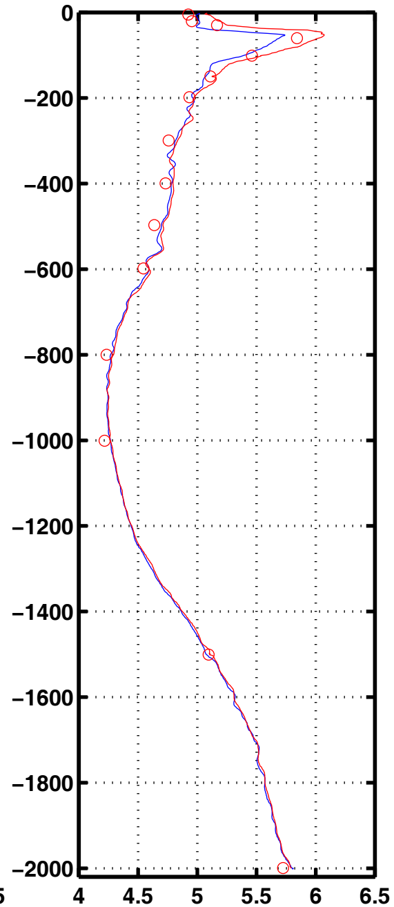
Oxyg 3037
