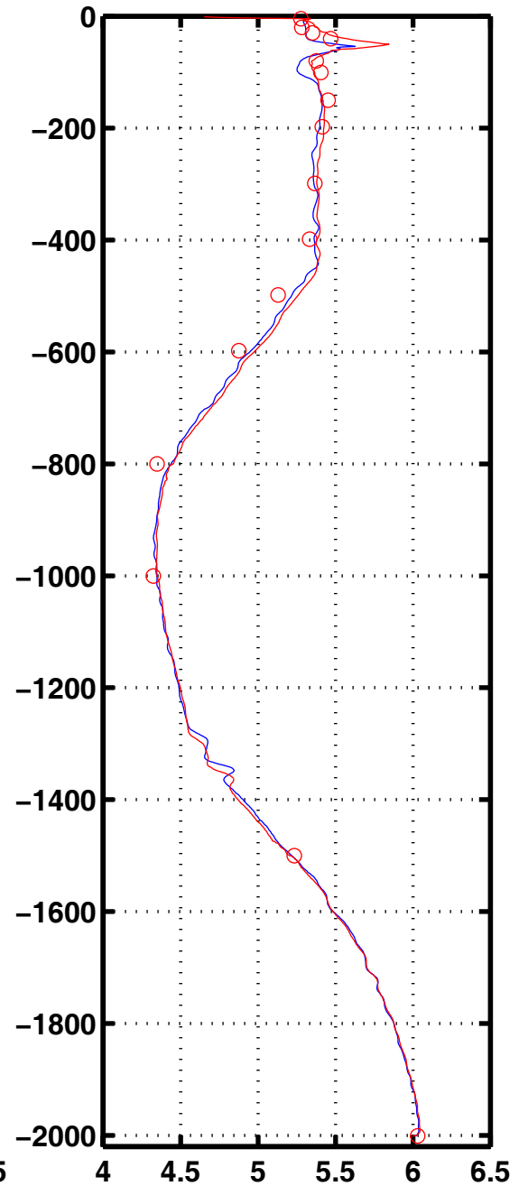
Oxyg 3023
