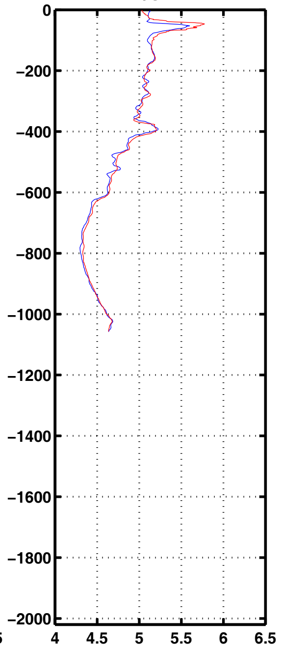
Oxyg 3158
