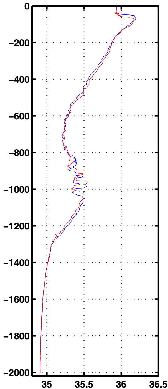
Sali 3067
