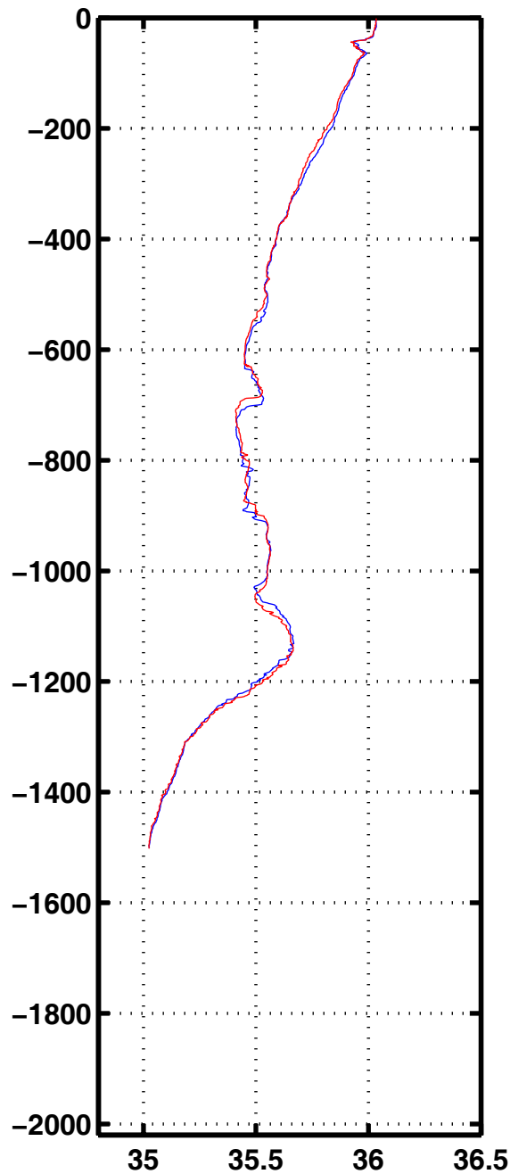
Sali 3167
