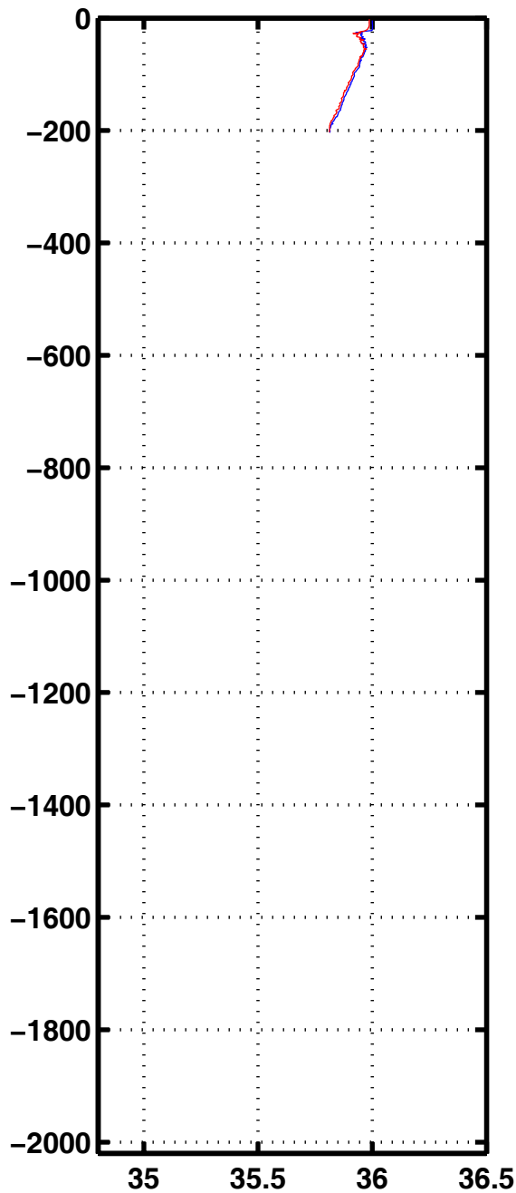
Sali 3165
