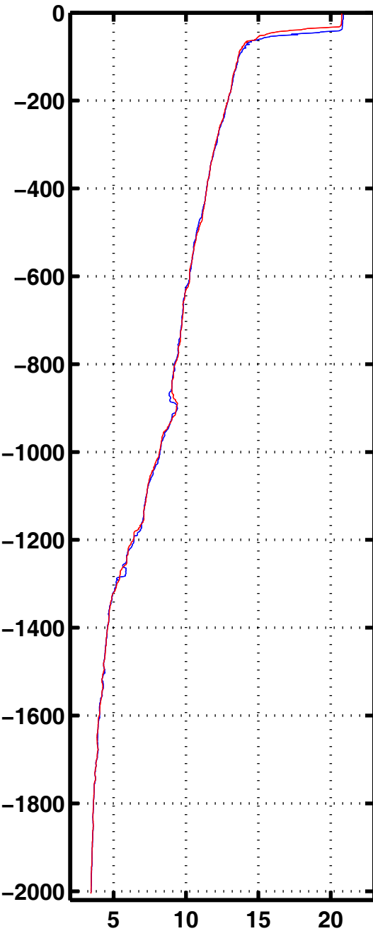
Tempe 3252
