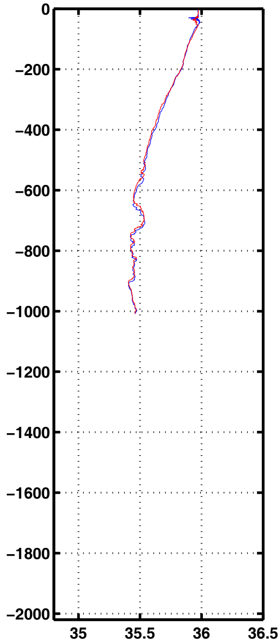
Sali 3160
