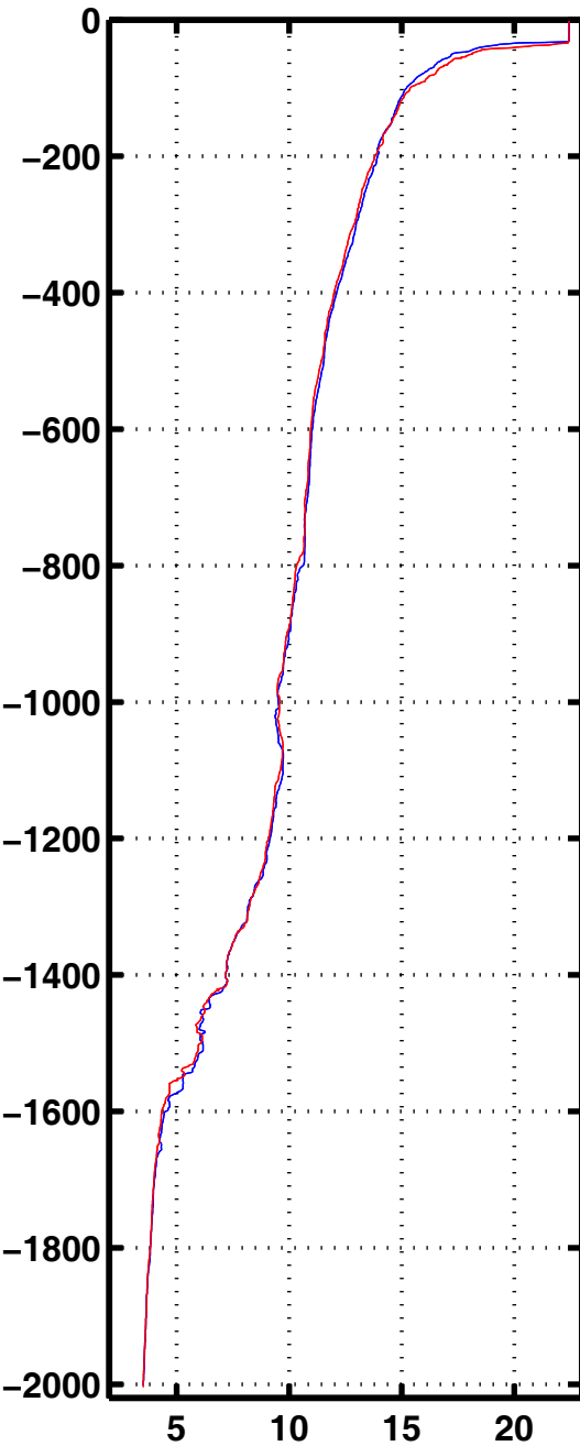
Tempe 3043
