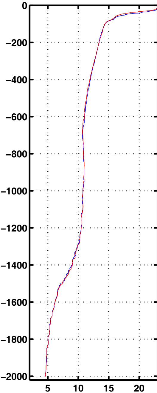
Tempe 3012
