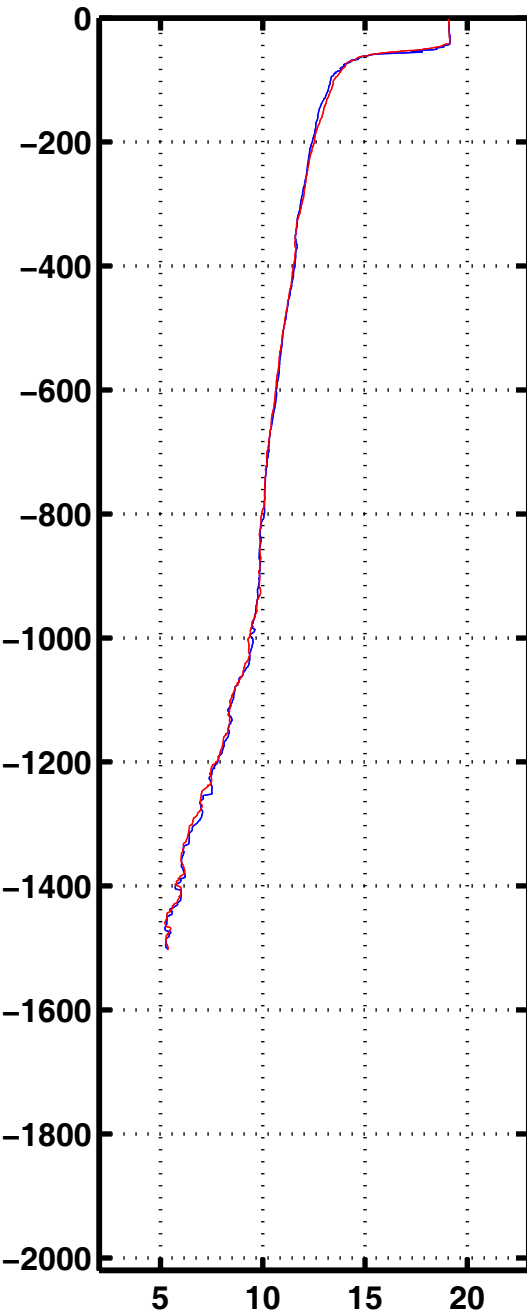
Tempe 3323
