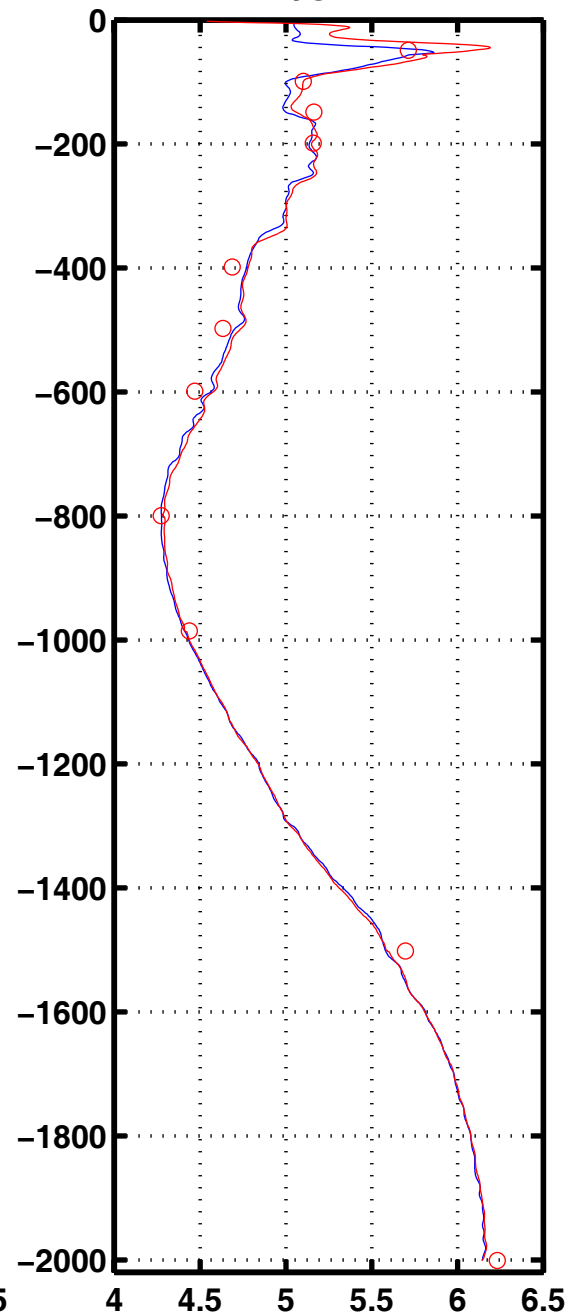
Oxyg 3078
