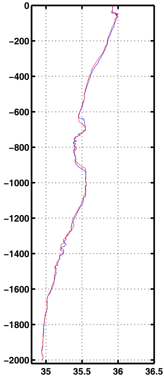
Sali 3053
