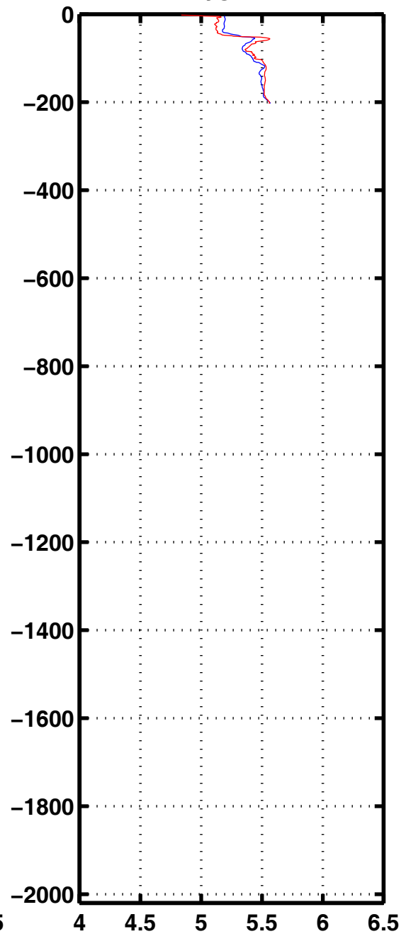
Oxyg 3331
