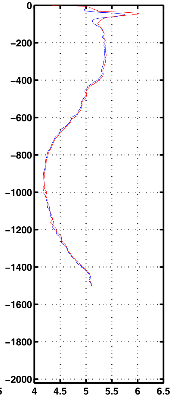
Oxyg 3085
