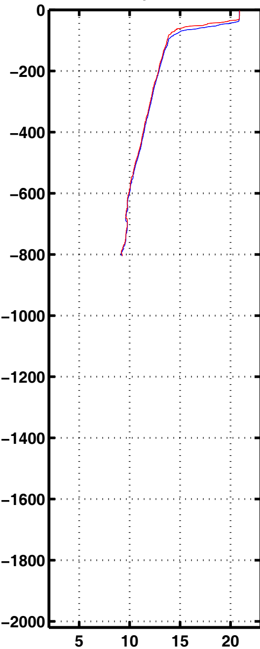
Tempe 3248
