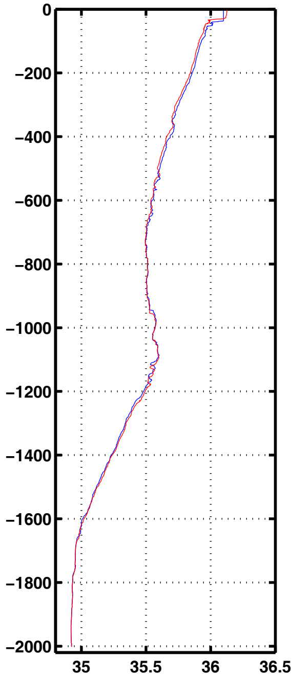
Sali 3056
