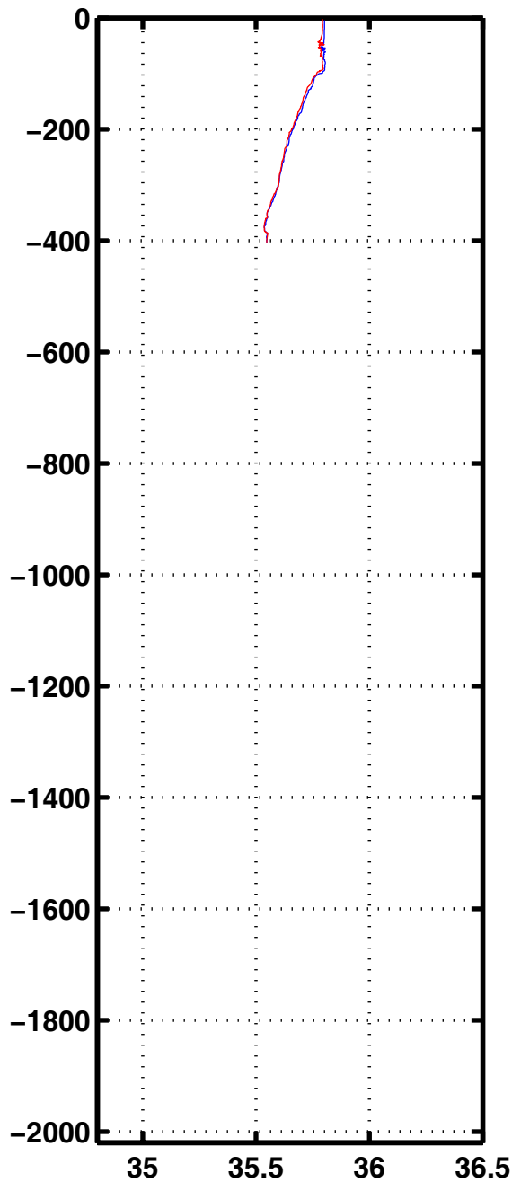
Sali 3329
