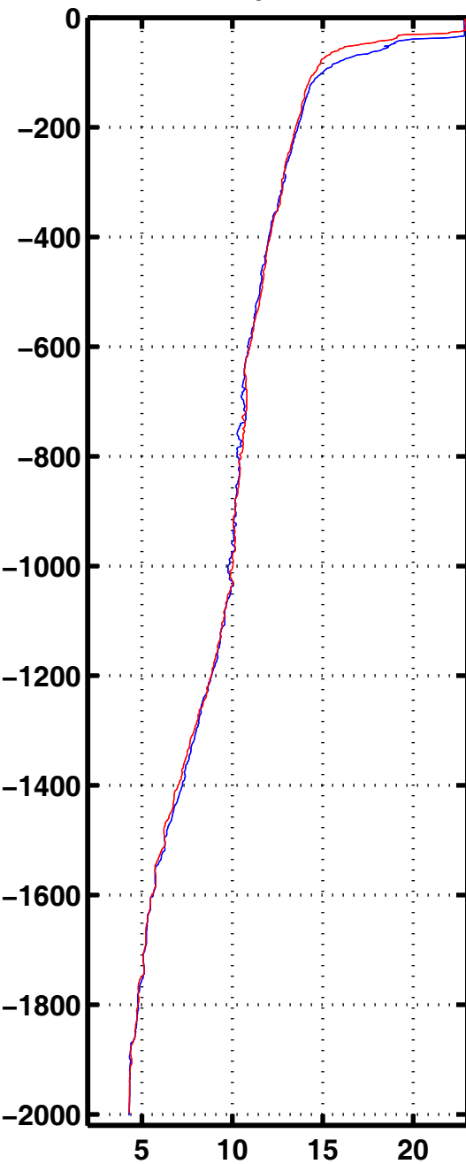
Tempe 3039
