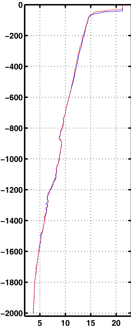
Tempe 3052
