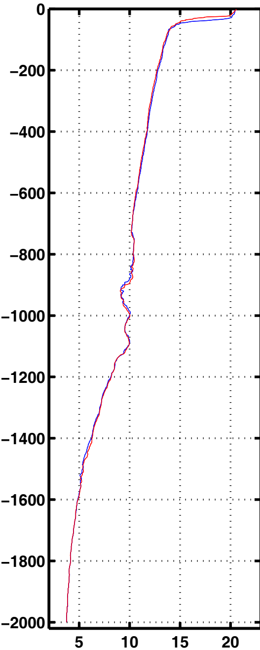
Tempe 3022
