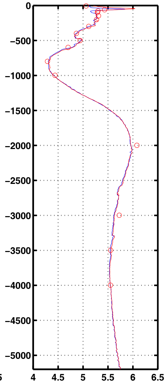
Oxyg 3031
