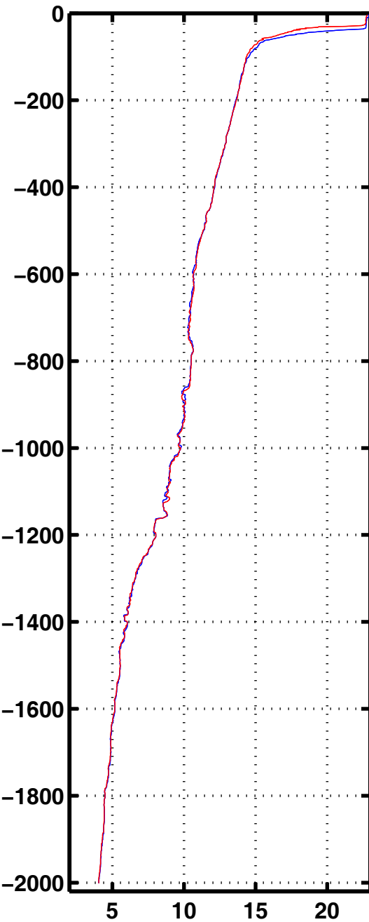
Tempe 3083
