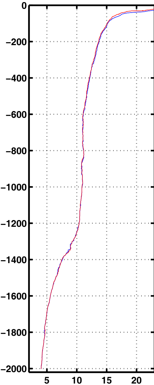
Tempe 3011
