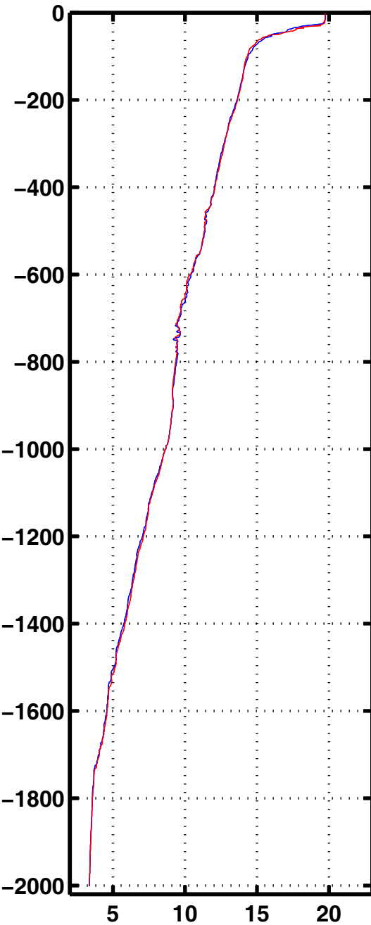
Tempe 3069
