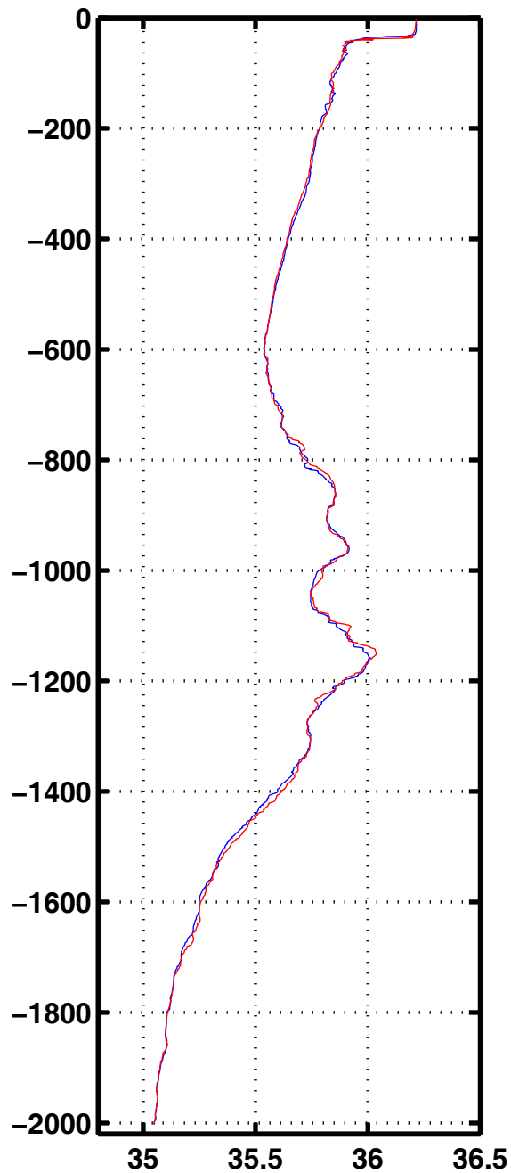
Sali 3099
