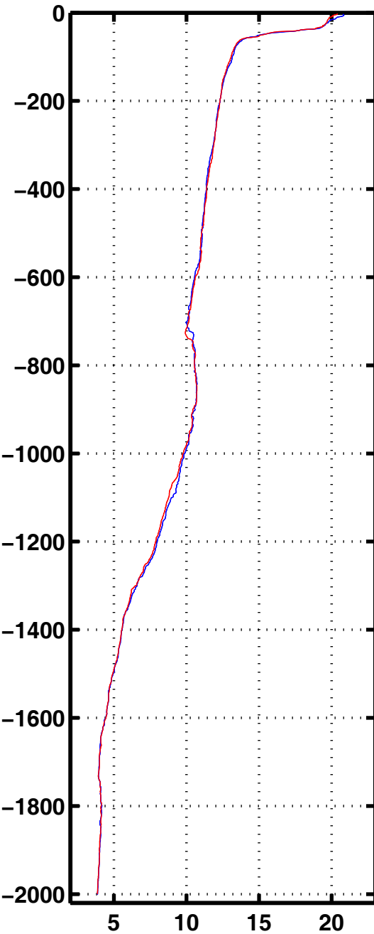
Tempe 3028
