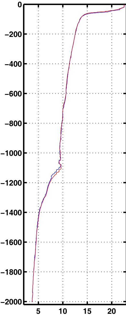
Tempe 3009
