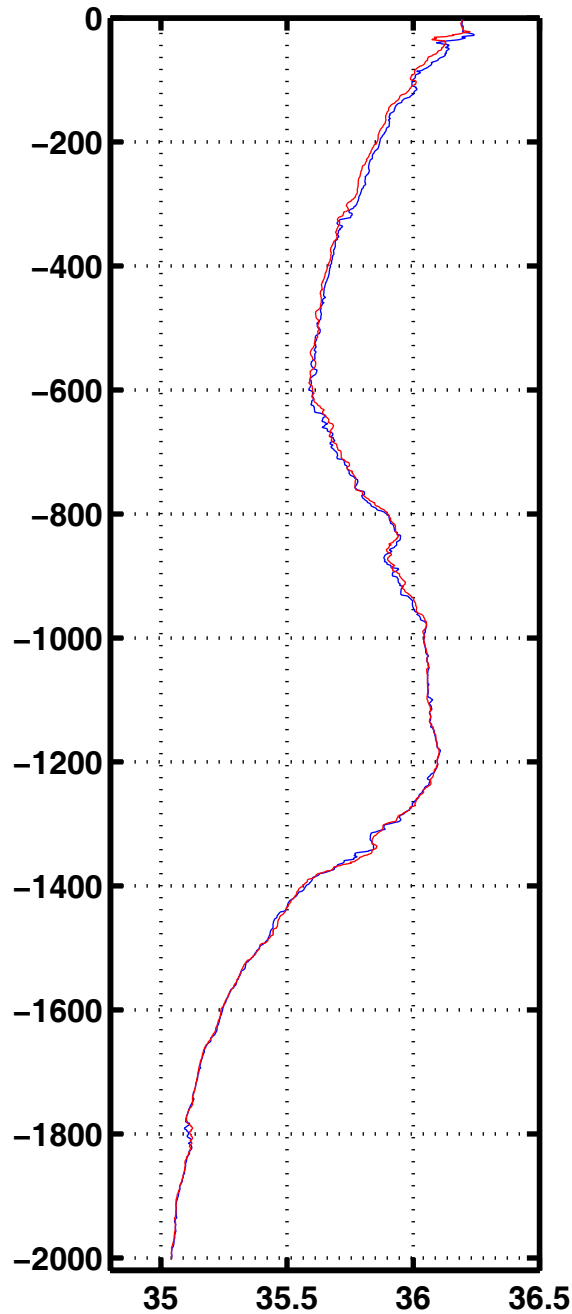
Sali 3011
