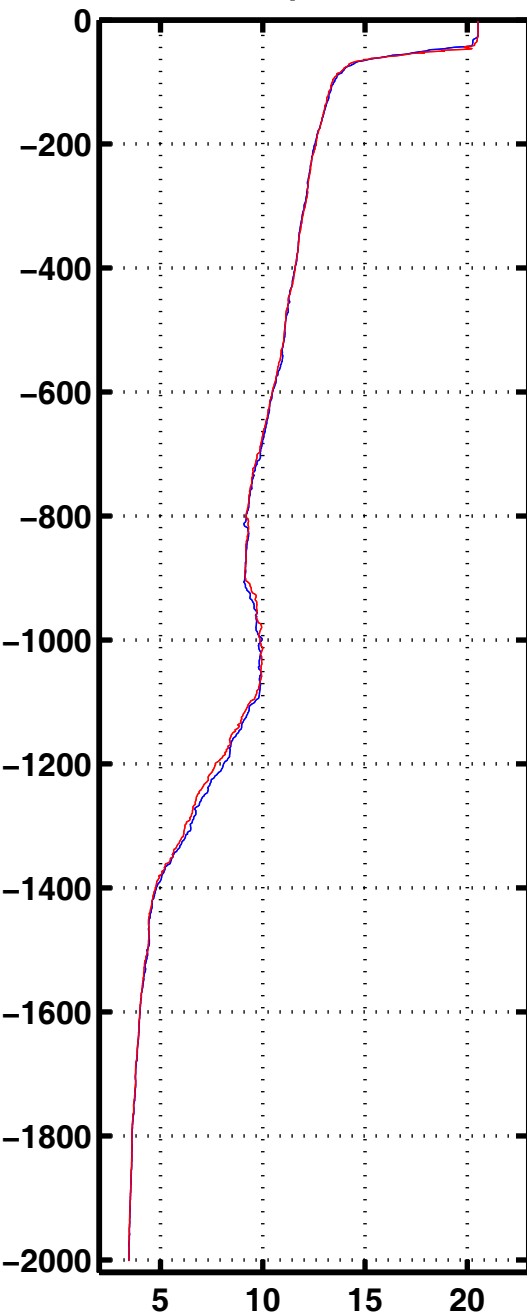
Tempe 3051
