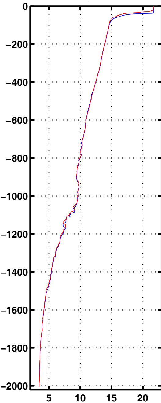
Tempe 3057
