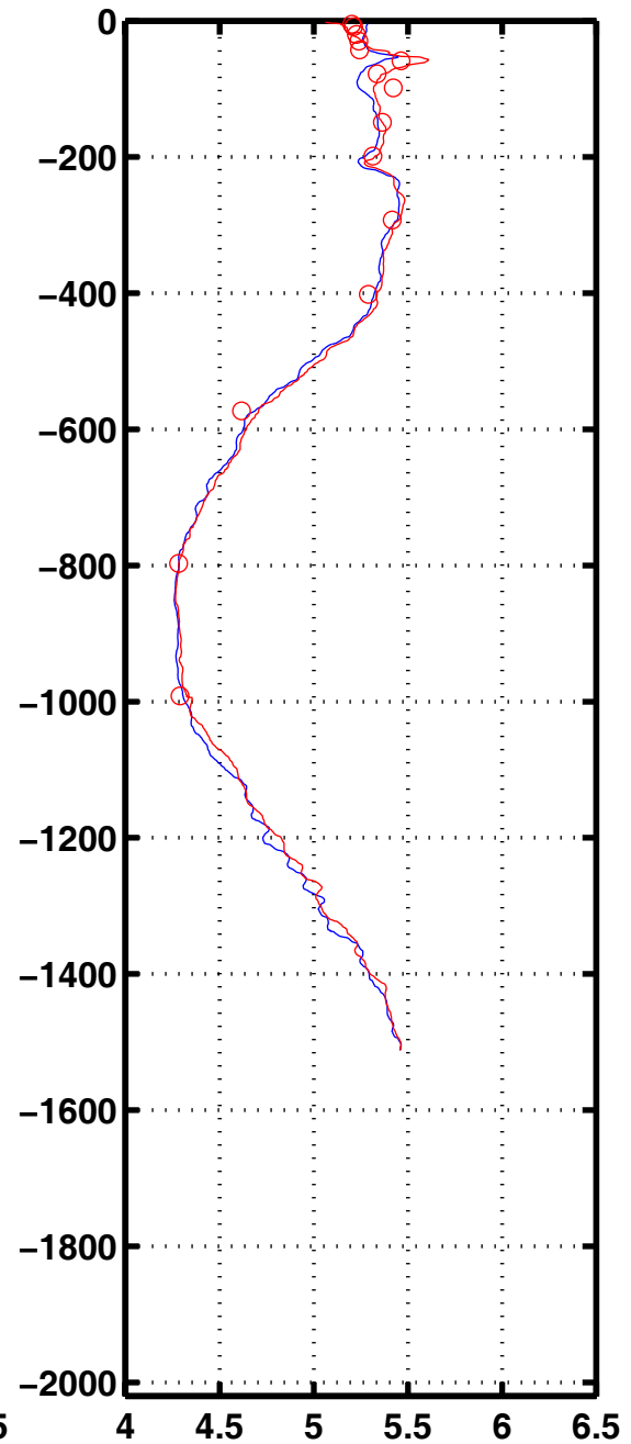
Oxyg 3334
