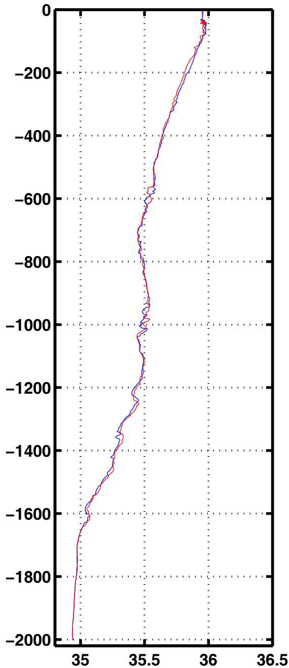
Sali 3055
