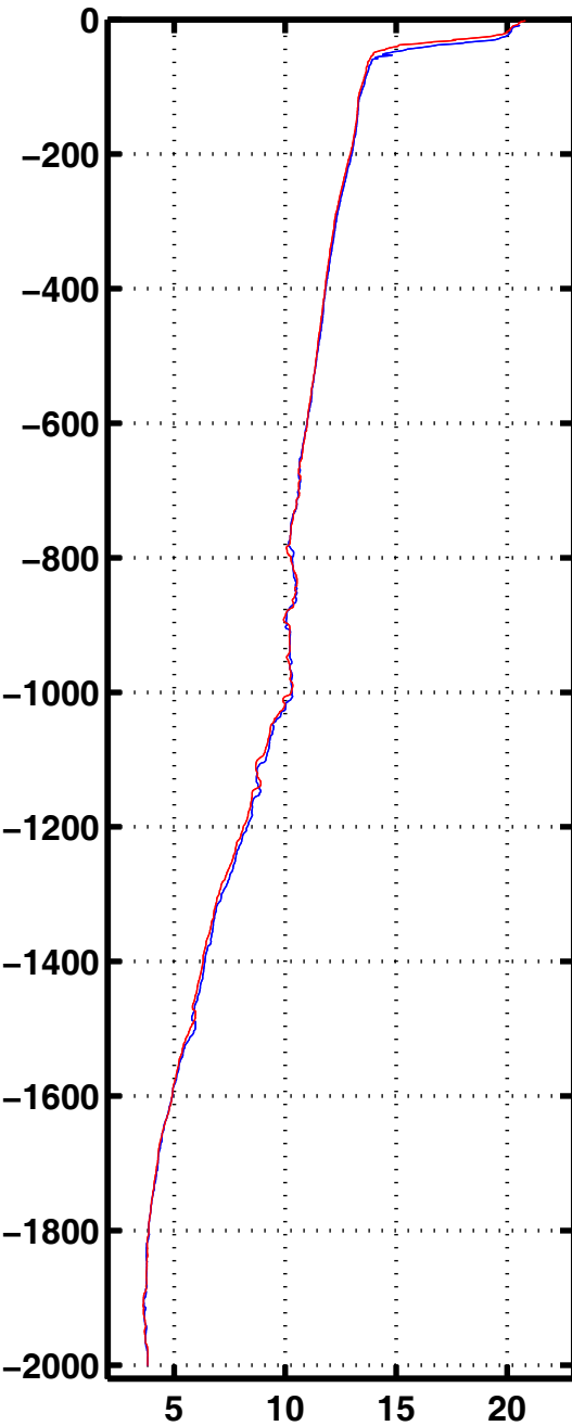
Tempe 3027
