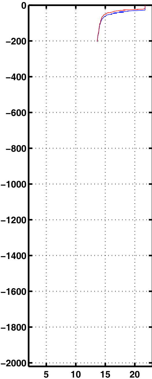
Tempe 3093
