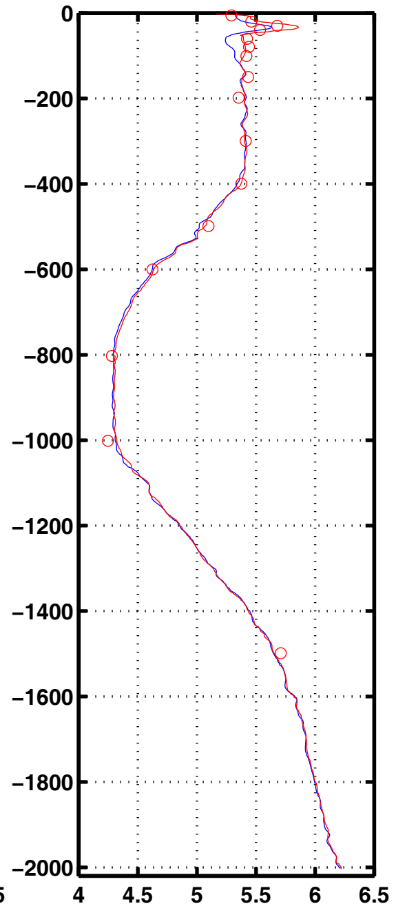
Oxyg 3021
