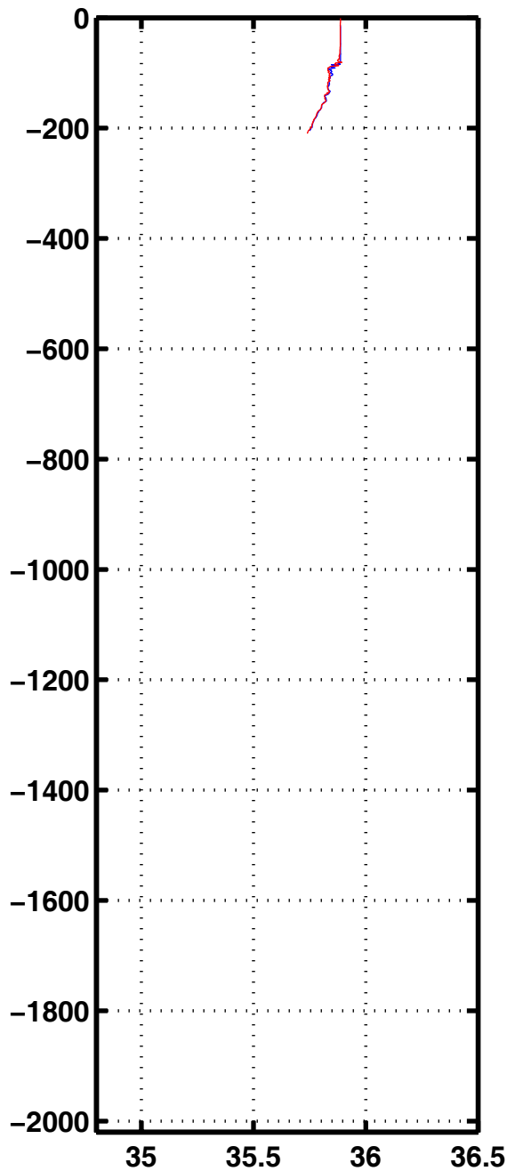
Sali 3337
