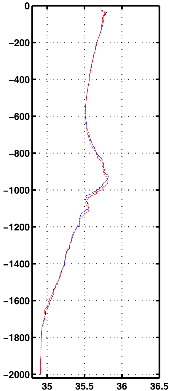
Sali 3001
