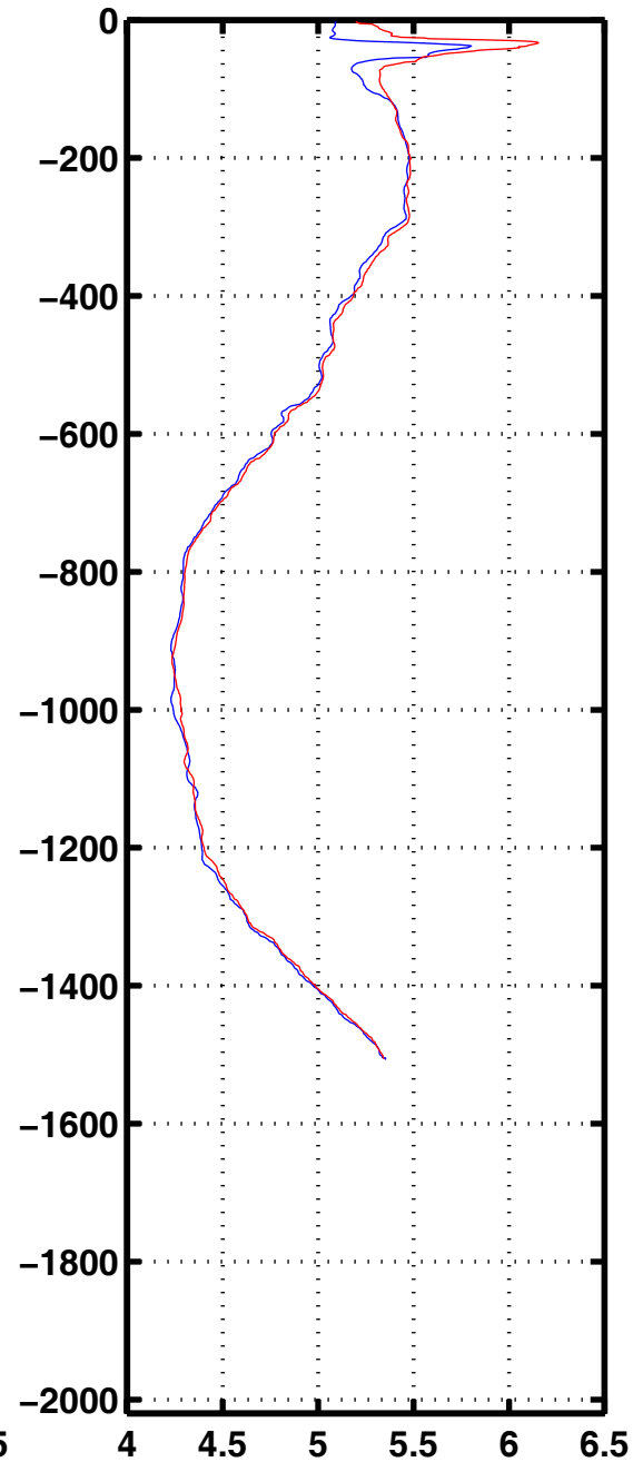
Oxyg 3098
