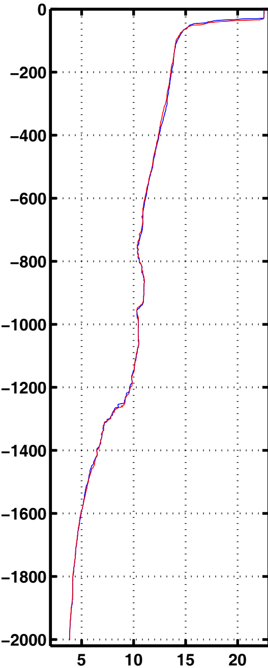
Tempe 3041
