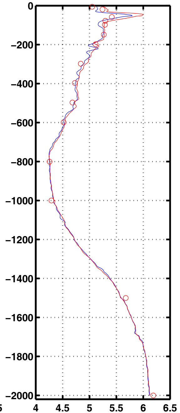
Oxyg 3080
