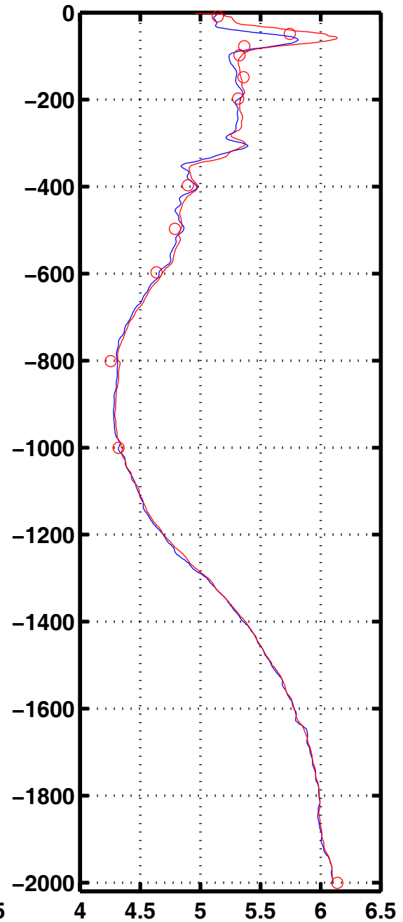
Oxyg 3033
