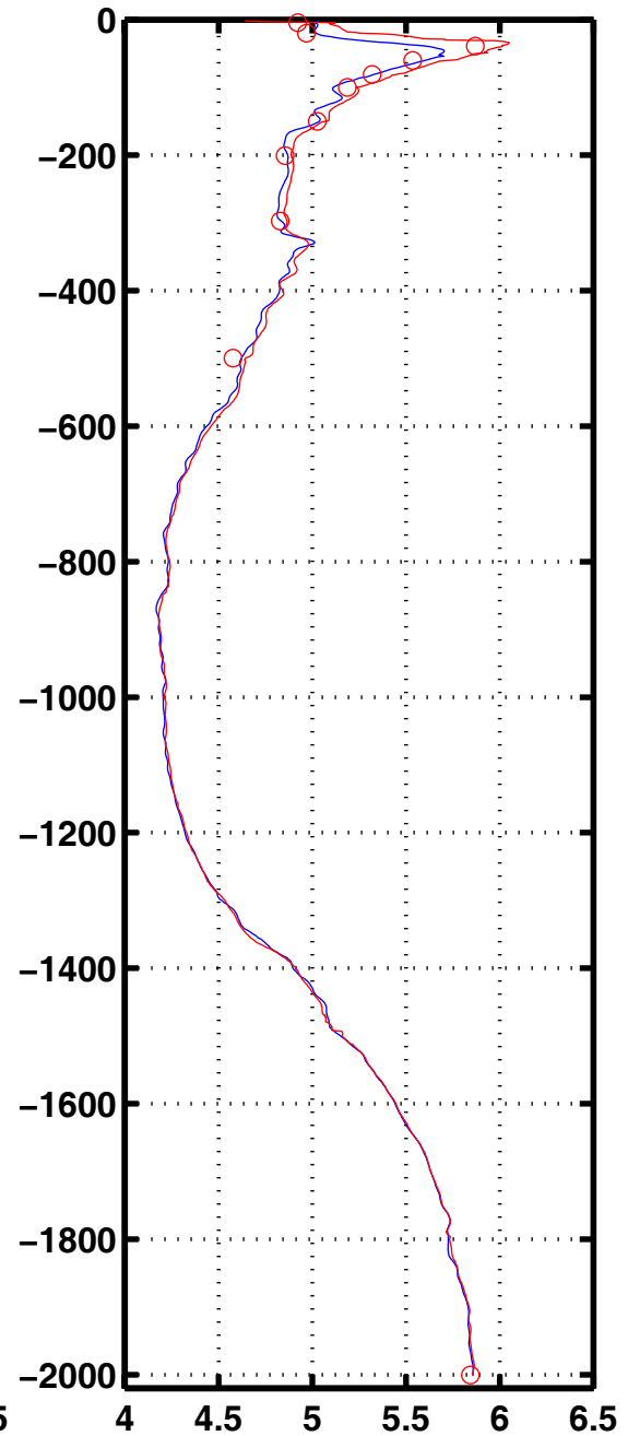
Oxyg 3011
