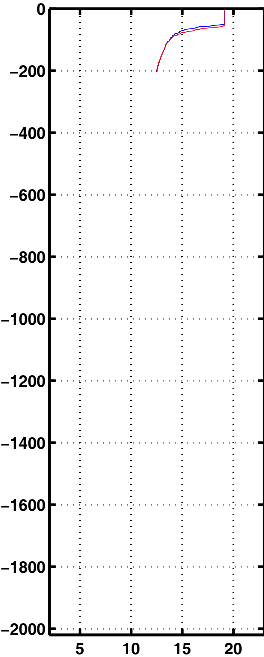
Tempe 3330
