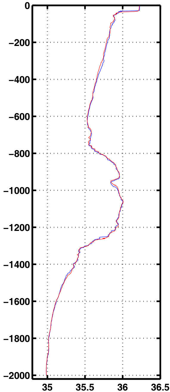
Sali 3041
