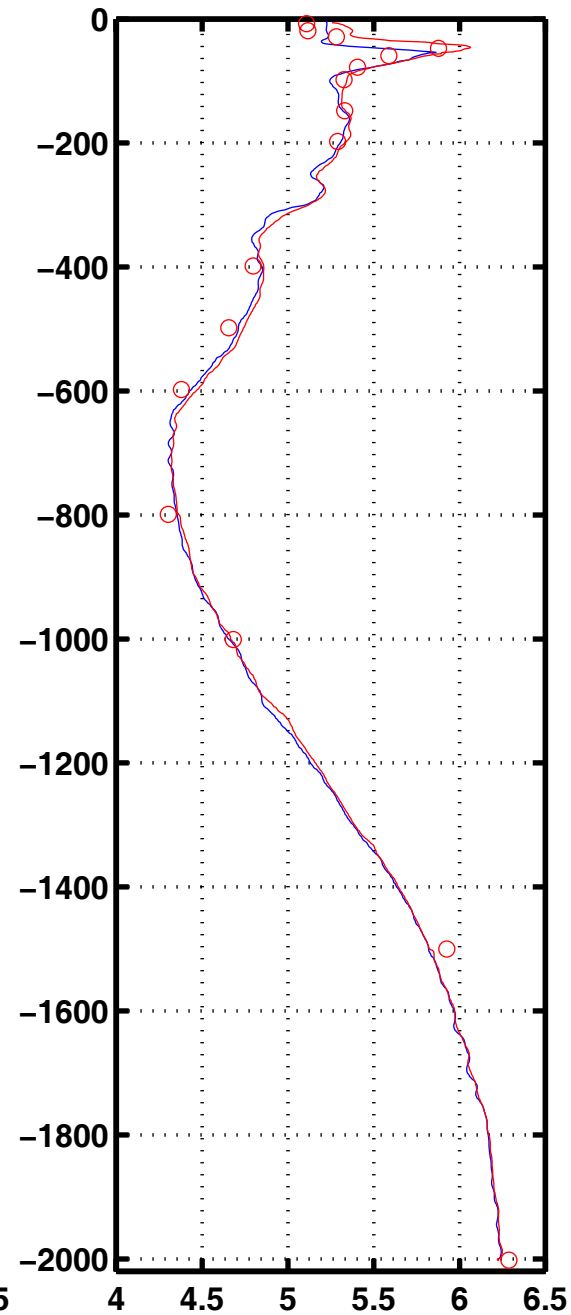
Oxyg 3072
