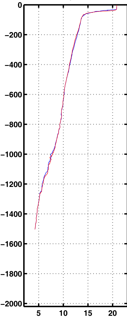
Tempe 3239
