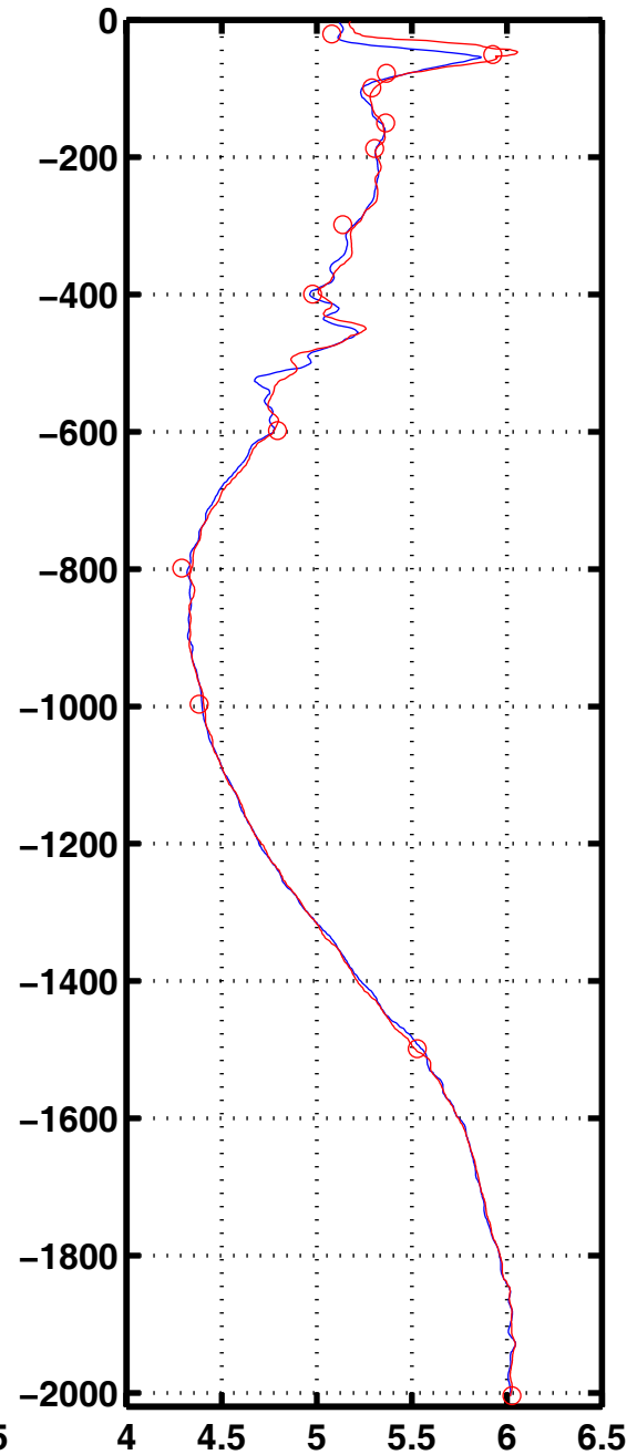
Oxyg 3034
