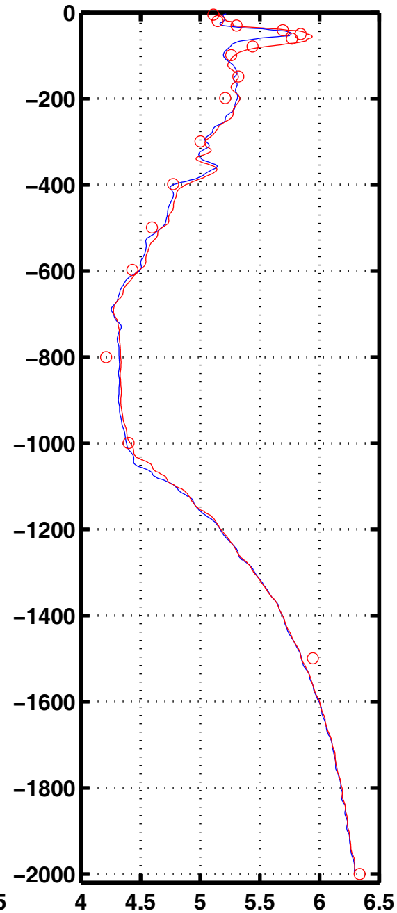
Oxyg 3061
