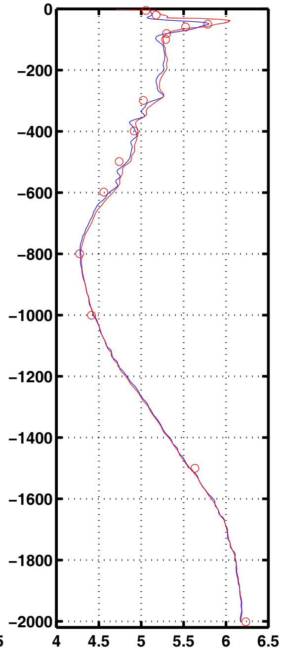
Oxyg 3056
