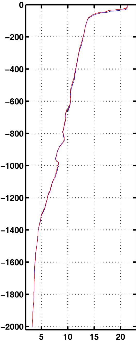
Tempe 3074
