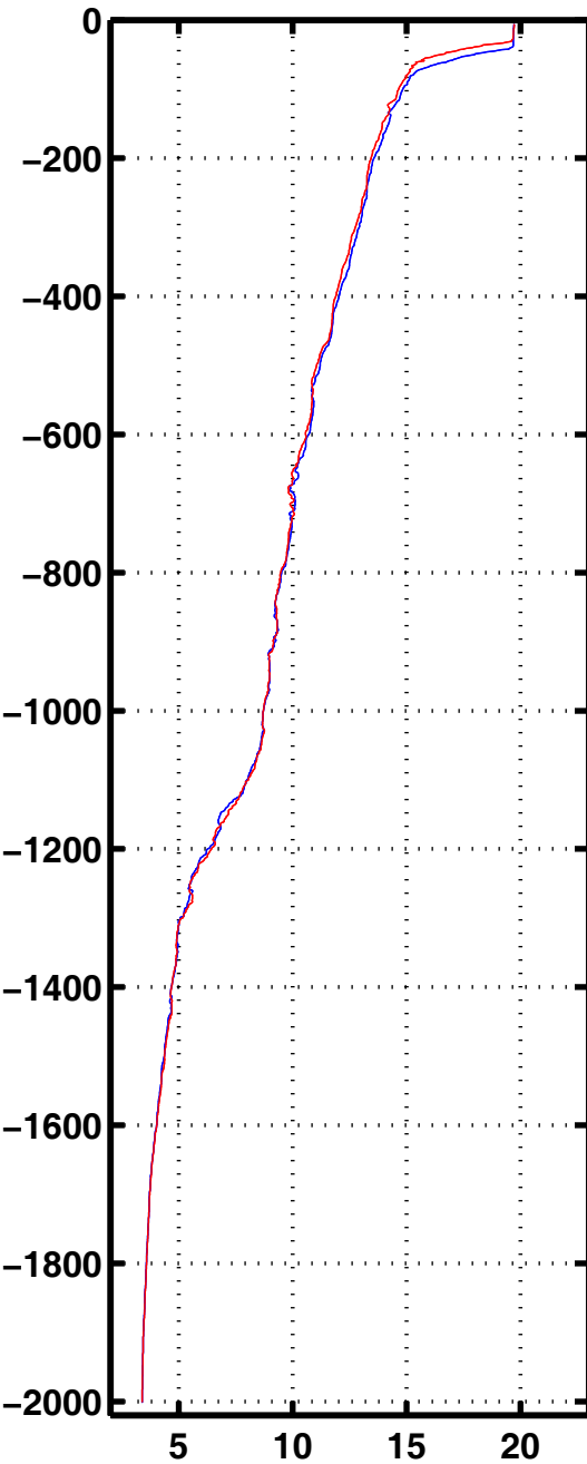
Tempe 3063
