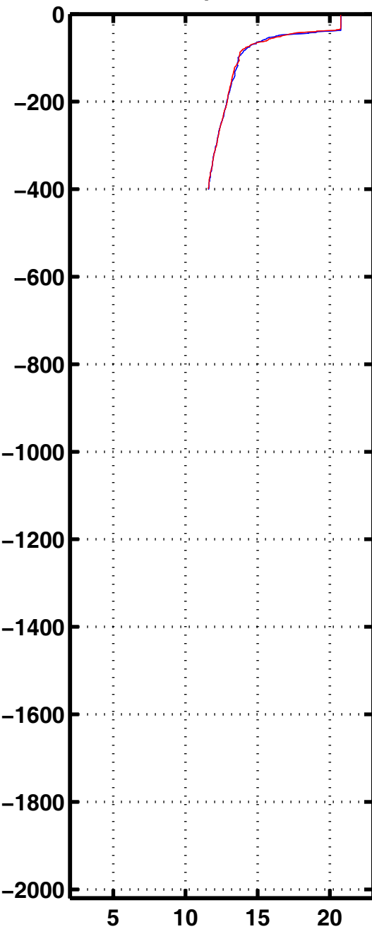
Tempe 3245
