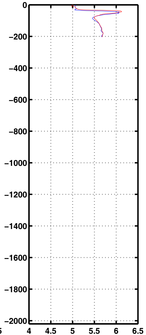
Oxyg 3096
