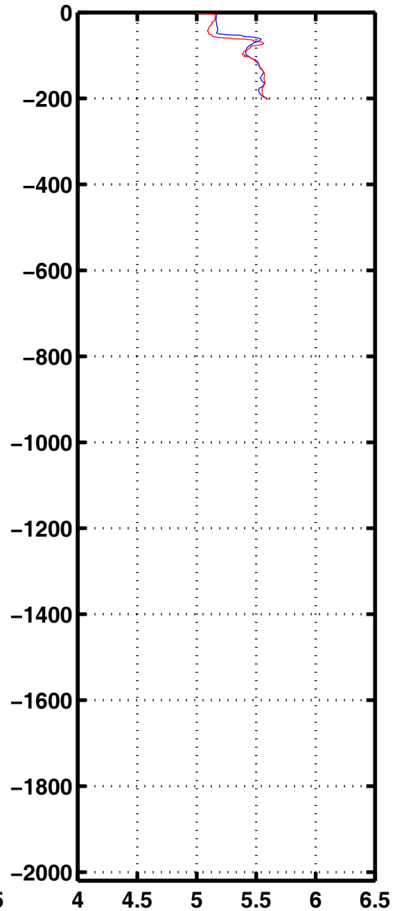
Oxyg 3330
