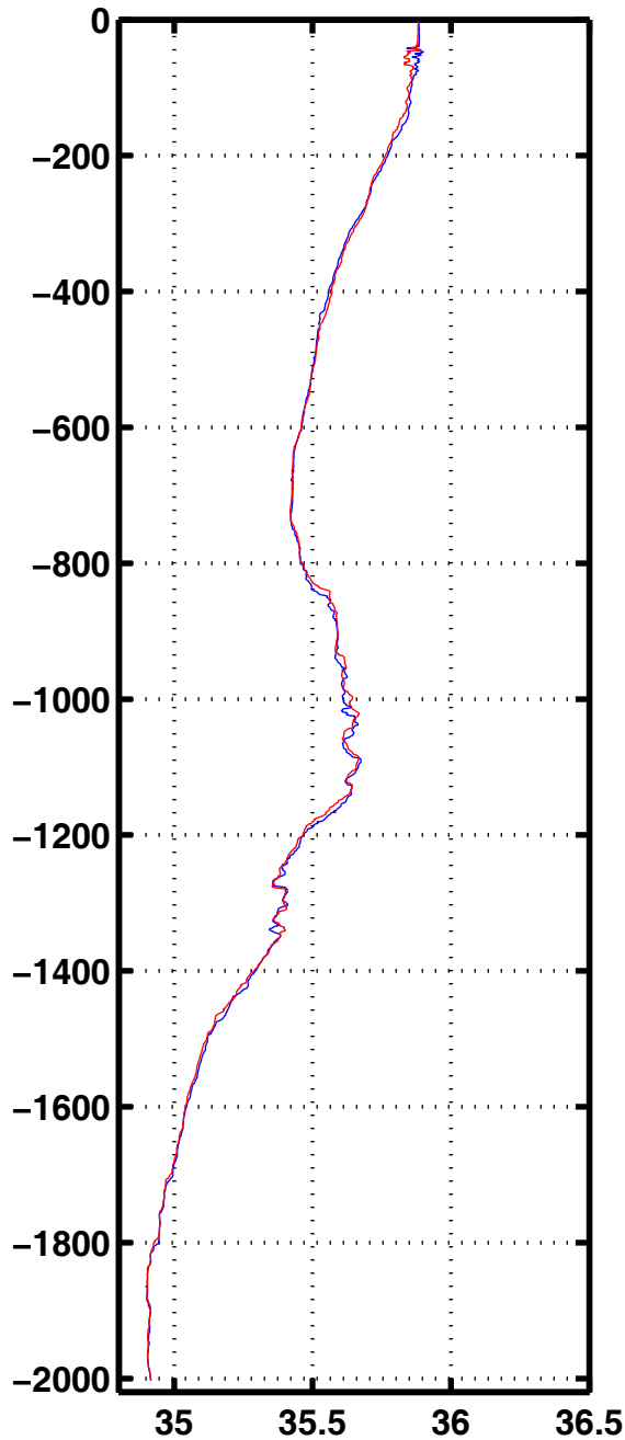
Sali 3060
