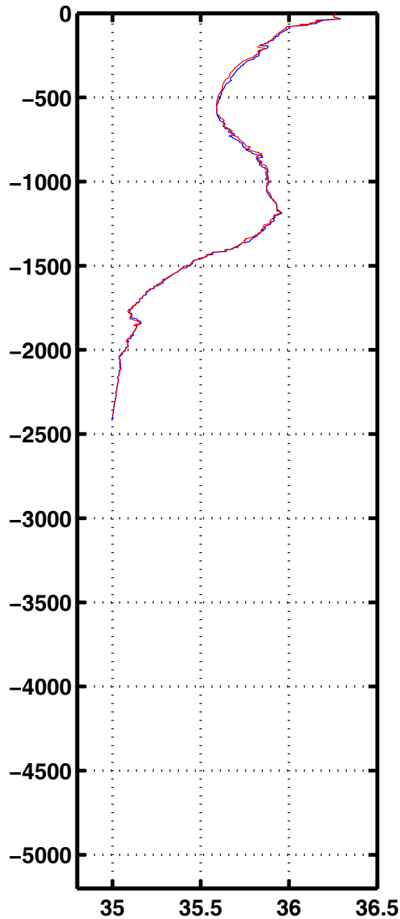
Sali 3013
