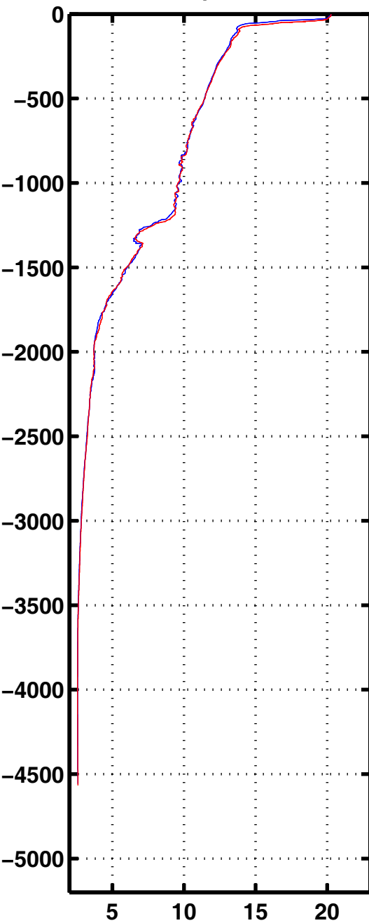
Tempe 3025
