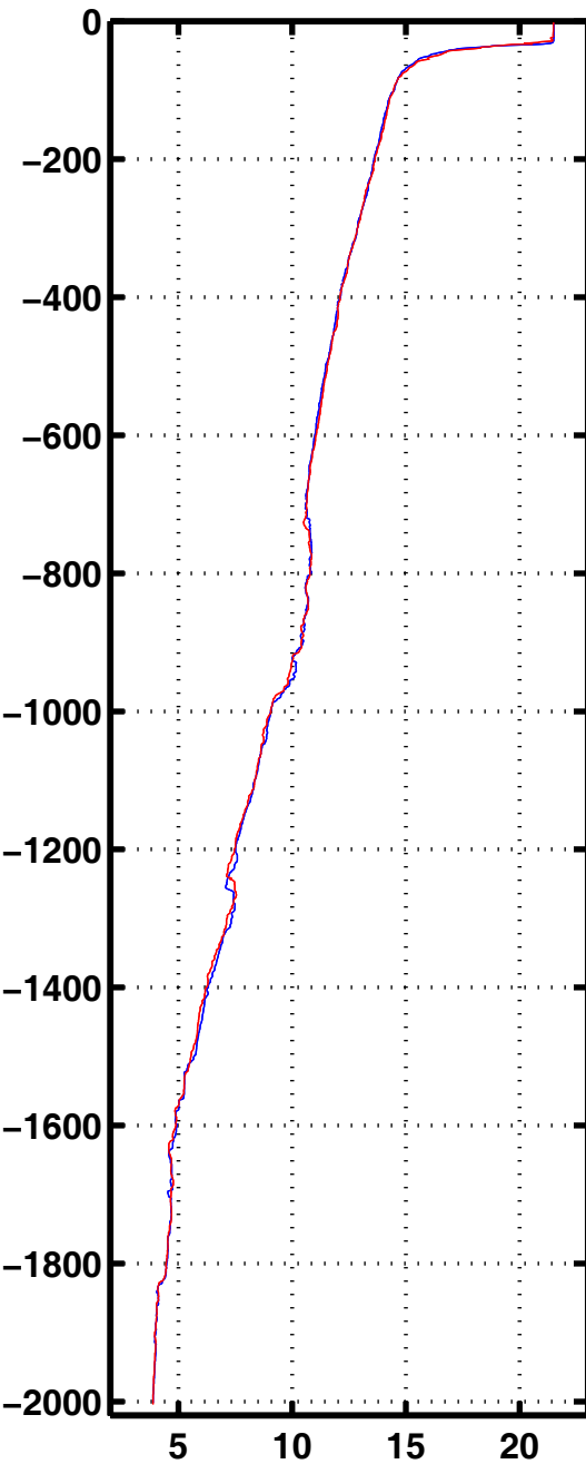
Tempe 3047
