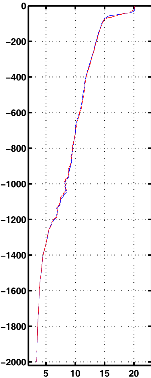
Tempe 3062
