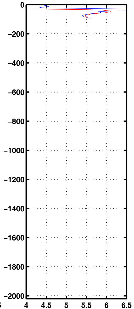
Oxyg 3090
