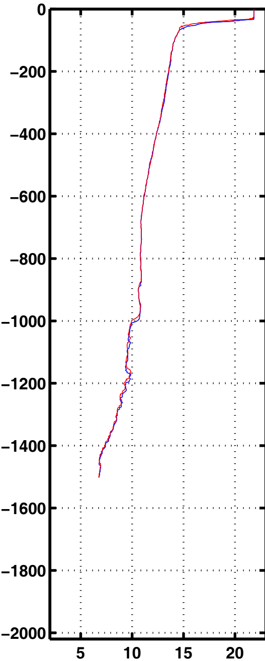
Tempe 3085
