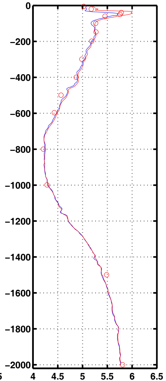
Oxyg 3083
