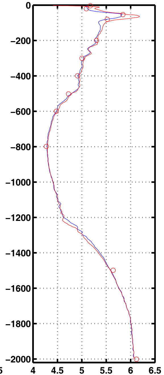
Oxyg 3016
