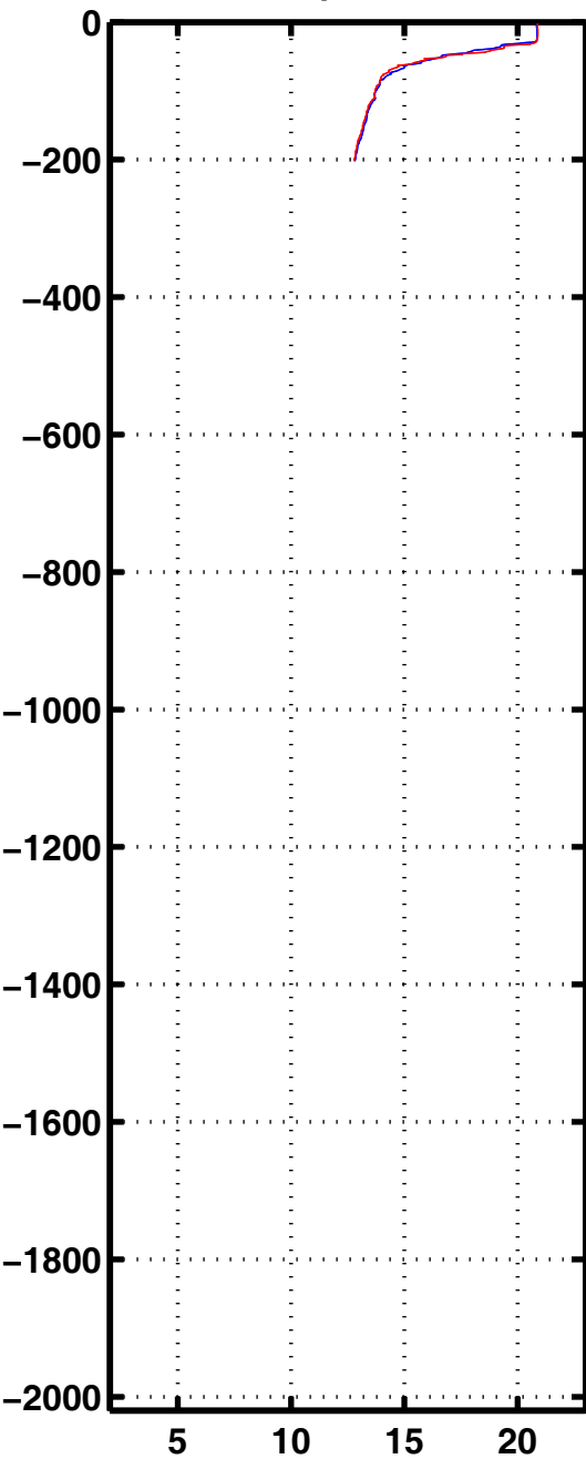
Tempe 3246
