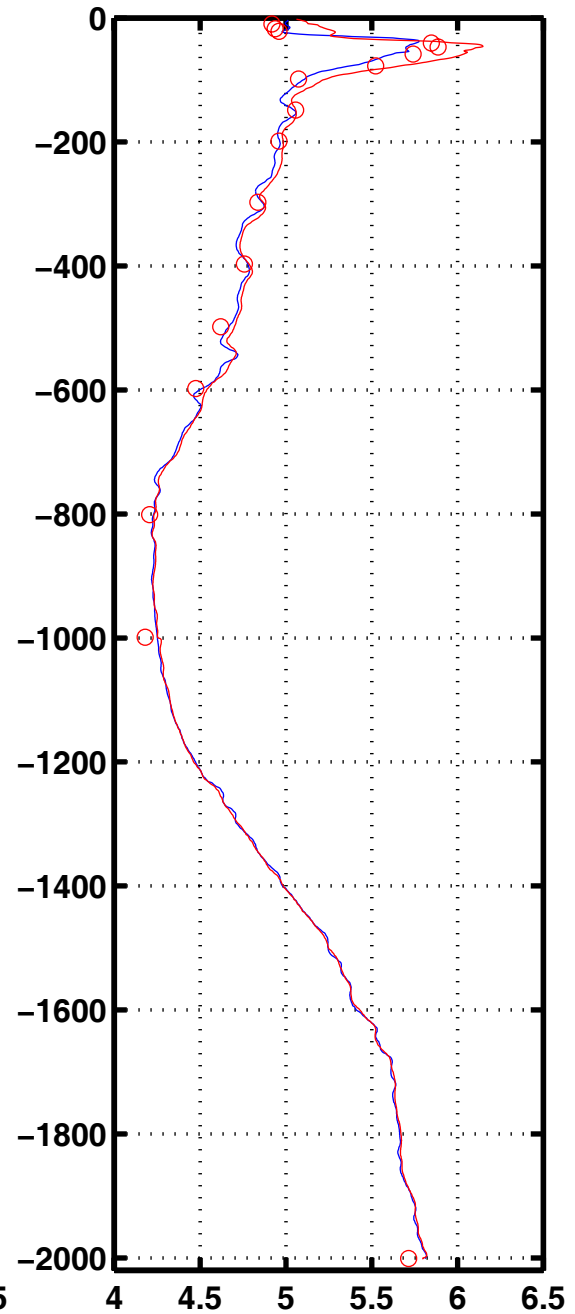
Oxyg 3038
