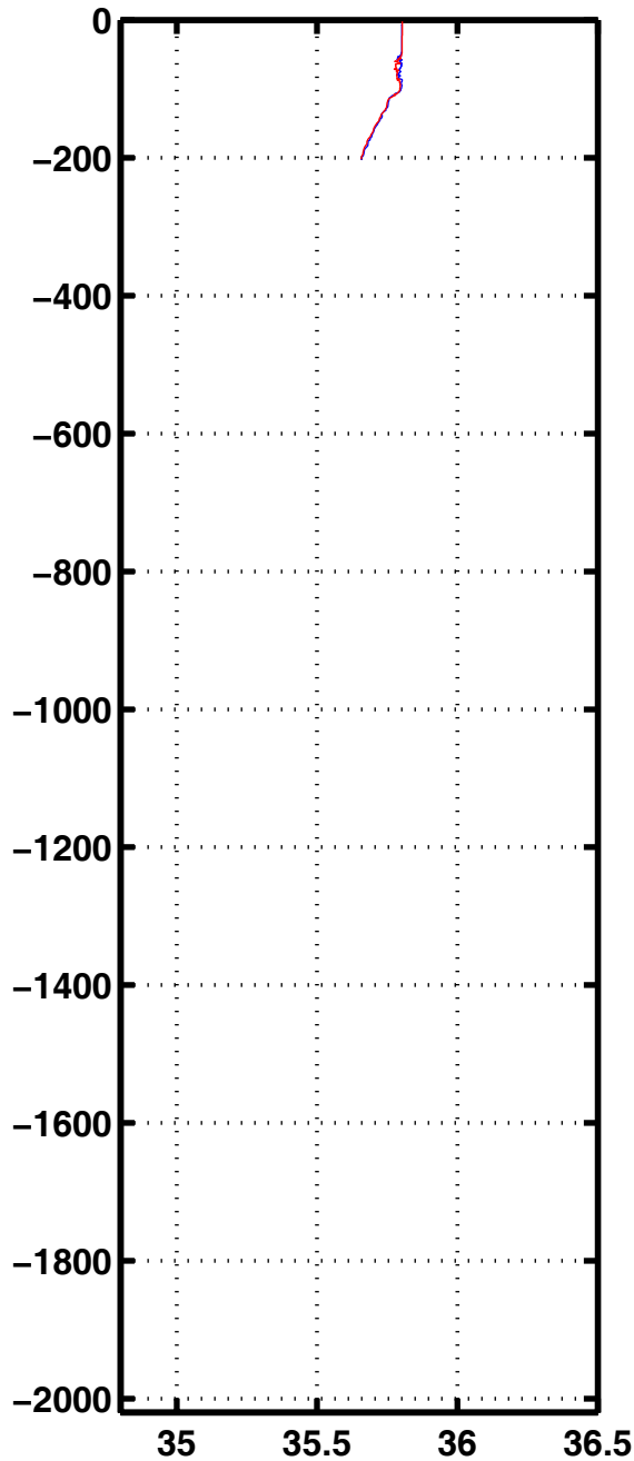
Sali 3330
