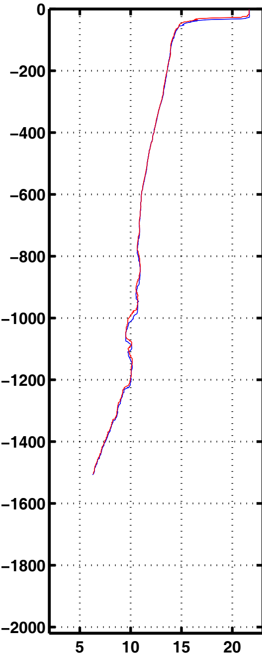
Tempe 3098
