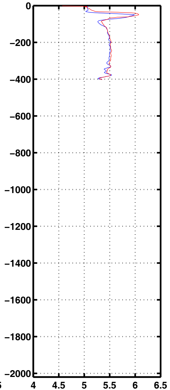
Oxyg 3092
