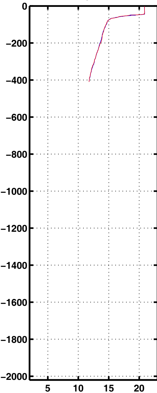
Tempe 3161
