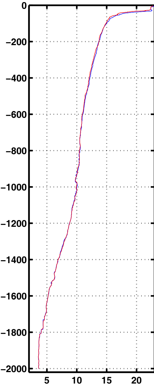
Tempe 3079
