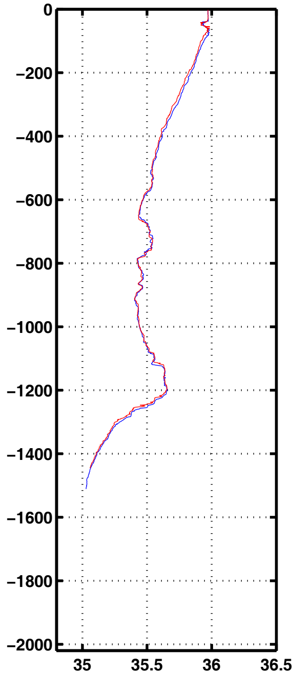
Sali 3157
