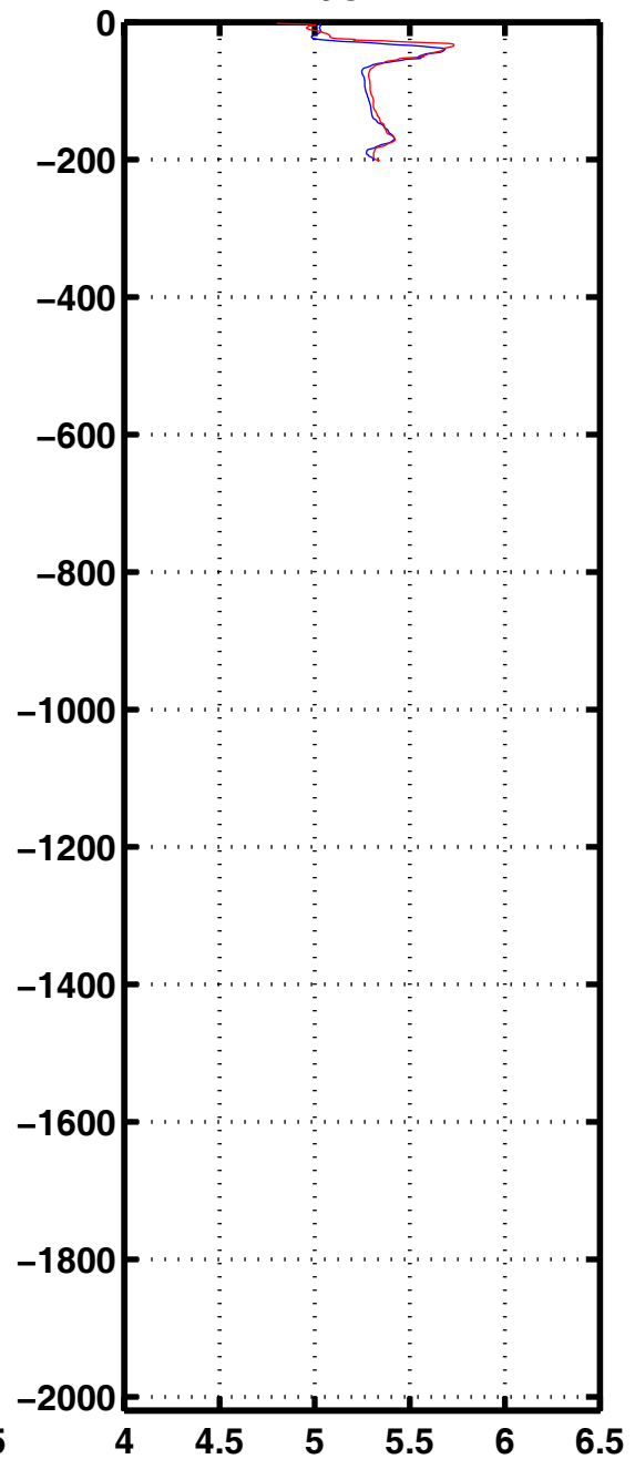
Oxyg 3156
