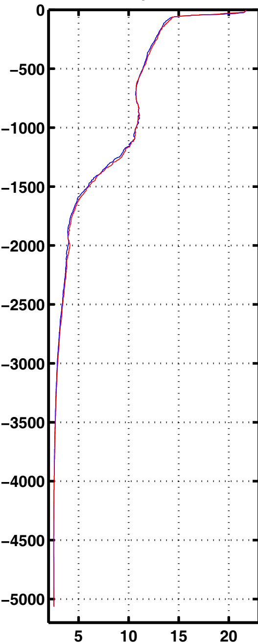
Tempe 3006
