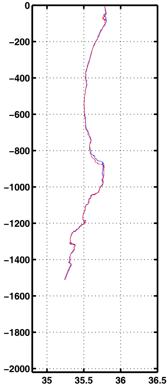
Sali 3327
