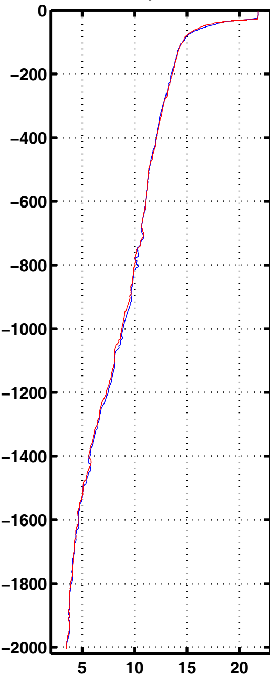
Tempe 3045
