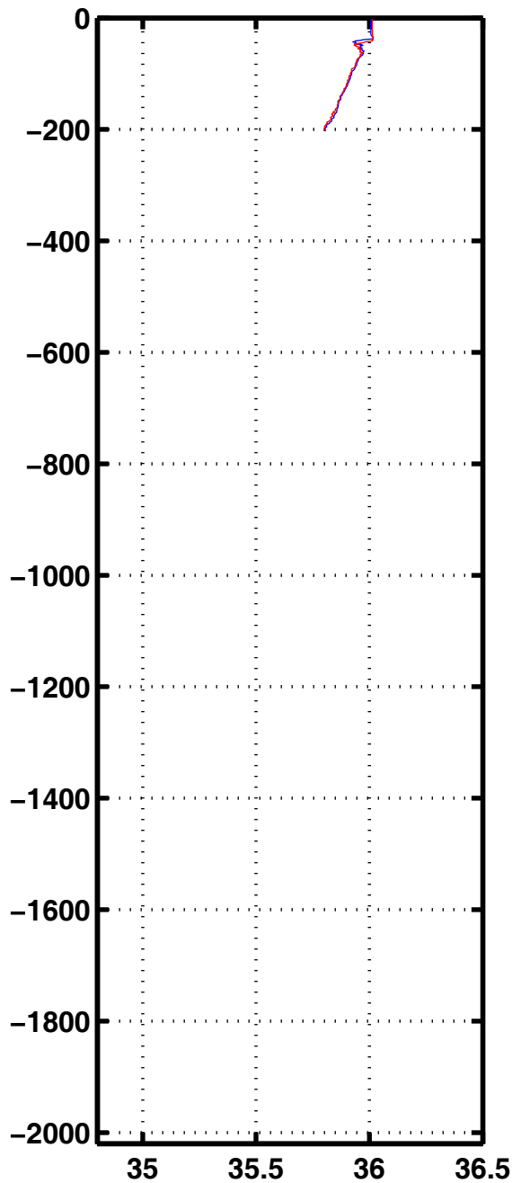
Sali 3162
