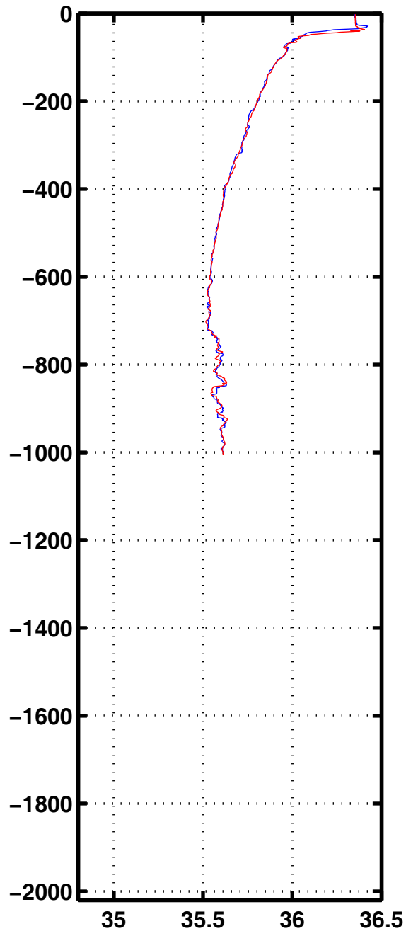
Sali 3084
