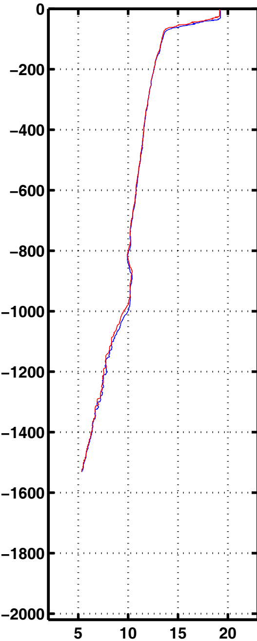
Tempe 3335
