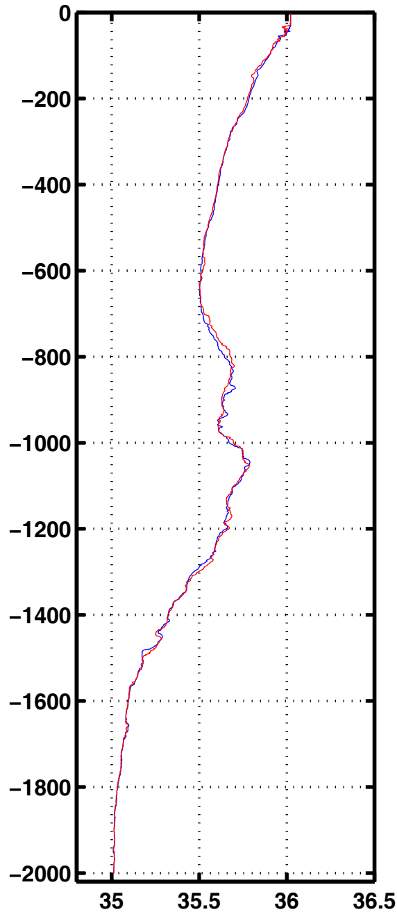
Sali 3035
