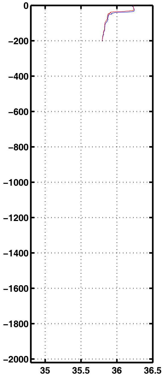
Sali 3096
