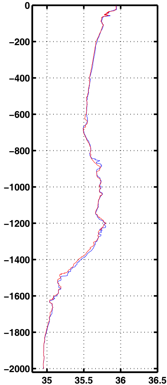
Sali 3017
