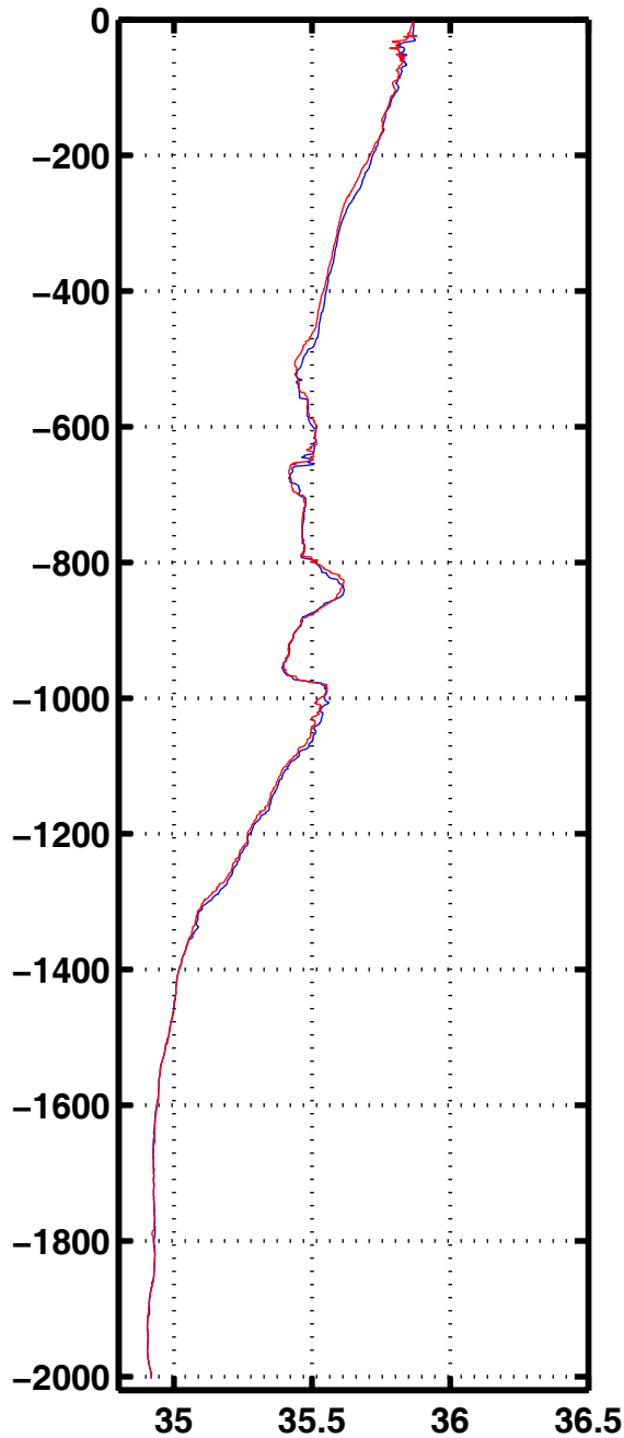
Sali 3074
