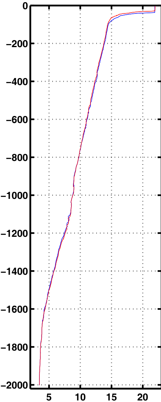
Tempe 3056
