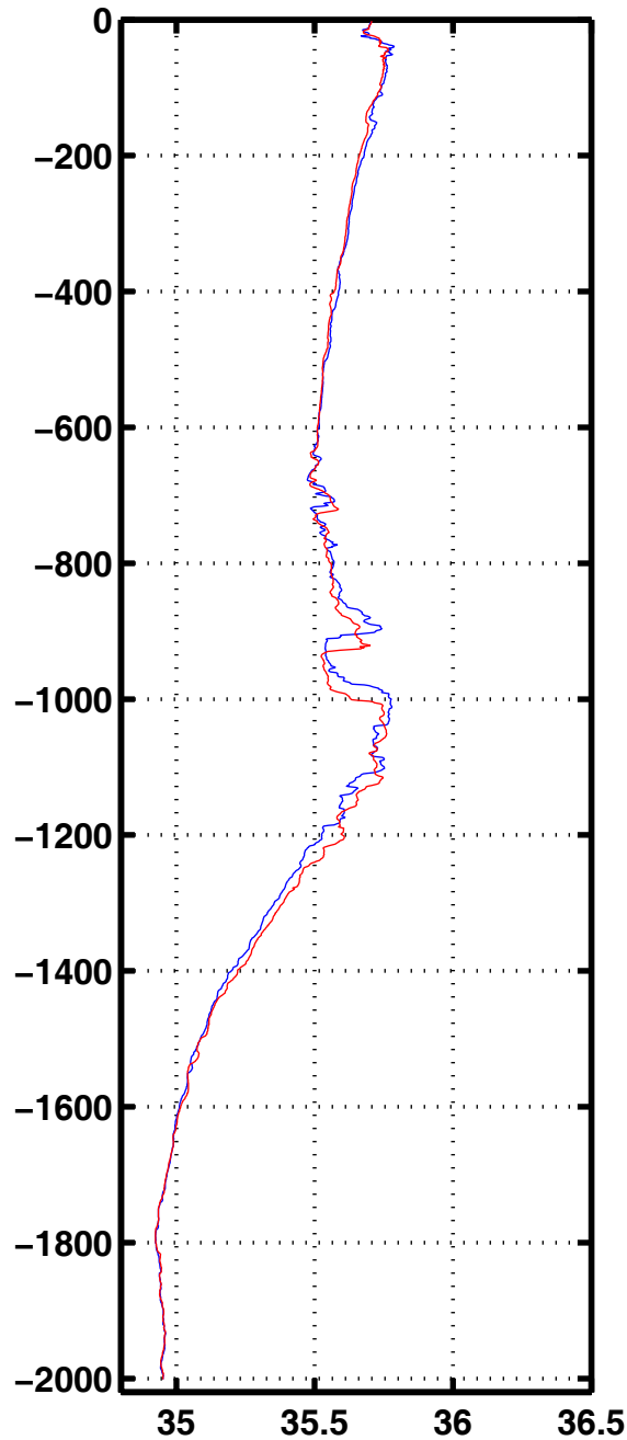
Sali 3029
