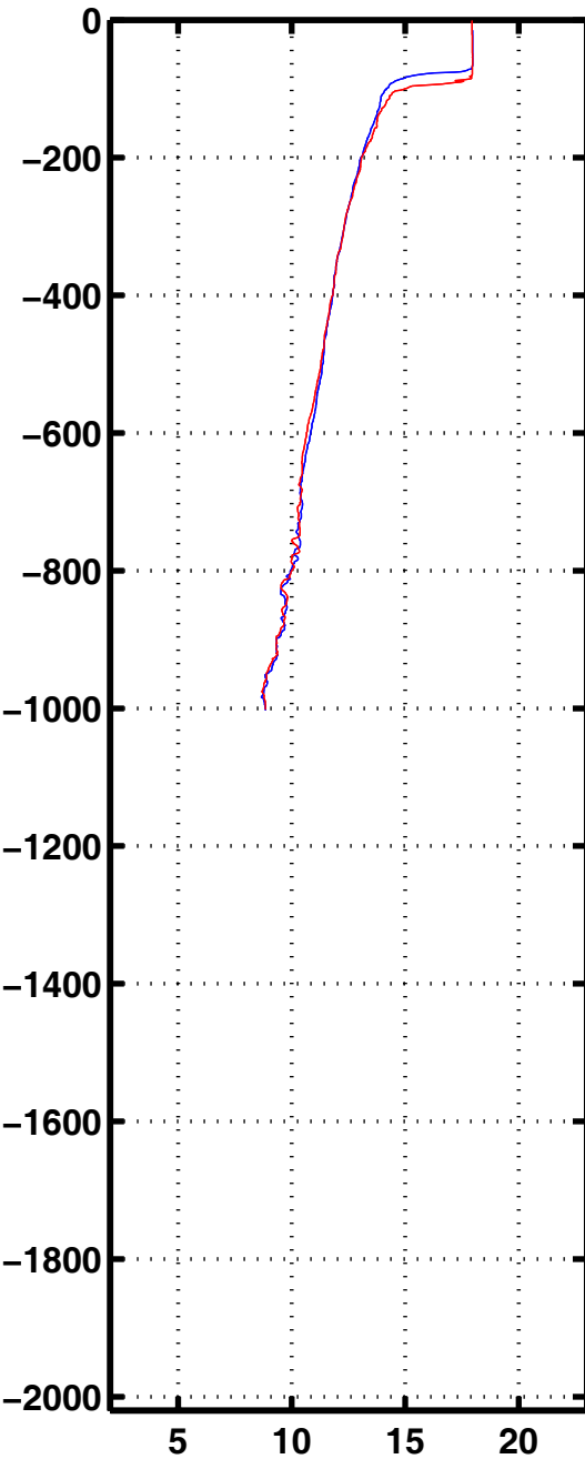
Tempe 3338
