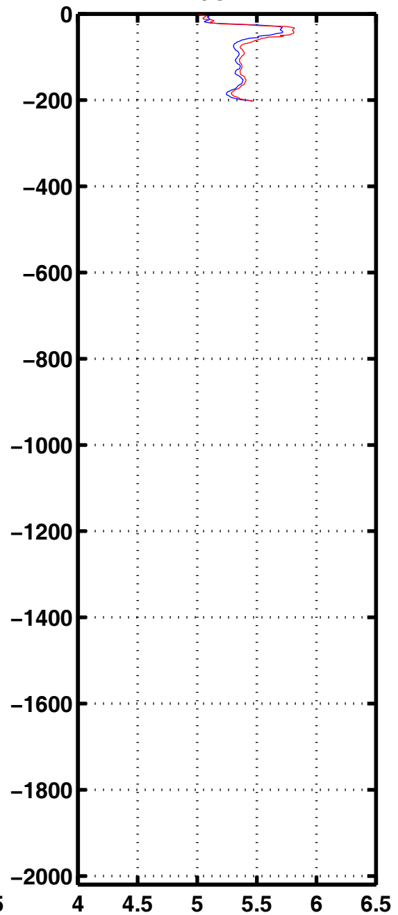
Oxyg 3165
