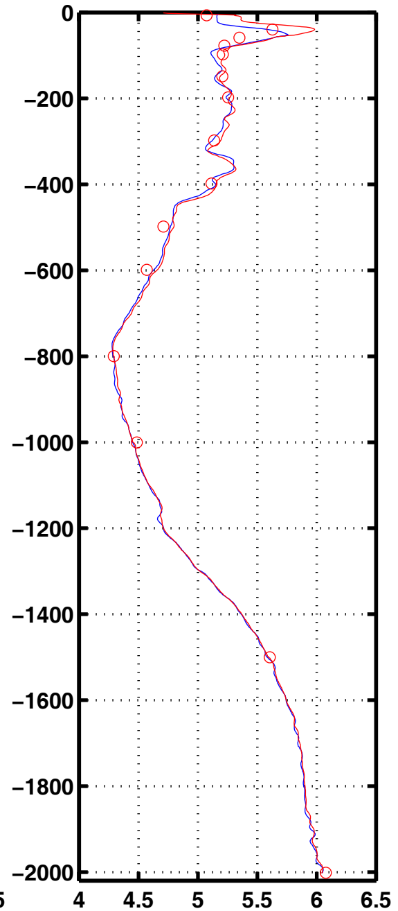
Oxyg 3077
