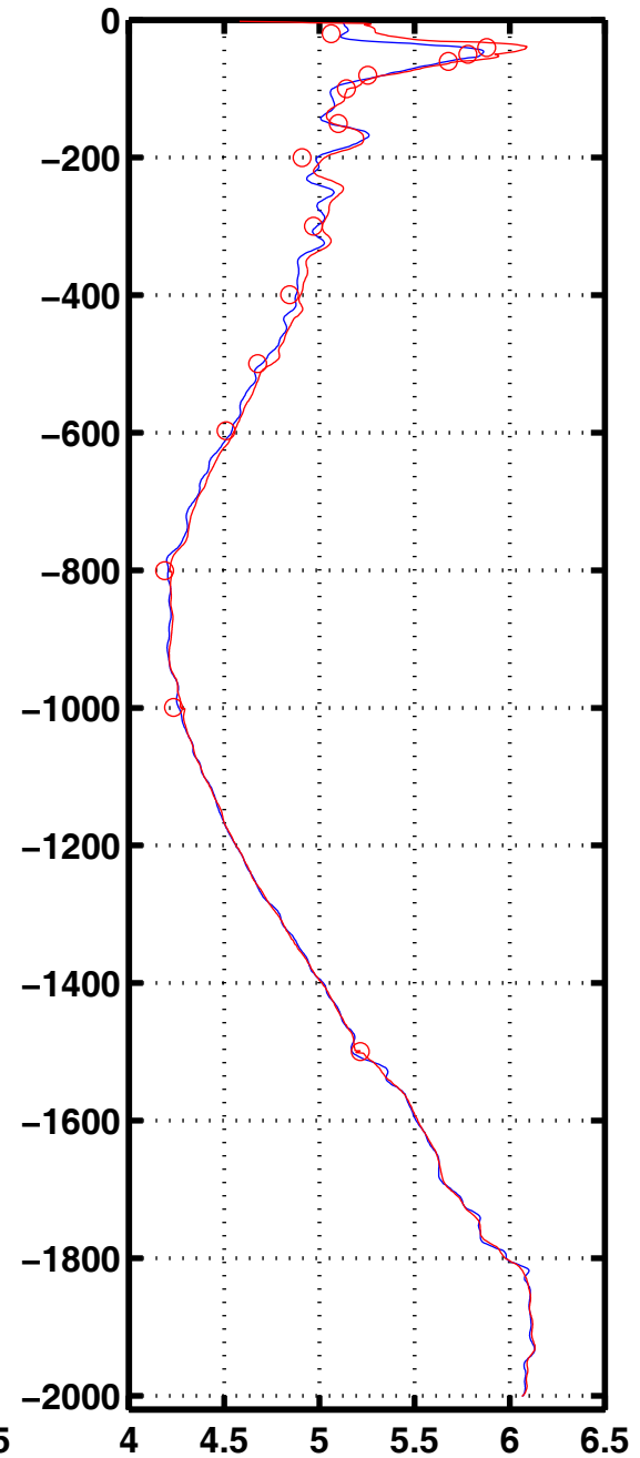
Oxyg 3079
