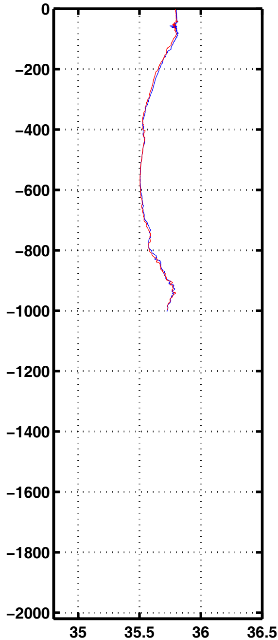
Sali 3326
