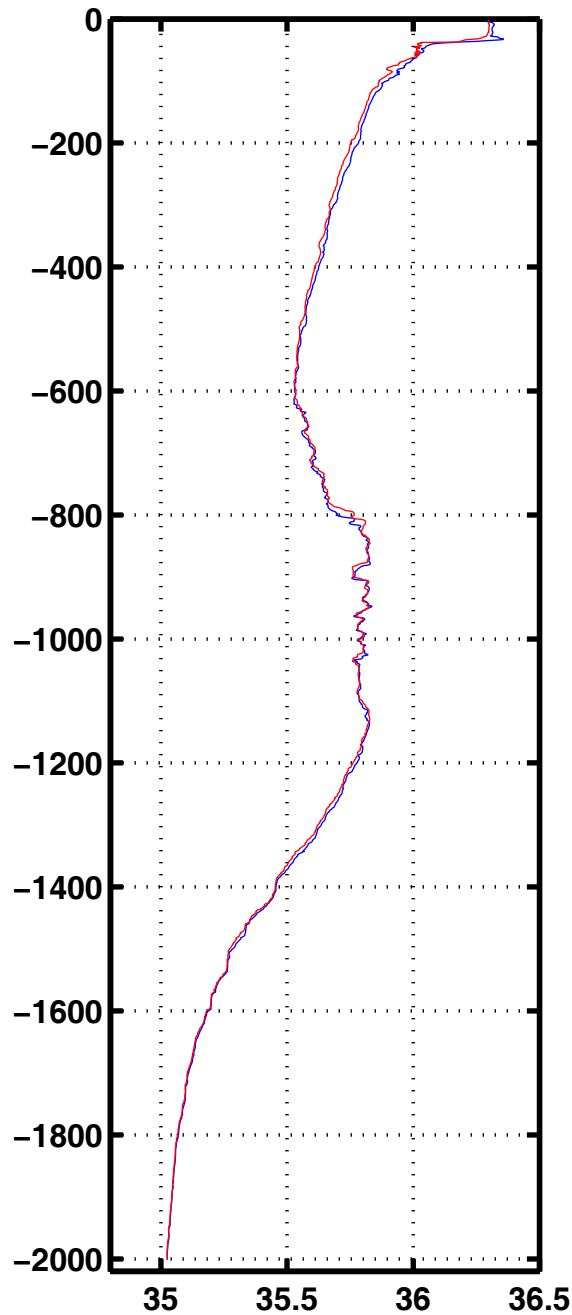
Sali 3082
