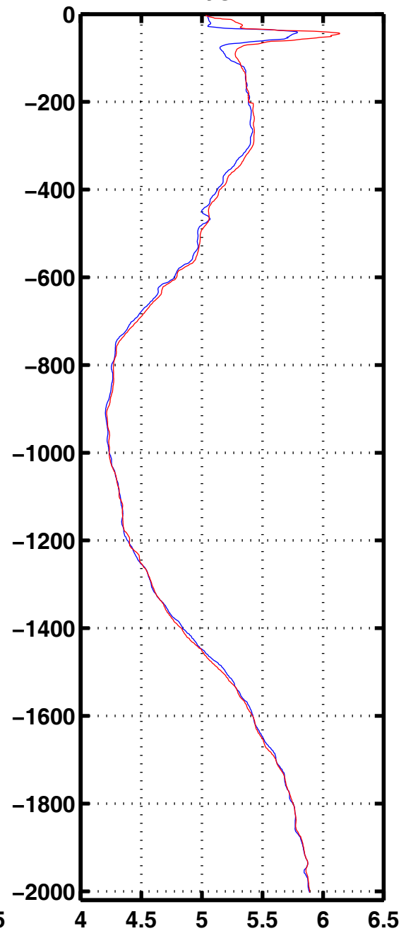
Oxyg 3099
