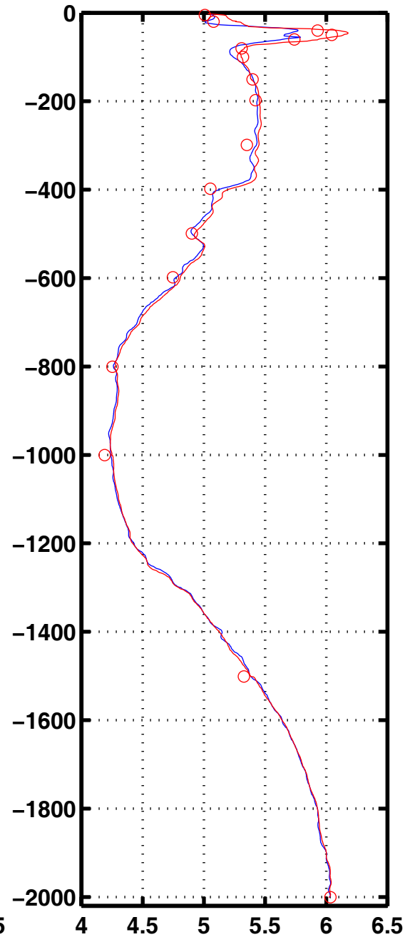
Oxyg 3041
