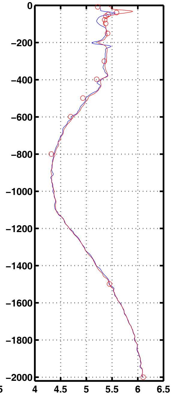
Oxyg 3022
