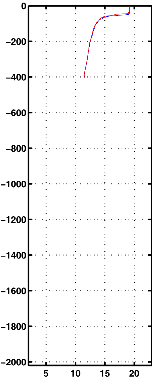
Tempe 3329
