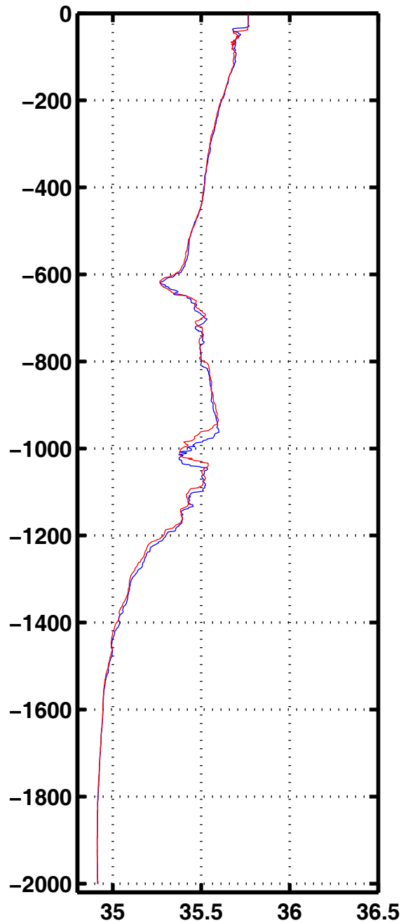
Sali 3066
