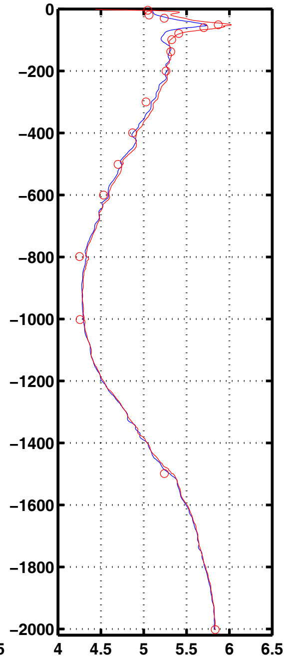
Oxyg 3018
