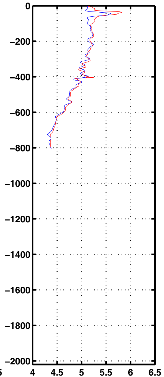
Oxyg 3164
