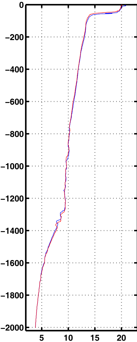
Tempe 3023
