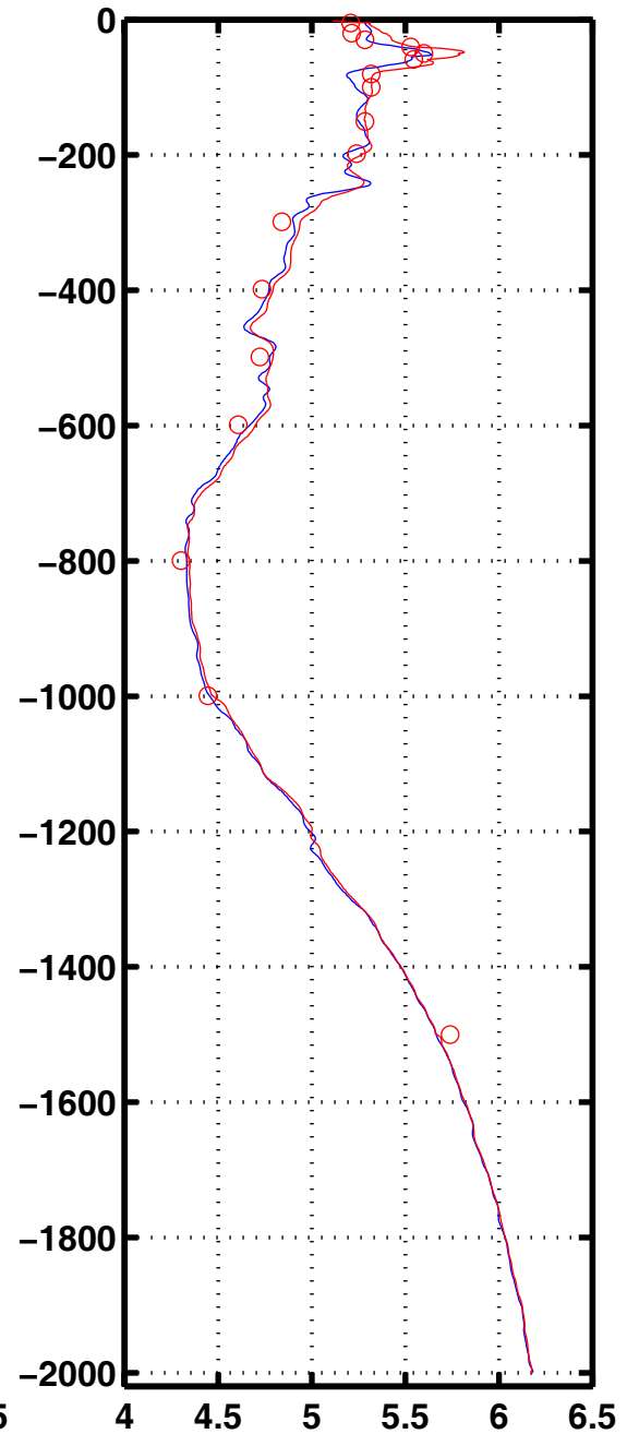
Oxyg 3064
