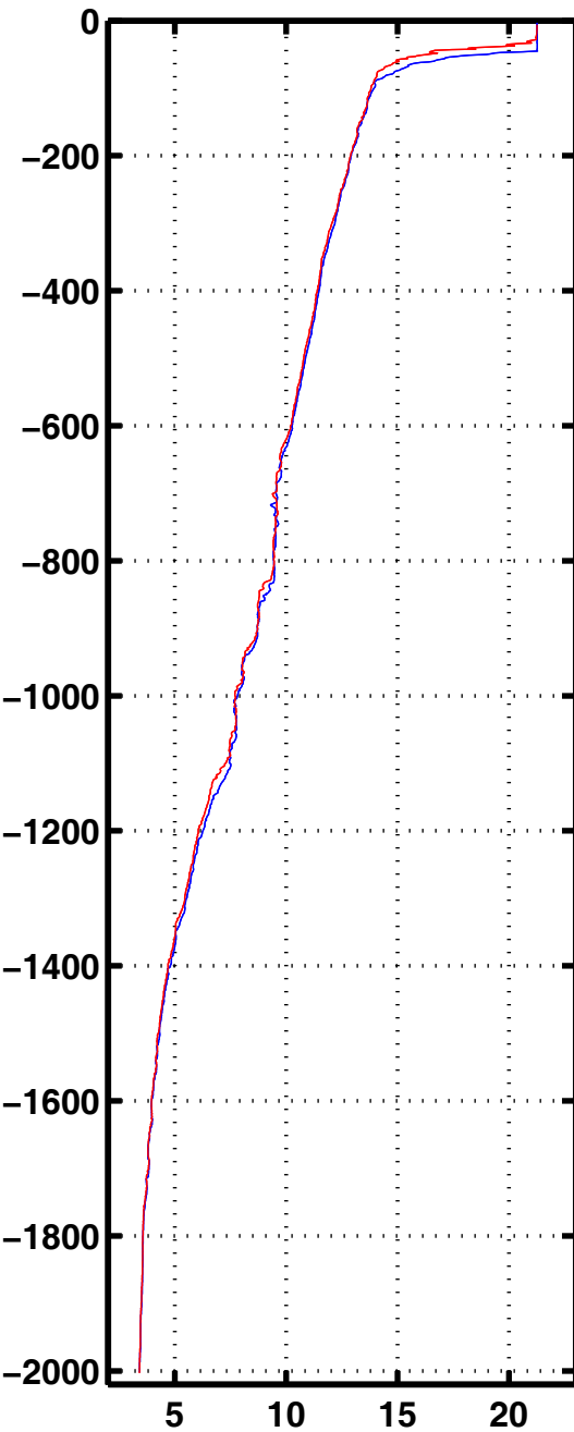
Tempe 3072
