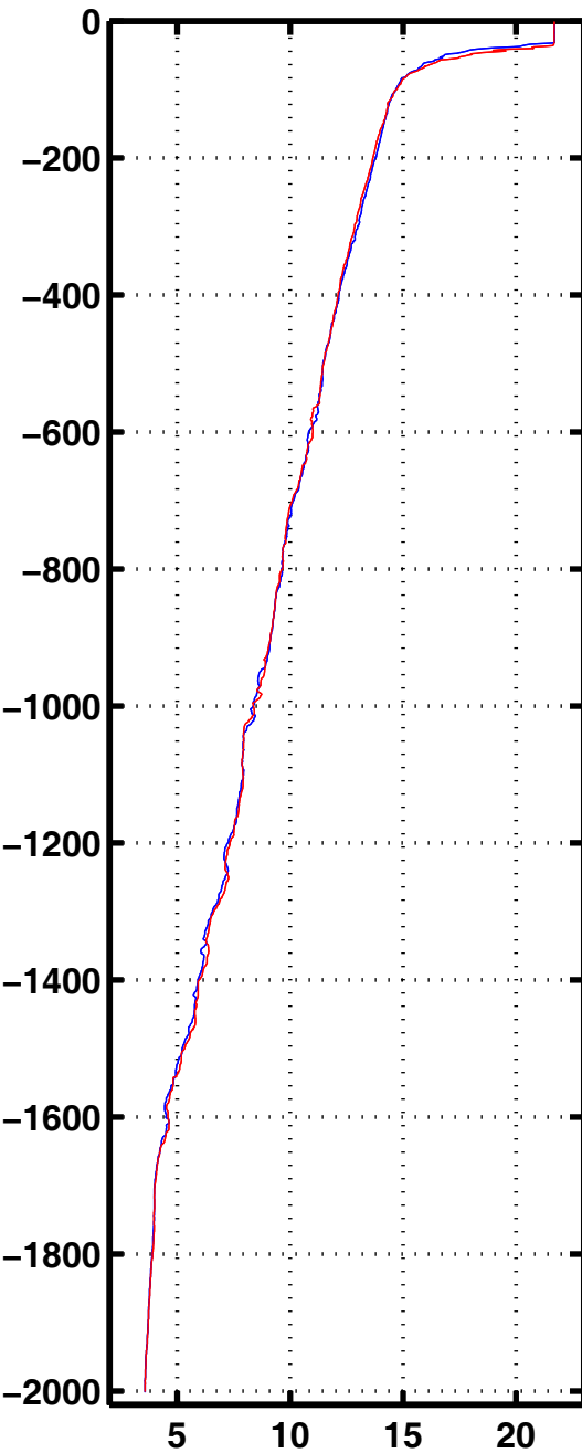
Tempe 3055
