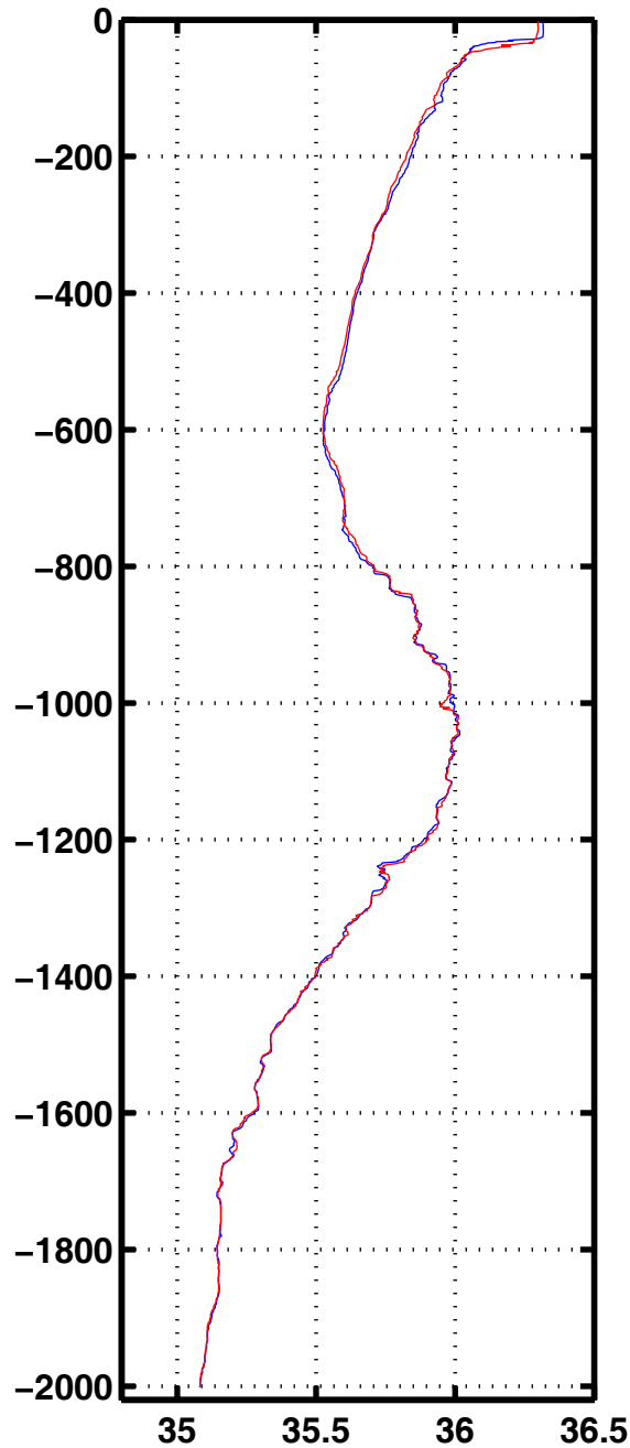
Sali 3038
