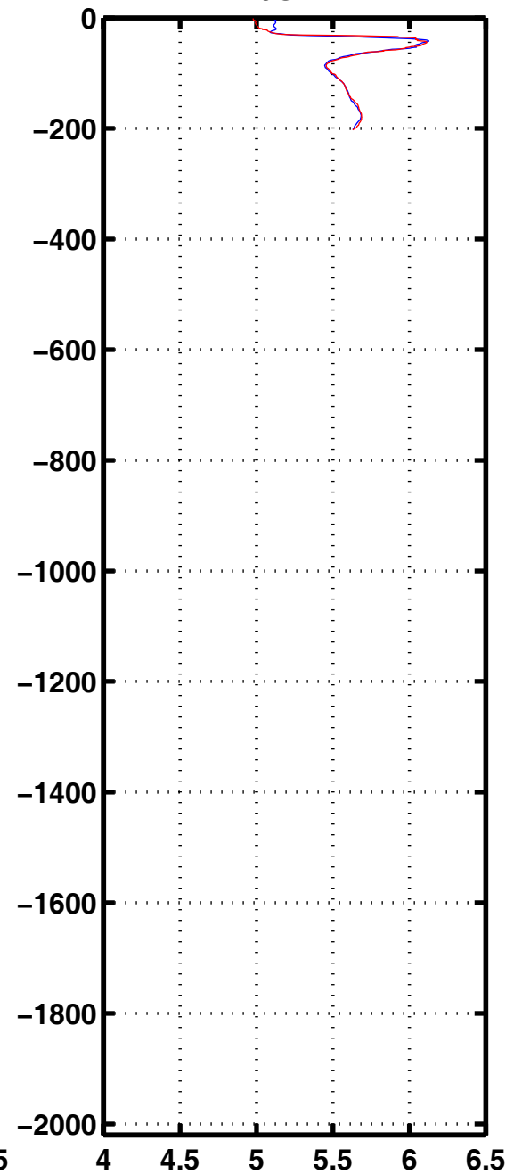
Oxyg 3094
