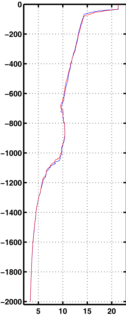
Tempe 3061
