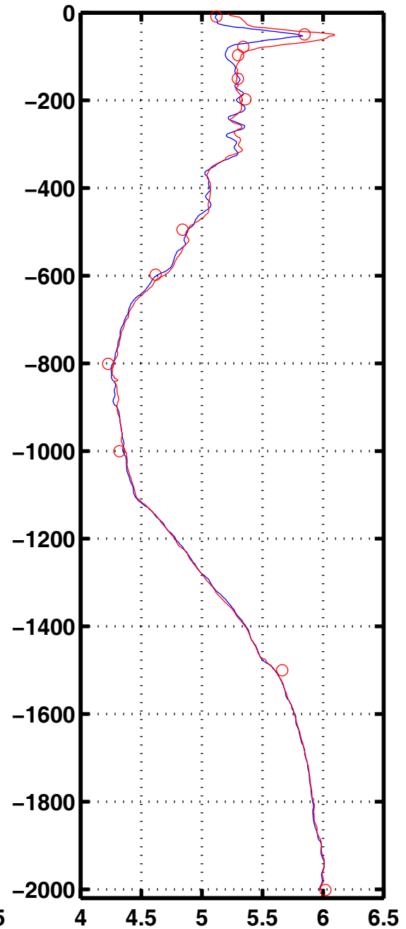
Oxyg 3015
