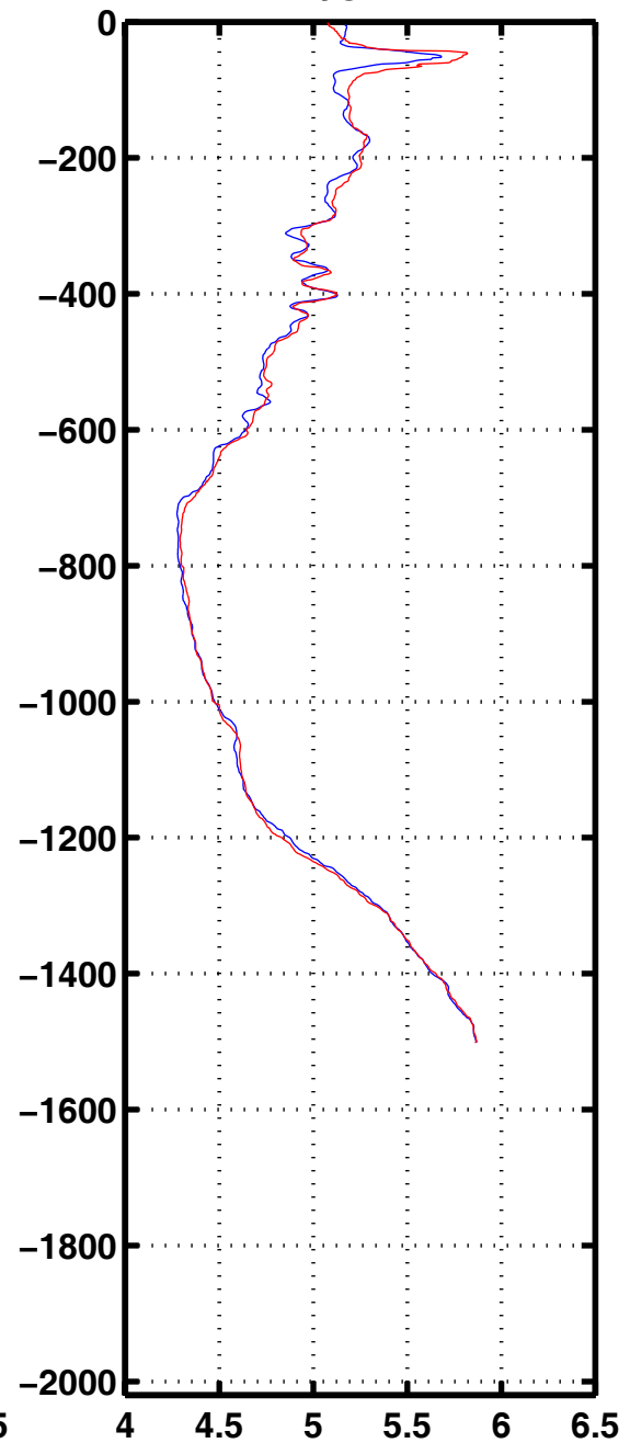
Oxyg 3167
