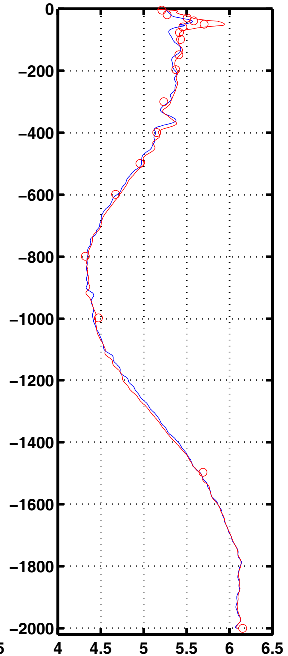
Oxyg 3029
