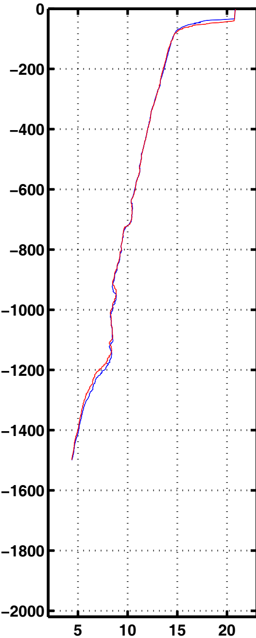
Tempe 3166
