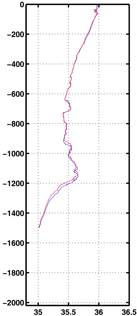
Sali 3166
