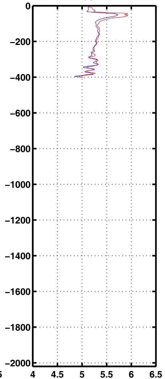
Oxyg 3245
