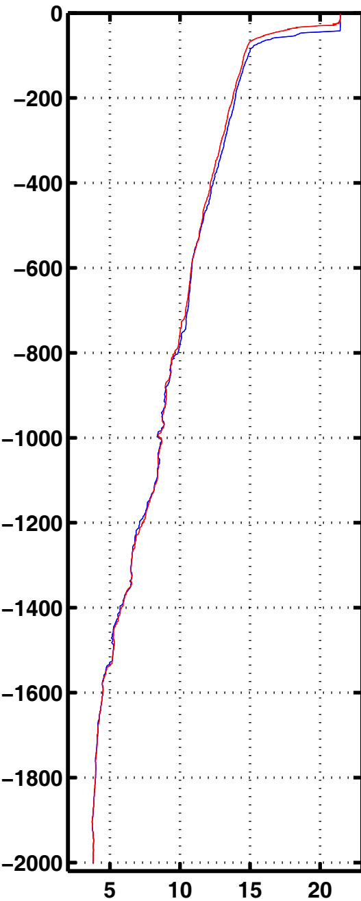
Tempe 3054
