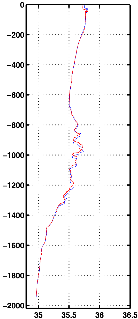
Sali 3049
