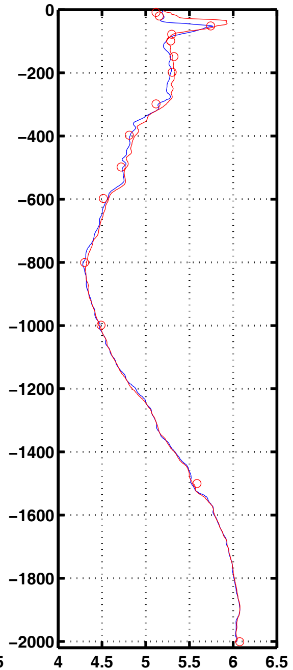
Oxyg 3054
