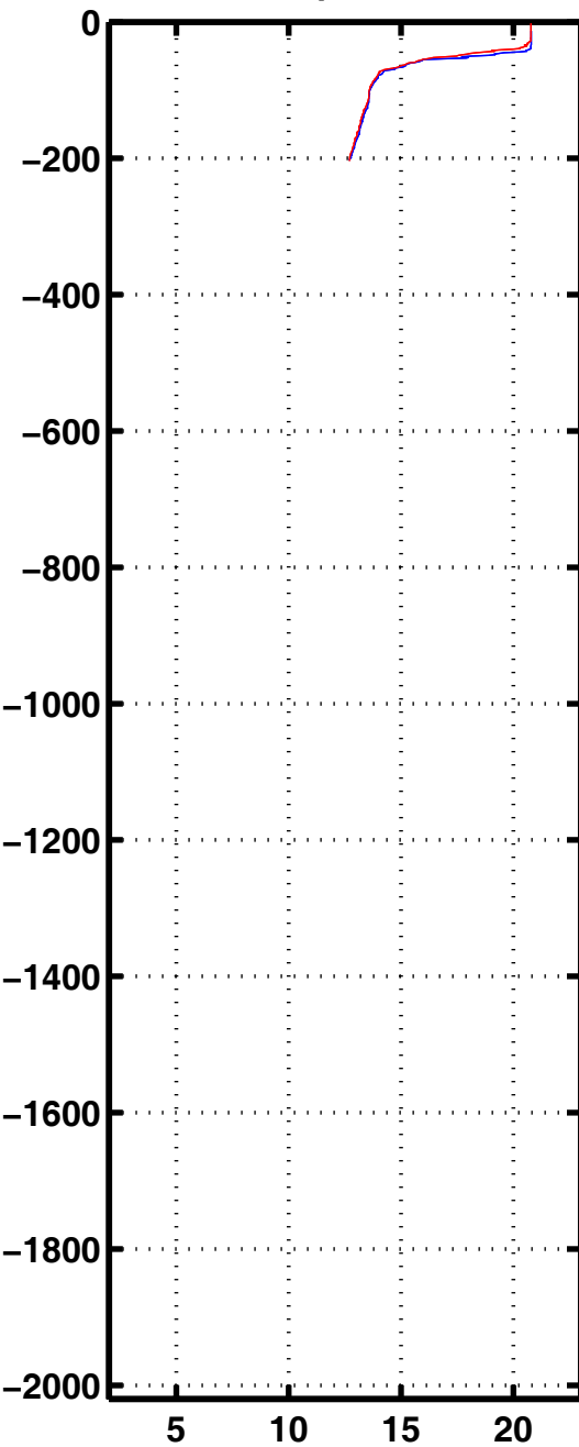
Tempe 3240
