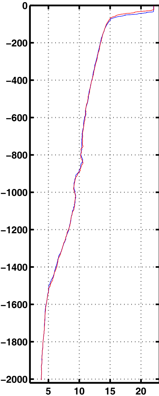
Tempe 3034
