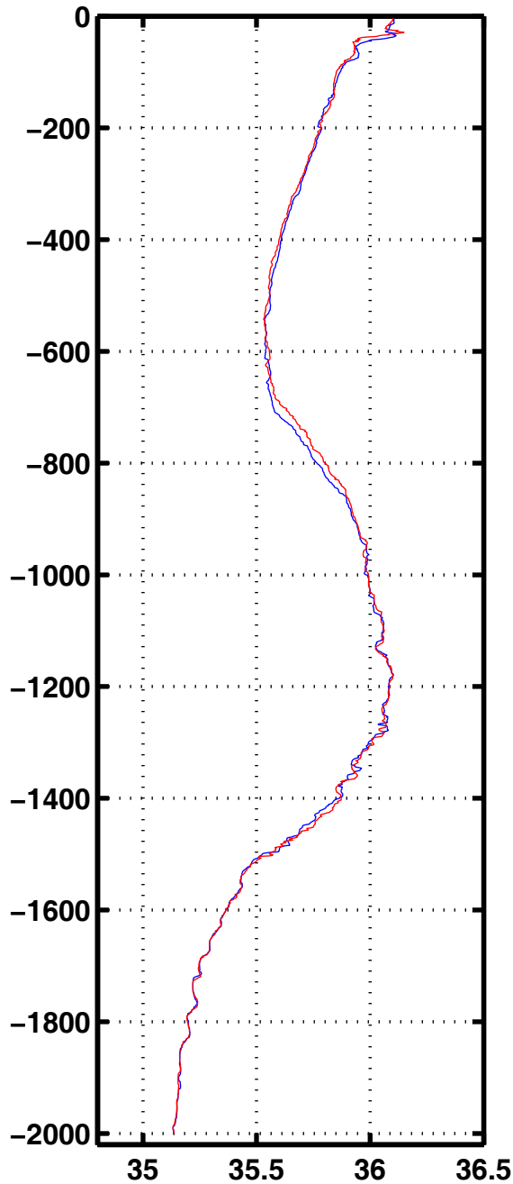
Sali 3012
