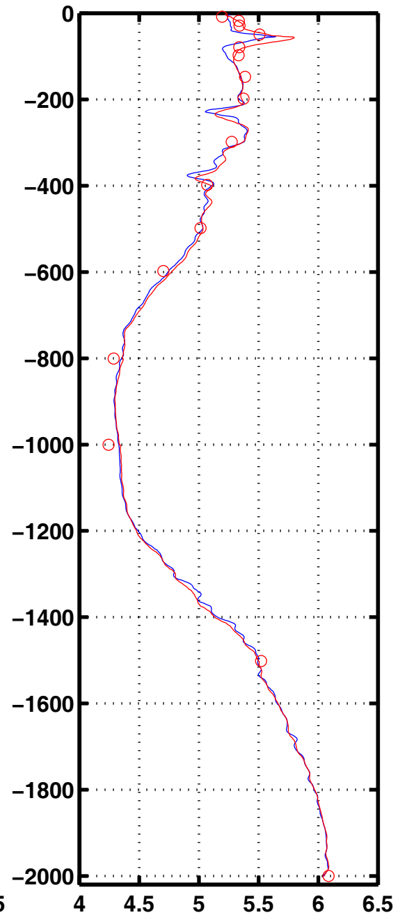
Oxyg 3024
