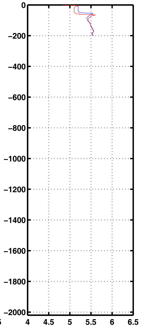
Oxyg 3324
