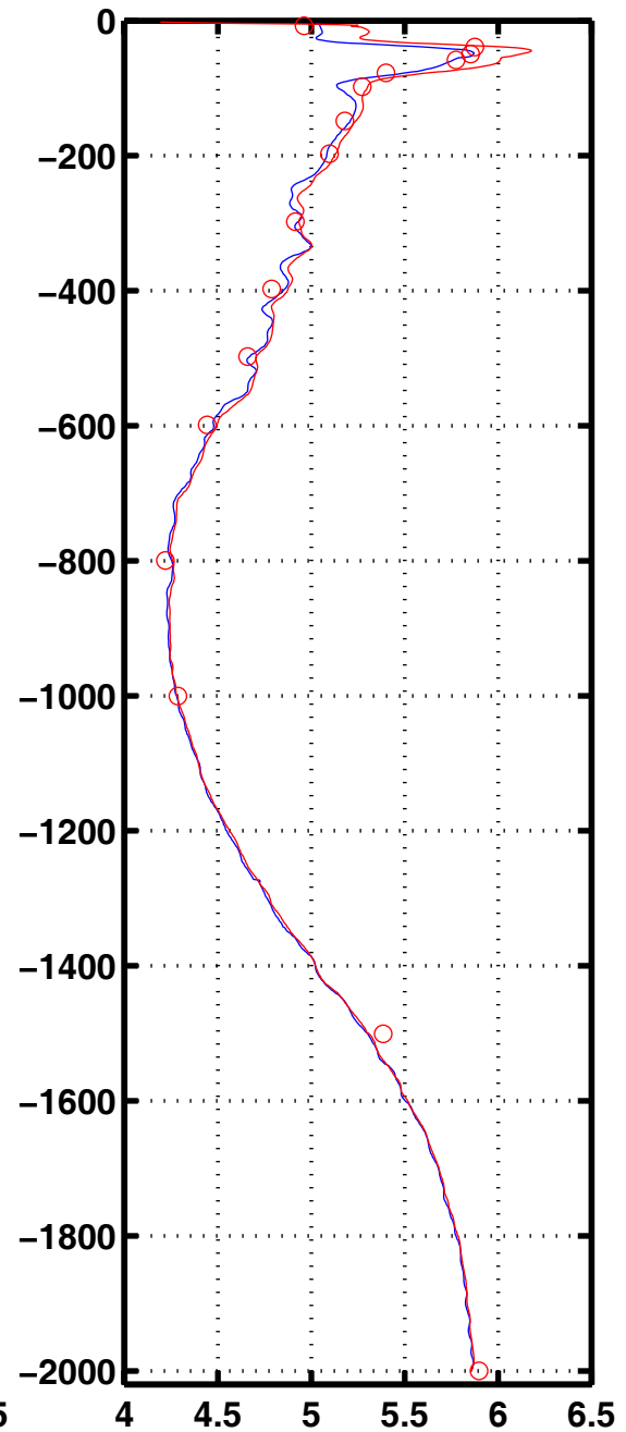
Oxyg 3082
