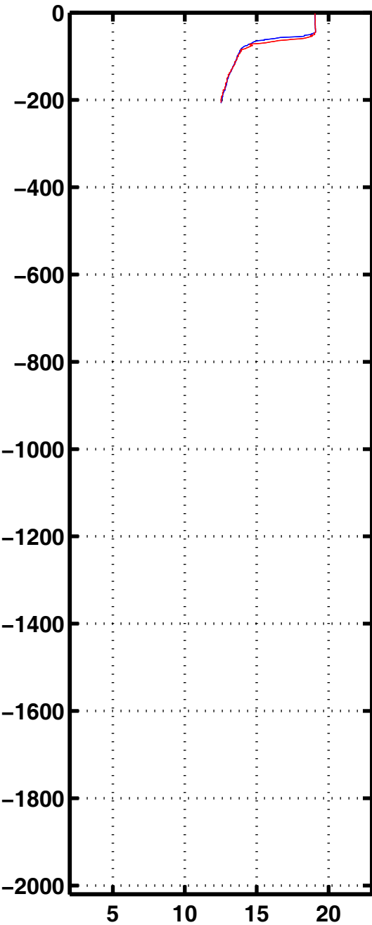
Tempe 3333
