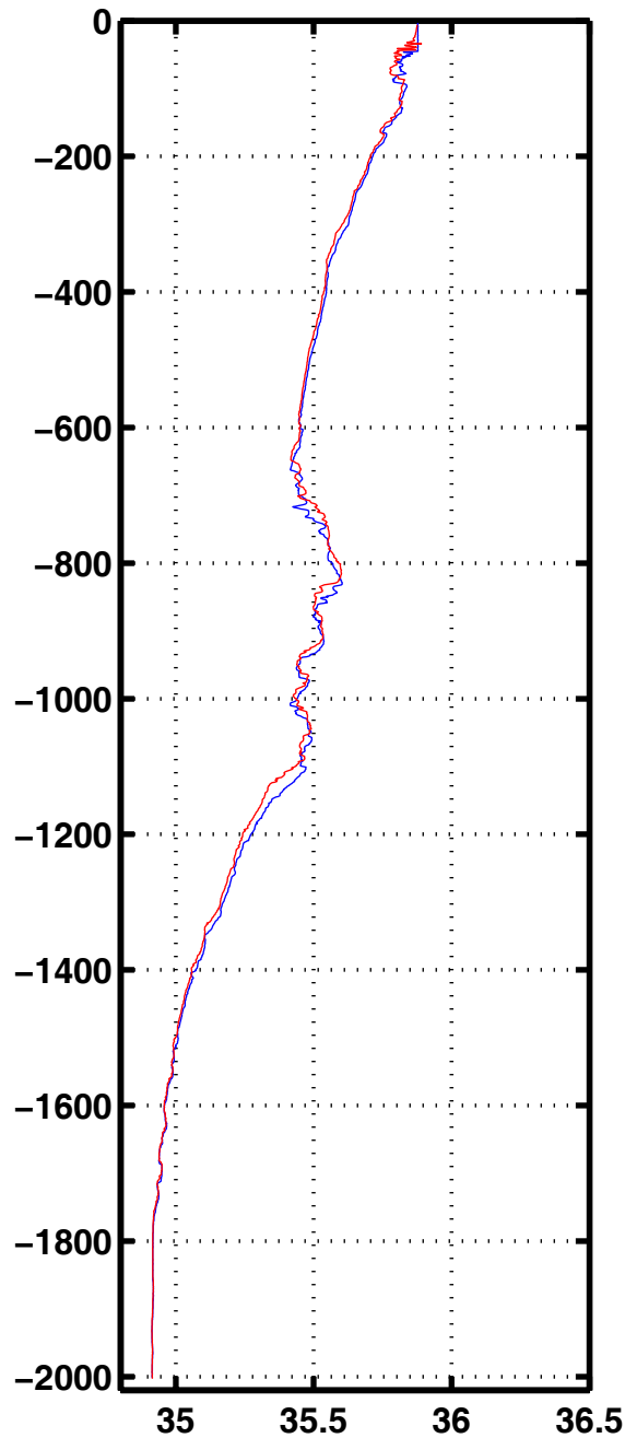
Sali 3072
