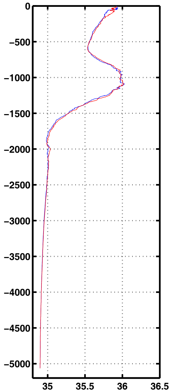
Sali 3006
