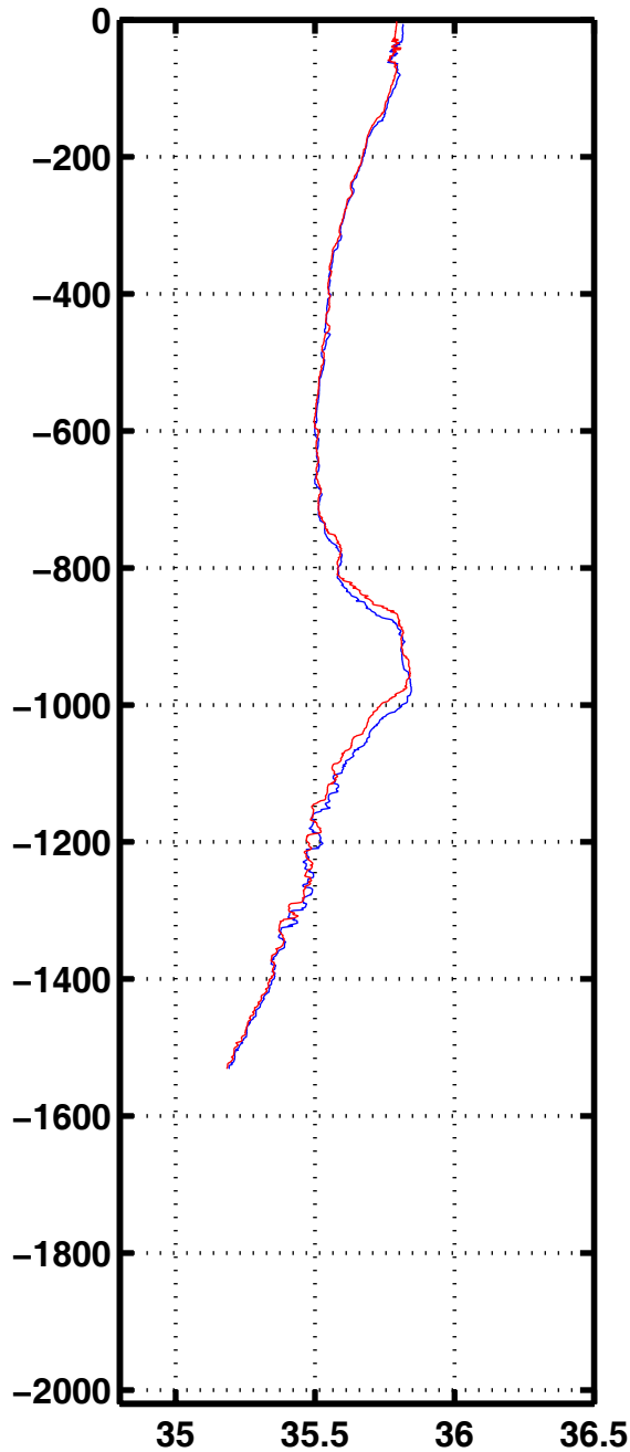
Sali 3335
