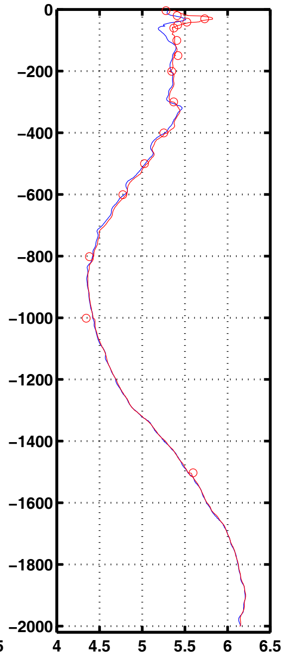
Oxyg 3002
