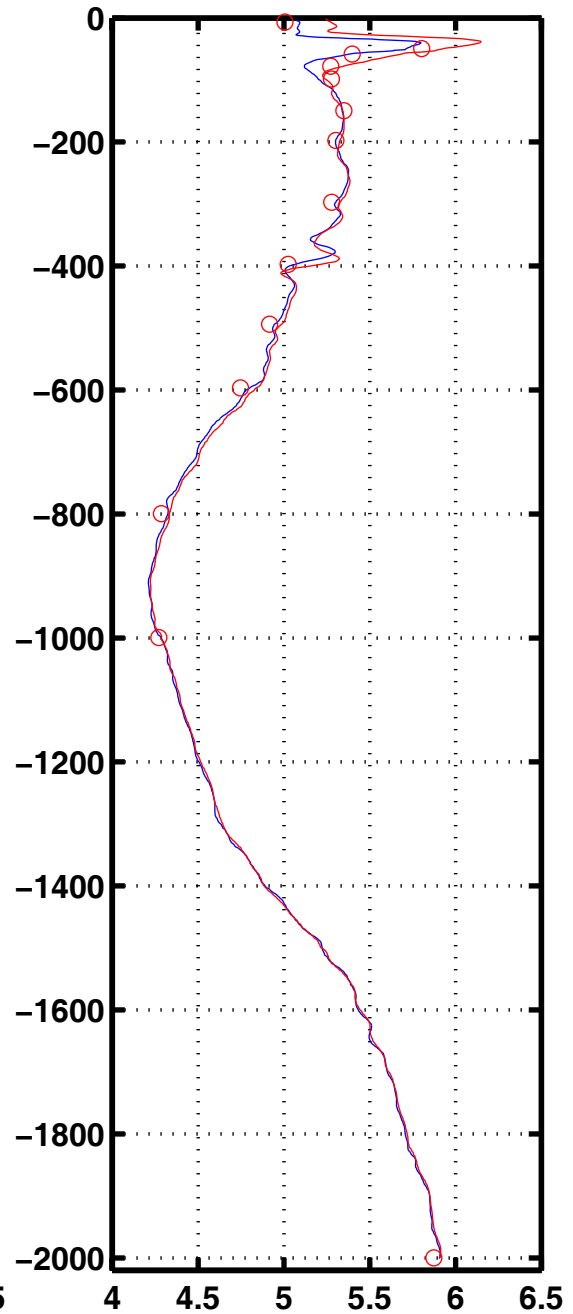
Oxyg 3042
