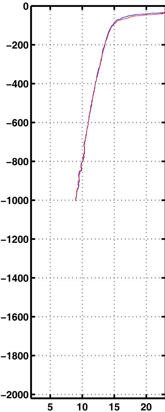
Tempe 3084
