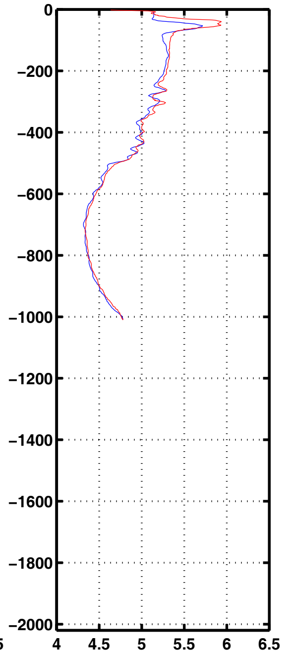
Oxyg 3242
