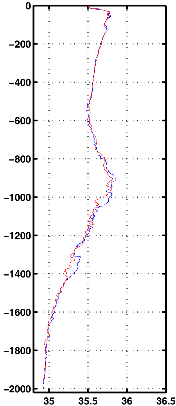
Sali 3003
