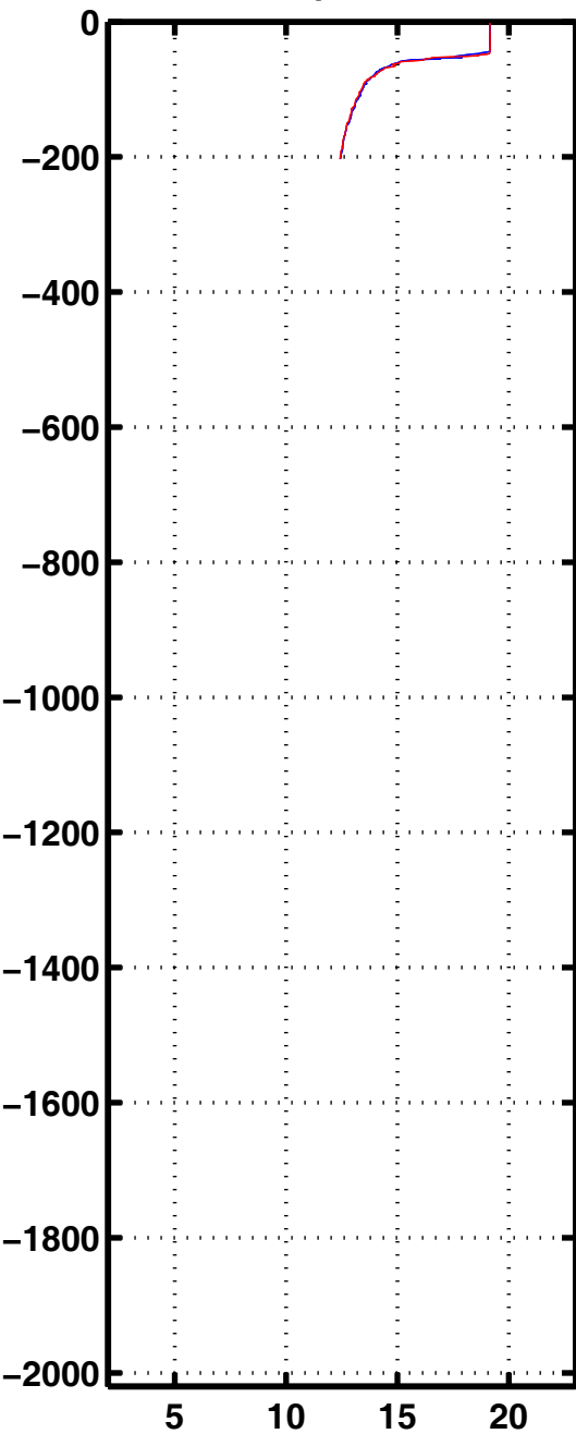
Tempe 3331
