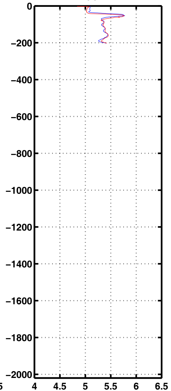
Oxyg 3162
