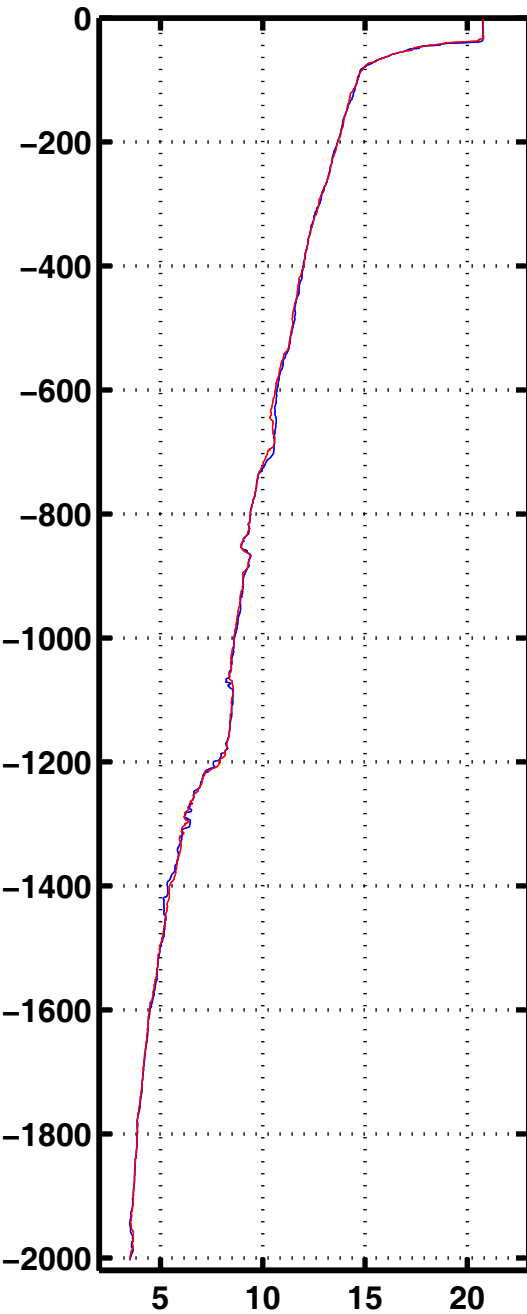
Tempe 3168
