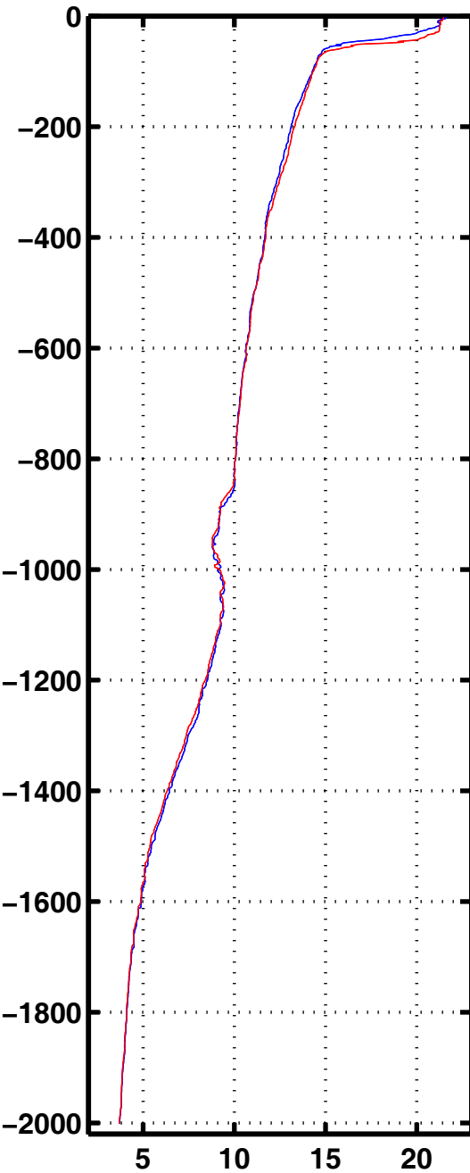
Tempe 3020
