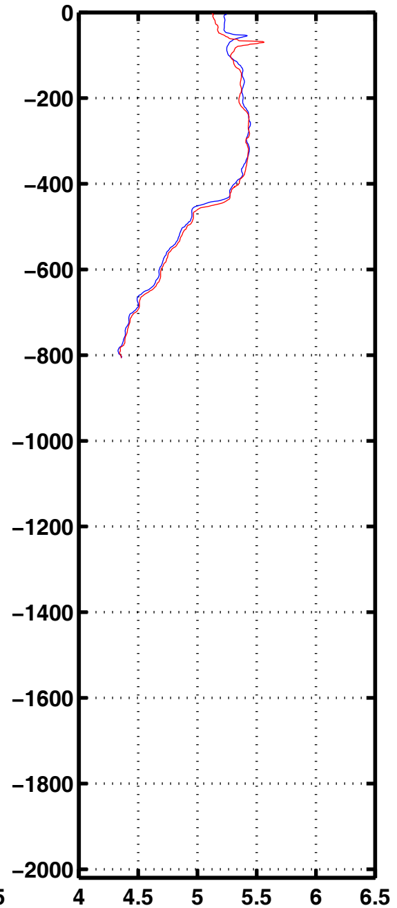
Oxyg 3332
