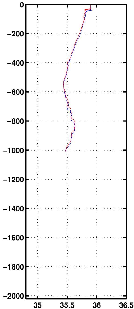
Sali 3242
