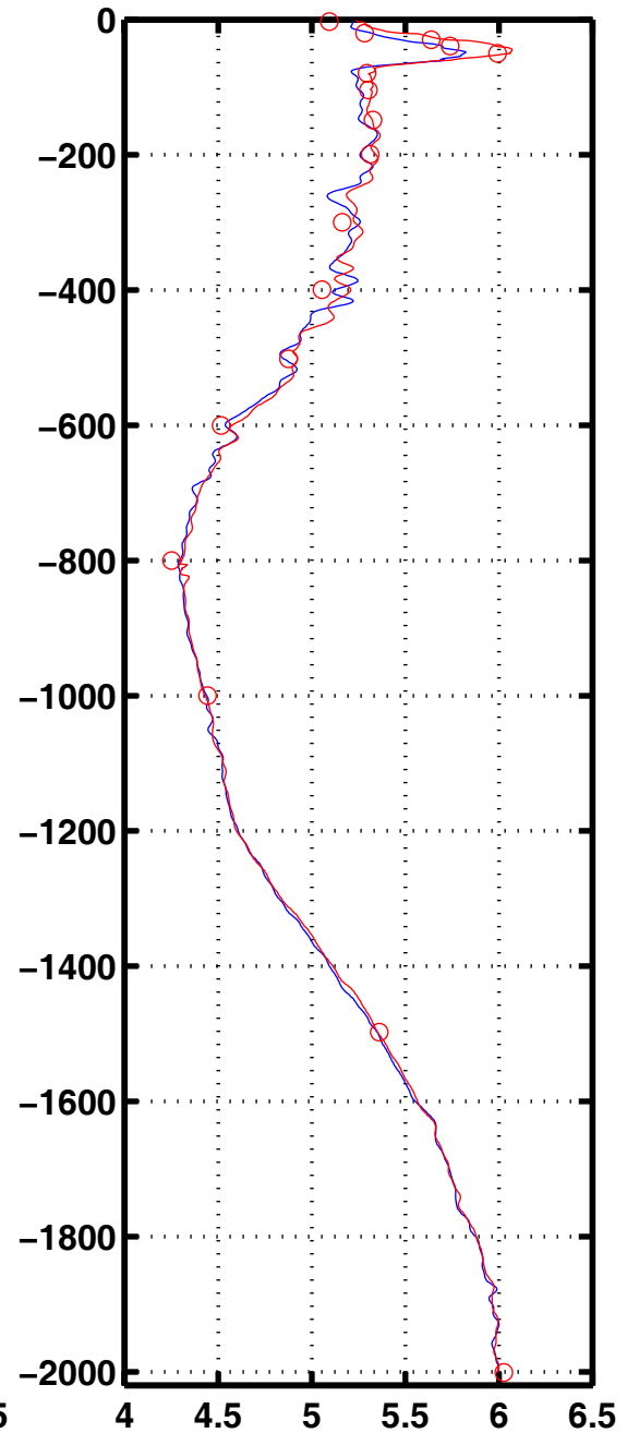
Oxyg 3008
