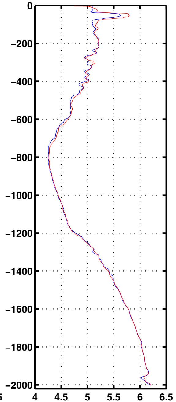
Oxyg 3168
