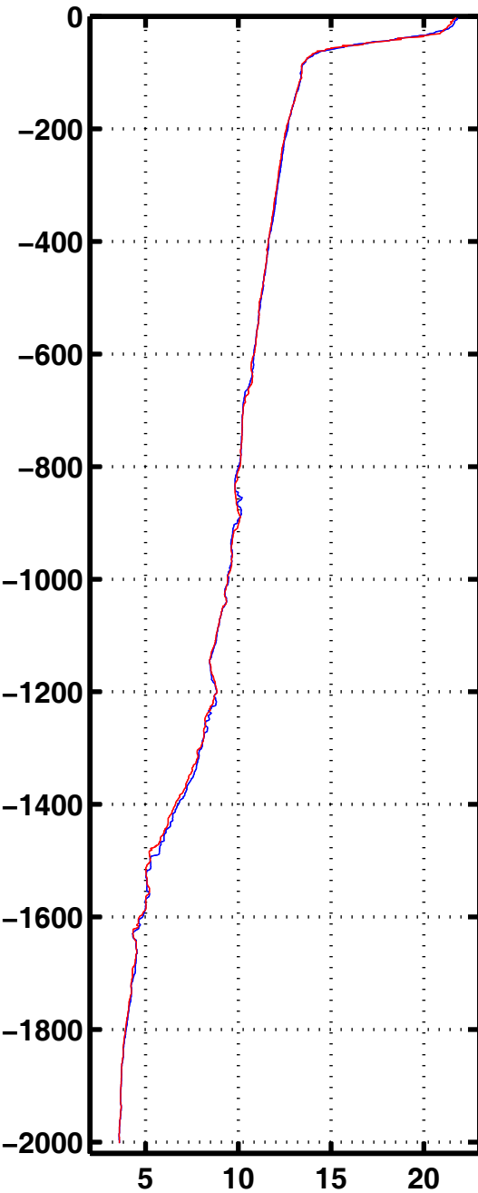
Tempe 3017
