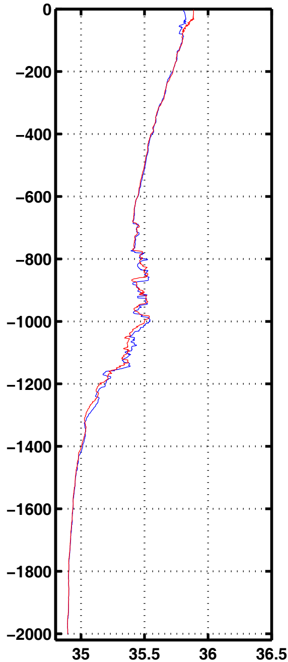
Sali 3071
