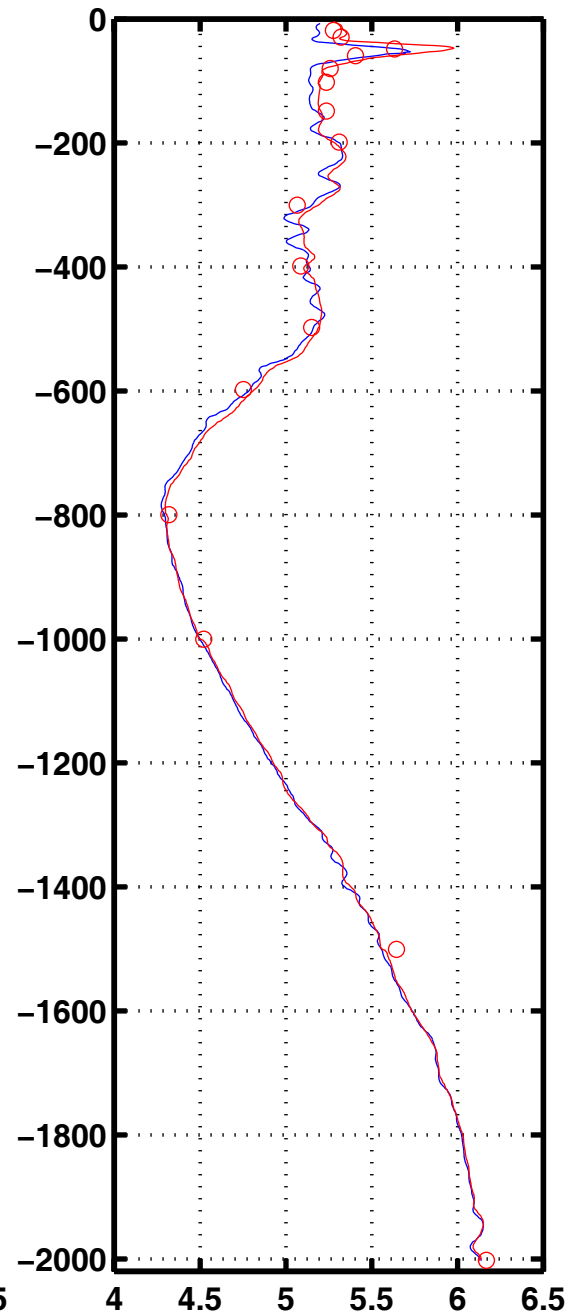
Oxyg 3053
