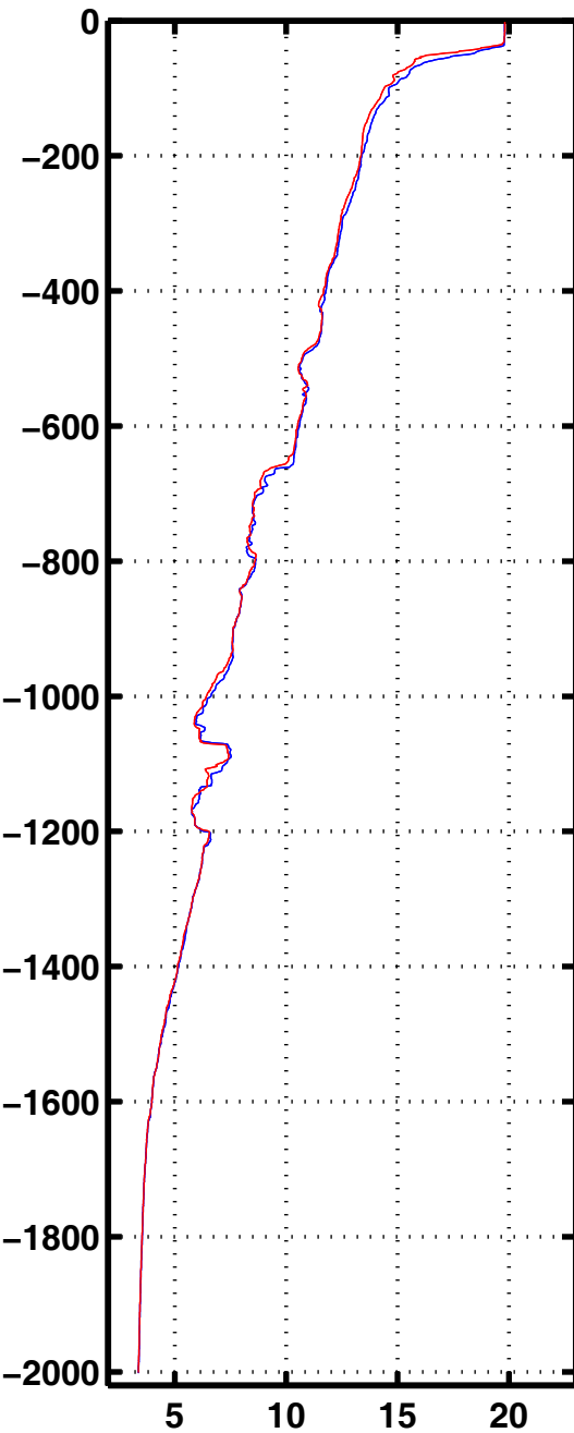
Tempe 3068
