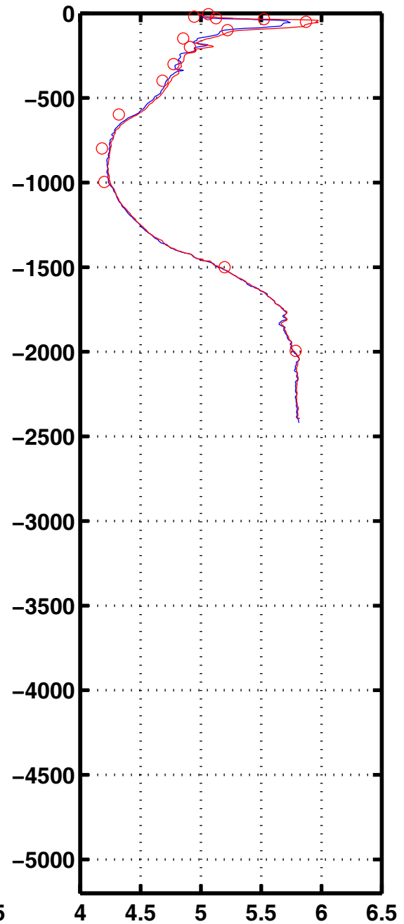
Oxyg 3013
