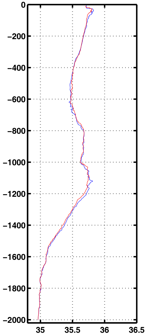
Sali 3005
