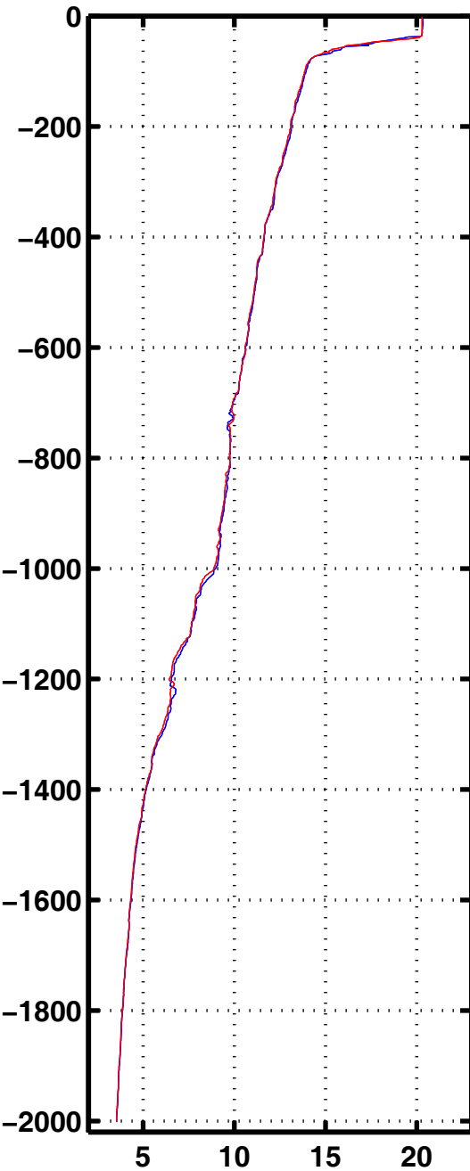
Tempe 3064
