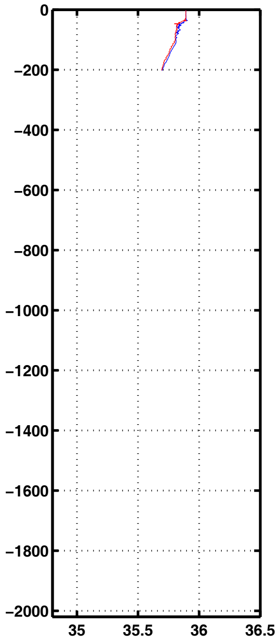
Sali 3247
