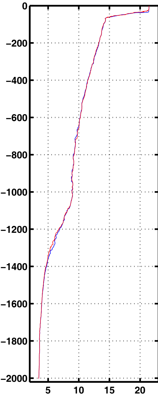
Tempe 3073
