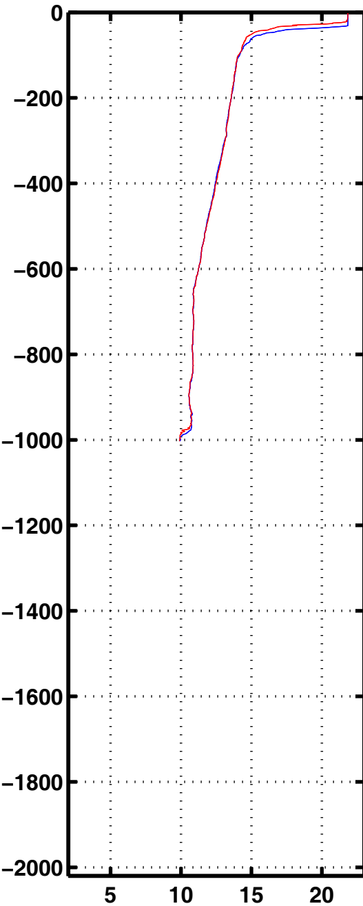
Tempe 3088
