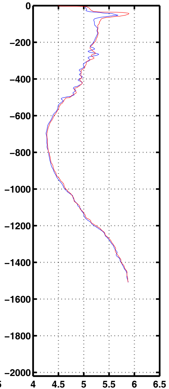
Oxyg 3243
