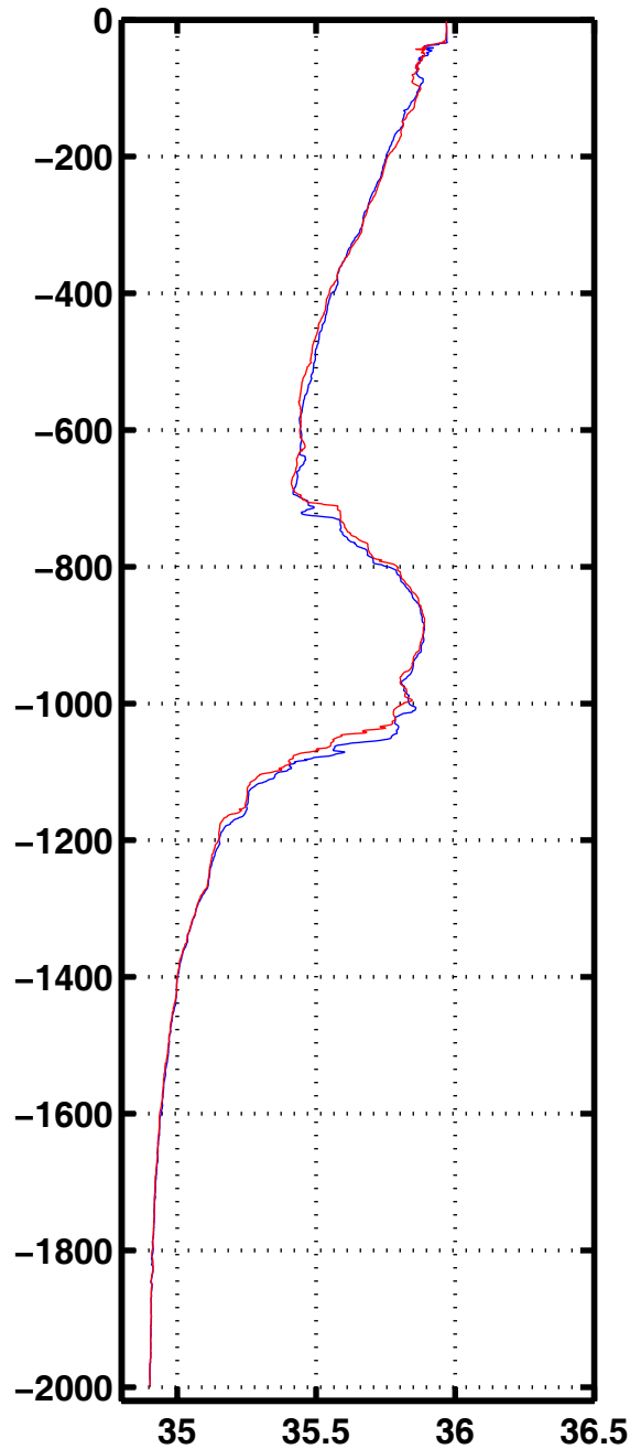
Sali 3061
