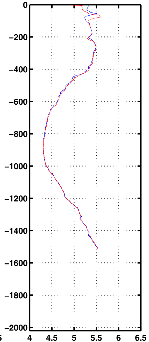
Oxyg 3327
