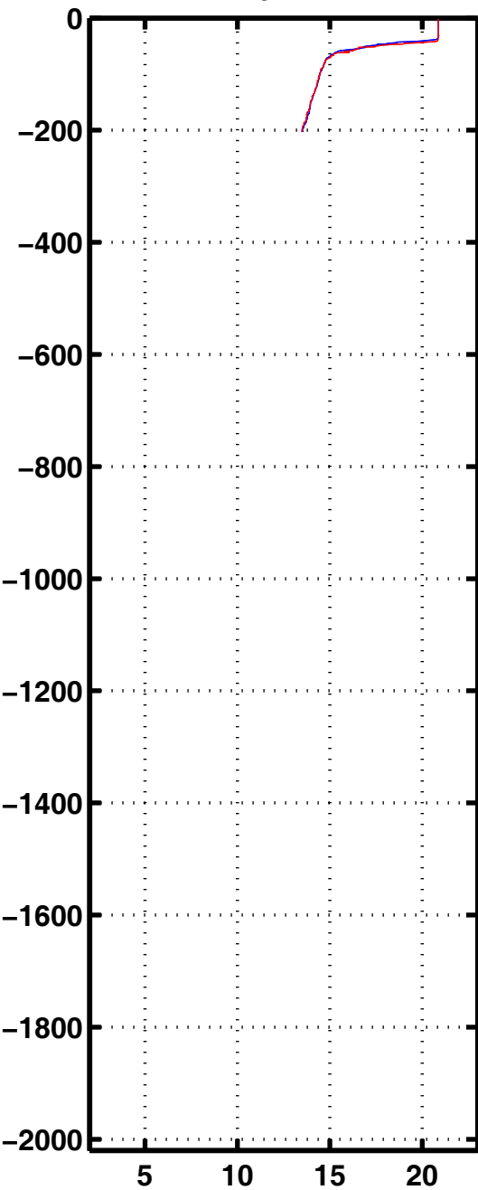
Tempe 3162
