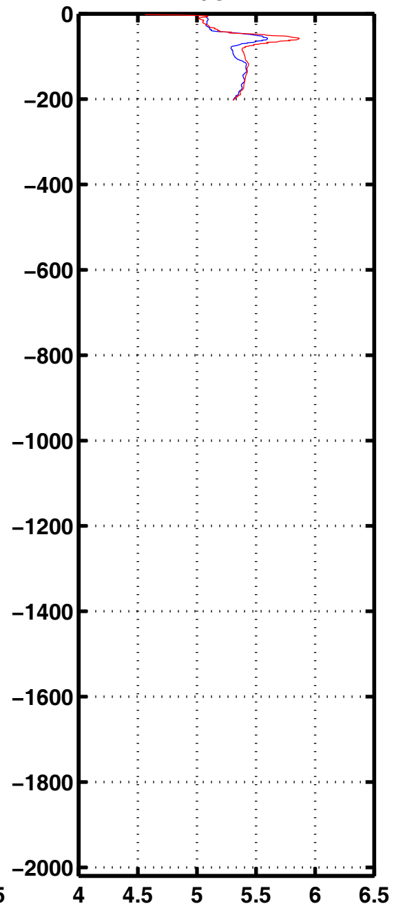
Oxyg 3238
