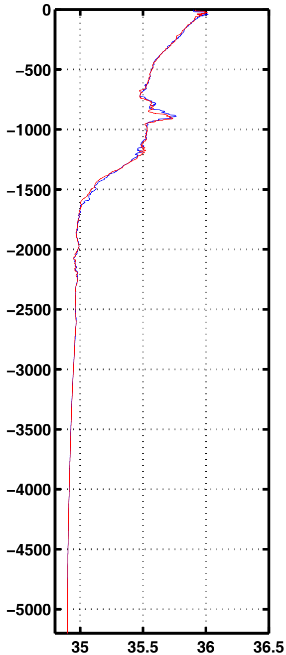
Sali 3031
