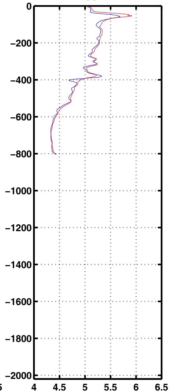
Oxyg 3248
