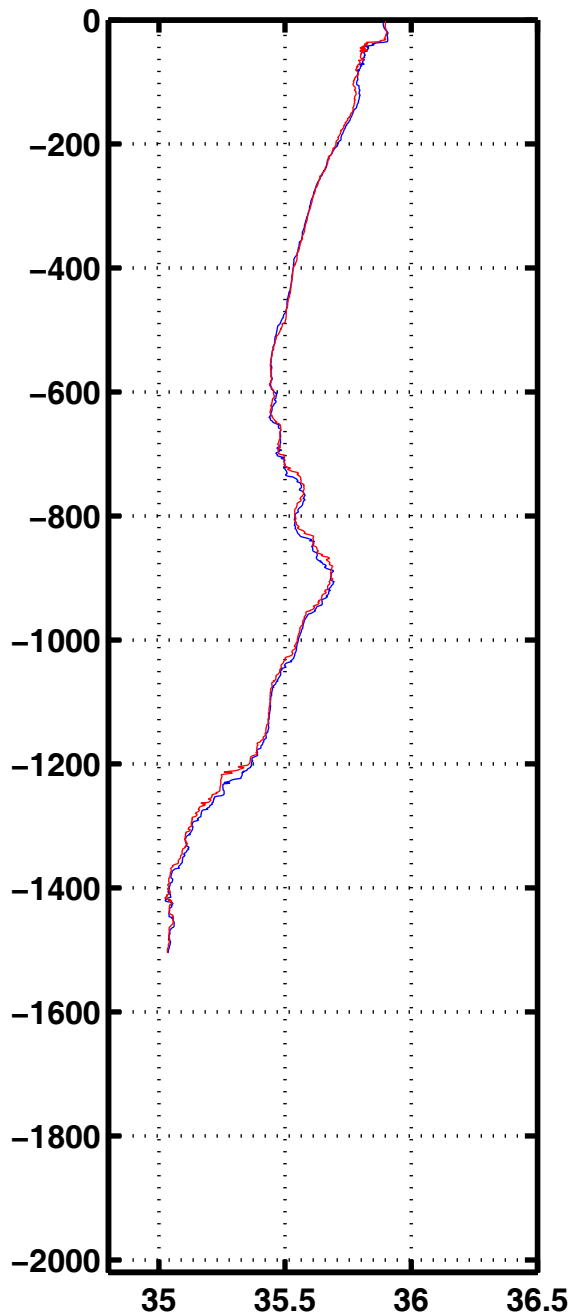
Sali 3251
