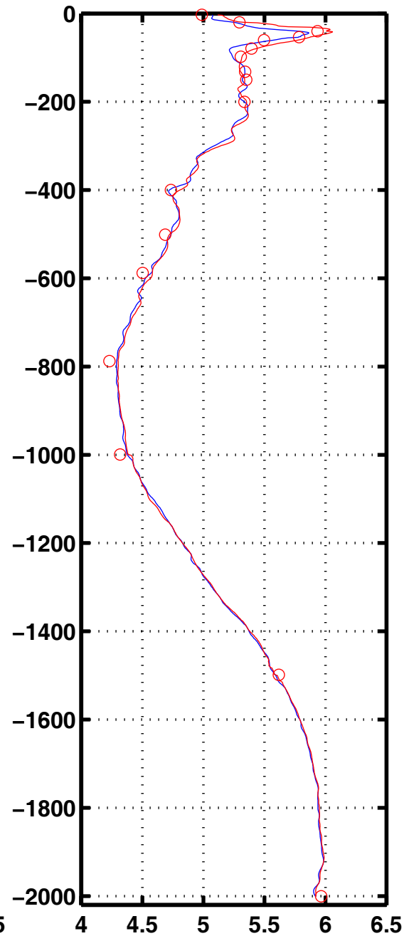
Oxyg 3010
