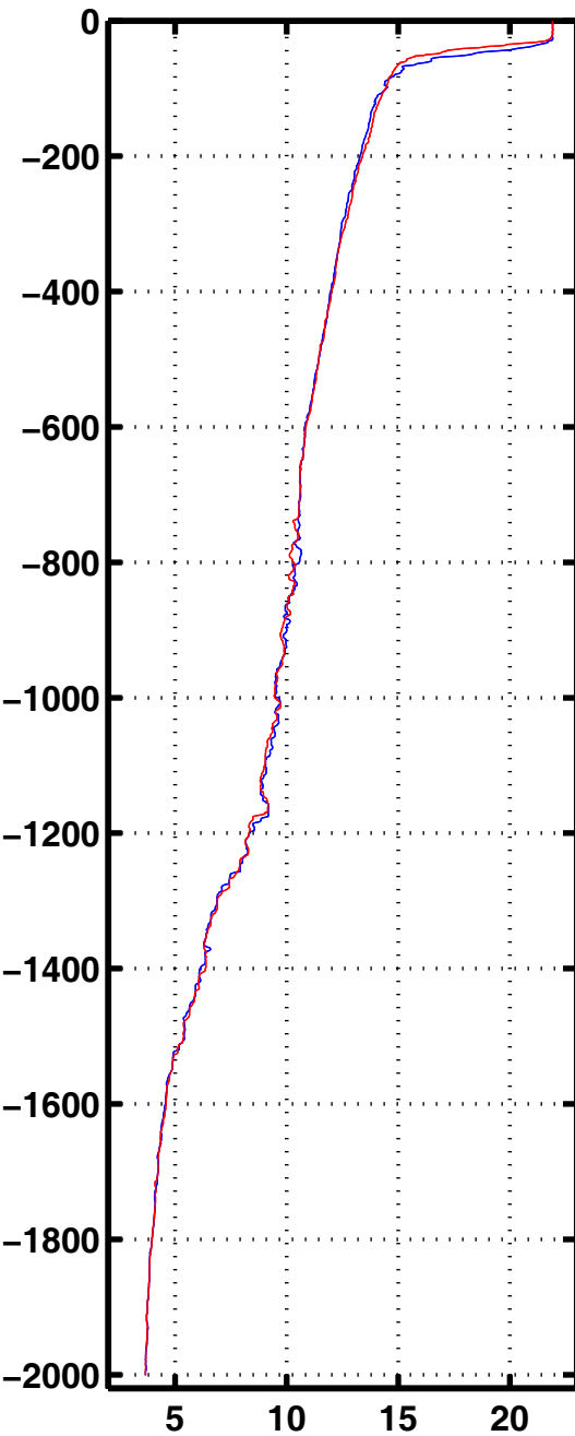
Tempe 3032
