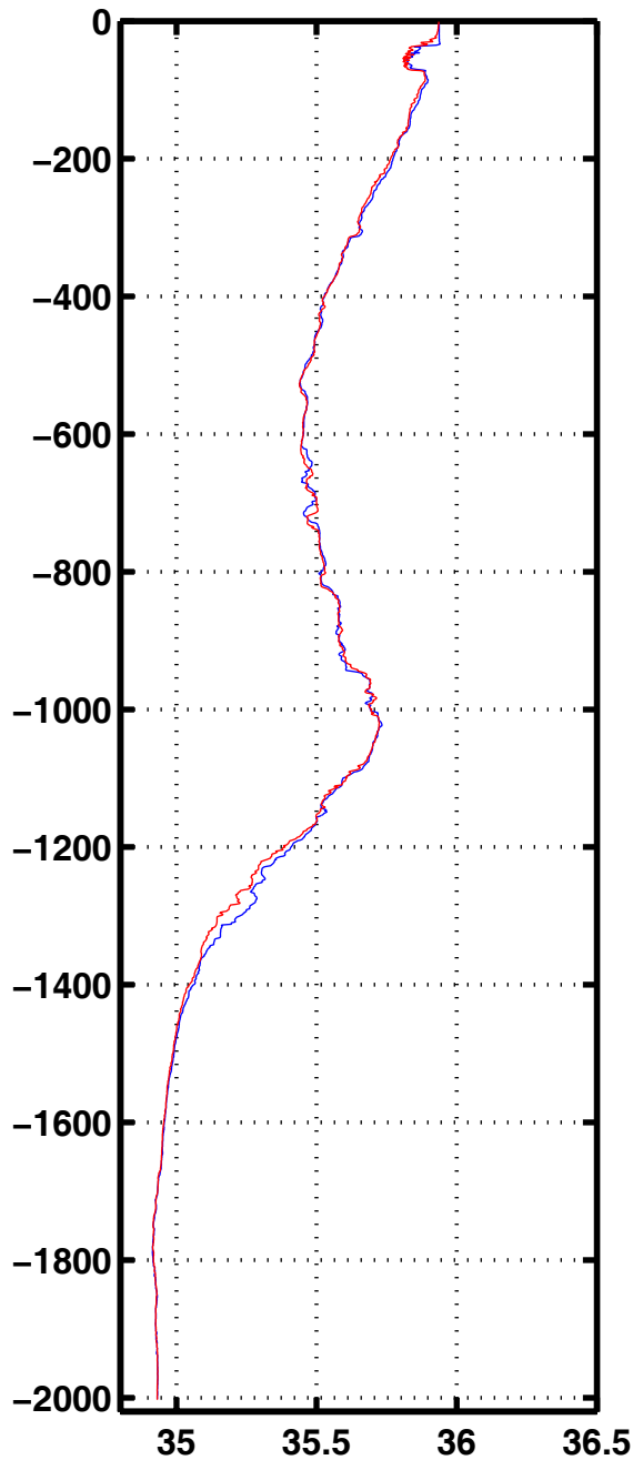
Sali 3073
