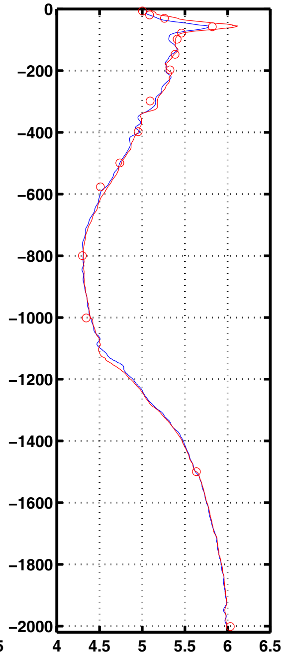
Oxyg 3009
