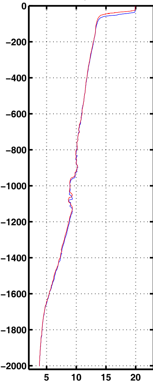
Tempe 3065
