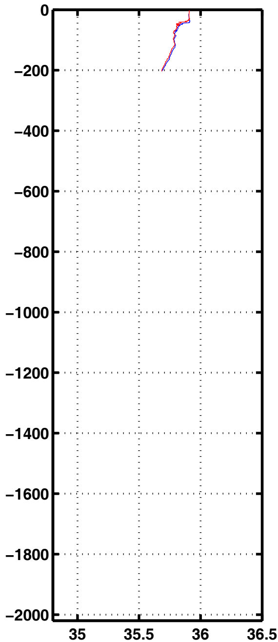
Sali 3240
