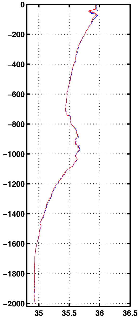
Sali 3075
