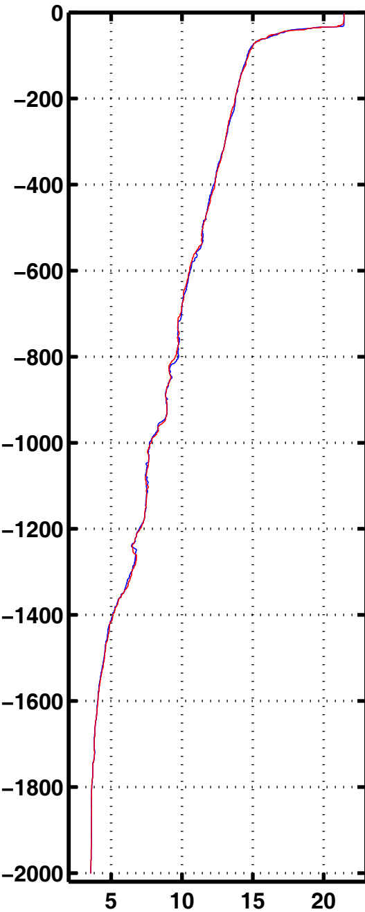
Tempe 3076
