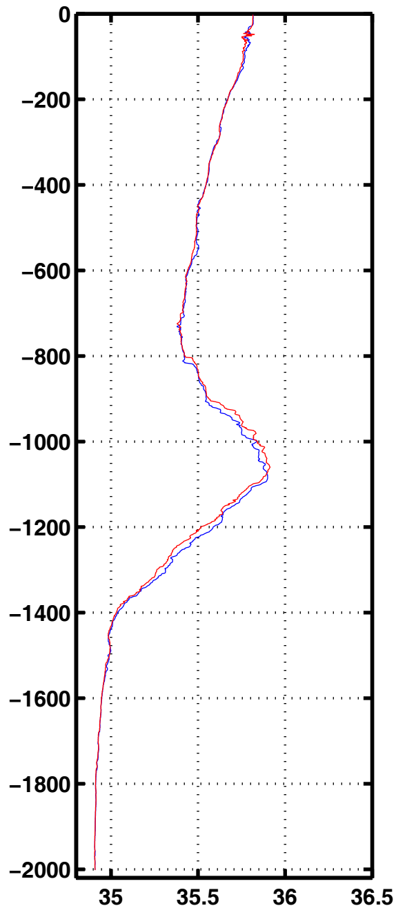
Sali 3051
