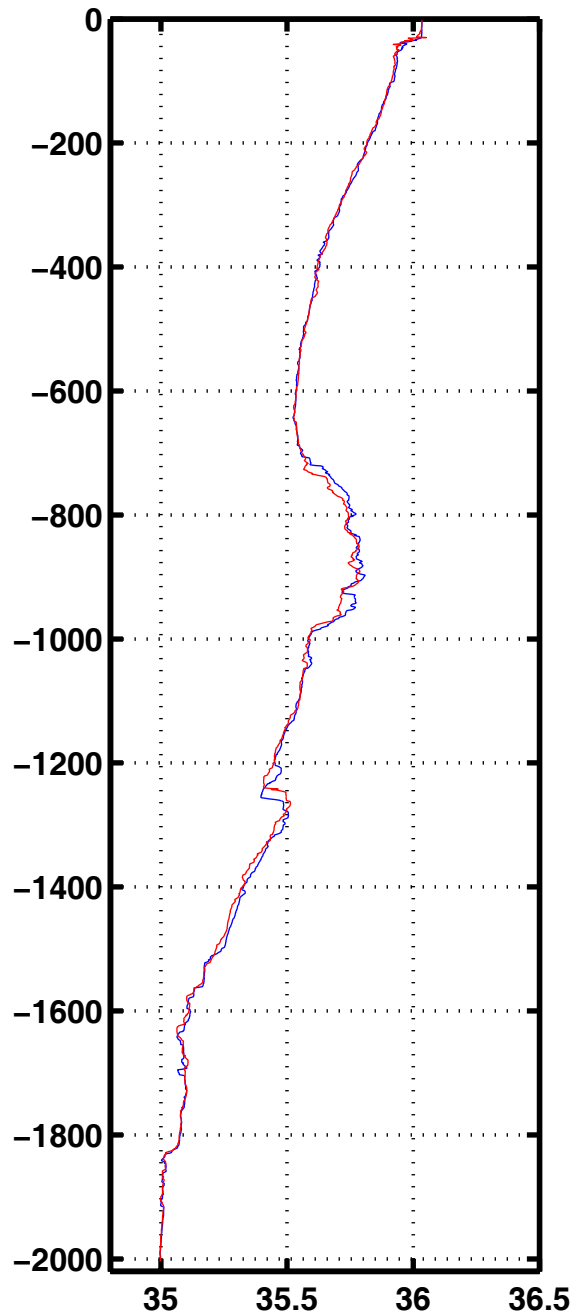
Sali 3047
