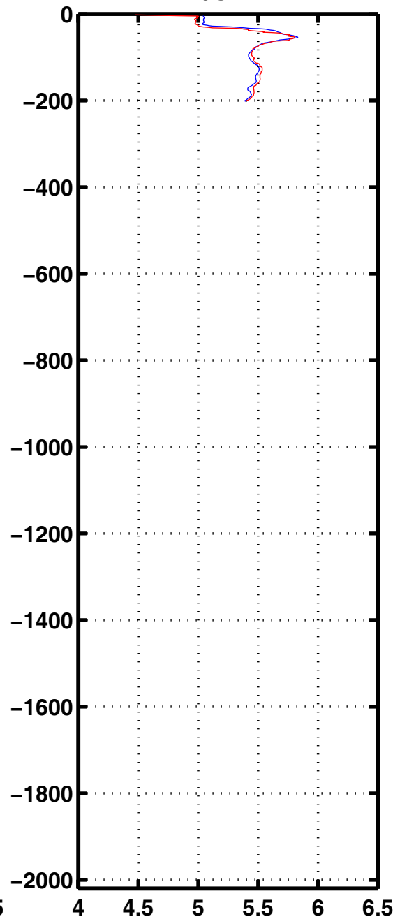
Oxyg 3246
