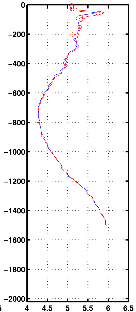
Oxyg 3250
