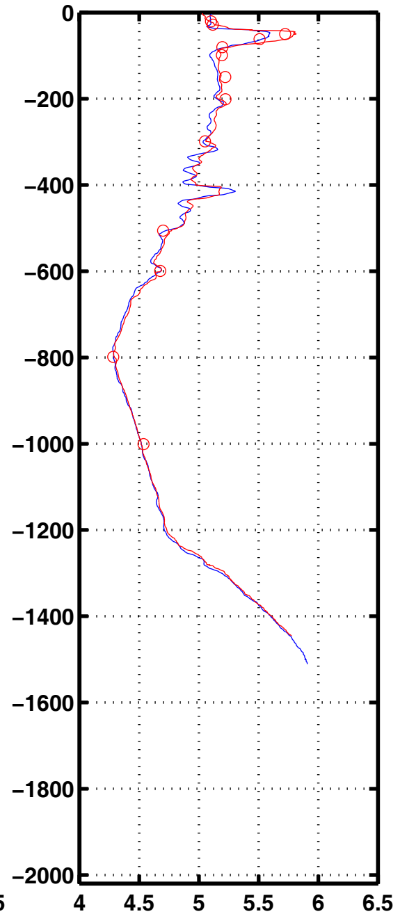
Oxyg 3157
