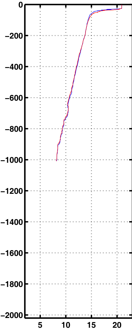
Tempe 3160
