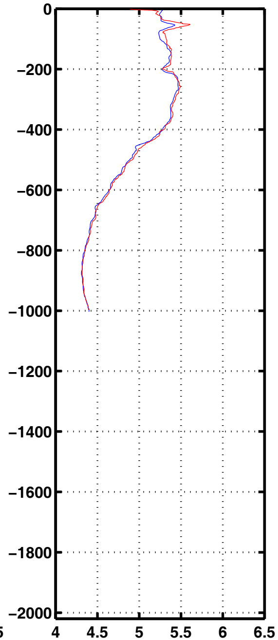
Oxyg 3326
