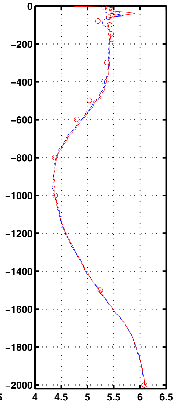
Oxyg 3065
