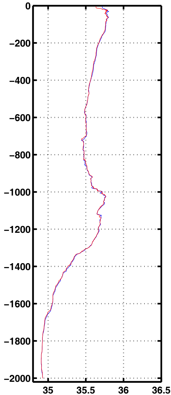
Sali 3002
