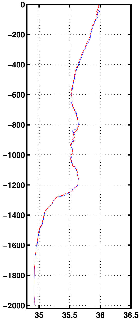
Sali 3059
