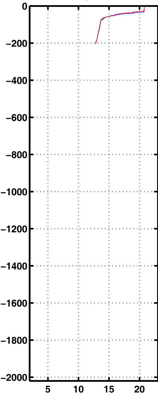
Tempe 3249
