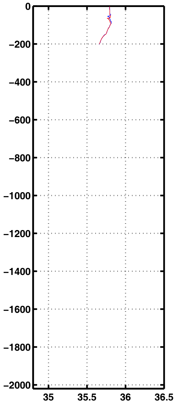
Sali 3324
