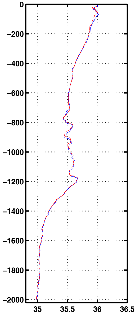
Sali 3077
