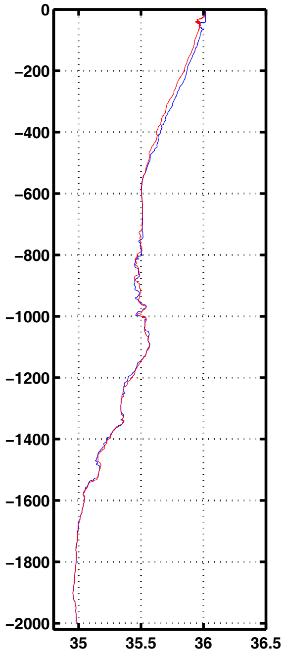
Sali 3054
