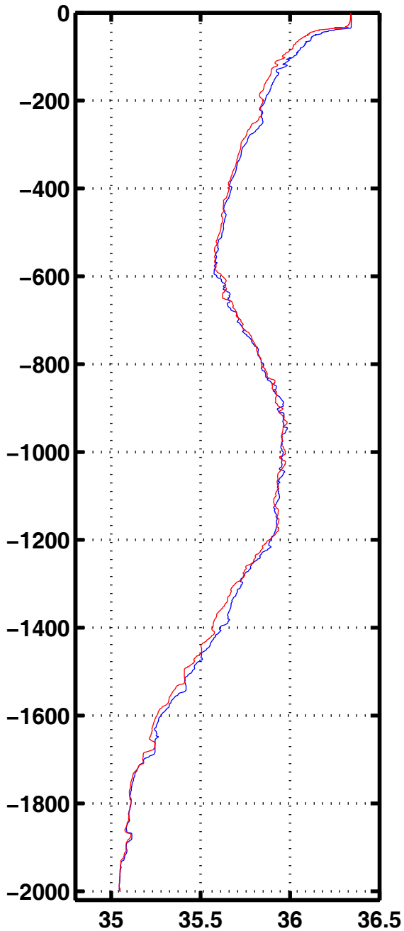
Sali 3014
