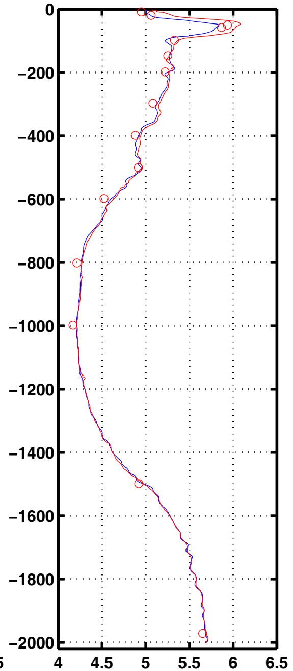
Oxyg 3012
