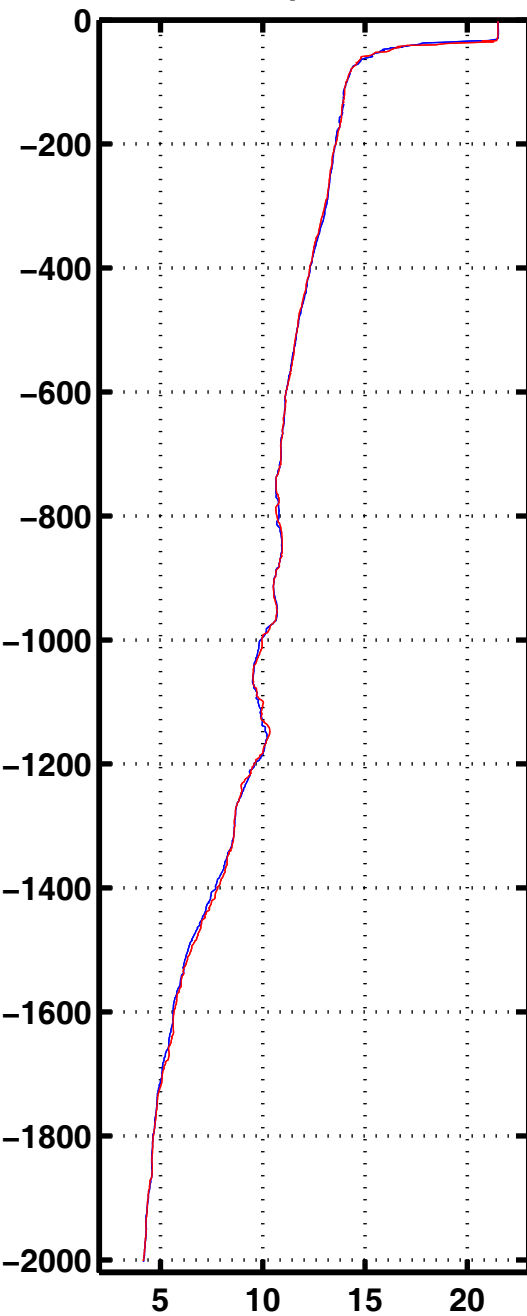
Tempe 3099
