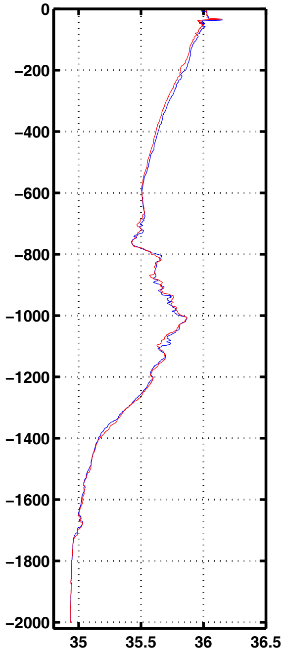
Sali 3080
