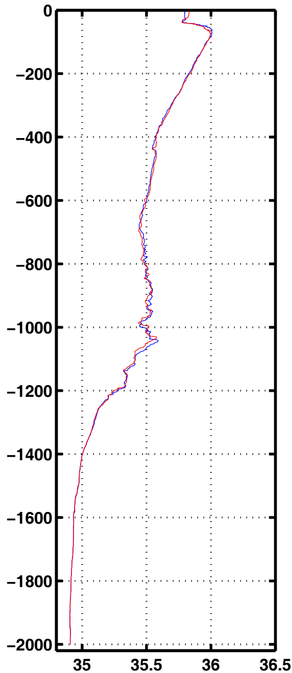
Sali 3062
