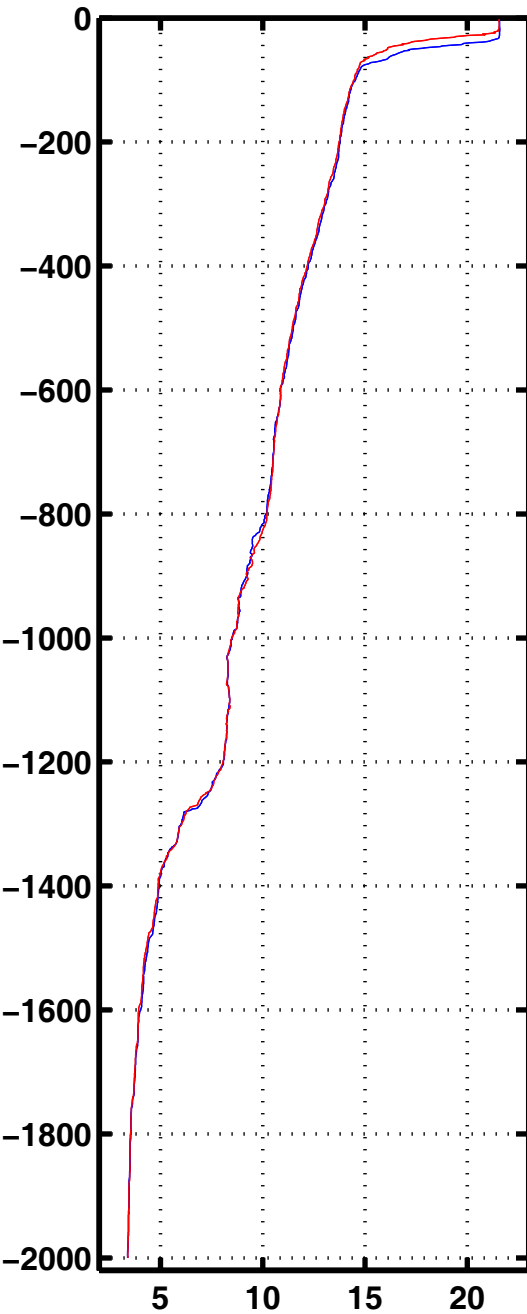
Tempe 3059
