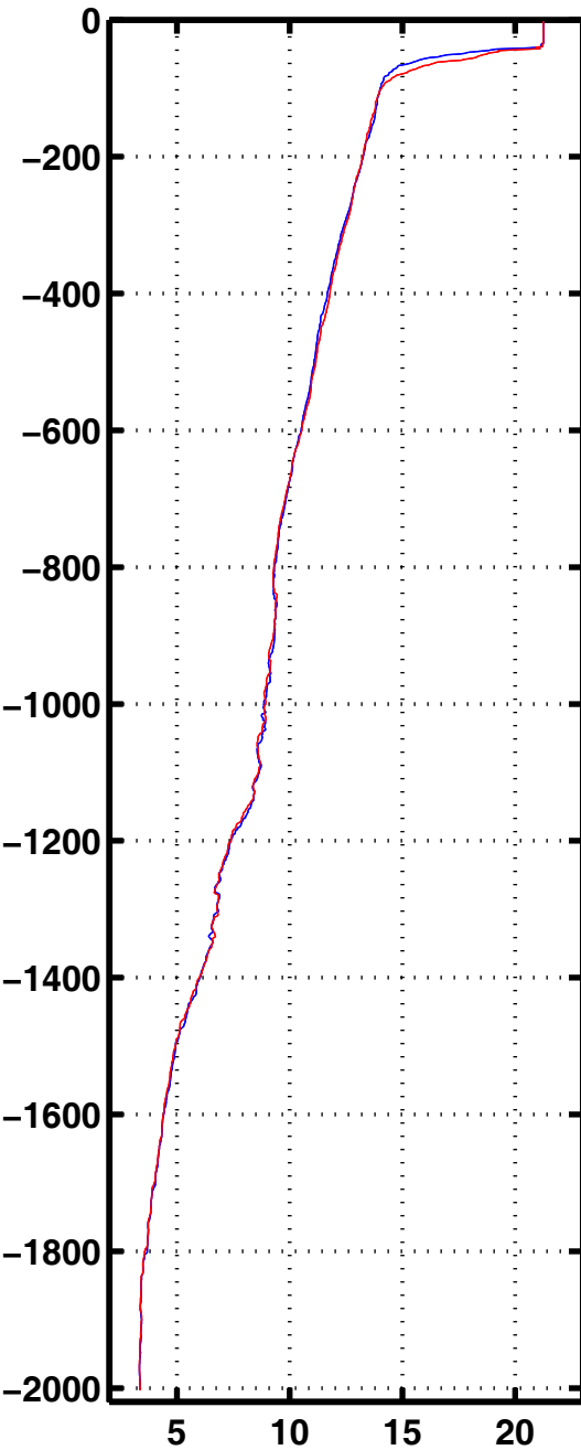
Tempe 3060
