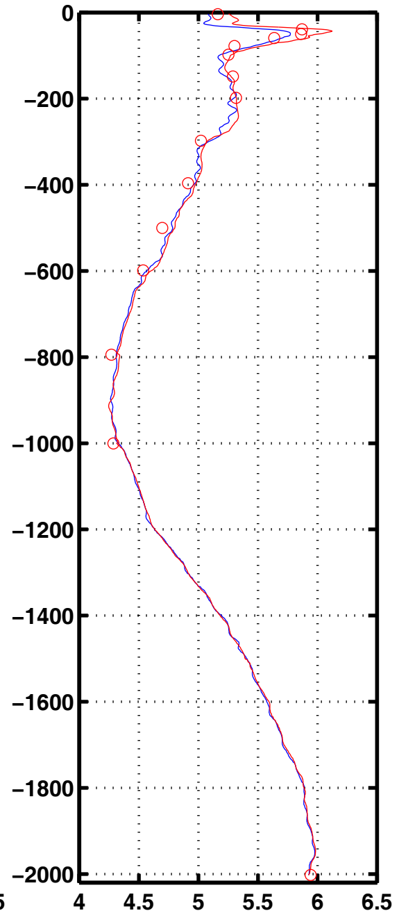
Oxyg 3040
