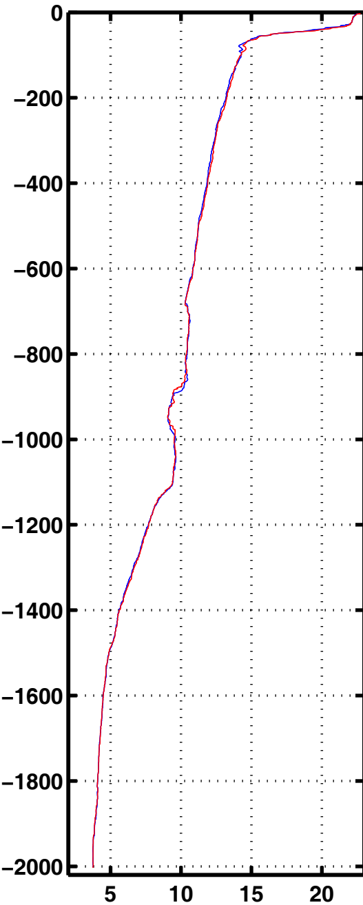
Tempe 3015
