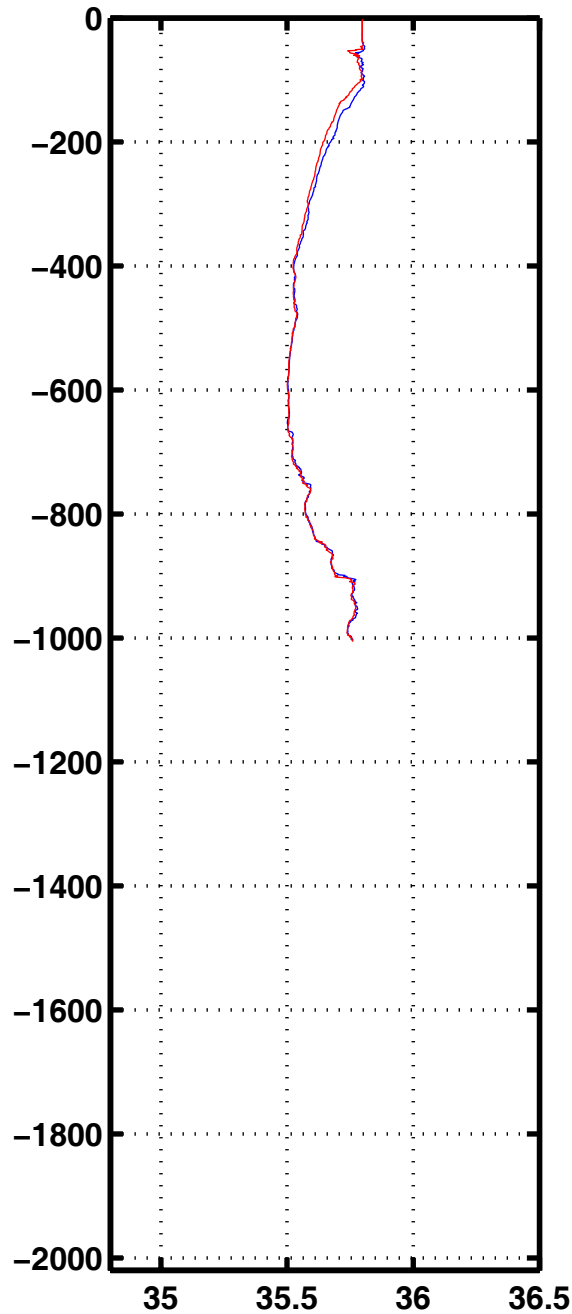
Sali 3328
