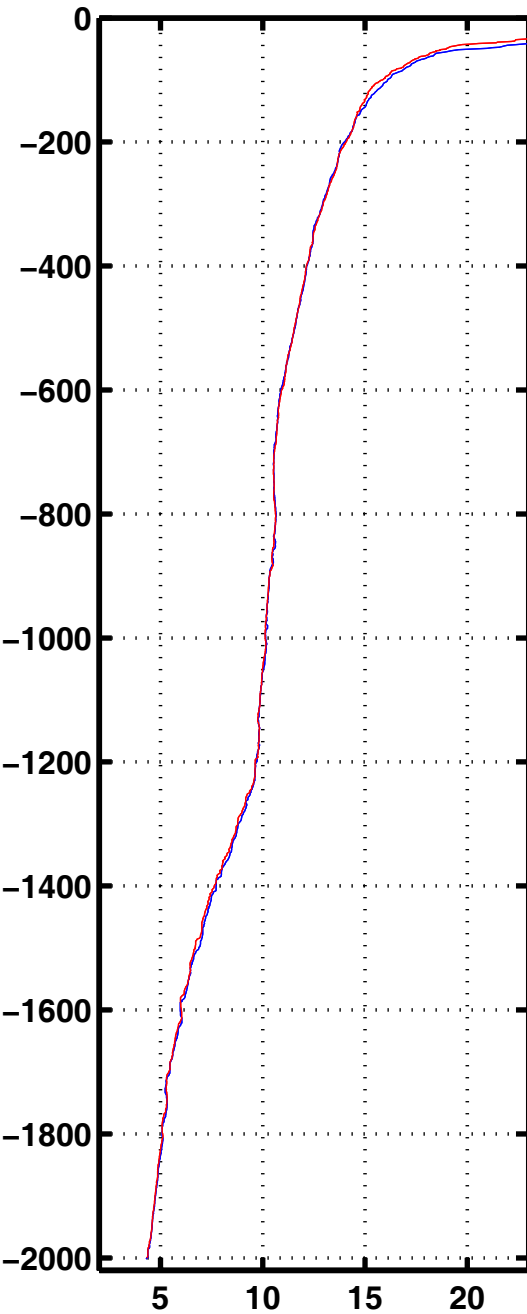
Tempe 3037
