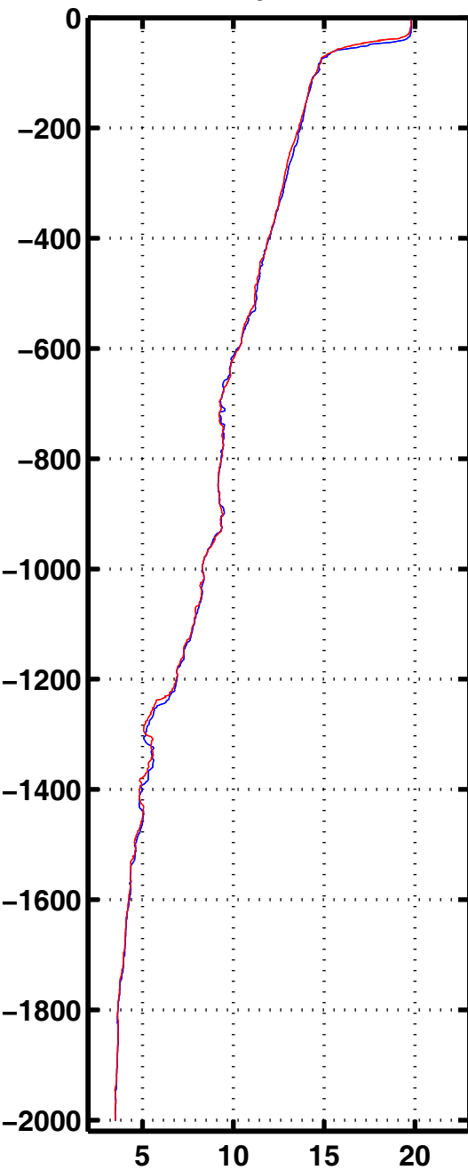
Tempe 3070
