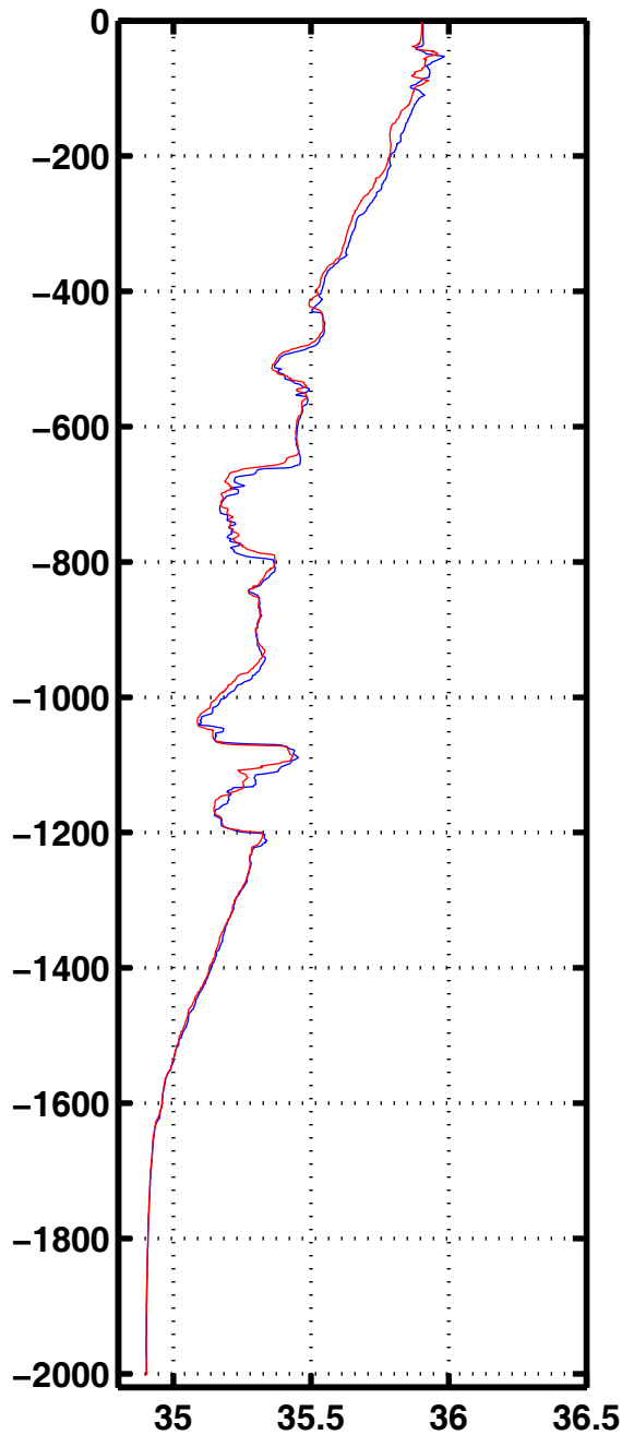
Sali 3068
