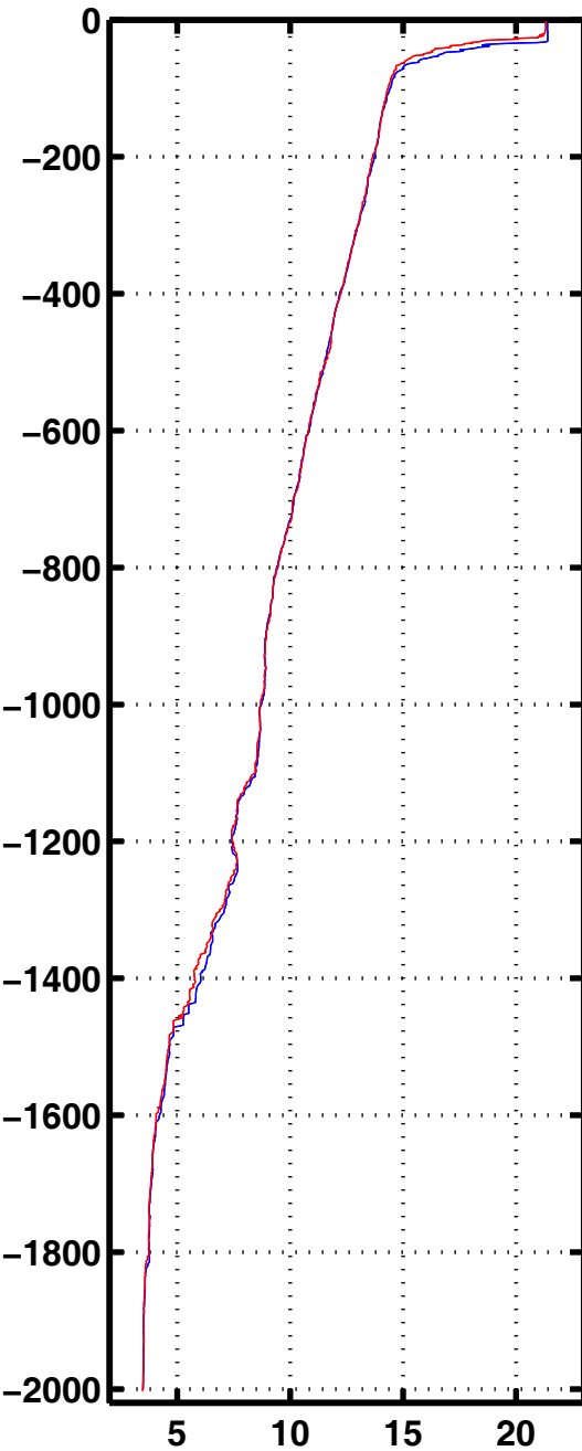
Tempe 3048
