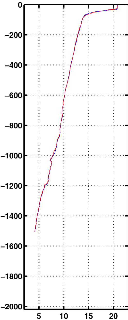
Tempe 3241
