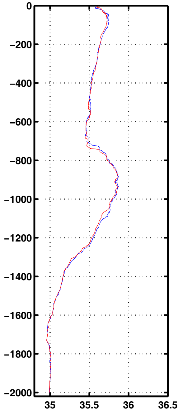
Sali 3028
