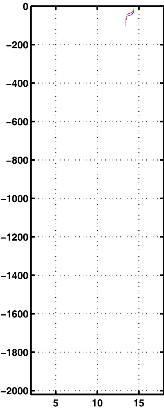
Tempe 2177
