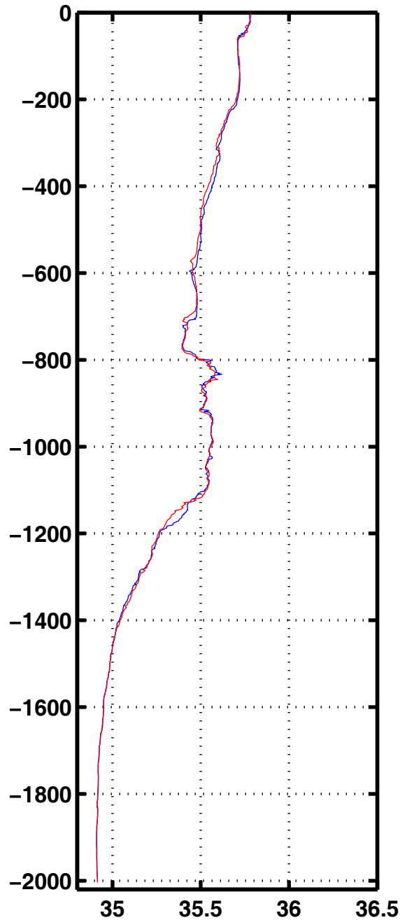
Sali 2052
