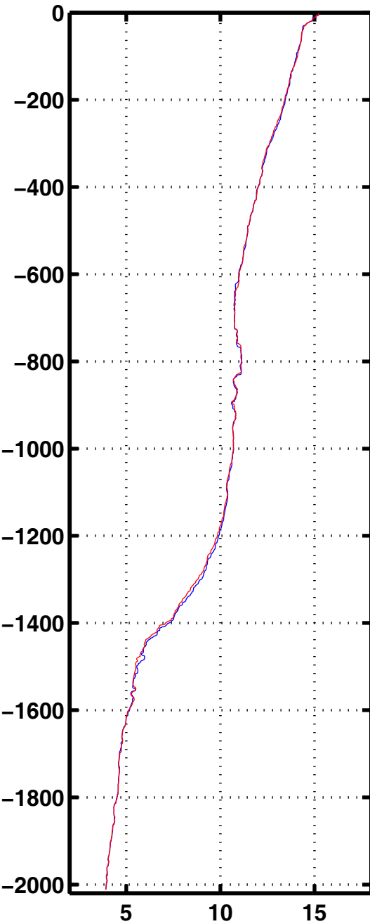
Tempe 2075
