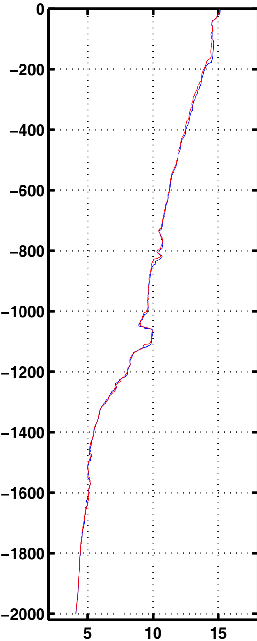
Tempe 2073
