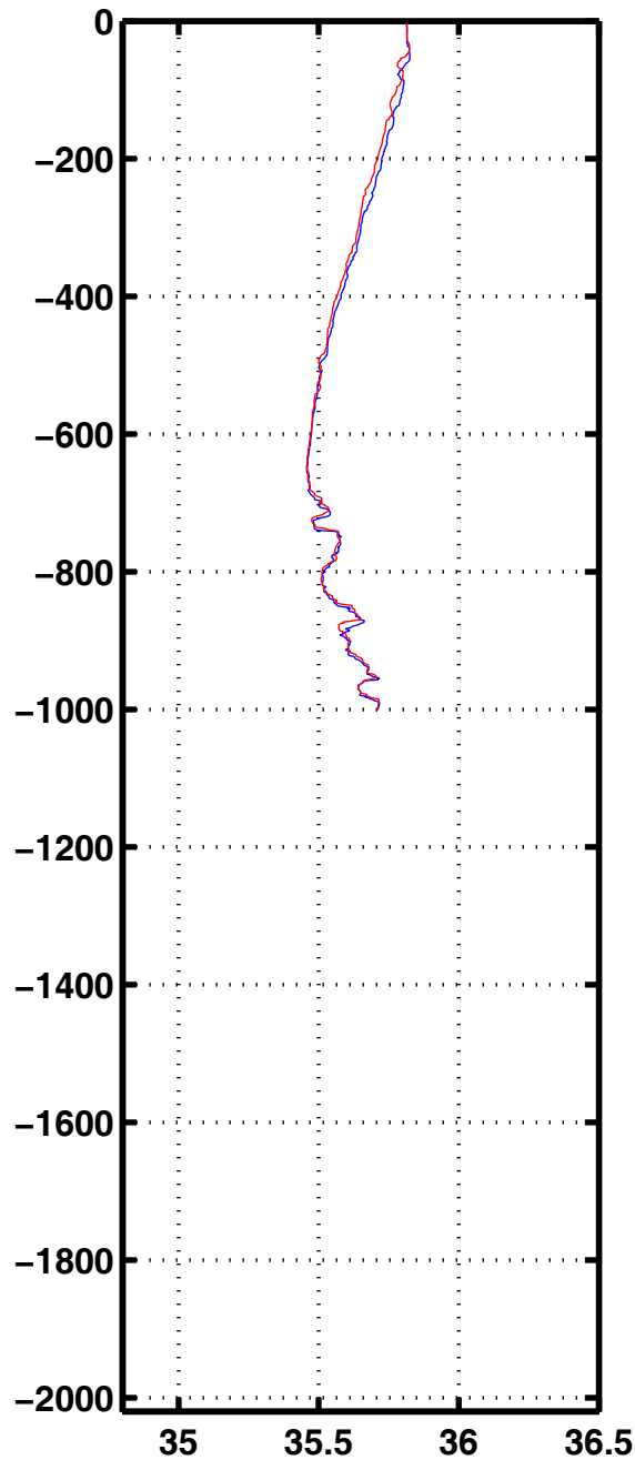
Sali 2276
