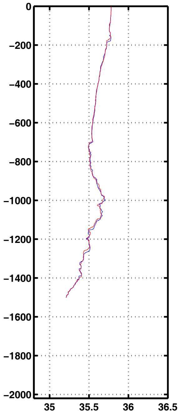
Sali 2404
