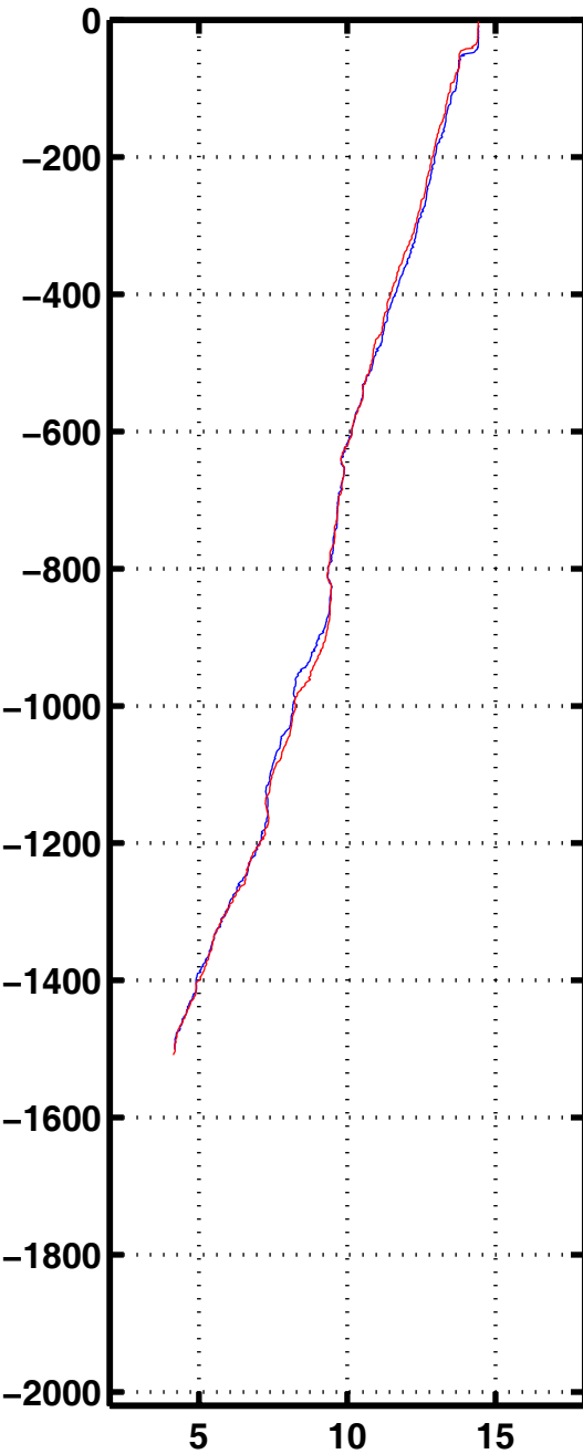
Tempe 2171
