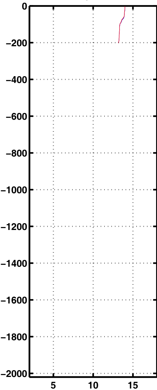
Tempe 2401
