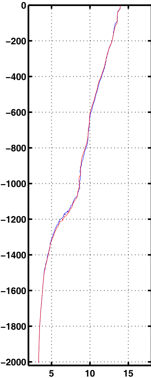
Tempe 2059
