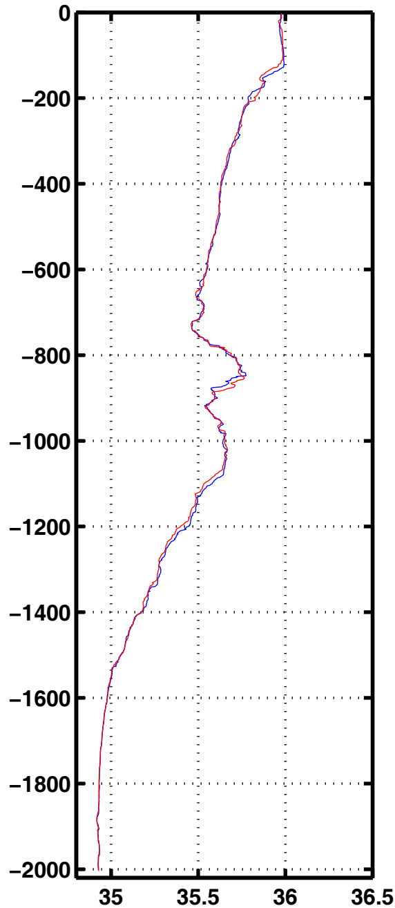
Sali 2067
