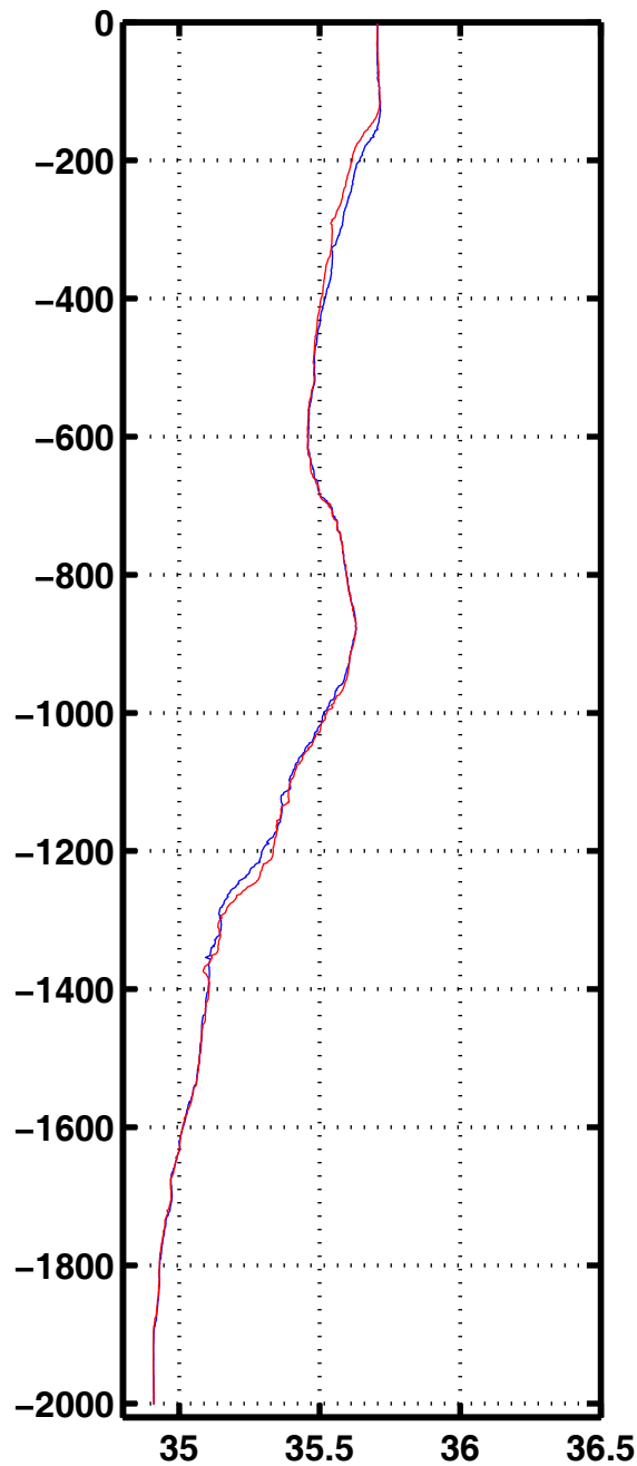
Sali 2056
