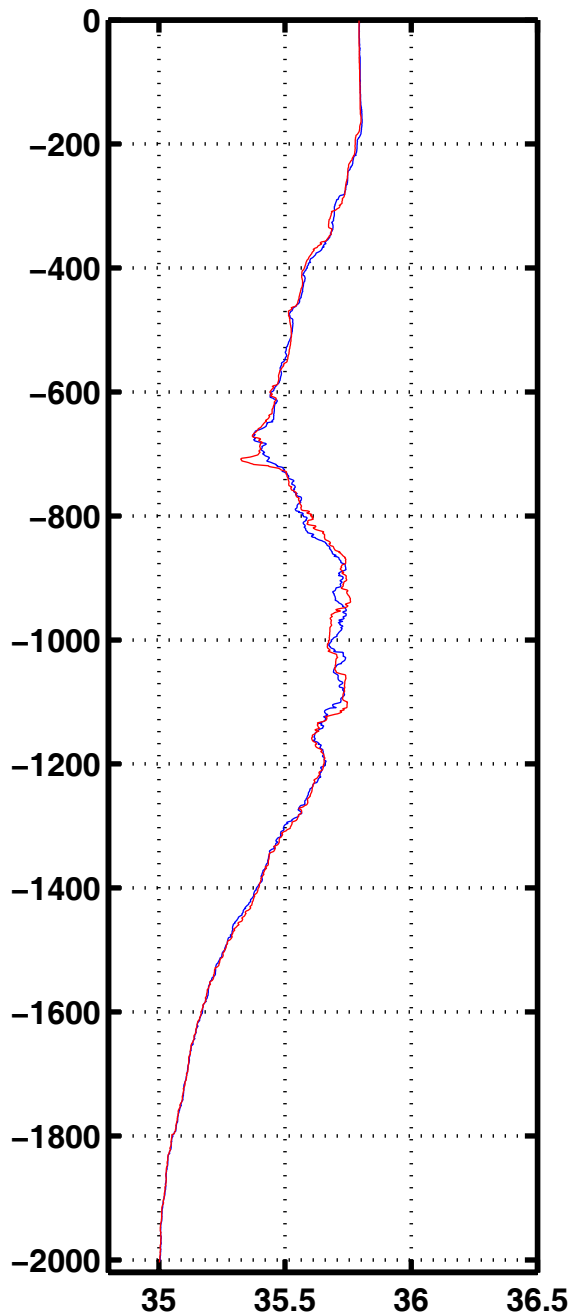
Sali 2017
