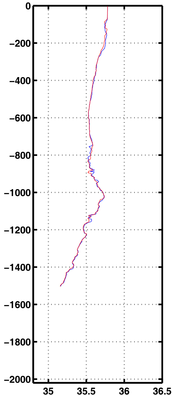
Sali 2402
