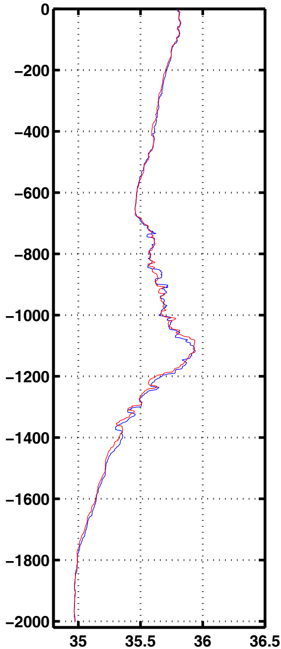
Sali 2278
