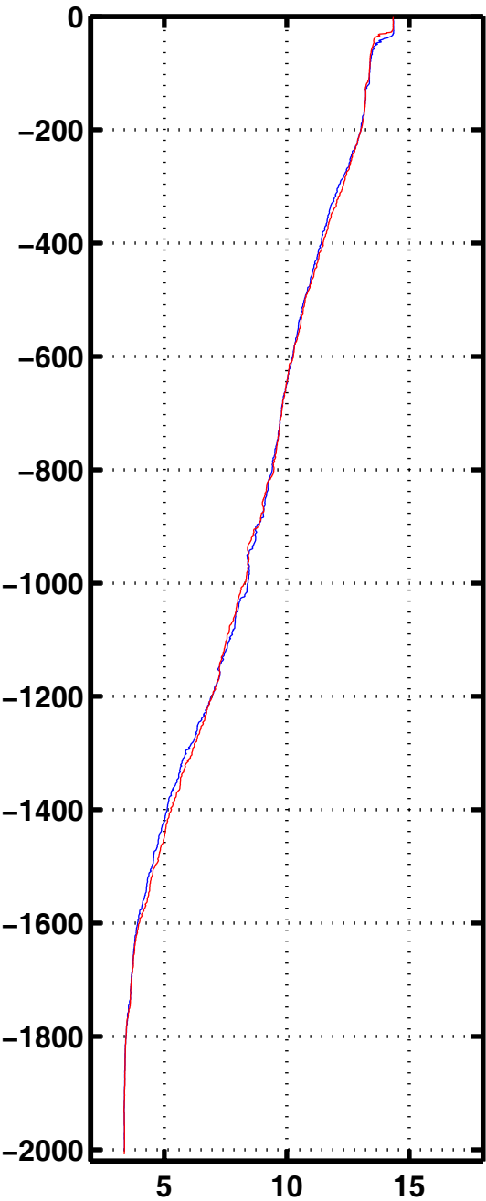
Tempe 2183
