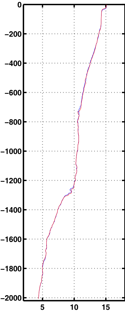
Tempe 2077
