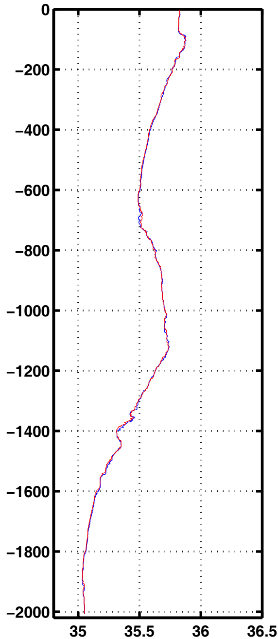
Sali 2032
