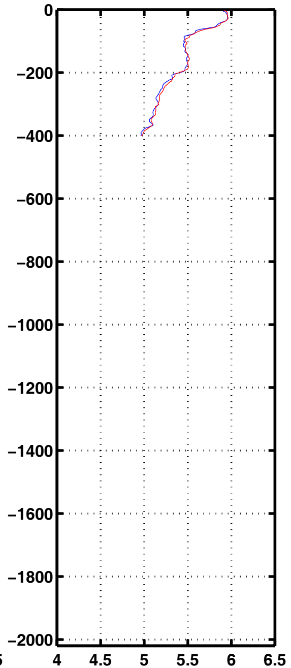
Oxyg 2271
