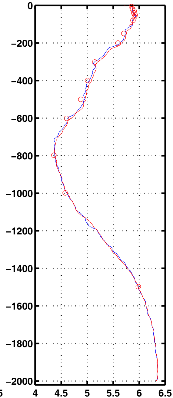
Oxyg 2052
