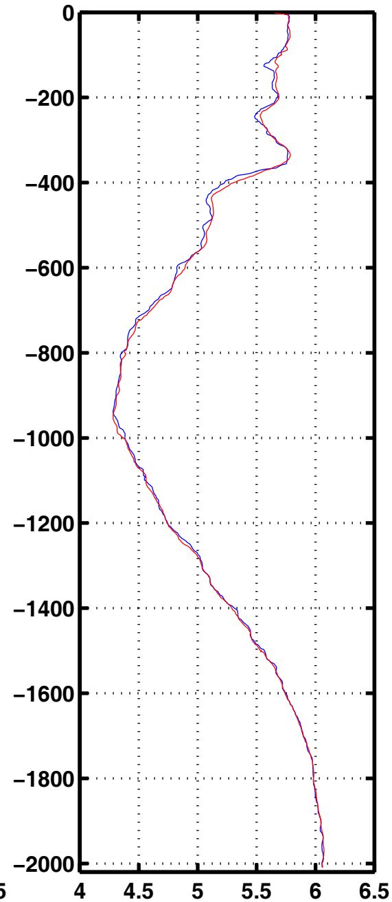
Oxyg 2005
