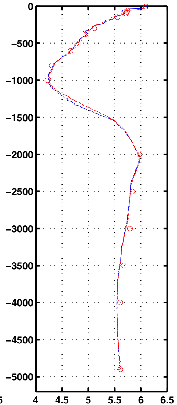
Oxyg 2076
