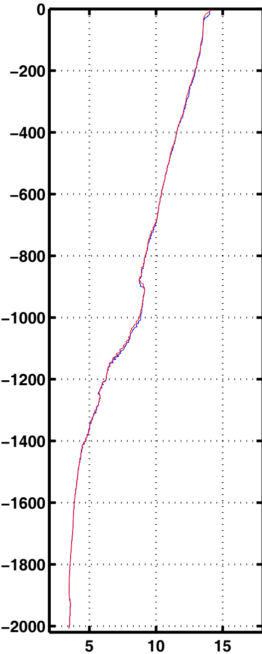
Tempe 2063
