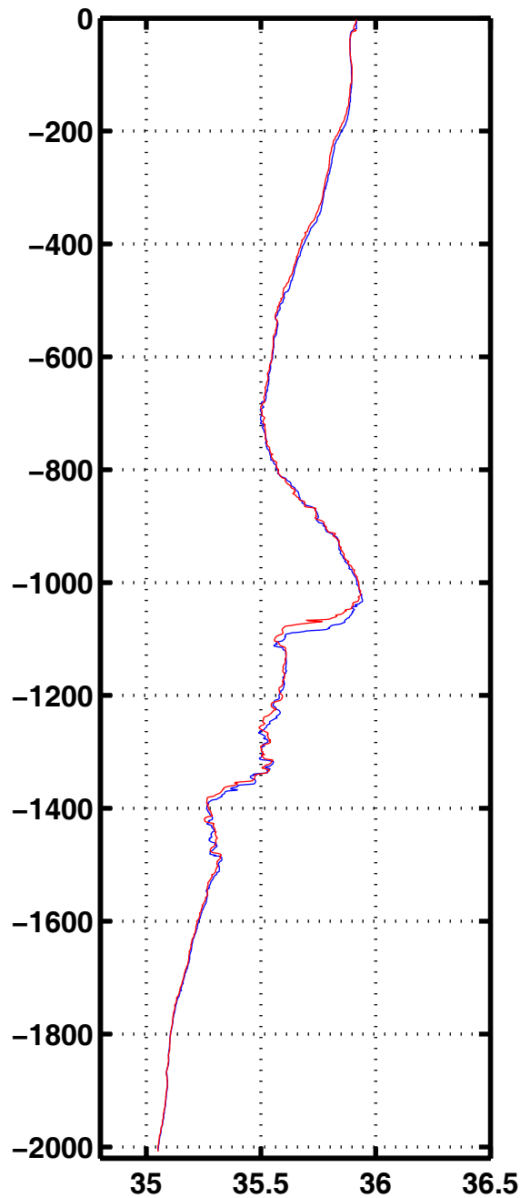
Sali 2072
