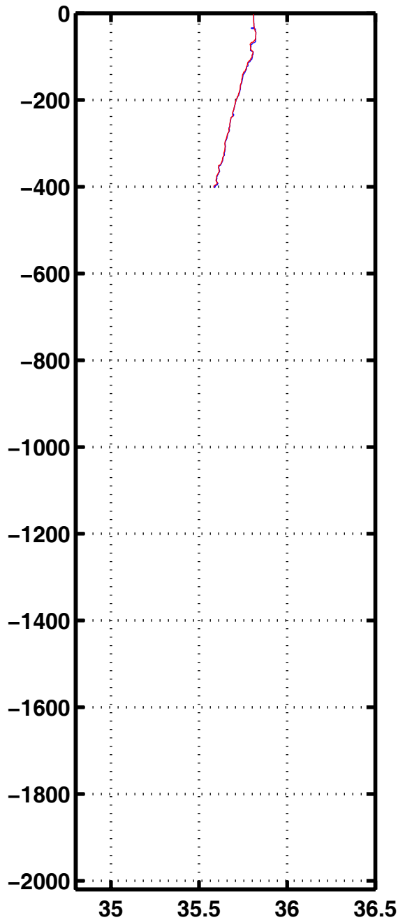
Sali 2273
