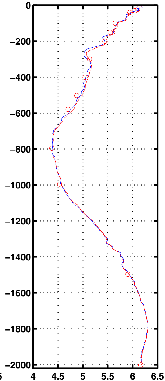
Oxyg 2065
