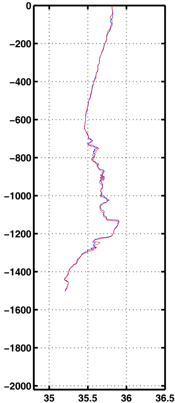
Sali 2269
