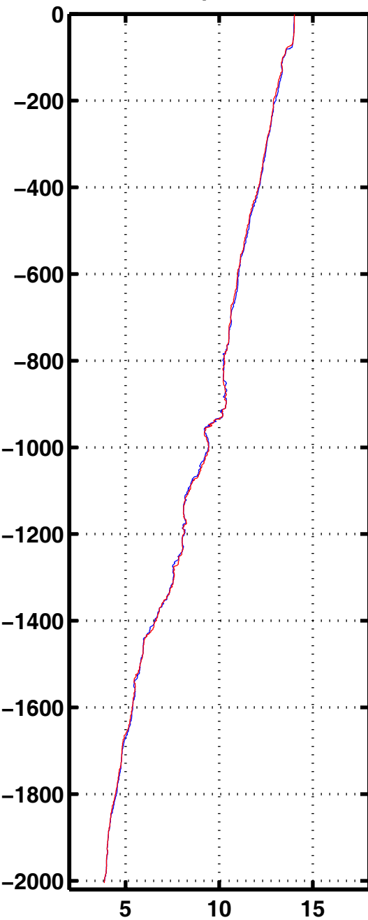
Tempe 2416
