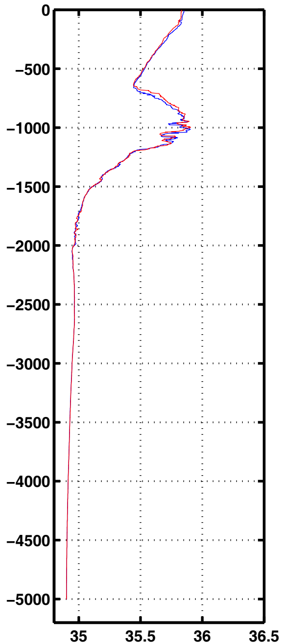
Sali 2038
