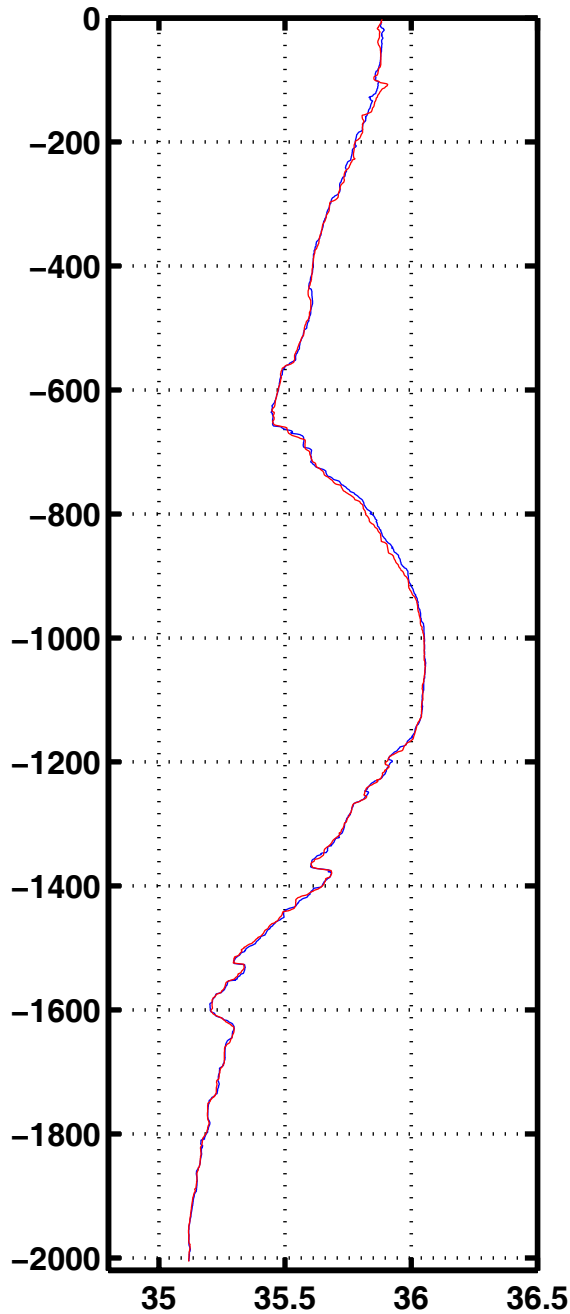
Sali 2079
