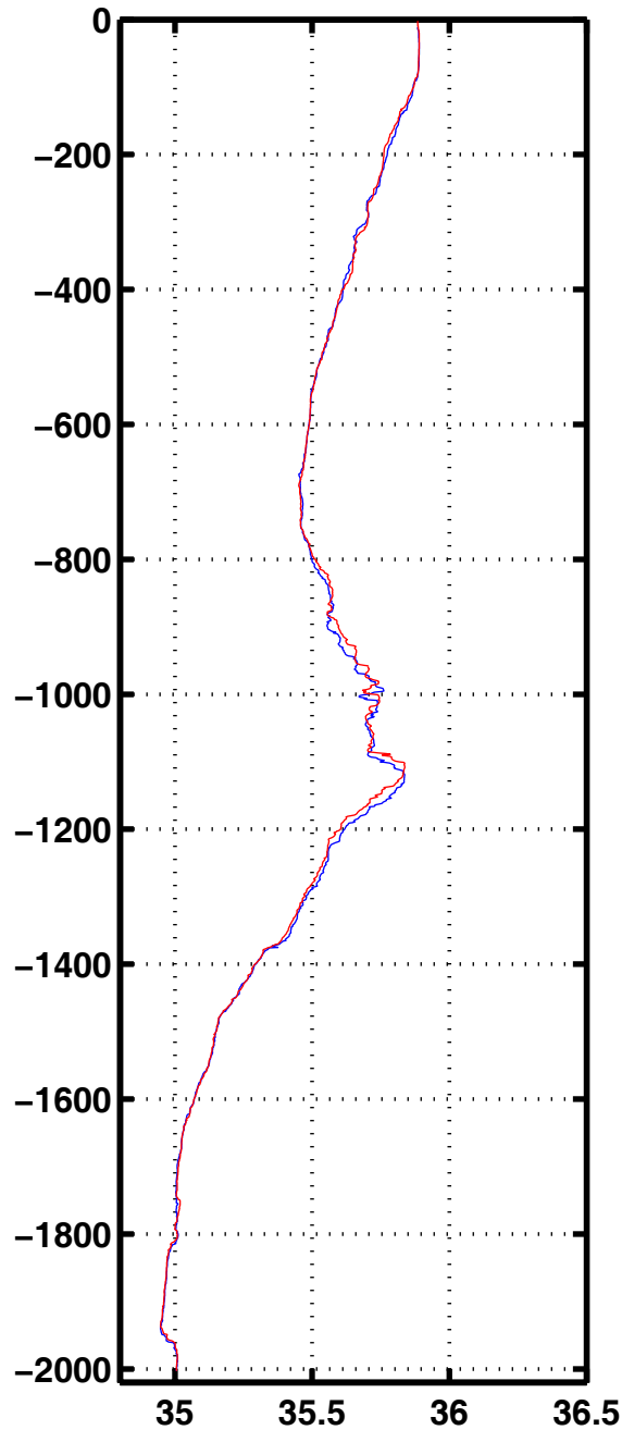
Sali 2006
