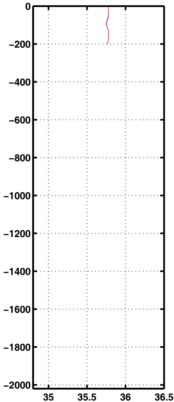
Sali 2401
