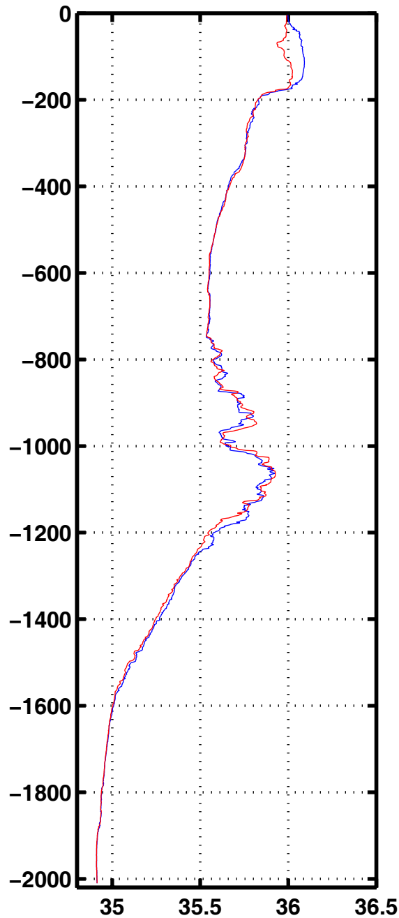
Sali 2068
