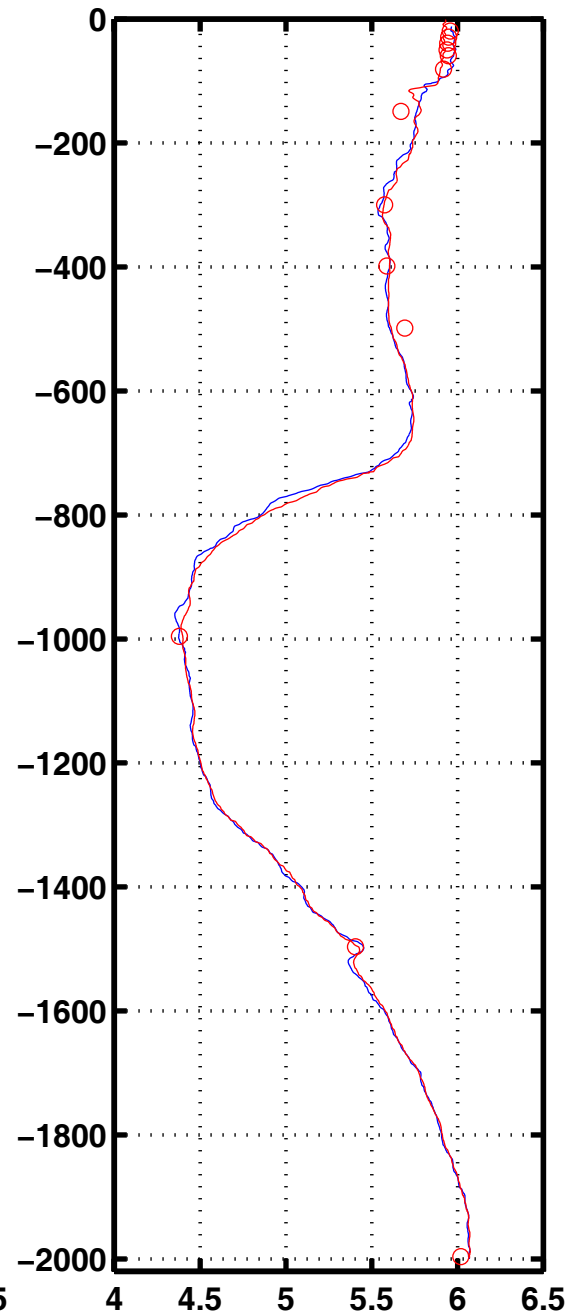
Oxyg 2041
