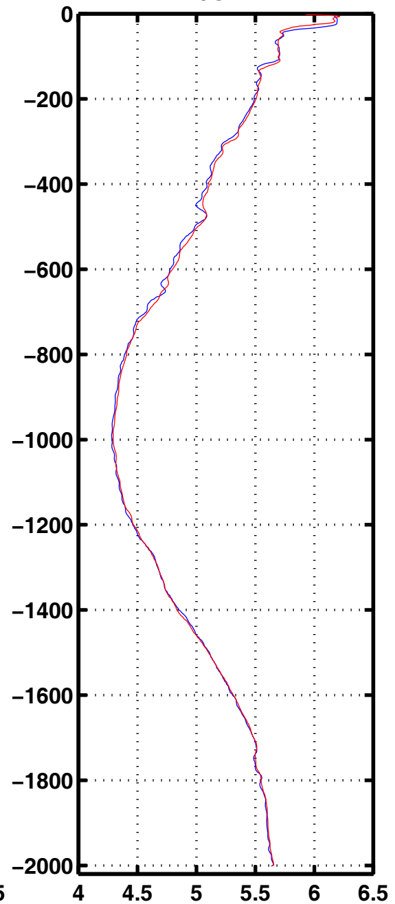
Oxyg 2095
