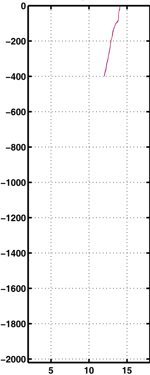
Tempe 2408
