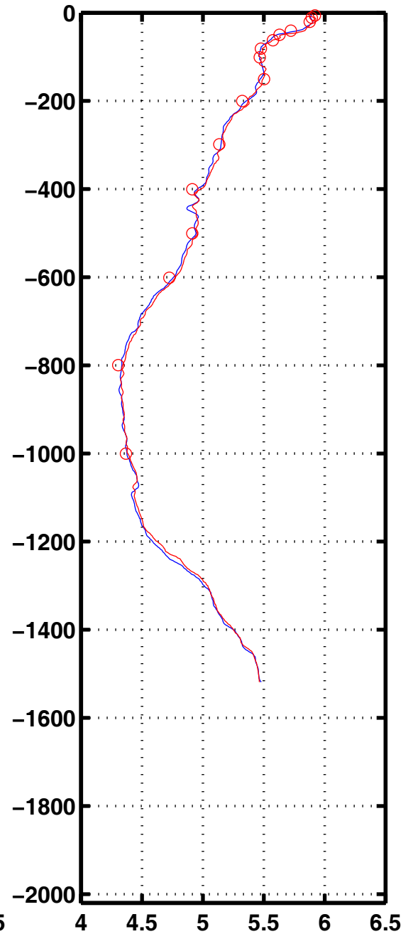
Oxyg 2267
