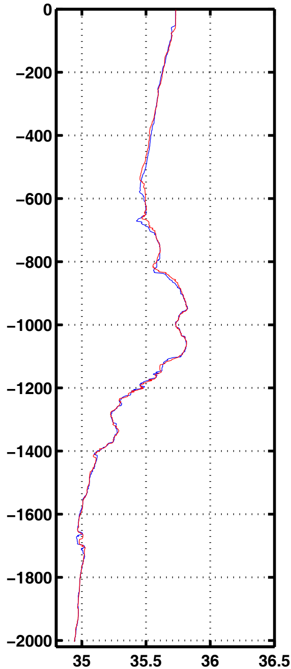
Sali 2024
