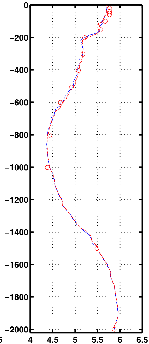
Oxyg 2002
