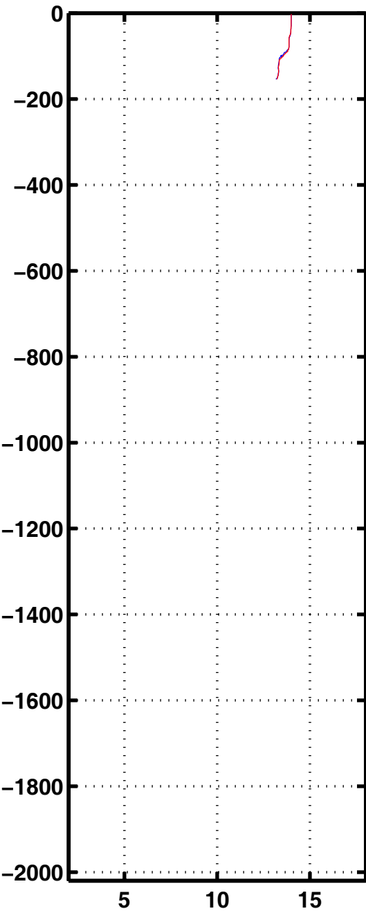
Tempe 2403
