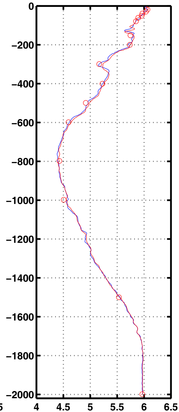
Oxyg 2008
