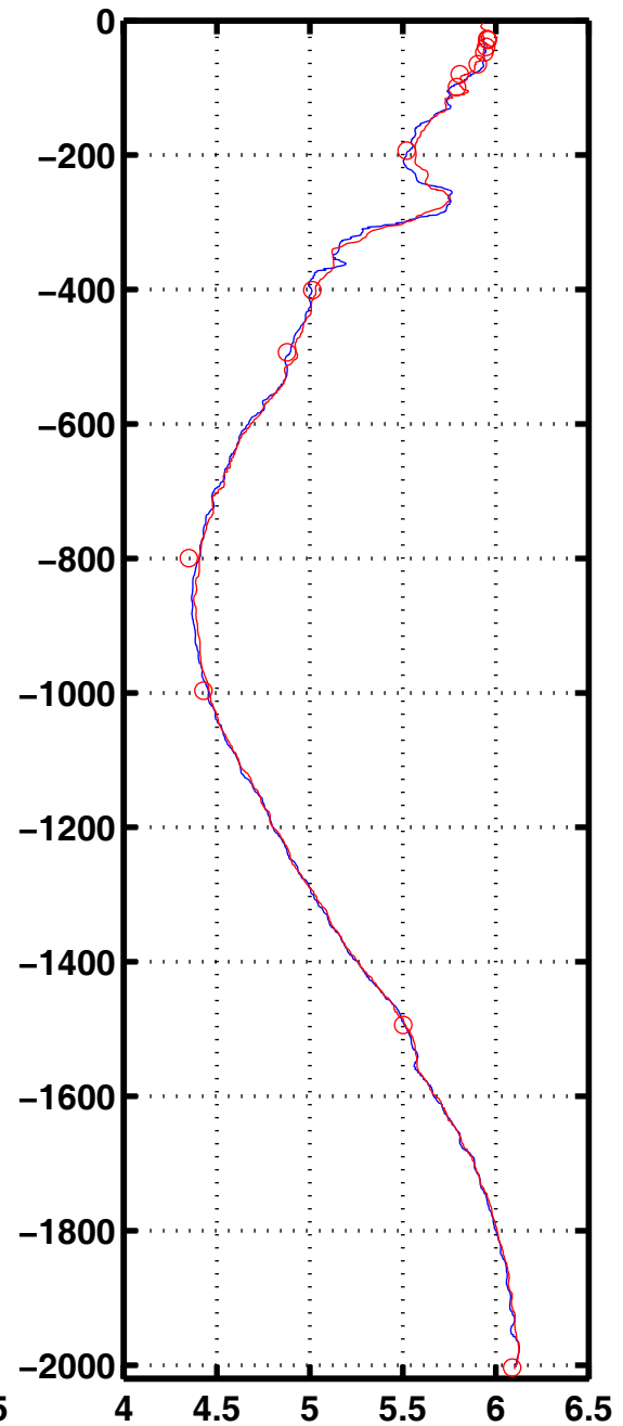
Oxyg 2016
