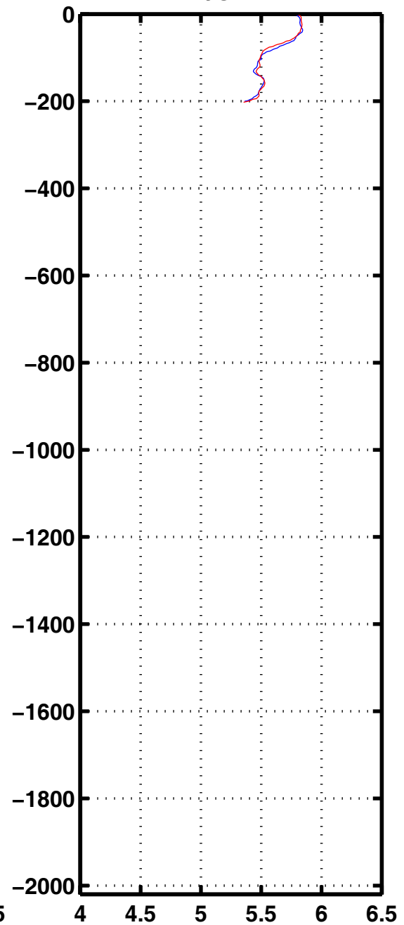
Oxyg 2265
