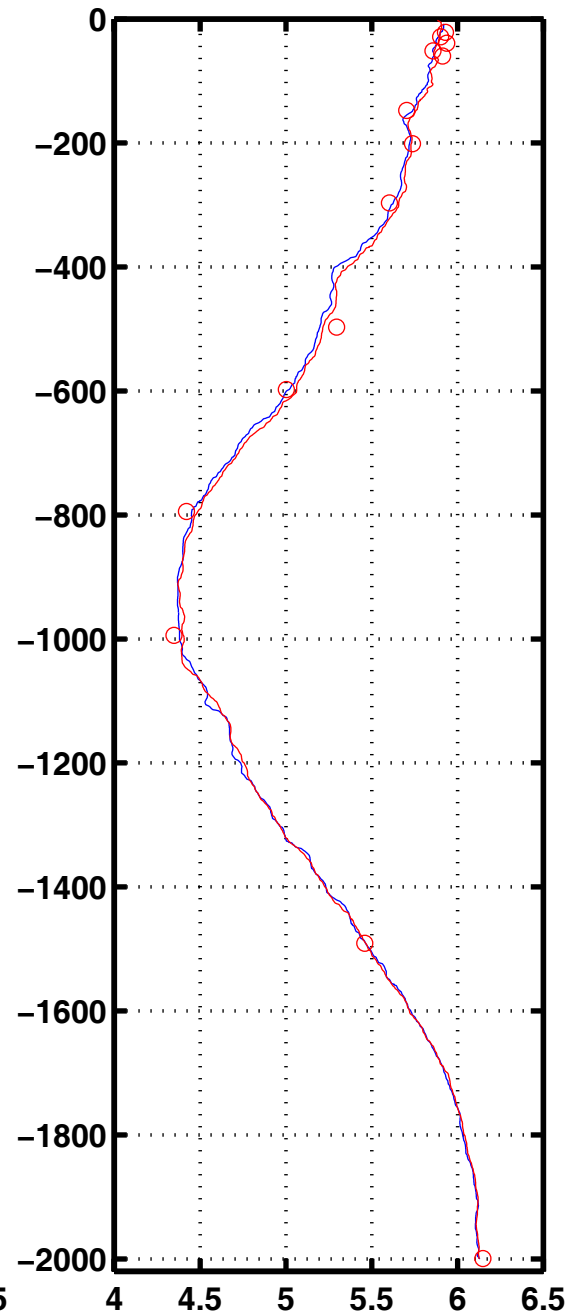
Oxyg 2043
