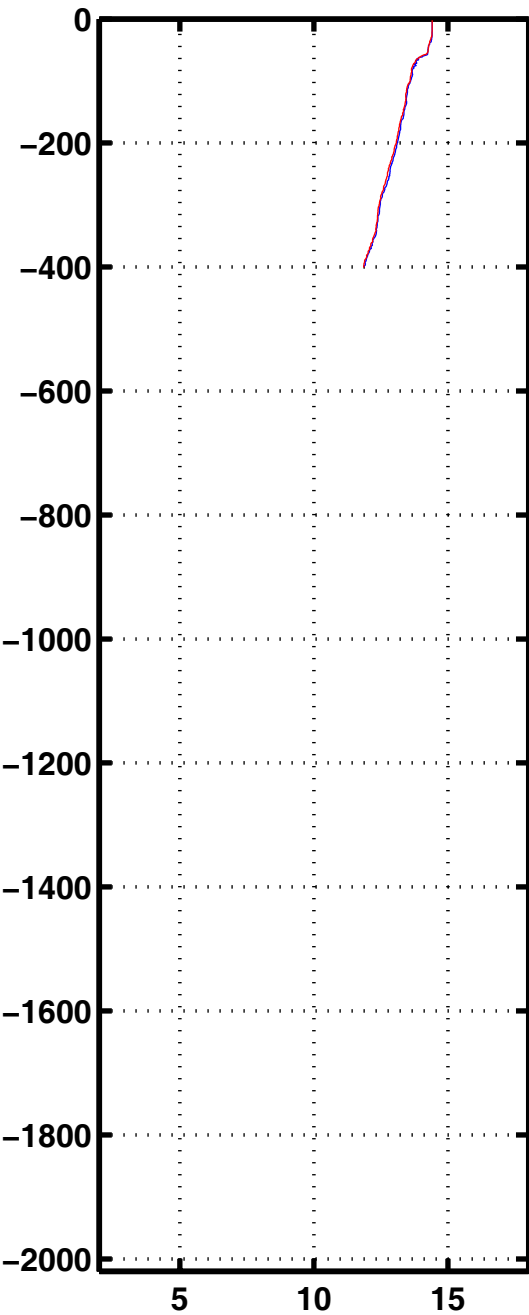
Tempe 2271
