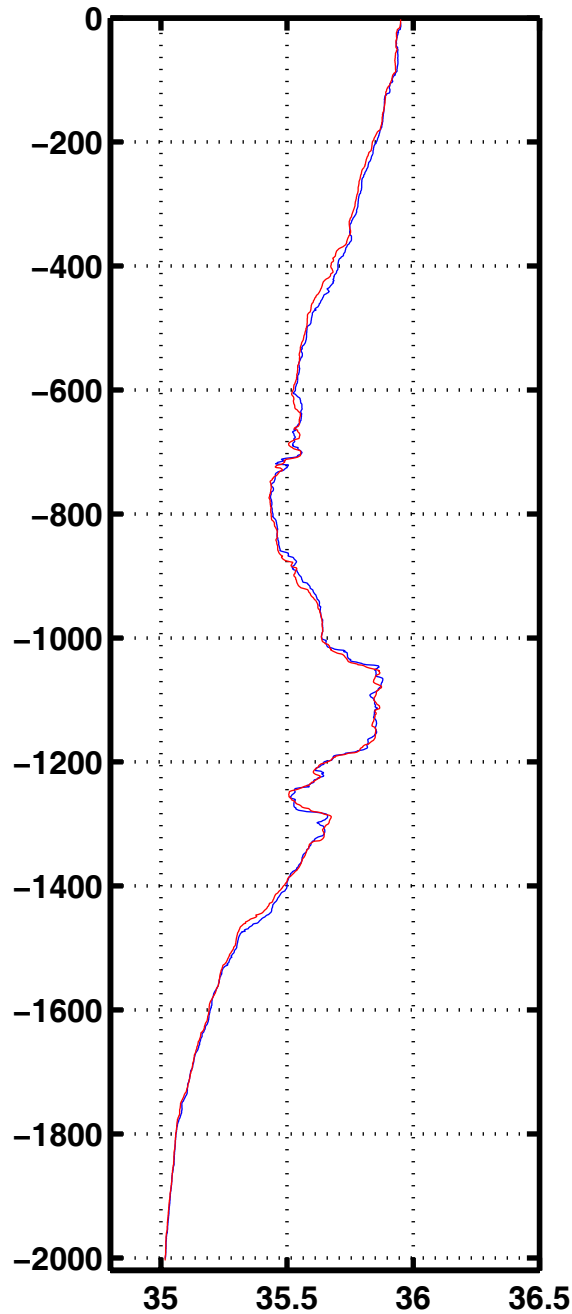
Sali 2074
