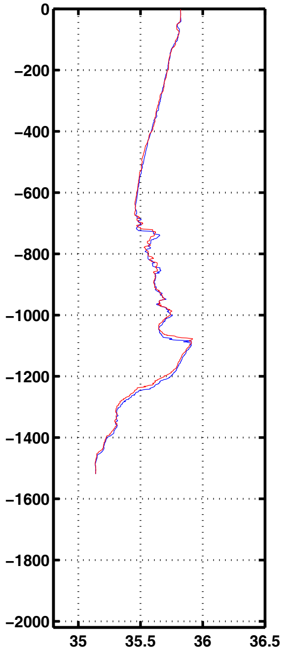
Sali 2267
