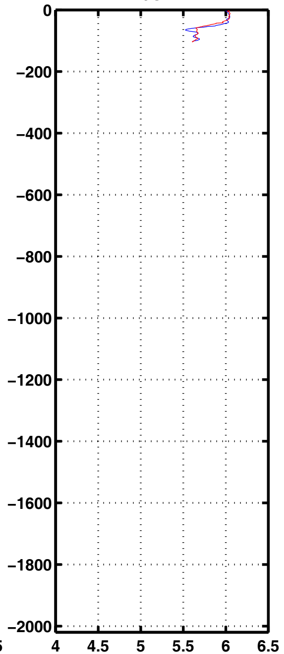
Oxyg 2178
