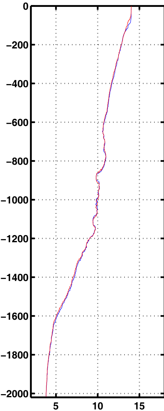
Tempe 2004
