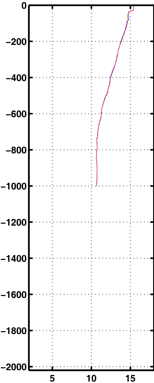
Tempe 2086
