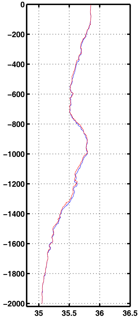
Sali 2001
