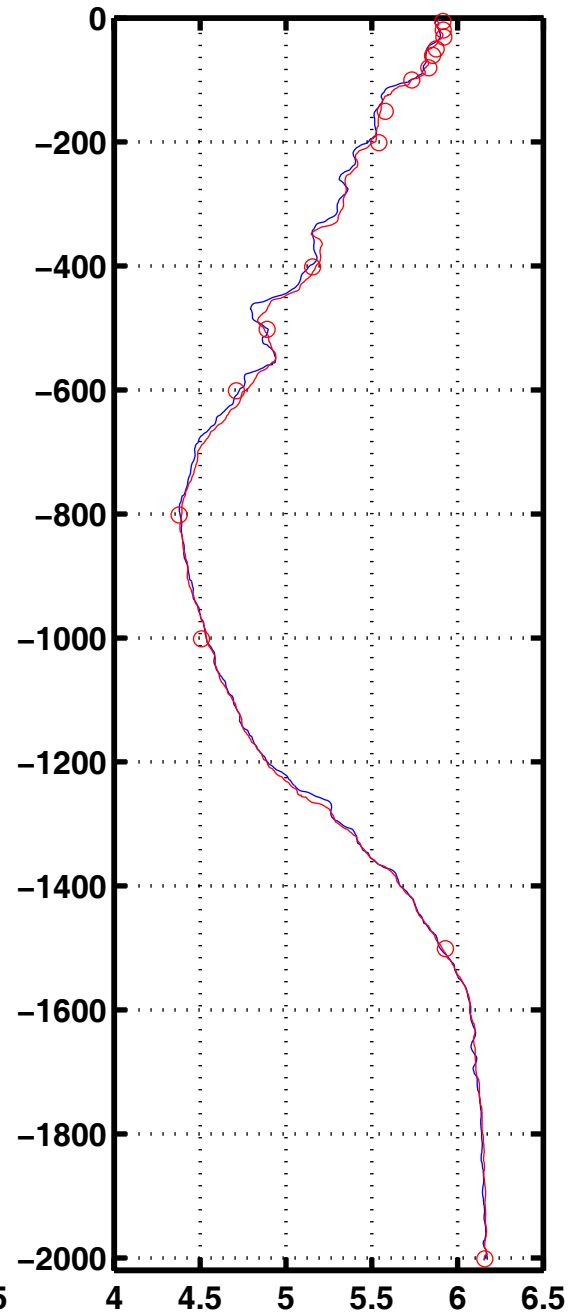
Oxyg 2058
