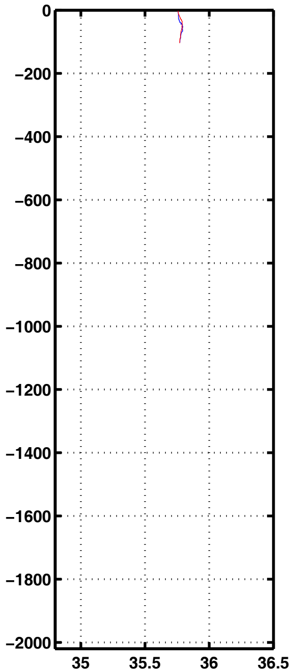
Sali 2178
