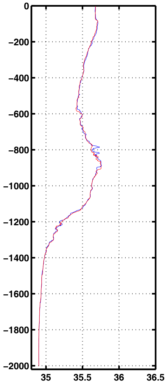
Sali 2047
