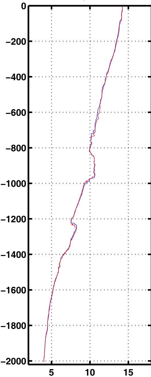
Tempe 2028
