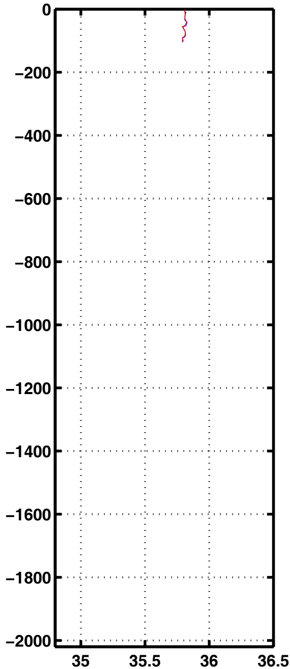
Sali 2277
