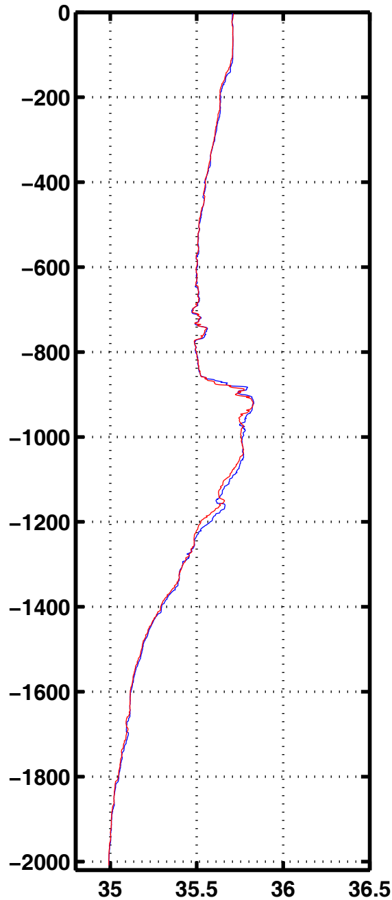
Sali 2007
