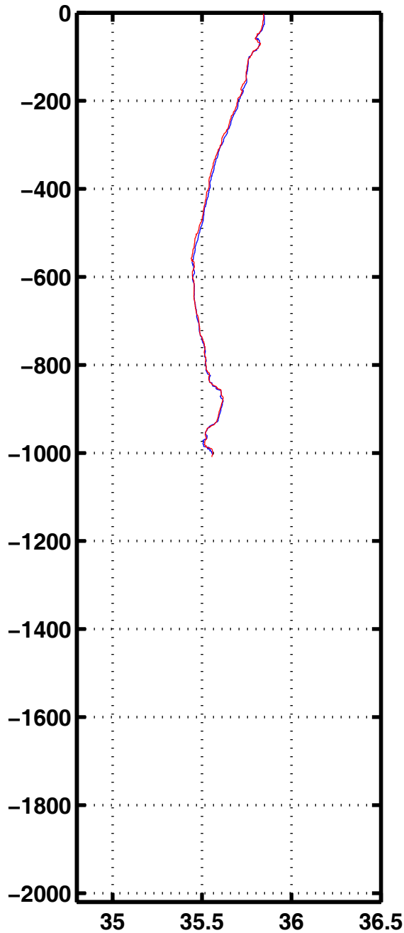
Sali 2175
