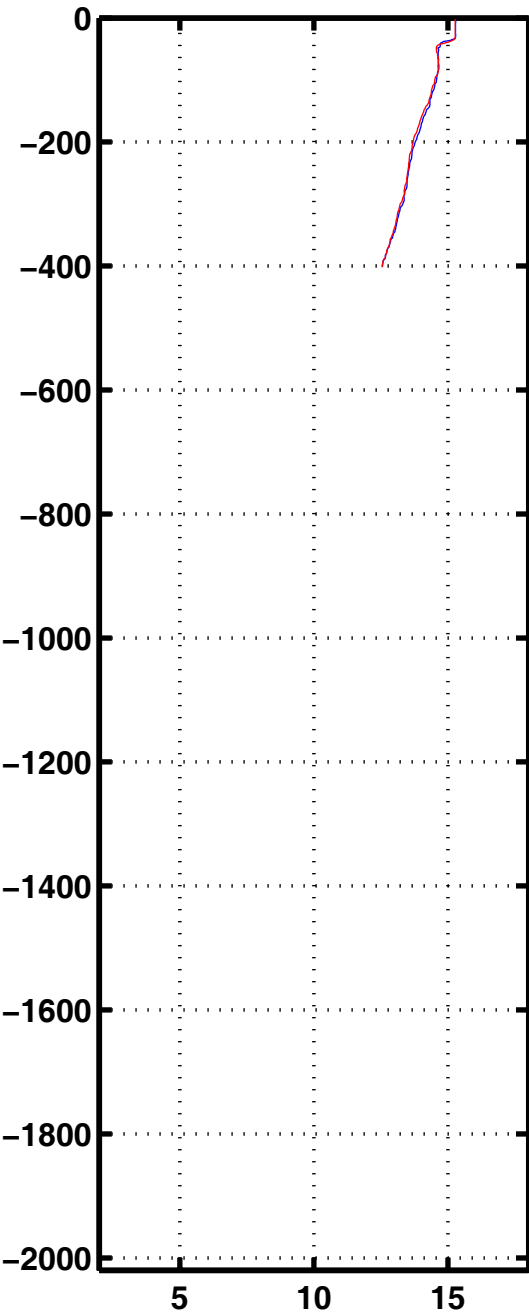
Tempe 2091
