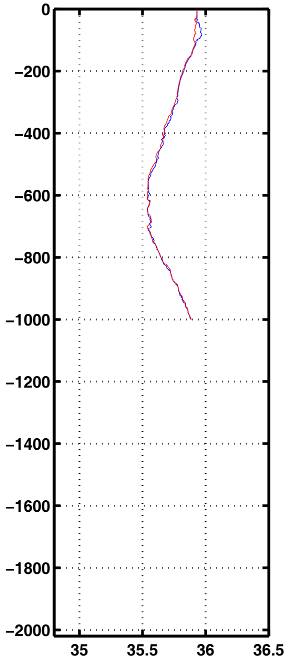
Sali 2088
