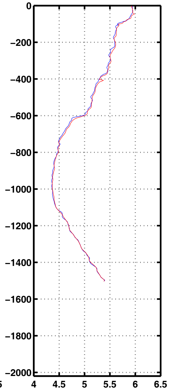
Oxyg 2402
