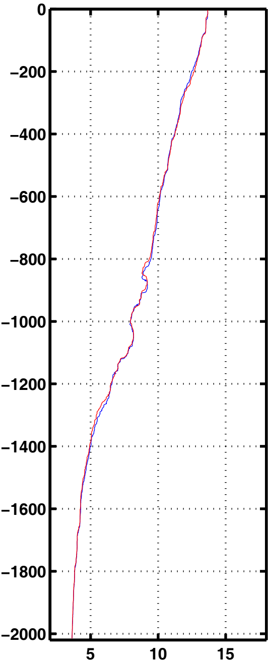
Tempe 2051
