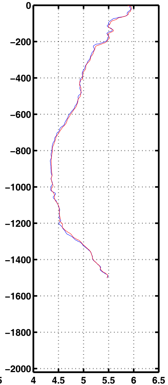
Oxyg 2266
