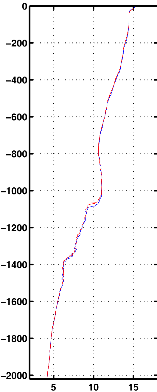
Tempe 2072
