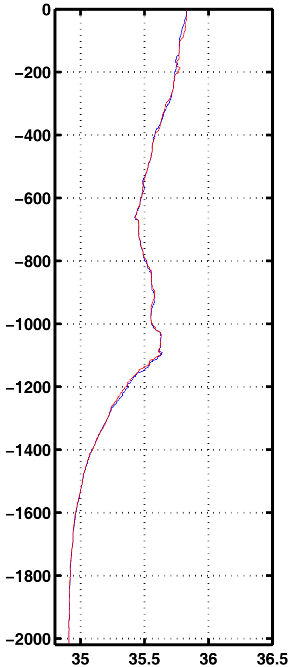
Sali 2054
