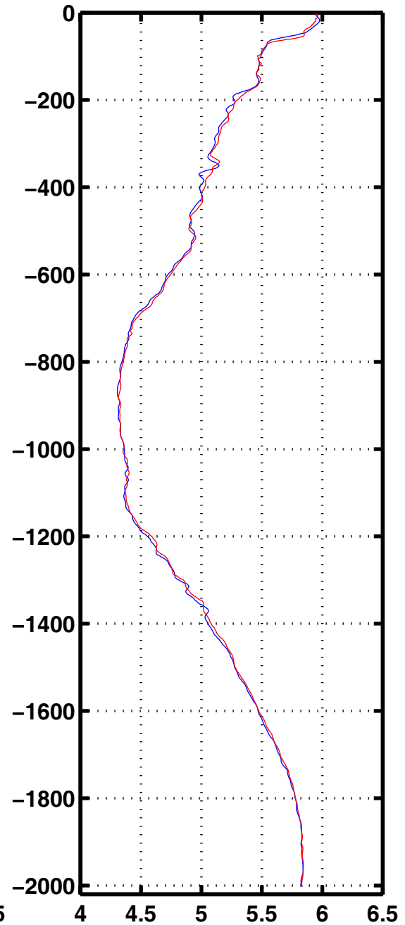
Oxyg 2278
