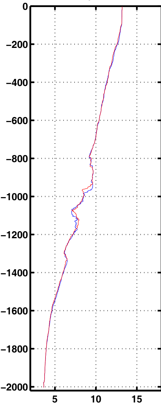
Tempe 2045
