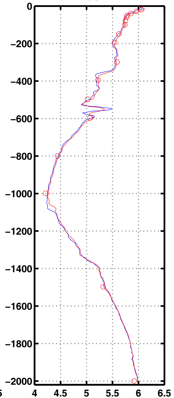
Oxyg 2072
