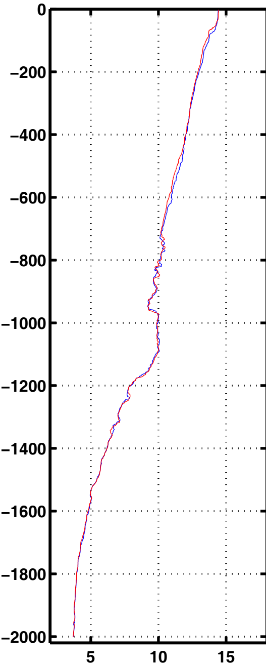
Tempe 2279
