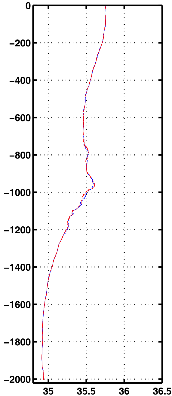
Sali 2064
