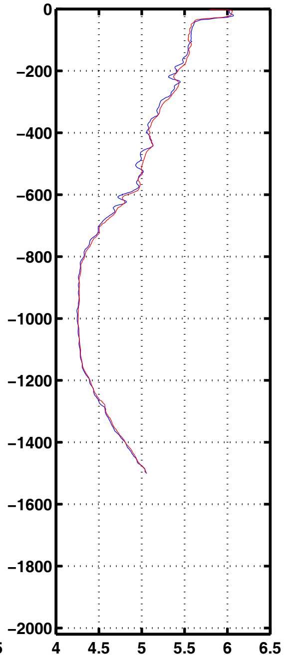
Oxyg 2084
