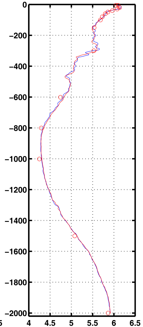
Oxyg 2080
