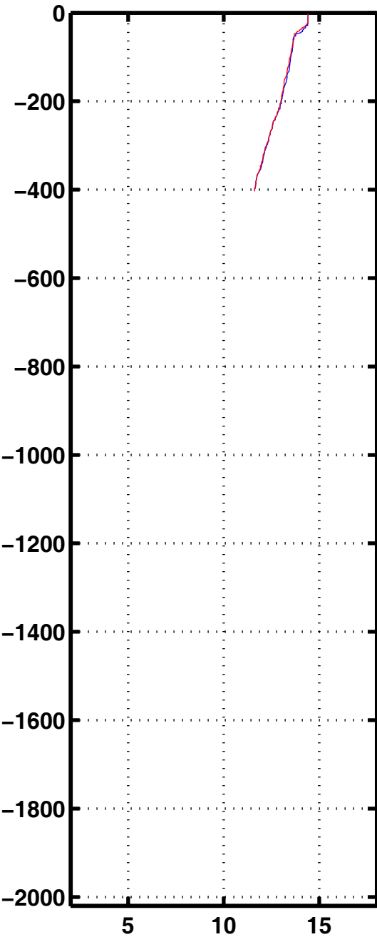
Tempe 2179
