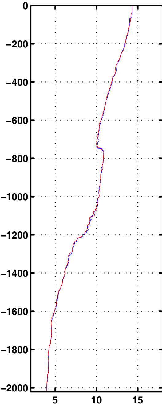
Tempe 2037
