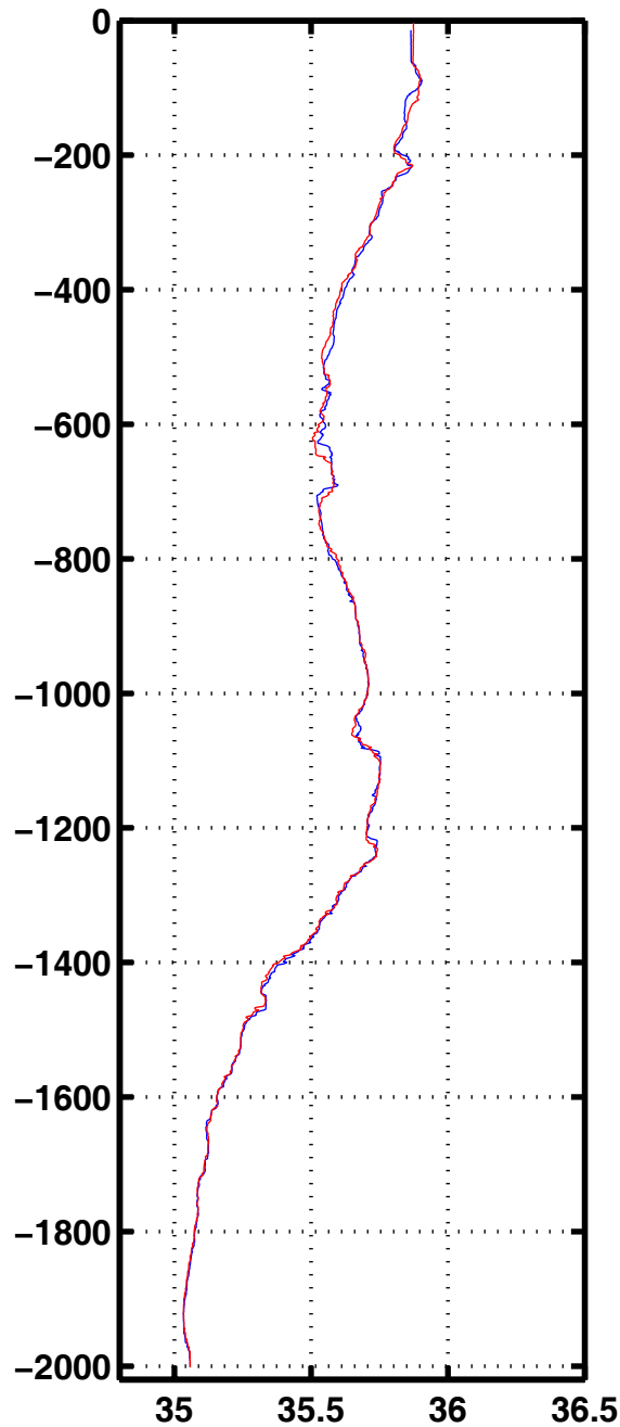
Sali 2002
