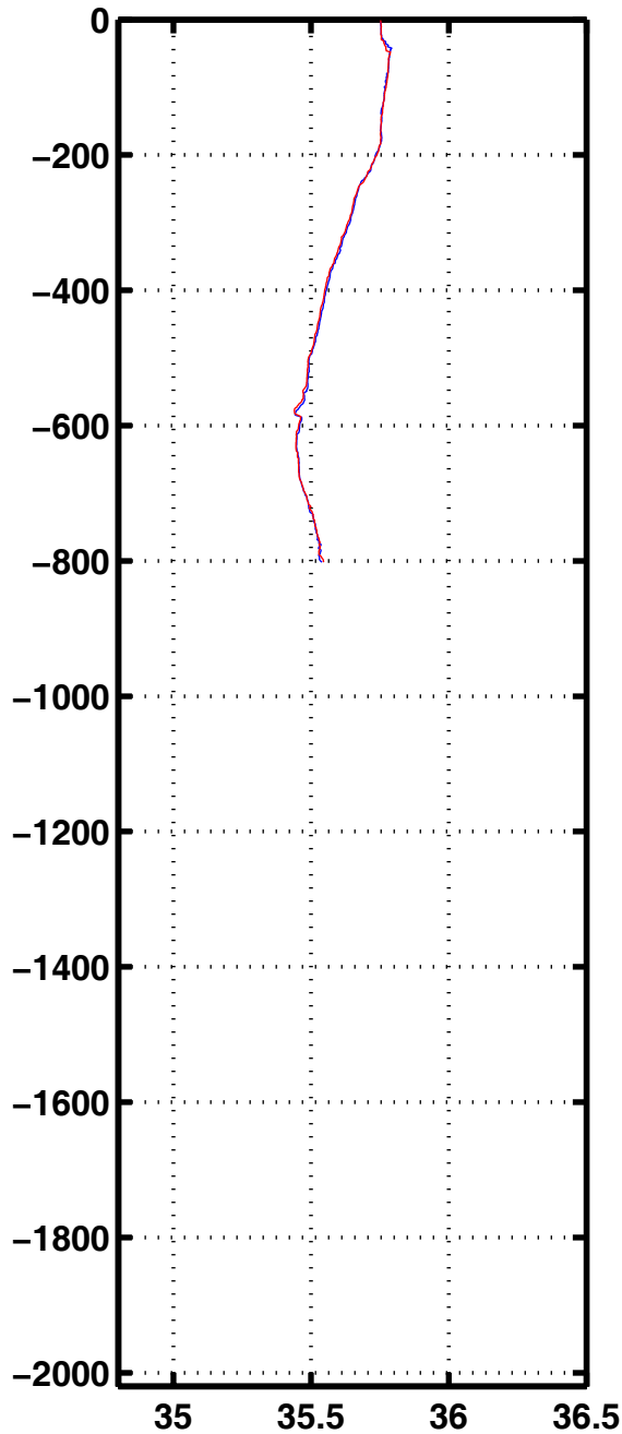
Sali 2180
