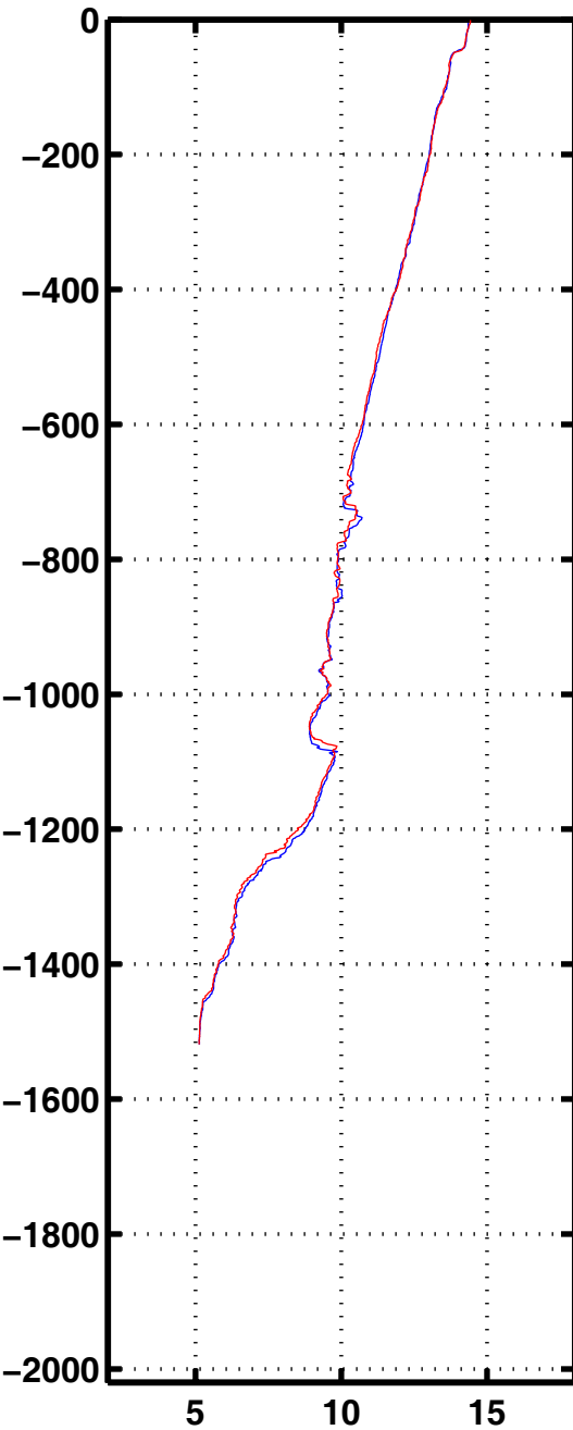
Tempe 2267
