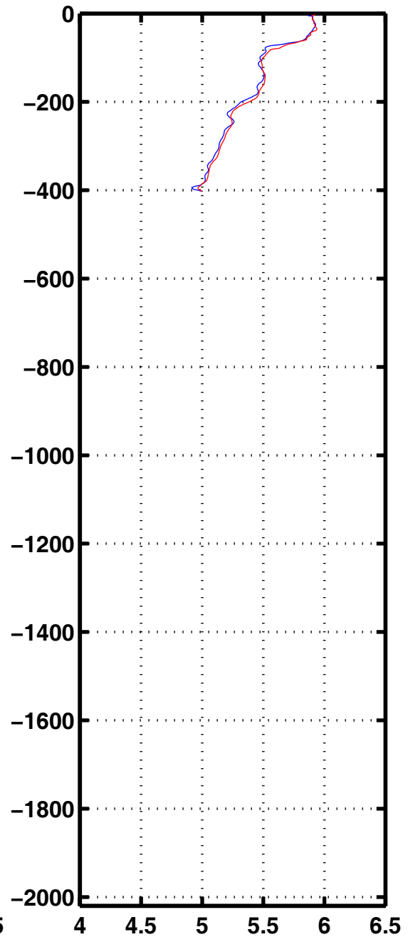
Oxyg 2273
