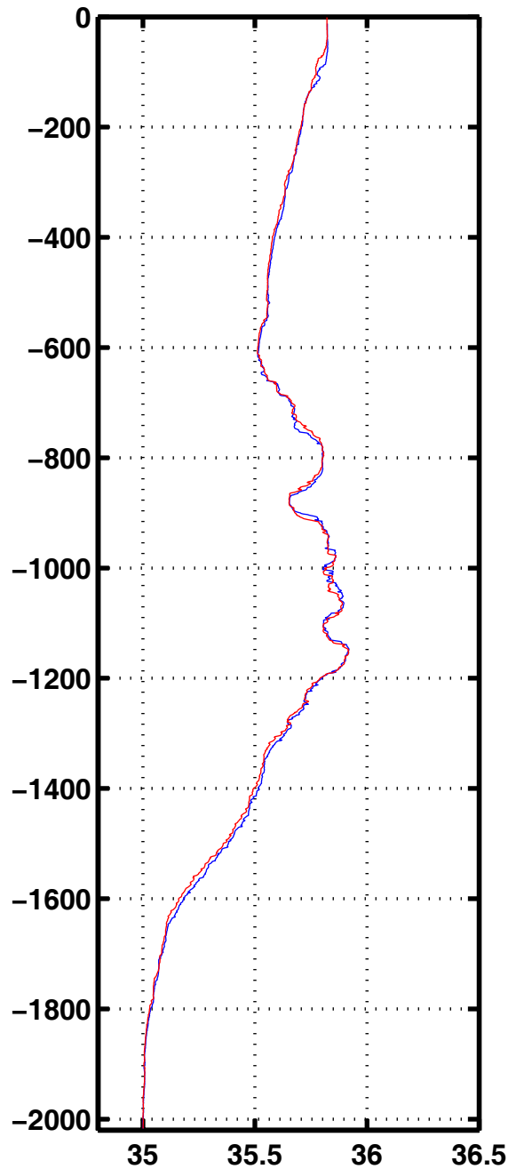
Sali 2004
