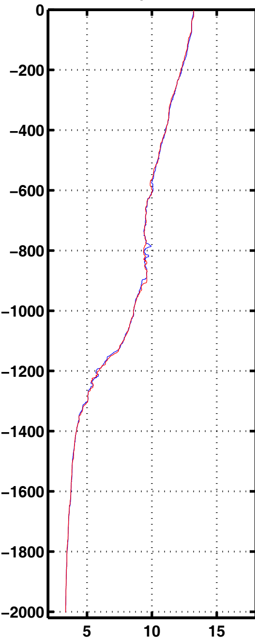
Tempe 2047
