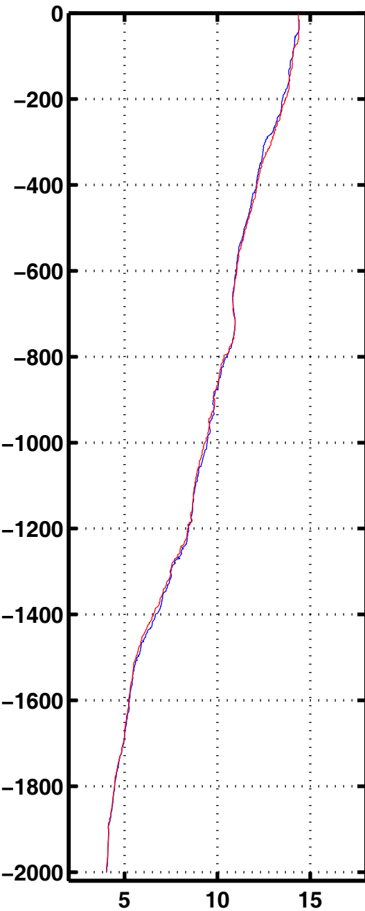
Tempe 2036
