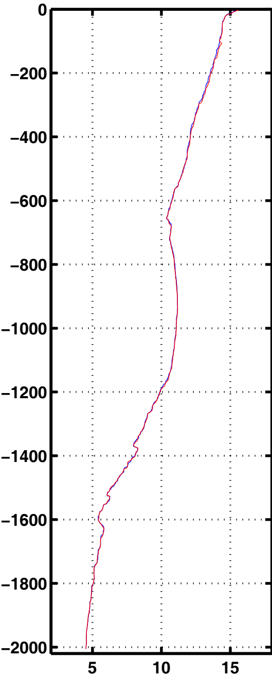
Tempe 2079
