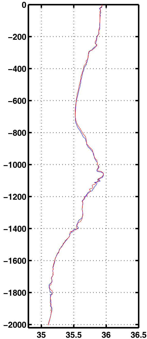
Sali 2082
