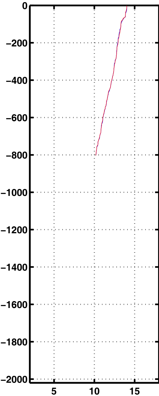
Tempe 2411
