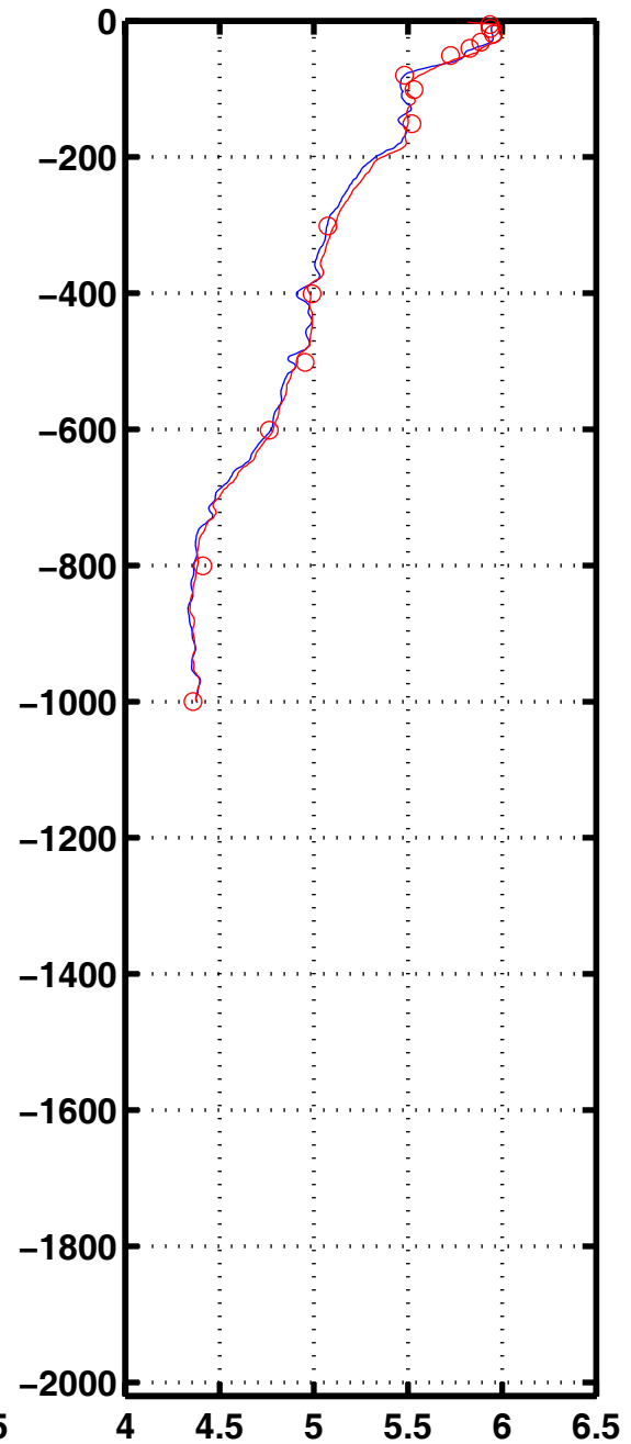
Oxyg 2276
