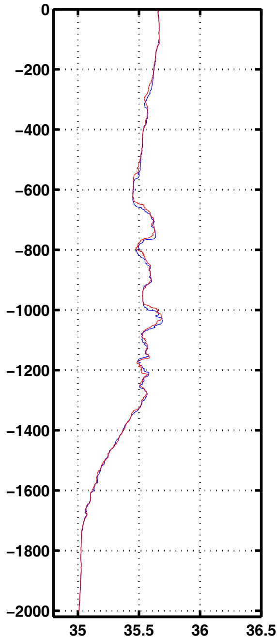
Sali 2008
