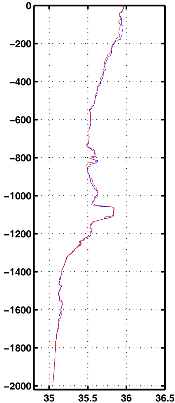
Sali 2073
