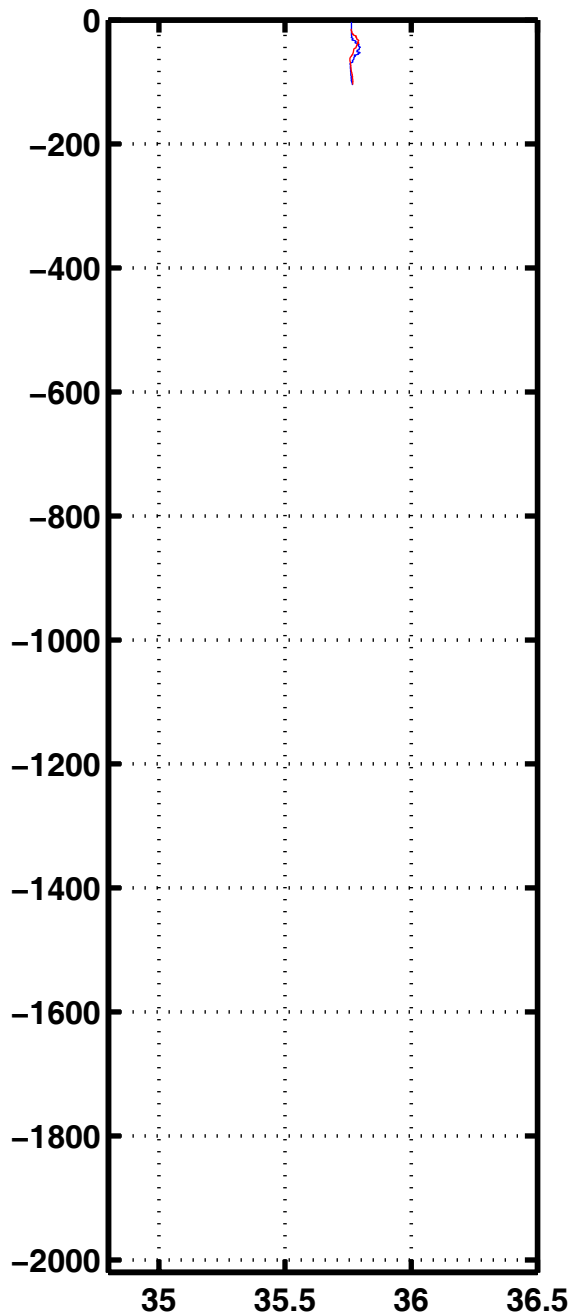
Sali 2177
