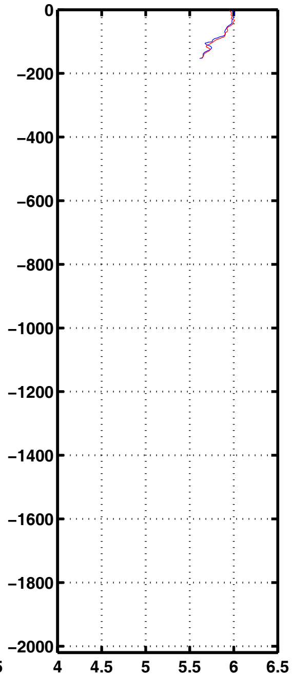
Oxyg 2403
