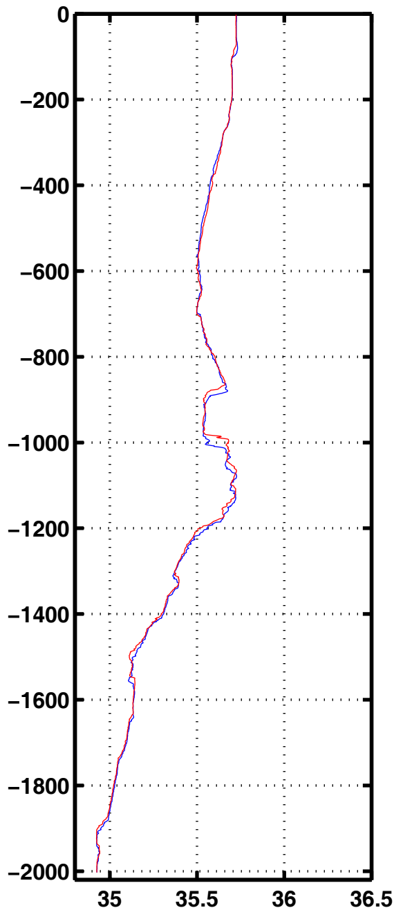
Sali 2026
