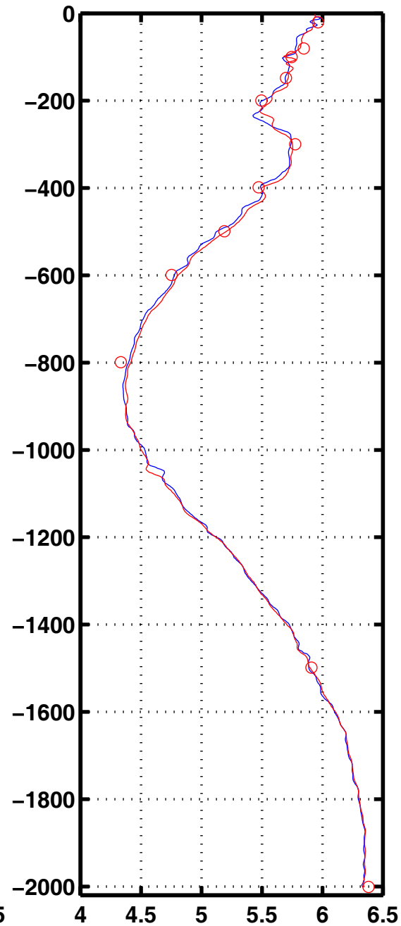
Oxyg 2012
