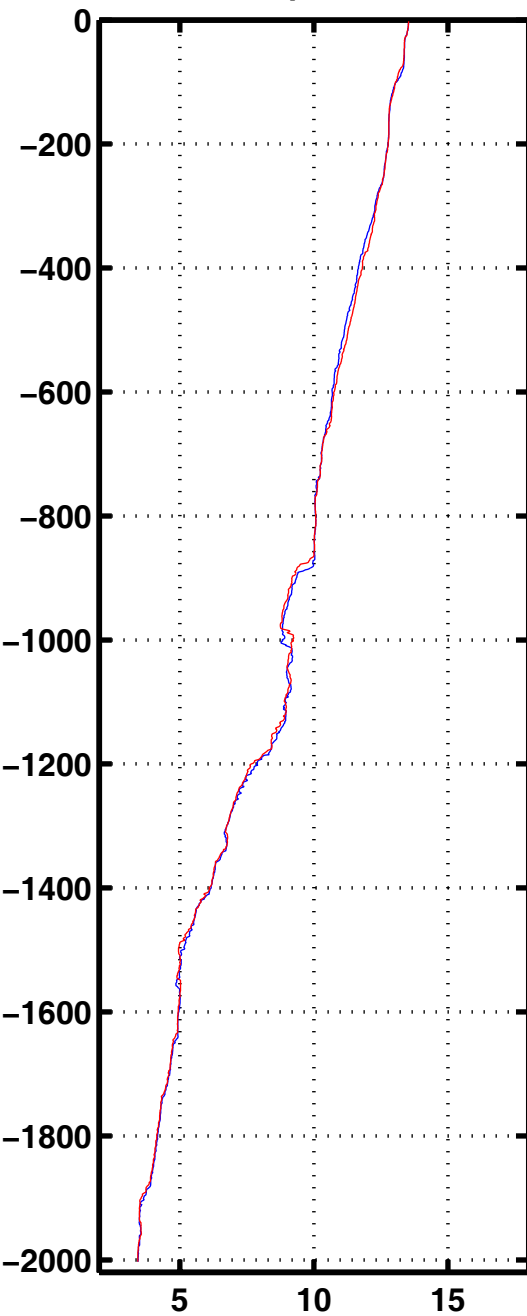
Tempe 2026
