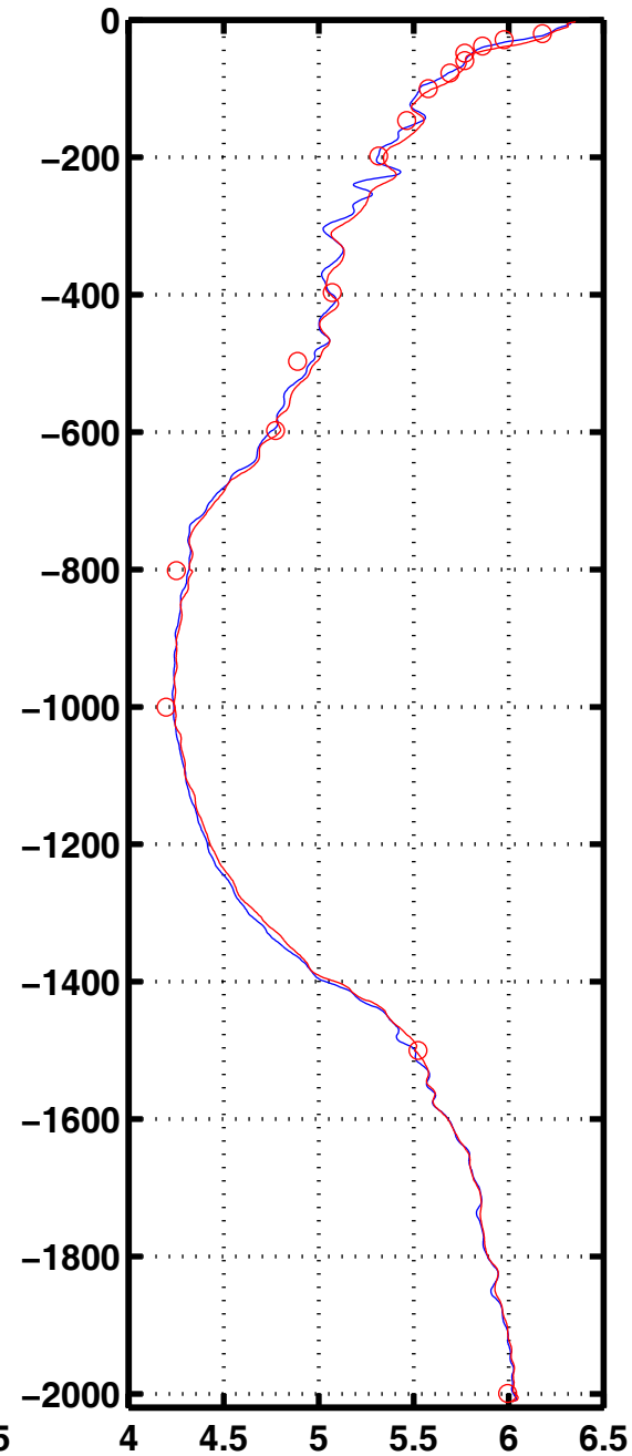
Oxyg 2075
