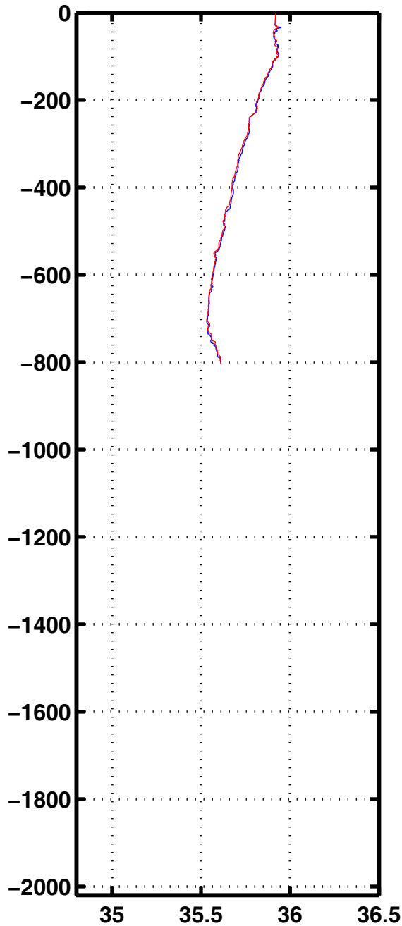
Sali 2092
