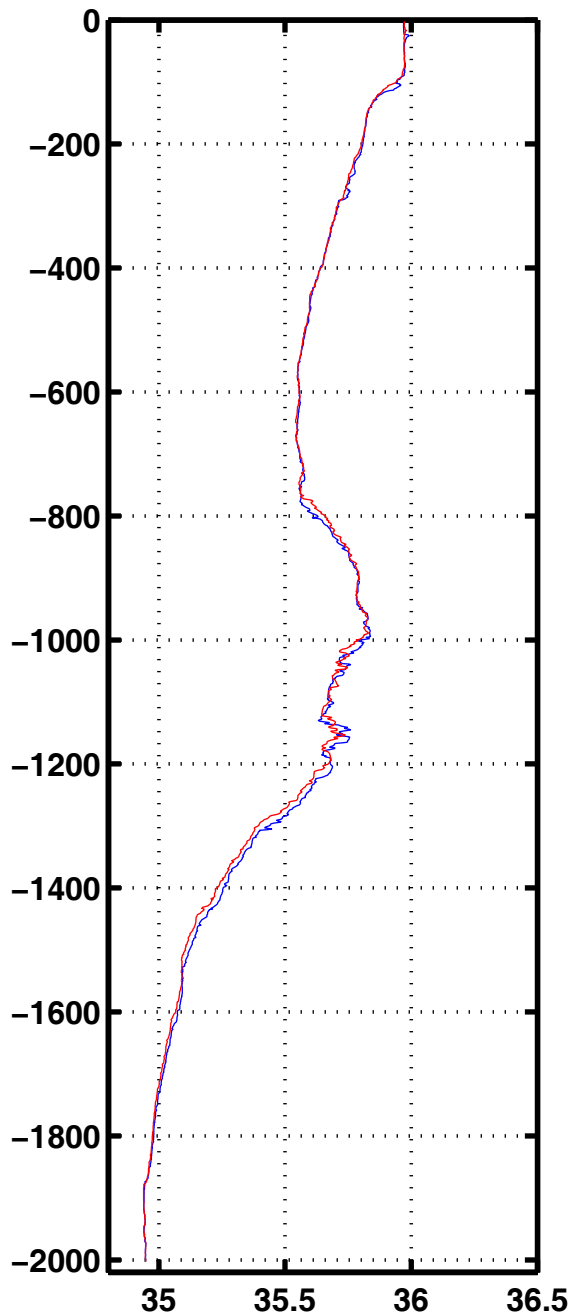
Sali 2069
