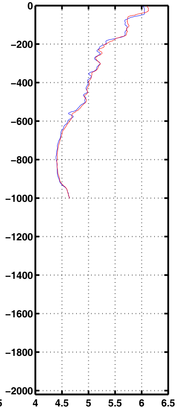
Oxyg 2172
