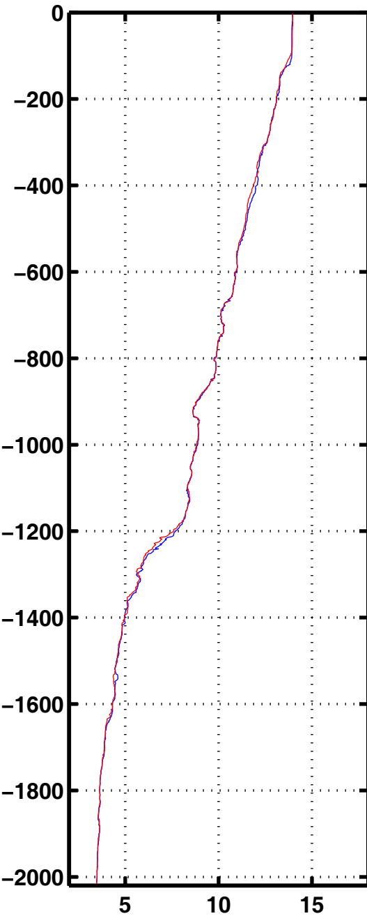
Tempe 2044
