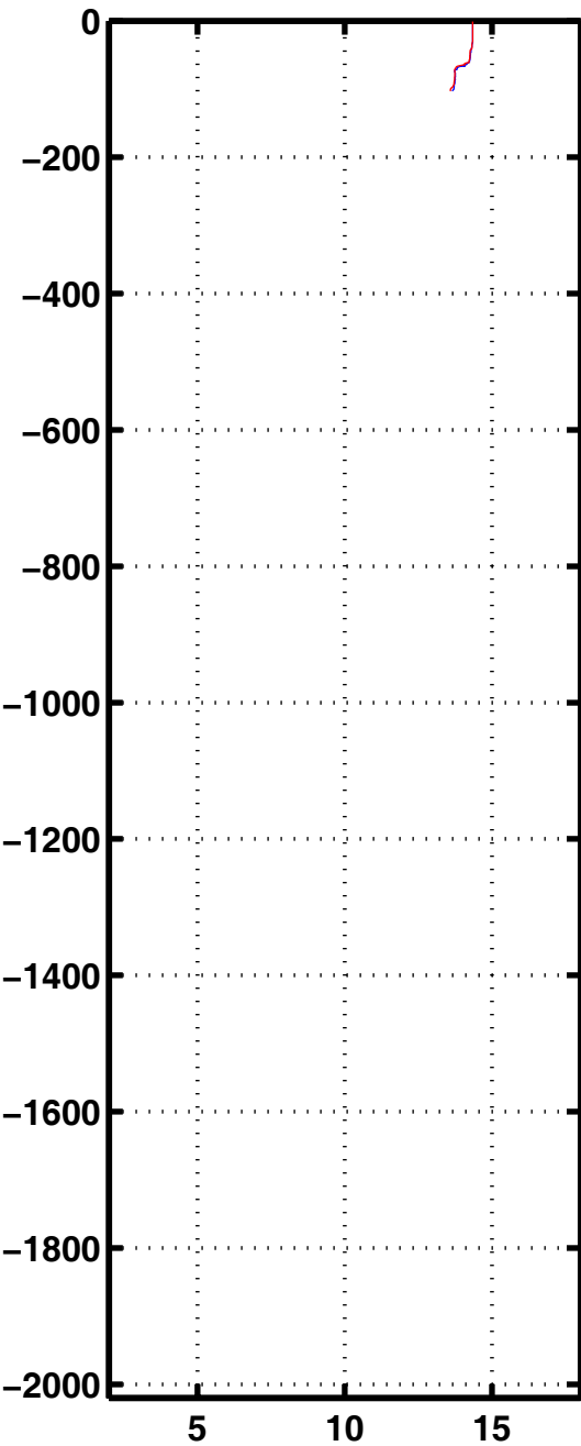
Tempe 2272
