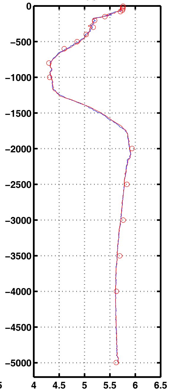
Oxyg 2003
