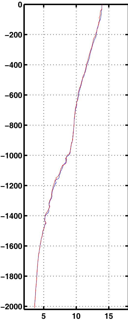
Tempe 2050
