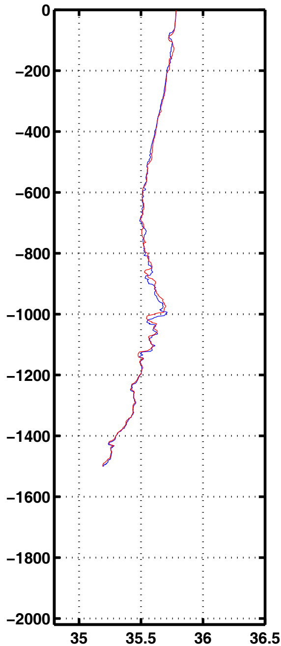
Sali 2406
