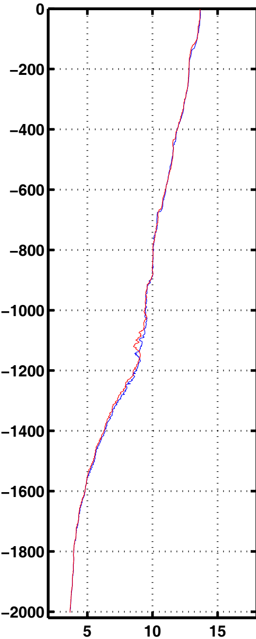
Tempe 2040
