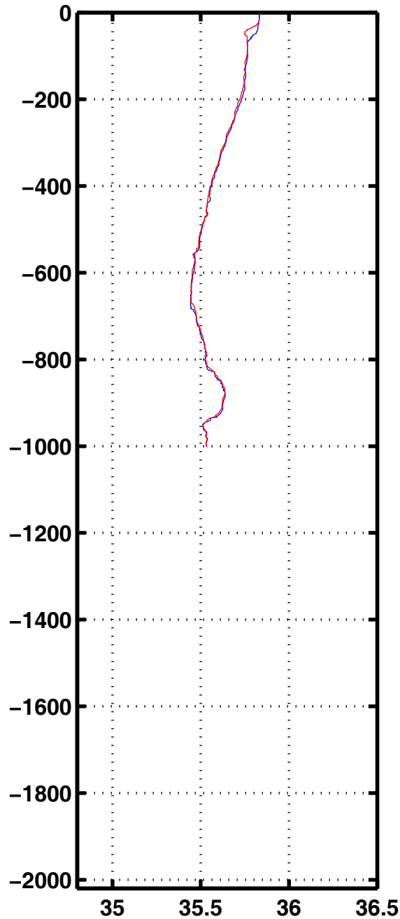
Sali 2172
