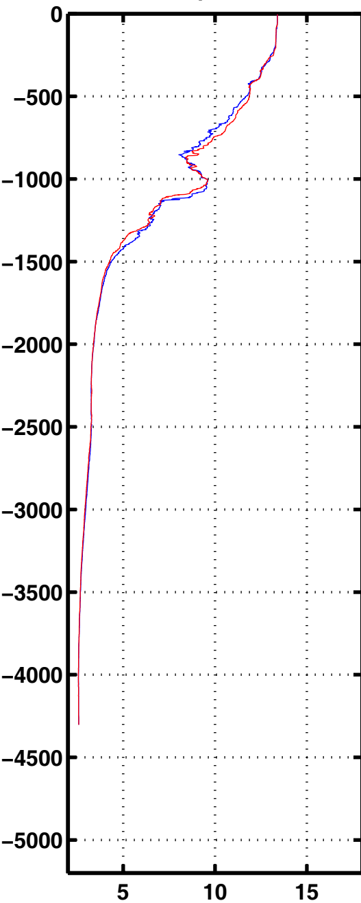
Tempe 2014
