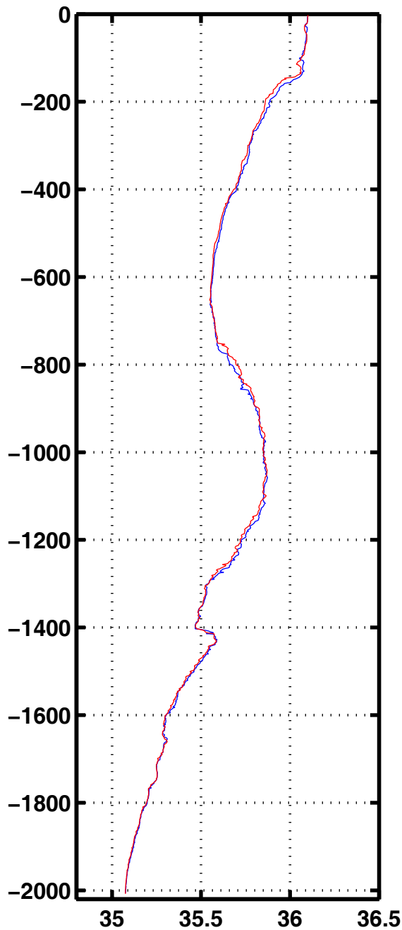
Sali 2070
