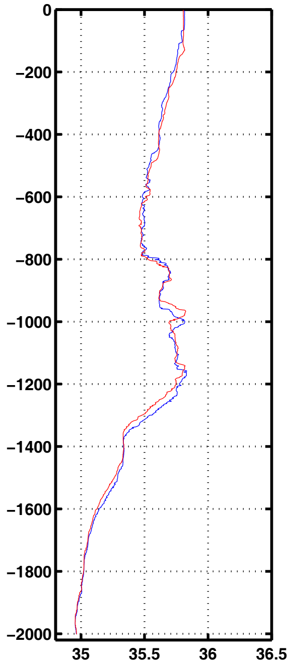
Sali 2021
