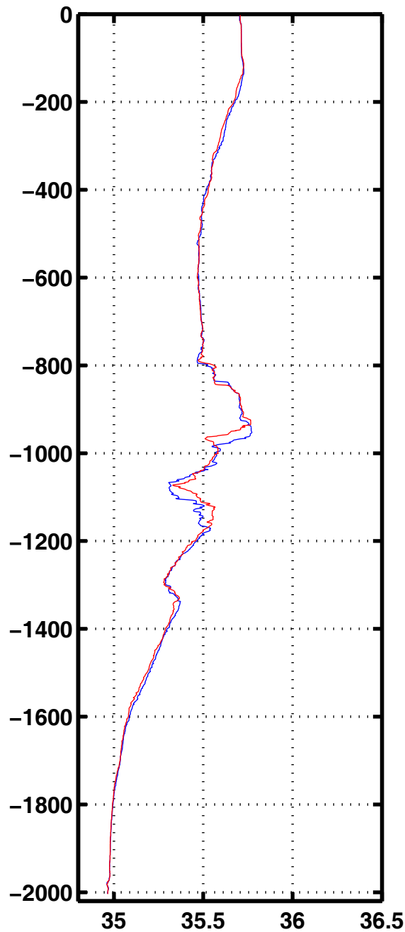
Sali 2045
