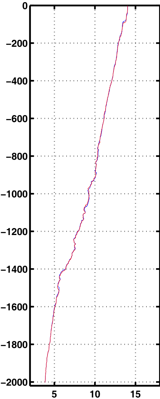
Tempe 2414
