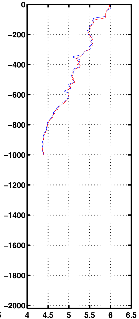
Oxyg 2407
