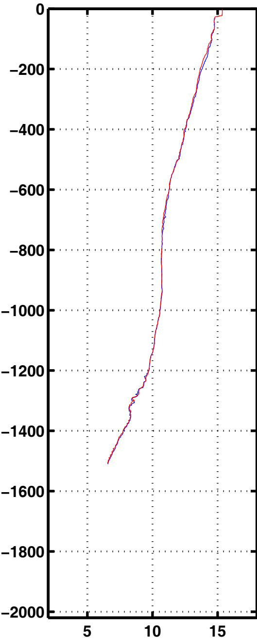
Tempe 2087
