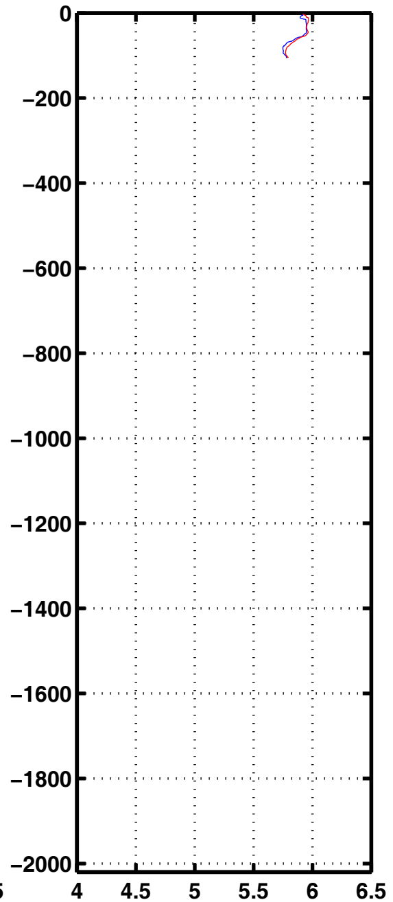
Oxyg 2415
