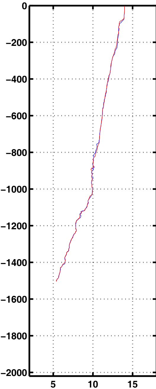
Tempe 2402
