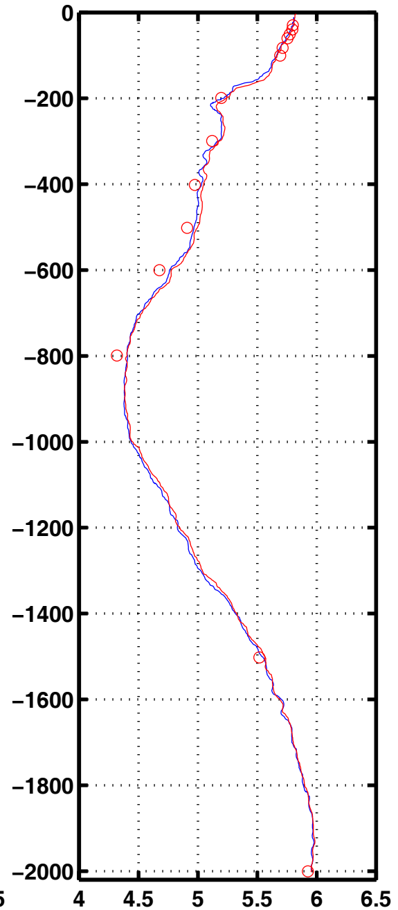
Oxyg 2001
