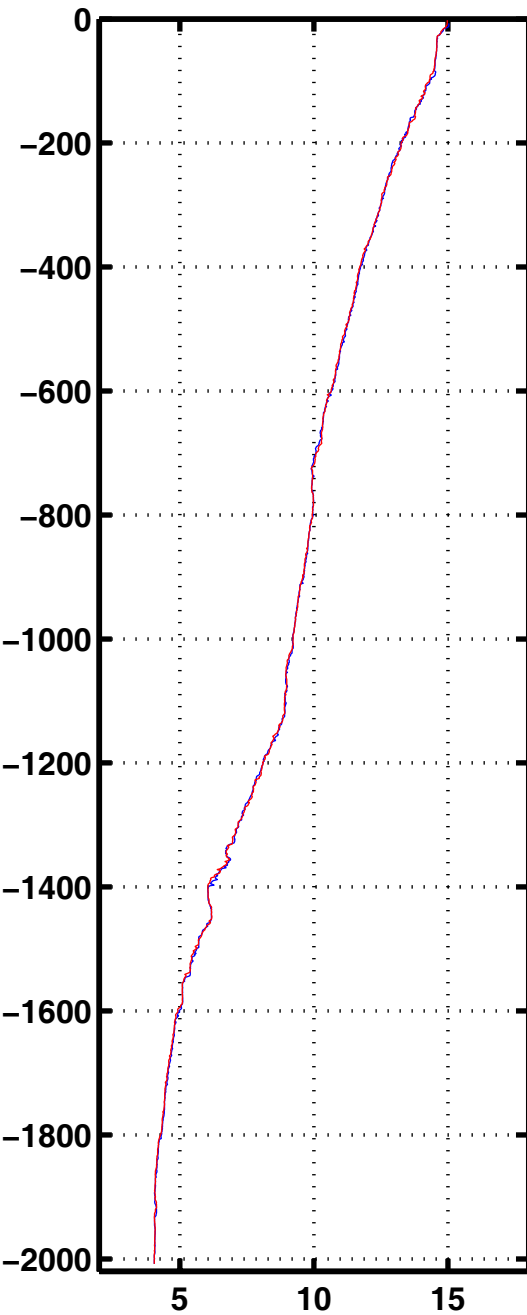
Tempe 2032
