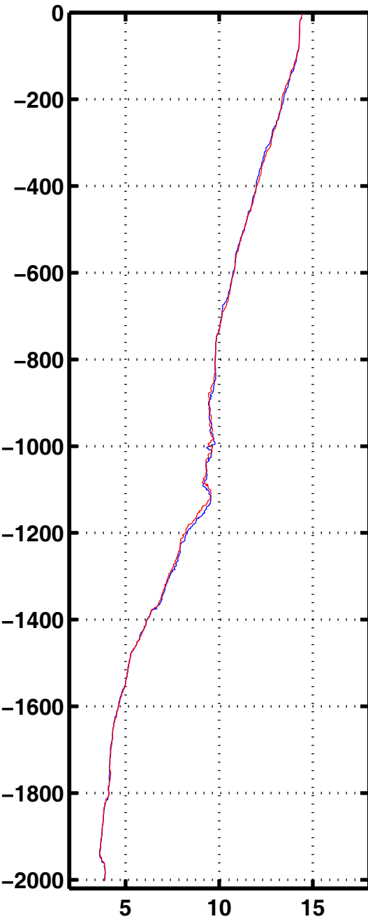
Tempe 2006
