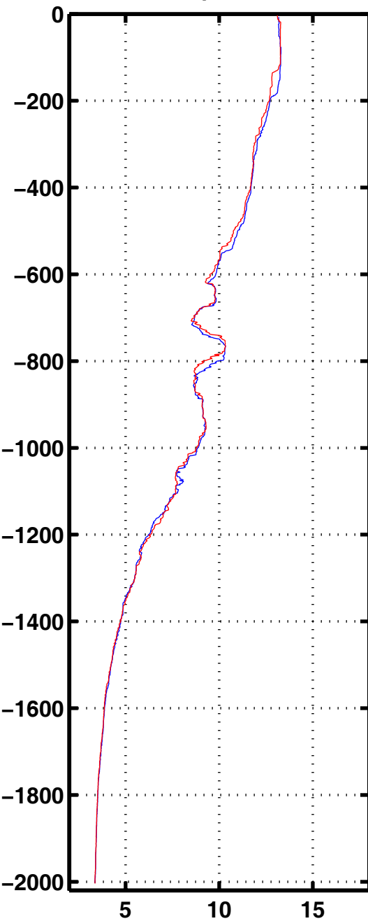
Tempe 2013
