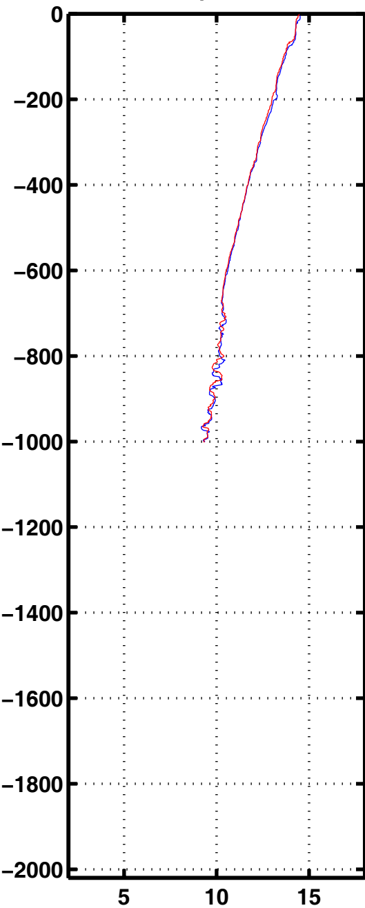
Tempe 2268
