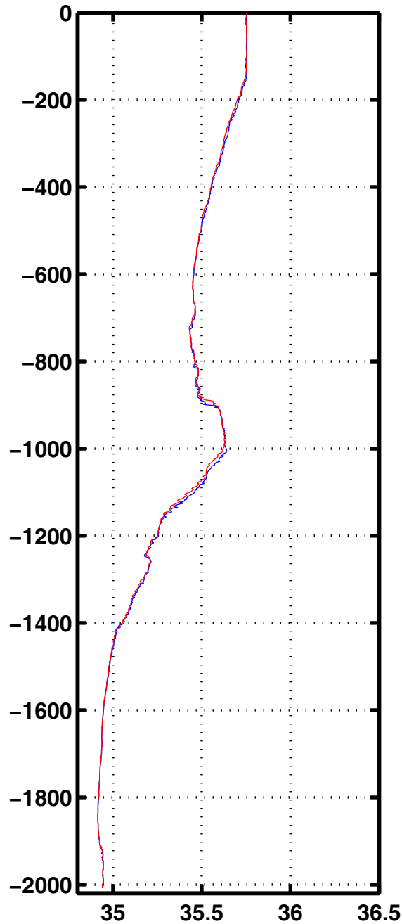
Sali 2063
