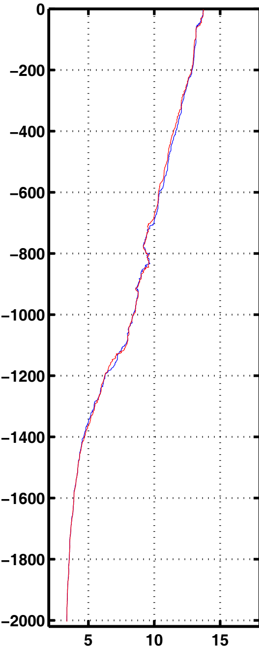
Tempe 2052
