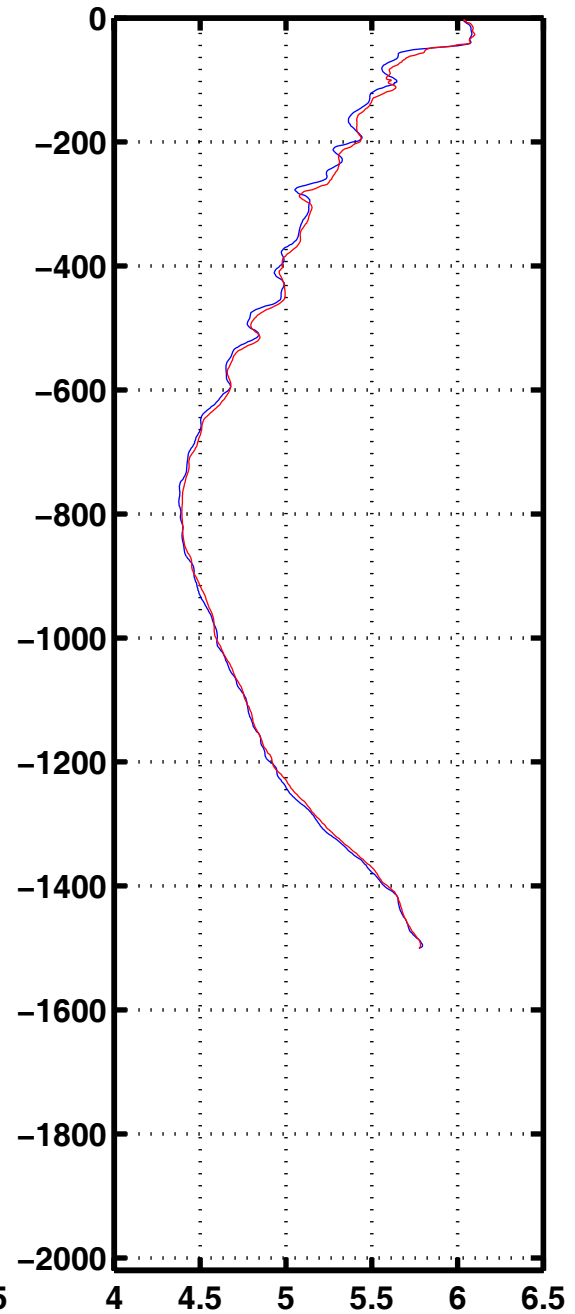
Oxyg 2170
