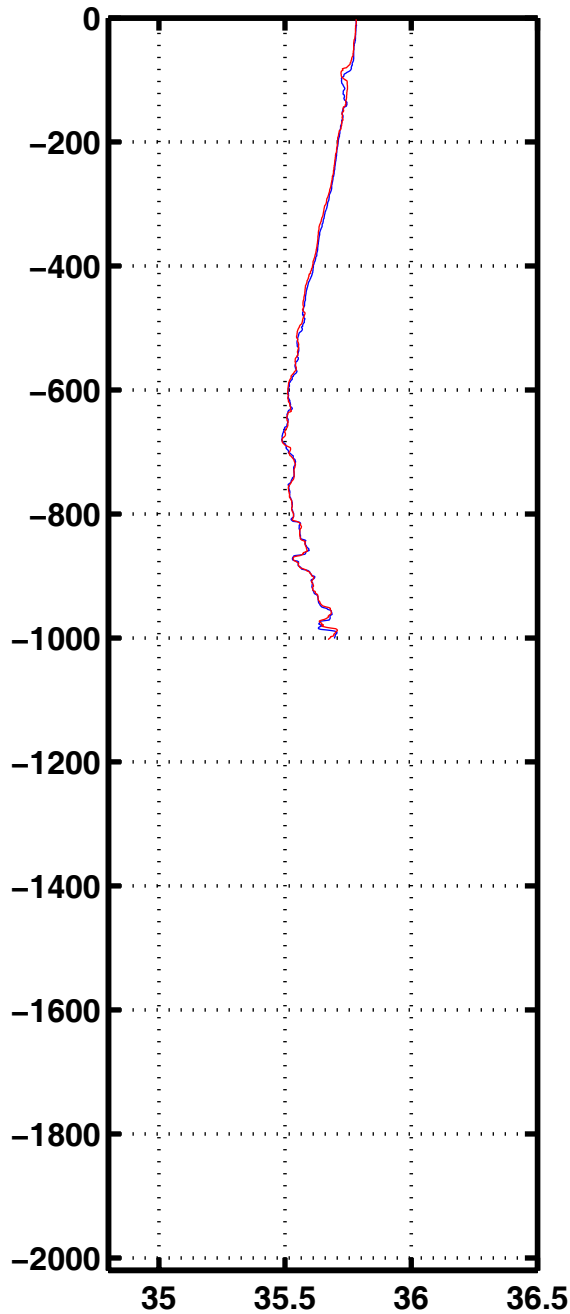
Sali 2405
