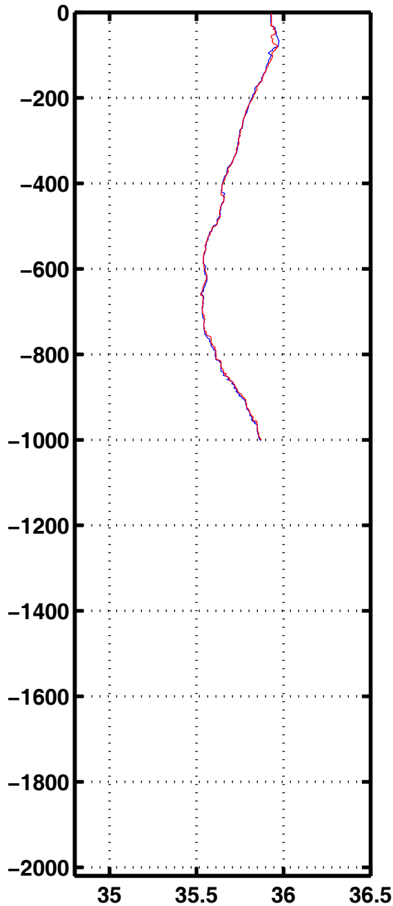
Sali 2086
