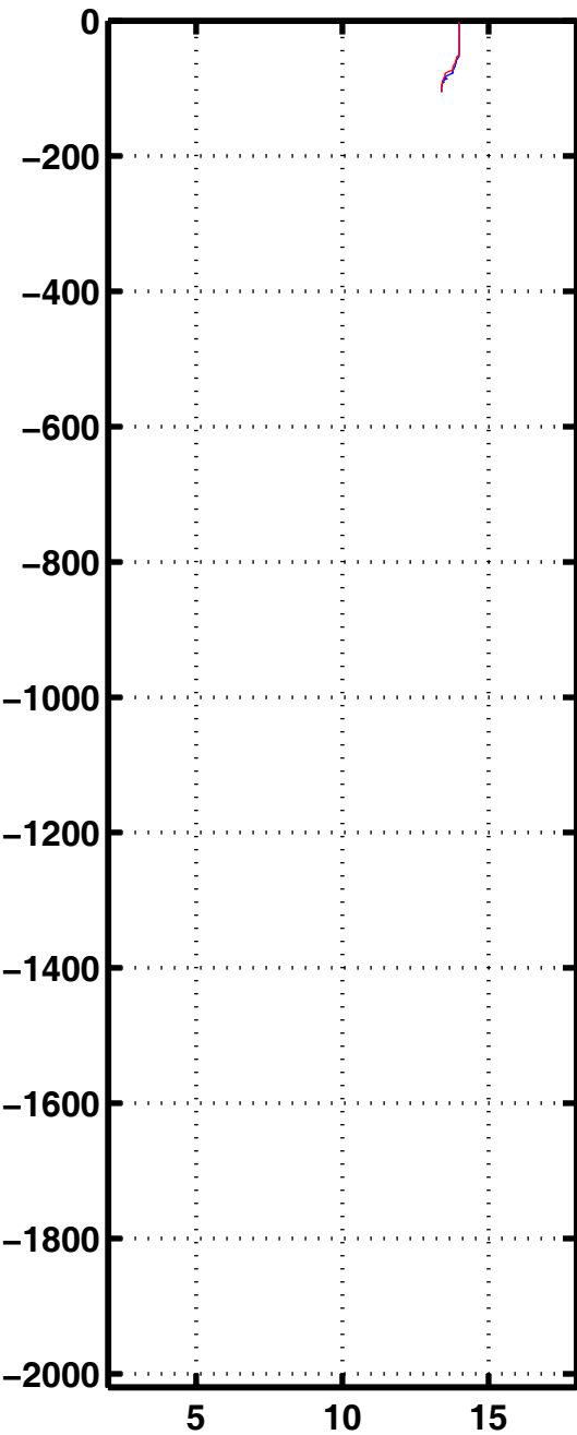
Tempe 2415
