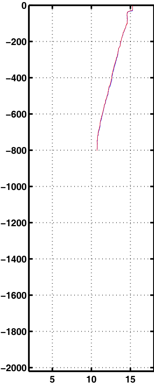
Tempe 2092
