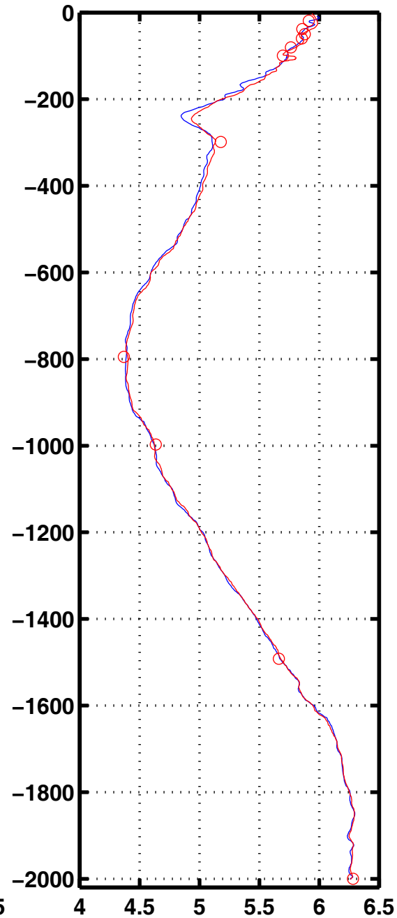
Oxyg 2048
