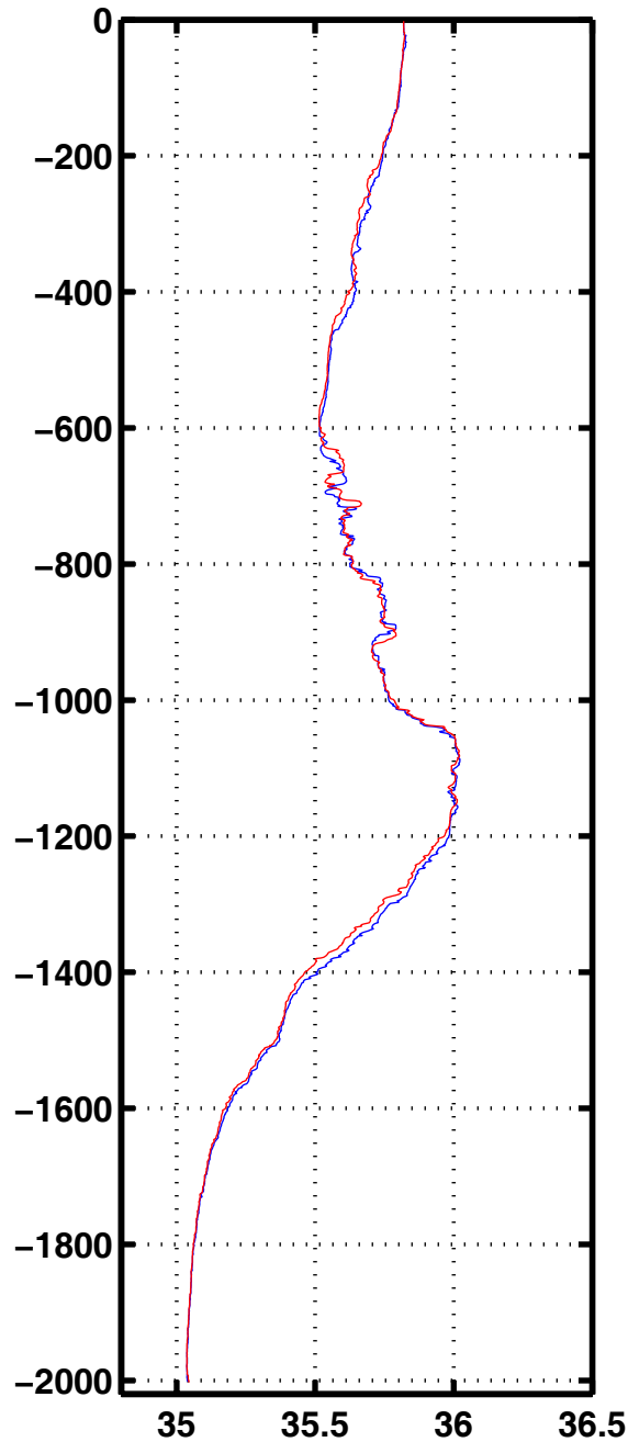
Sali 2035
