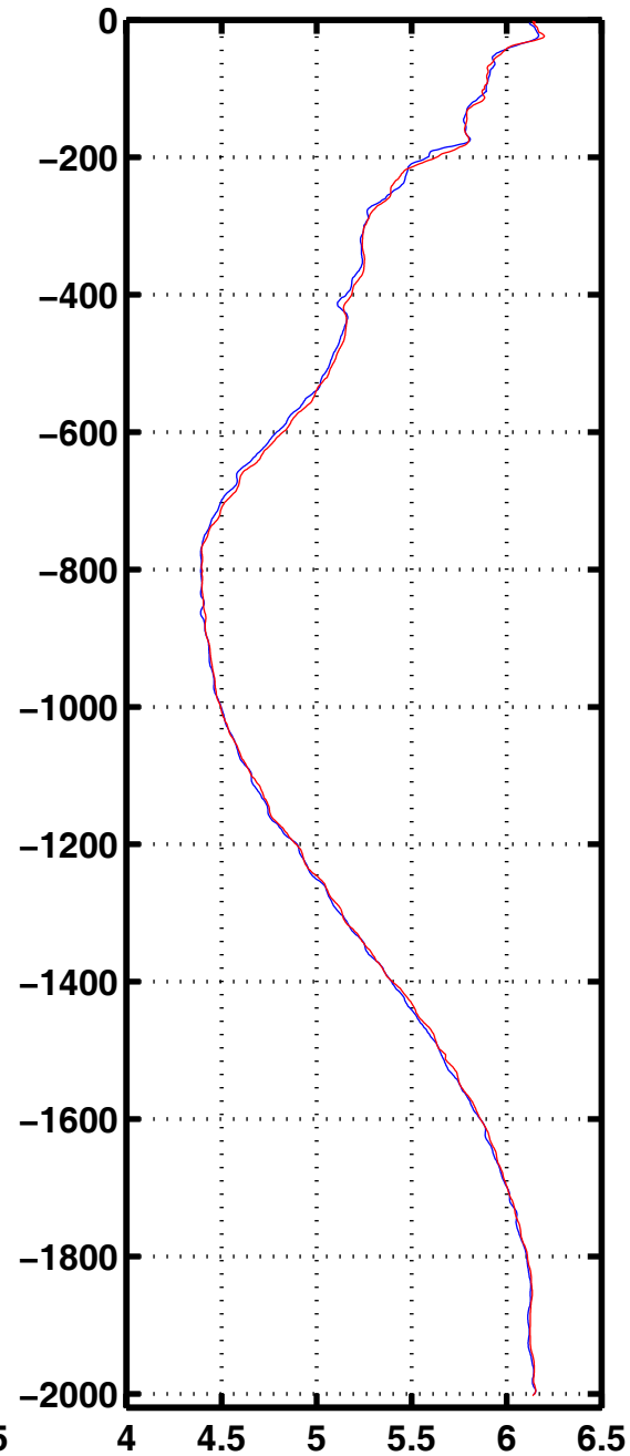
Oxyg 2010
