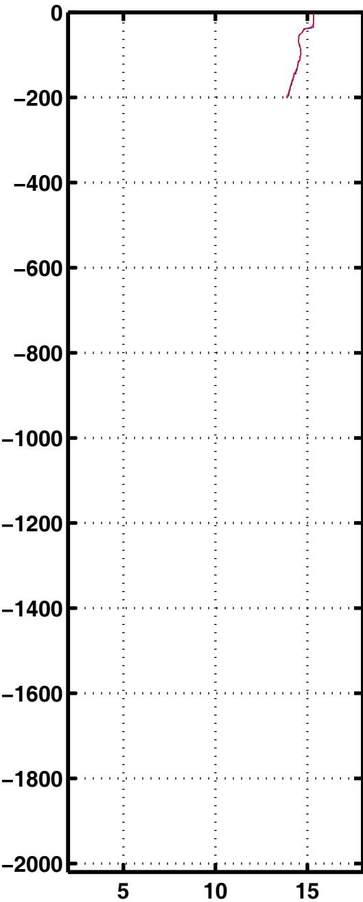
Tempe 2083
