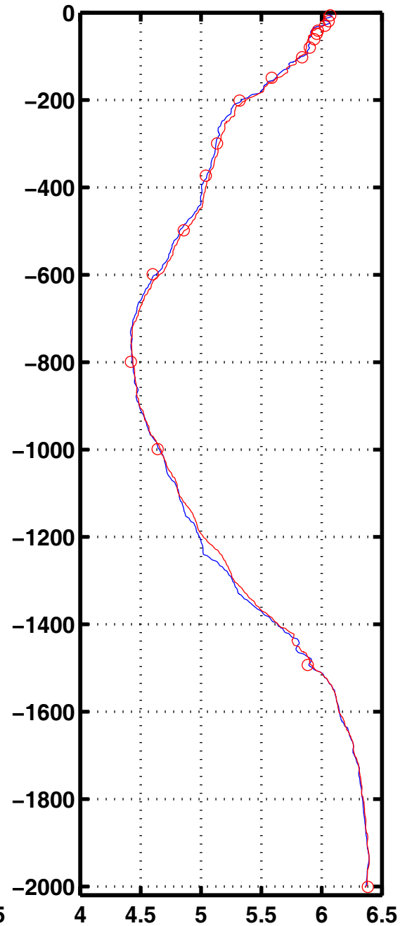
Oxyg 2060
