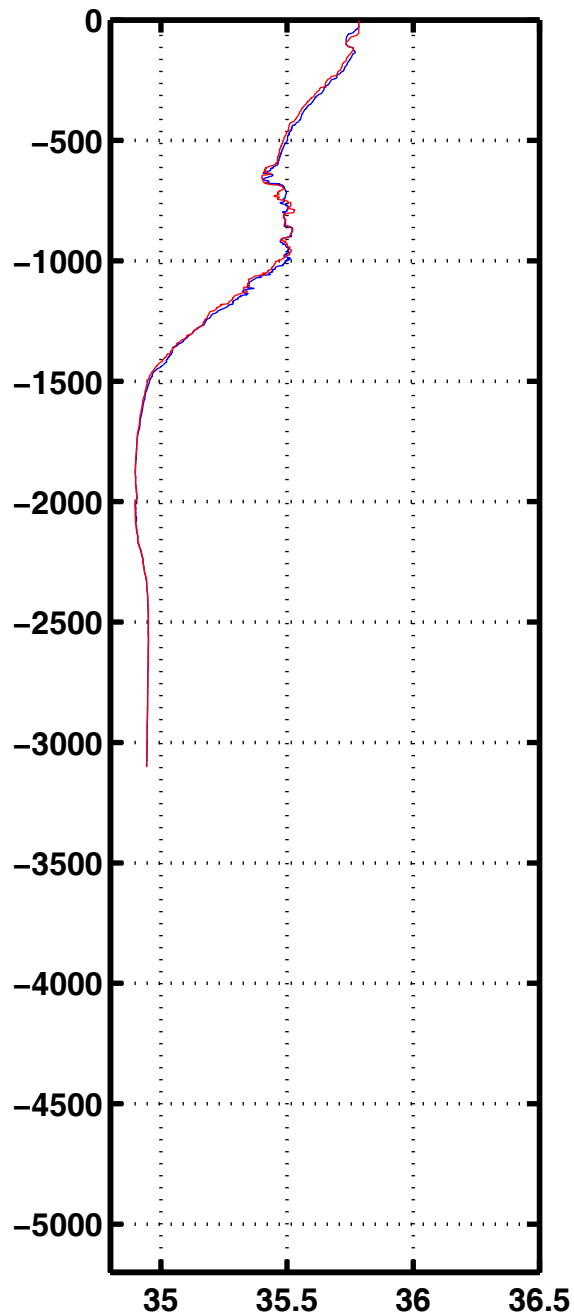
Sali 2046
