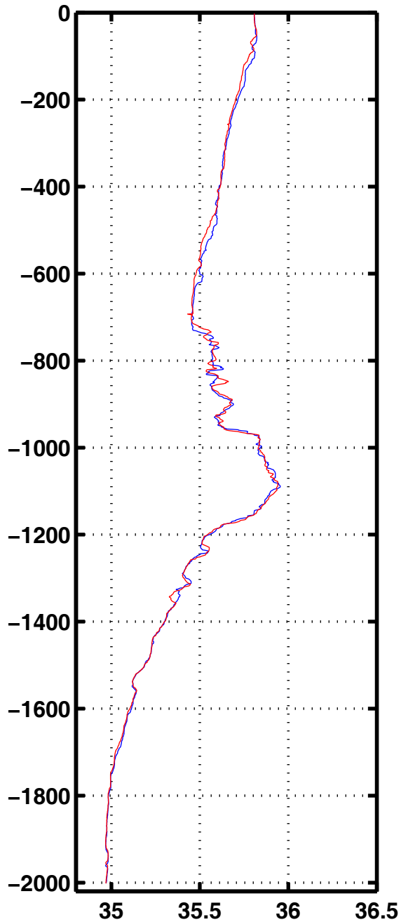
Sali 2279
