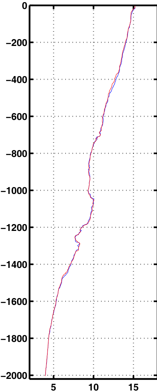
Tempe 2074
