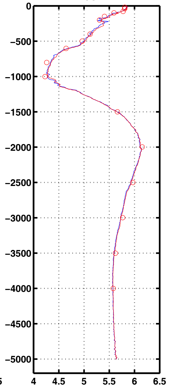
Oxyg 2038
