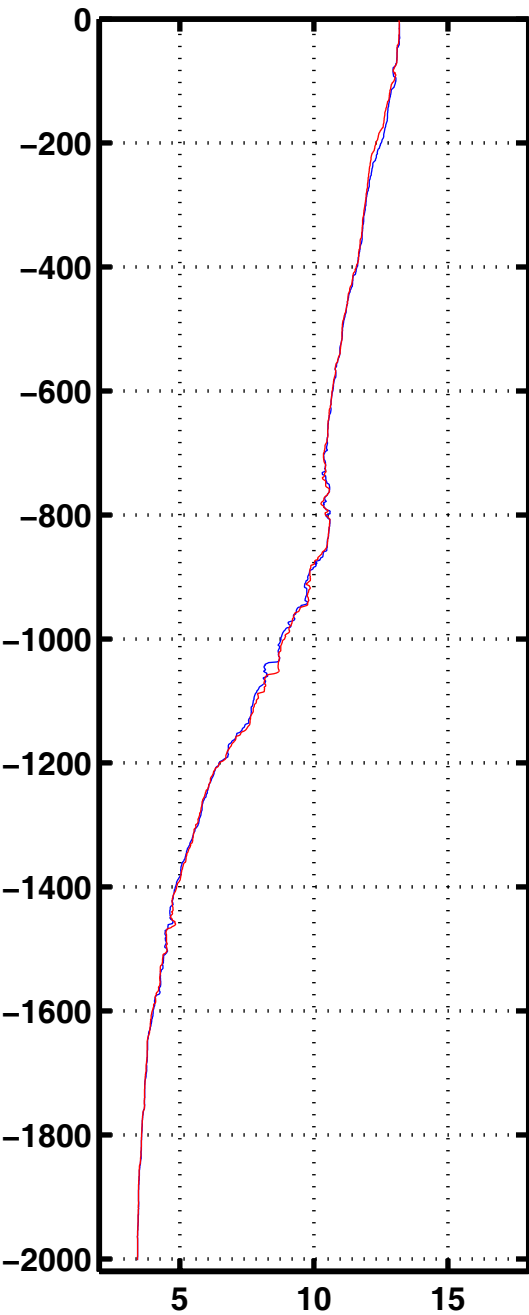
Tempe 2012
