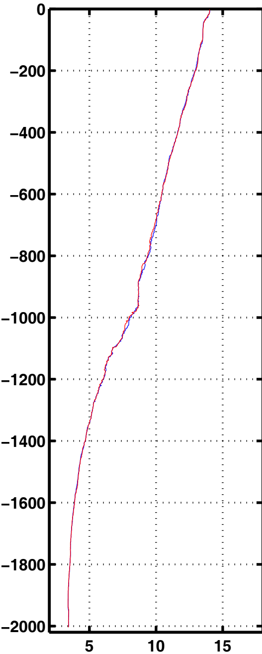
Tempe 2064
