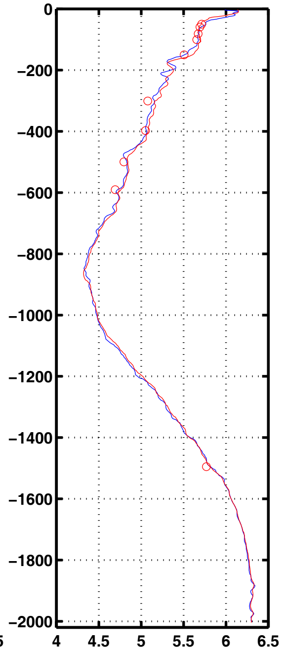
Oxyg 2067
