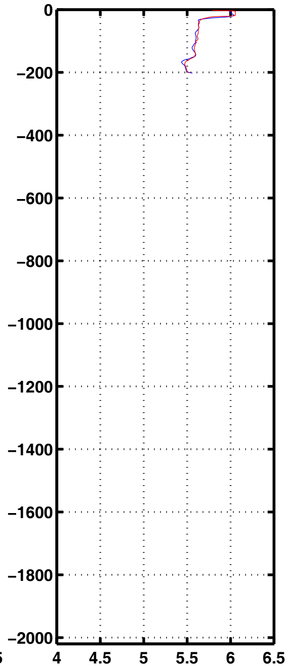
Oxyg 2093
