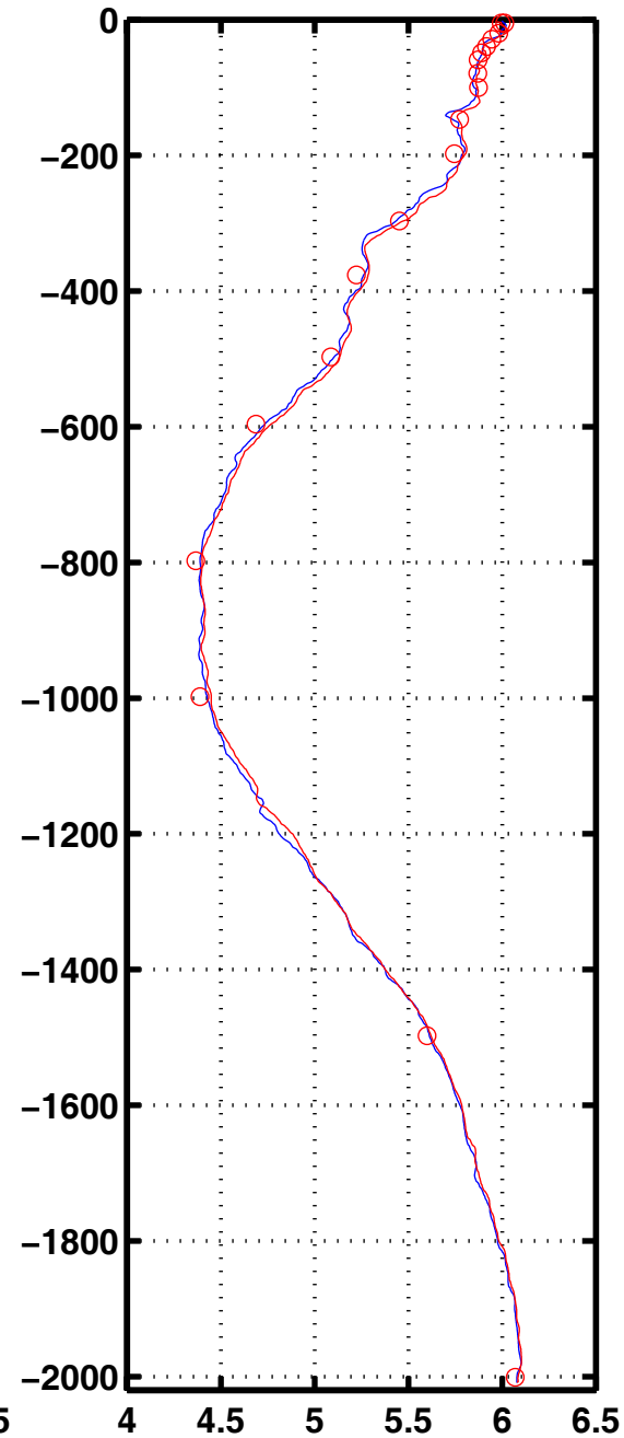
Oxyg 2007
