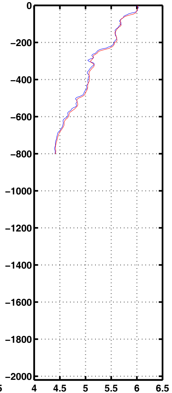
Oxyg 2180
