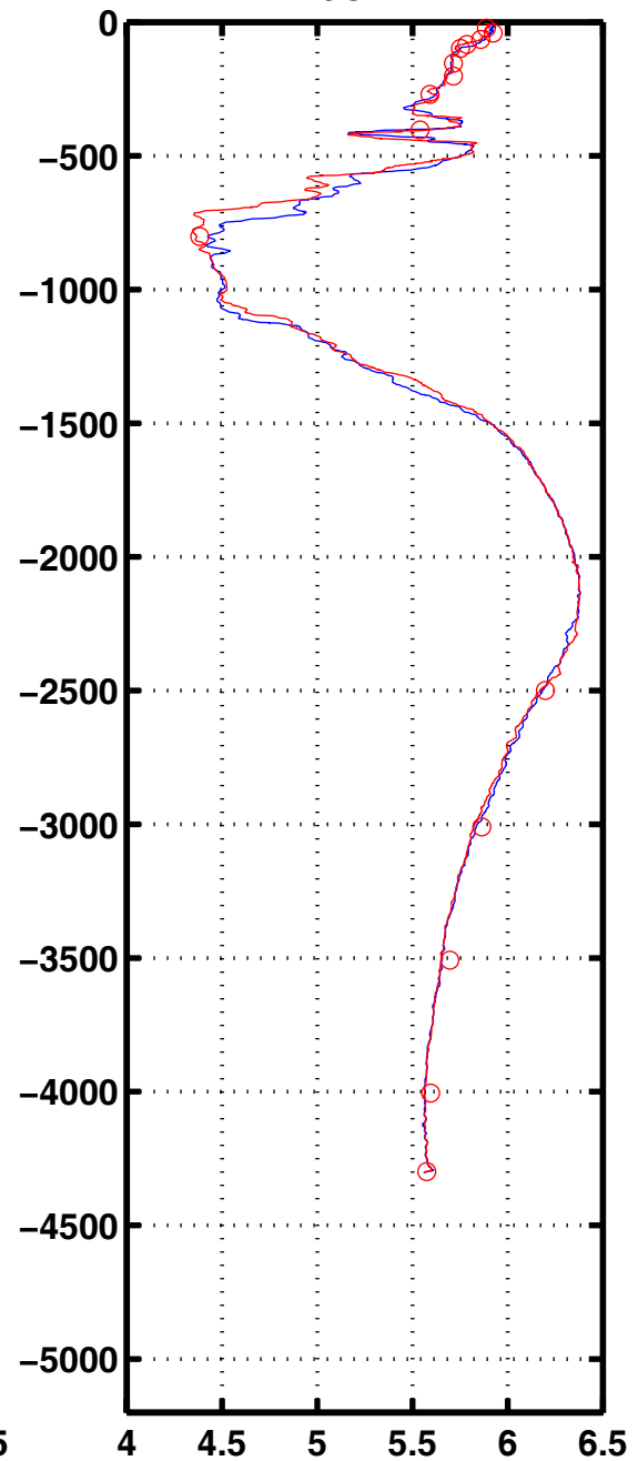
Oxyg 2014
