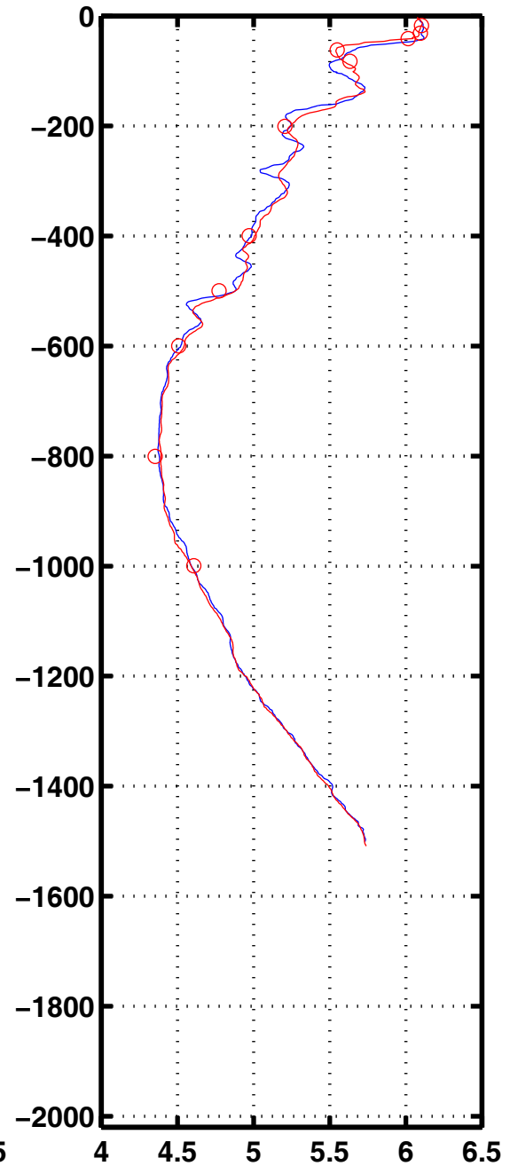
Oxyg 2171
