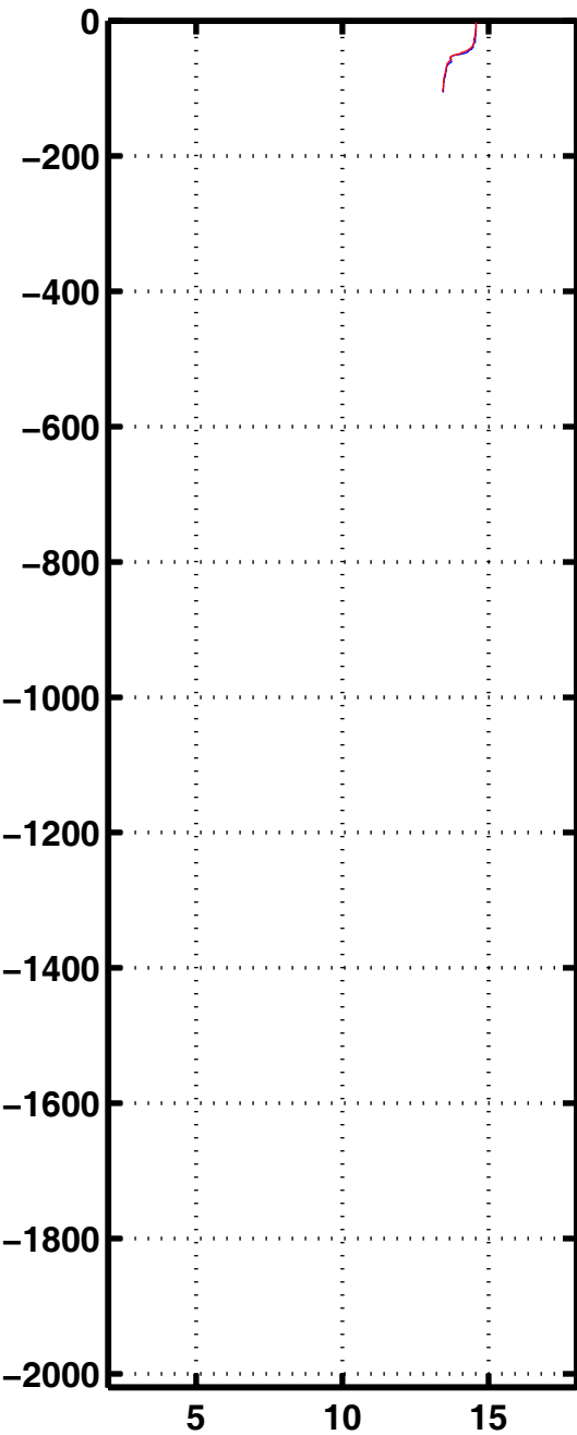
Tempe 2173
