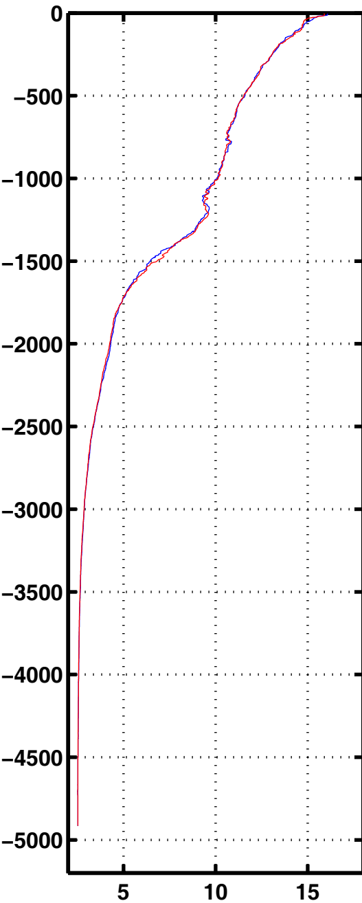
Tempe 2081
