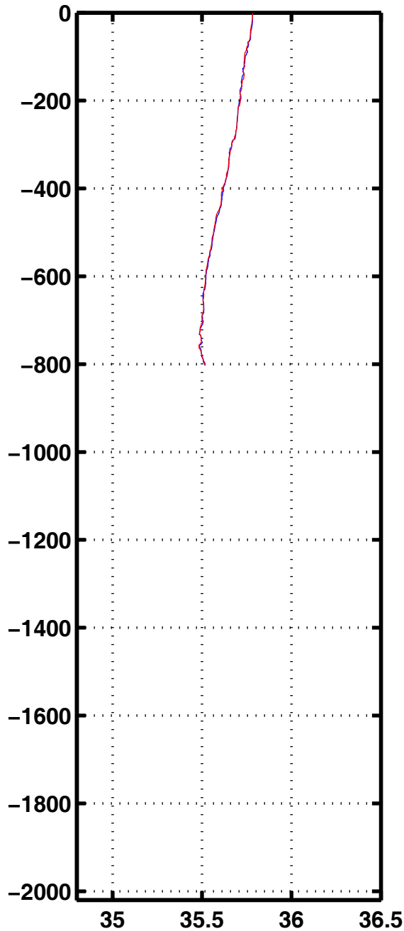
Sali 2411
