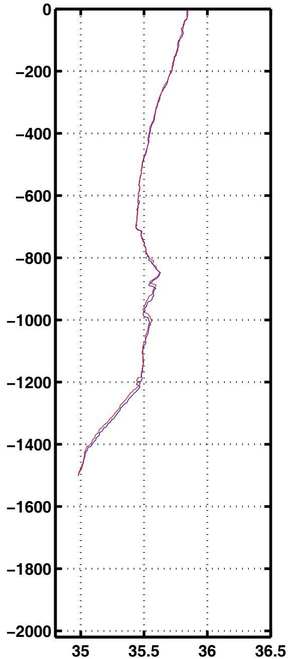
Sali 2170
