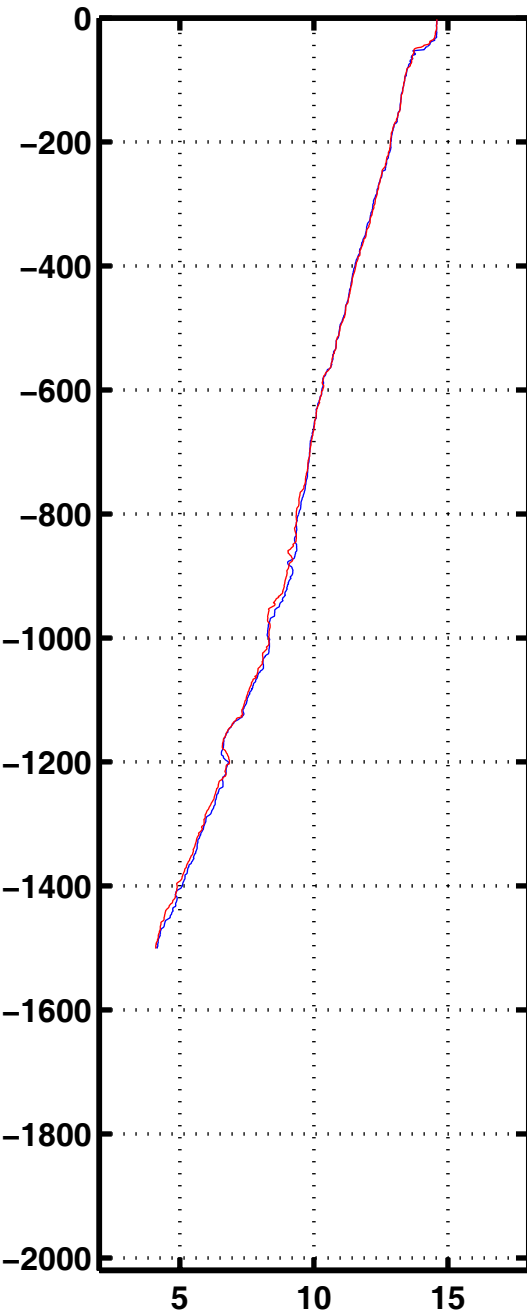
Tempe 2174
