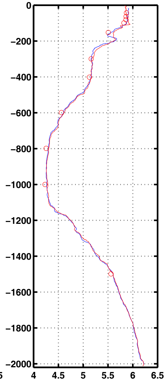
Oxyg 2039
