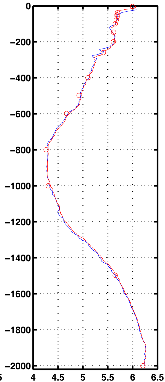
Oxyg 2069
