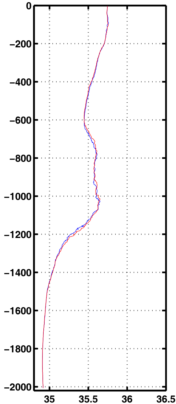
Sali 2059
