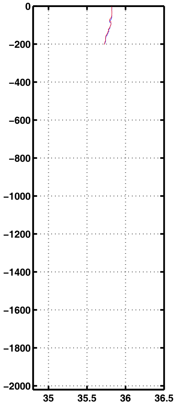
Sali 2265
