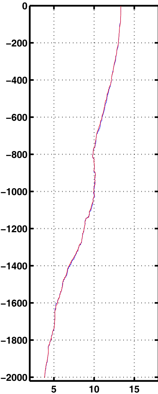
Tempe 2022
