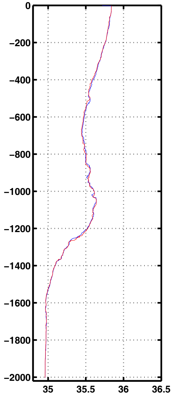
Sali 2058
