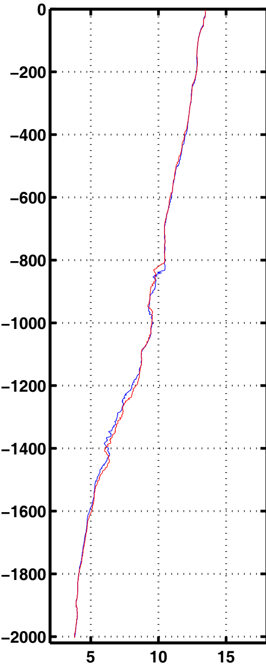
Tempe 2027
