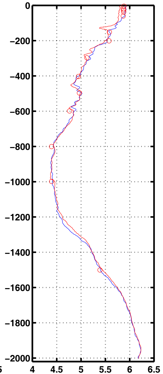
Oxyg 2021
