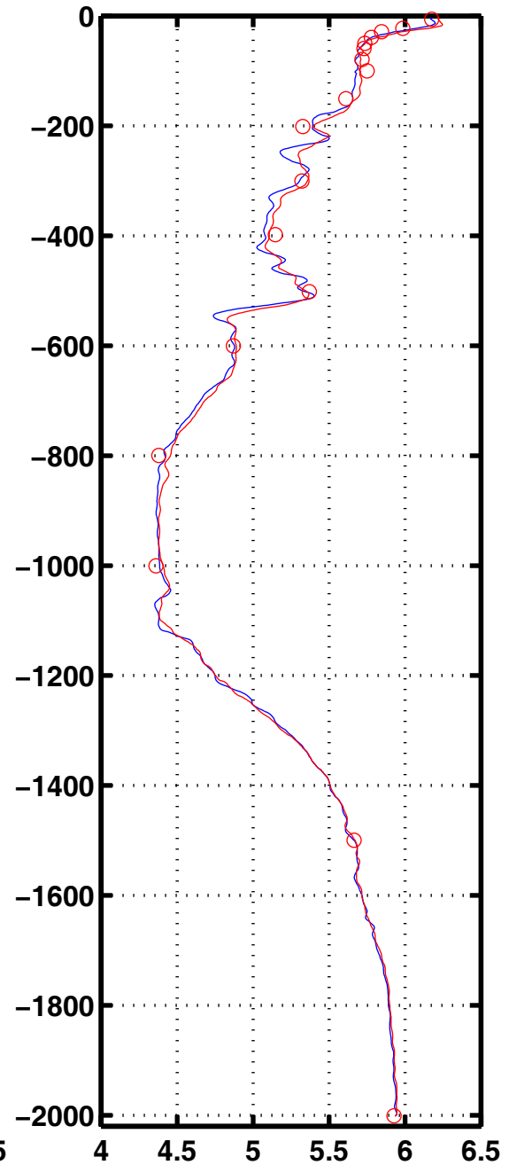
Oxyg 2073
