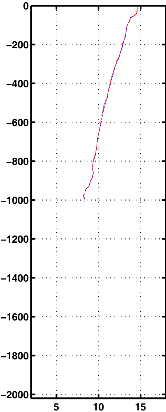
Tempe 2175
