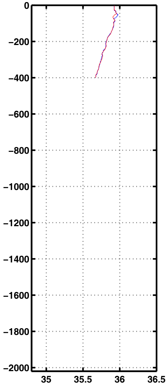
Sali 2089
