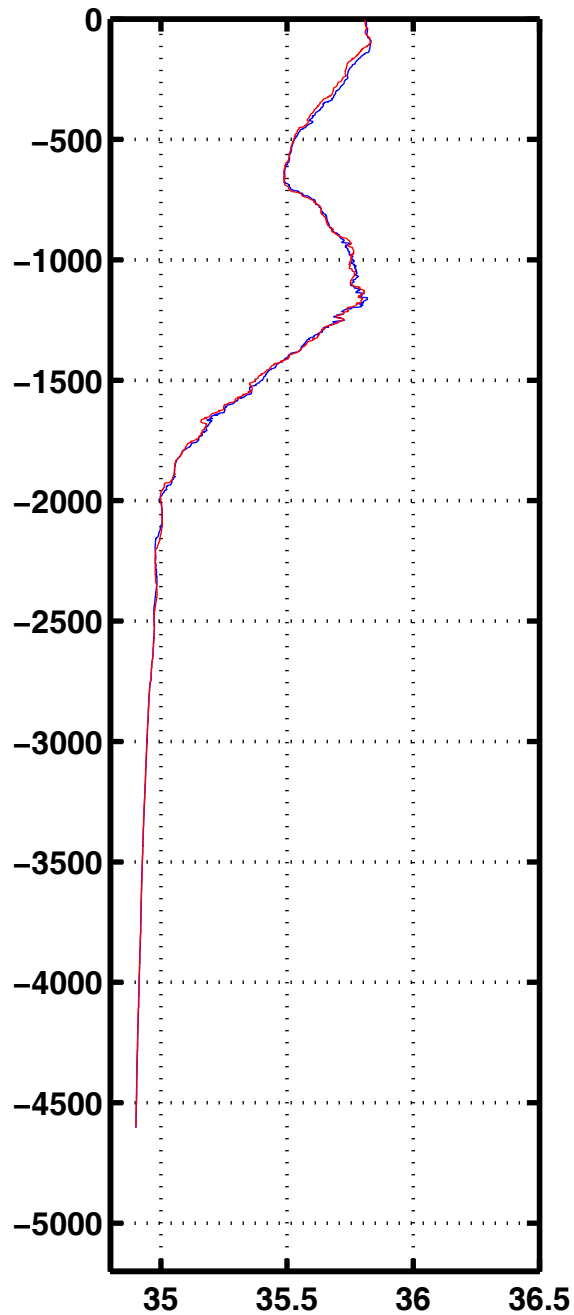
Sali 2034
