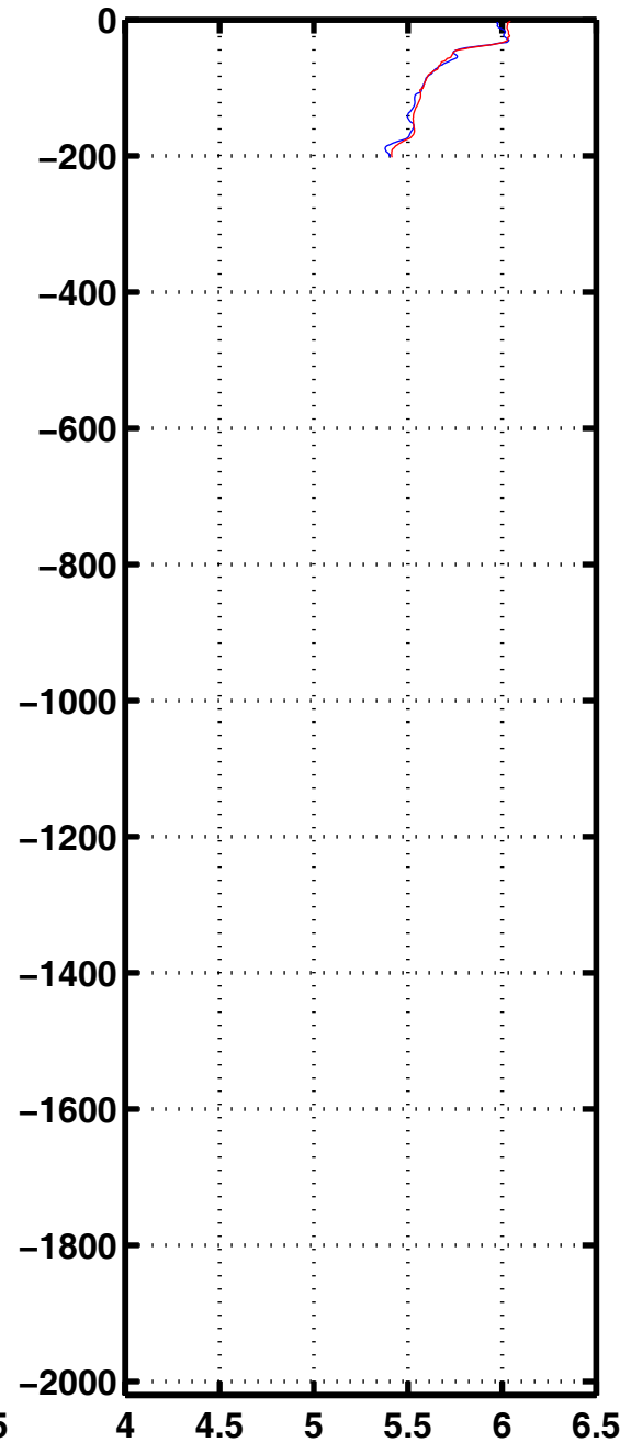
Oxyg 2083
