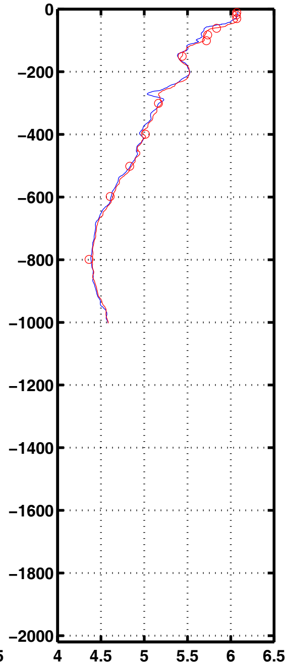
Oxyg 2182
