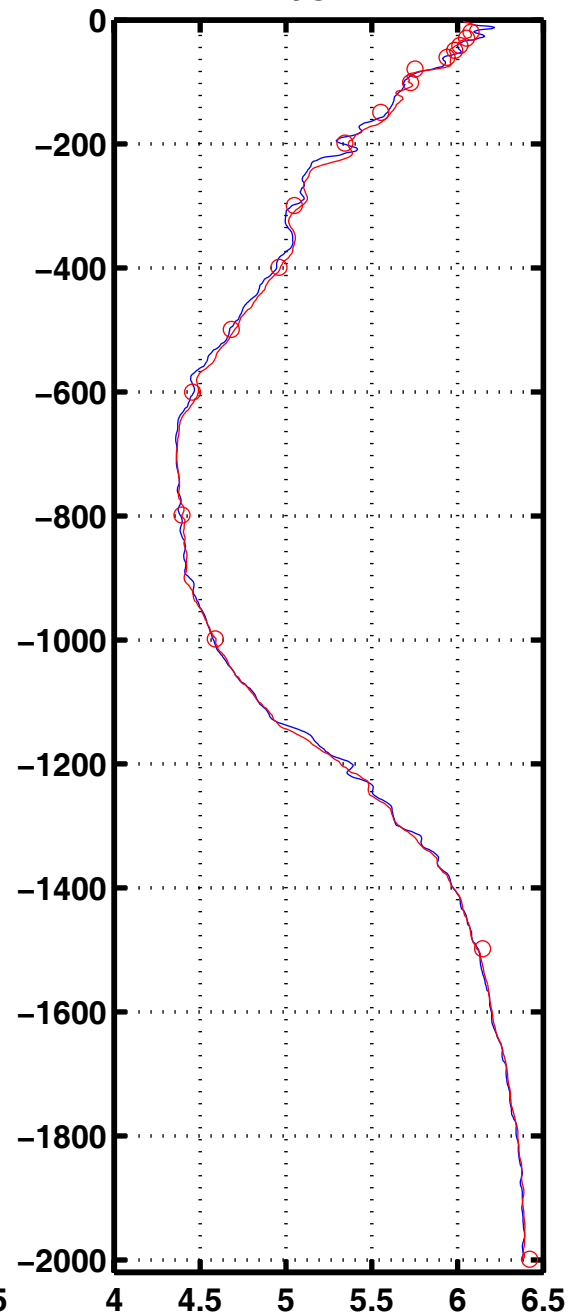
Oxyg 2047
