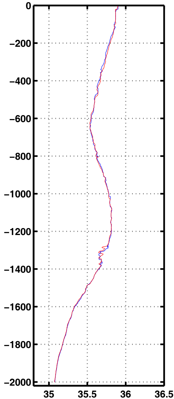
Sali 2080
