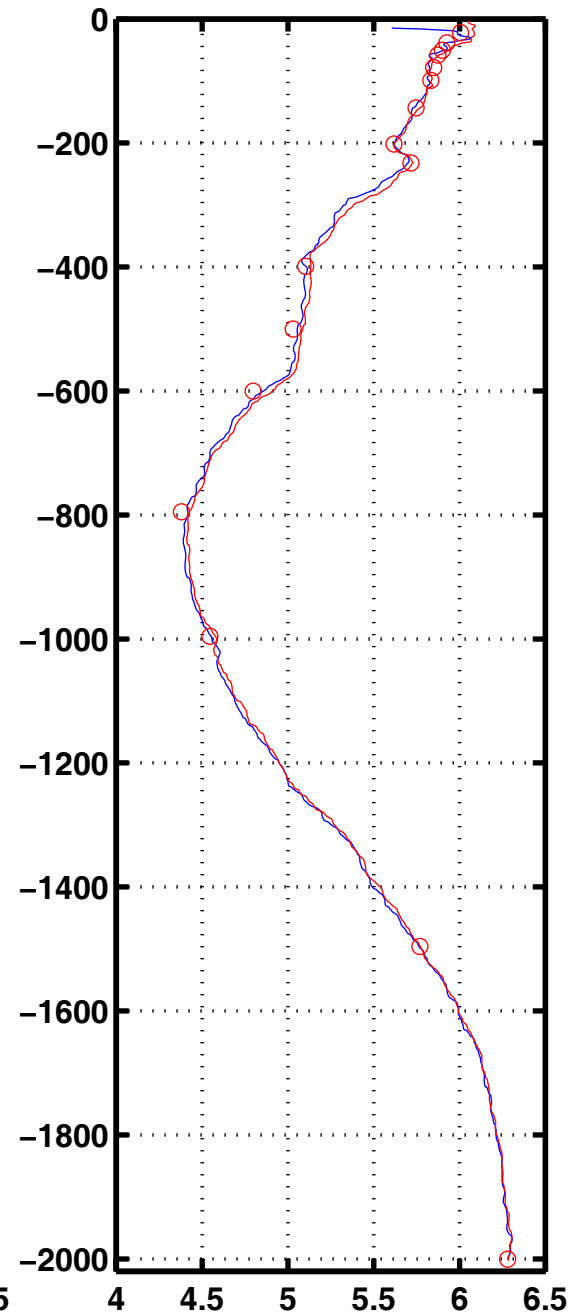
Oxyg 2062
