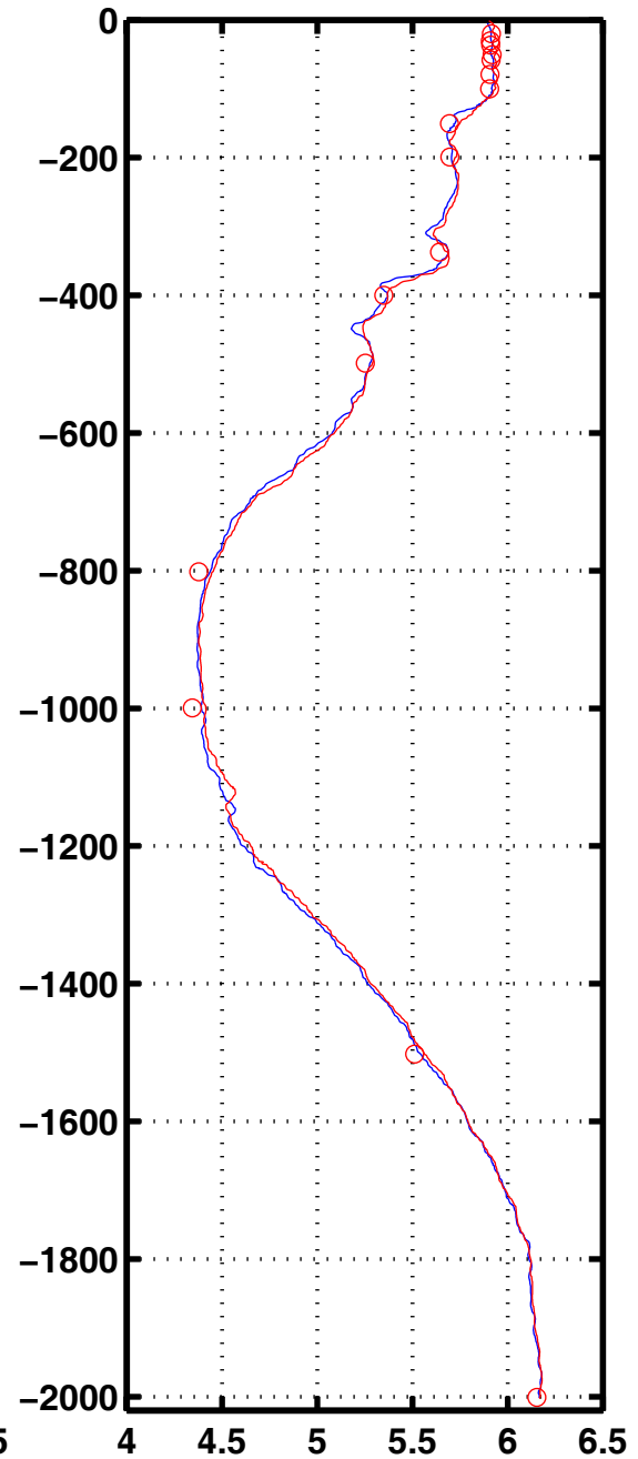
Oxyg 2040
