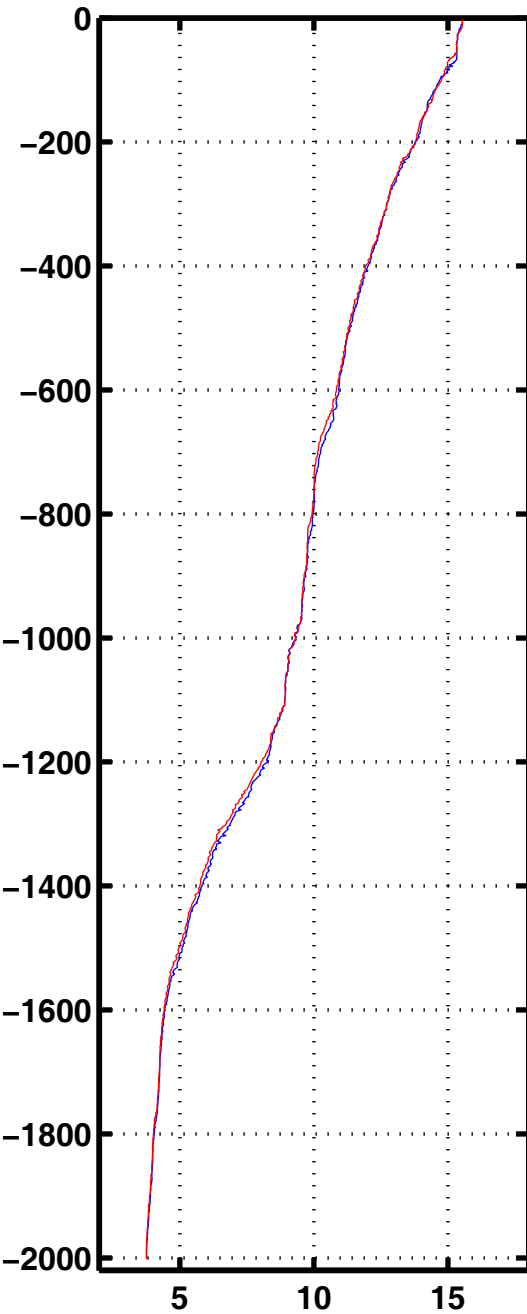
Tempe 2033
