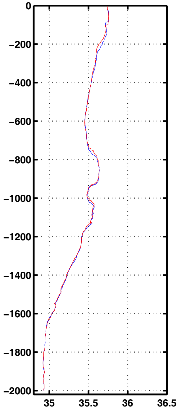
Sali 2048
