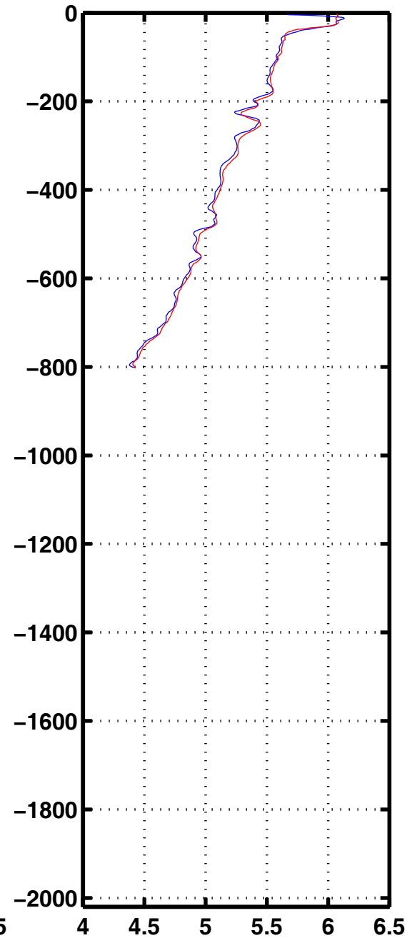
Oxyg 2092
