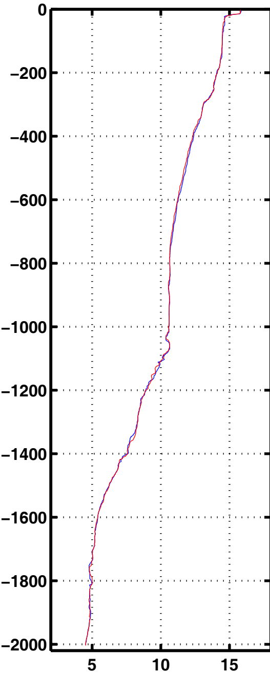
Tempe 2082
