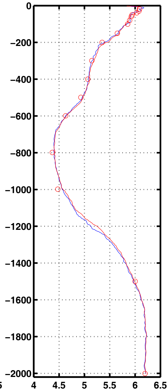
Oxyg 2057
