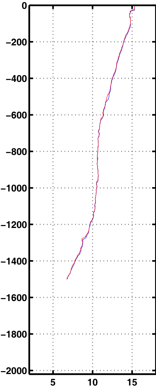
Tempe 2084
