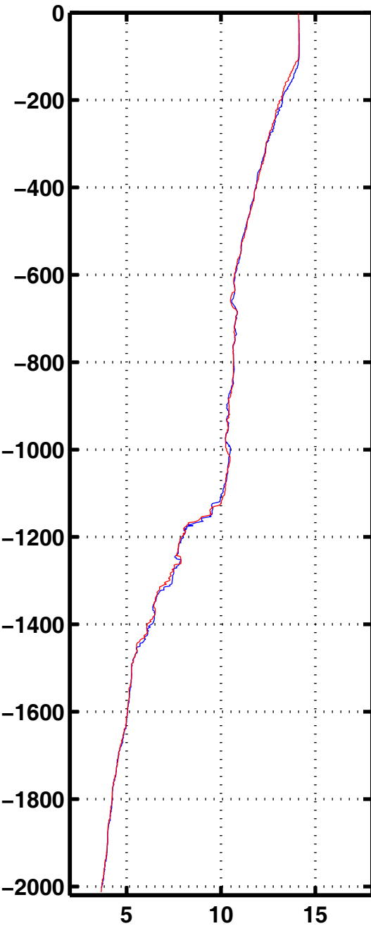
Tempe 2039
