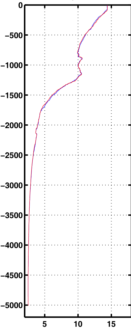
Tempe 2003
