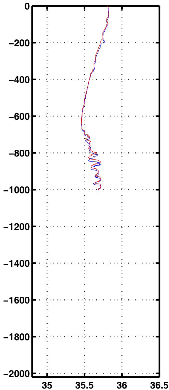
Sali 2268
