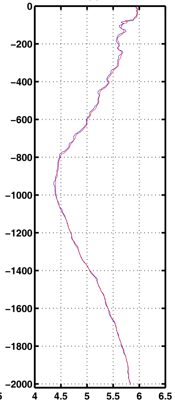
Oxyg 2416
