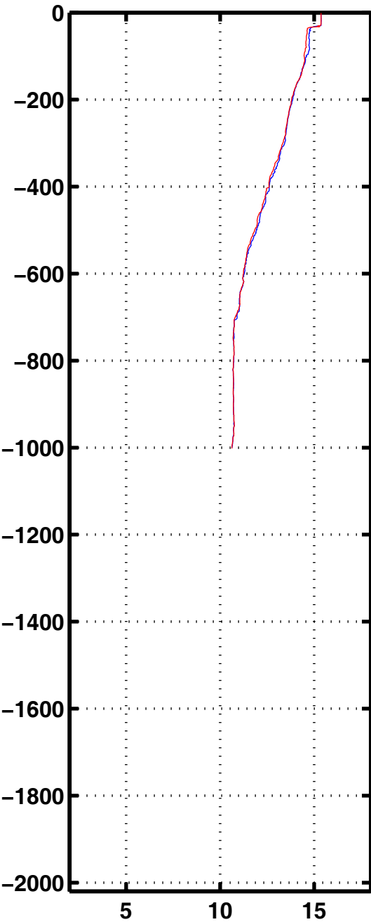
Tempe 2088
