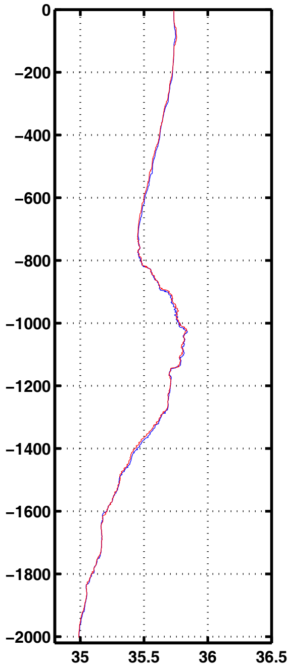
Sali 2022
