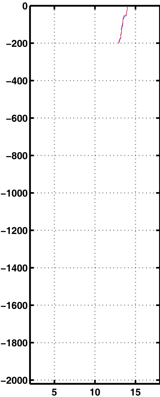
Tempe 2412
