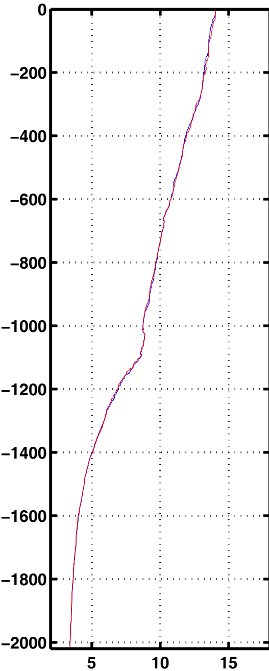
Tempe 2054
