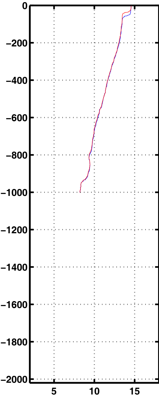
Tempe 2172
