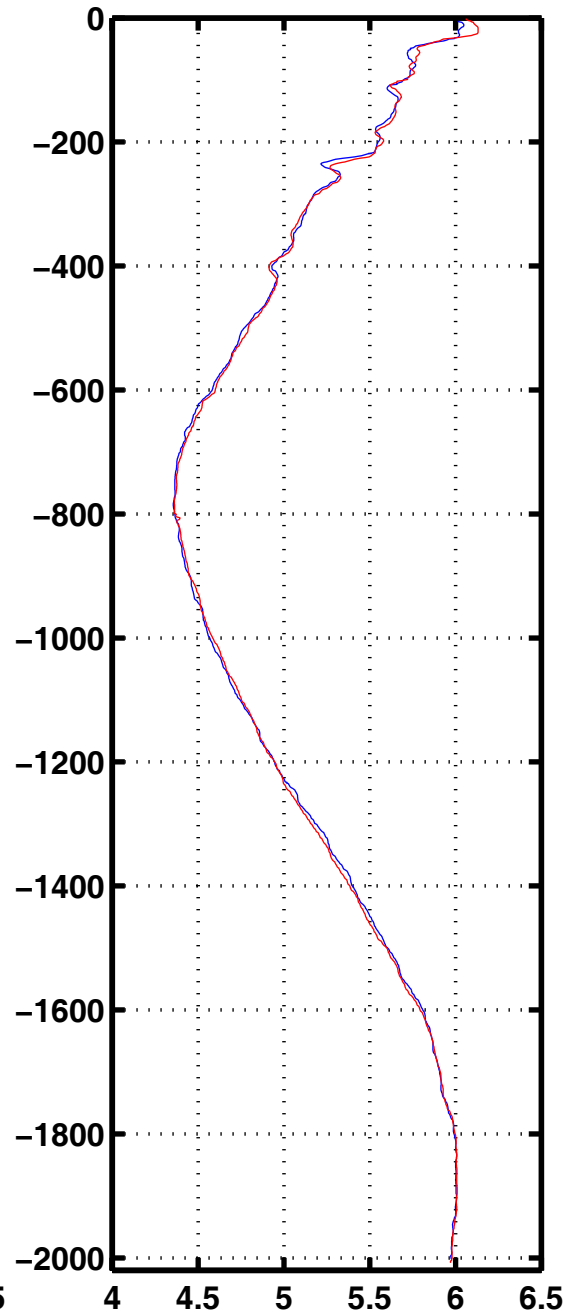
Oxyg 2183
