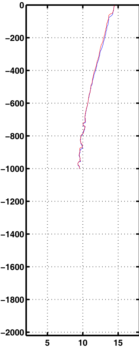
Tempe 2276
