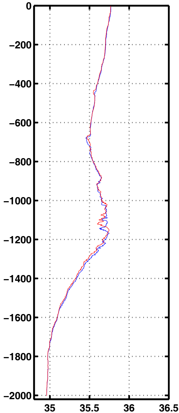
Sali 2040
