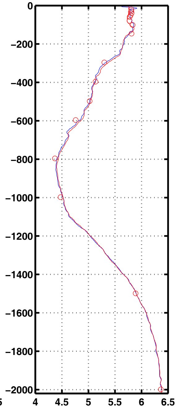
Oxyg 2054
