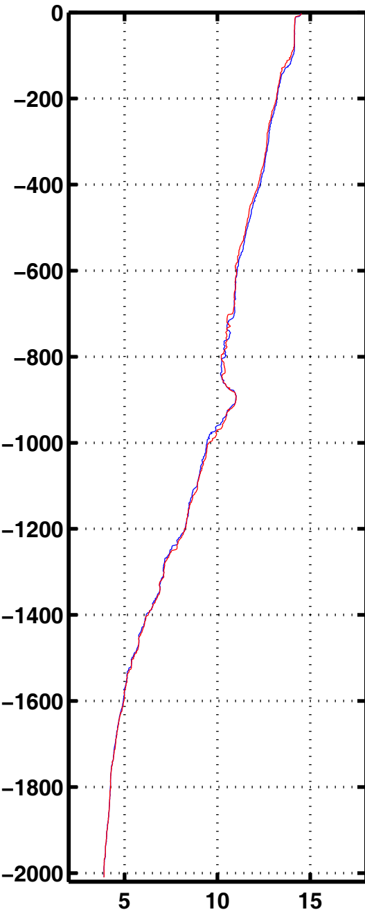
Tempe 2005
