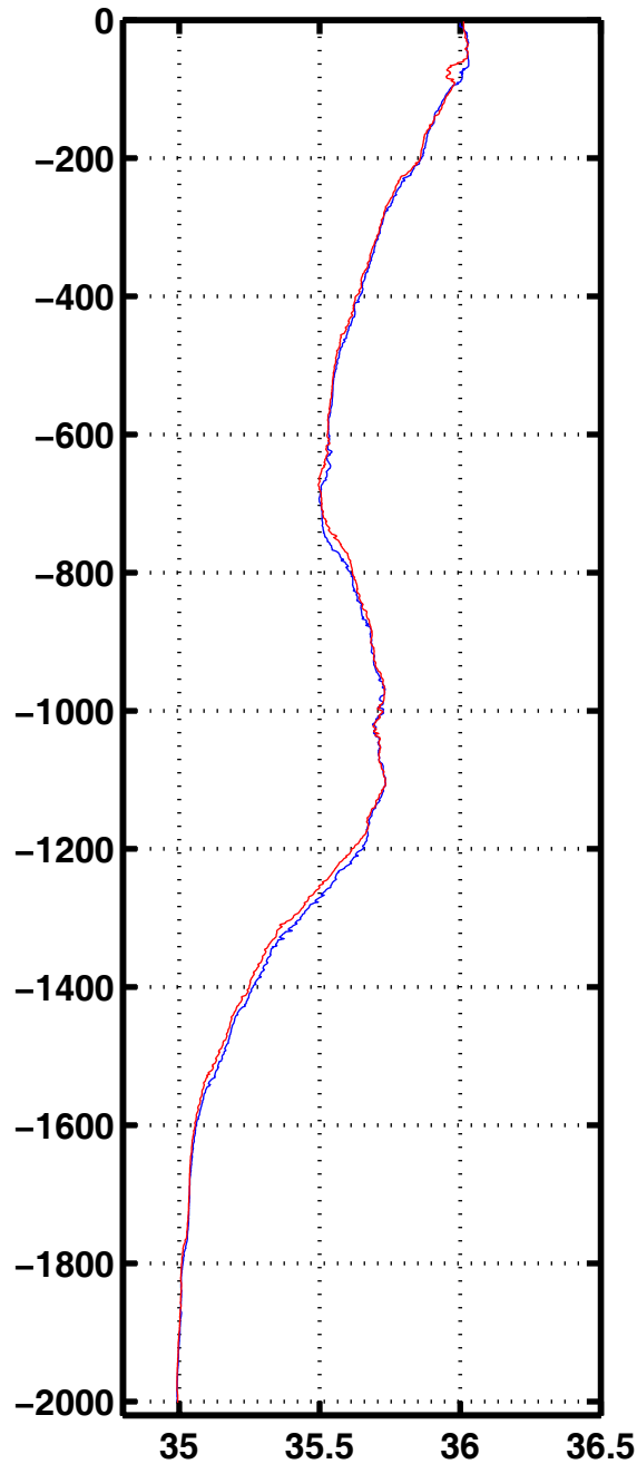
Sali 2033
