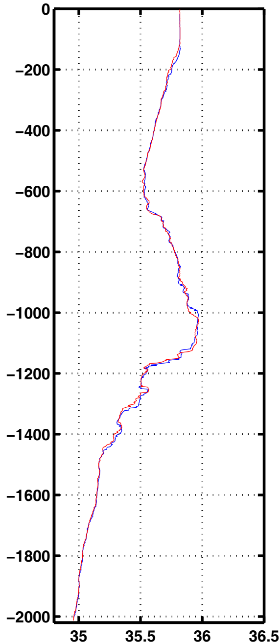
Sali 2039
