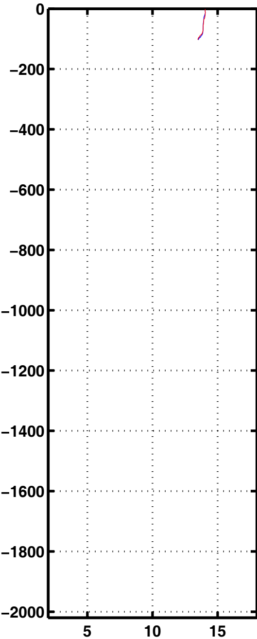
Tempe 2409
