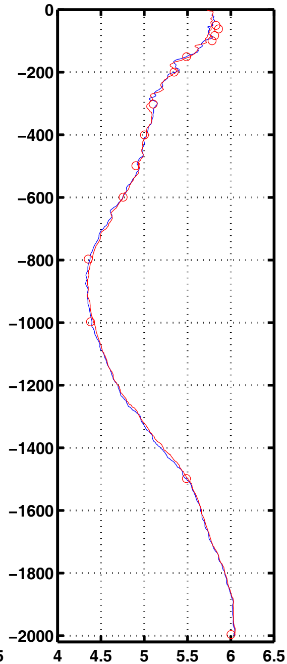
Oxyg 2036
