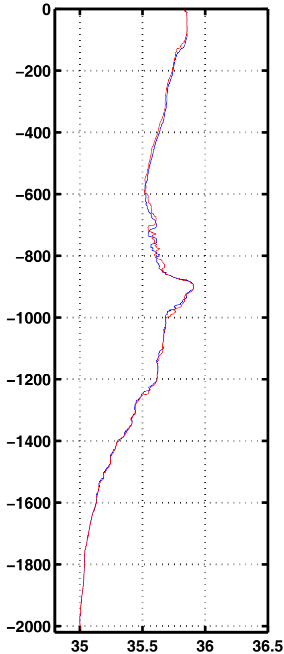
Sali 2005
