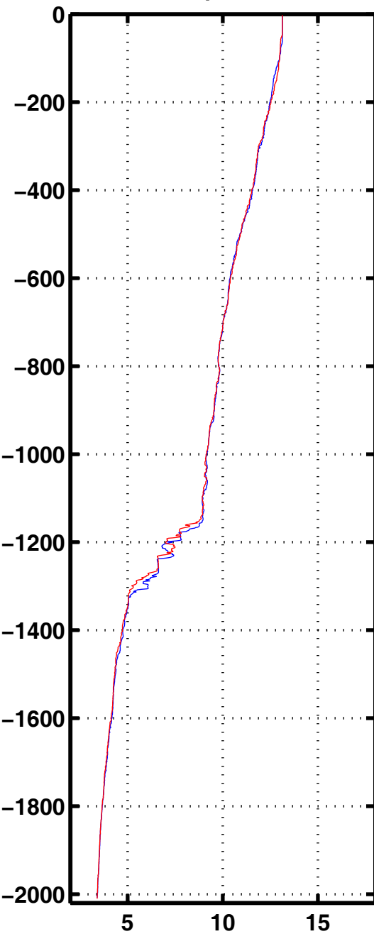
Tempe 2019
