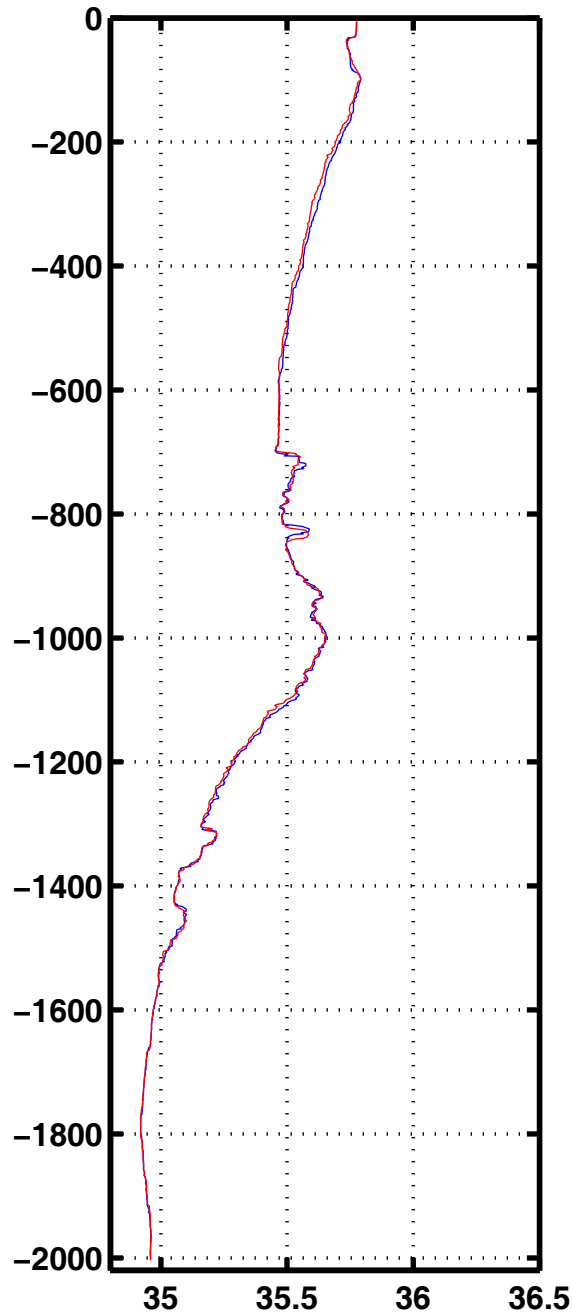
Sali 2065
