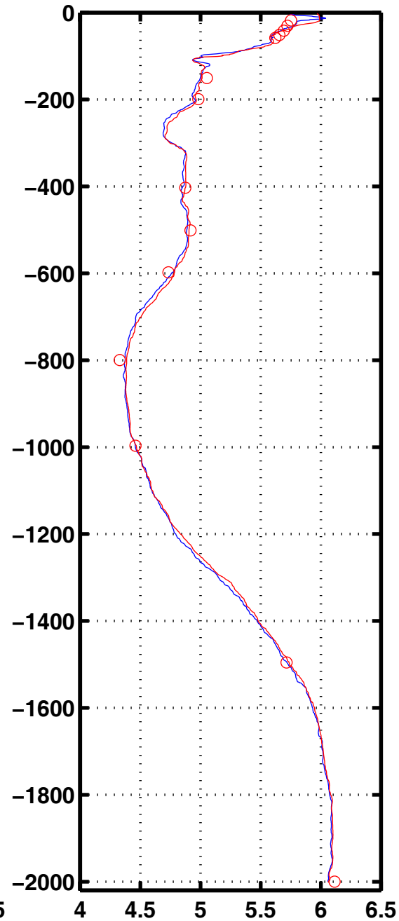
Oxyg 2033
