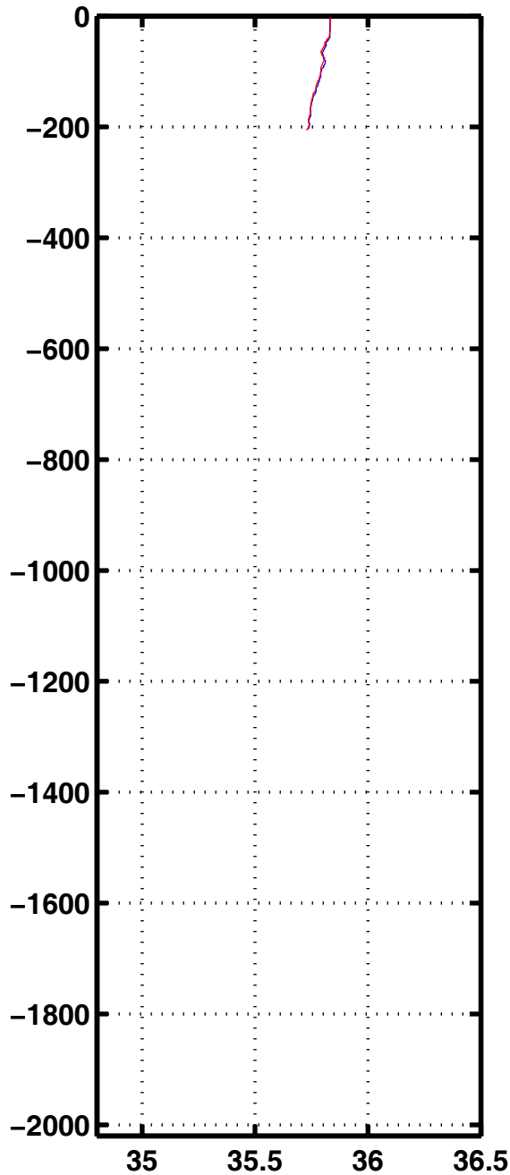
Sali 2169
