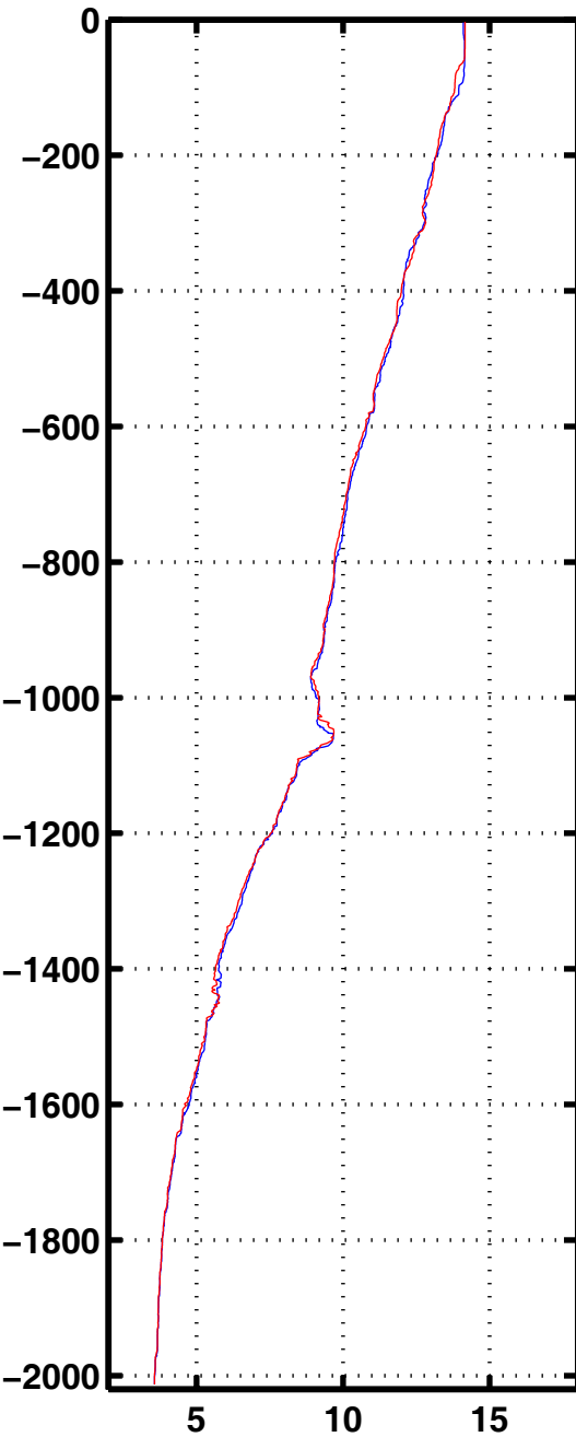
Tempe 2049
