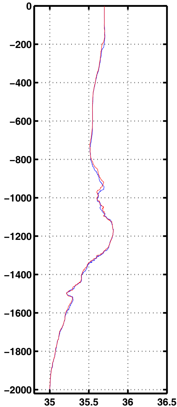
Sali 2041
