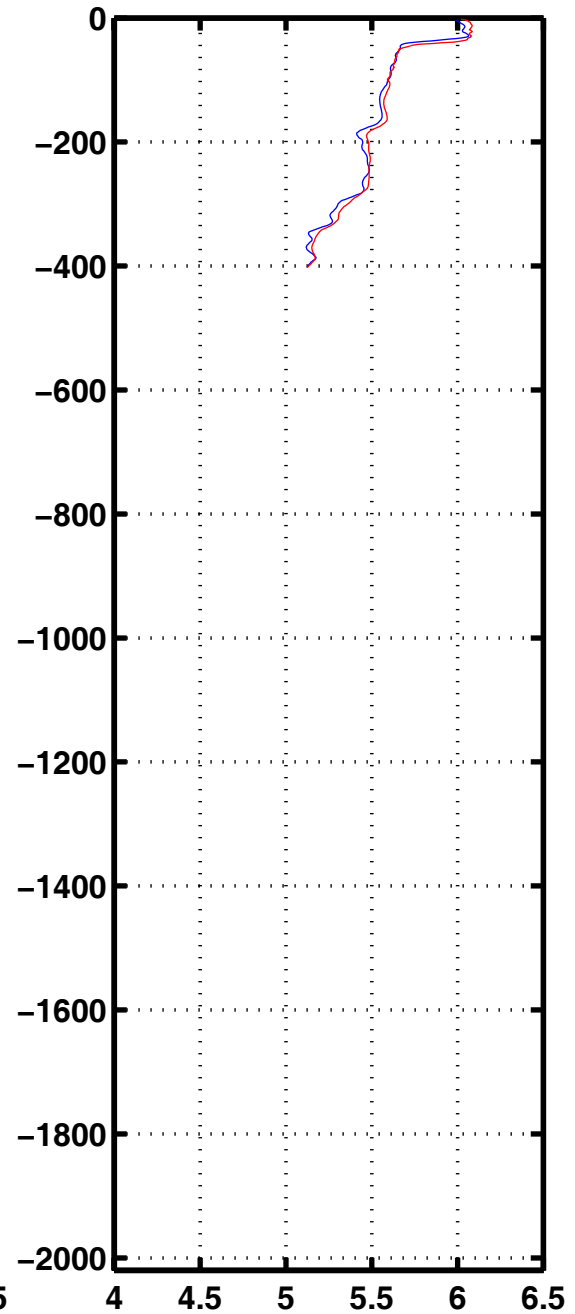
Oxyg 2091
