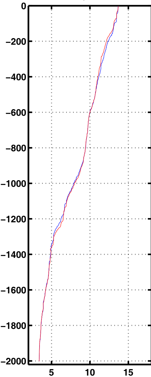
Tempe 2056
