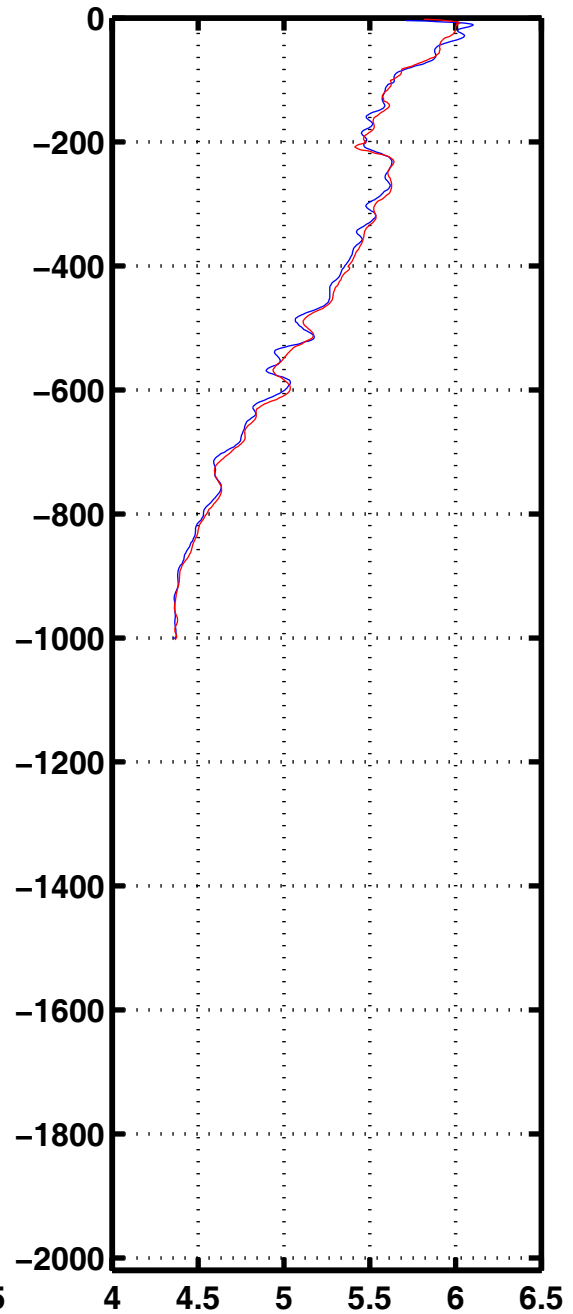
Oxyg 2405
