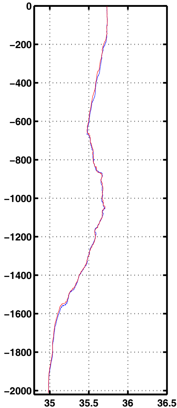
Sali 2015
