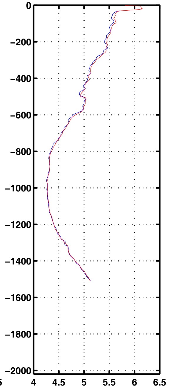
Oxyg 2087
