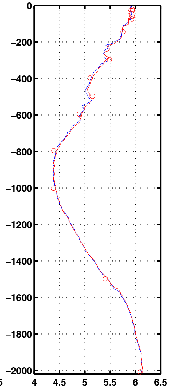
Oxyg 2015
