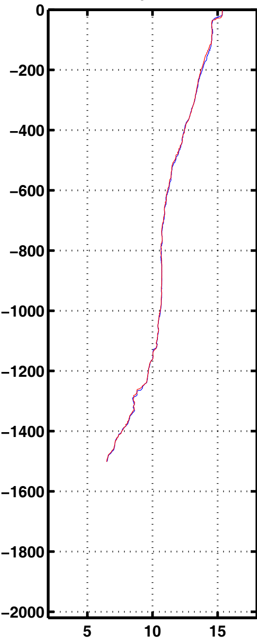
Tempe 2085
