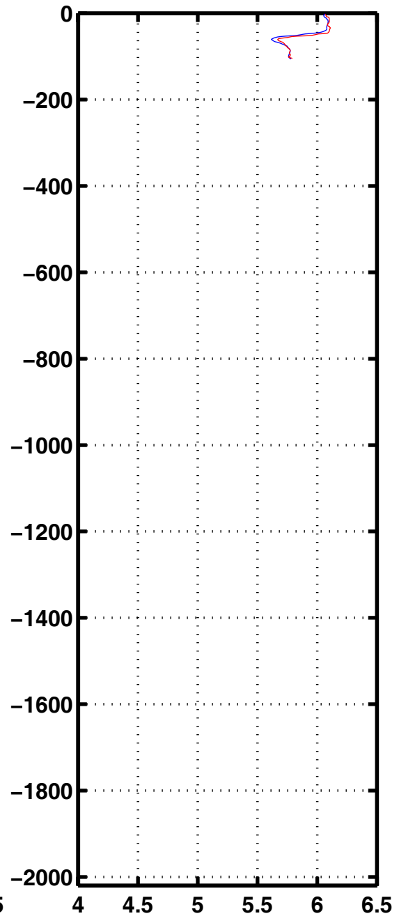
Oxyg 2173
