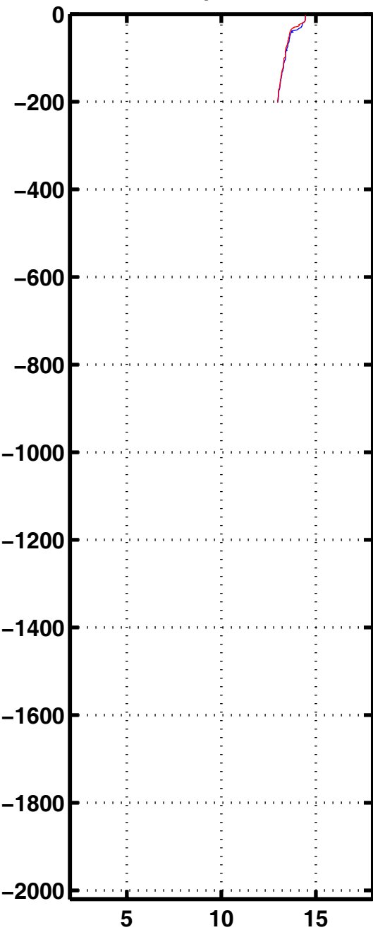
Tempe 2181
