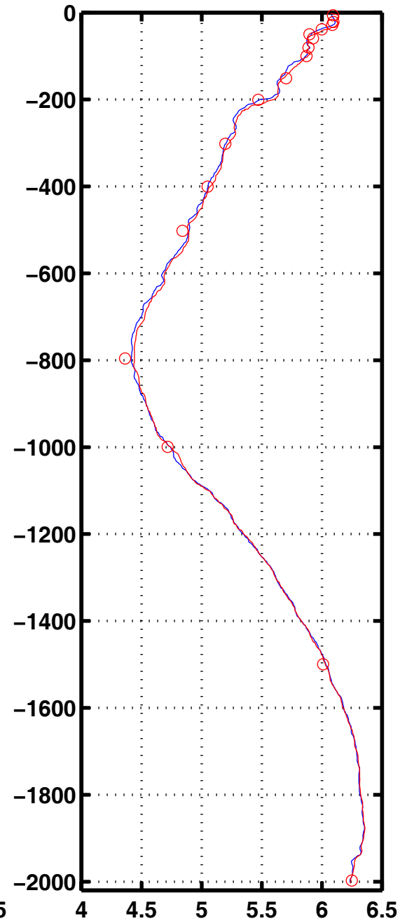
Oxyg 2064
