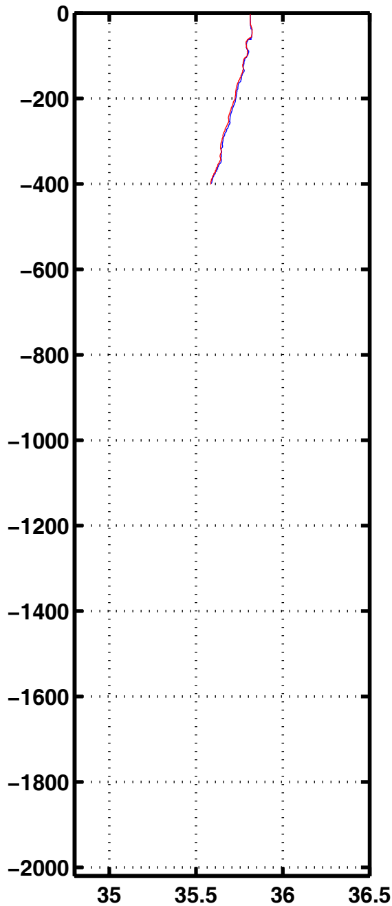
Sali 2271
