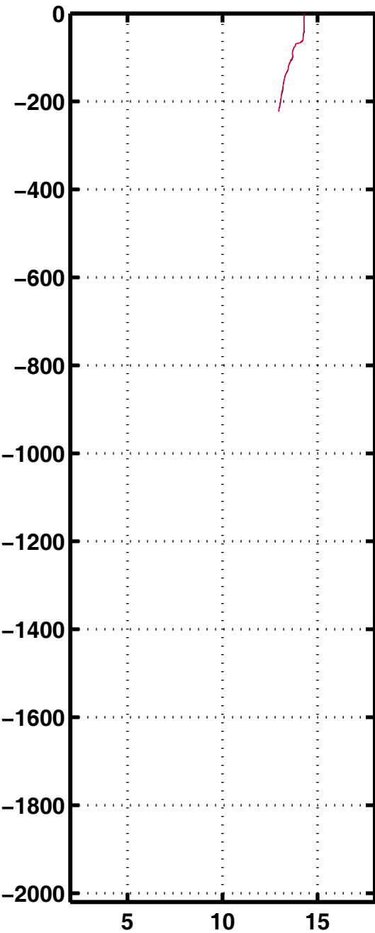
Tempe 2275
