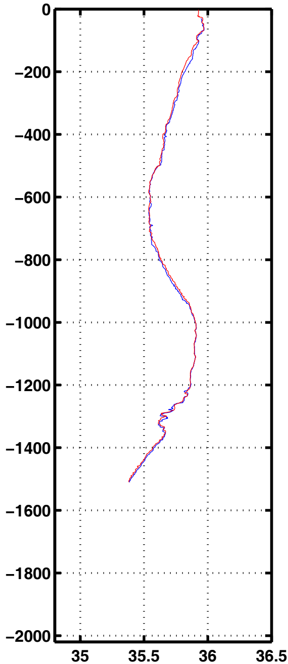
Sali 2087
