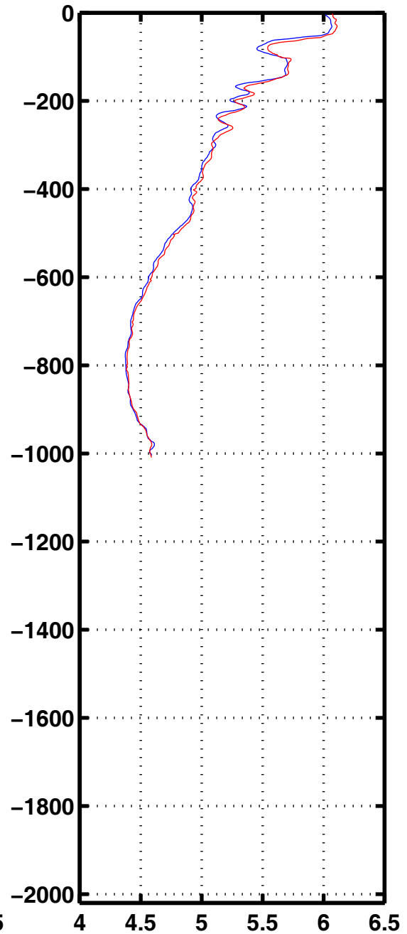
Oxyg 2175
