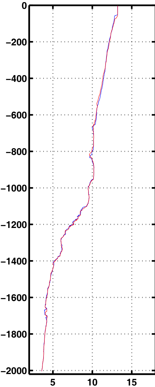
Tempe 2024
