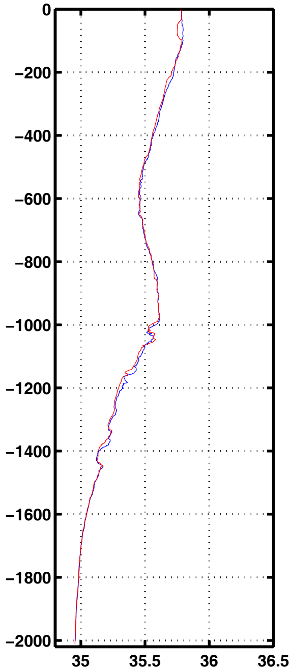
Sali 2050
