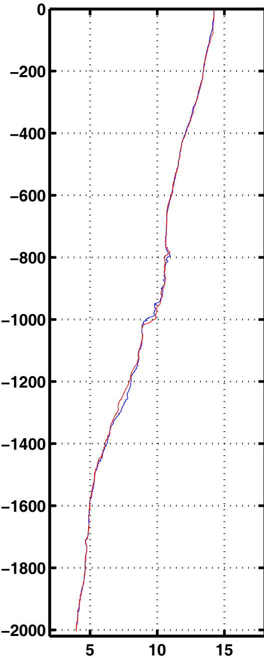
Tempe 2029
