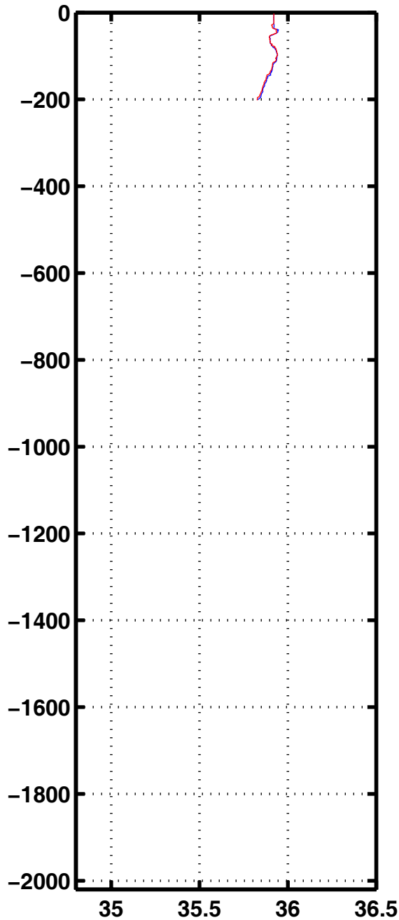
Sali 2083
