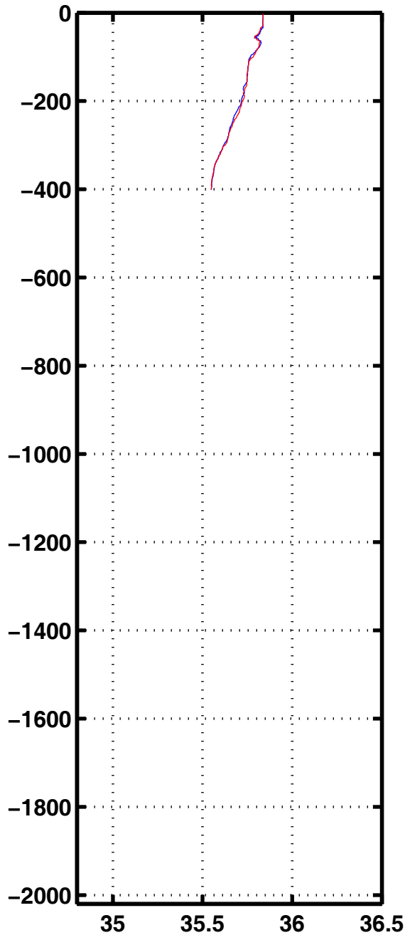
Sali 2176
