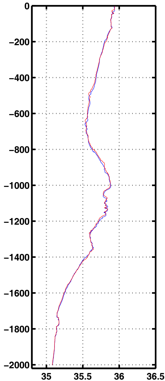
Sali 2095
