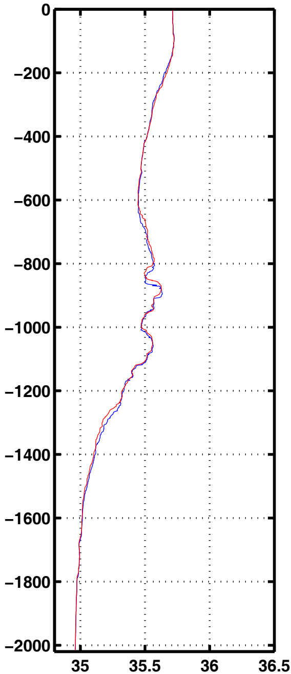
Sali 2051
