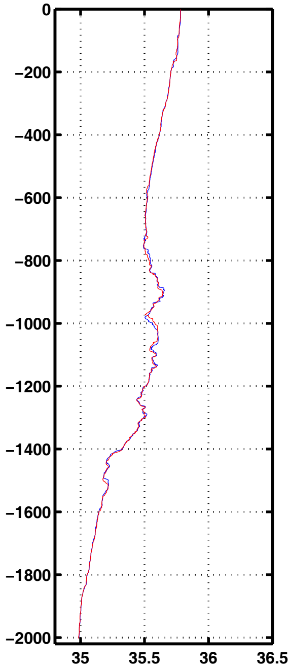
Sali 2414
