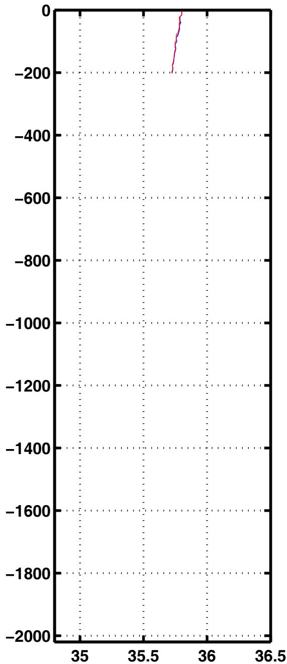
Sali 2181
