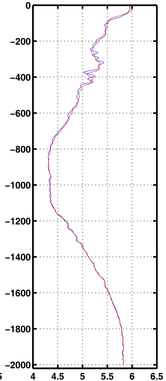
Oxyg 2279
