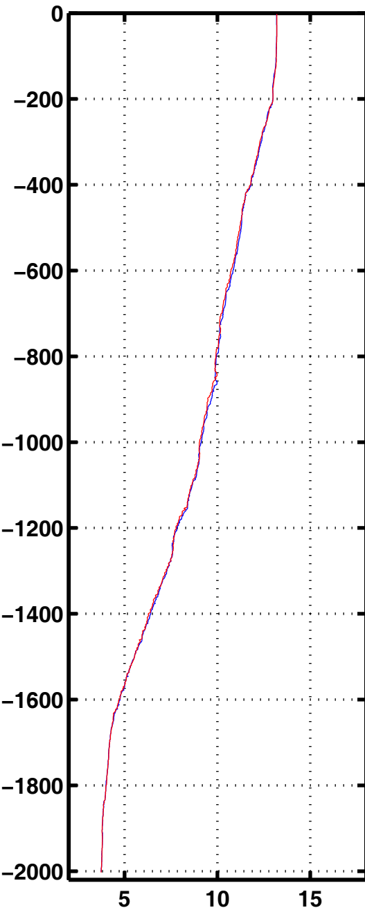
Tempe 2020
