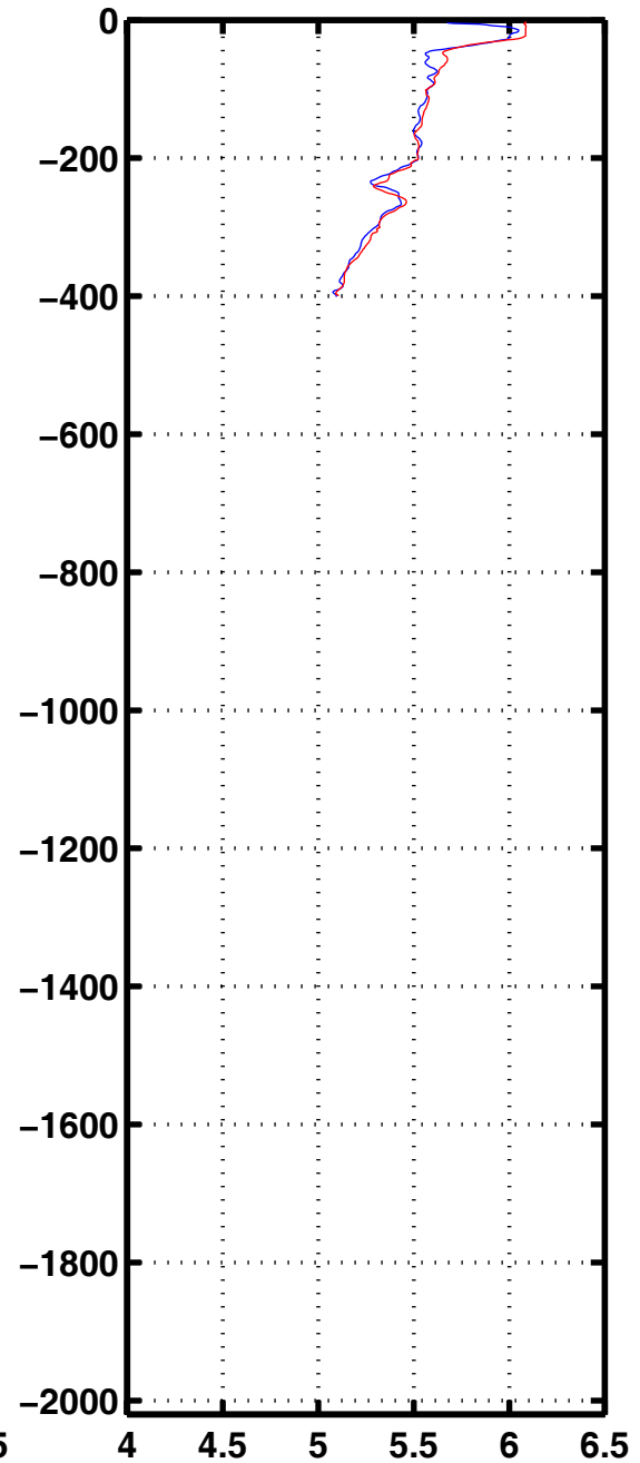
Oxyg 2089
