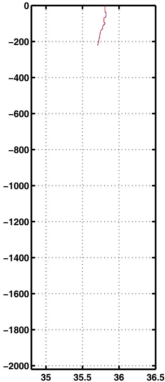
Sali 2275
