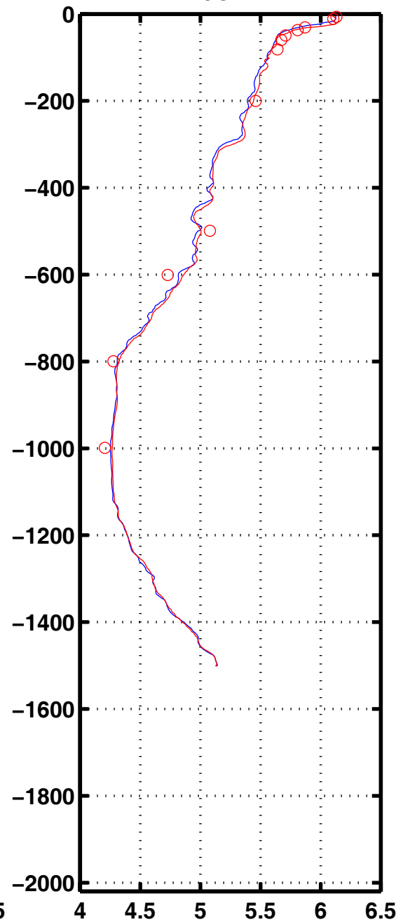
Oxyg 2085
