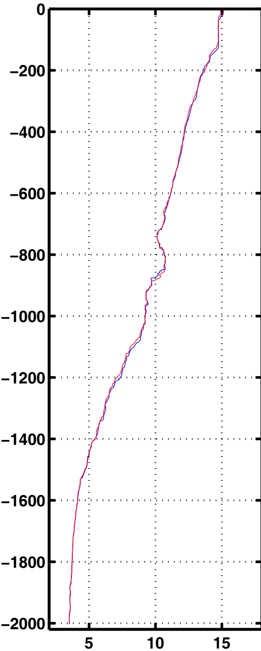
Tempe 2067
