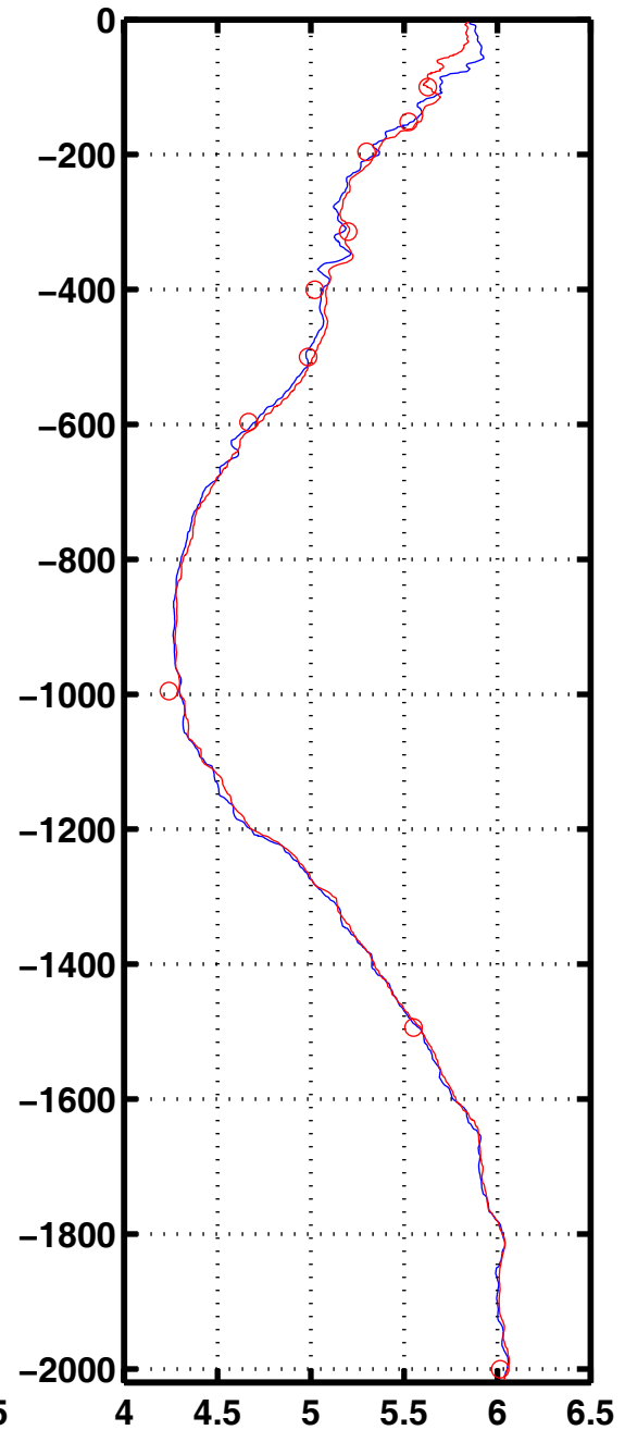
Oxyg 2037
