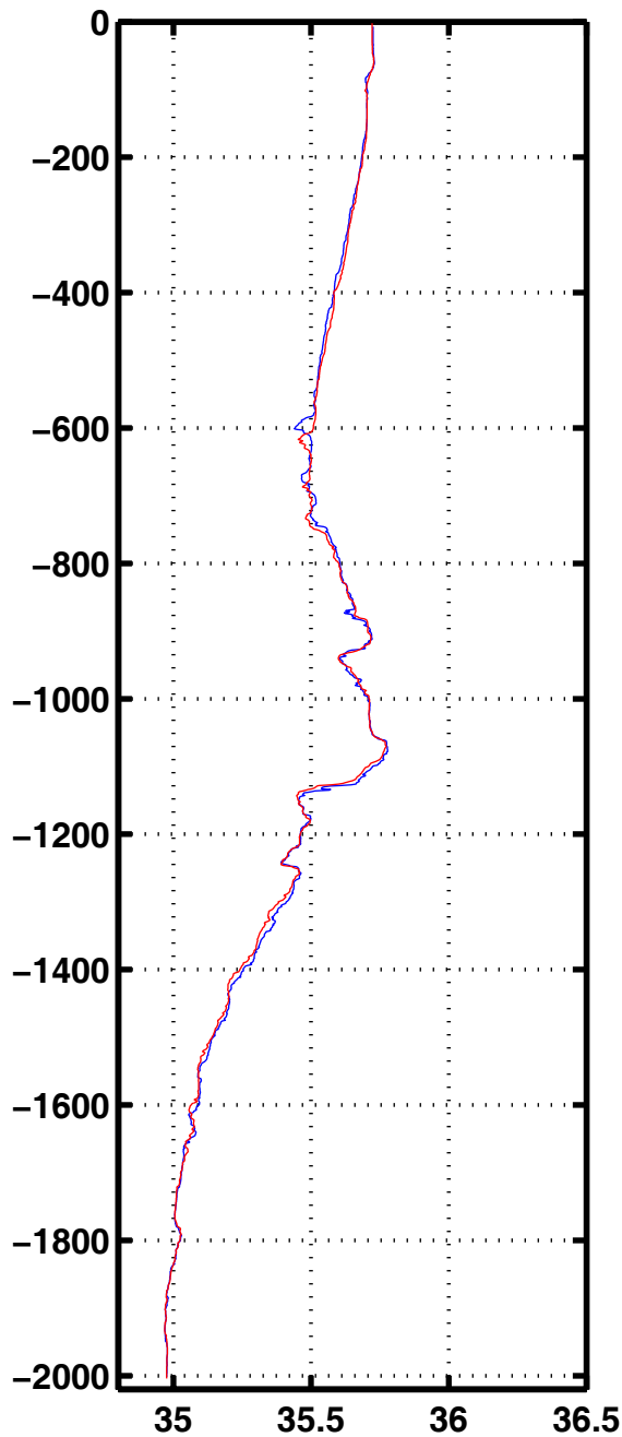
Sali 2025
