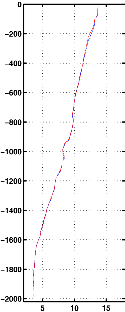
Tempe 2048
