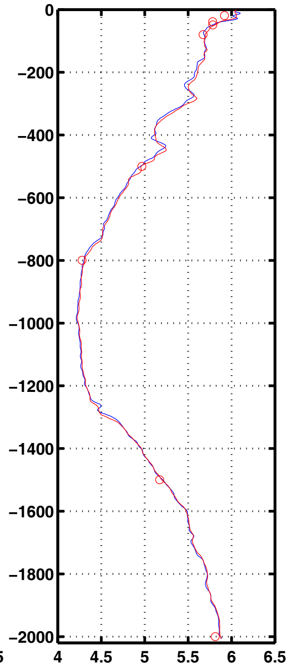
Oxyg 2077
