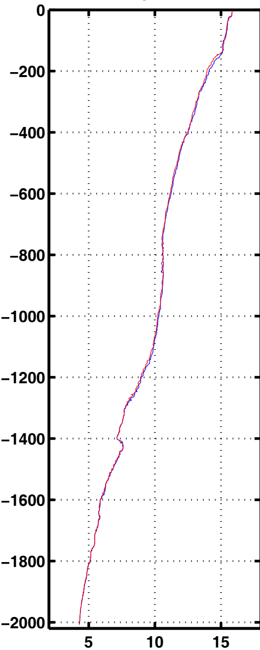
Tempe 2070
