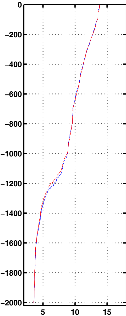
Tempe 2057
