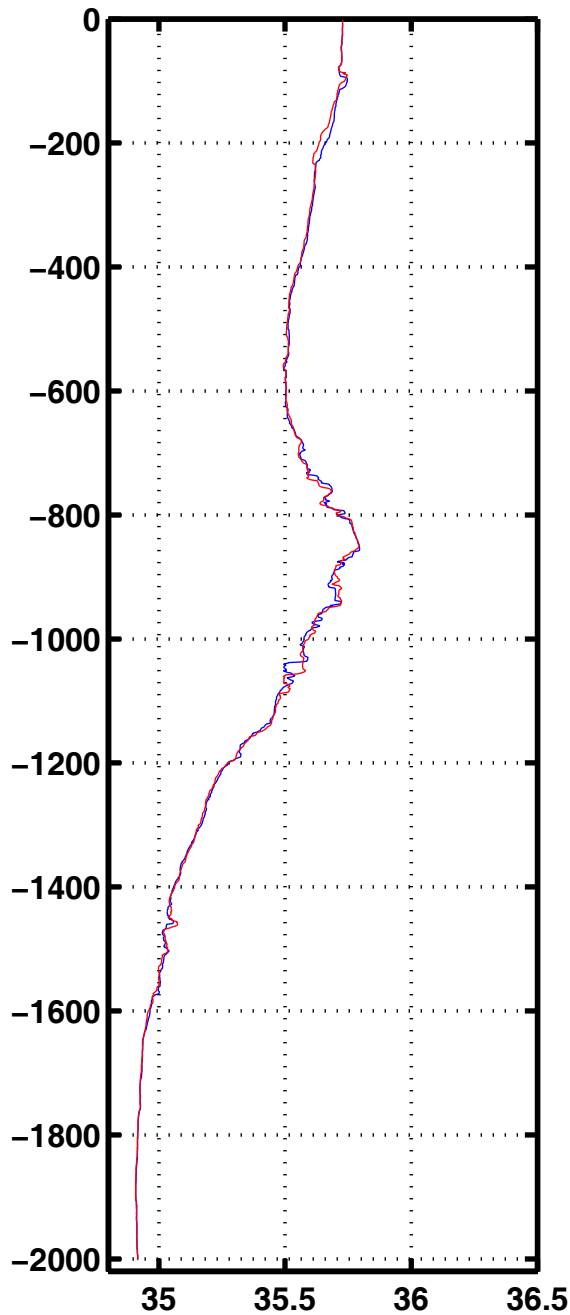
Sali 2012
