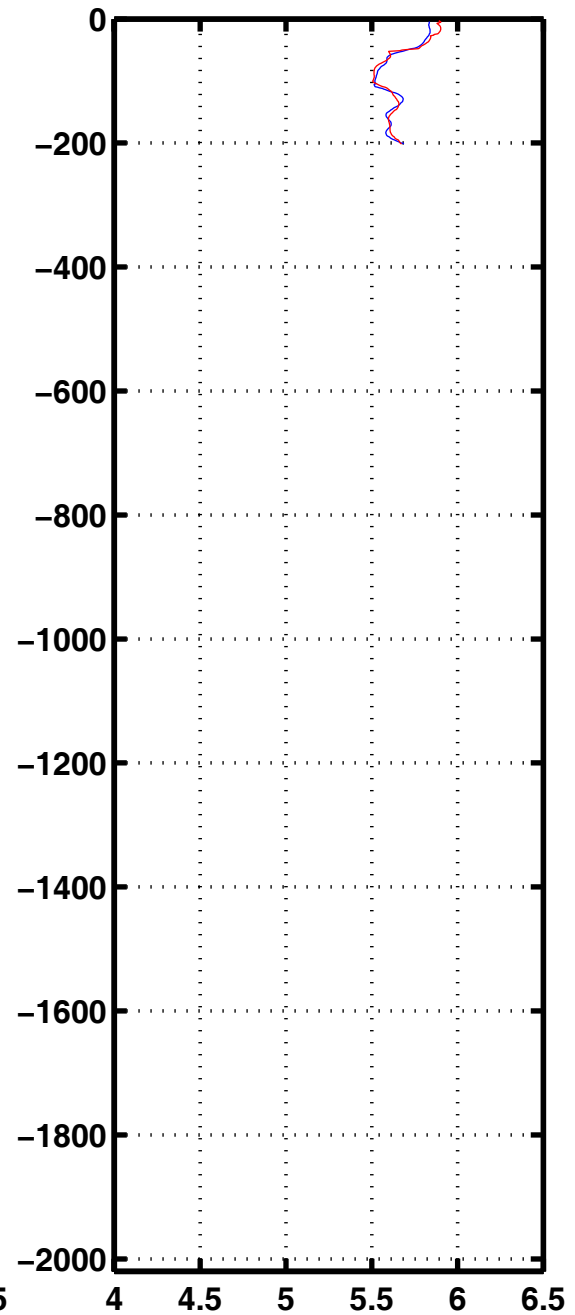
Oxyg 2412
