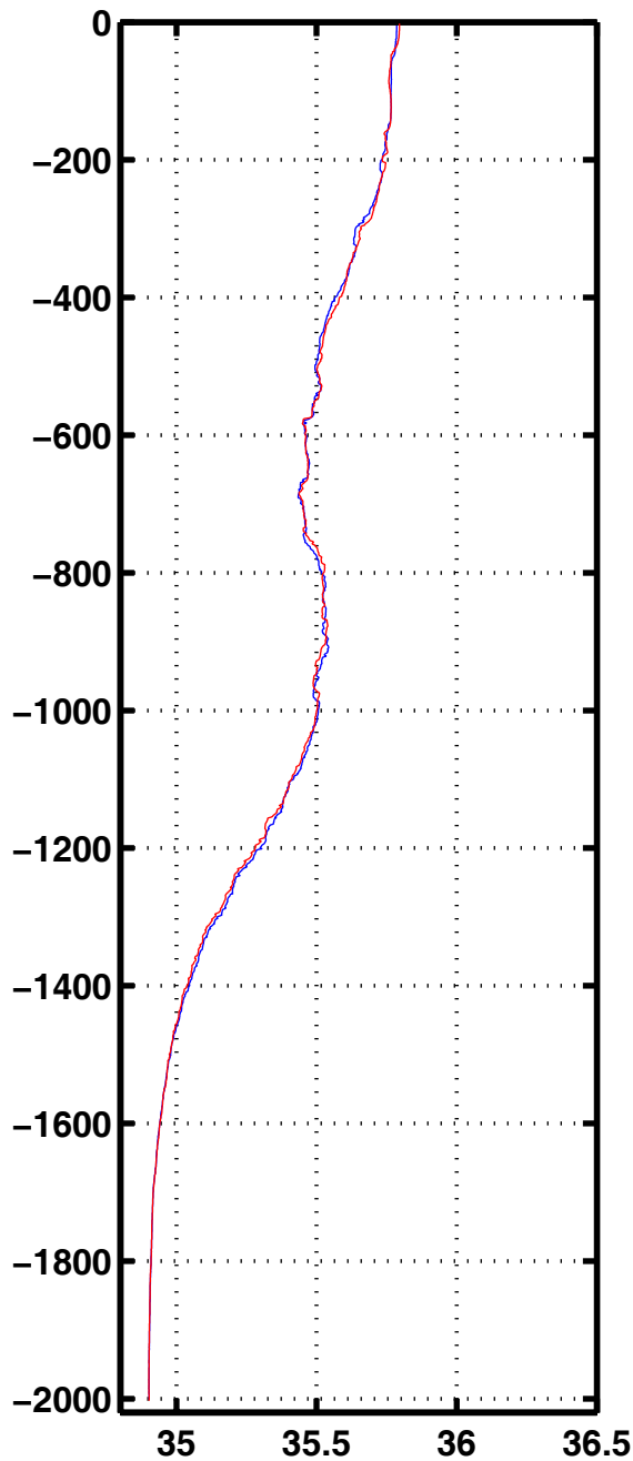
Sali 2053
