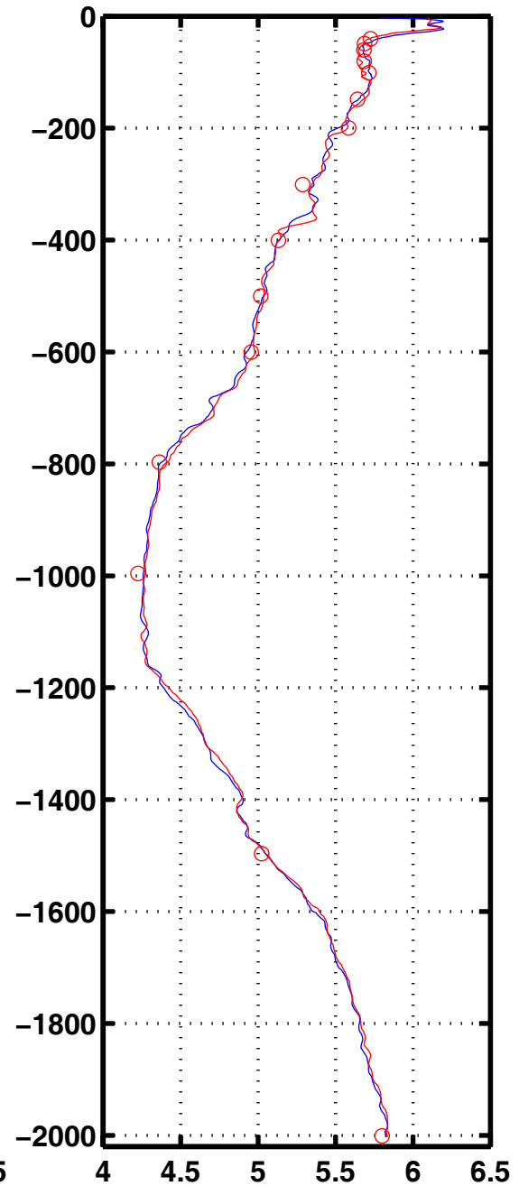
Oxyg 2078
