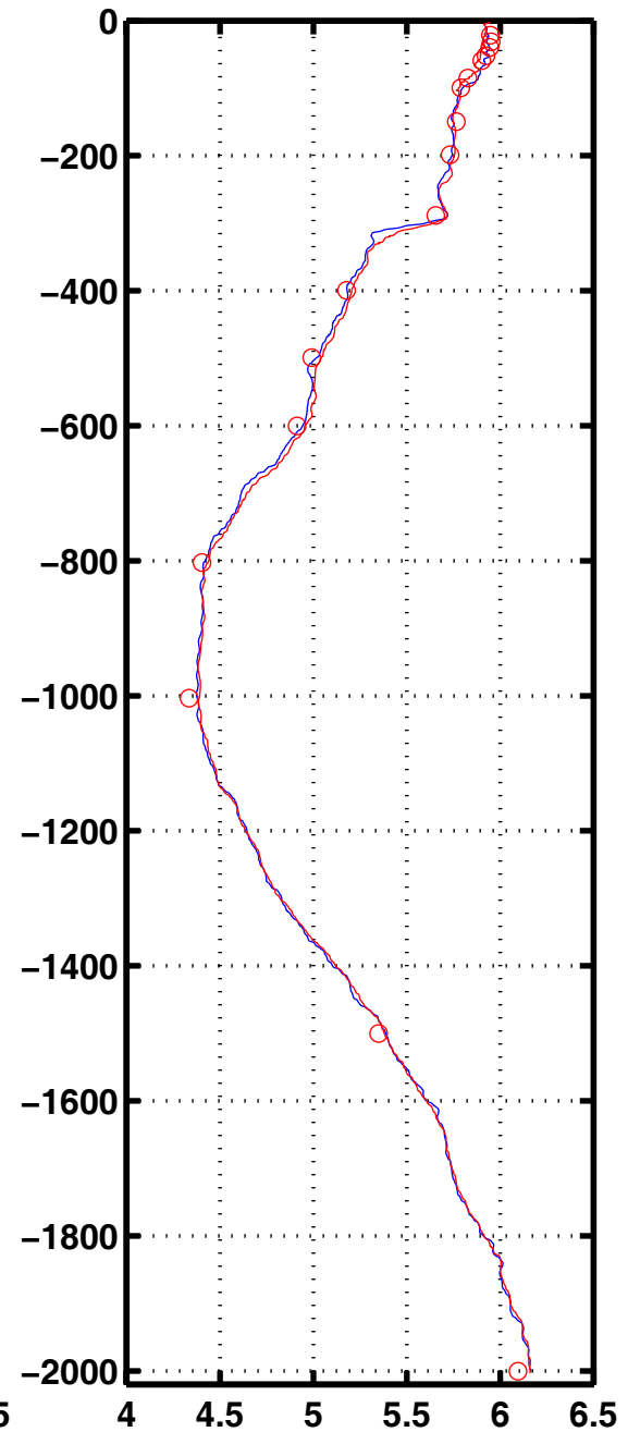
Oxyg 2022
