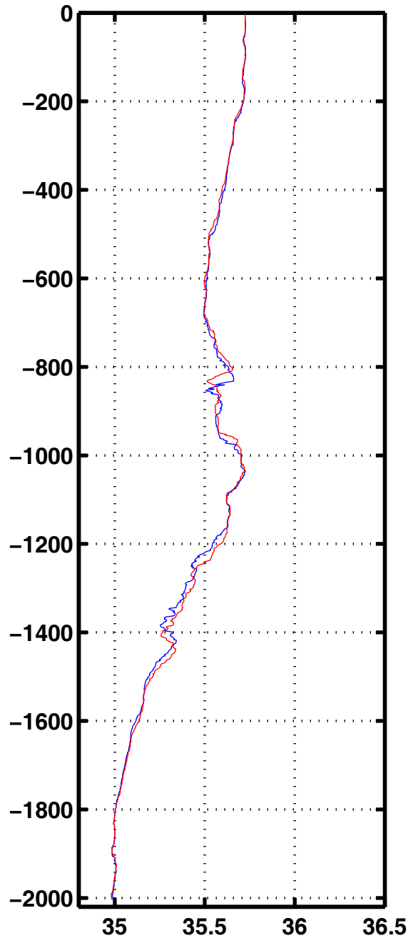
Sali 2027
