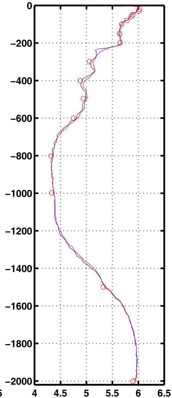
Oxyg 2035
