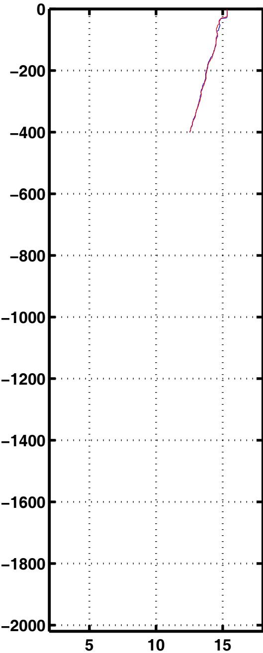
Tempe 2089
