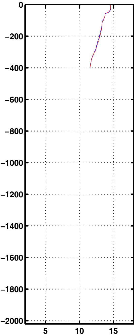
Tempe 2176
