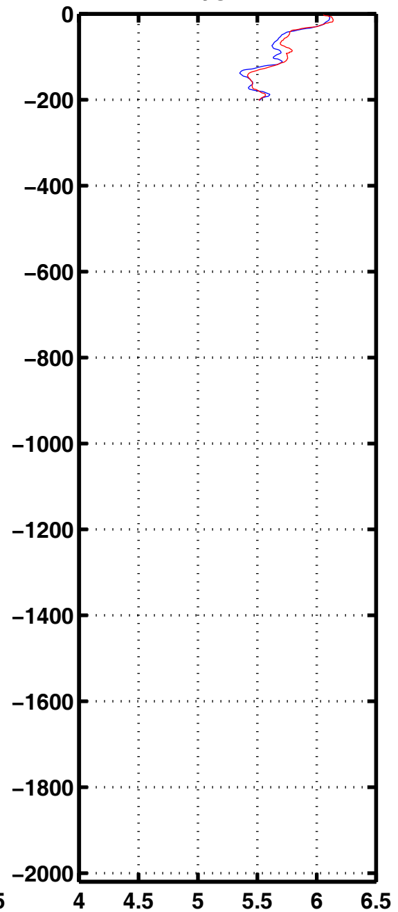
Oxyg 2181
