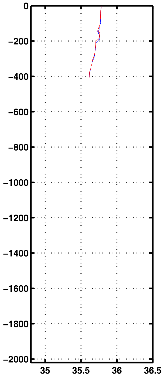
Sali 2410
