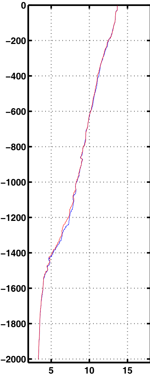
Tempe 2060
