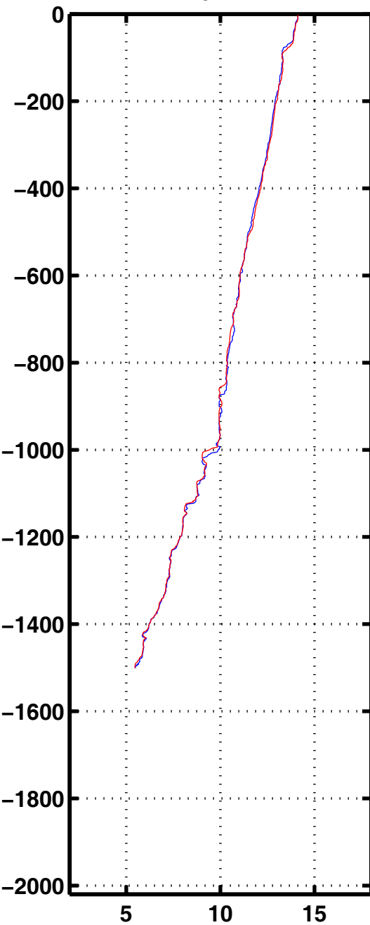
Tempe 2406
