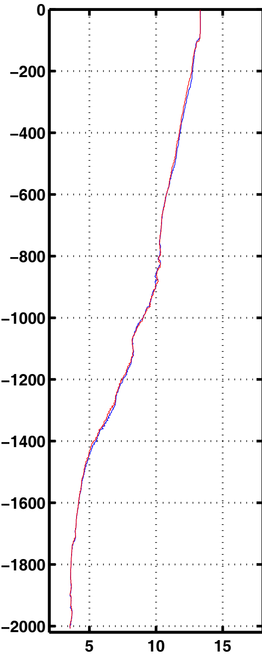
Tempe 2023
