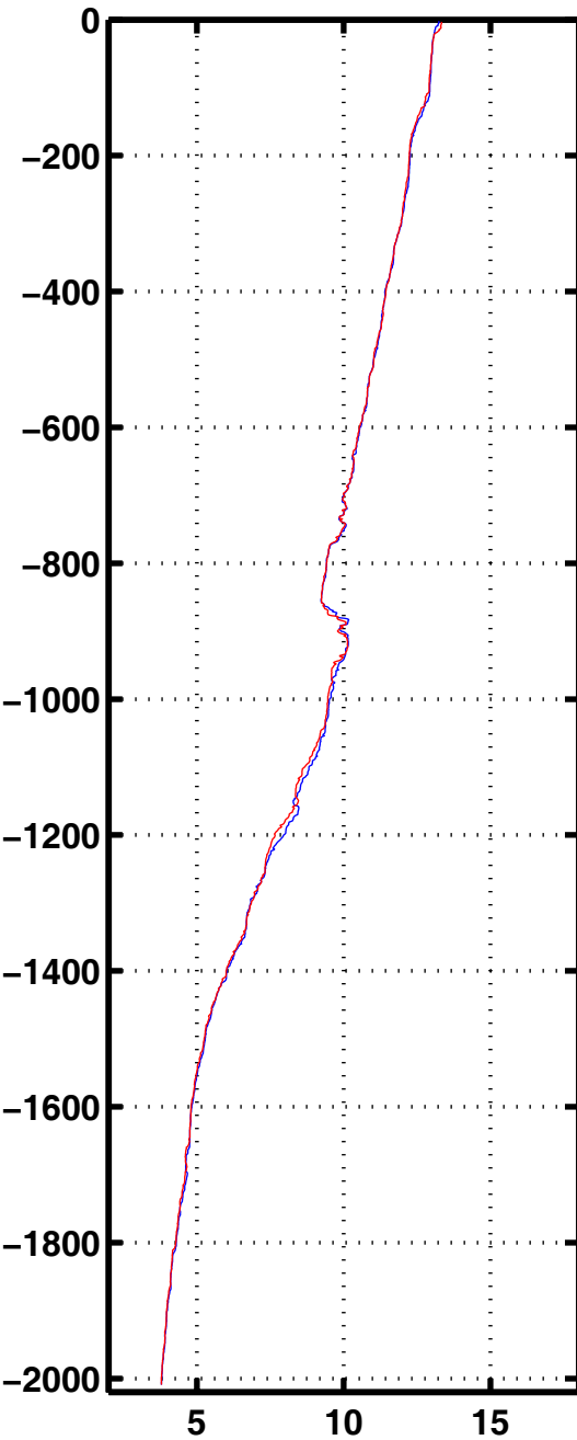
Tempe 2007
