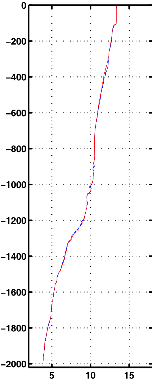
Tempe 2042
