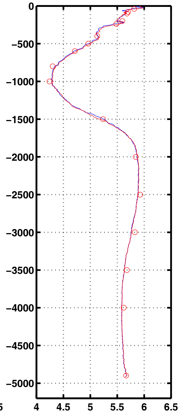
Oxyg 2081
