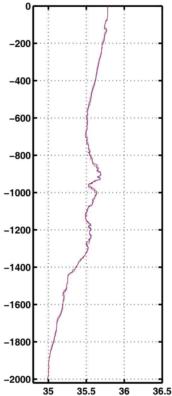
Sali 2416
