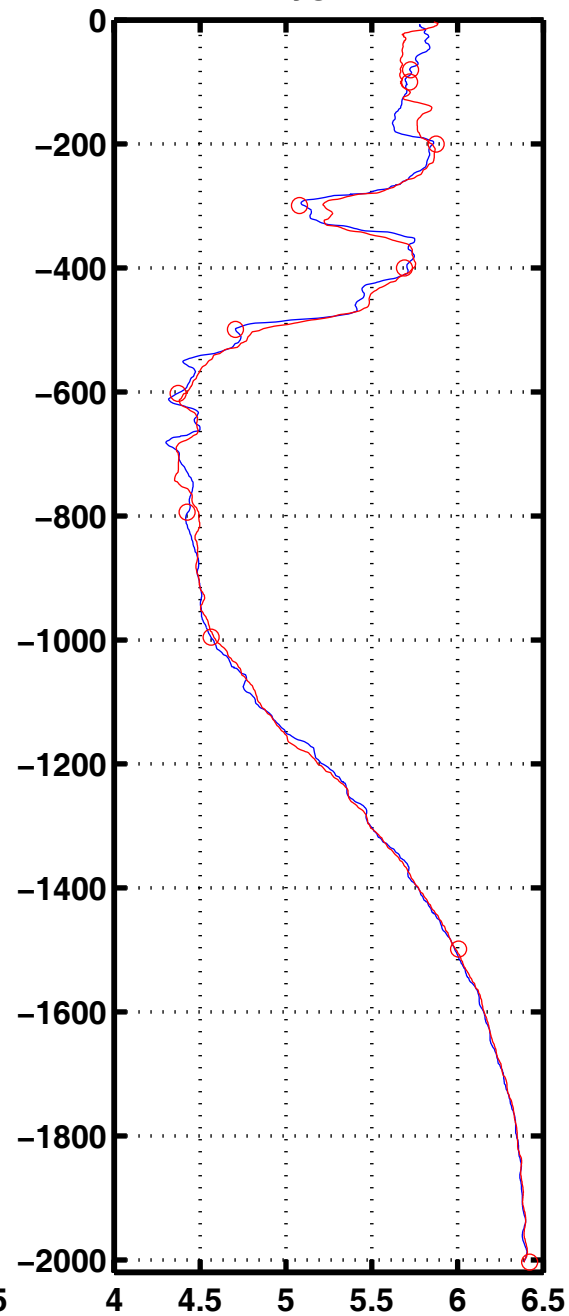
Oxyg 2013
