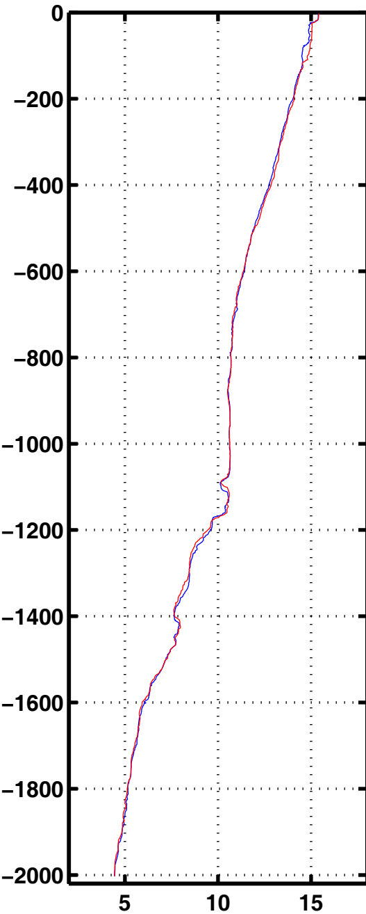
Tempe 2078
