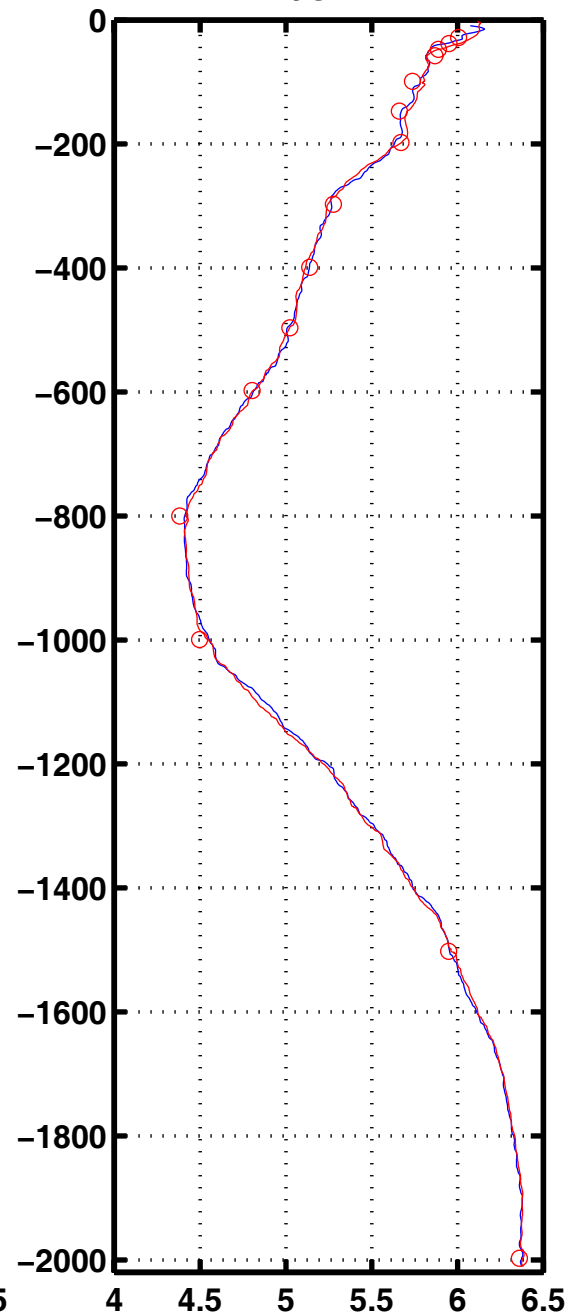
Oxyg 2061
