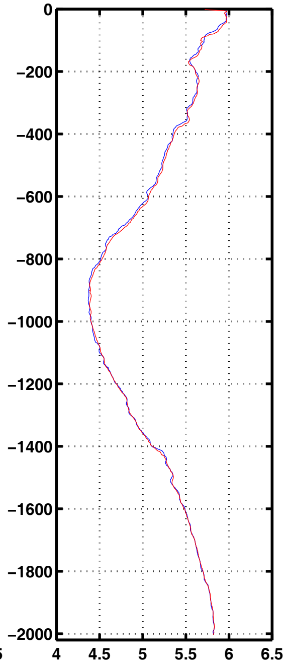
Oxyg 2414
