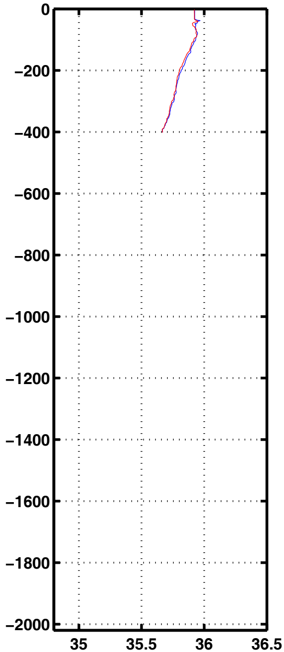
Sali 2091
