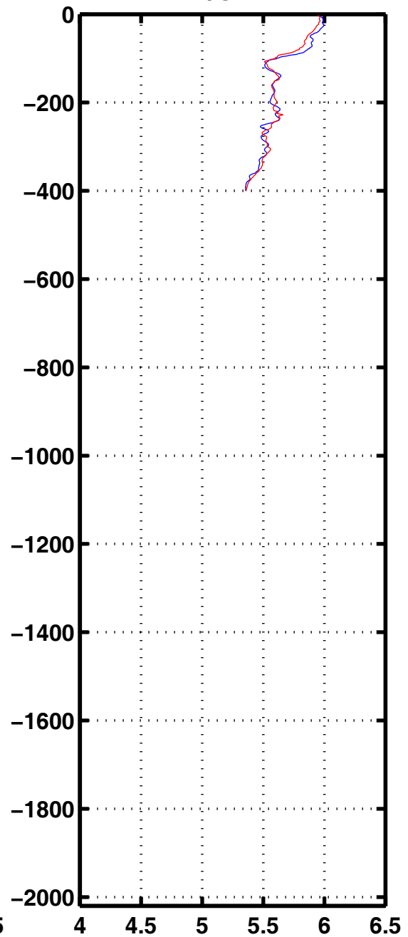
Oxyg 2408
