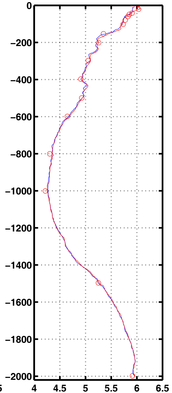
Oxyg 2031
