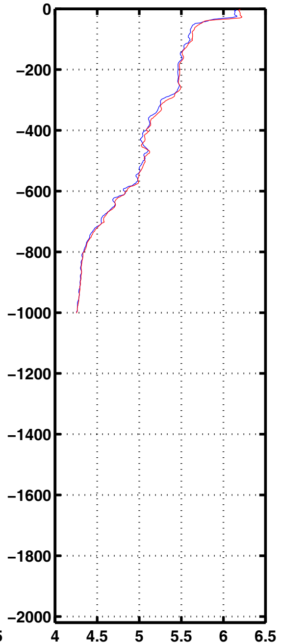
Oxyg 2088
