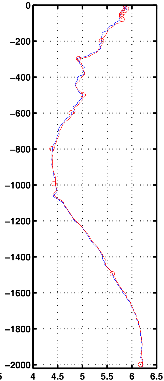
Oxyg 2049
