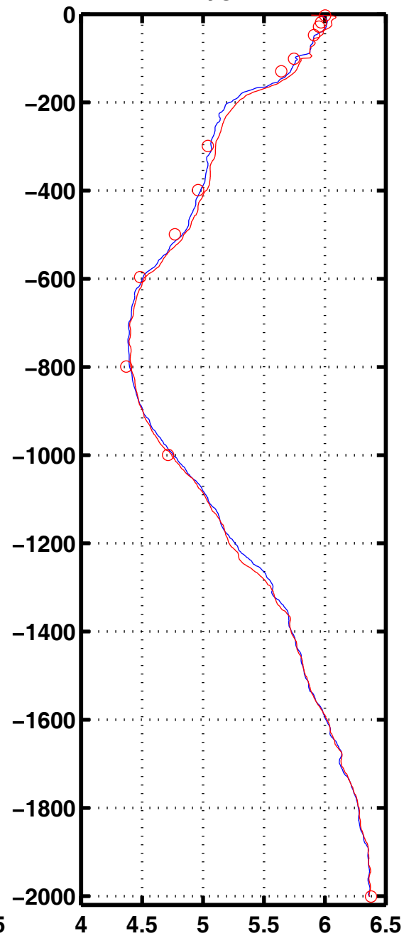
Oxyg 2056
