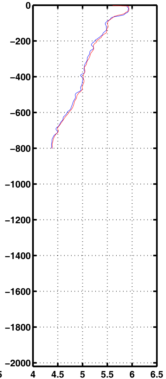
Oxyg 2274
