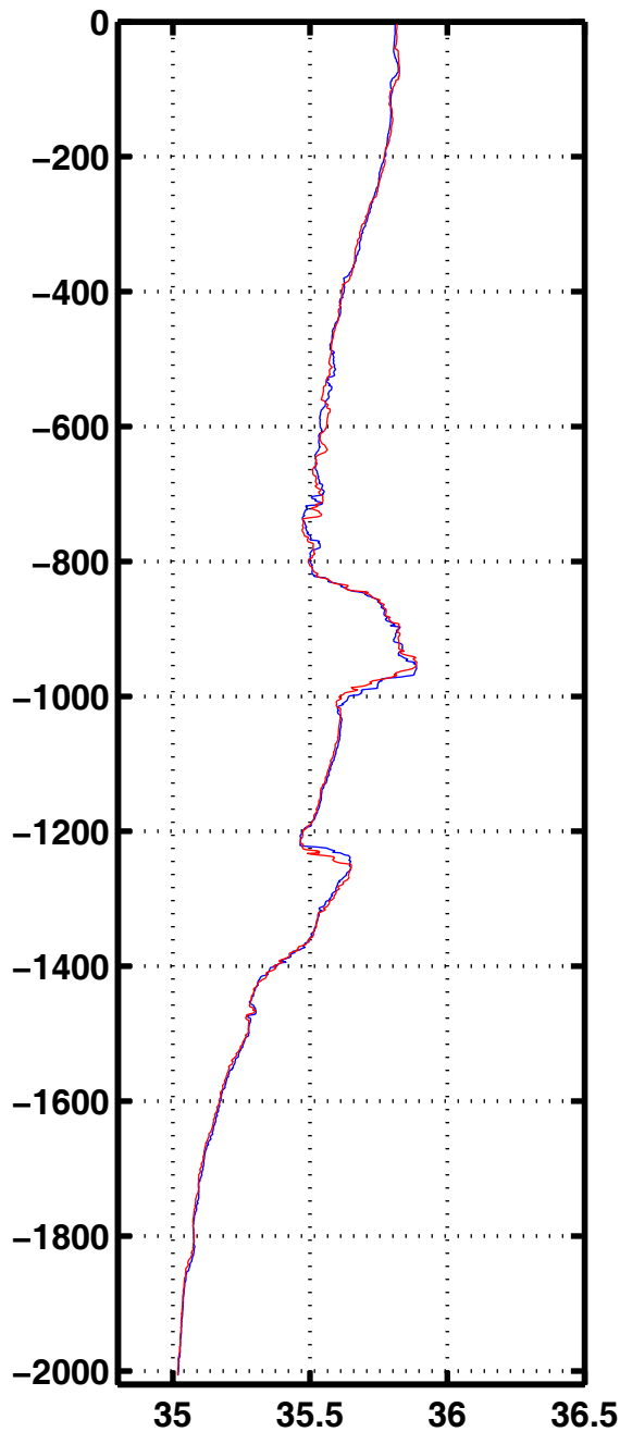
Sali 2028
