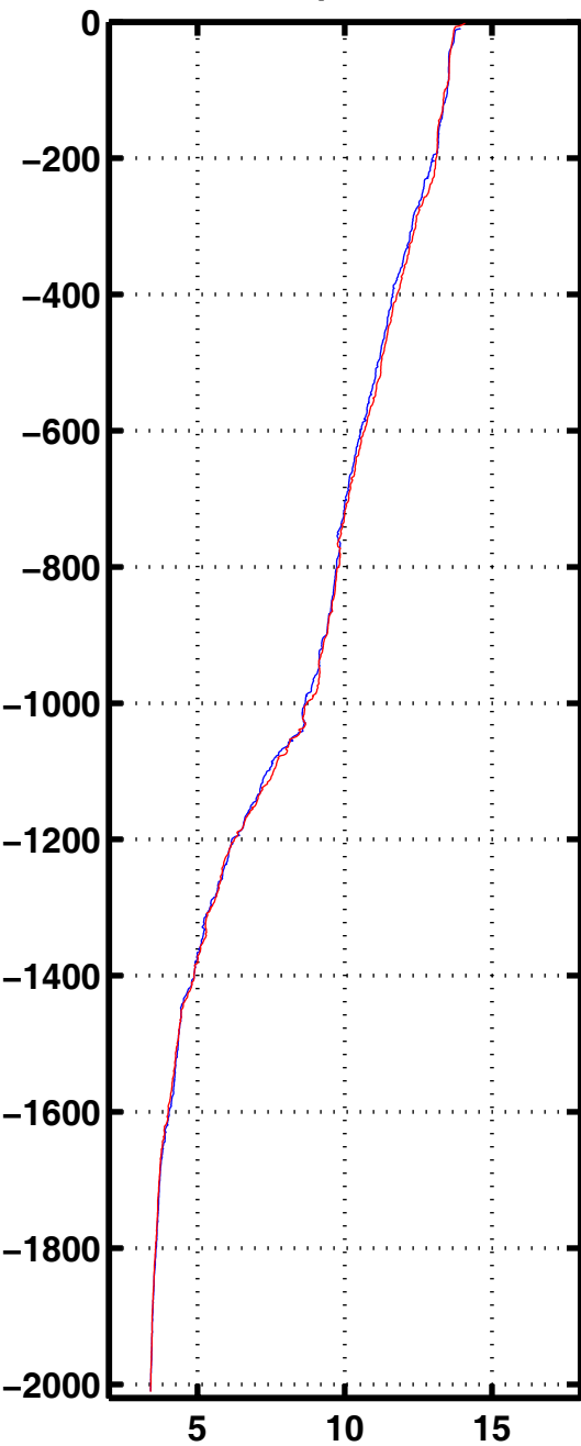
Tempe 2061
