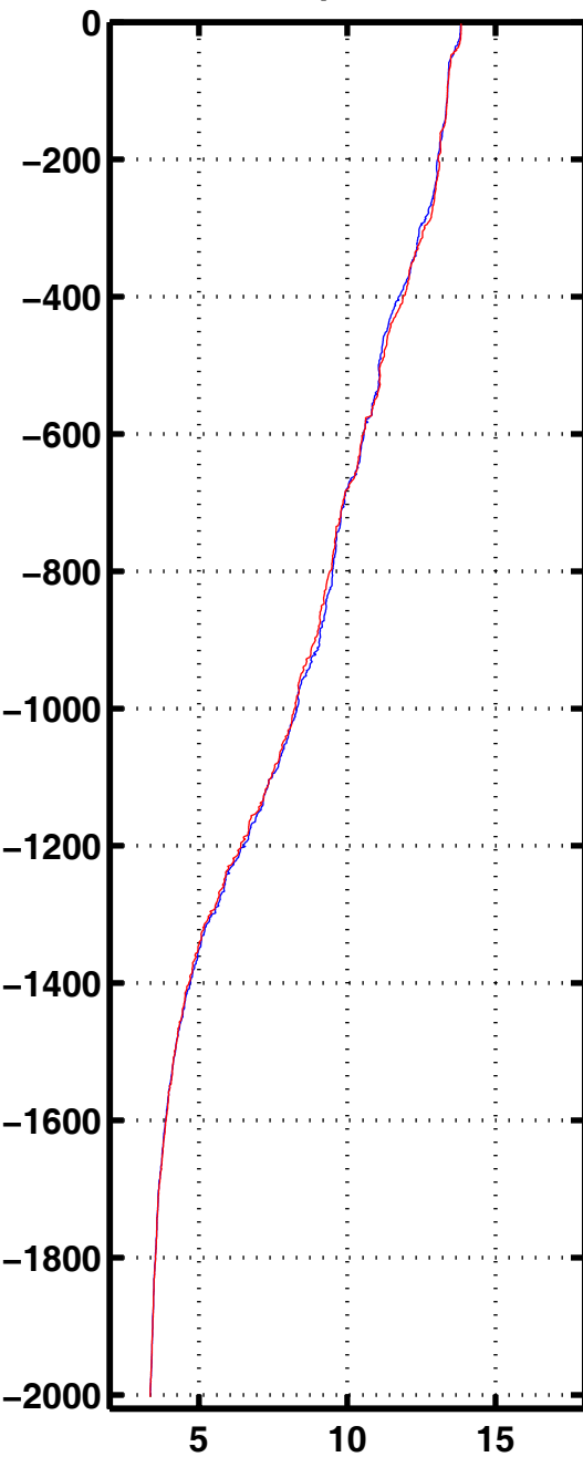
Tempe 2053
