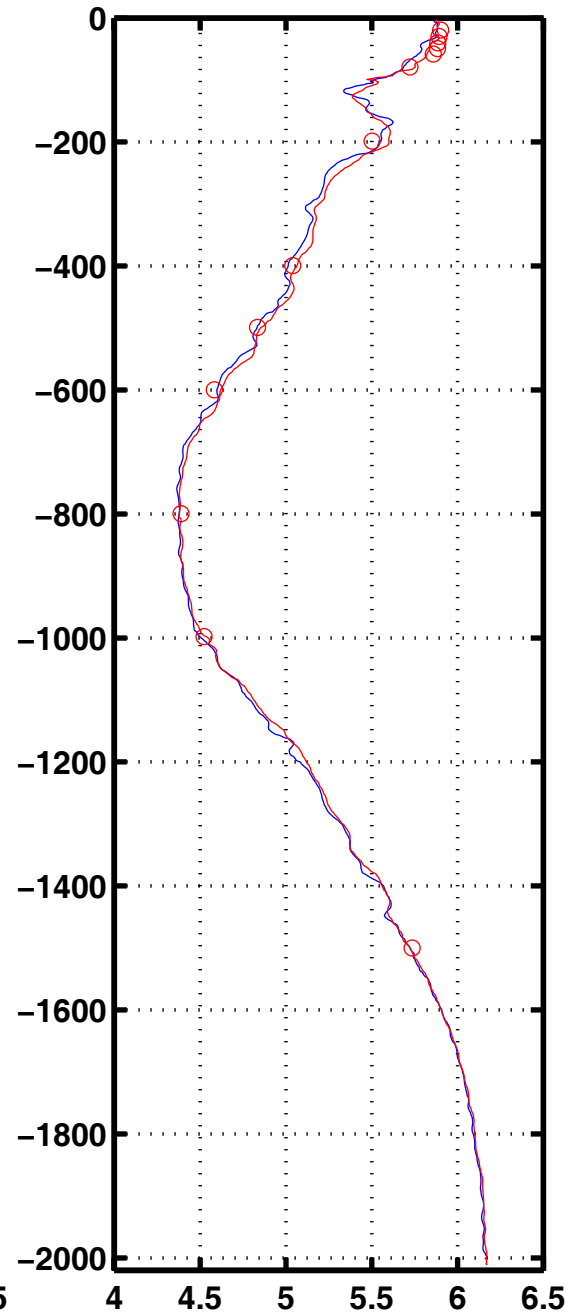
Oxyg 2050
