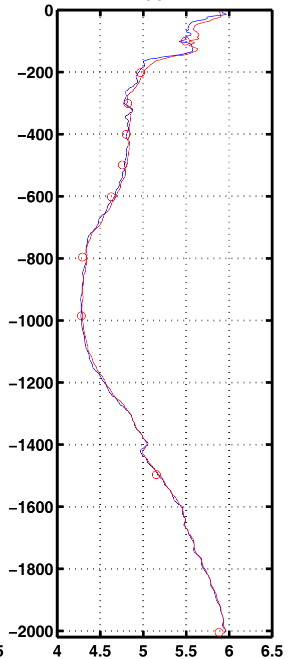
Oxyg 2070
