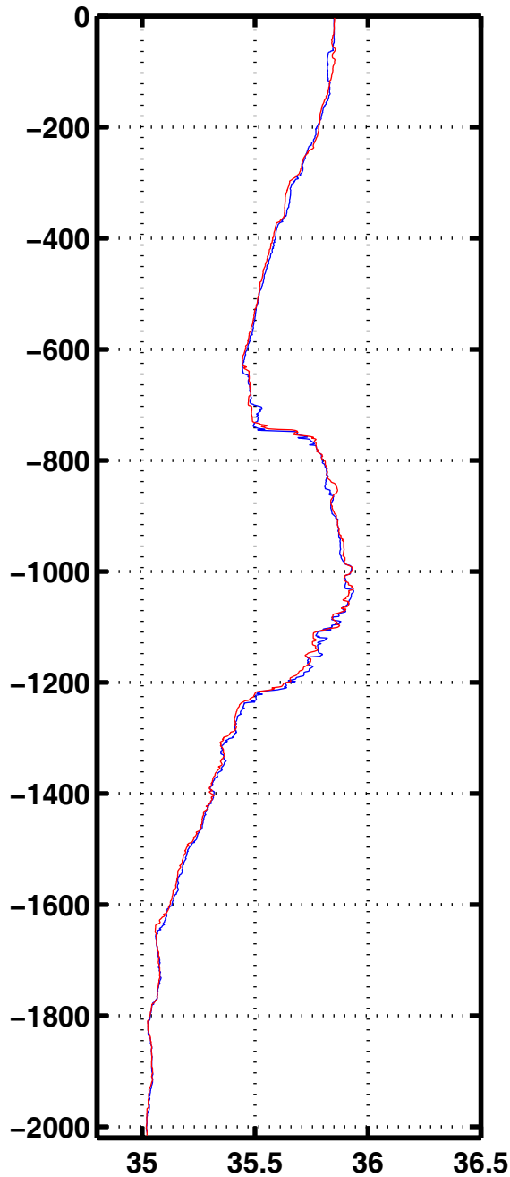
Sali 2037
