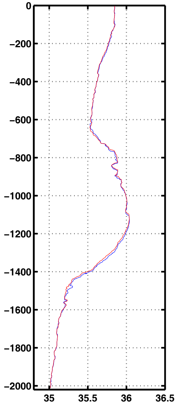
Sali 2075
