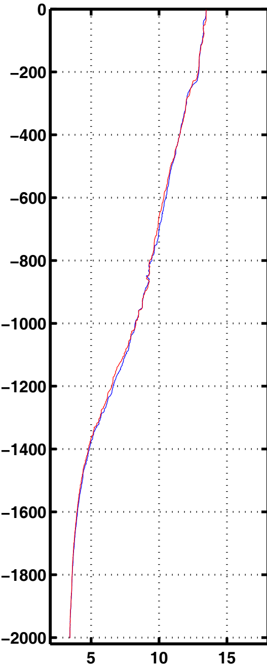
Tempe 1046
