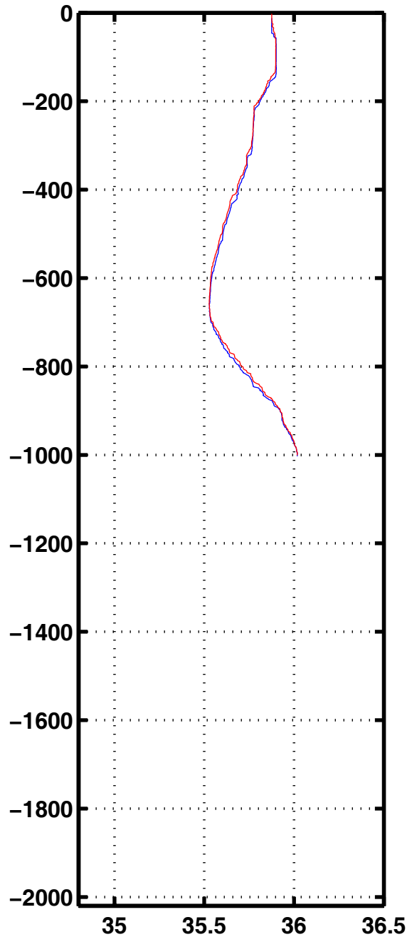
Sali 1099
