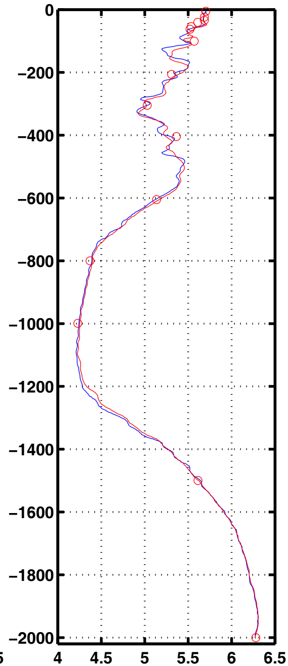
Oxyg 1070
