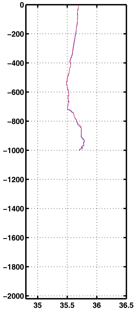
Sali 1188
