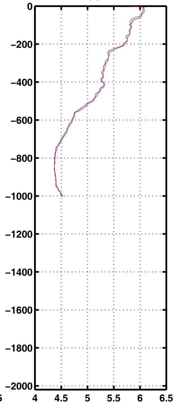
Oxyg 1188
