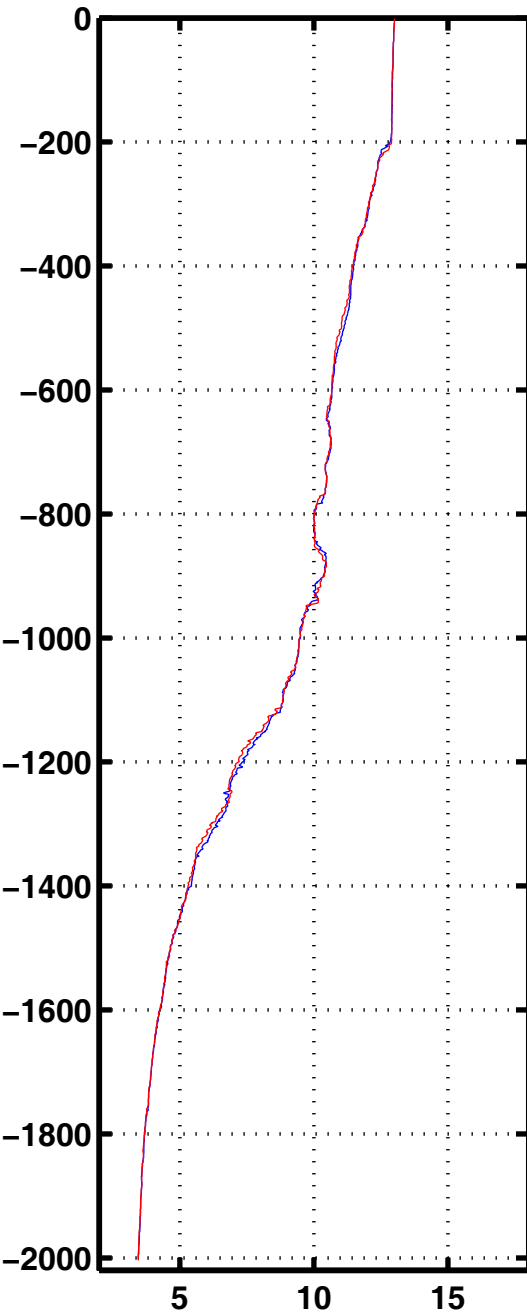
Tempe 1015
