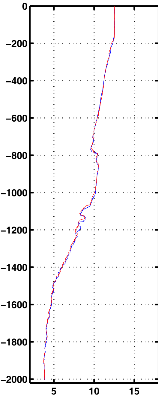
Tempe 1011
