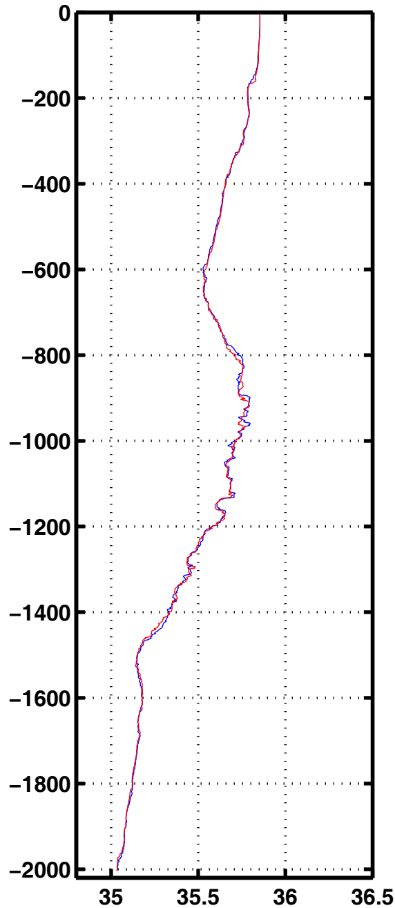
Sali 1028
