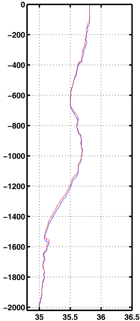
Sali 1006
