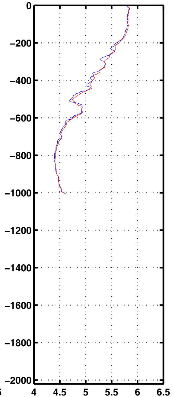
Oxyg 1127
