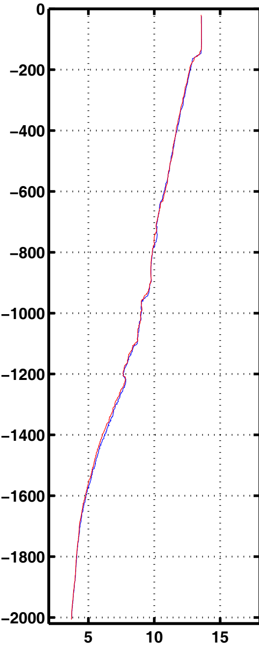
Tempe 1007
