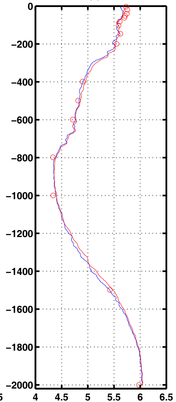
Oxyg 1029
