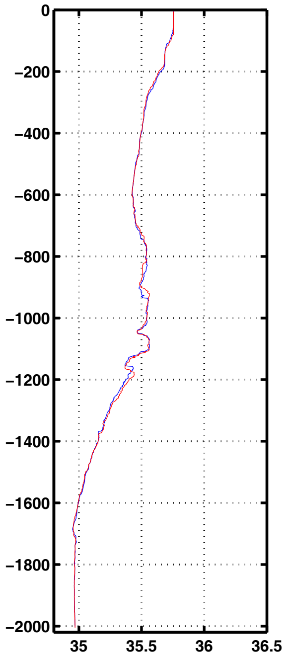
Sali 1062
