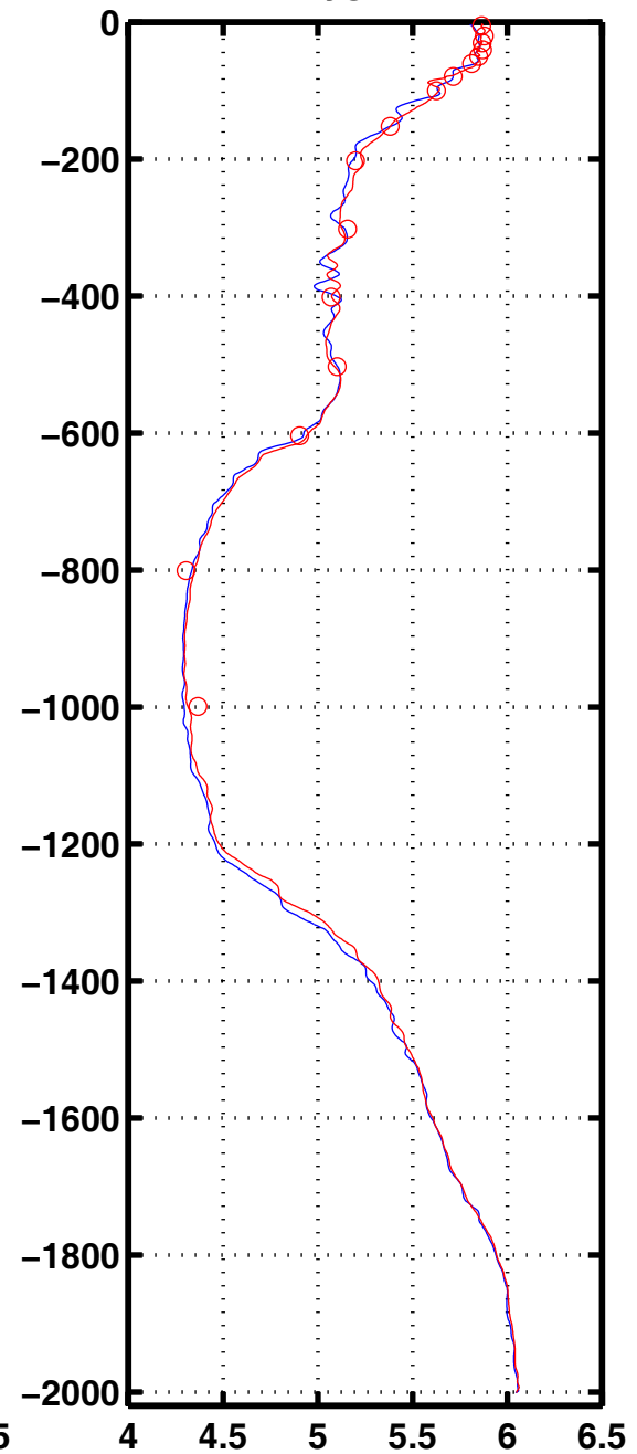
Oxyg 1055
