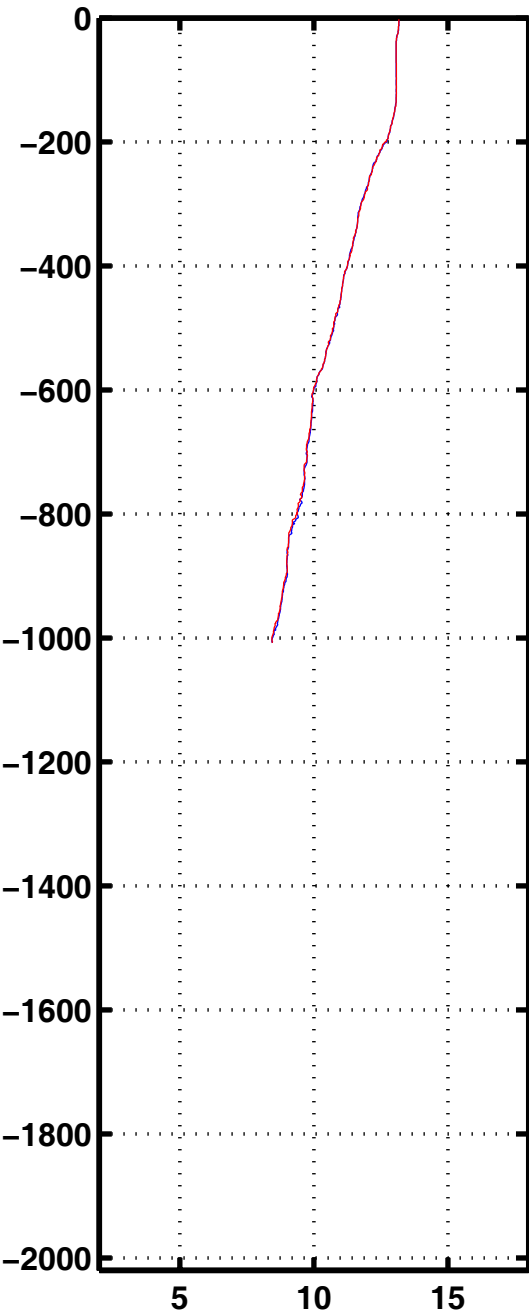
Tempe 1107
