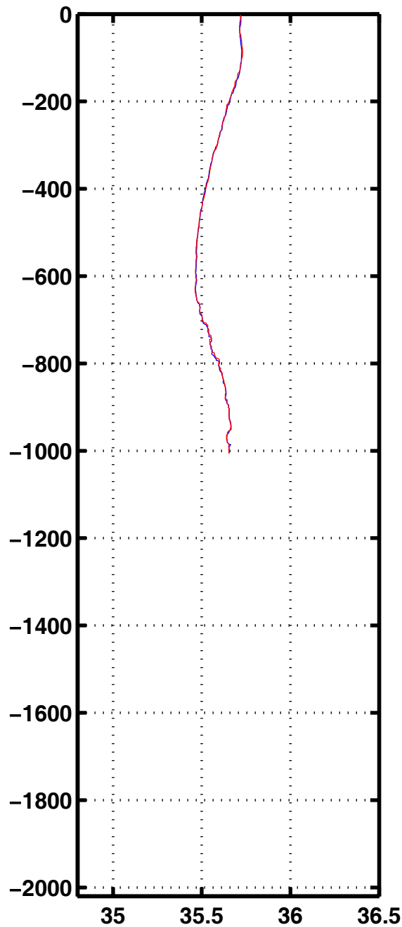
Sali 1106
