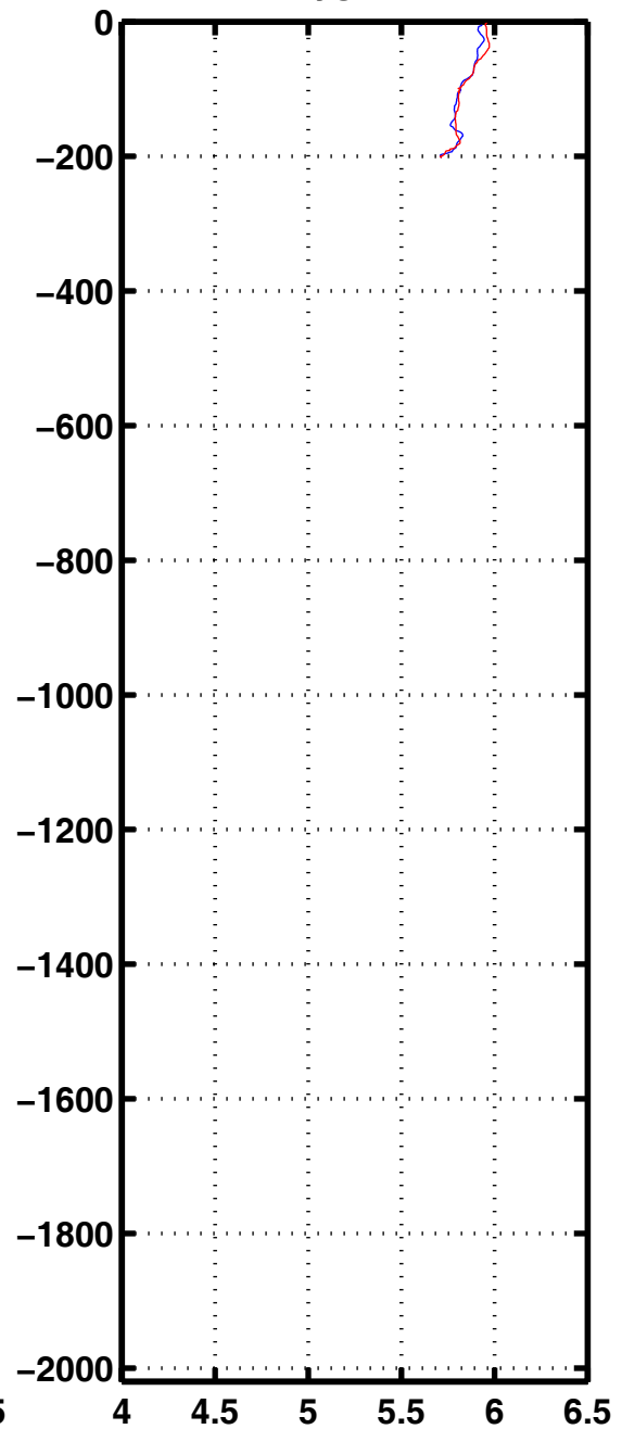
Oxyg 1166
