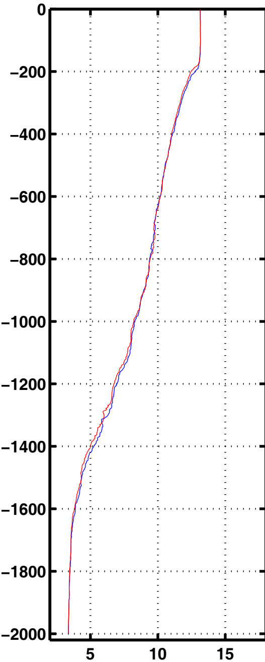
Tempe 1063
