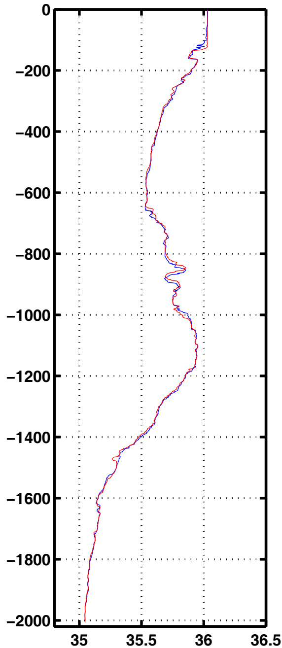
Sali 1060
