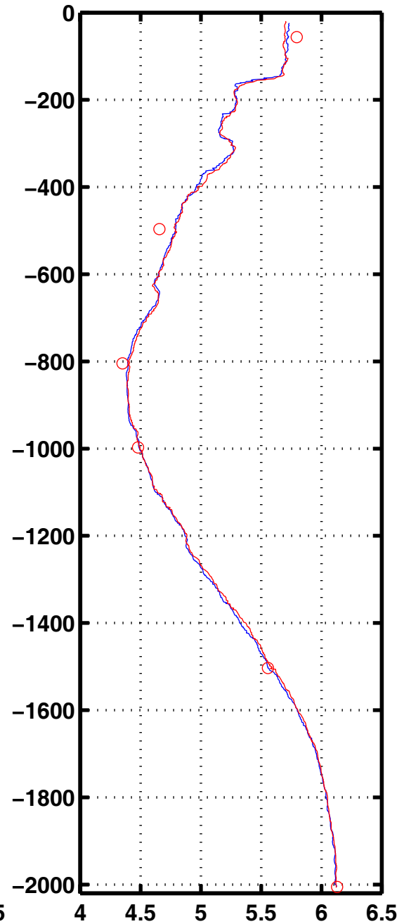
Oxyg 1007
