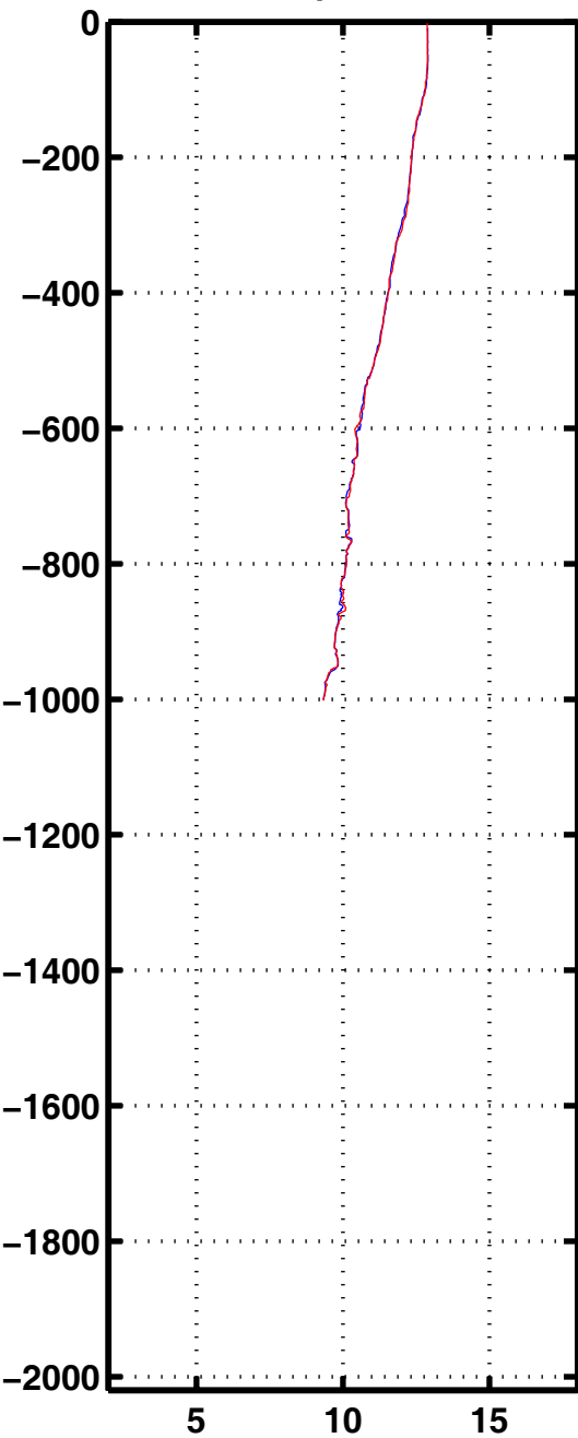
Tempe 1193
