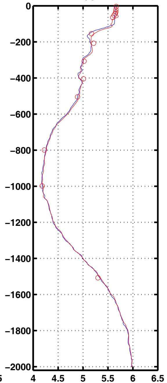
Oxyg 1075
