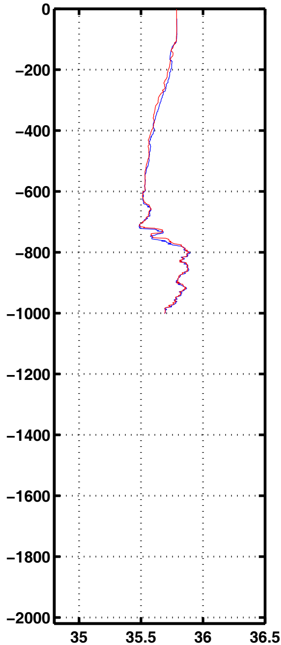
Sali 1113
