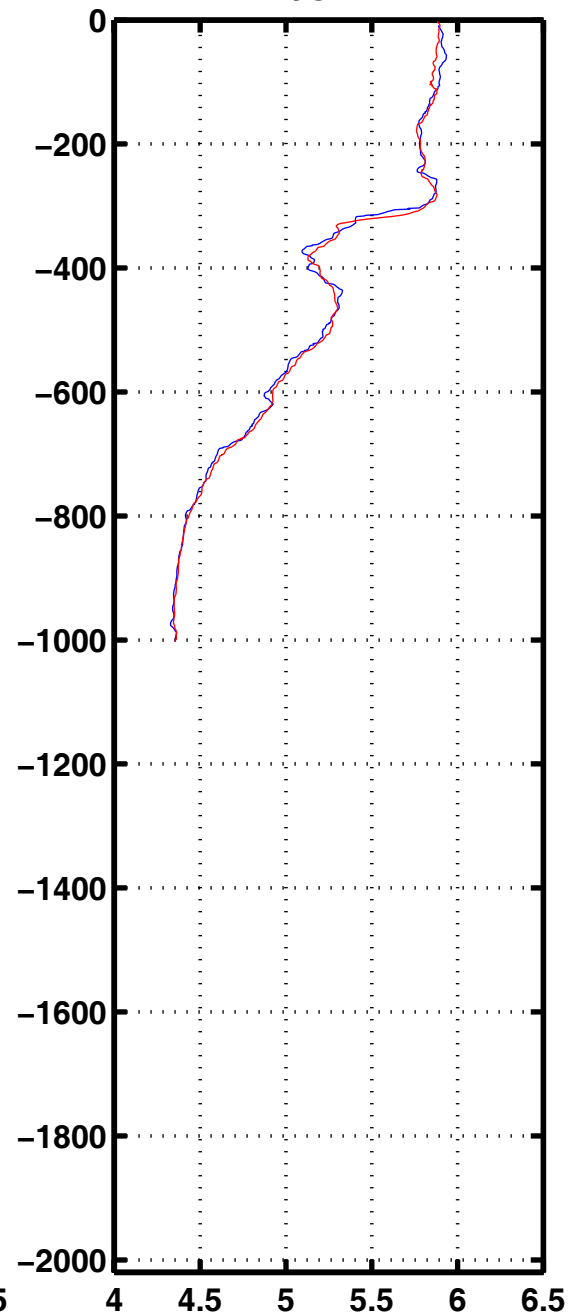
Oxyg 1164
