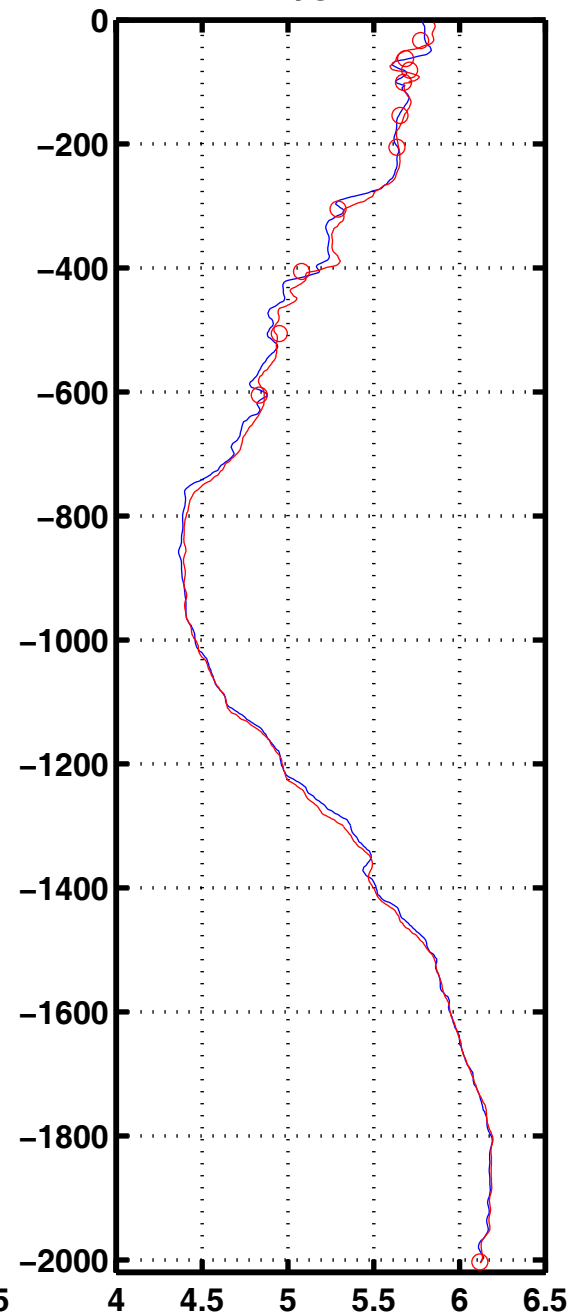
Oxyg 1061
