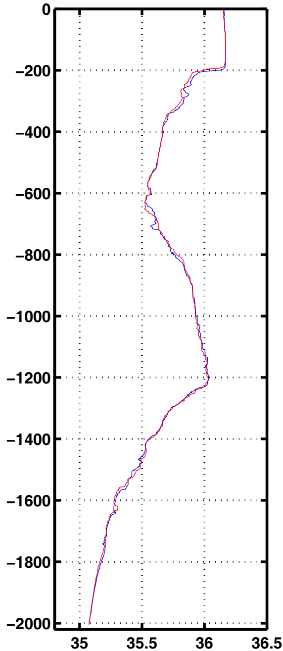
Sali 1080
