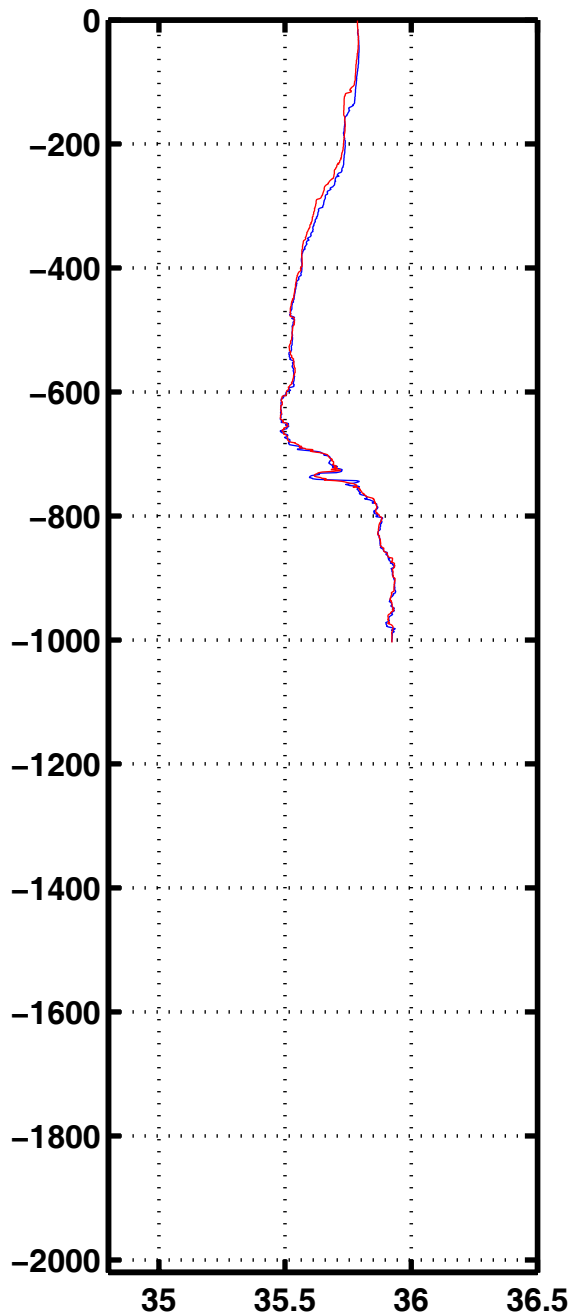
Sali 1110
