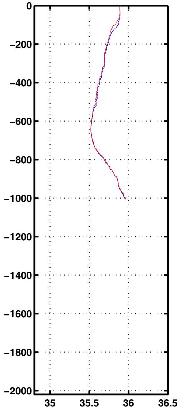
Sali 1096
