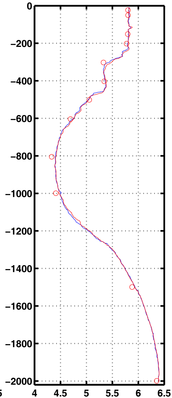
Oxyg 1012
