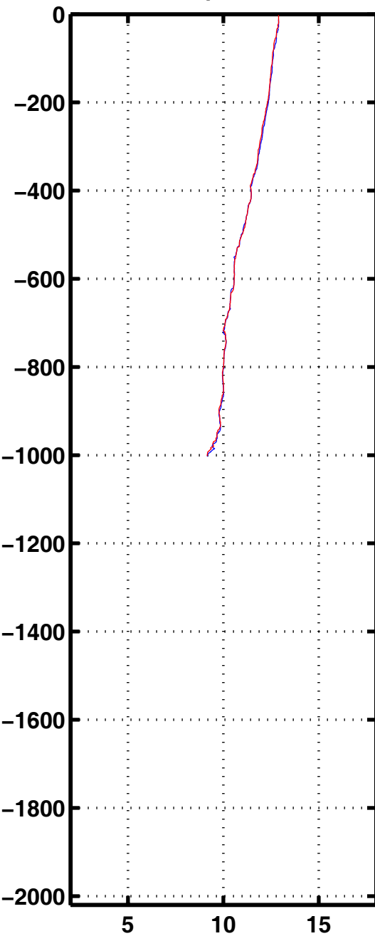
Tempe 1188
