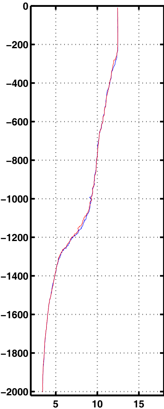
Tempe 1012
