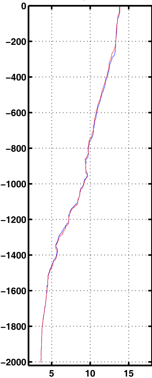
Tempe 1061
