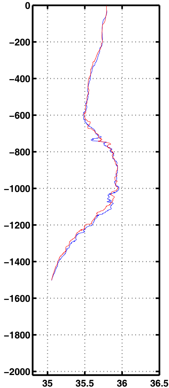
Sali 1109
