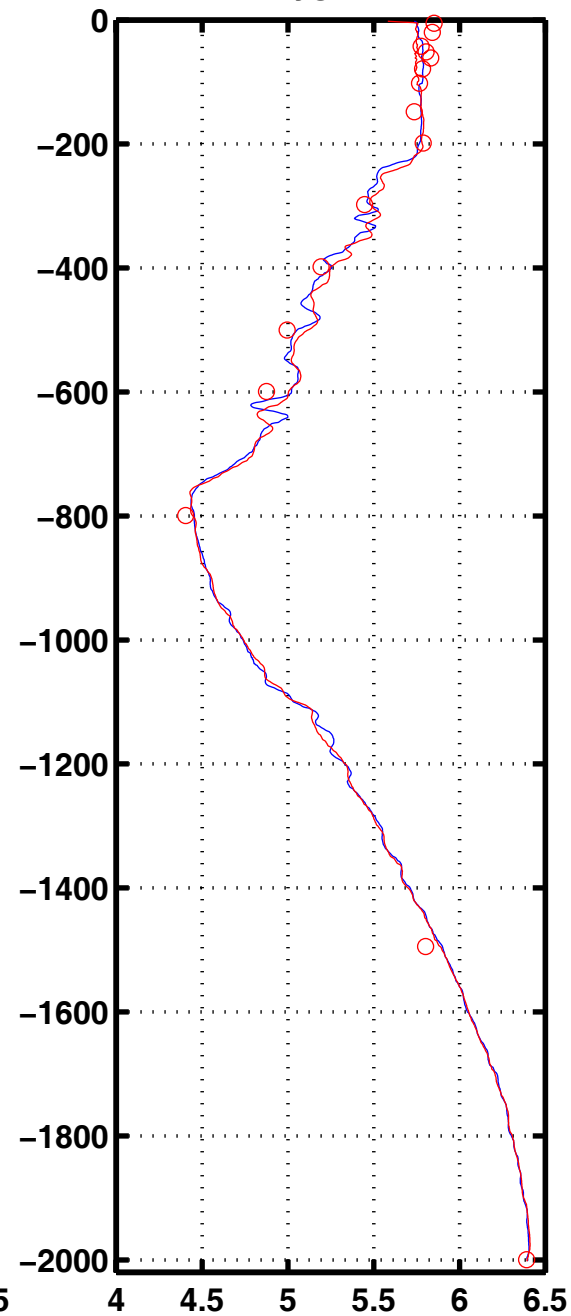
Oxyg 1018
