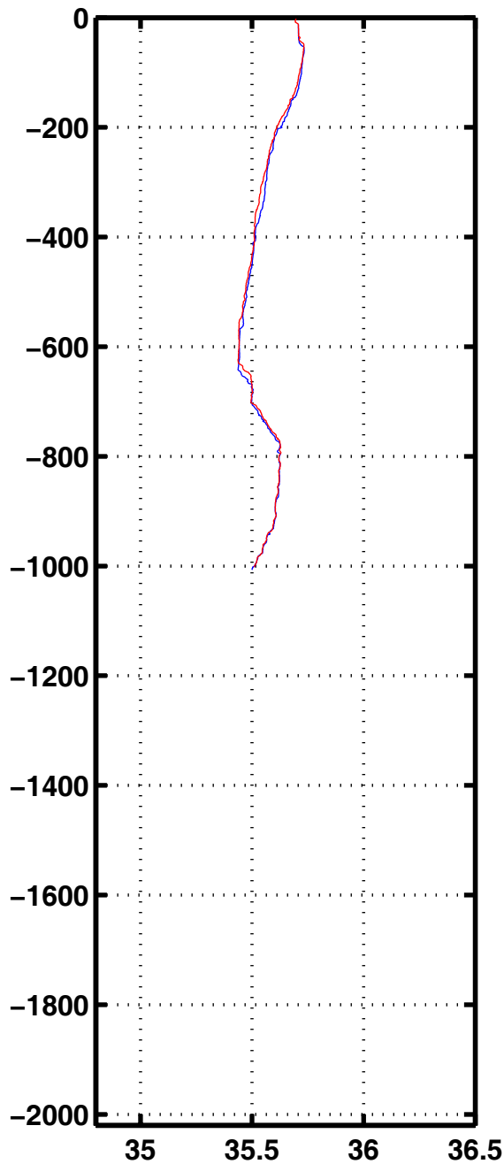
Sali 1142
