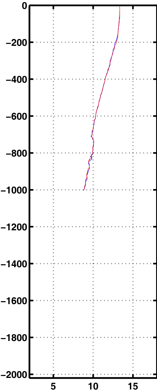
Tempe 1120
