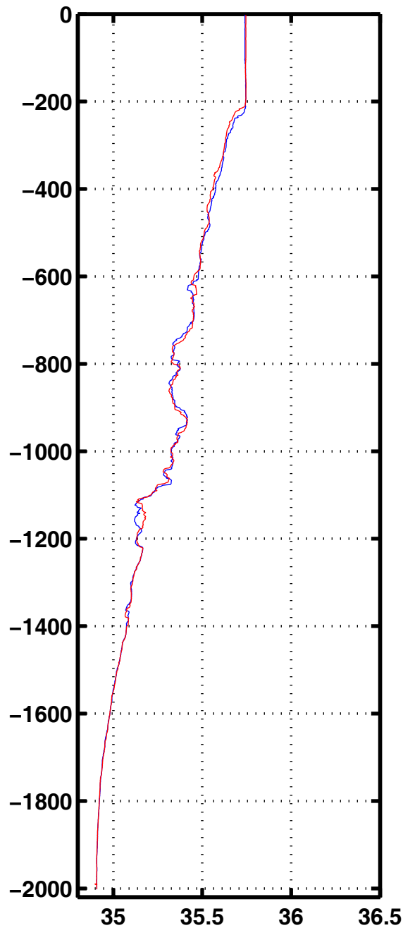
Sali 1018
