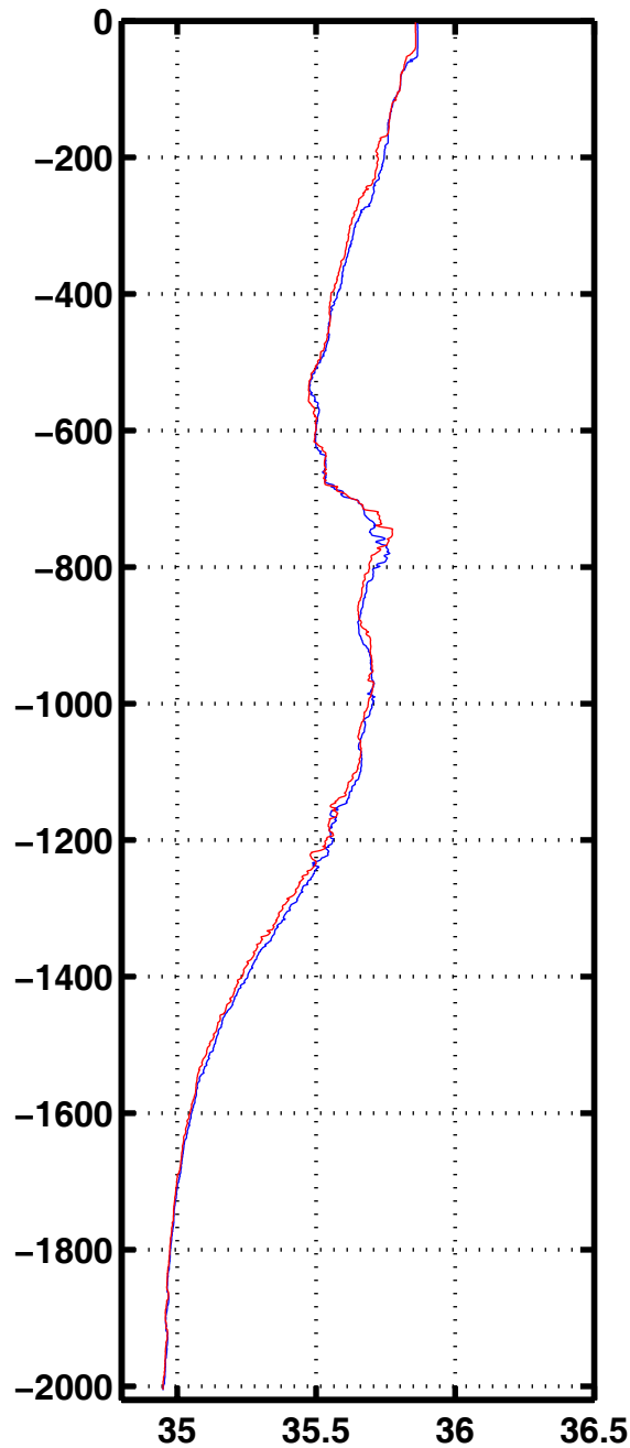
Sali 1026
