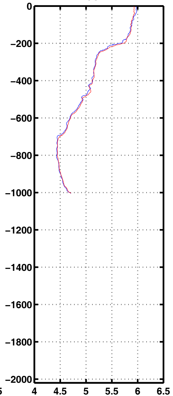
Oxyg 1155
