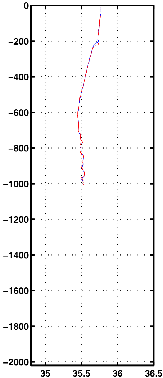
Sali 1154
