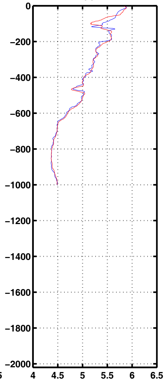
Oxyg 1104
