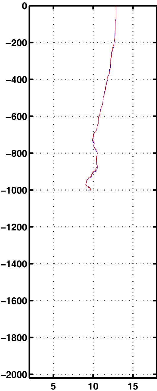
Tempe 1158
