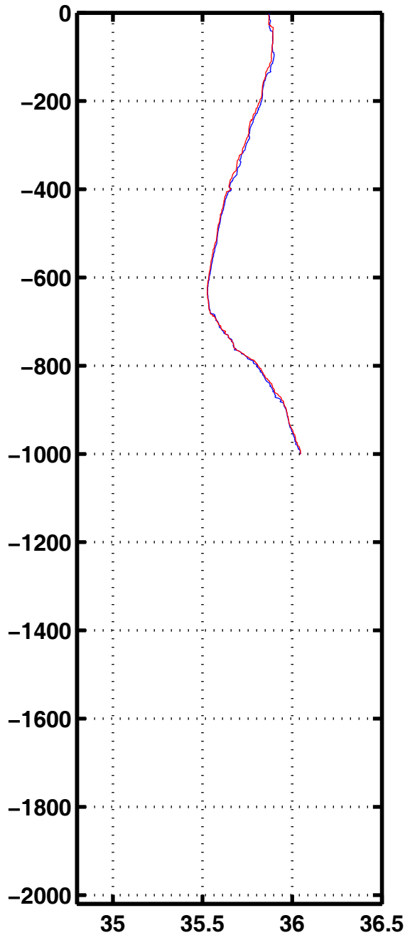
Sali 1098
