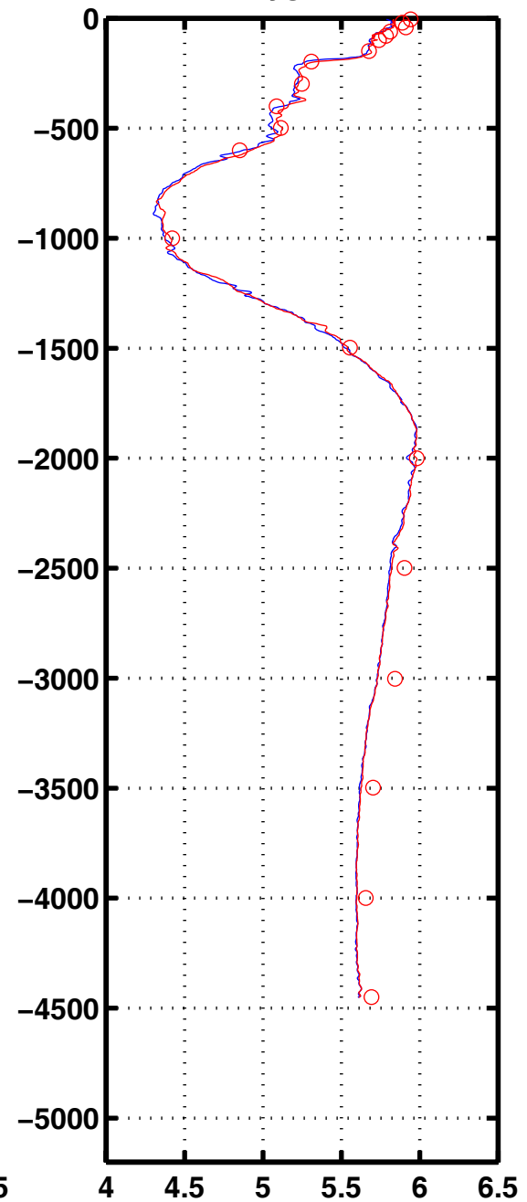
Oxyg 1032
