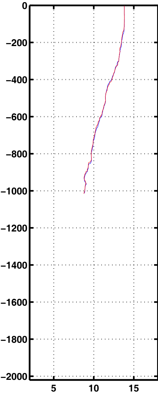
Tempe 1126
