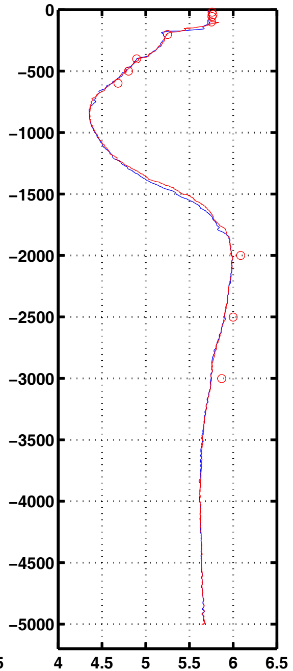
Oxyg 1003
