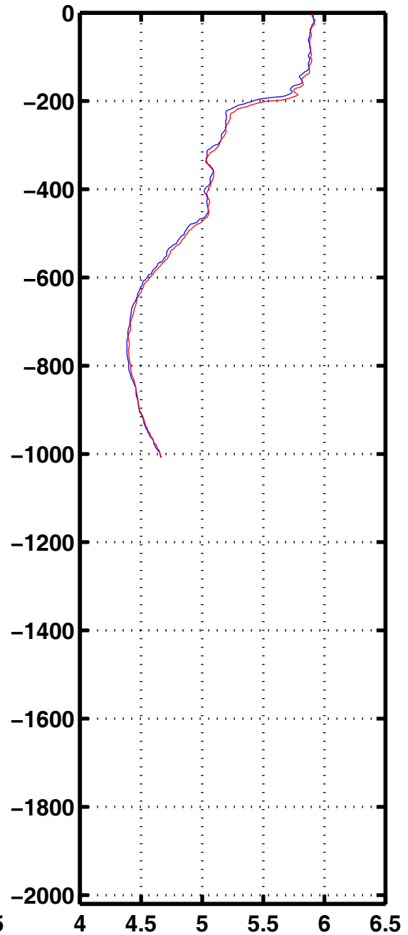
Oxyg 1107
