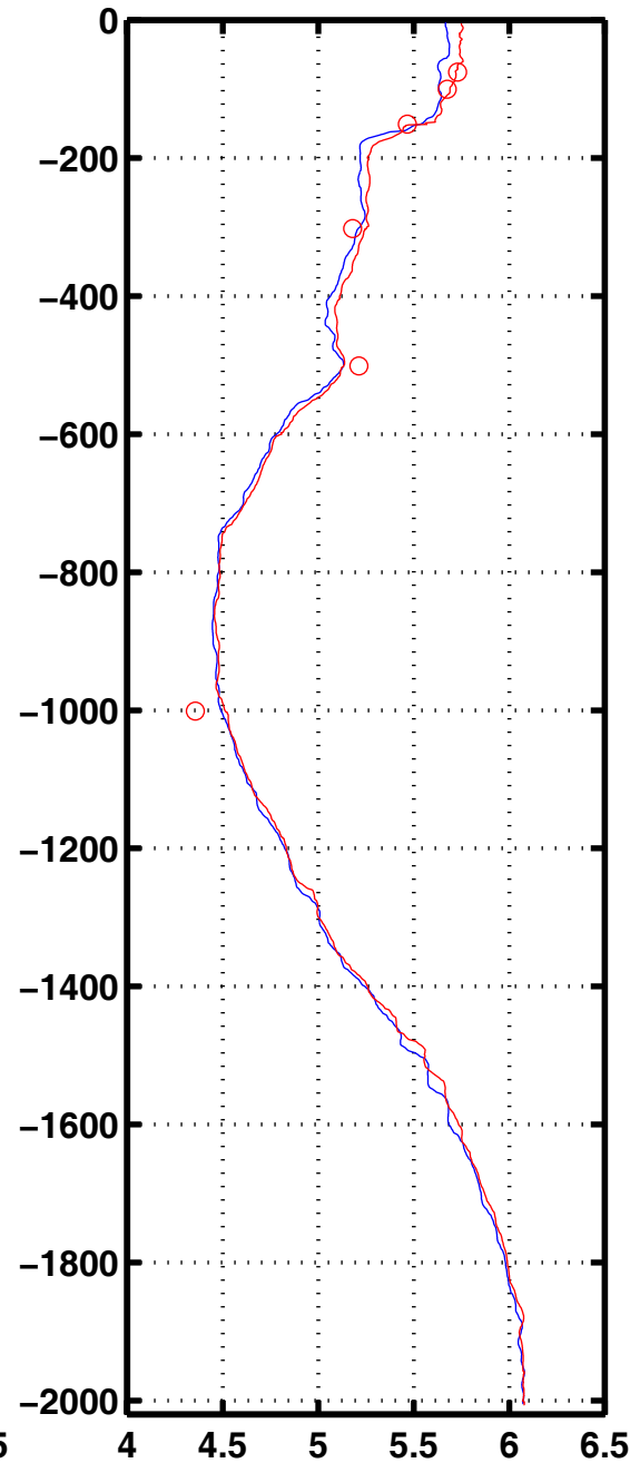
Oxyg 1001
