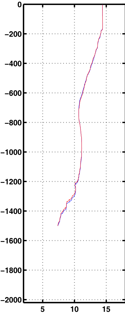
Tempe 1083
