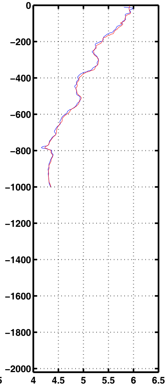
Oxyg 1200
