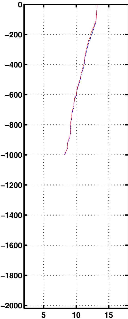
Tempe 1152
