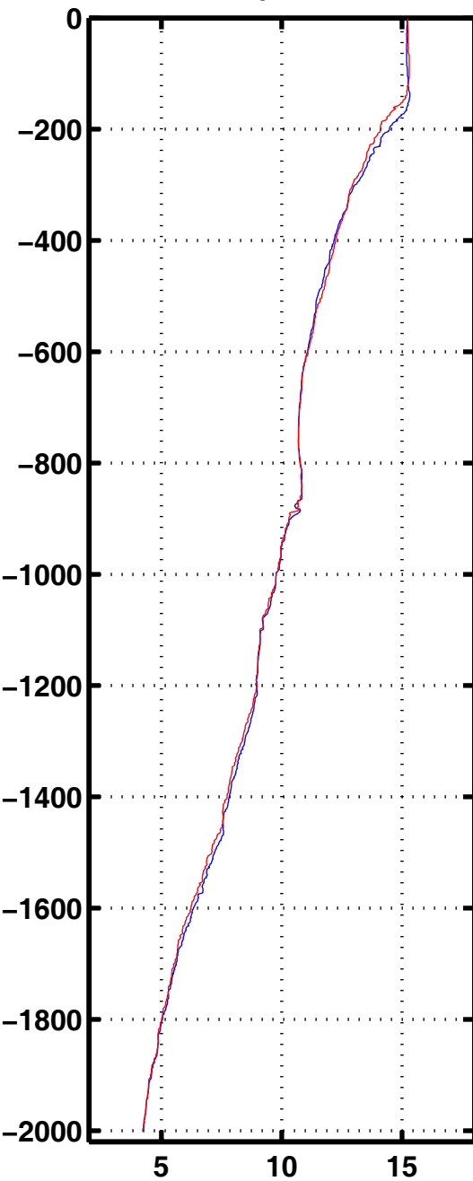
Tempe 1076
