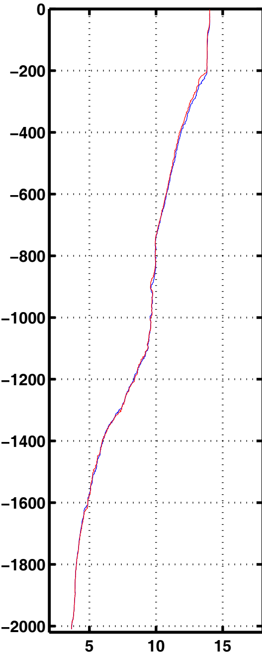
Tempe 1030
