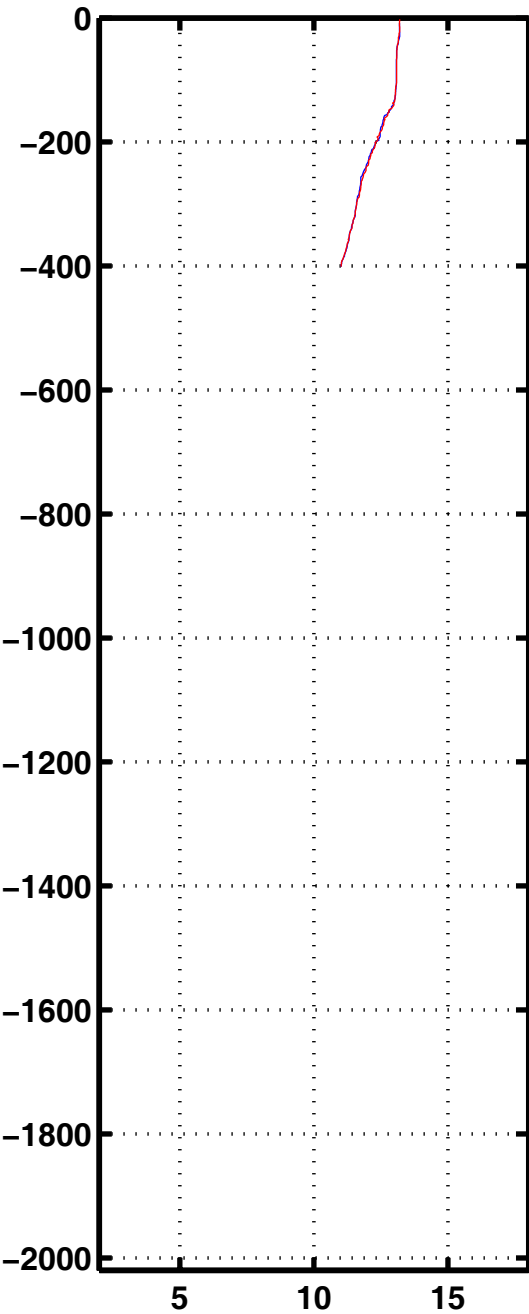
Tempe 1146
