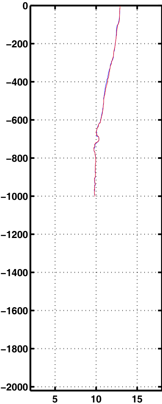
Tempe 1187
