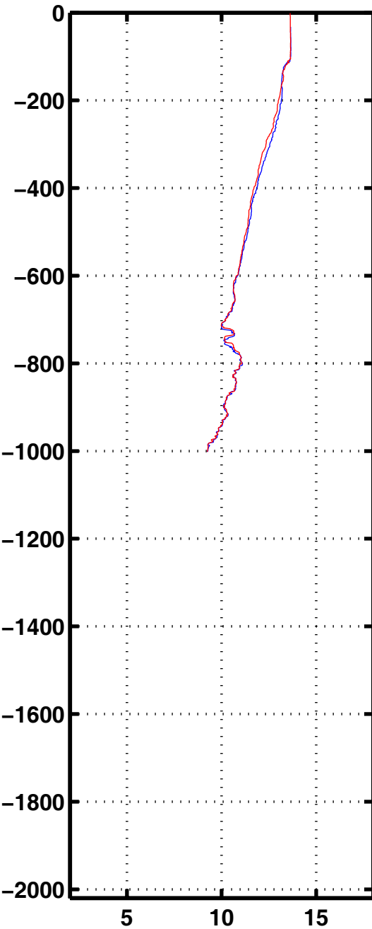
Tempe 1113
