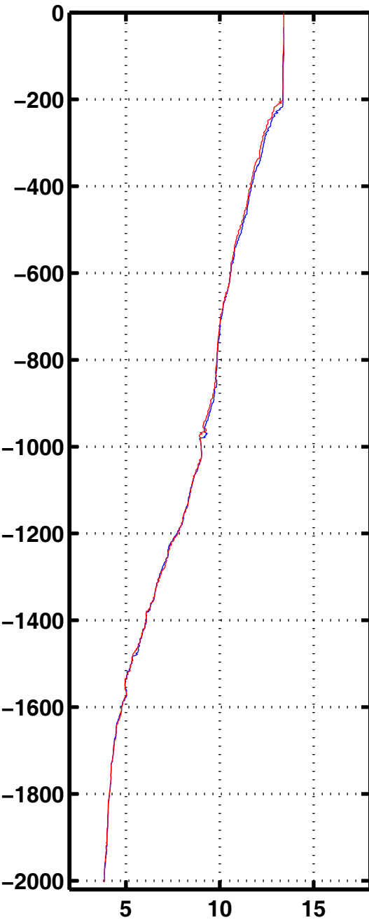
Tempe 1025
