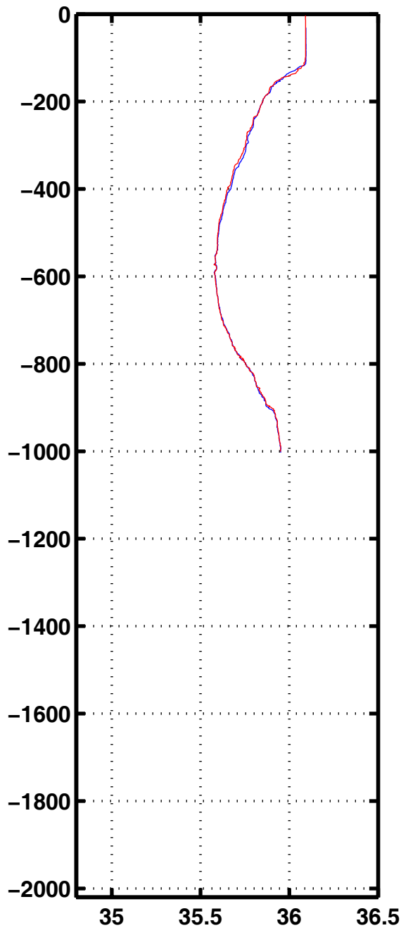
Sali 1123
