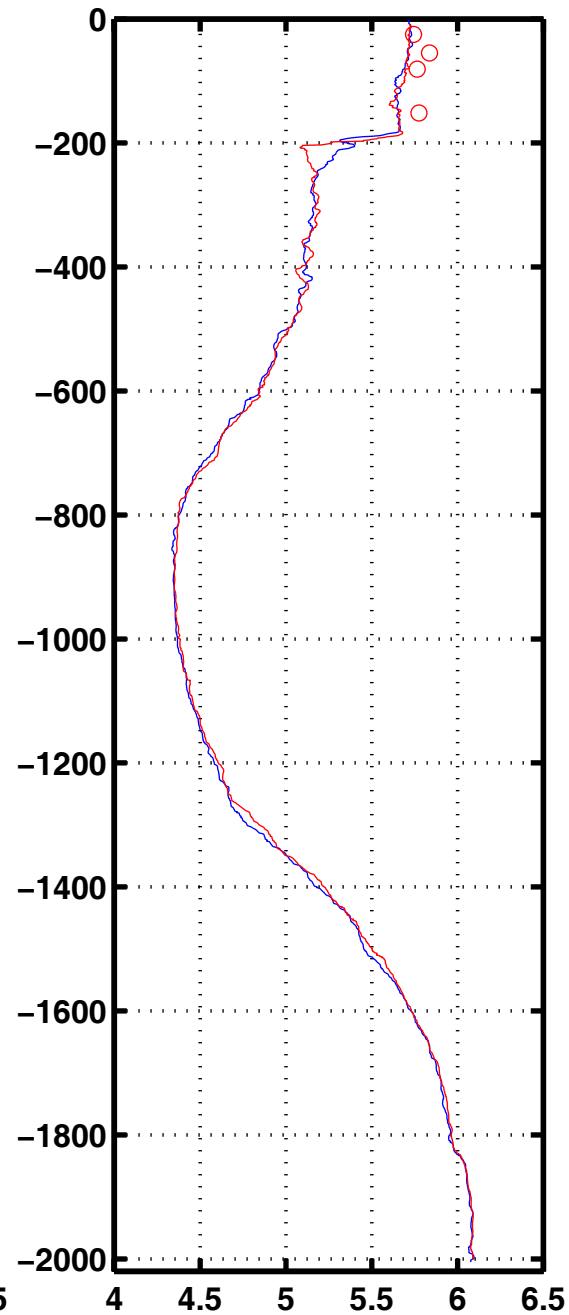
Oxyg 1005
