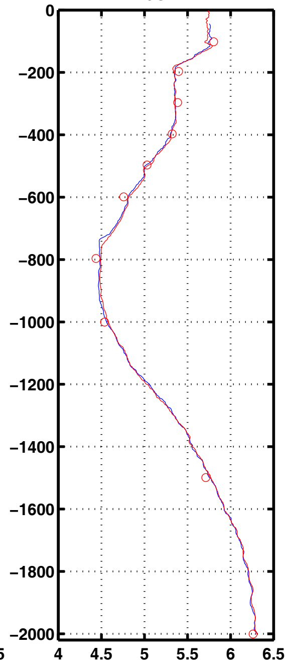
Oxyg 1013
