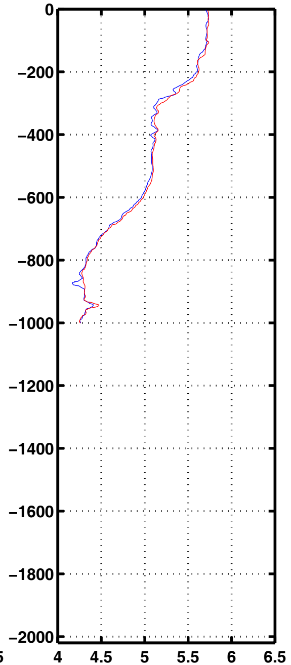
Oxyg 1098
