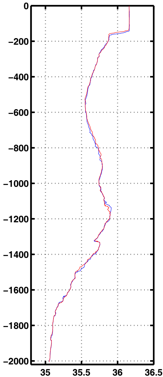
Sali 1078
