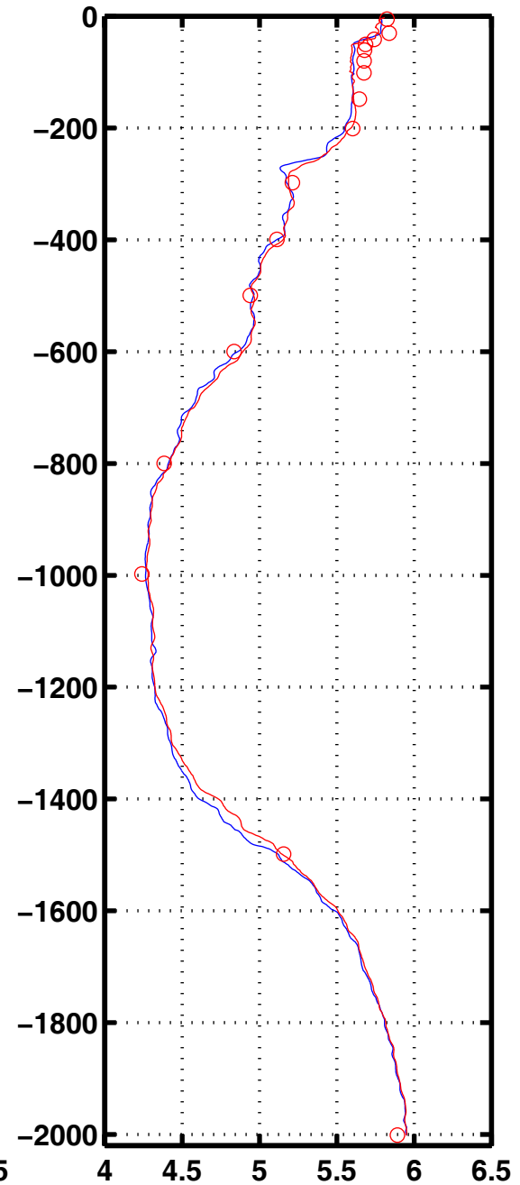
Oxyg 1059
