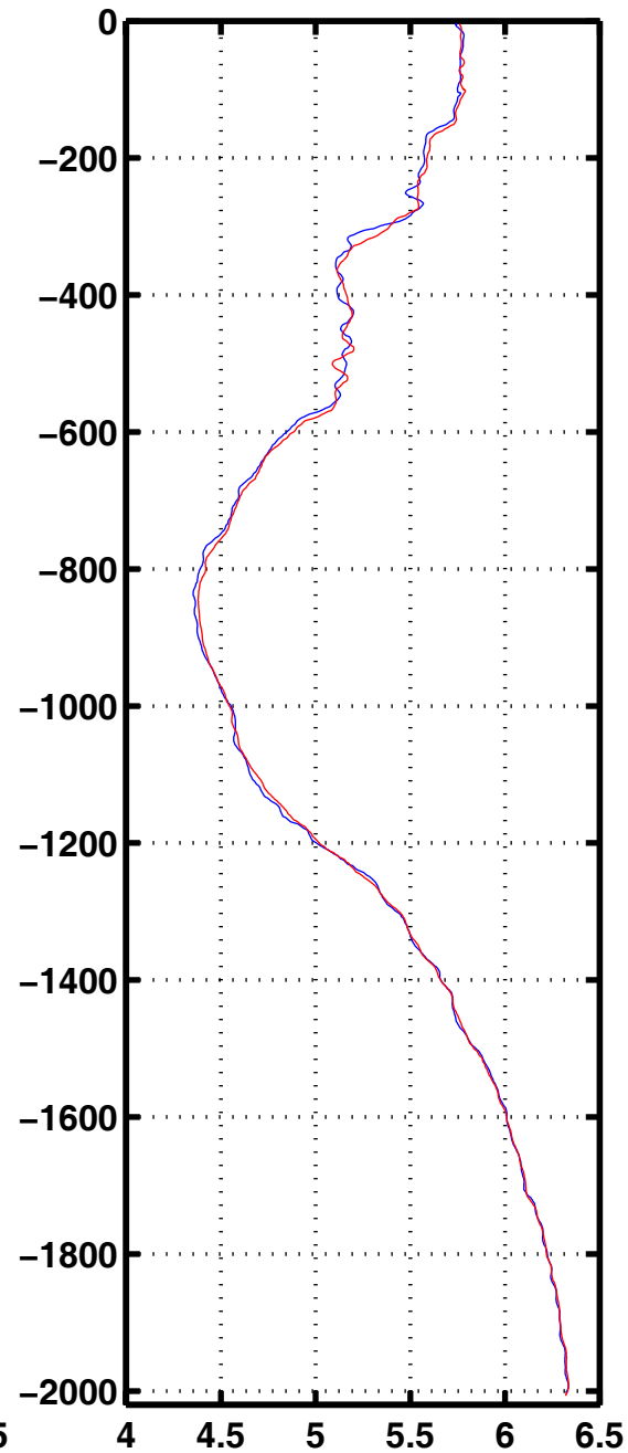
Oxyg 1066
