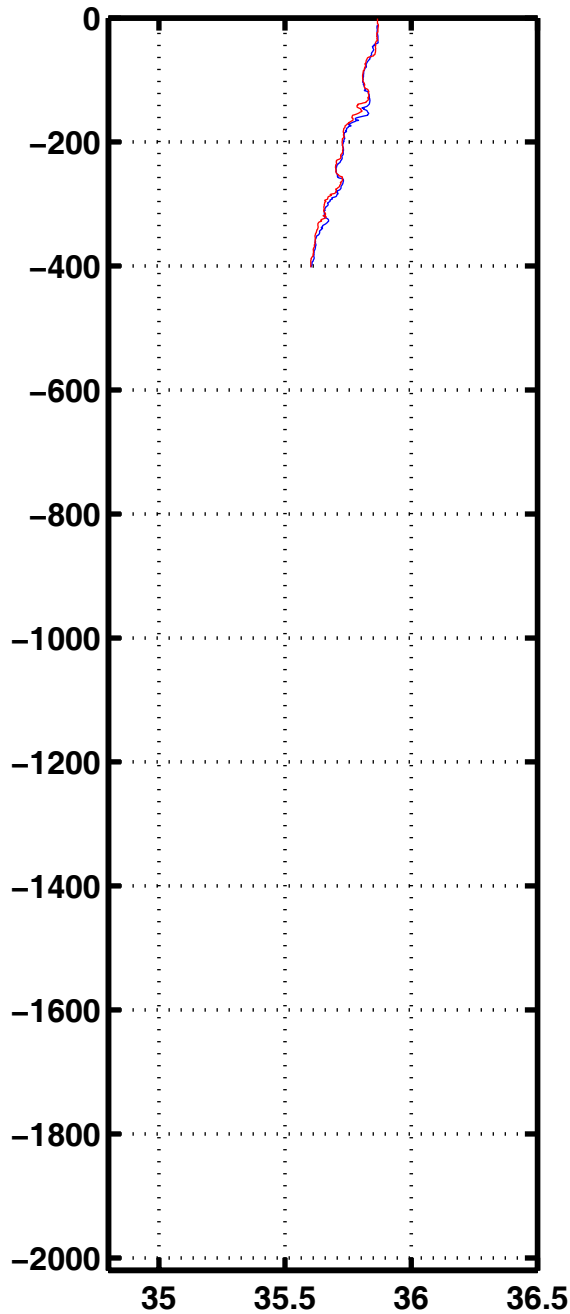
Sali 1117
