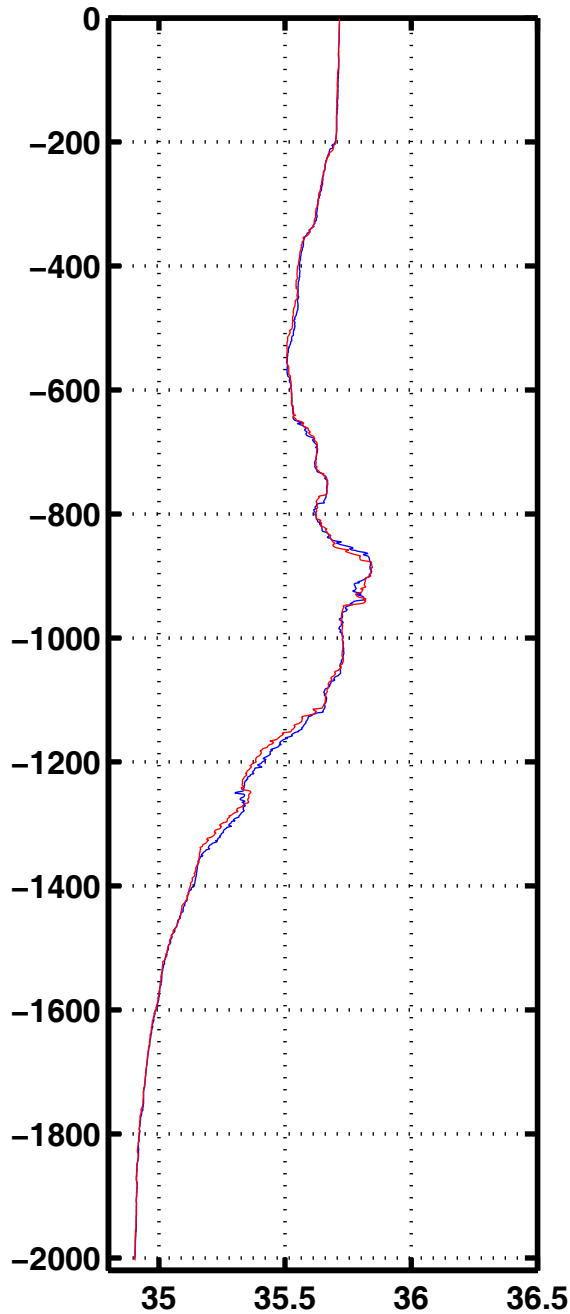
Sali 1015
