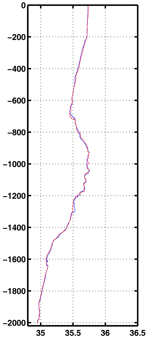
Sali 1021
