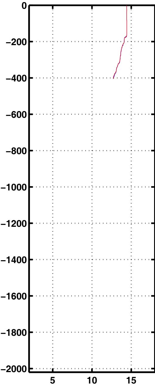
Tempe 1090
