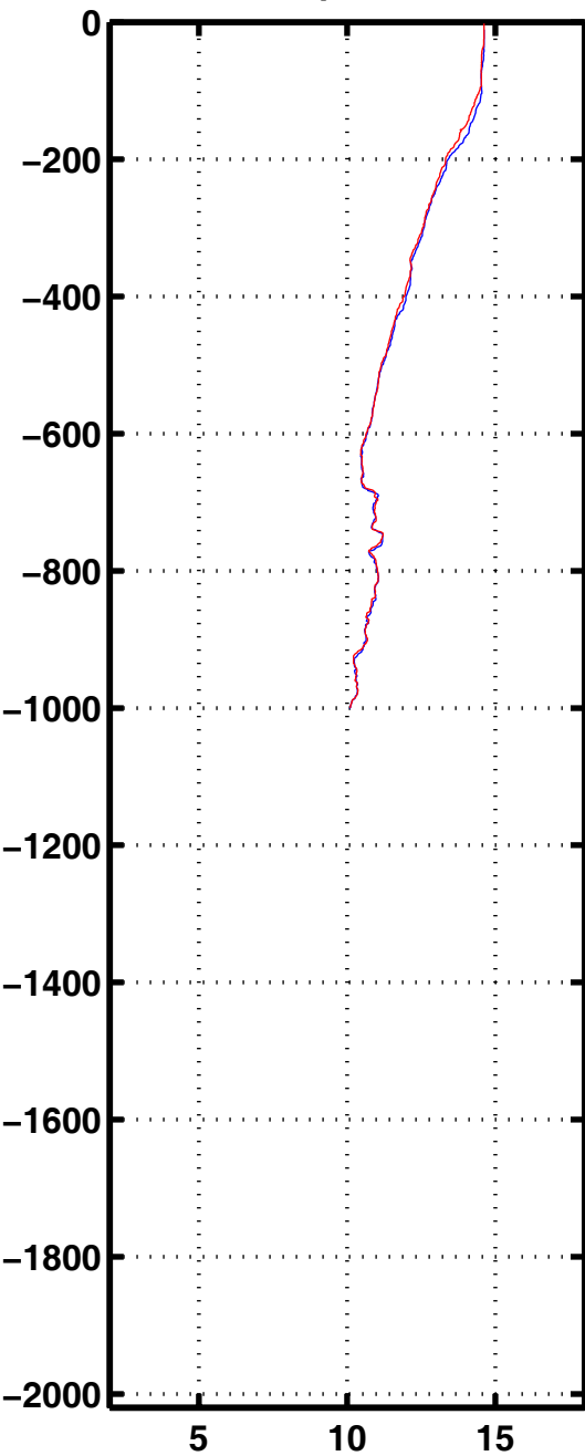
Tempe 1206
