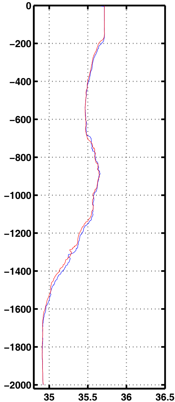
Sali 1063
