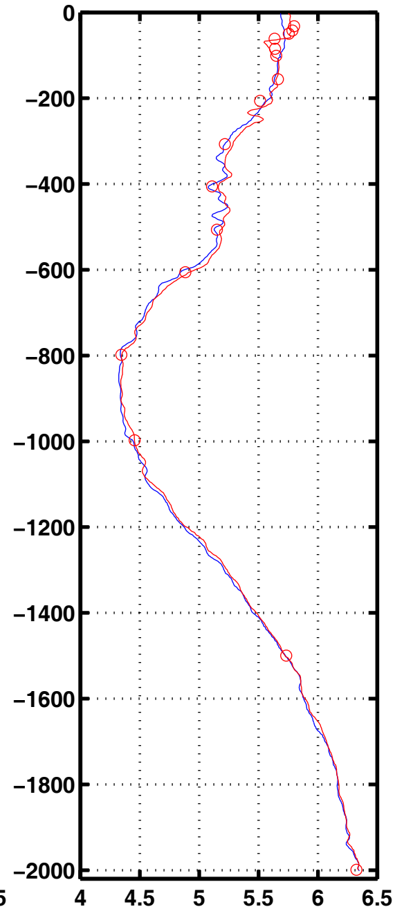
Oxyg 1069
