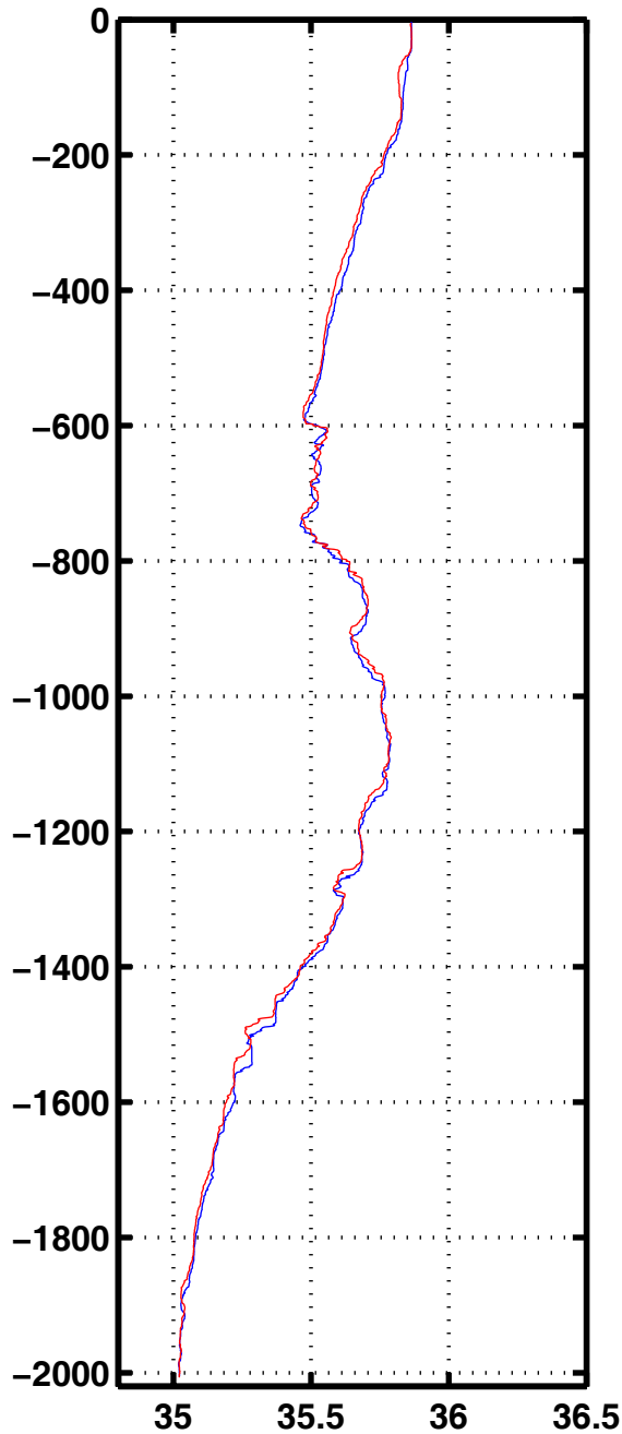
Sali 1001
