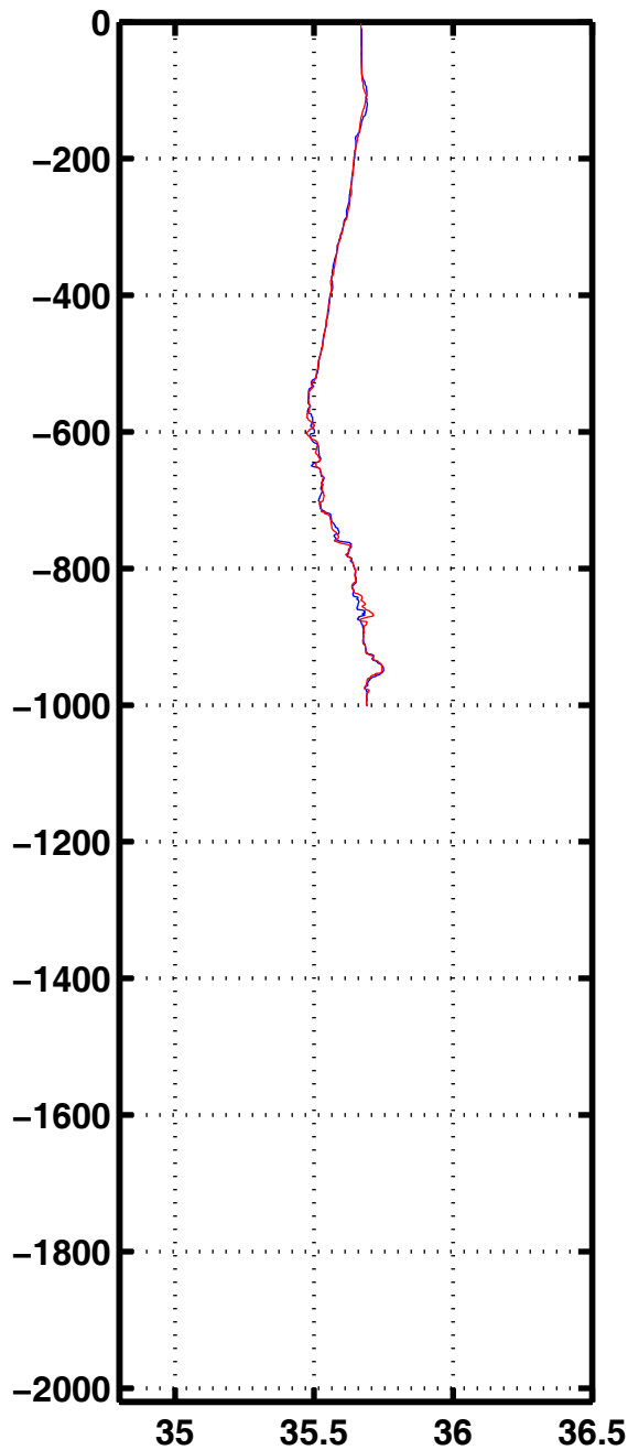
Sali 1193
