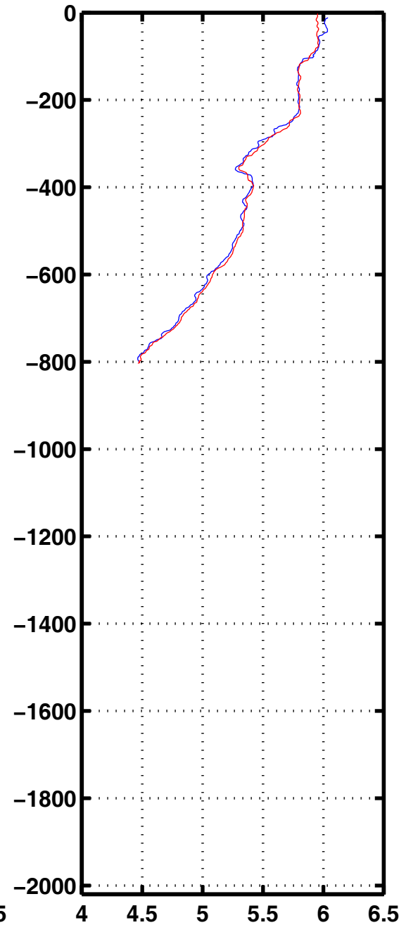
Oxyg 1174
