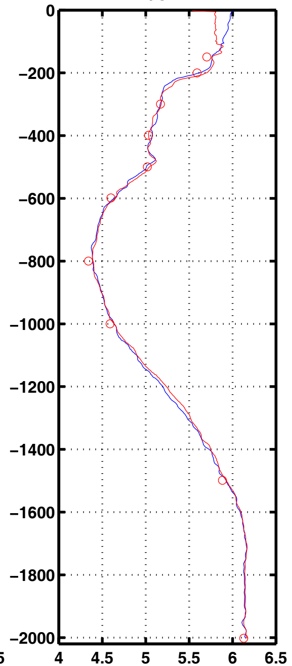
Oxyg 1068
