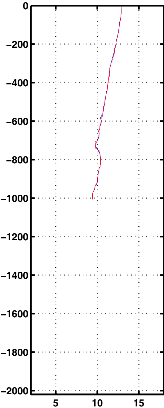
Tempe 1190
