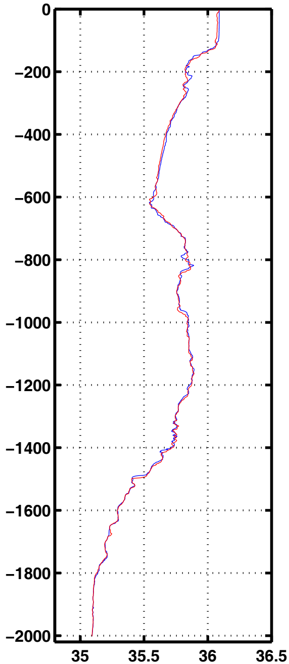
Sali 1057
