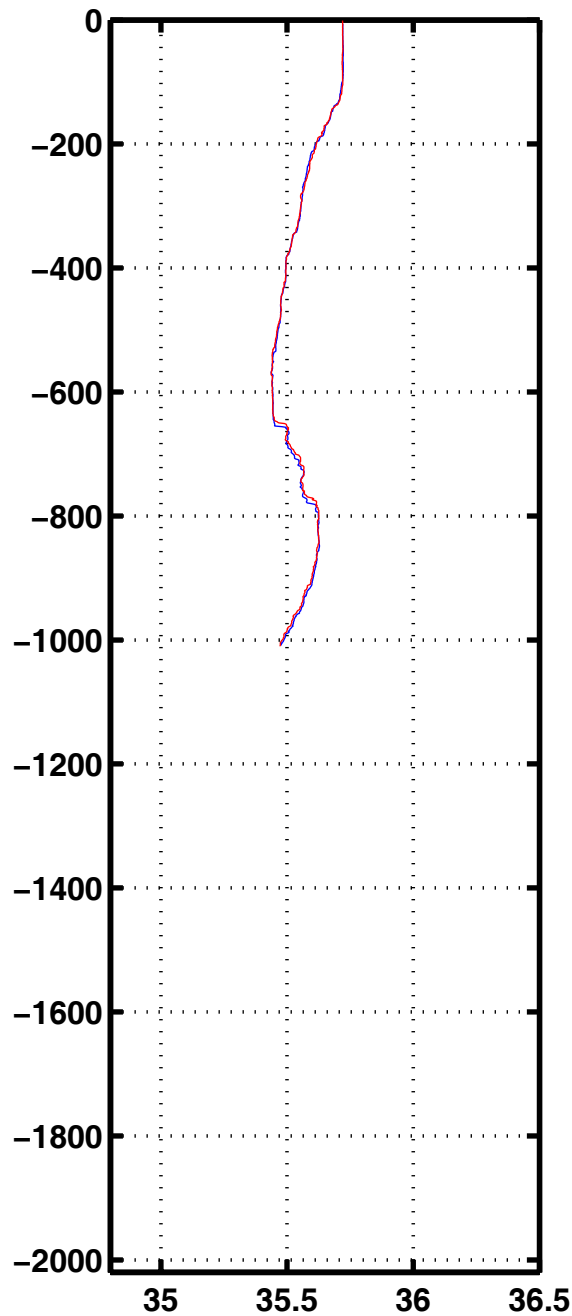
Sali 1135
