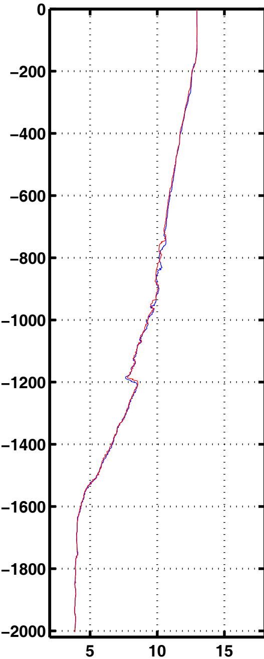
Tempe 1024
