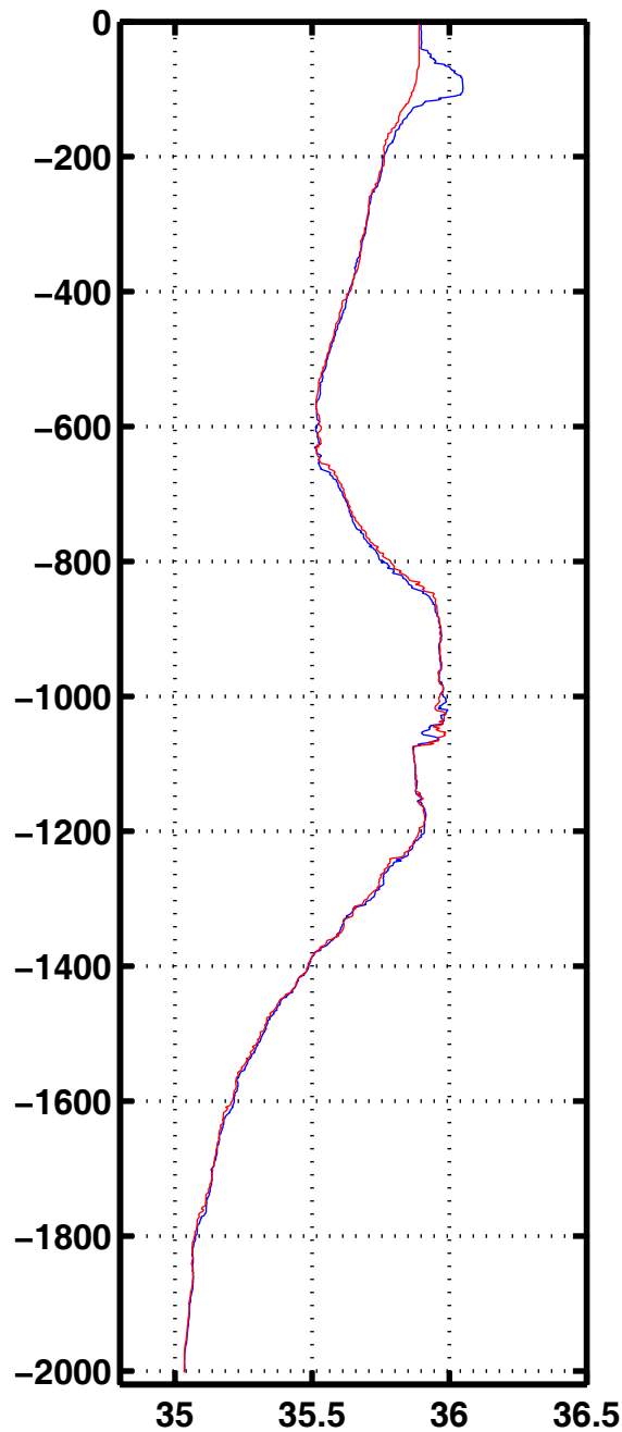
Sali 1075
