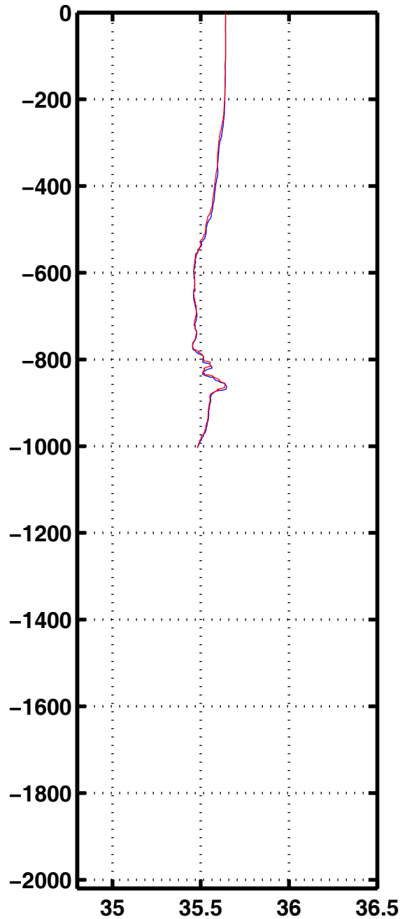
Sali 1165
