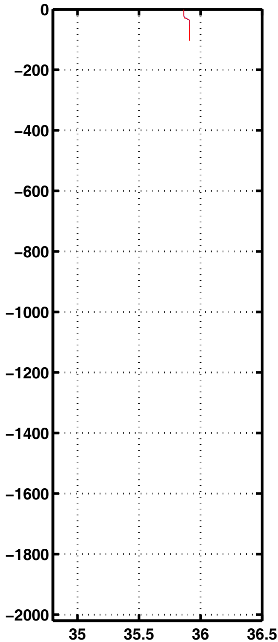
Sali 1088
