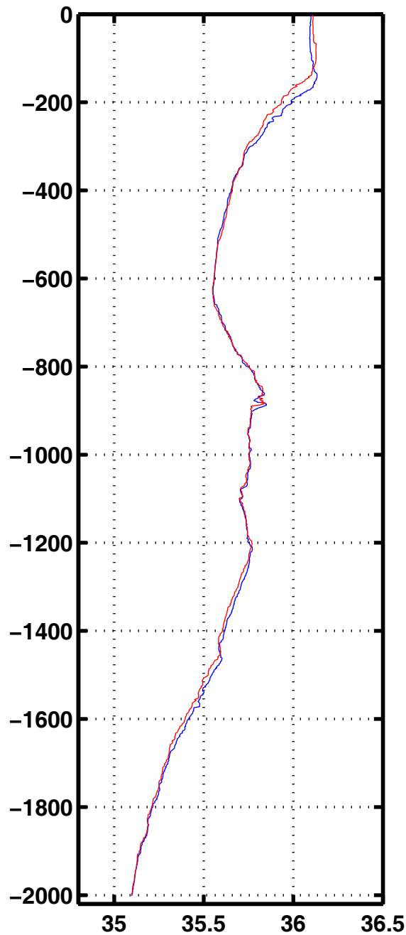
Sali 1076
