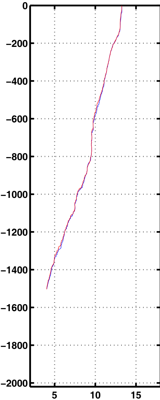
Tempe 1138
