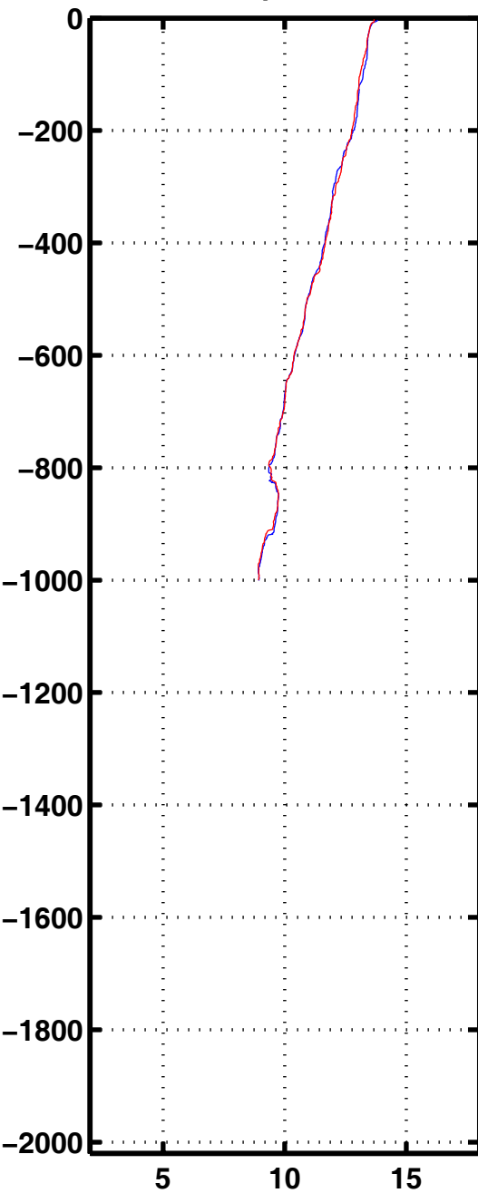
Tempe 1104
