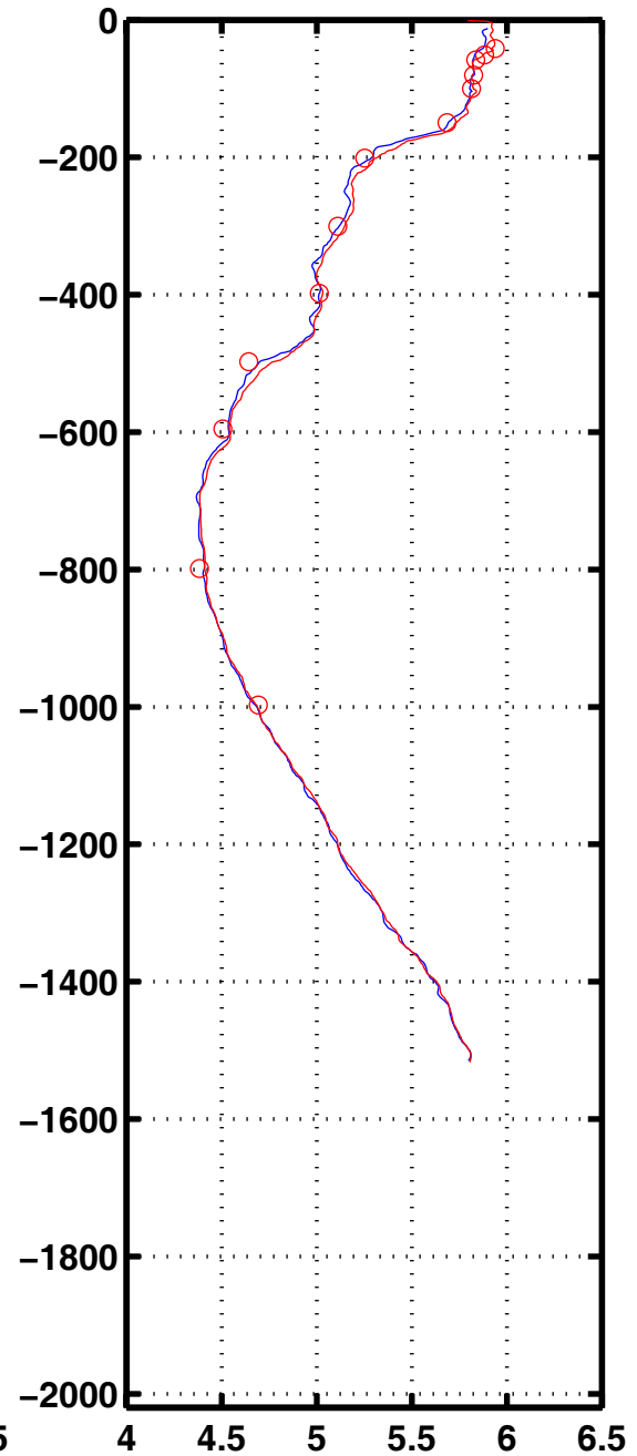
Oxyg 1148
