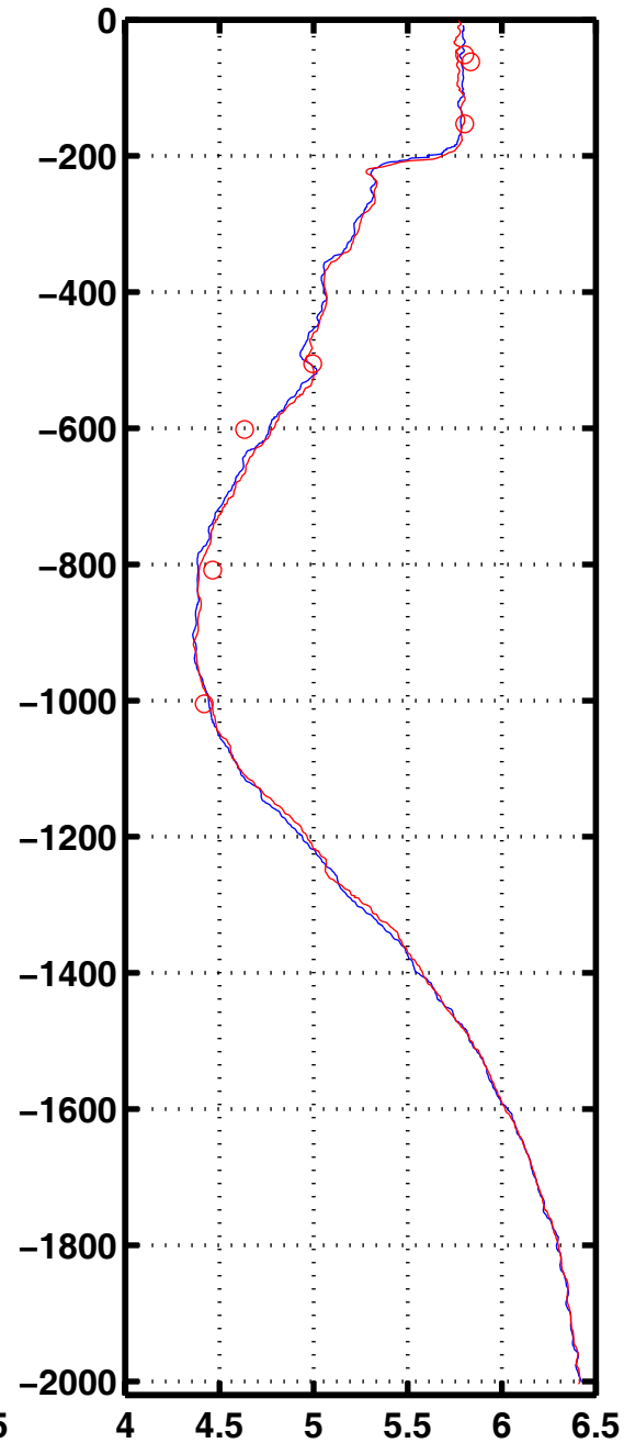
Oxyg 1015
