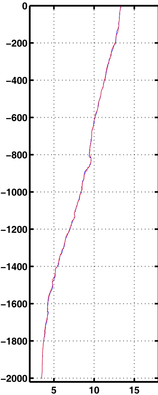
Tempe 1049
