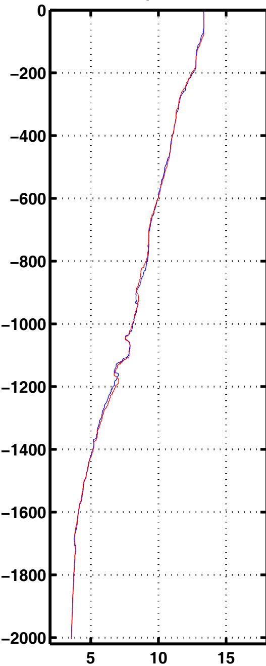
Tempe 1062
