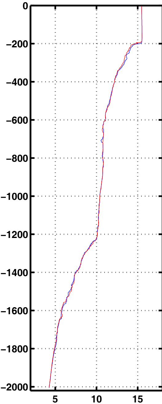
Tempe 1080
