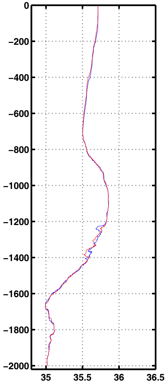
Sali 1023
