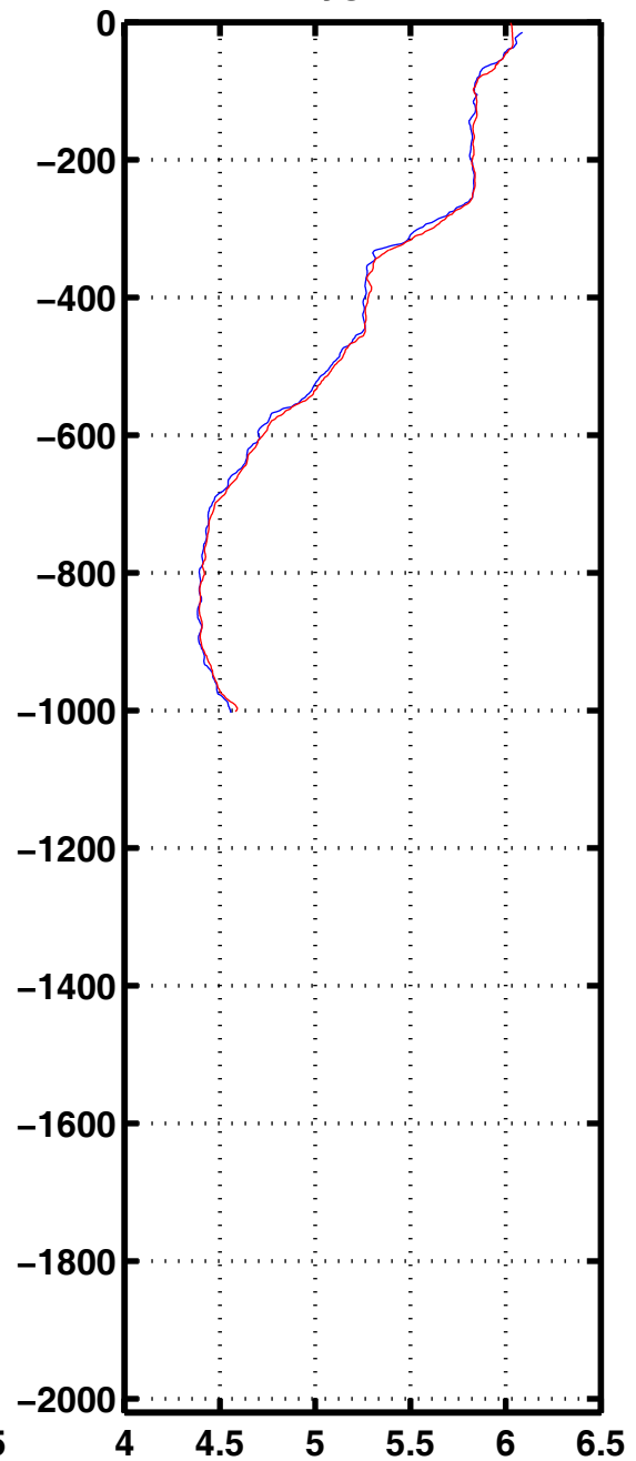
Oxyg 1189
