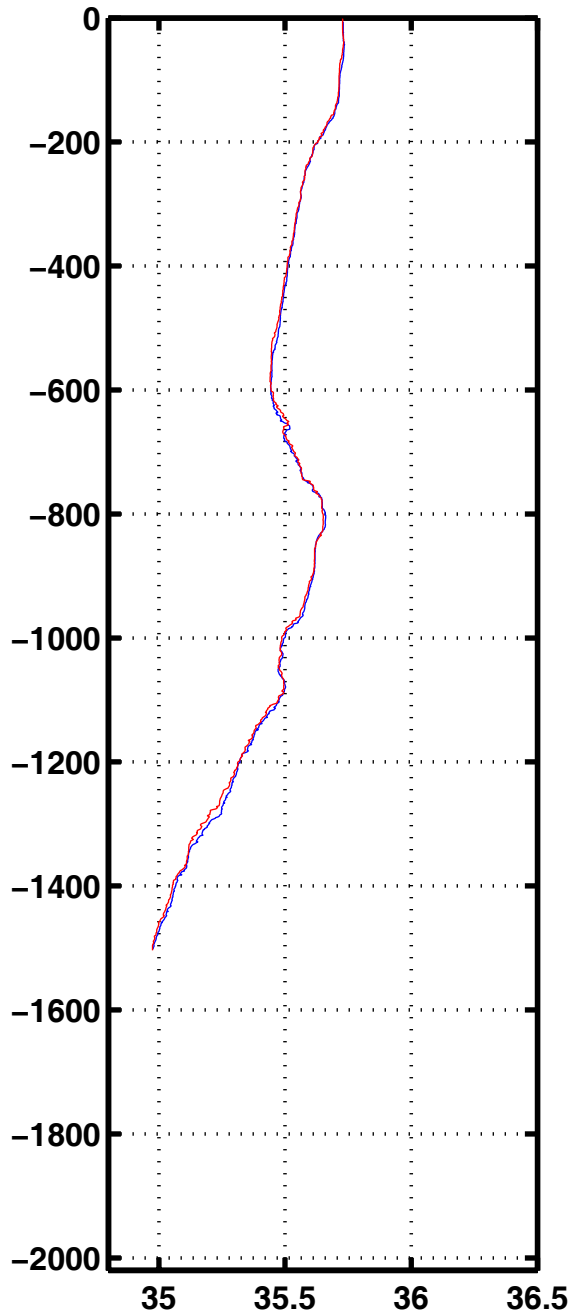
Sali 1138
