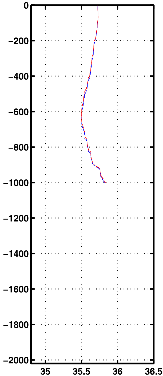
Sali 1163
