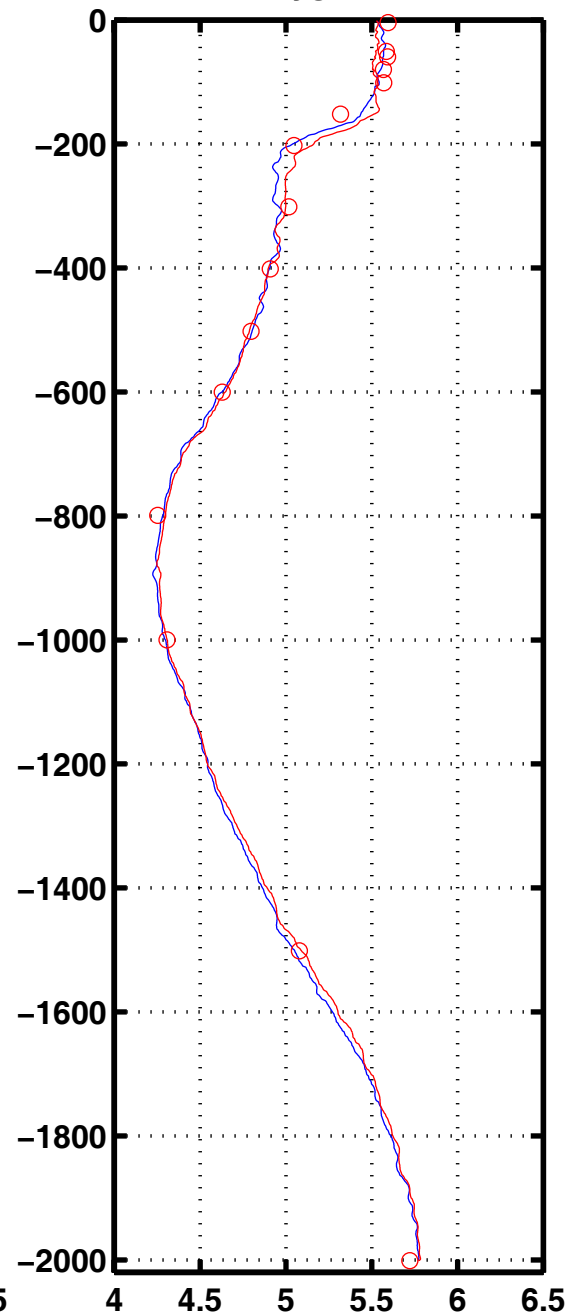
Oxyg 1076
