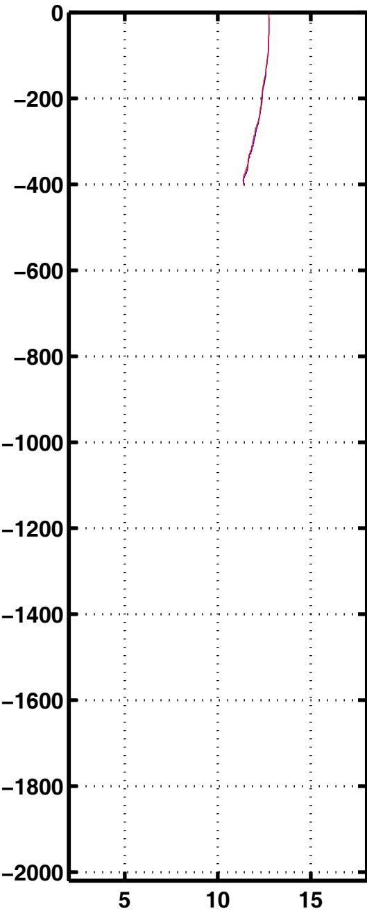
Tempe 1184
