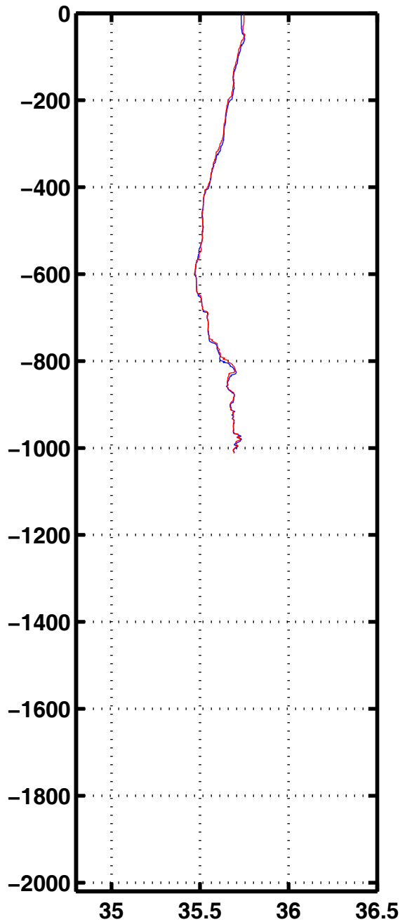
Sali 1191
