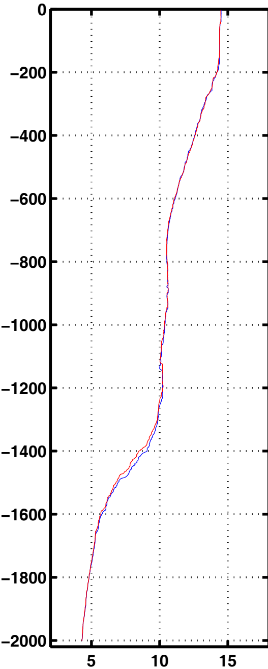
Tempe 1059
