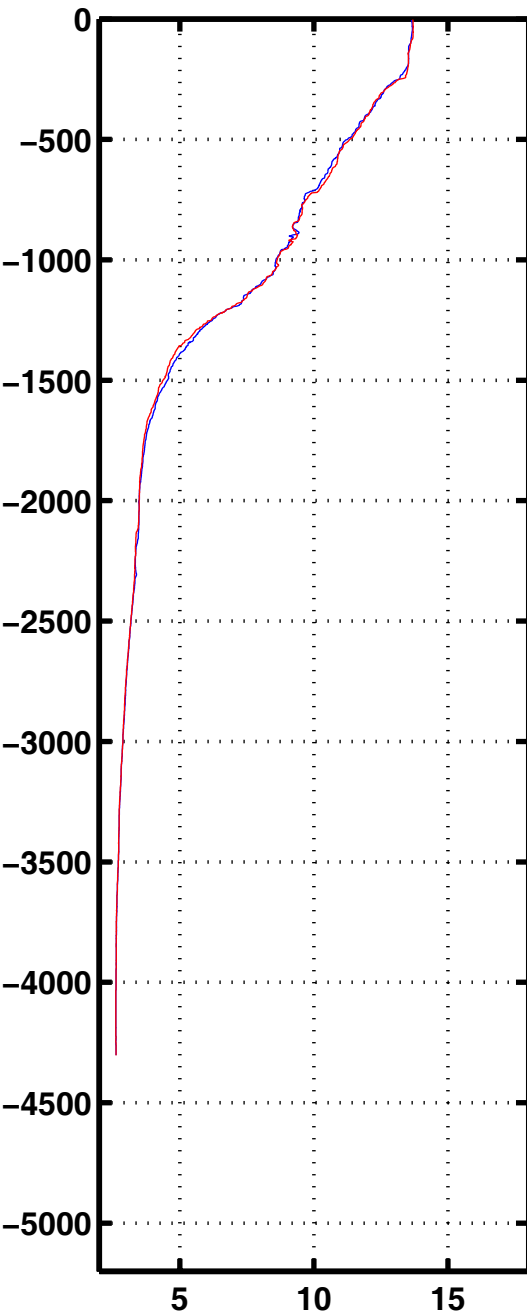
Tempe 1045
