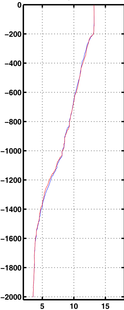
Tempe 1068
