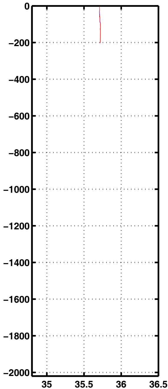
Sali 1180
