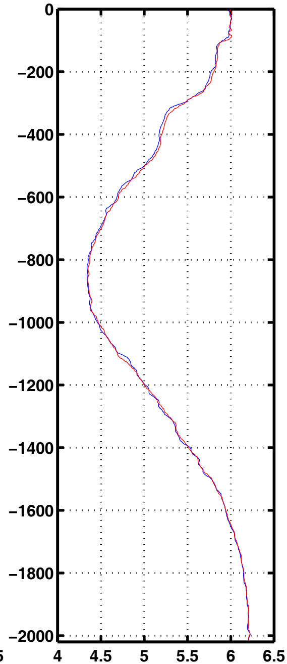
Oxyg 1182
