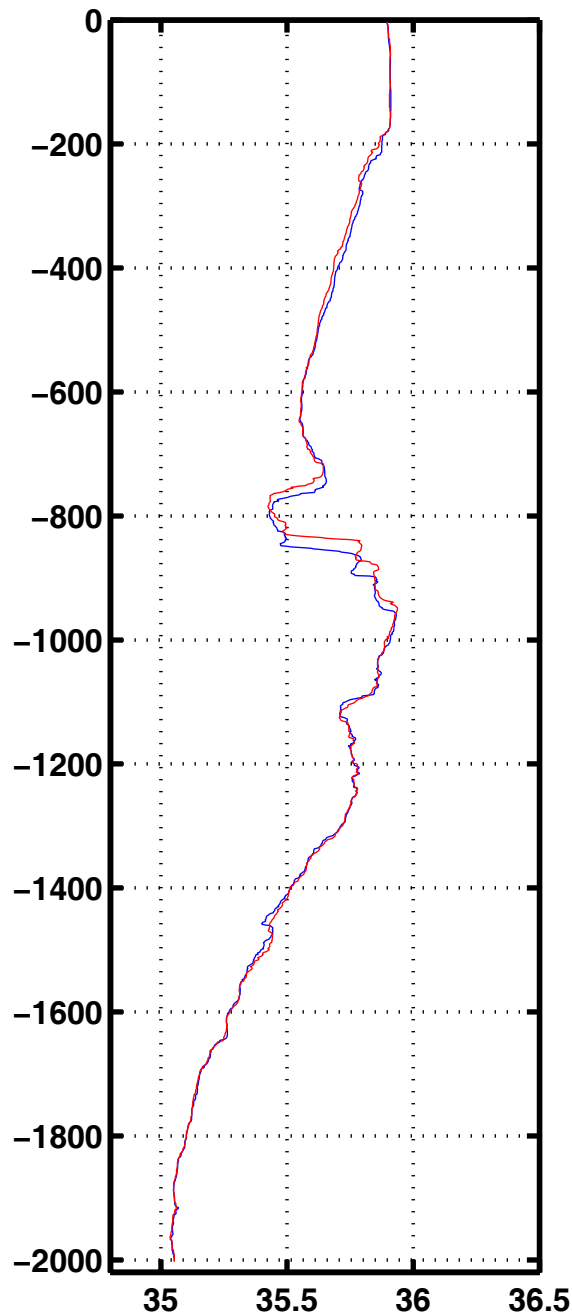
Sali 1035
