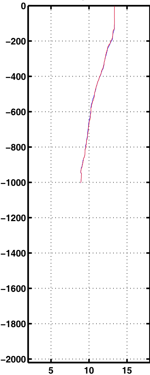
Tempe 1130
