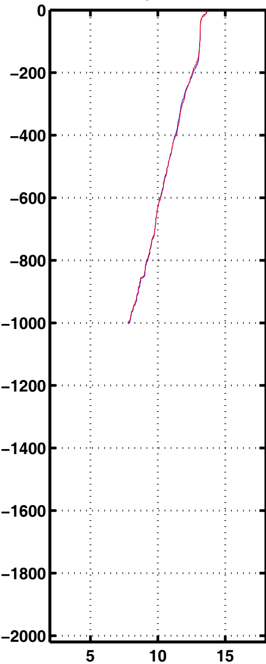
Tempe 1105
