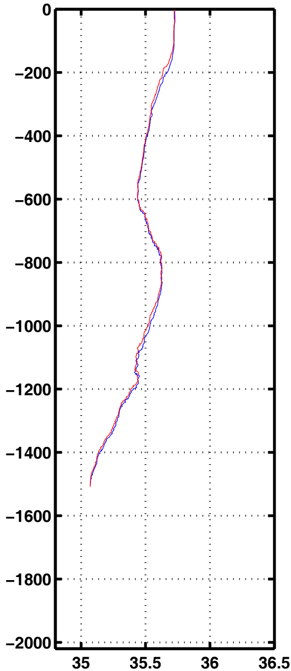
Sali 1140
