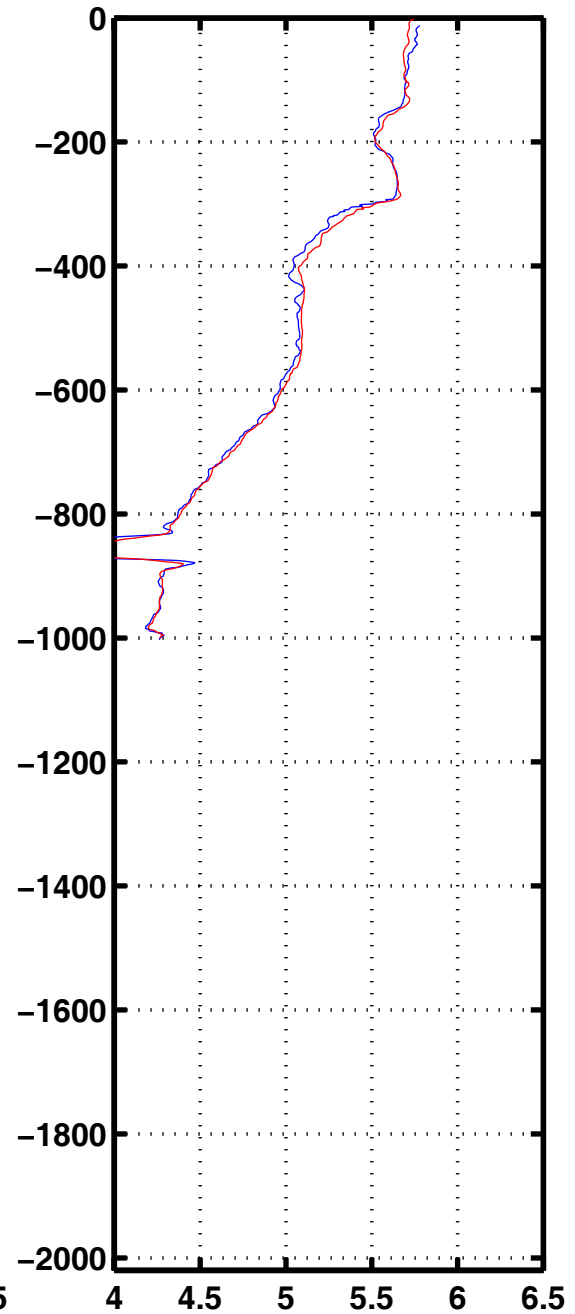
Oxyg 1099
