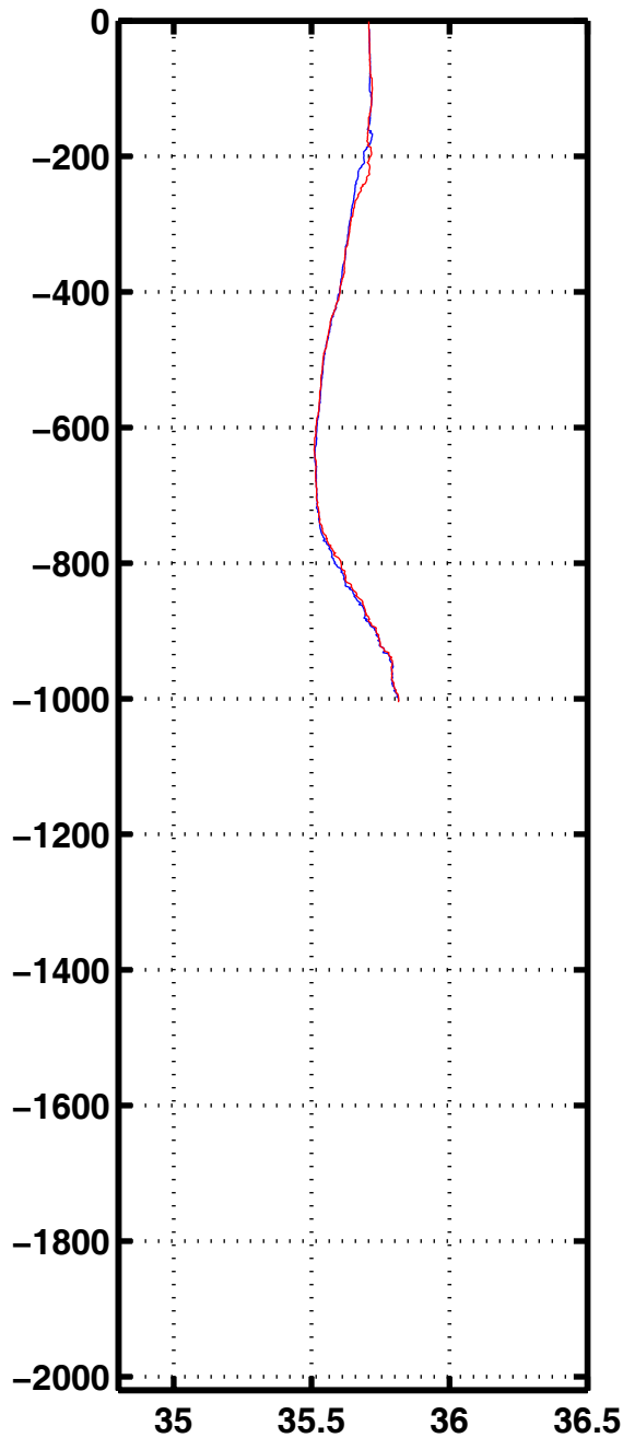
Sali 1169
