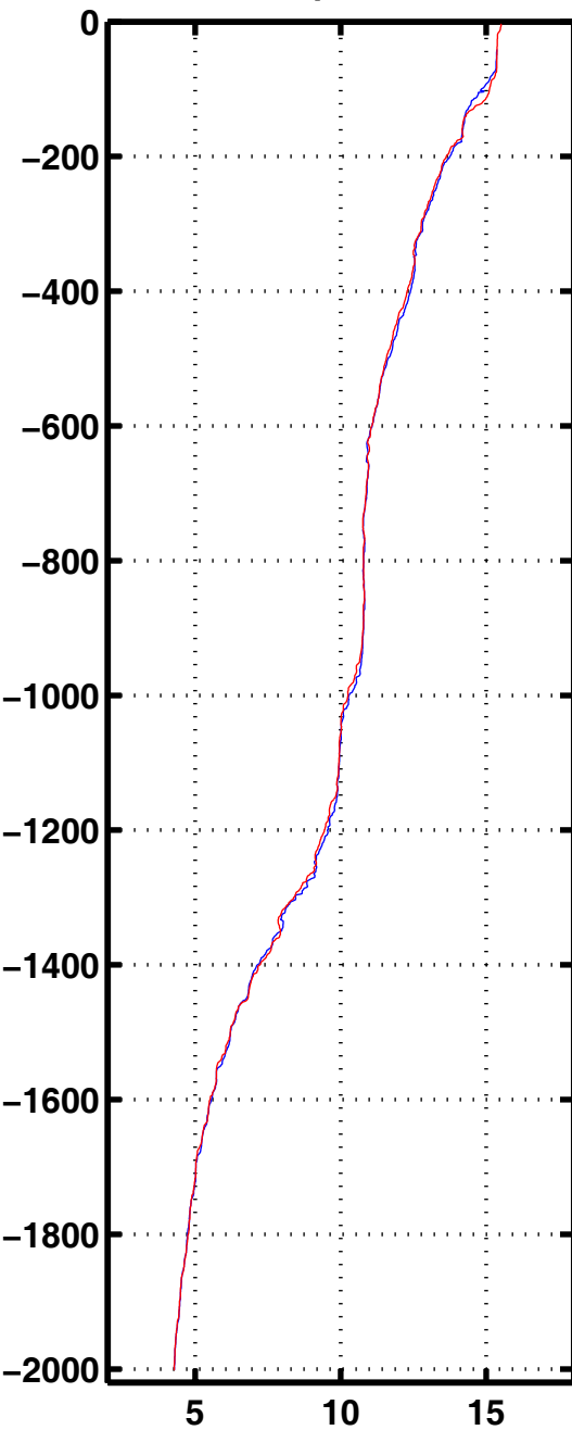
Tempe 1056
