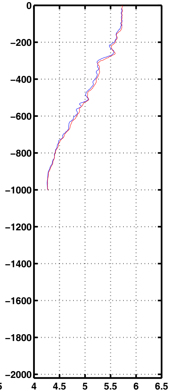
Oxyg 1100
