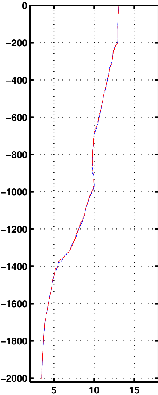
Tempe 1020
