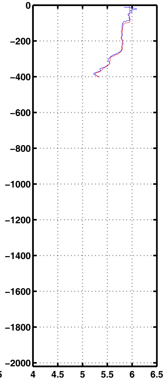
Oxyg 1175
