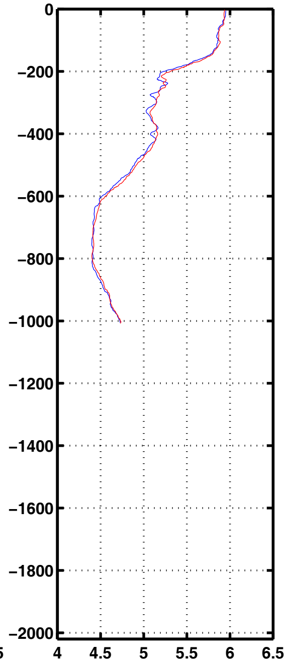
Oxyg 1134
