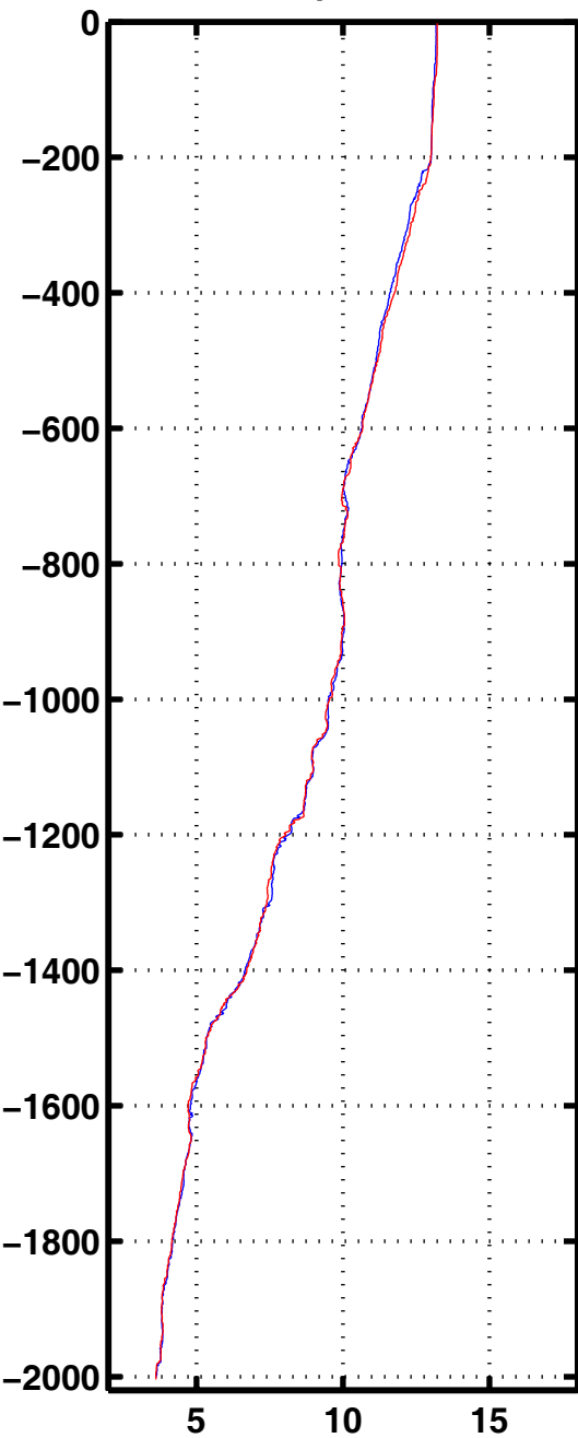
Tempe 1021
