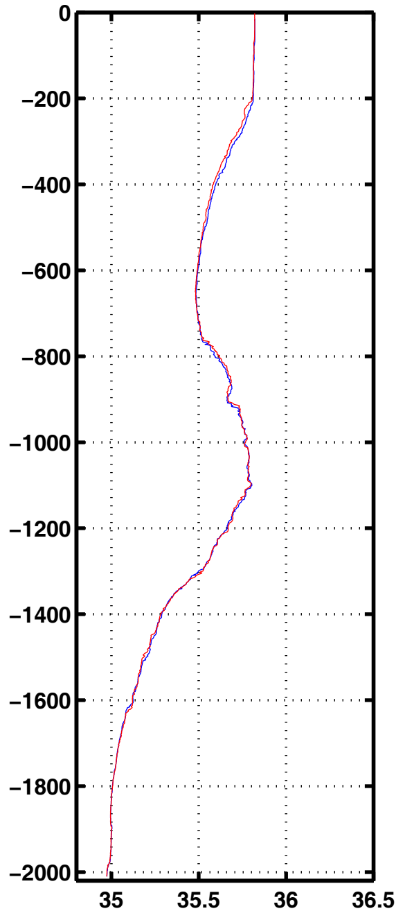
Sali 1030
