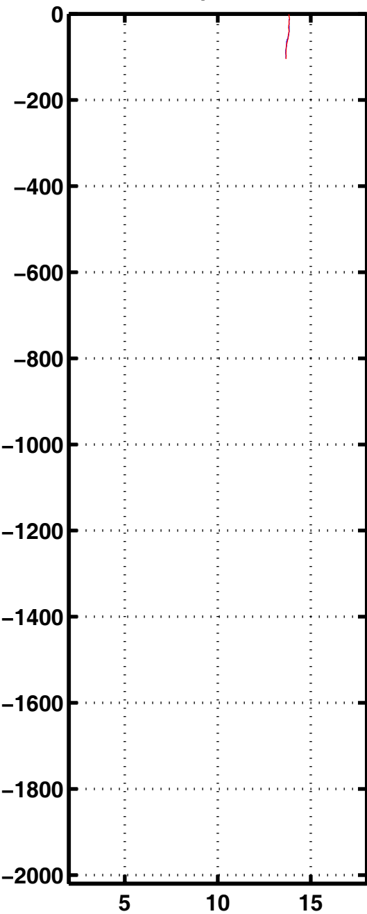
Tempe 1116
