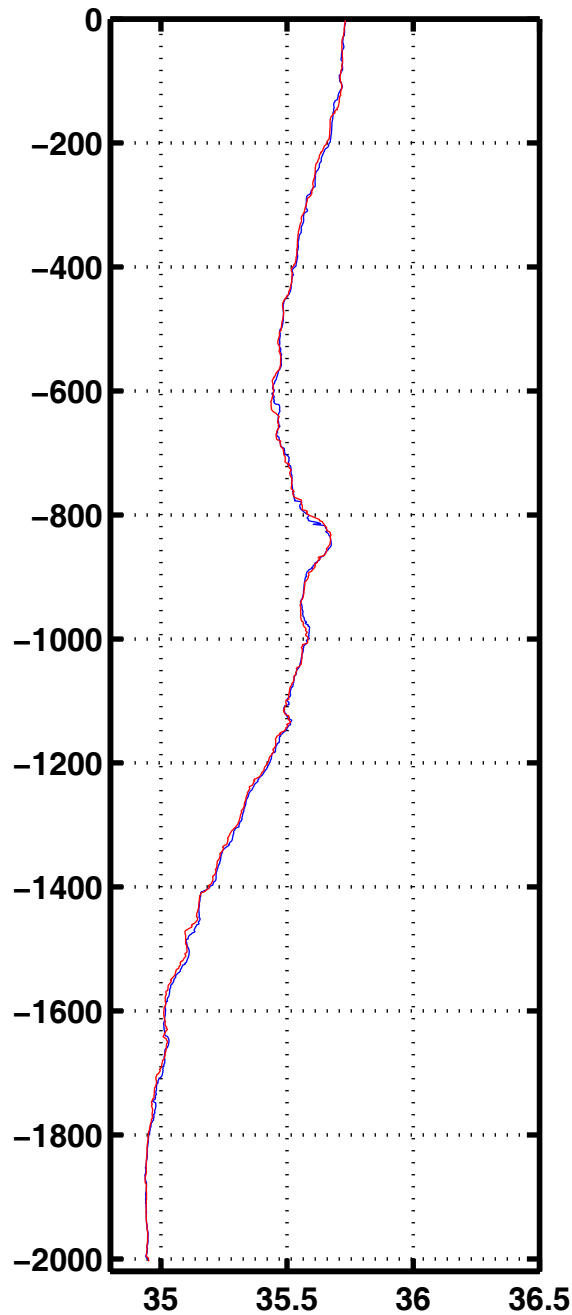
Sali 1049
