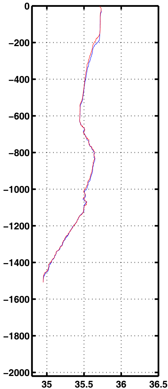
Sali 1139
