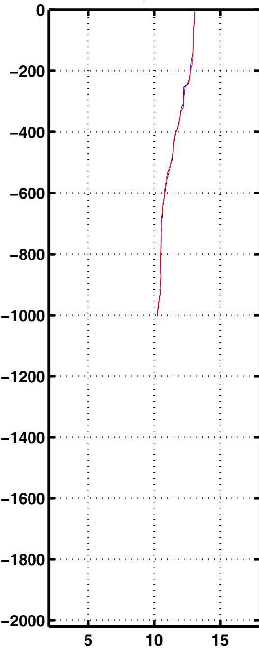
Tempe 1164
