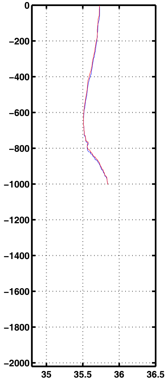
Sali 1160
