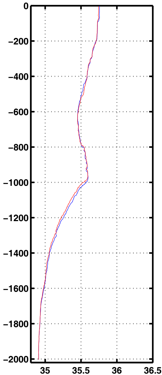
Sali 1065
