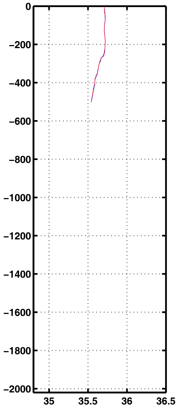
Sali 1179
