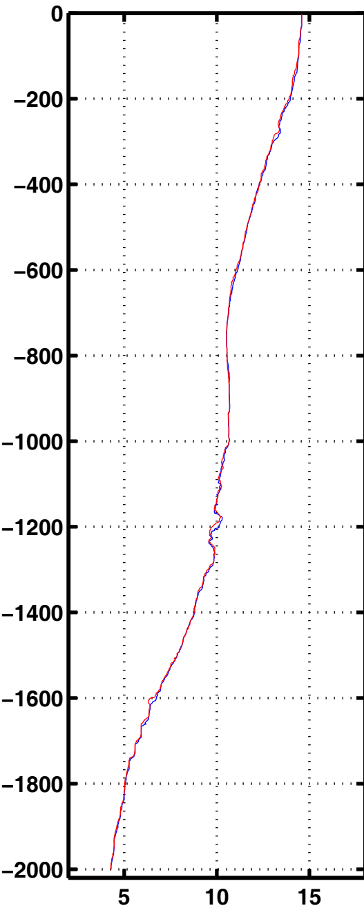
Tempe 1053
