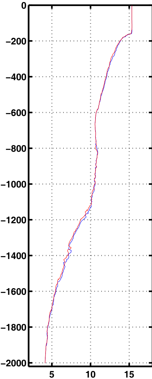
Tempe 1079
