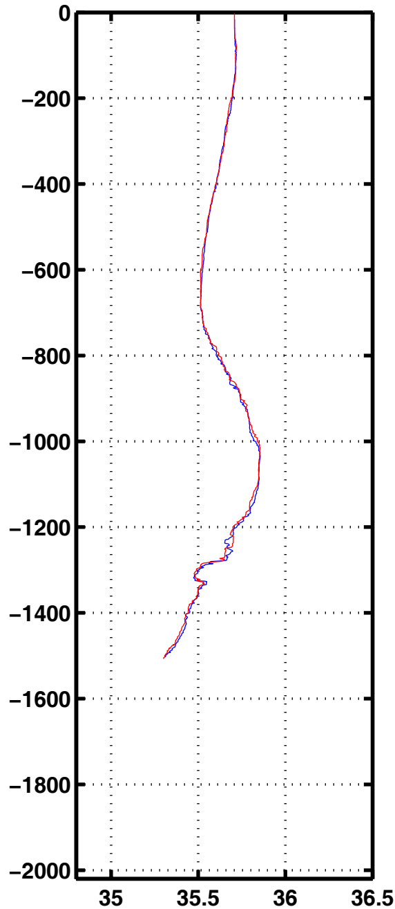
Sali 1170
