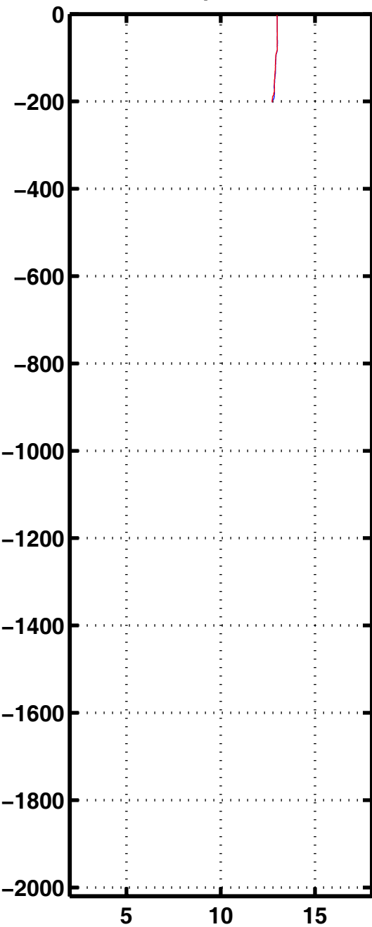
Tempe 1166
