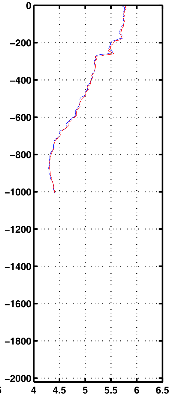
Oxyg 1095
