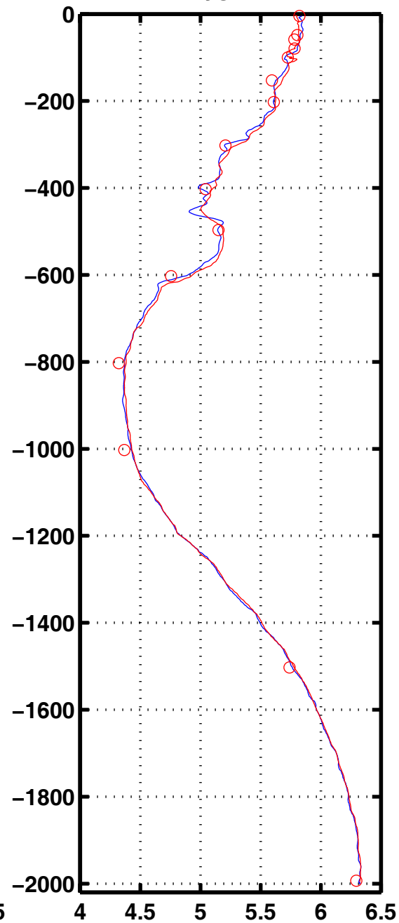
Oxyg 1067
