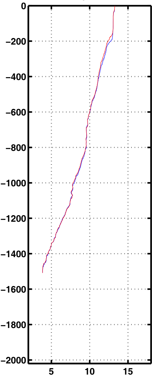
Tempe 1139
