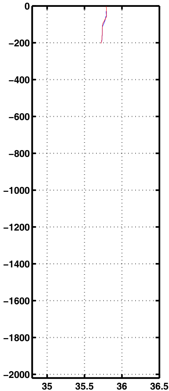
Sali 1112
