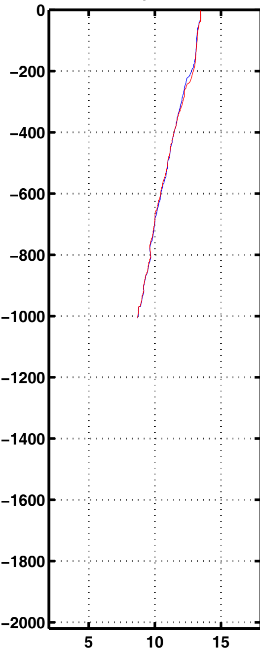
Tempe 1128
