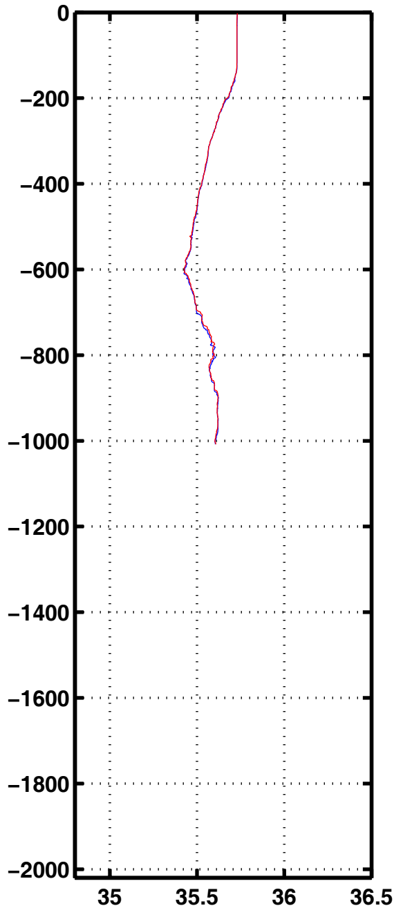
Sali 1107
