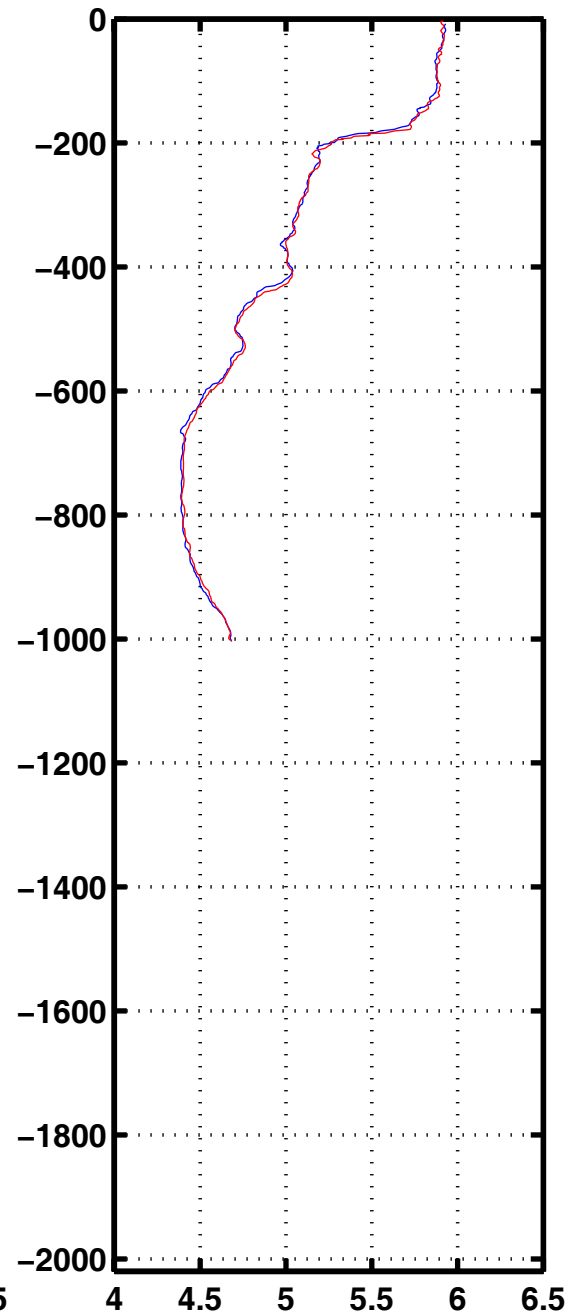
Oxyg 1133
