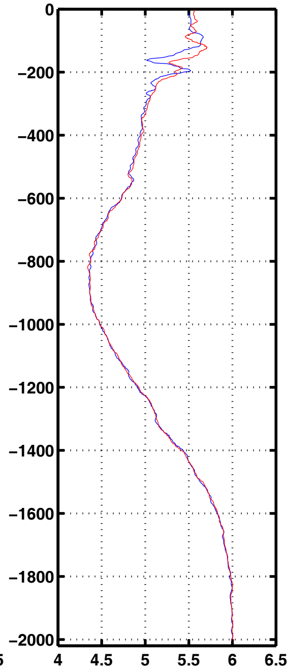
Oxyg 1118
