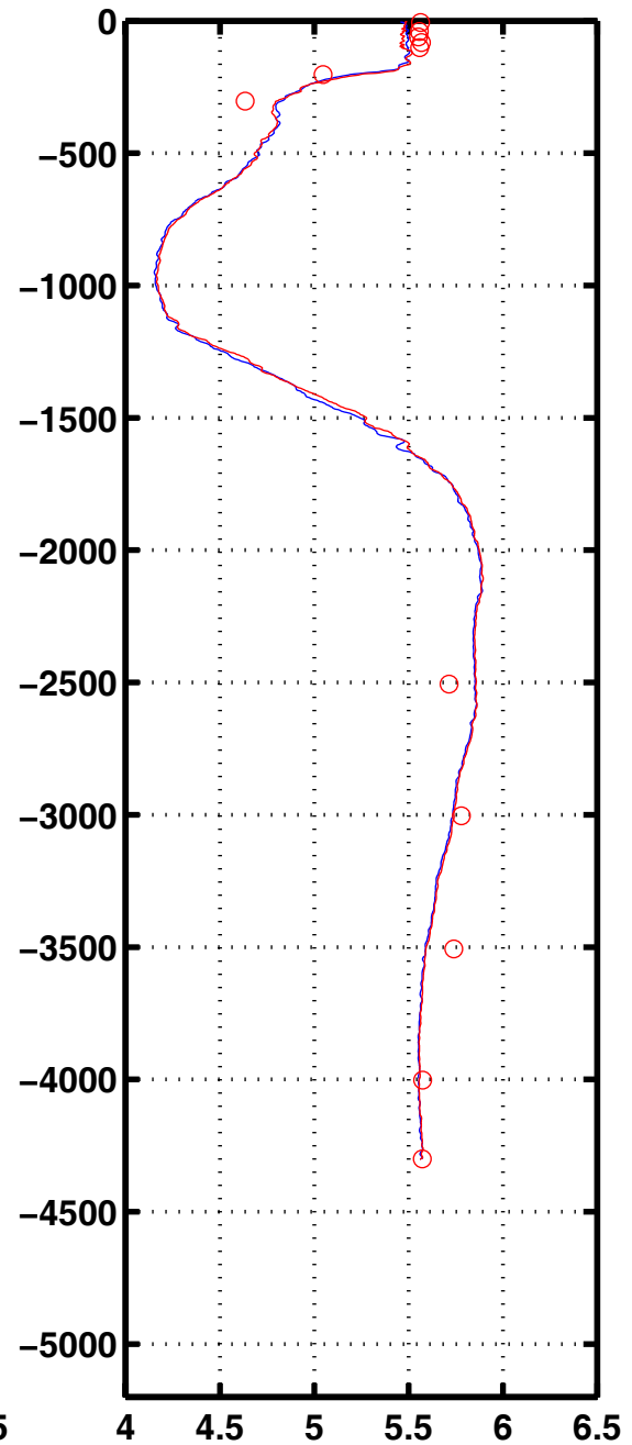
Oxyg 1074
