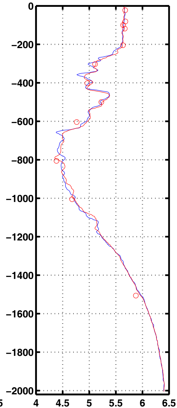
Oxyg 1016
