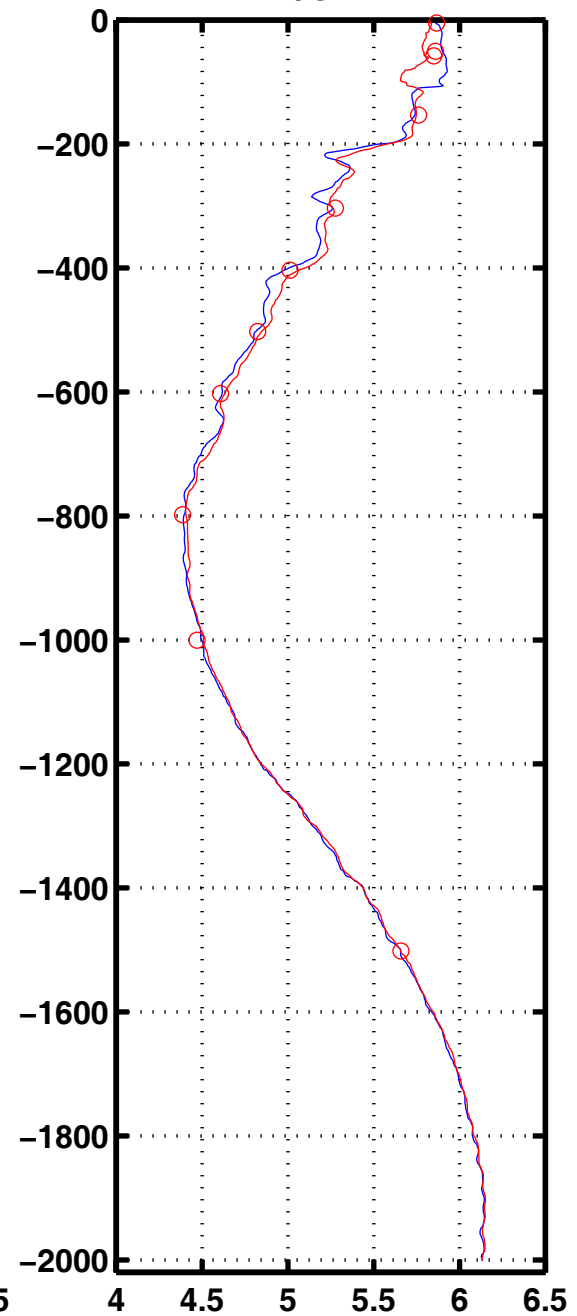
Oxyg 1048
