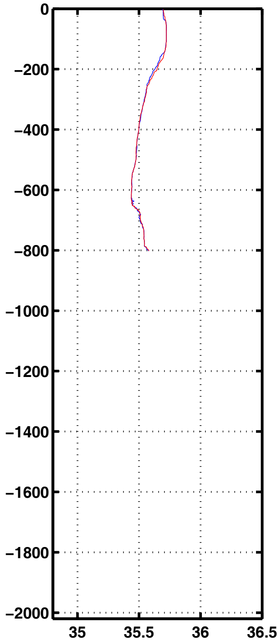
Sali 1147
