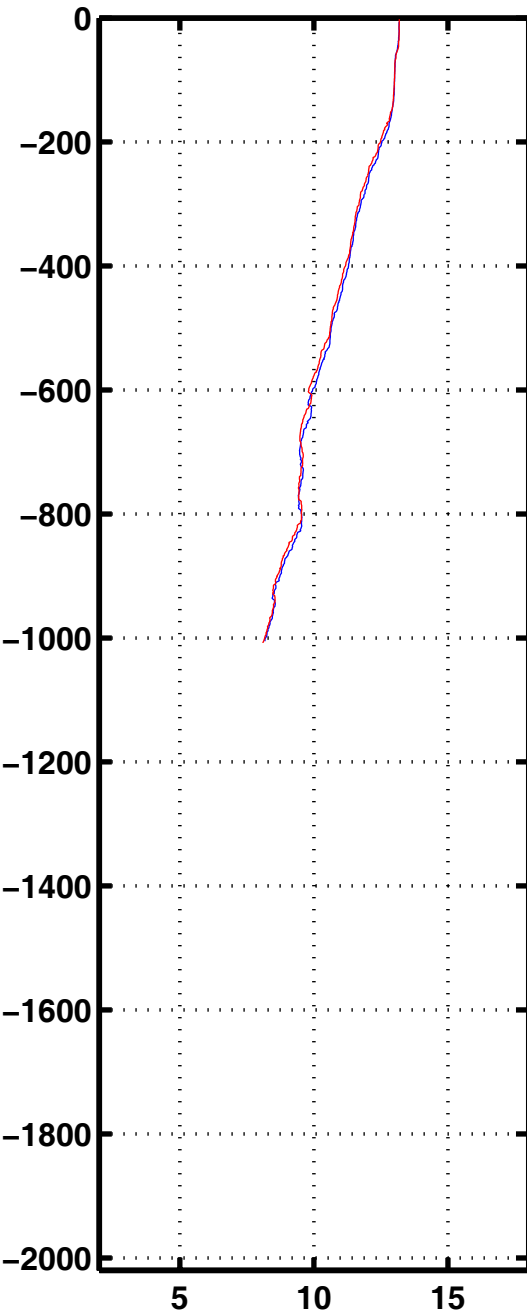
Tempe 1134
