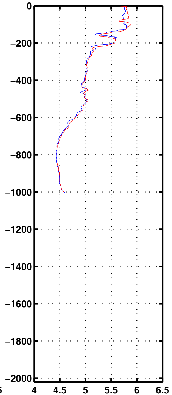
Oxyg 1156
