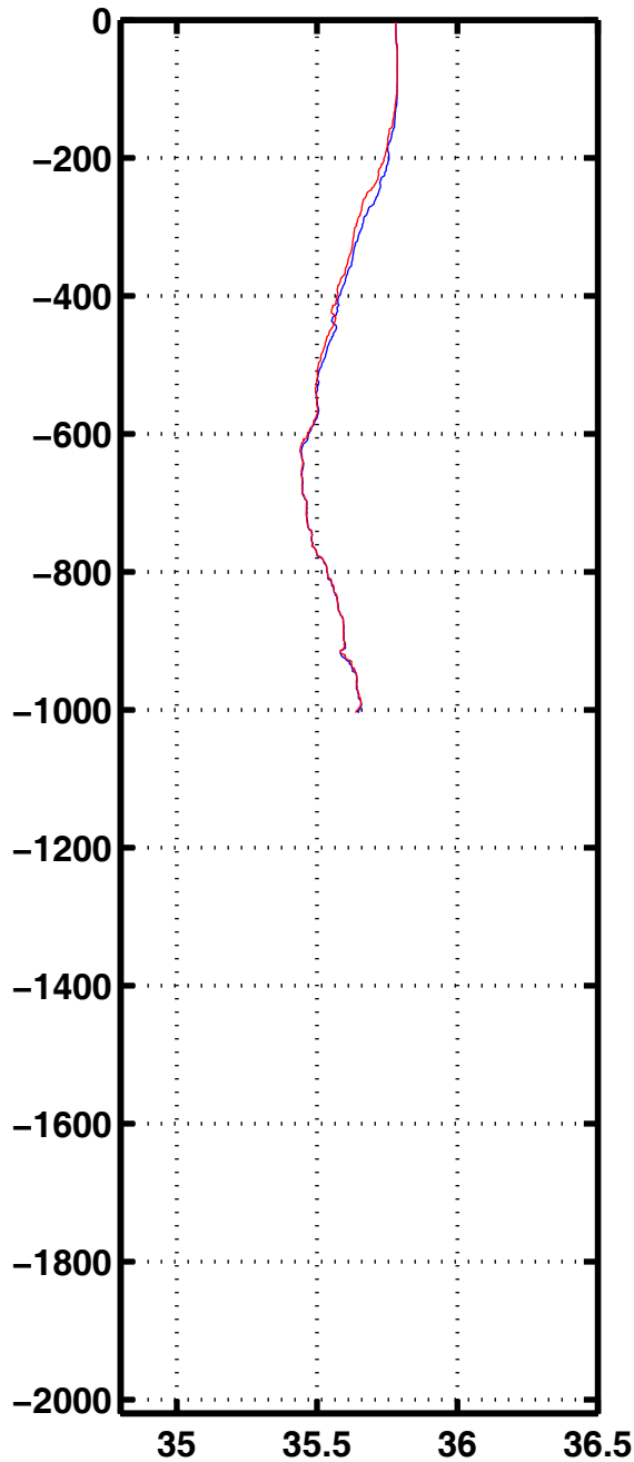
Sali 1127
