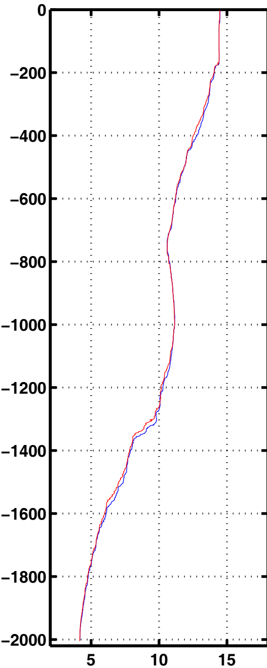
Tempe 1093
