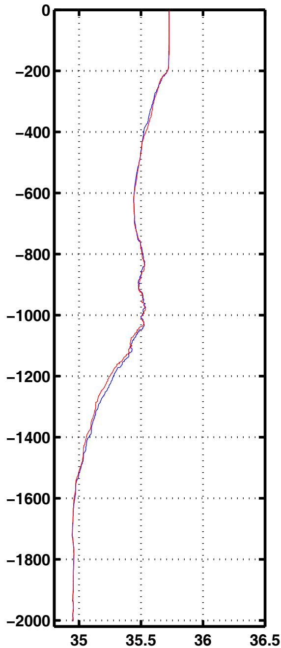
Sali 1068
