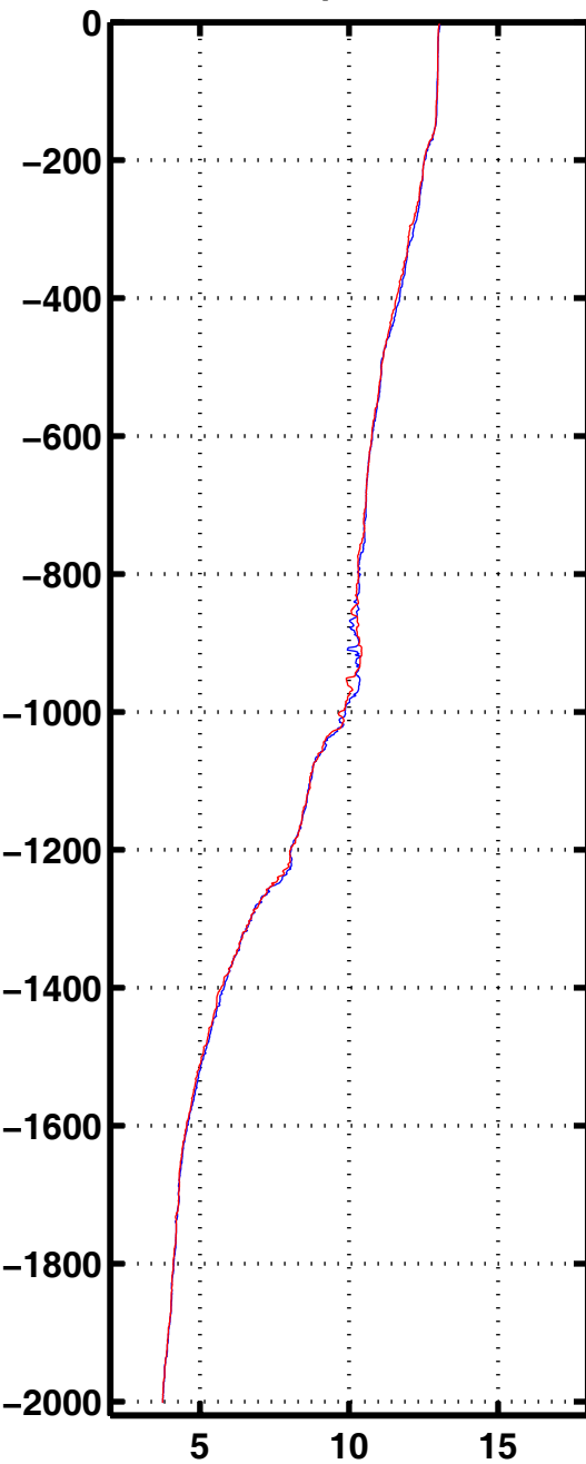
Tempe 1040
