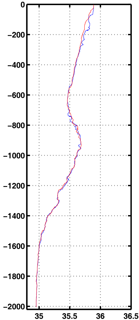
Sali 1118
