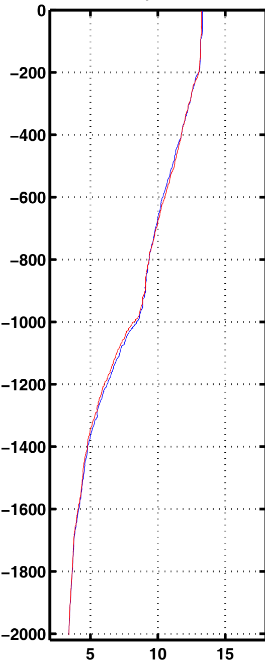
Tempe 1065
