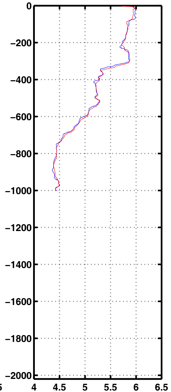
Oxyg 1158
