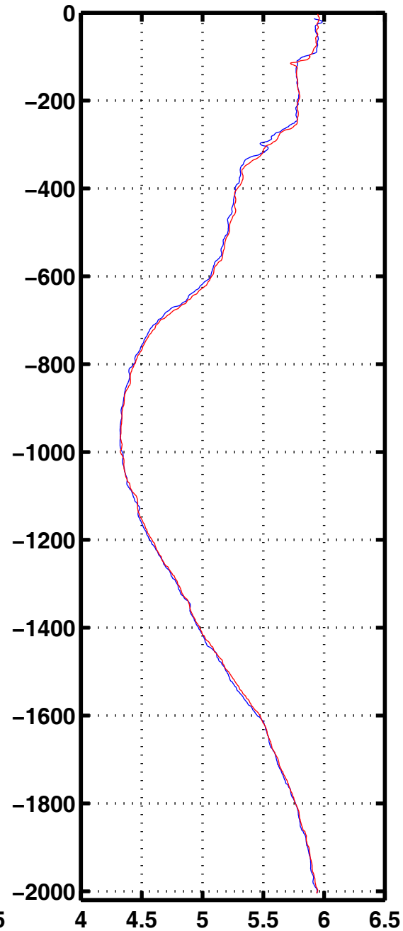
Oxyg 1181
