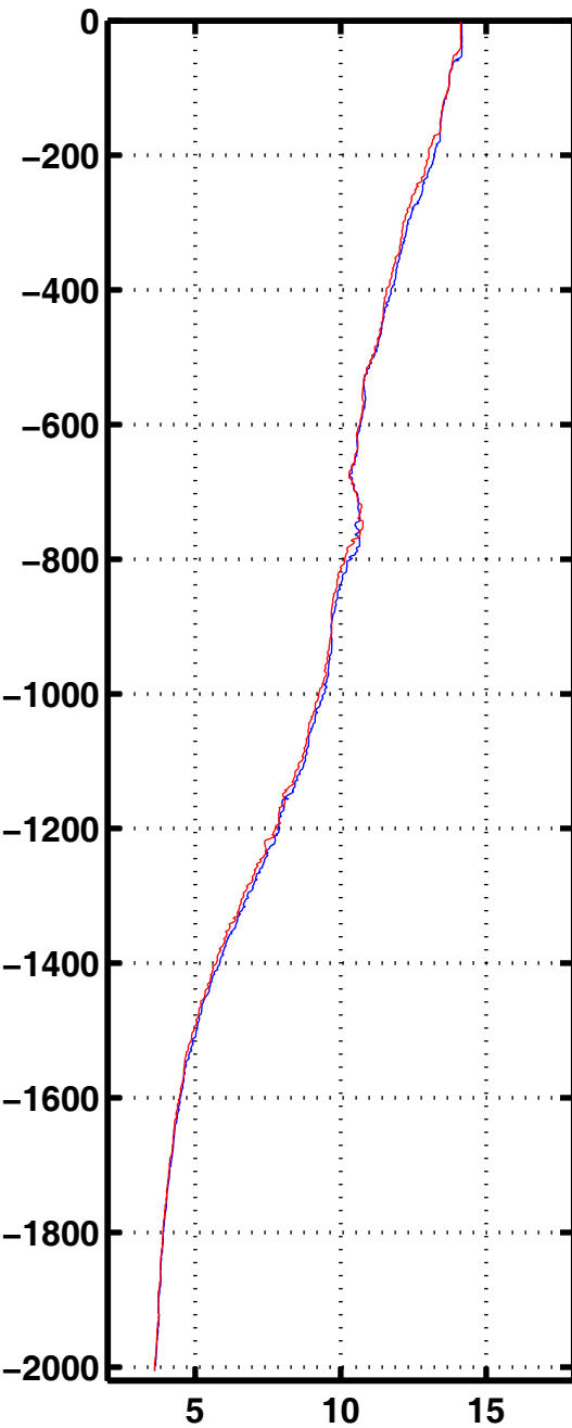
Tempe 1026
