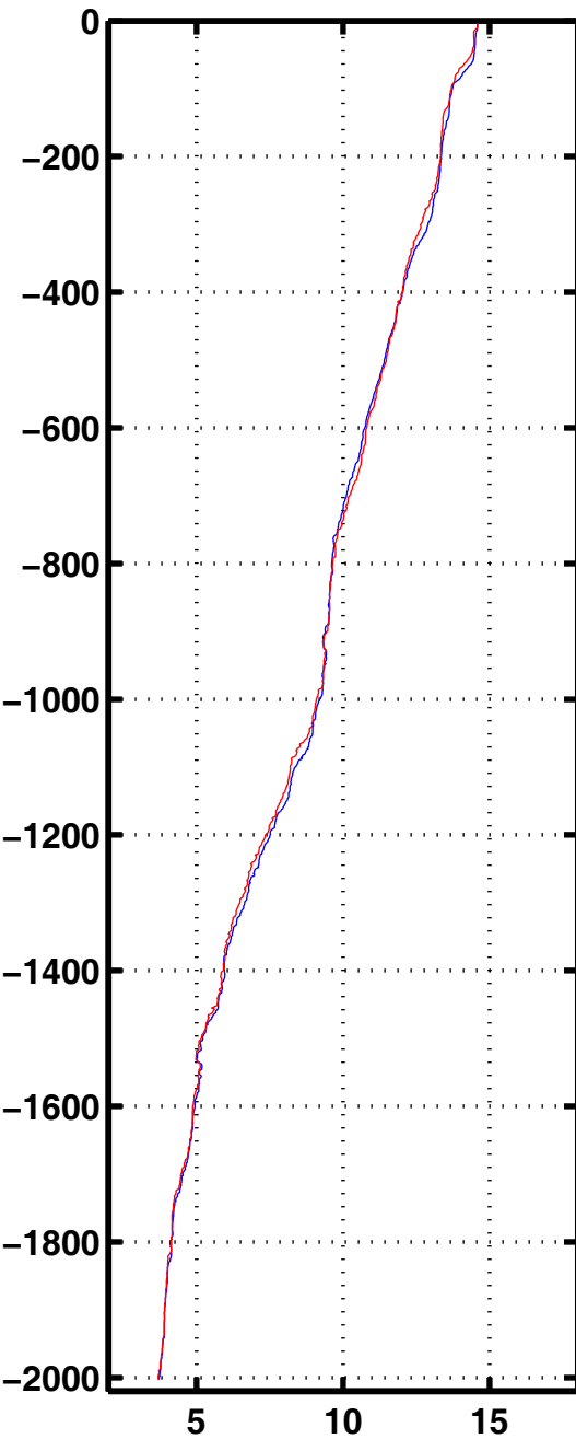
Tempe 1052
