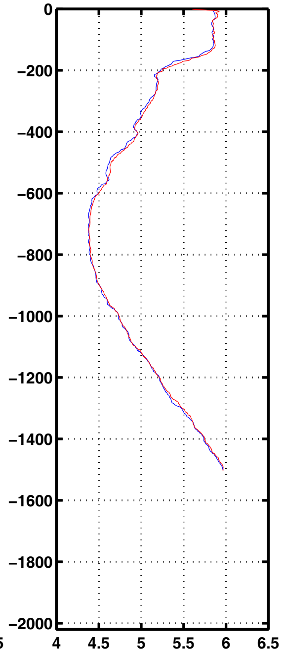
Oxyg 1138
