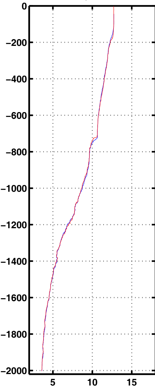
Tempe 1013
