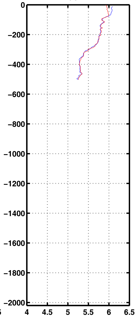
Oxyg 1179
