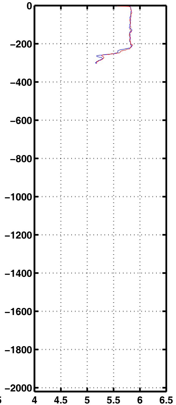
Oxyg 1111
