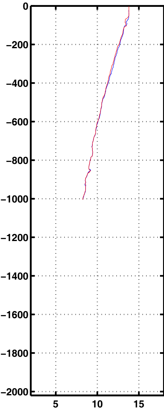
Tempe 1153
