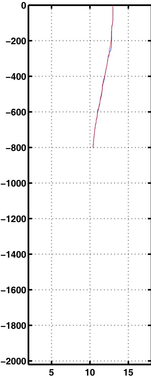
Tempe 1174
