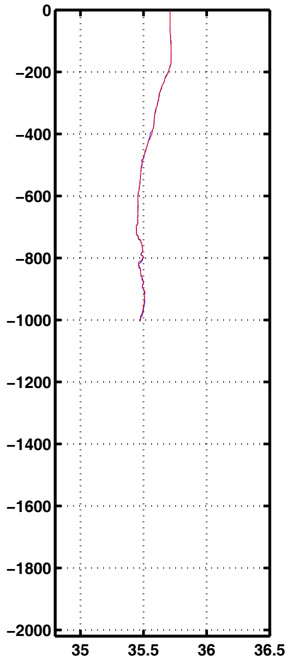
Sali 1155
