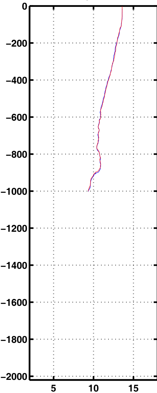
Tempe 1196
