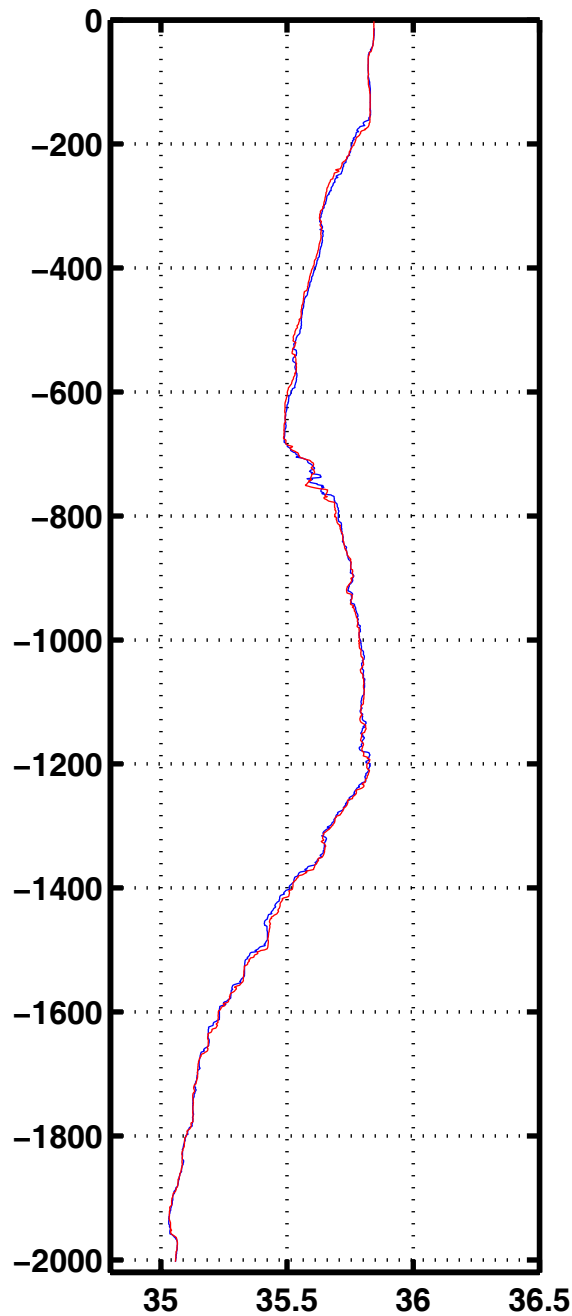
Sali 1031
