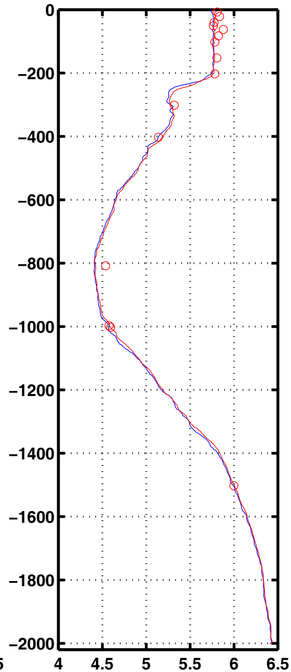
Oxyg 1019
