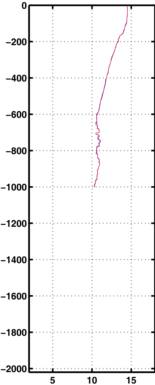
Tempe 1205
