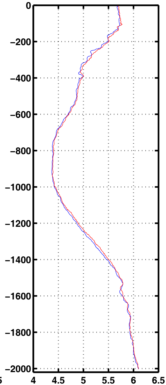
Oxyg 1006
