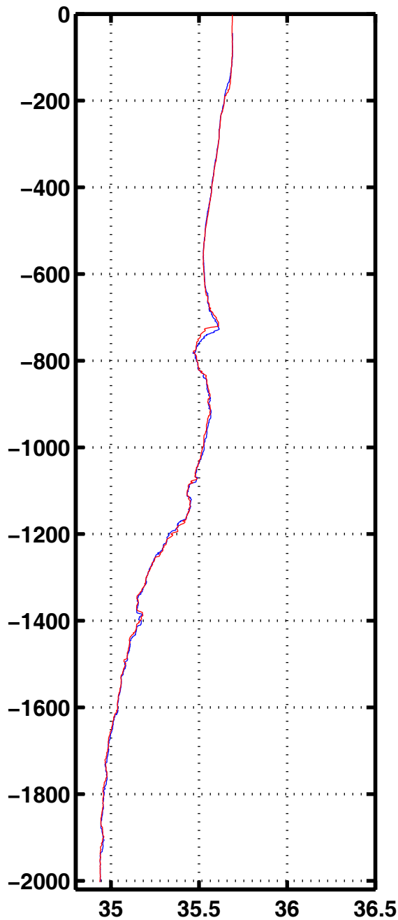
Sali 1013
