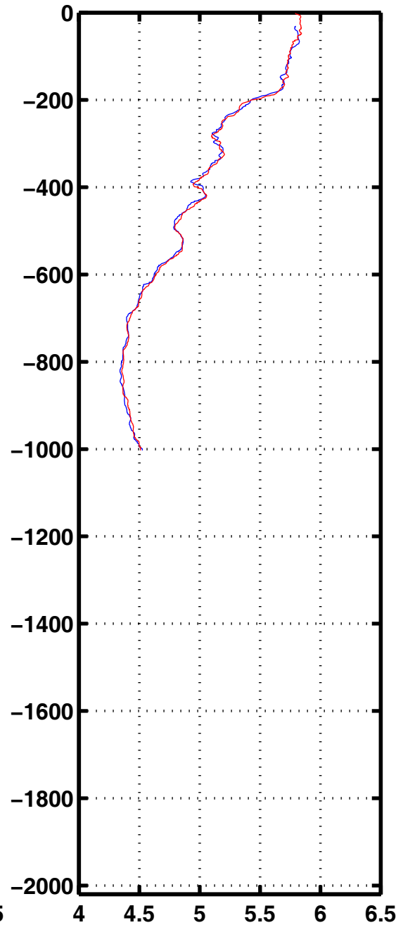
Oxyg 1120
