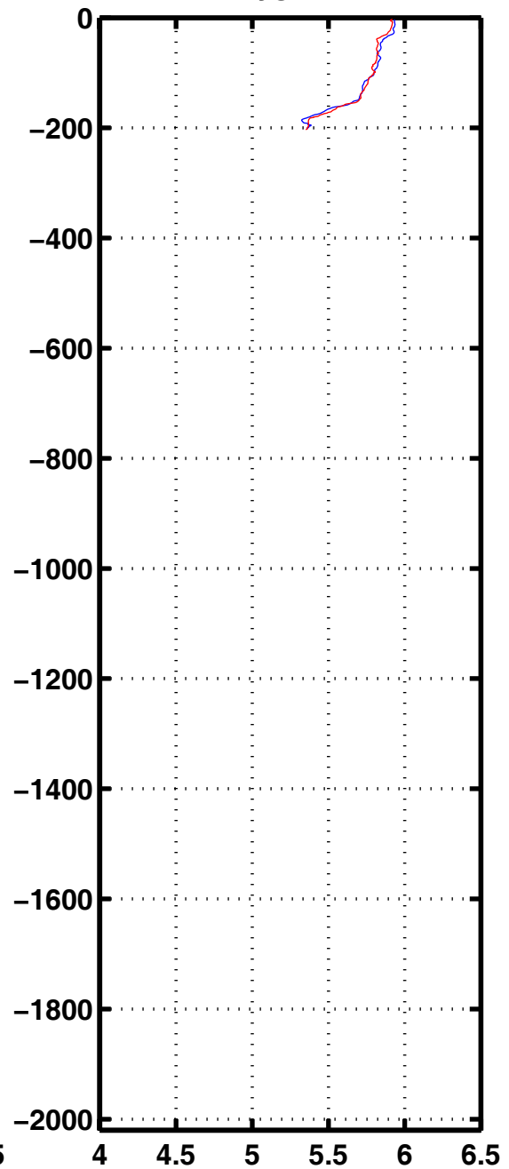
Oxyg 1144
