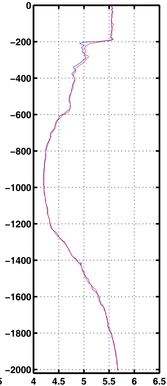
Oxyg 1080
