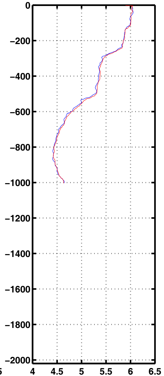
Oxyg 1165
