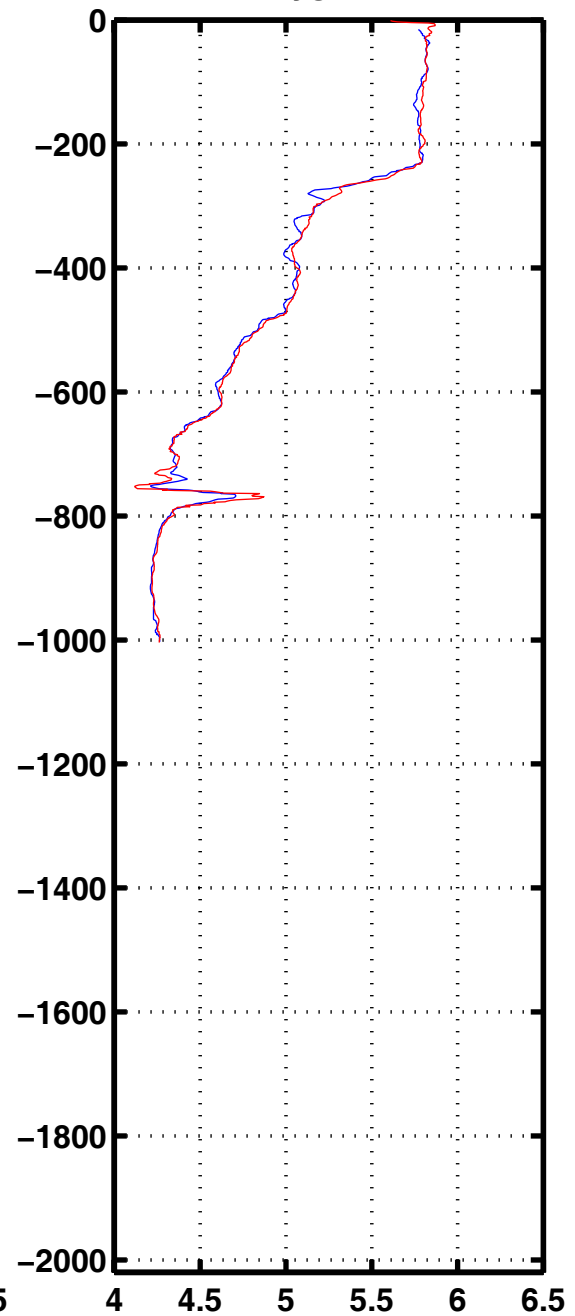
Oxyg 1110
