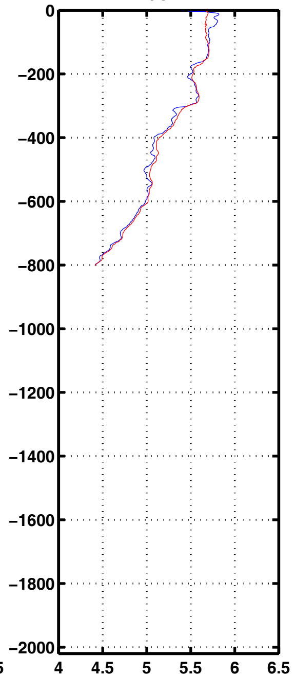
Oxyg 1091
