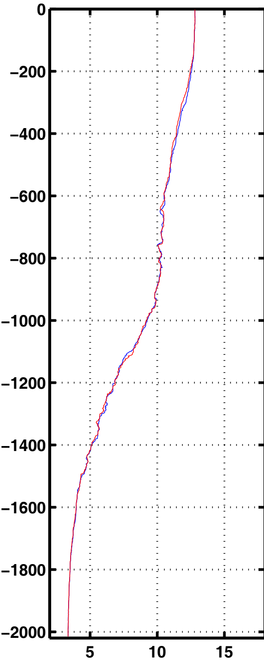
Tempe 1182
