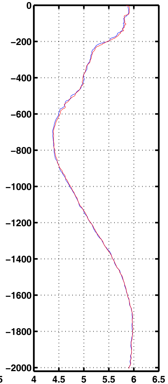
Oxyg 1150
