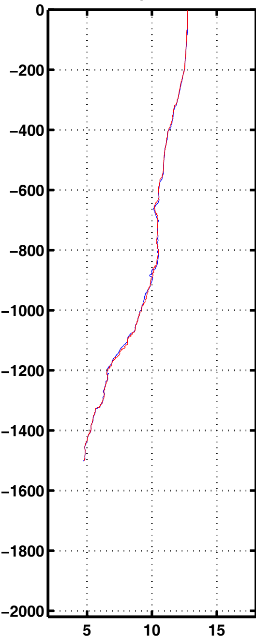
Tempe 1185
