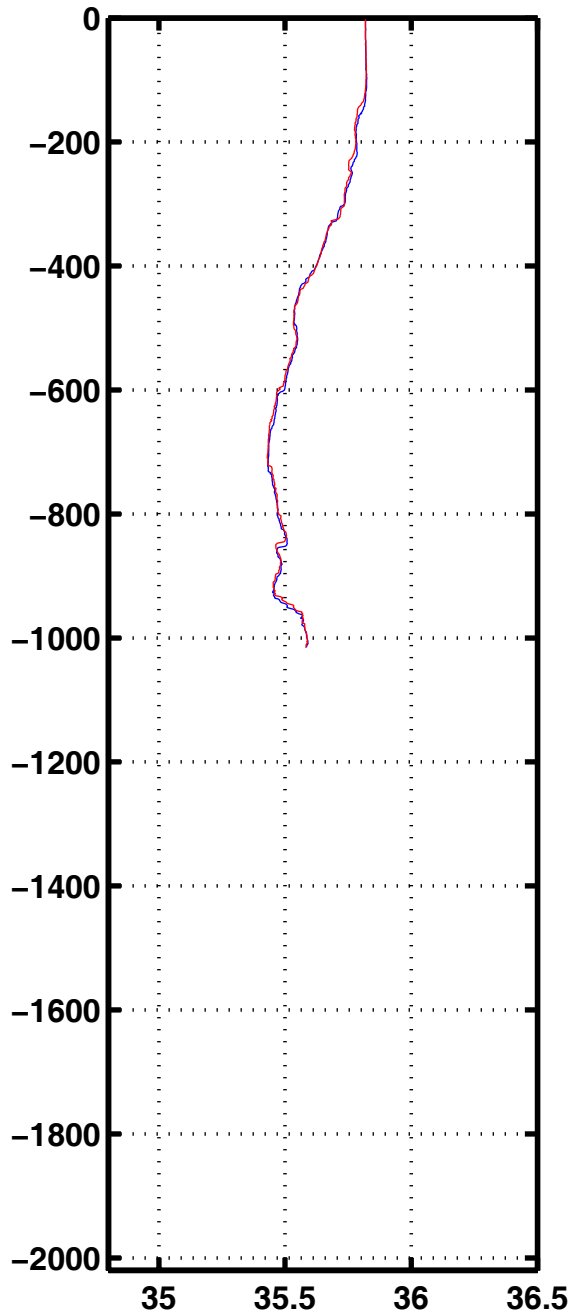
Sali 1126
