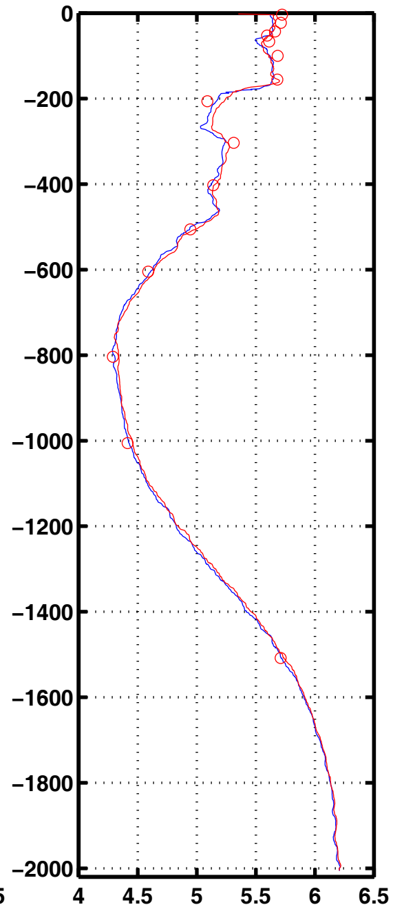
Oxyg 1026
