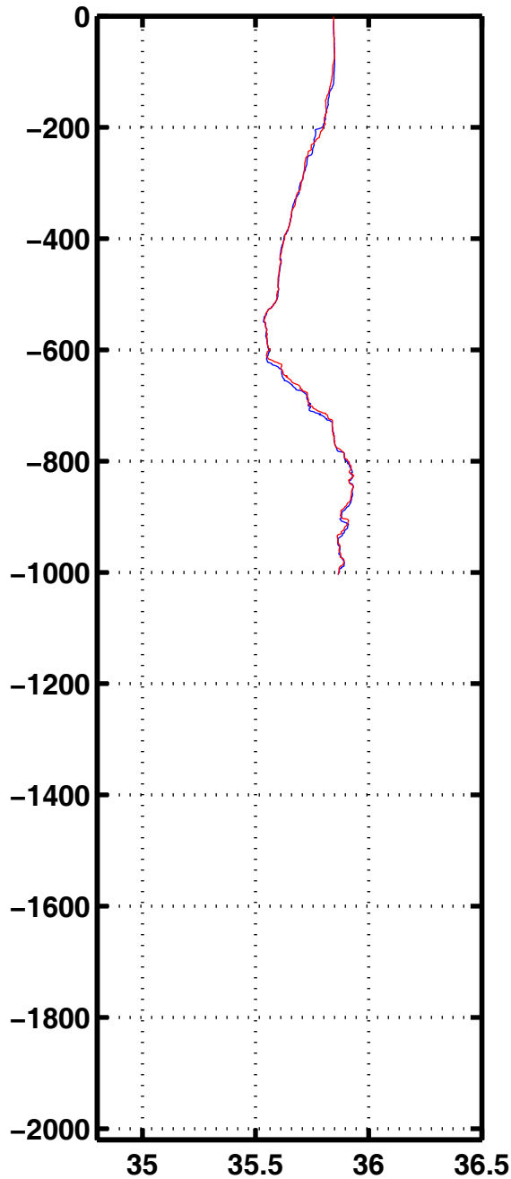
Sali 1202
