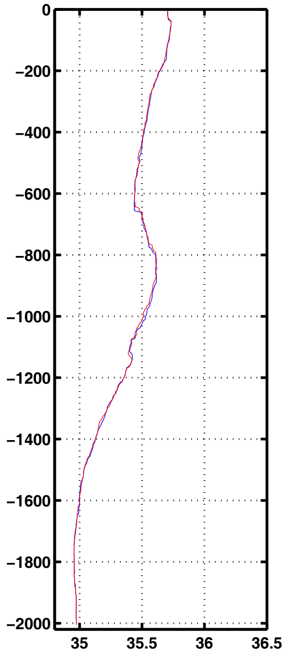
Sali 1149
