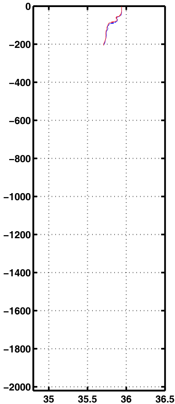
Sali 1108
