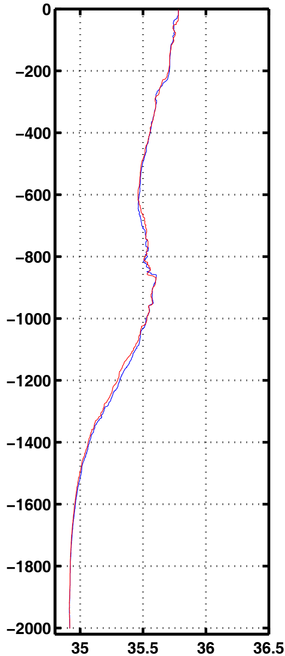
Sali 1046
