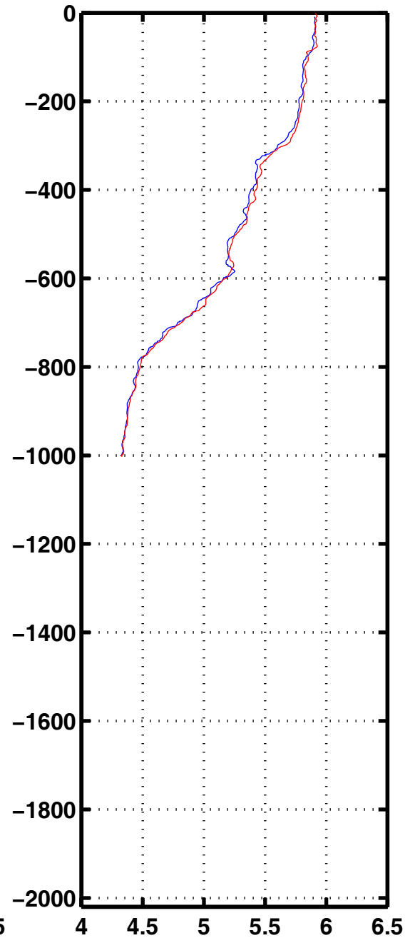
Oxyg 1160
