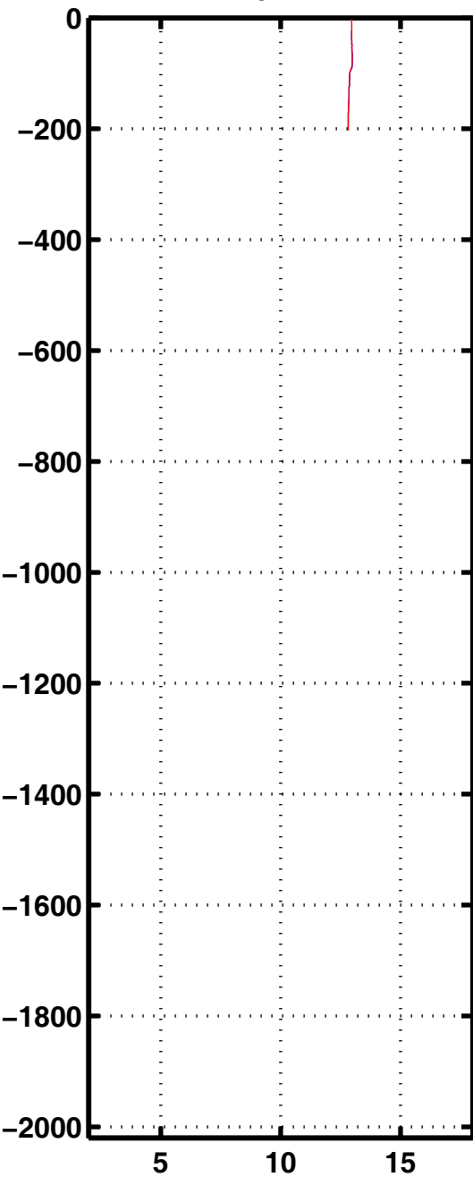
Tempe 1180
