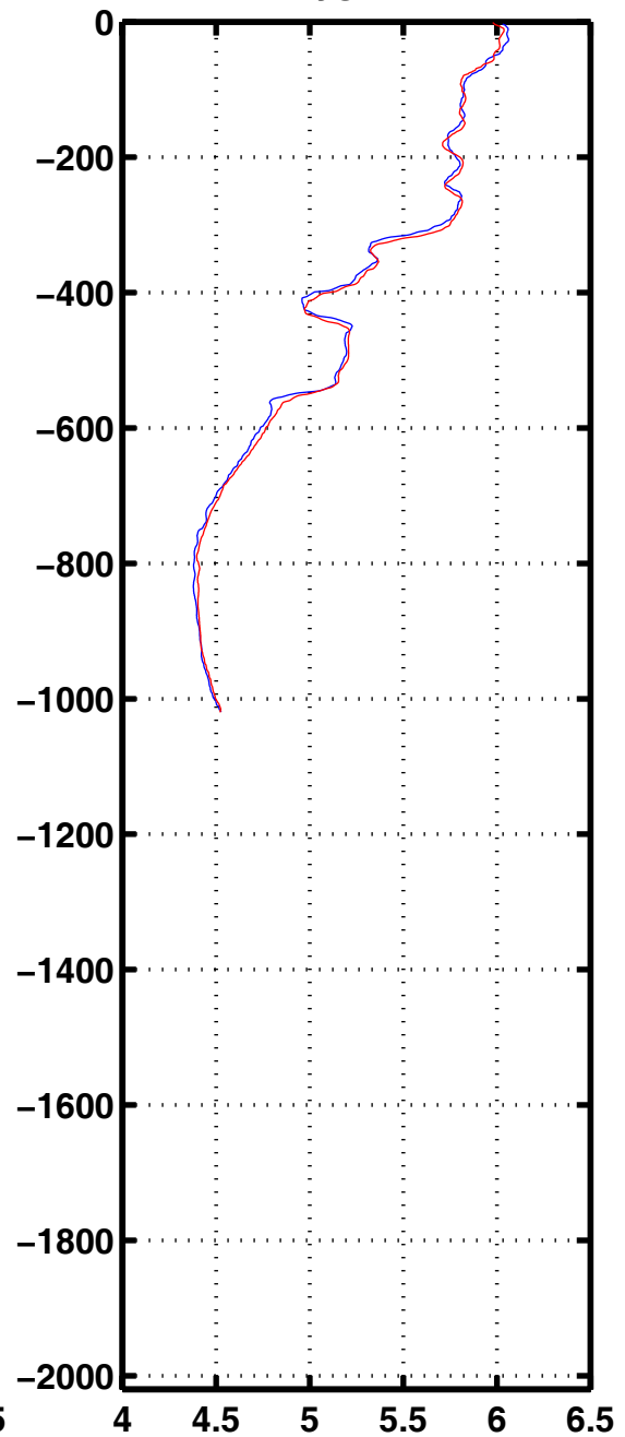
Oxyg 1192
