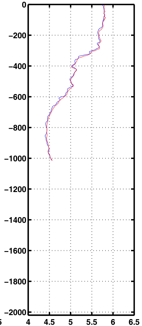
Oxyg 1126
