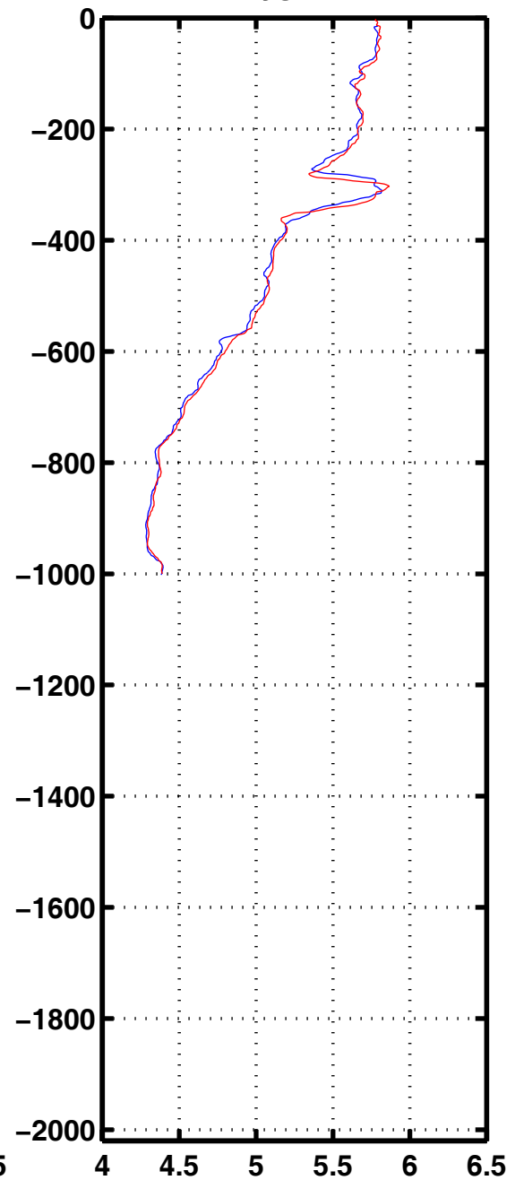
Oxyg 1195
