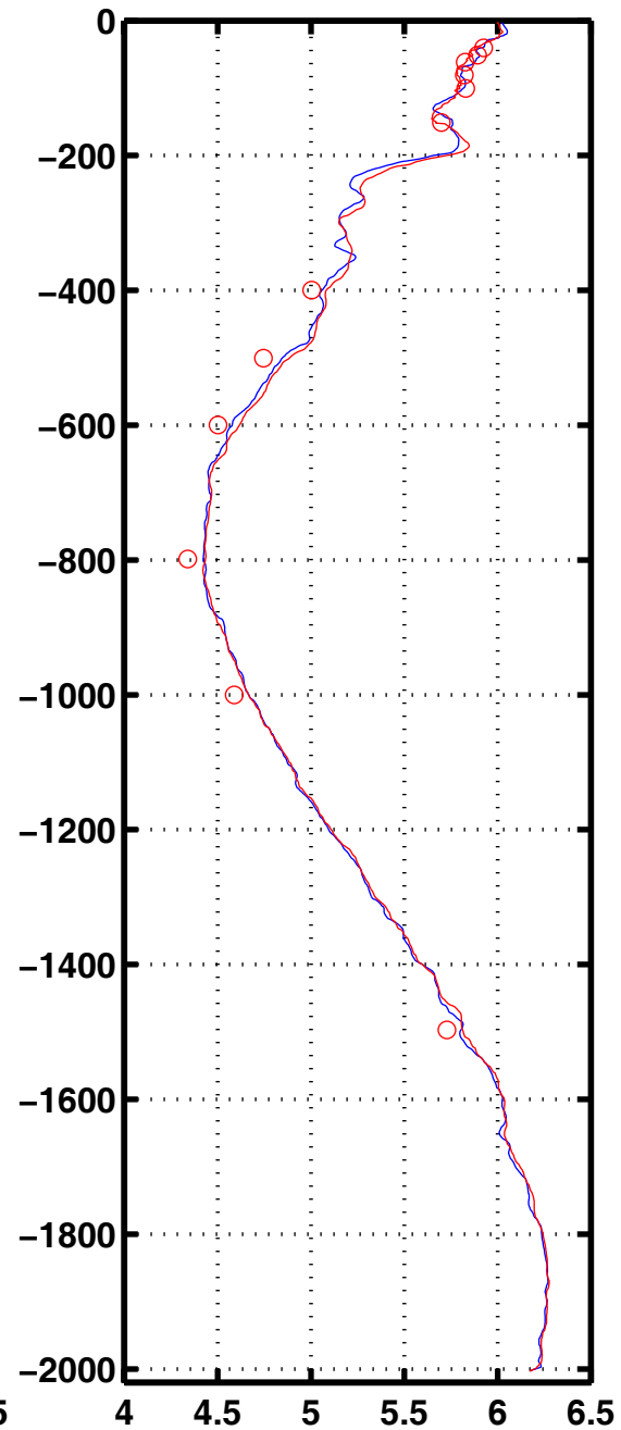
Oxyg 1049
