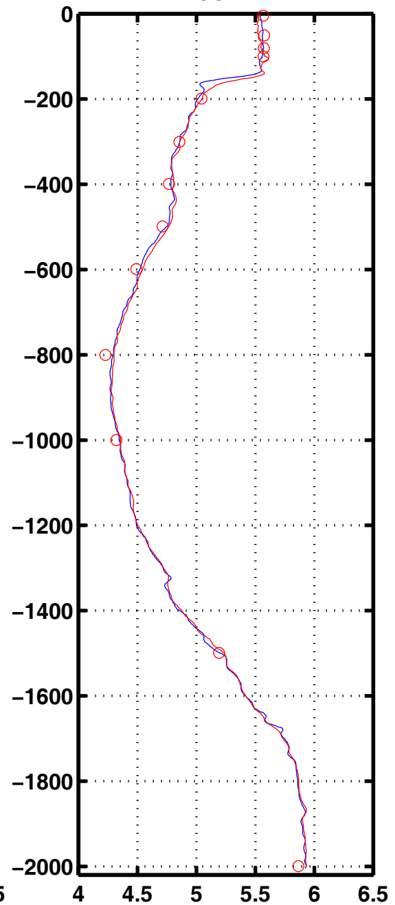
Oxyg 1078
