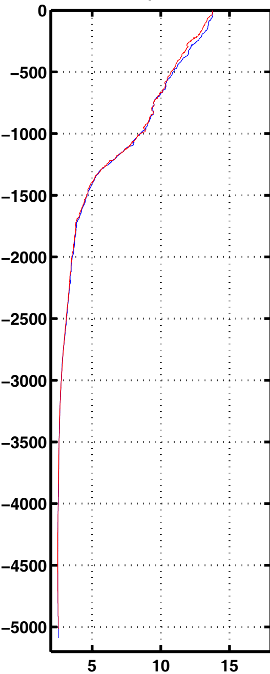
Tempe 1051
