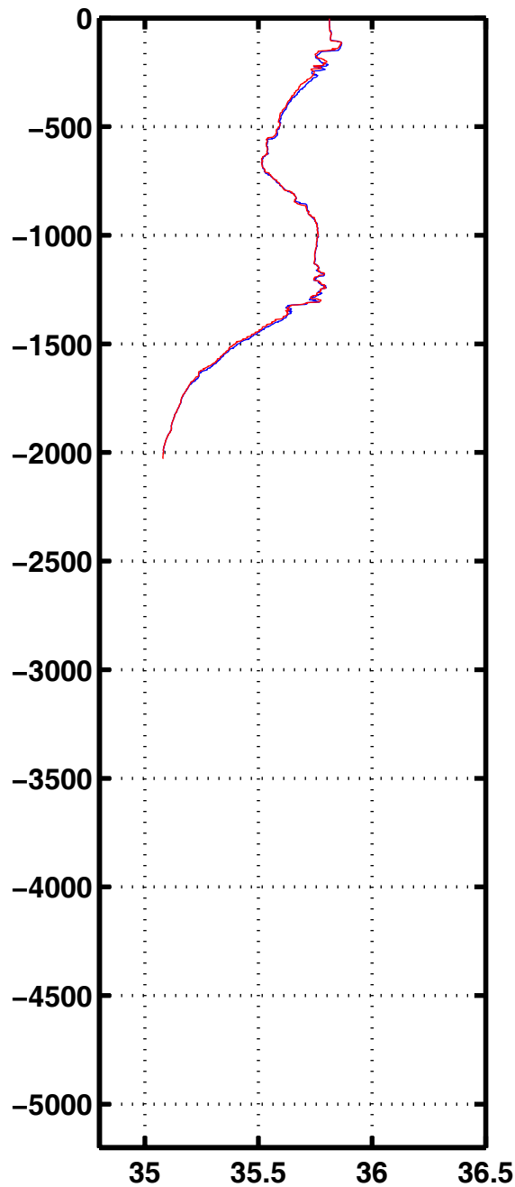
Sali 1002
