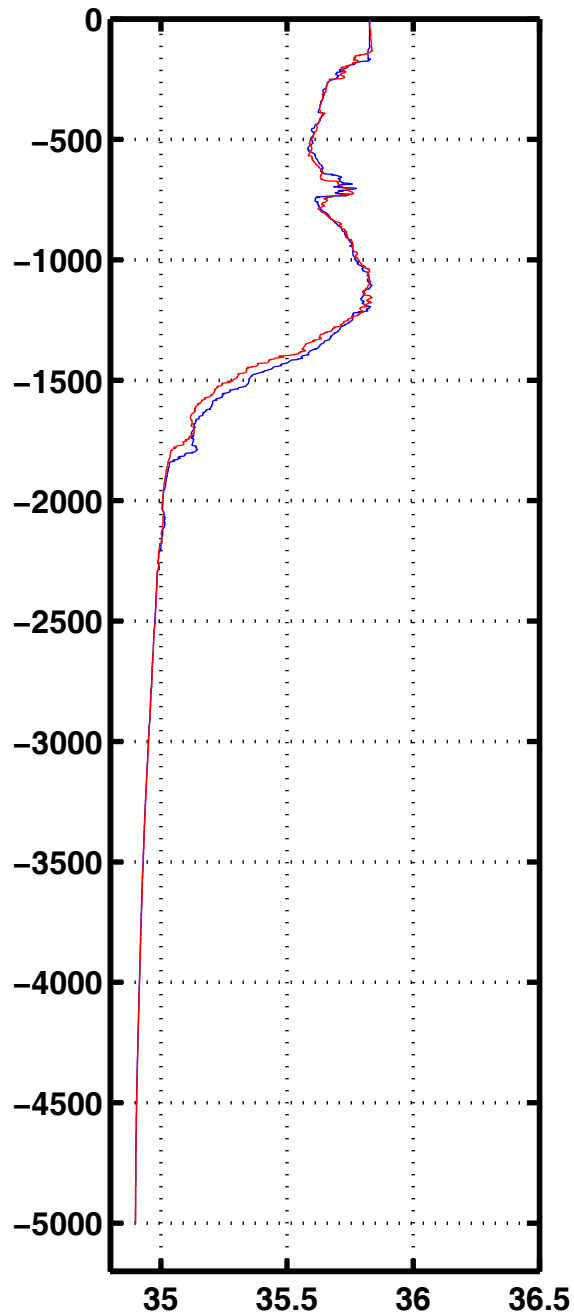
Sali 1003
