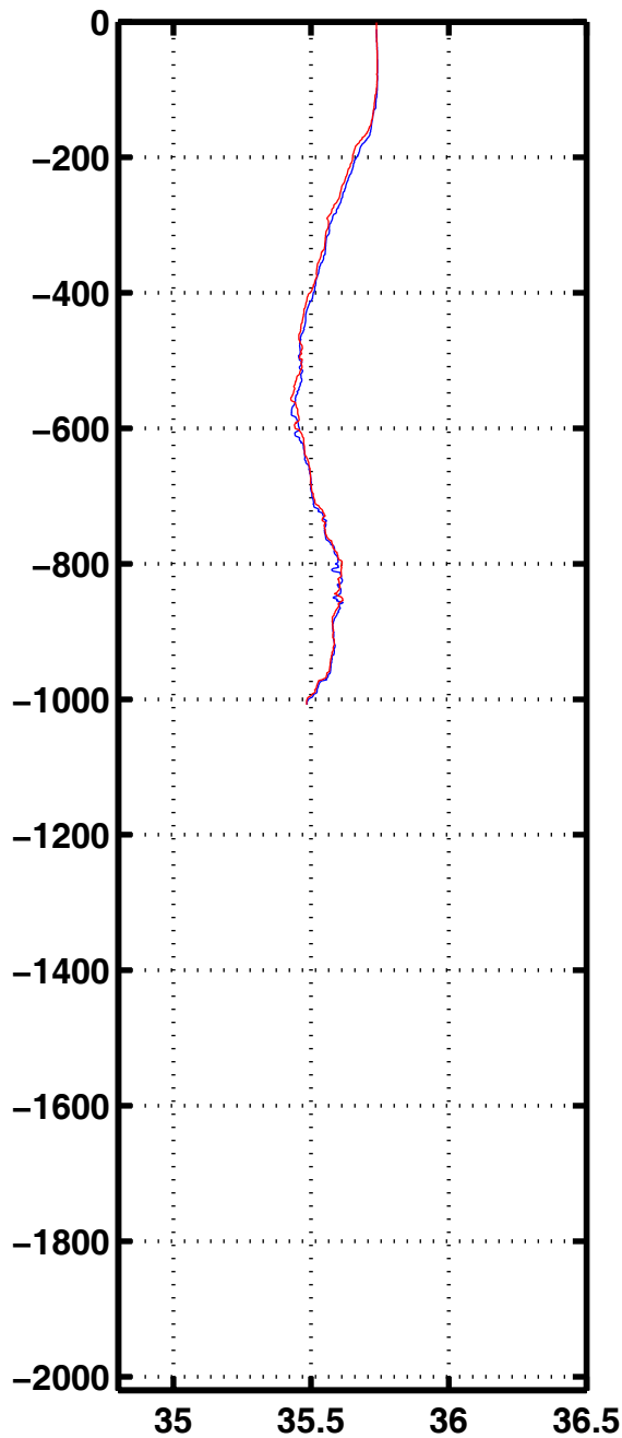
Sali 1136
