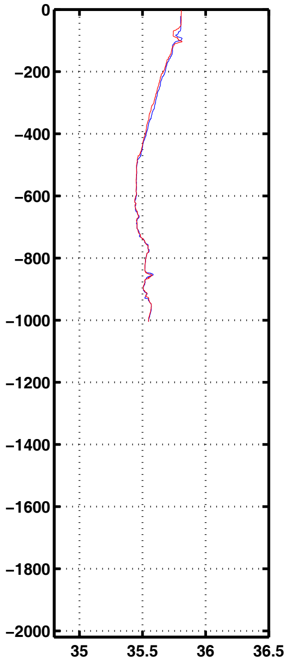
Sali 1153
