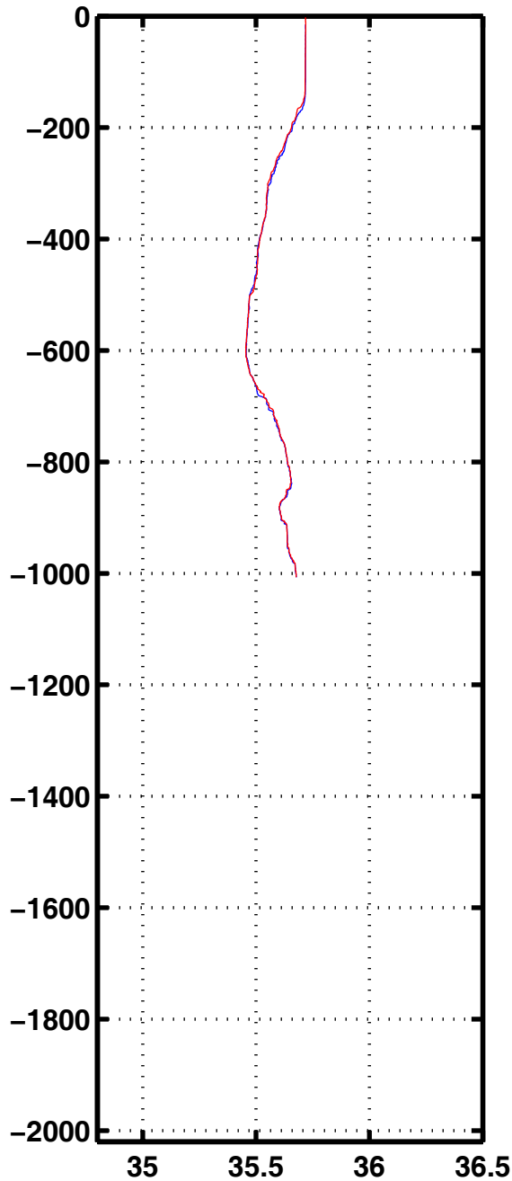
Sali 1131
