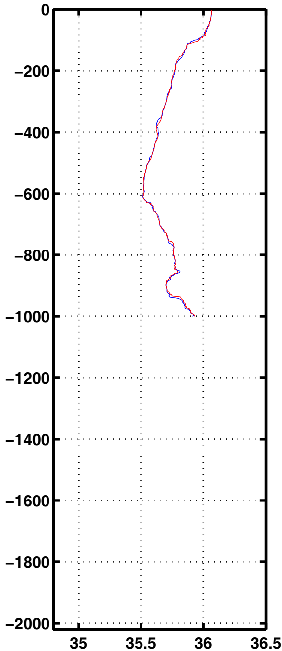
Sali 1102
