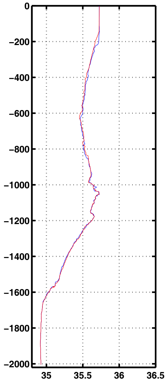
Sali 1042
