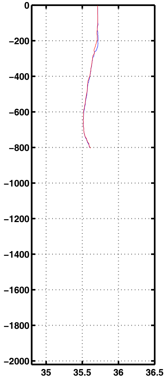
Sali 1174
