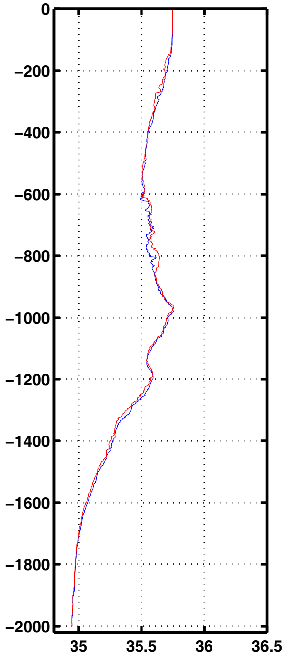
Sali 1039
