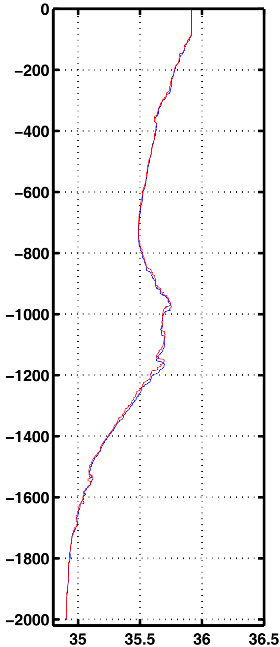
Sali 1071
