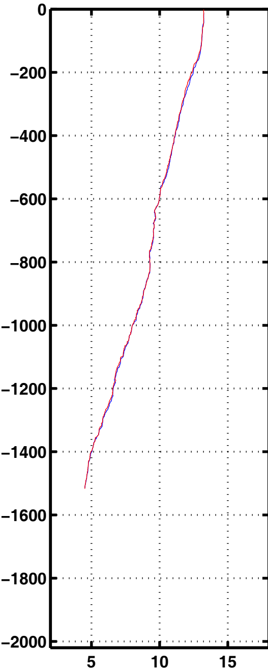
Tempe 1148
