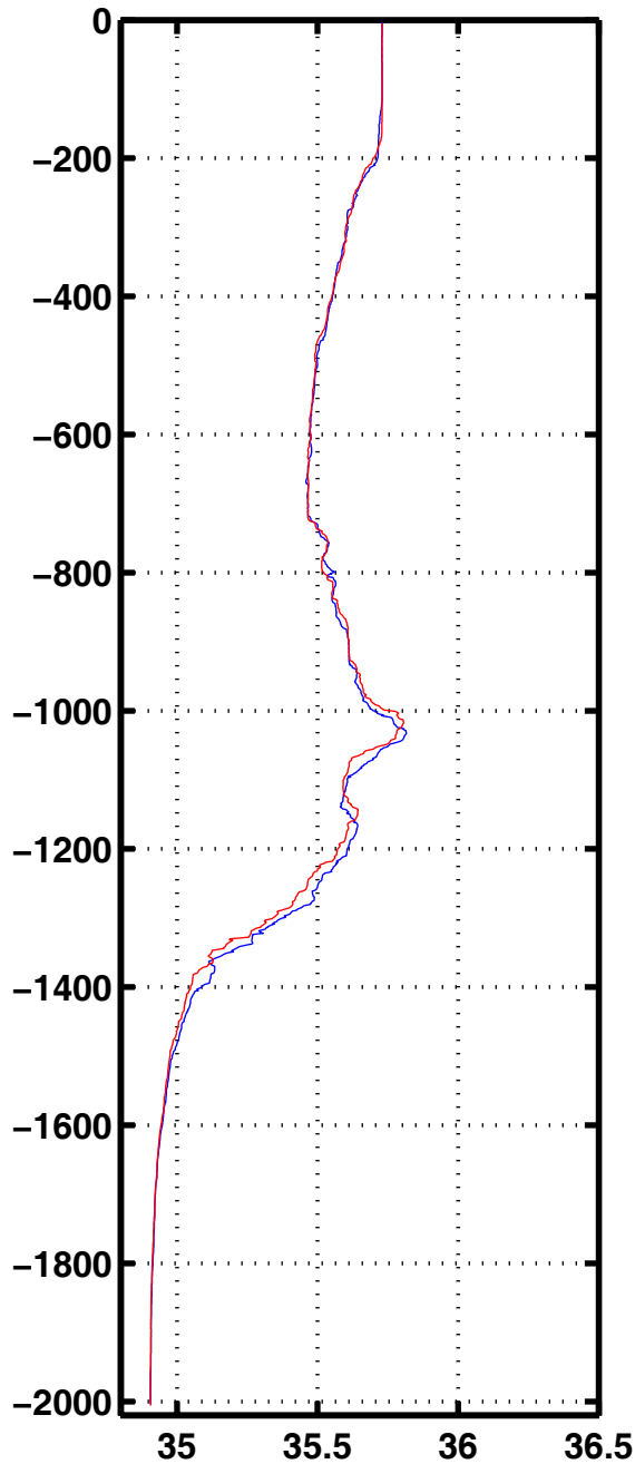
Sali 1043
