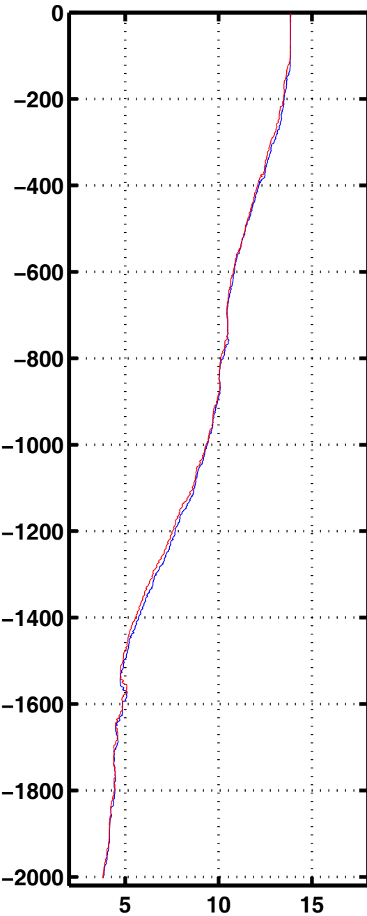
Tempe 1006
