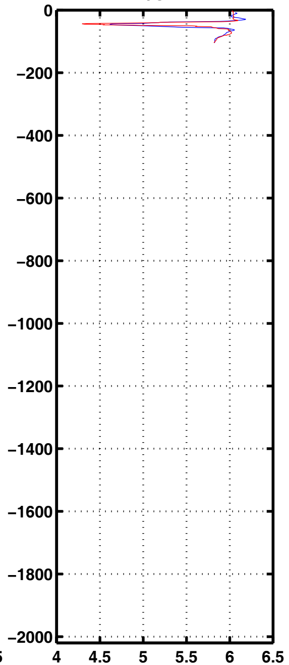
Oxyg 1183
