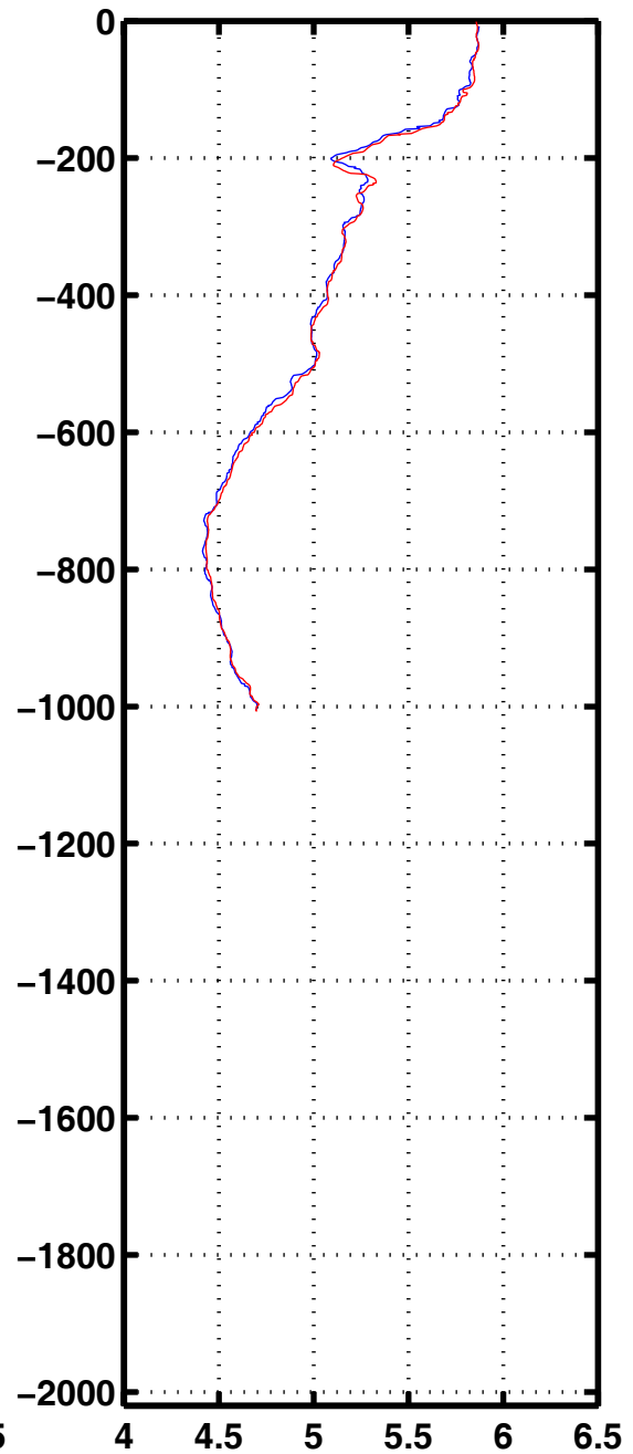
Oxyg 1154
