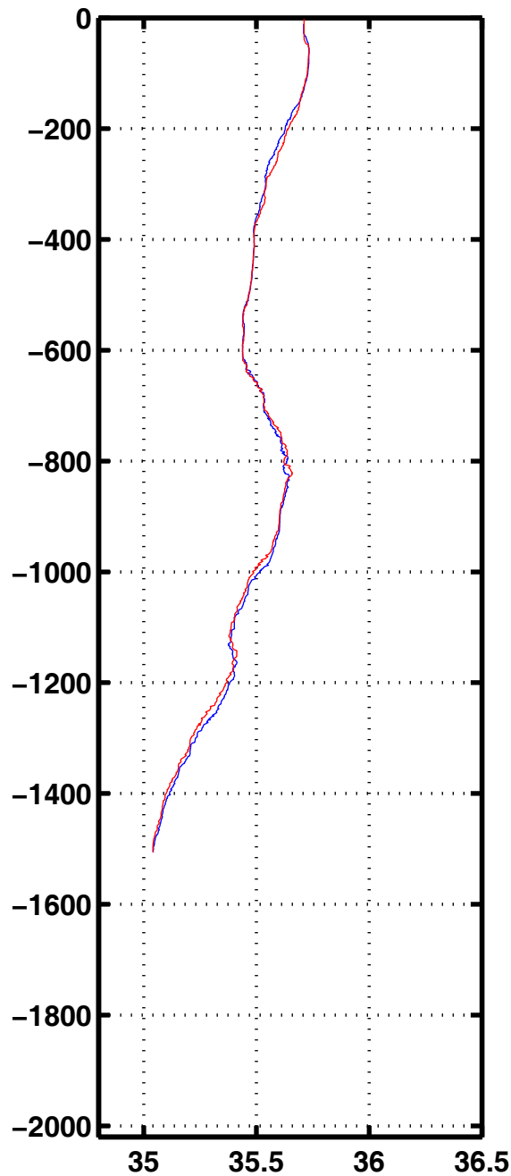
Sali 1141
