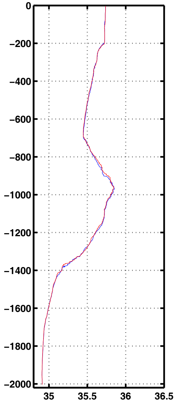
Sali 1020
