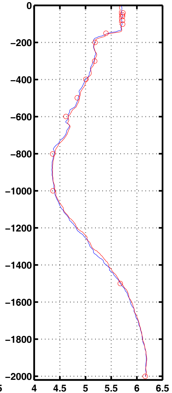
Oxyg 1072
