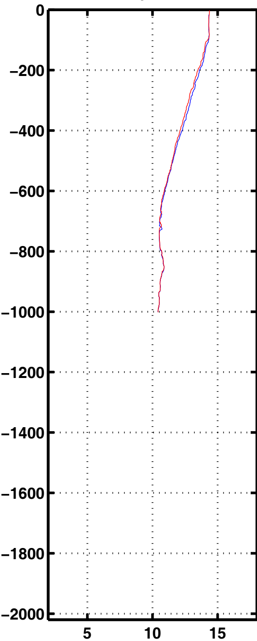
Tempe 1101
