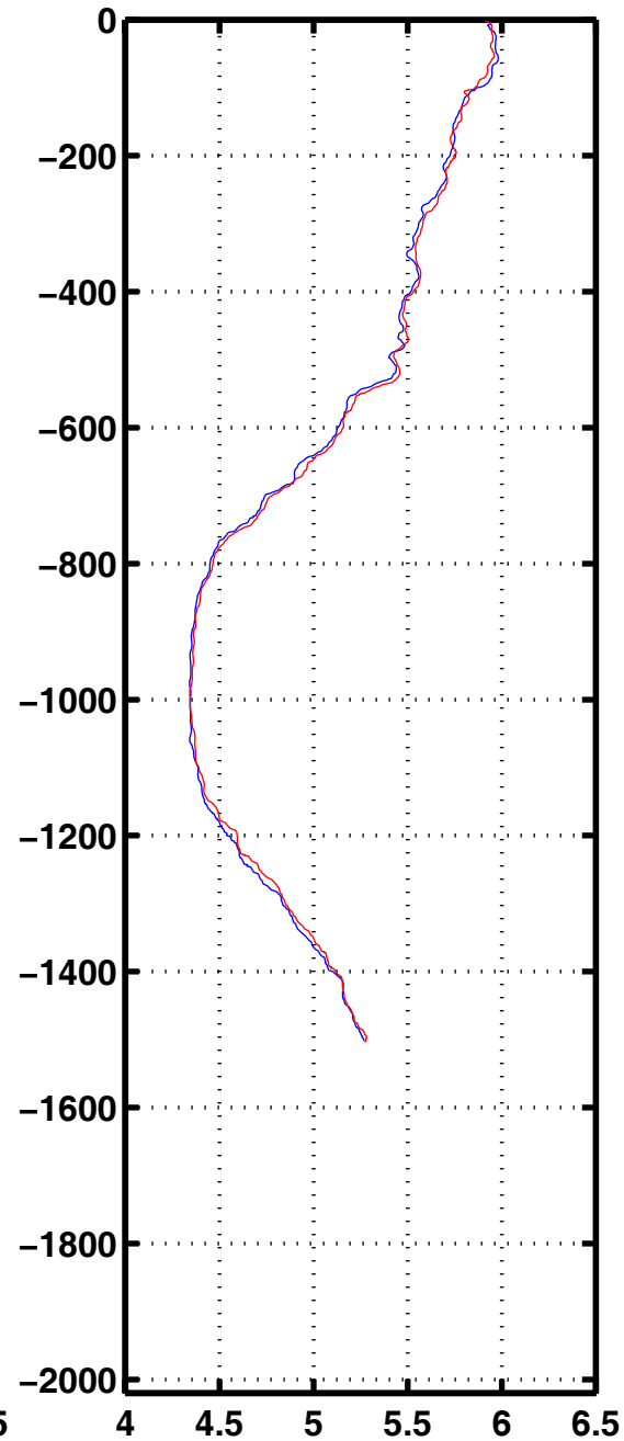
Oxyg 1167
