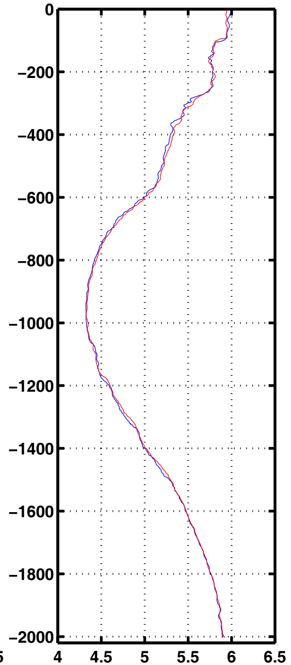
Oxyg 1177
