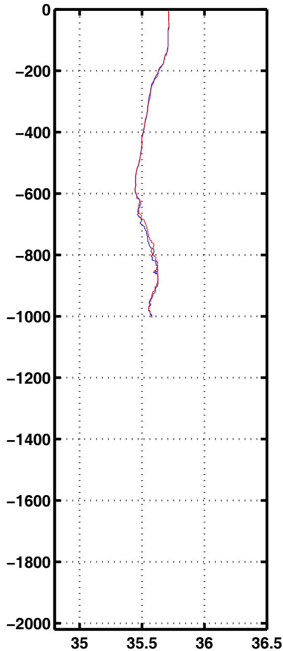
Sali 1133
