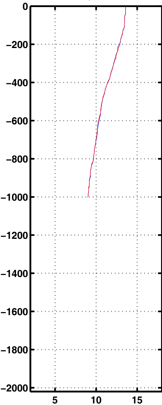
Tempe 1129
