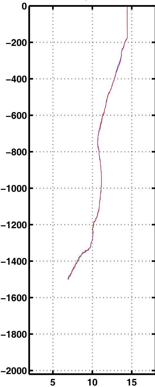
Tempe 1092
