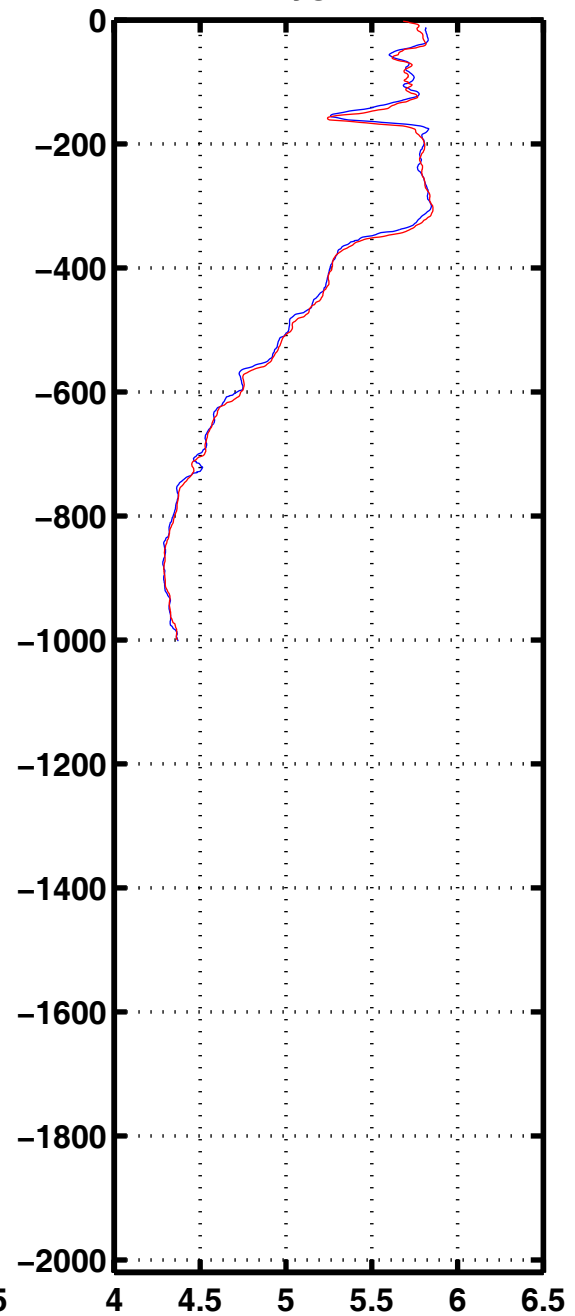
Oxyg 1194
