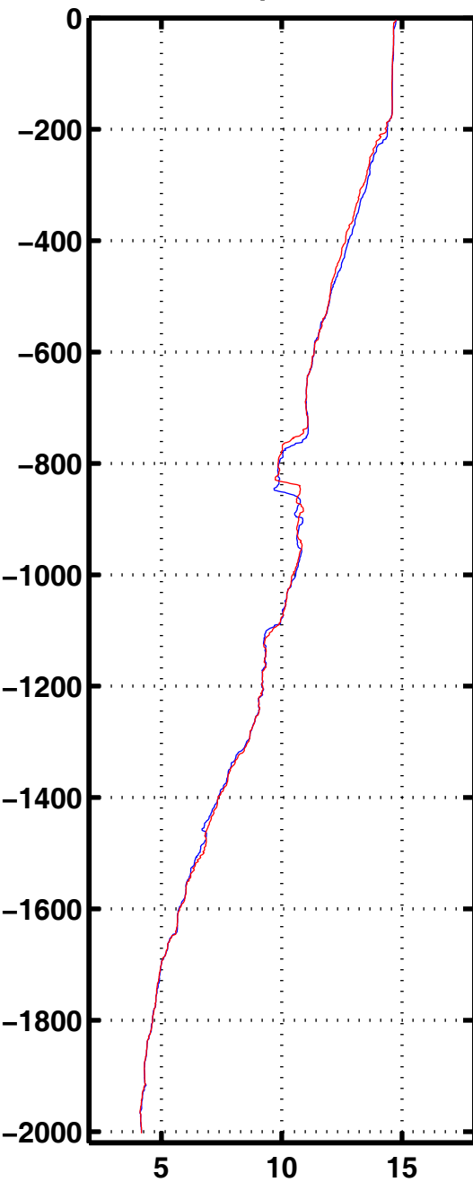
Tempe 1035
