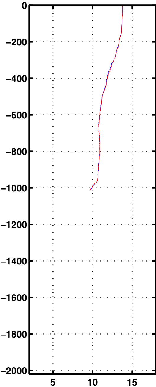
Tempe 1201
