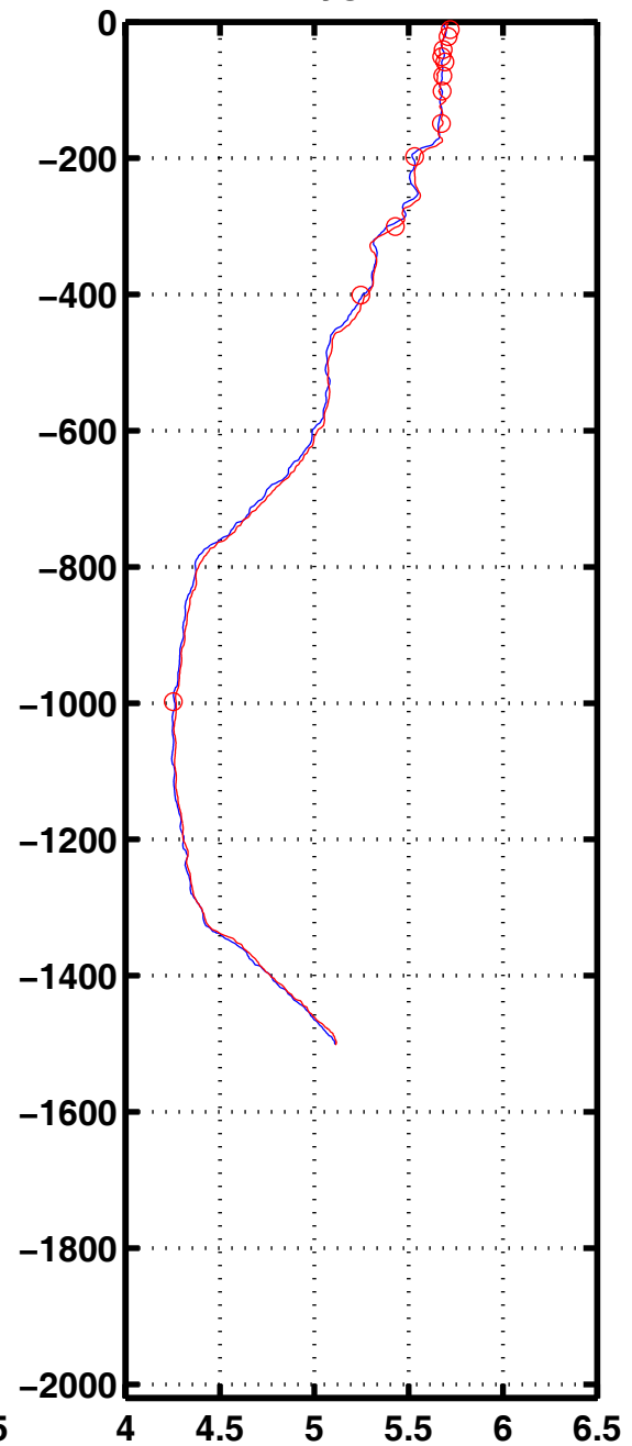
Oxyg 1092
