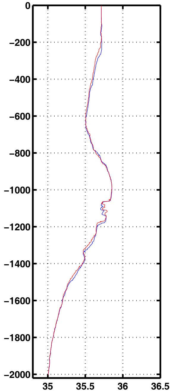
Sali 1177
