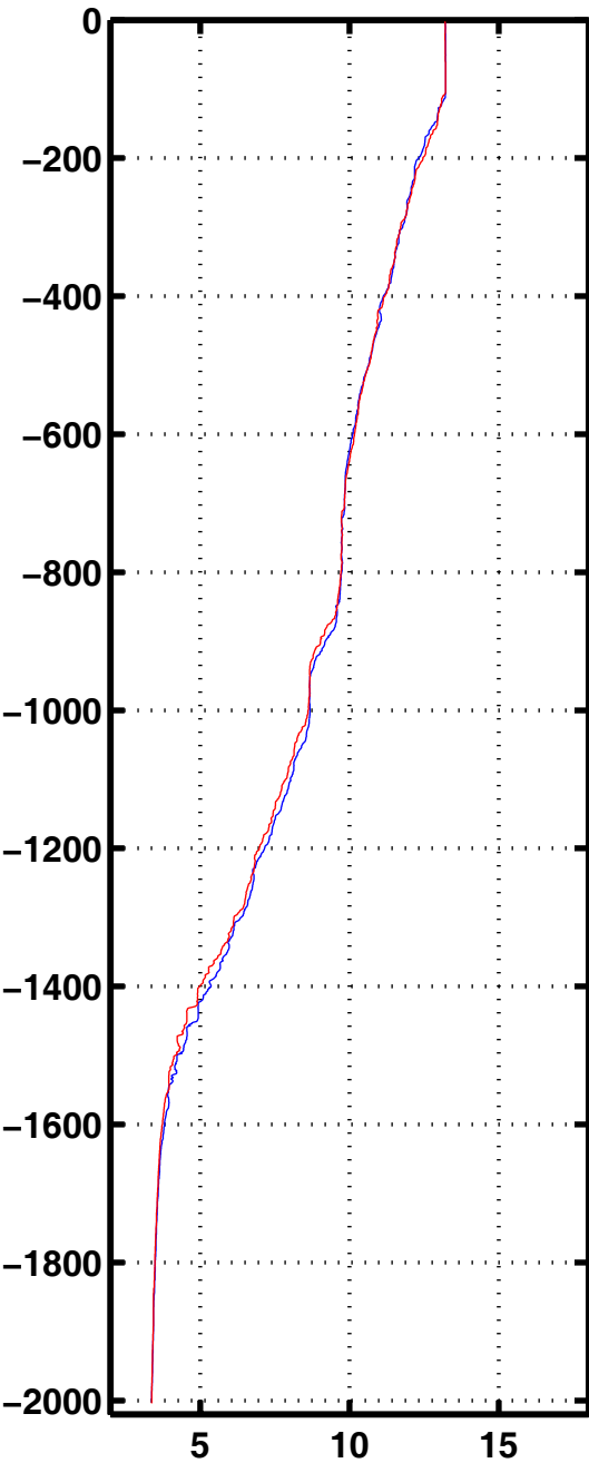
Tempe 1064
