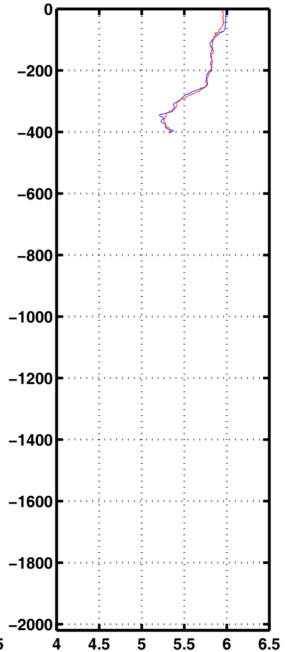
Oxyg 1173
