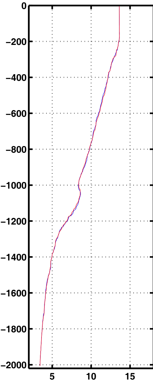
Tempe 1066
