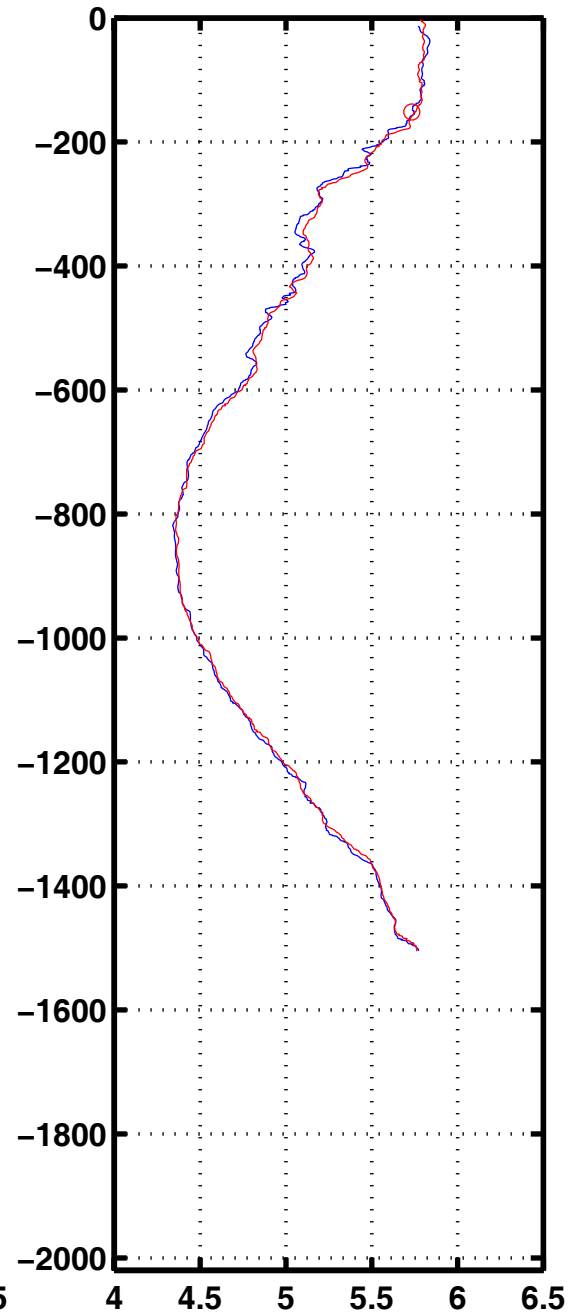
Oxyg 1119
