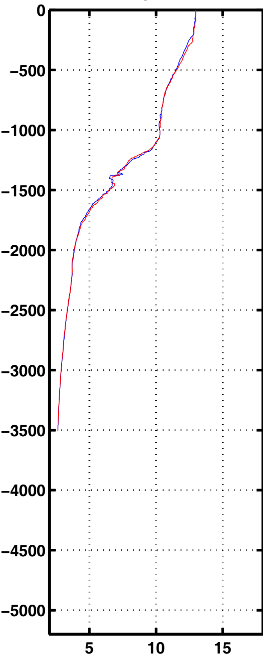
Tempe 1168
