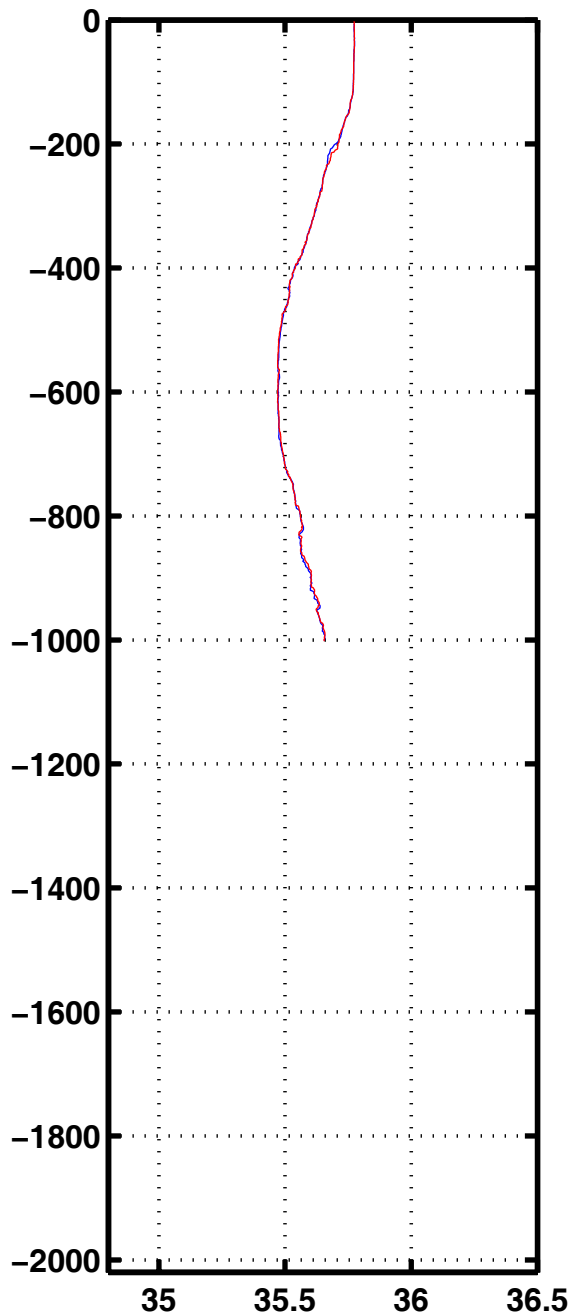
Sali 1129
