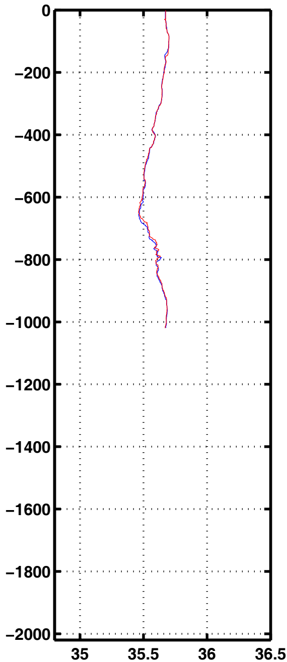
Sali 1192
