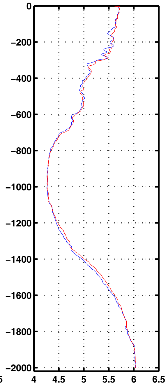
Oxyg 1034
