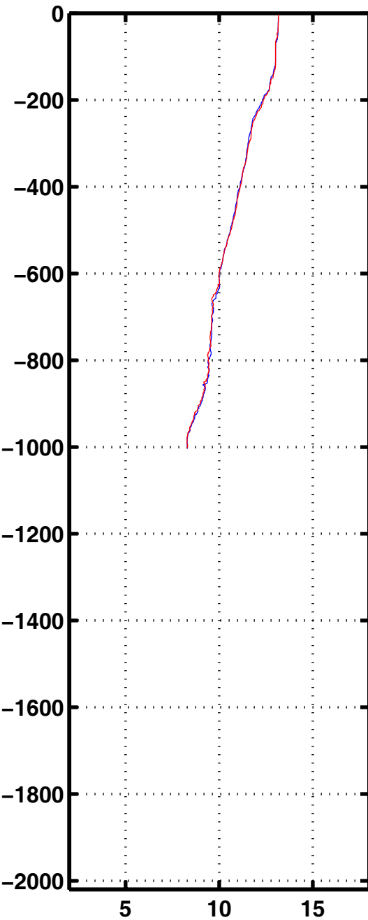
Tempe 1133
