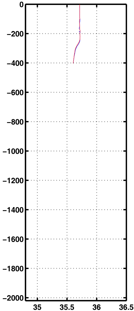
Sali 1175
