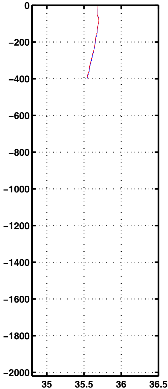
Sali 1184
