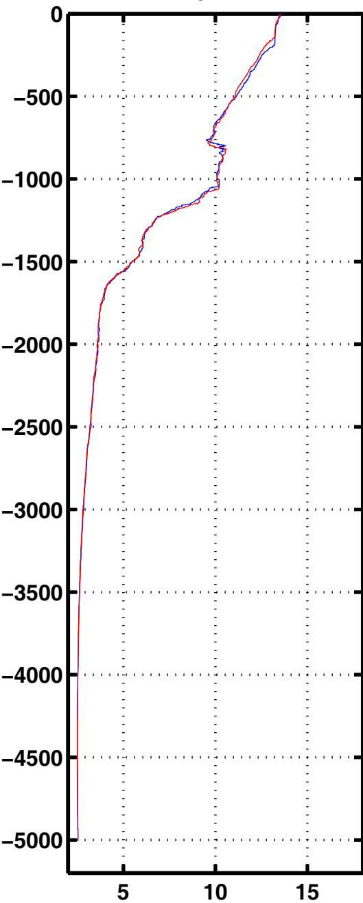
Tempe 1037
