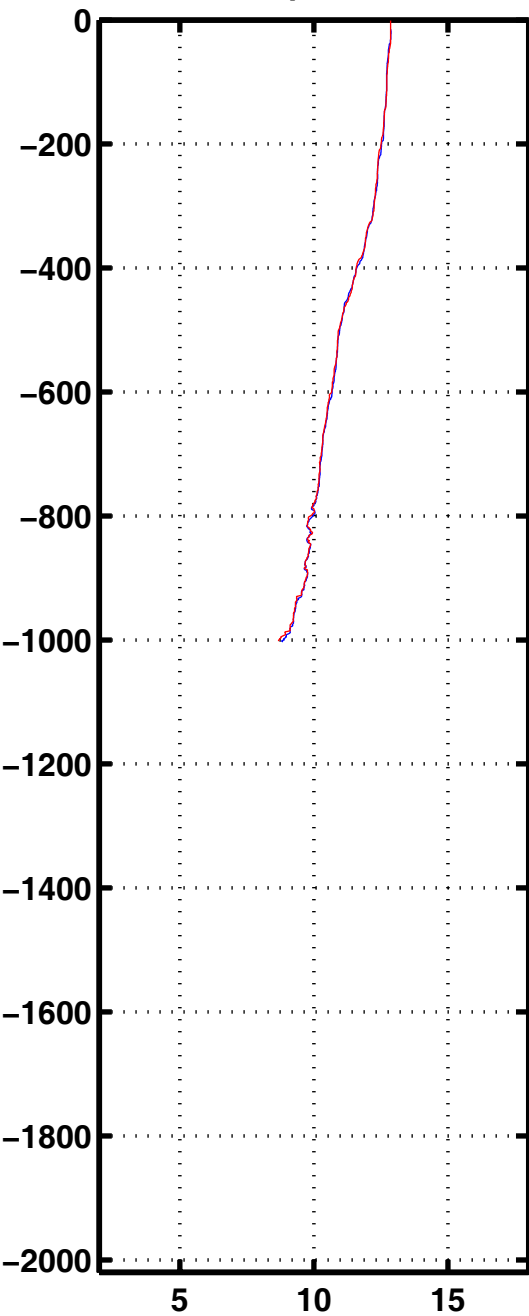
Tempe 1189
