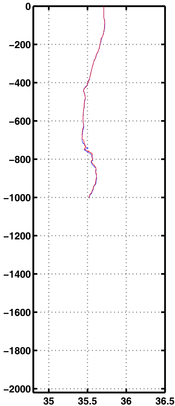
Sali 1151
