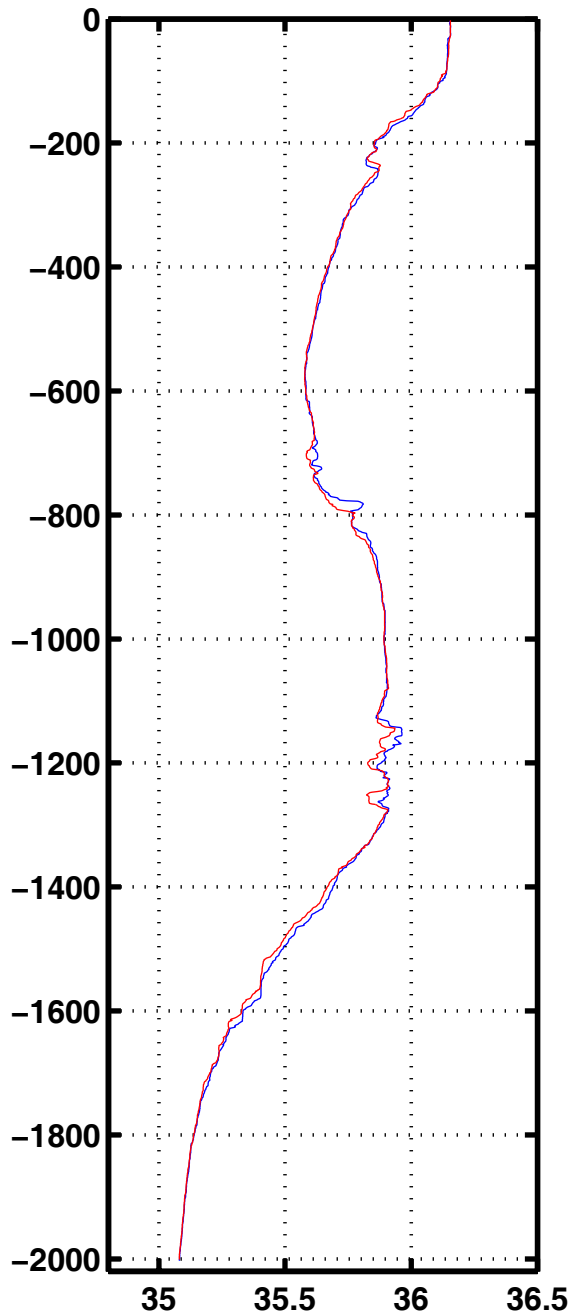
Sali 1058
