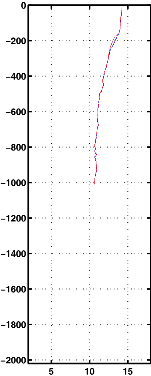
Tempe 1203
