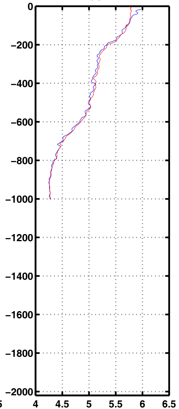
Oxyg 1101
