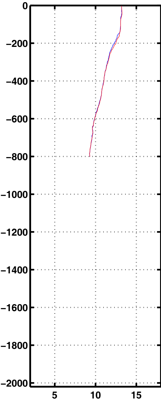
Tempe 1147
