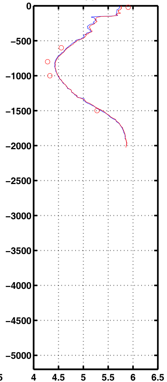
Oxyg 1002
