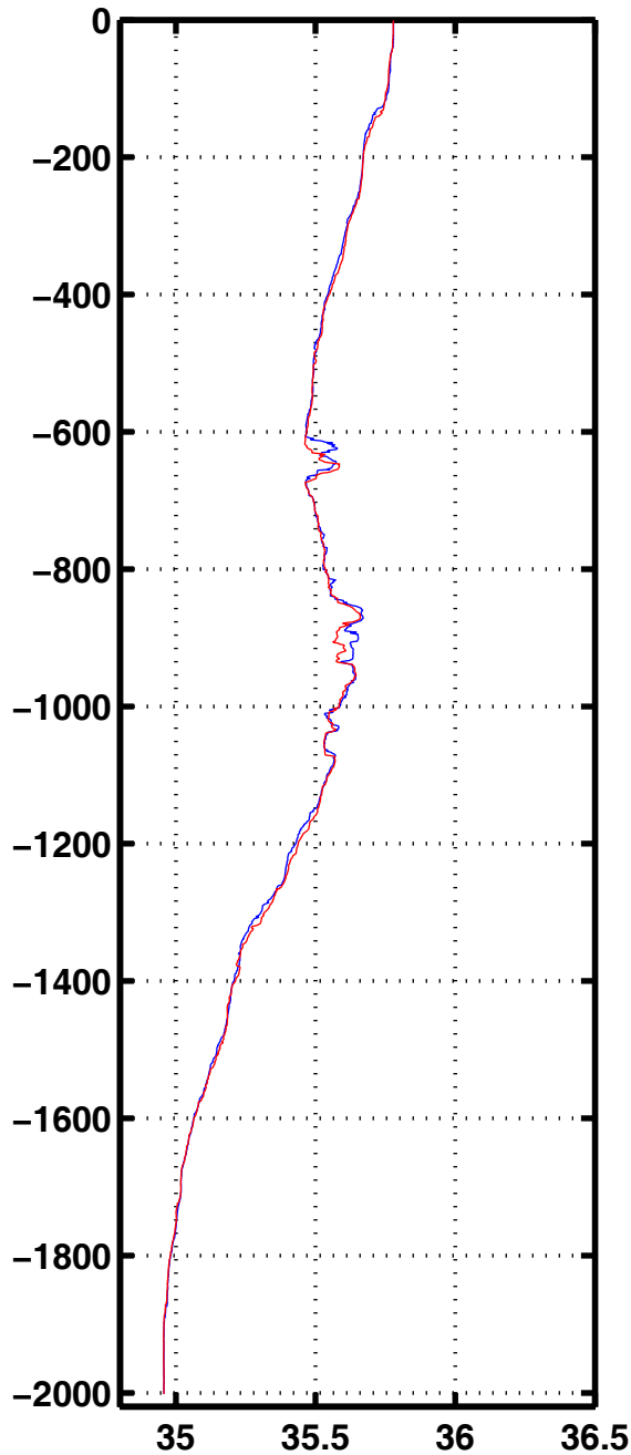
Sali 1038
