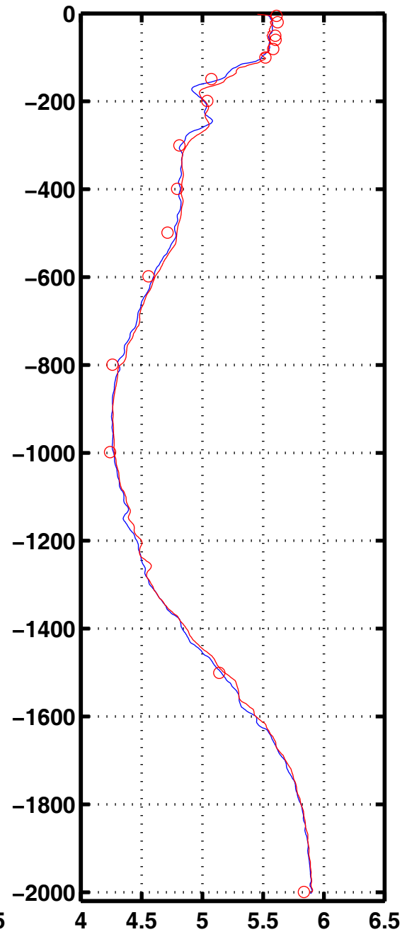
Oxyg 1058
