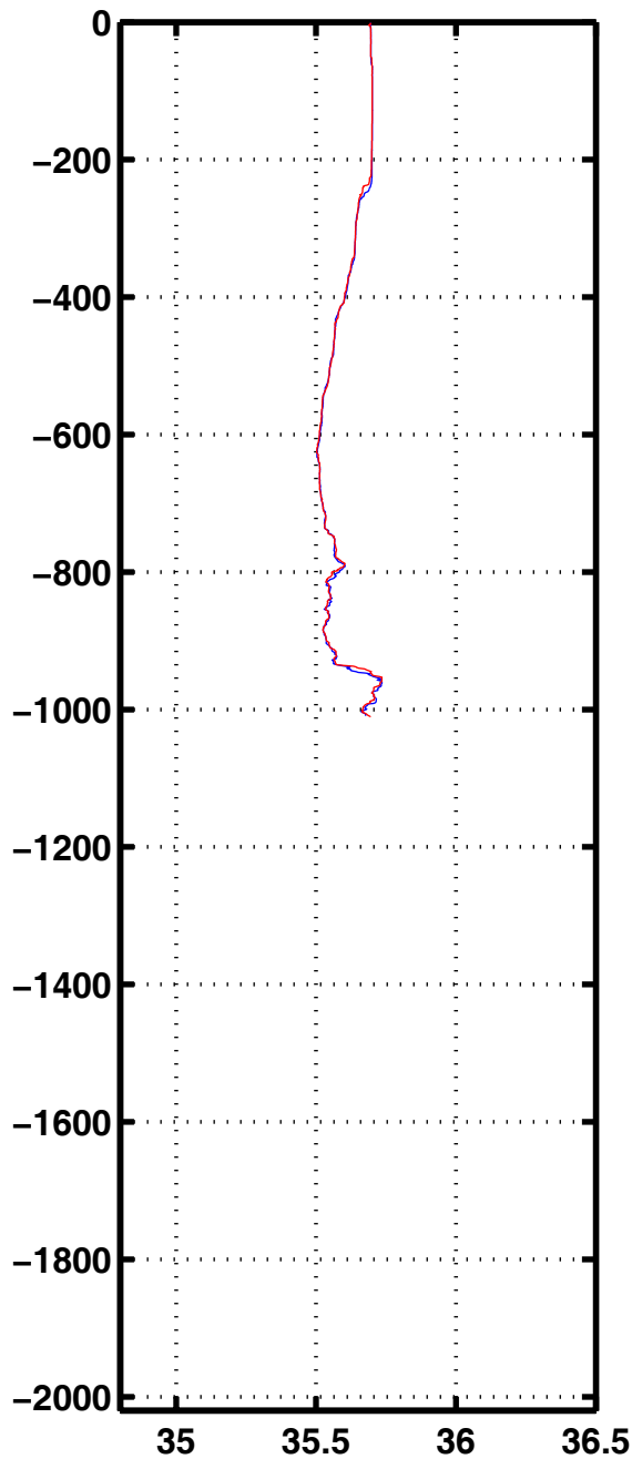
Sali 1159
