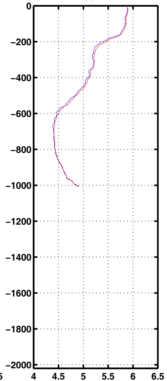
Oxyg 1136
