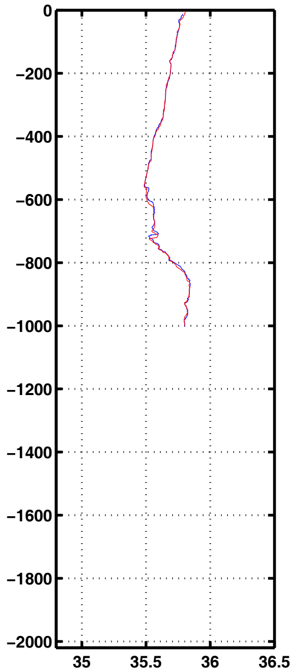
Sali 1194
