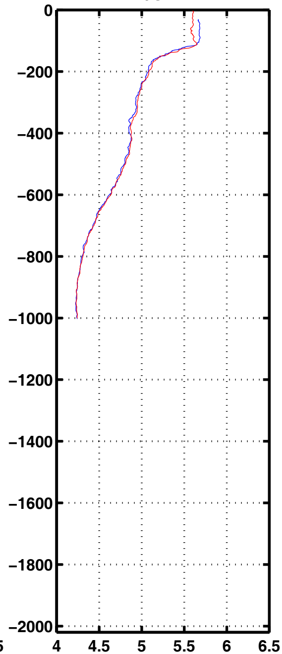
Oxyg 1123
