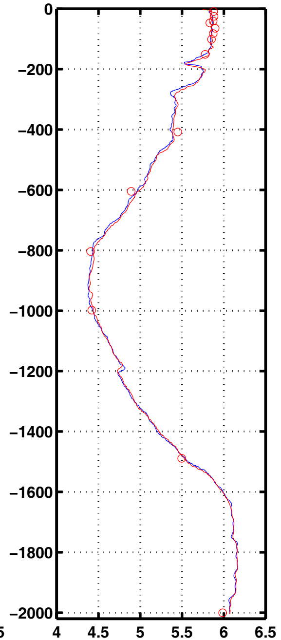
Oxyg 1024
