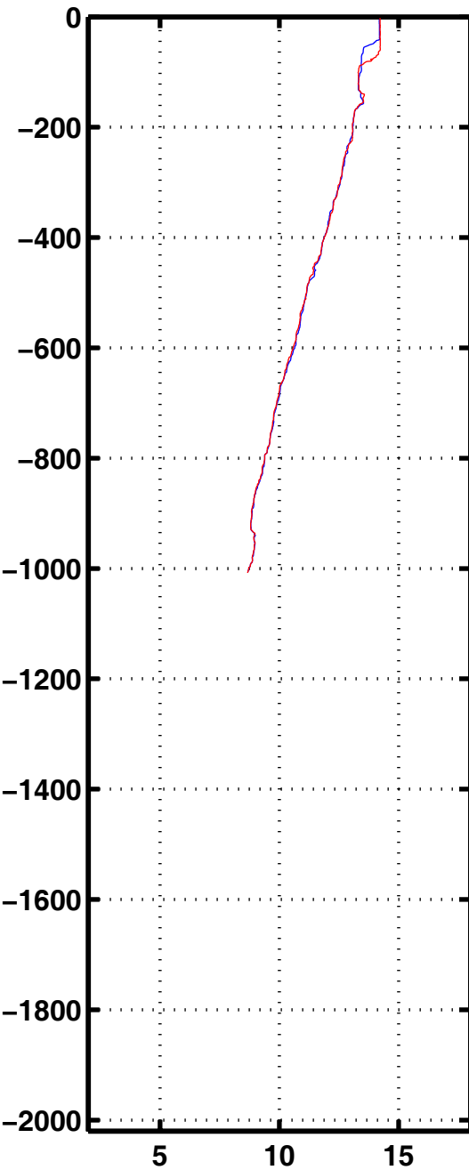
Tempe 1156
