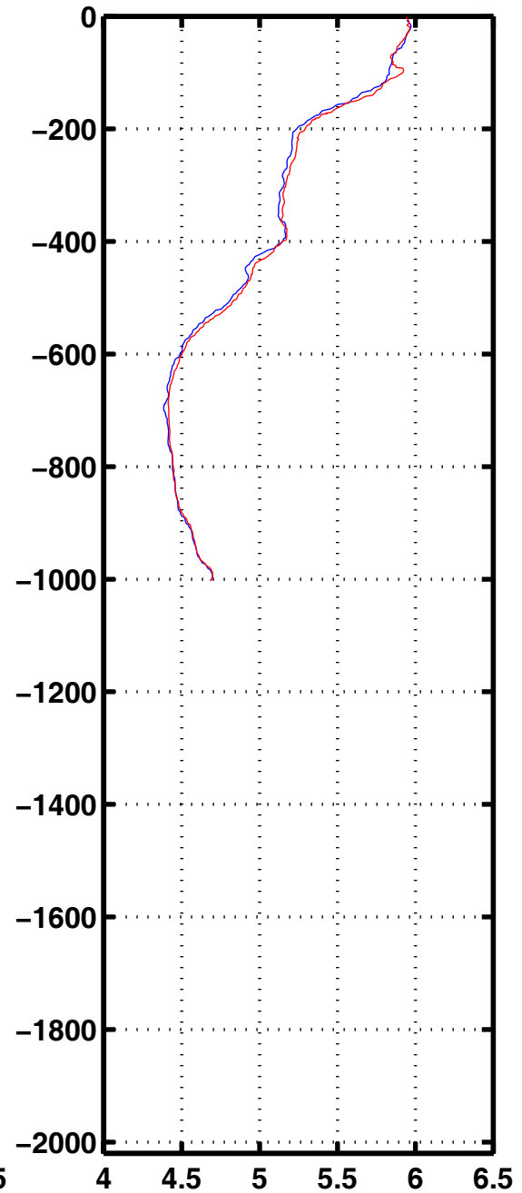
Oxyg 1152
