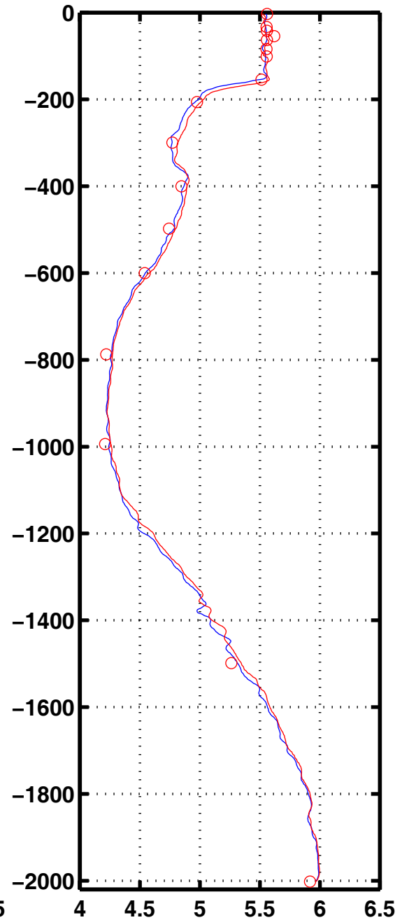
Oxyg 1079
