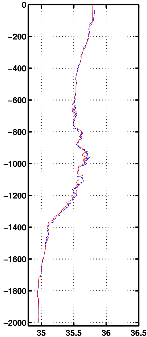
Sali 1115
