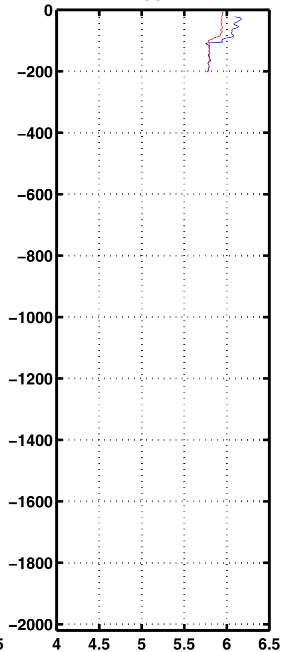
Oxyg 1180
