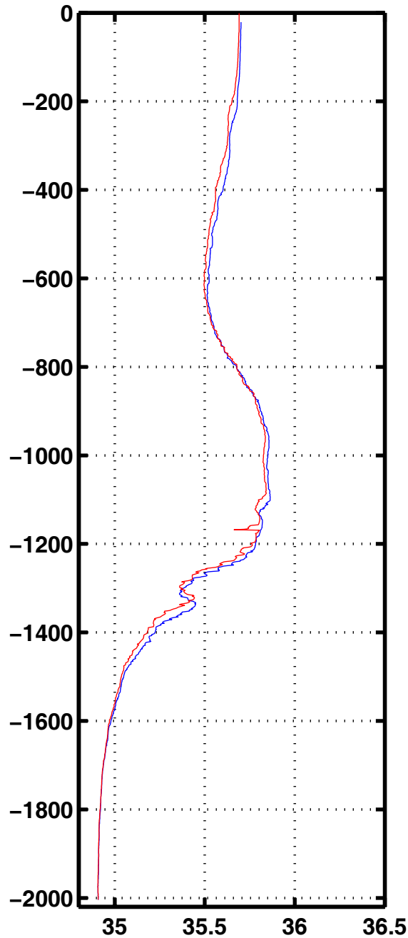
Sali 1010
