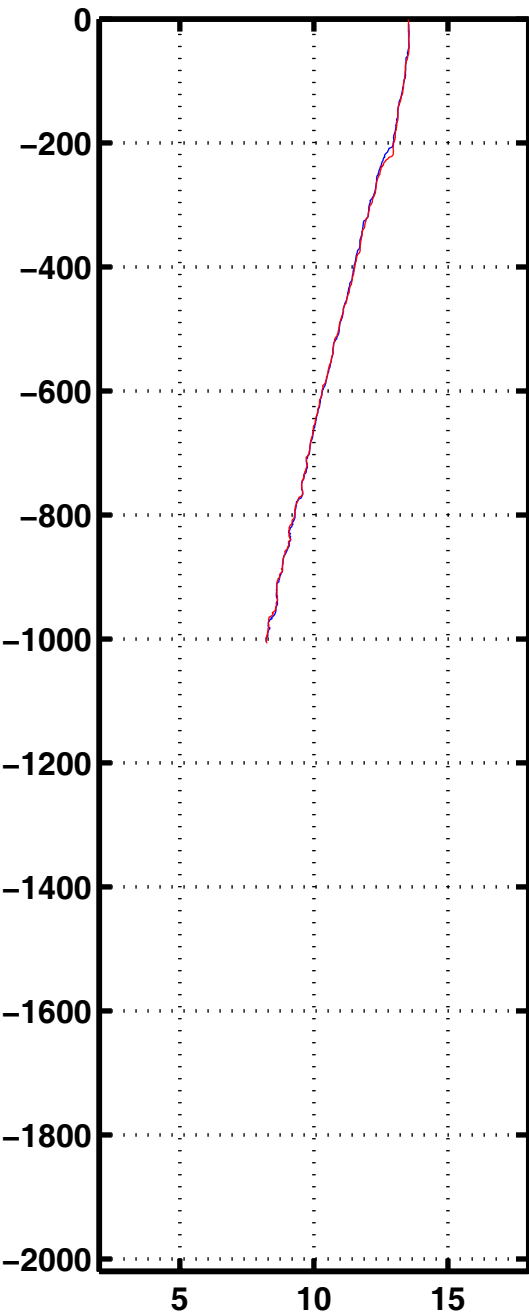
Tempe 1154
