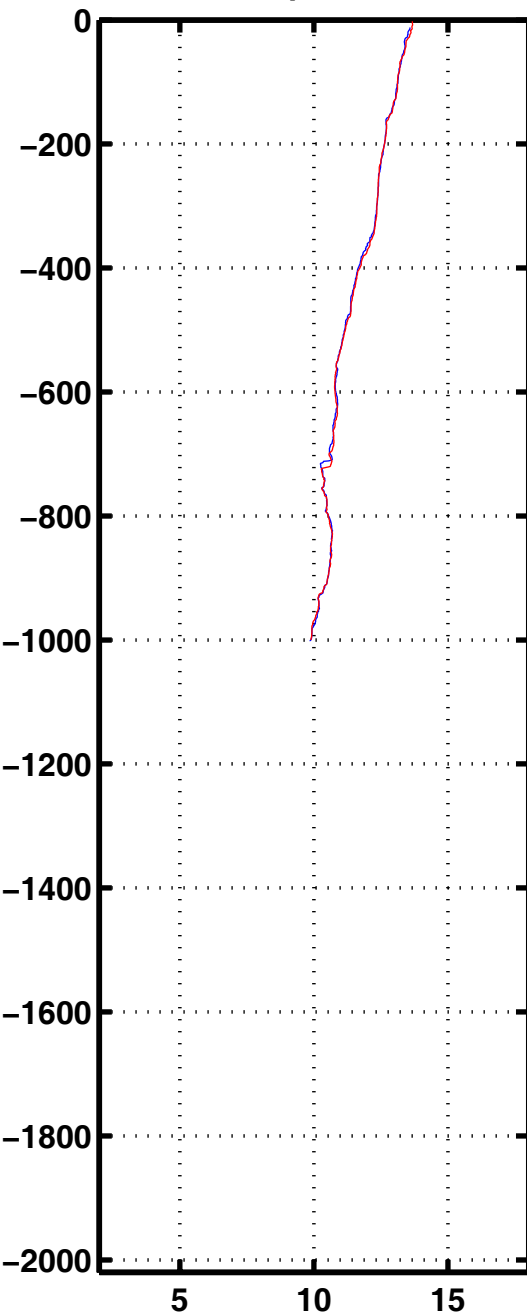
Tempe 1194
