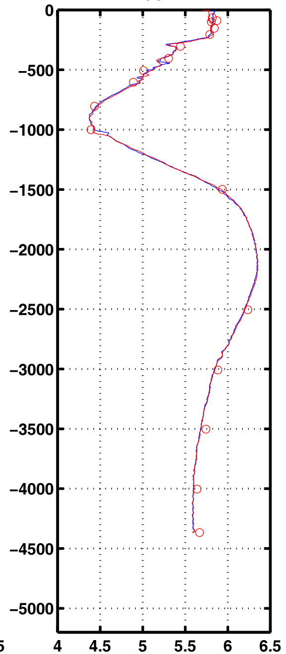
Oxyg 1014
