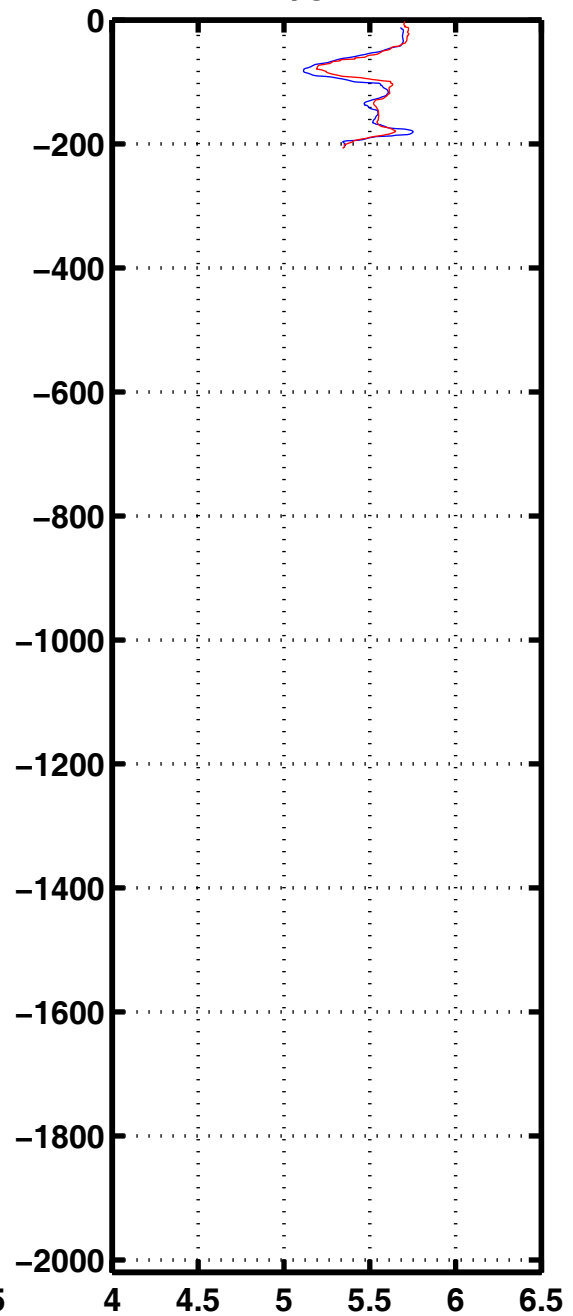
Oxyg 1108
