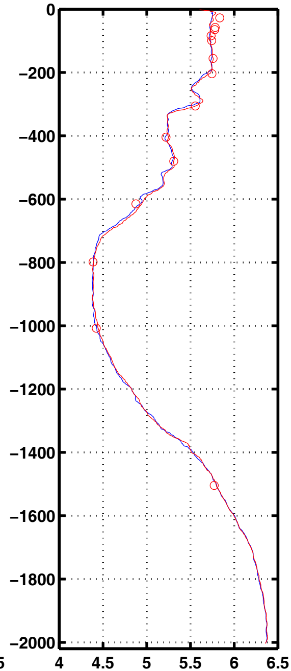
Oxyg 1020
