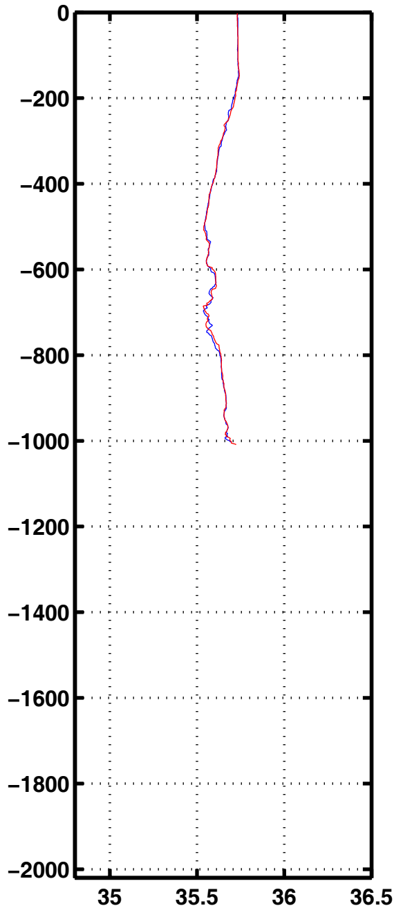
Sali 1197
