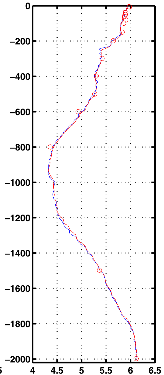
Oxyg 1041
