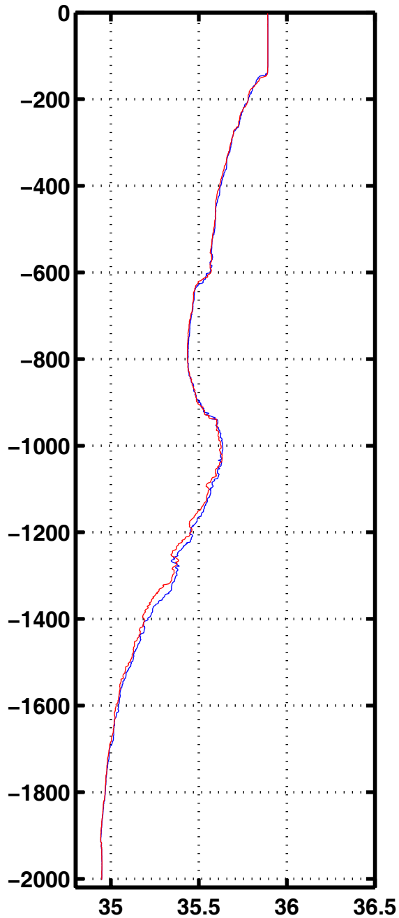
Sali 1072
