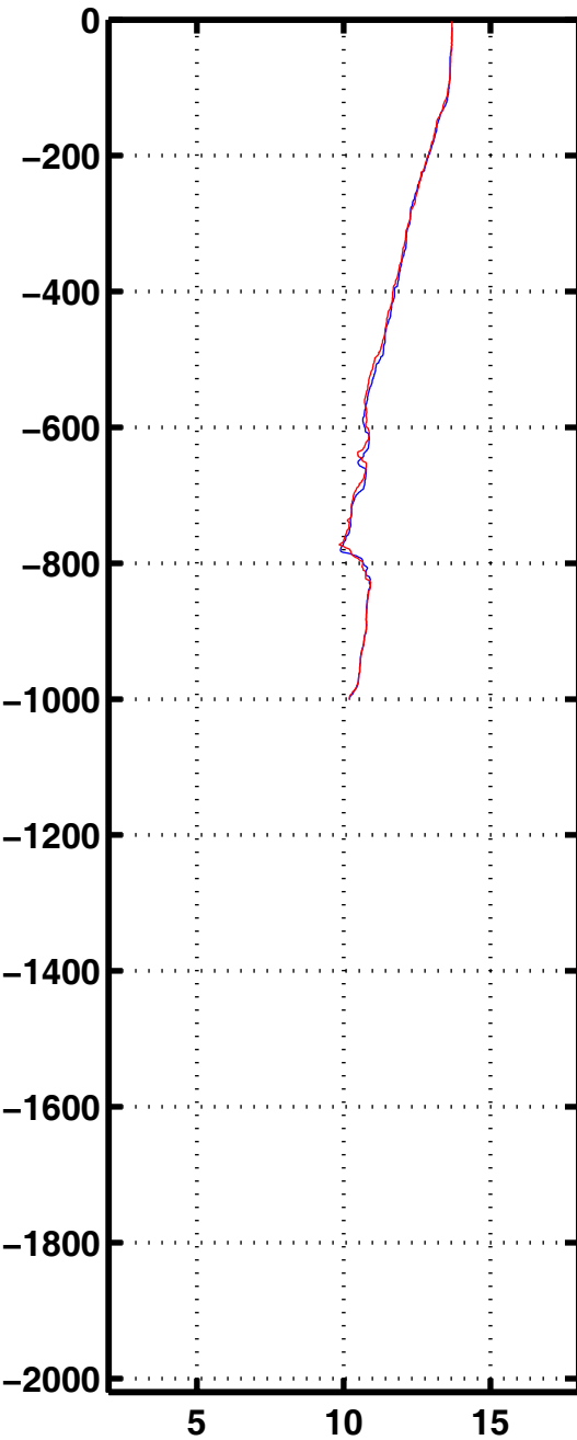
Tempe 1200
