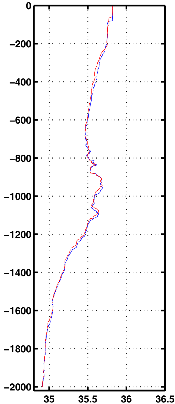
Sali 1069
