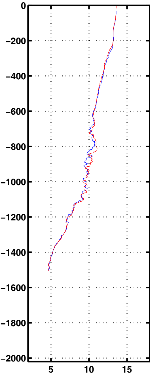
Tempe 1114
