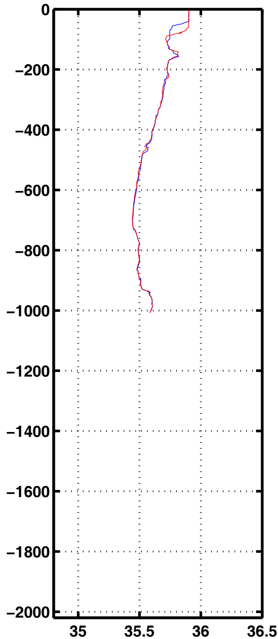
Sali 1156
