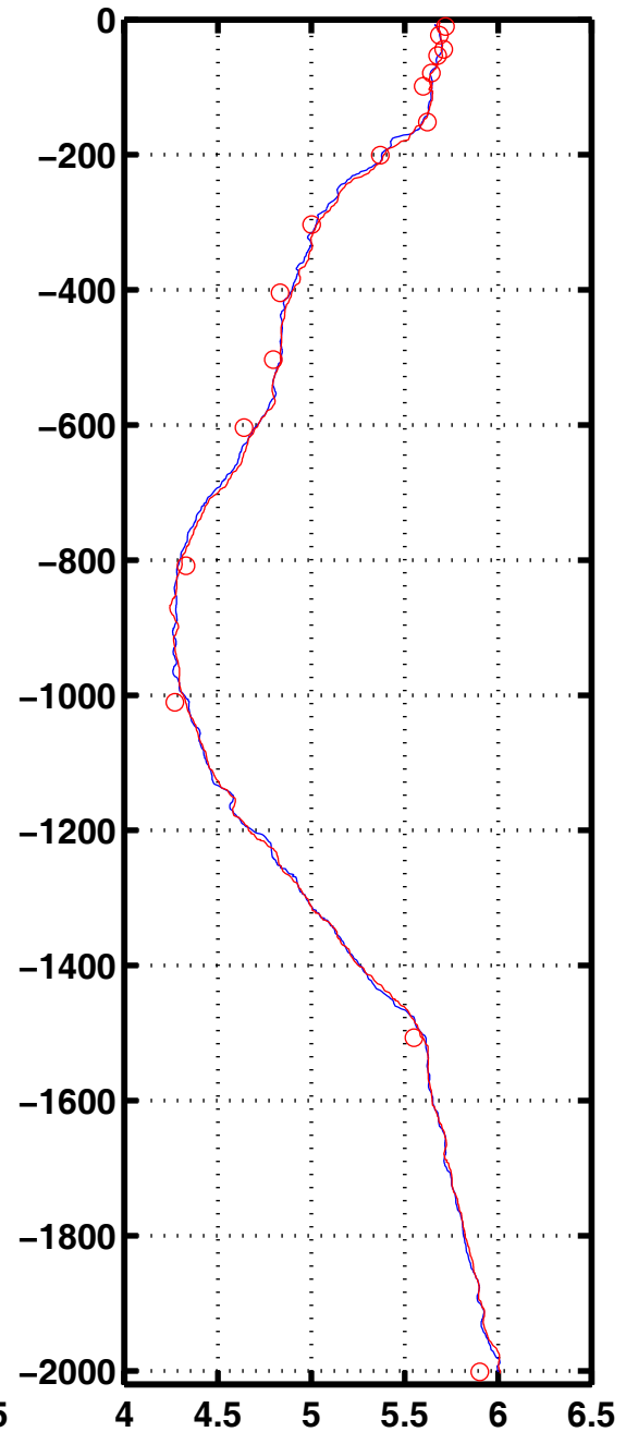
Oxyg 1028
