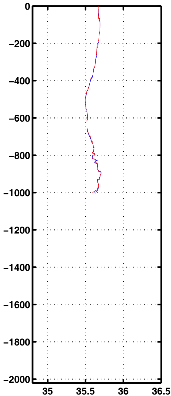
Sali 1189
