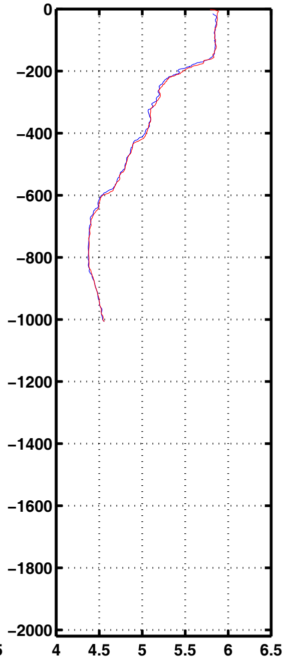
Oxyg 1131
