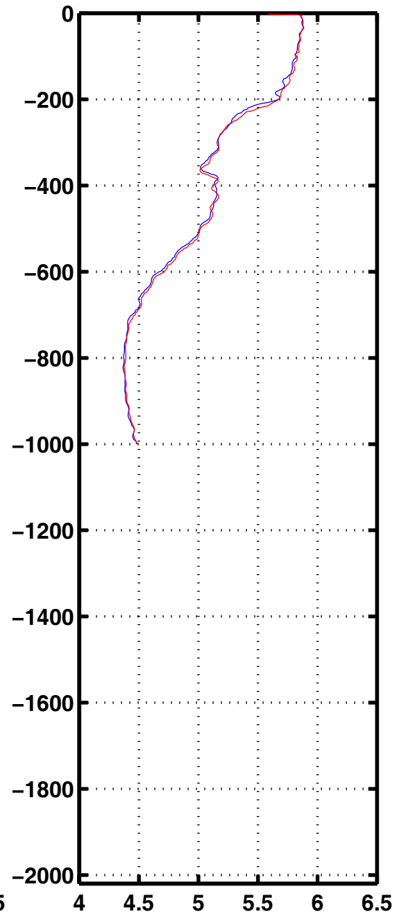
Oxyg 1198
