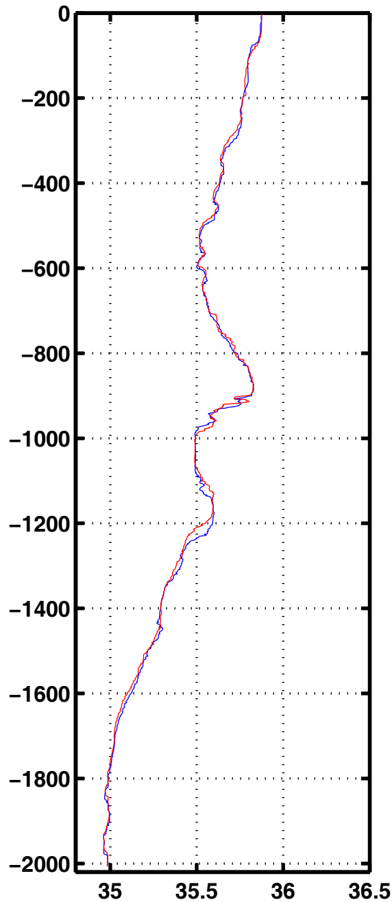
Sali 1027
