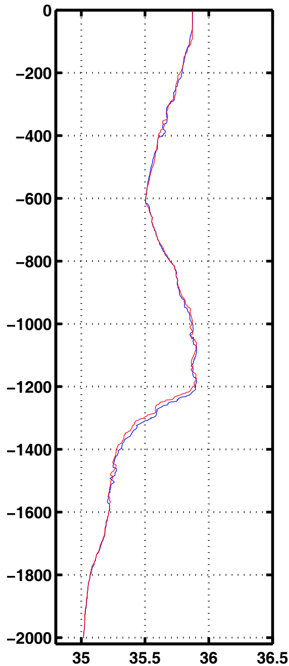
Sali 1055
