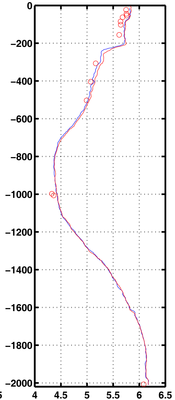
Oxyg 1030
