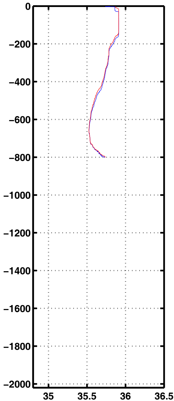
Sali 1091
