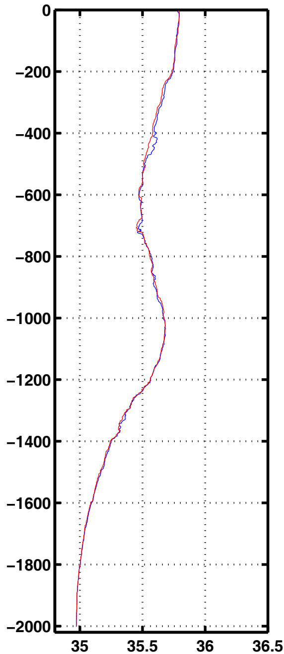
Sali 1048
