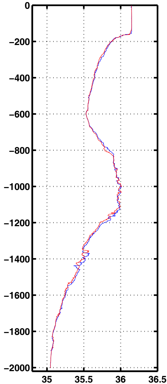
Sali 1079
