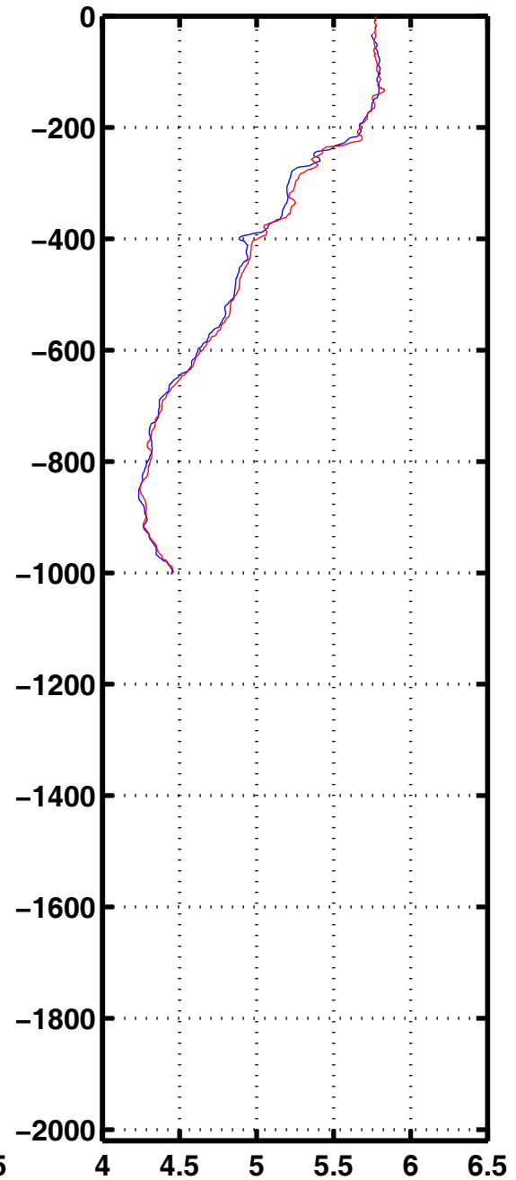
Oxyg 1113
