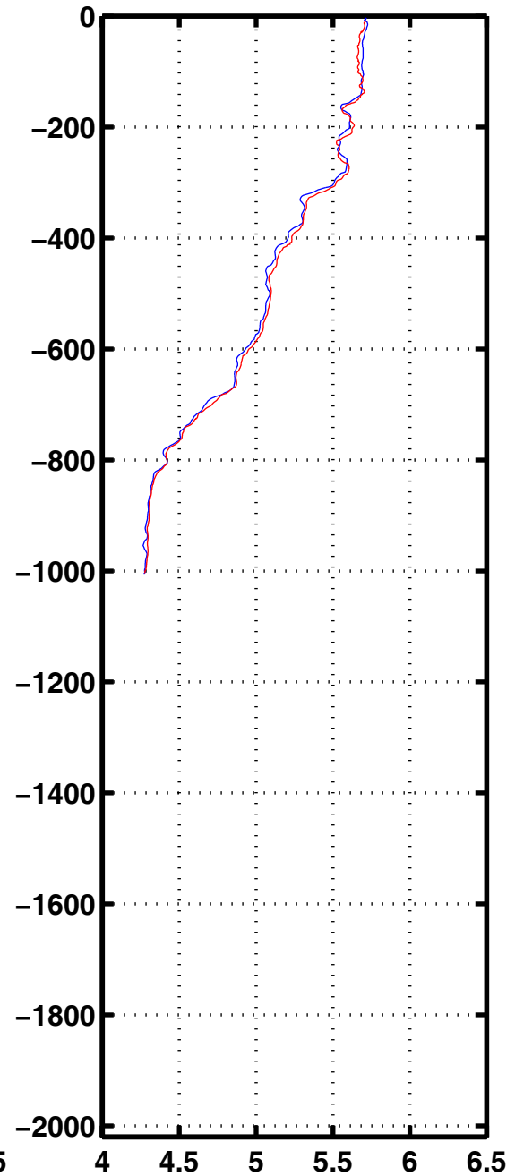
Oxyg 1084
