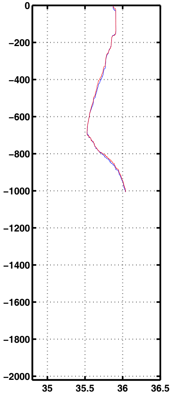
Sali 1086
