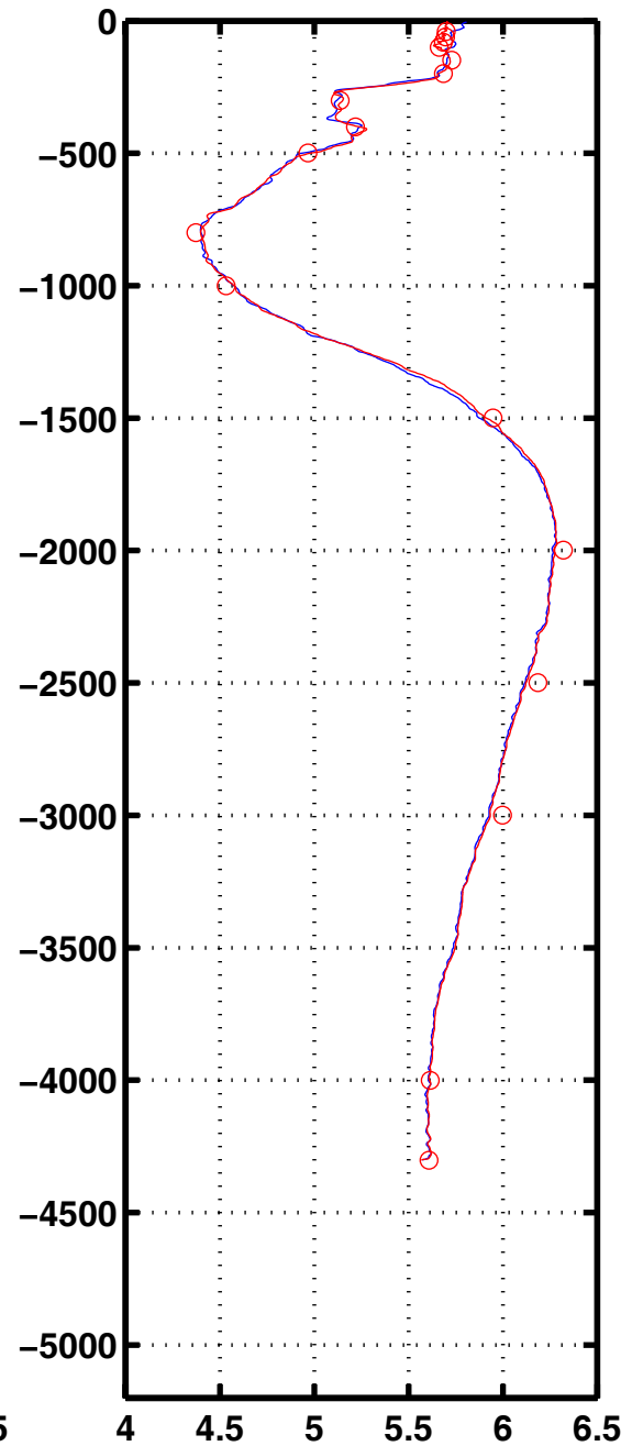
Oxyg 1045
