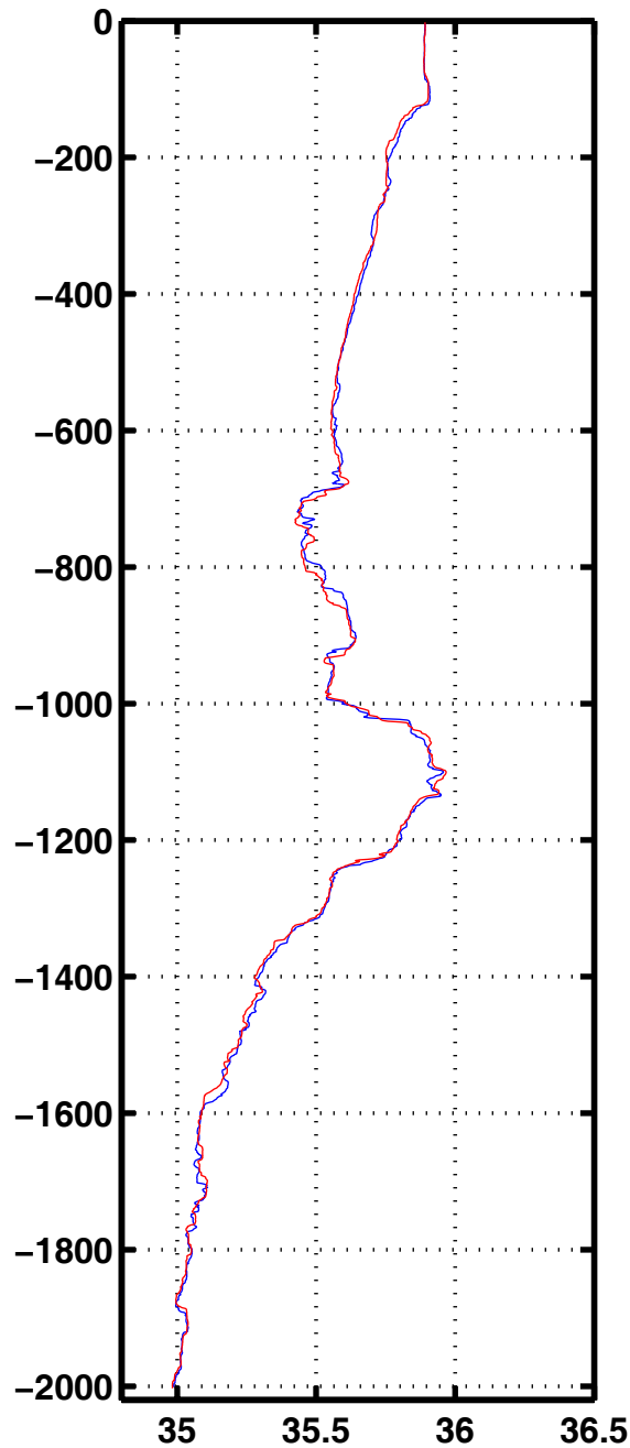
Sali 1036
