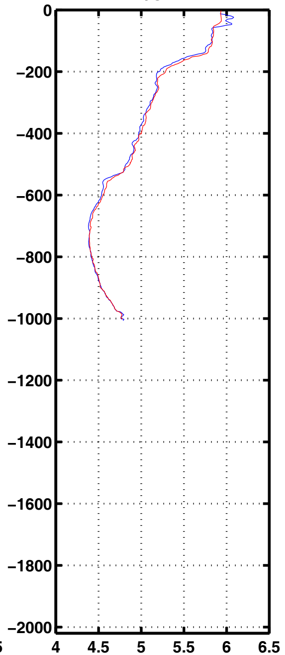
Oxyg 1142
