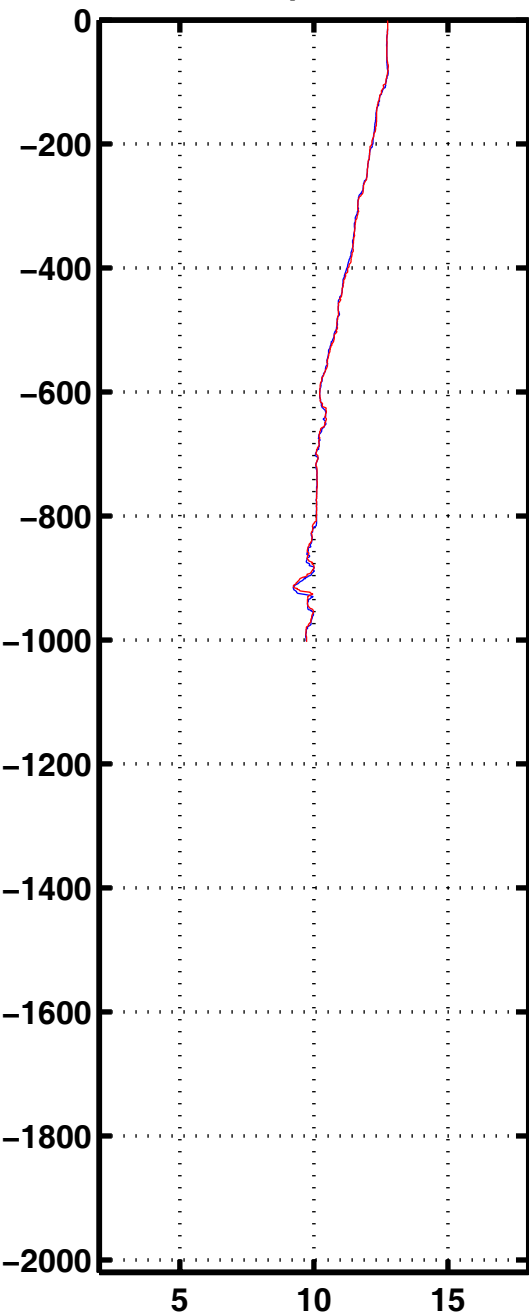
Tempe 1186
