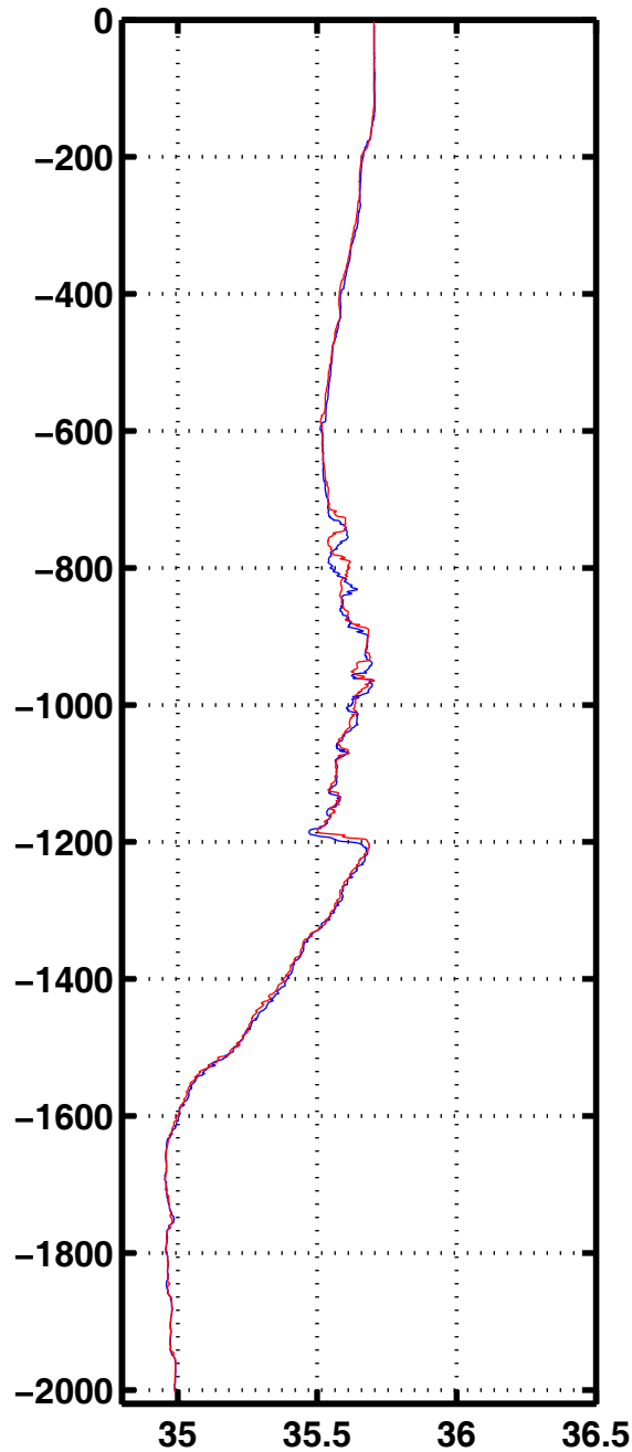
Sali 1024
