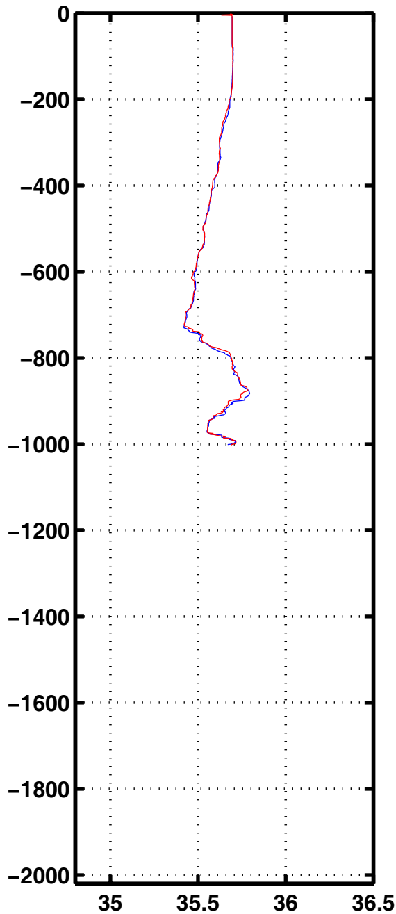
Sali 1158
