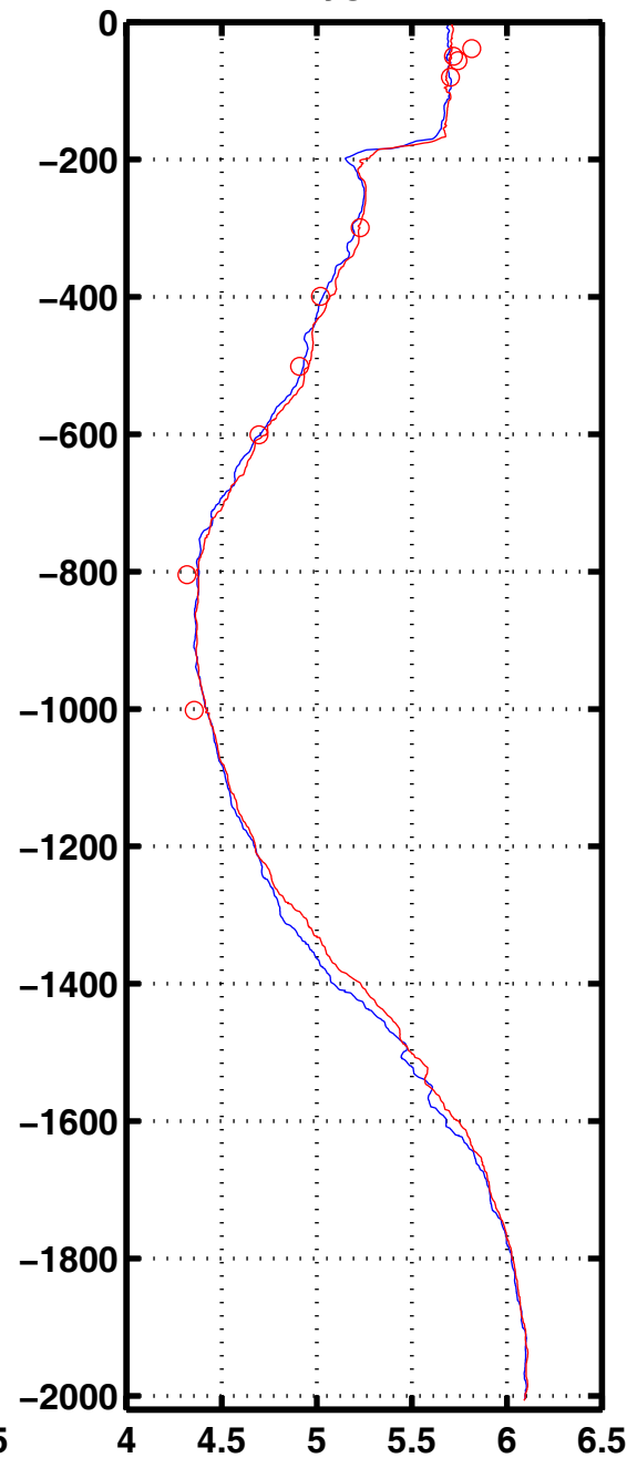
Oxyg 1004
