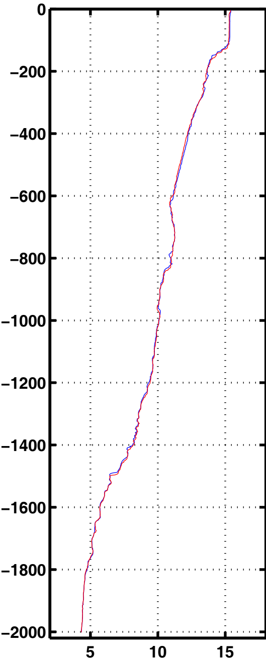
Tempe 1057
