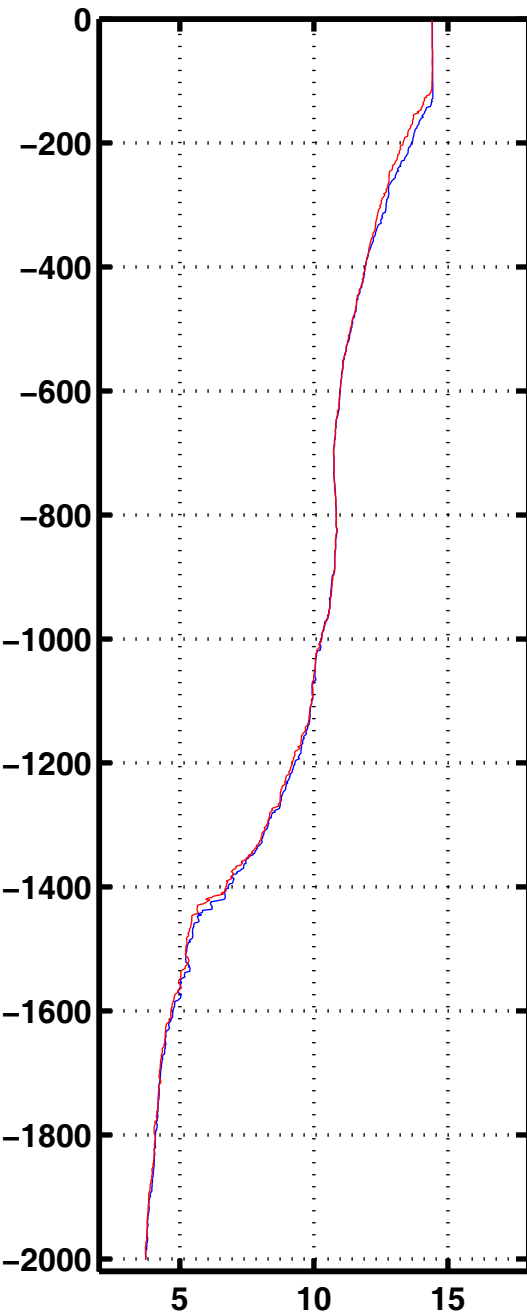
Tempe 1073
