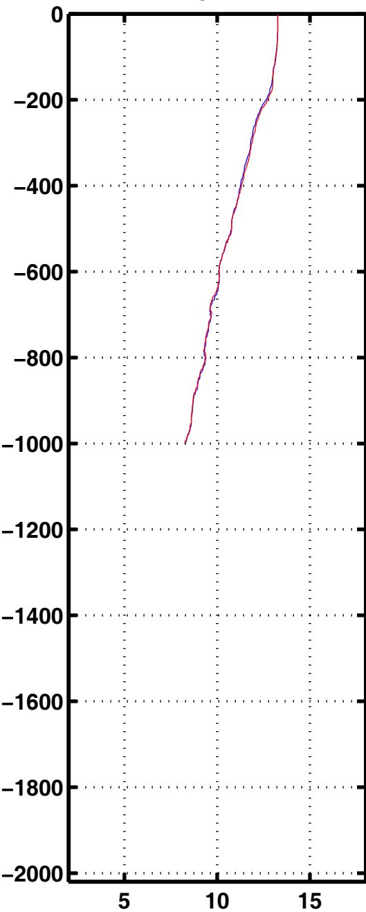
Tempe 1132
