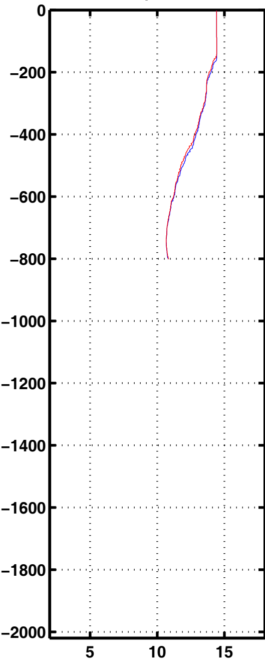
Tempe 1091
