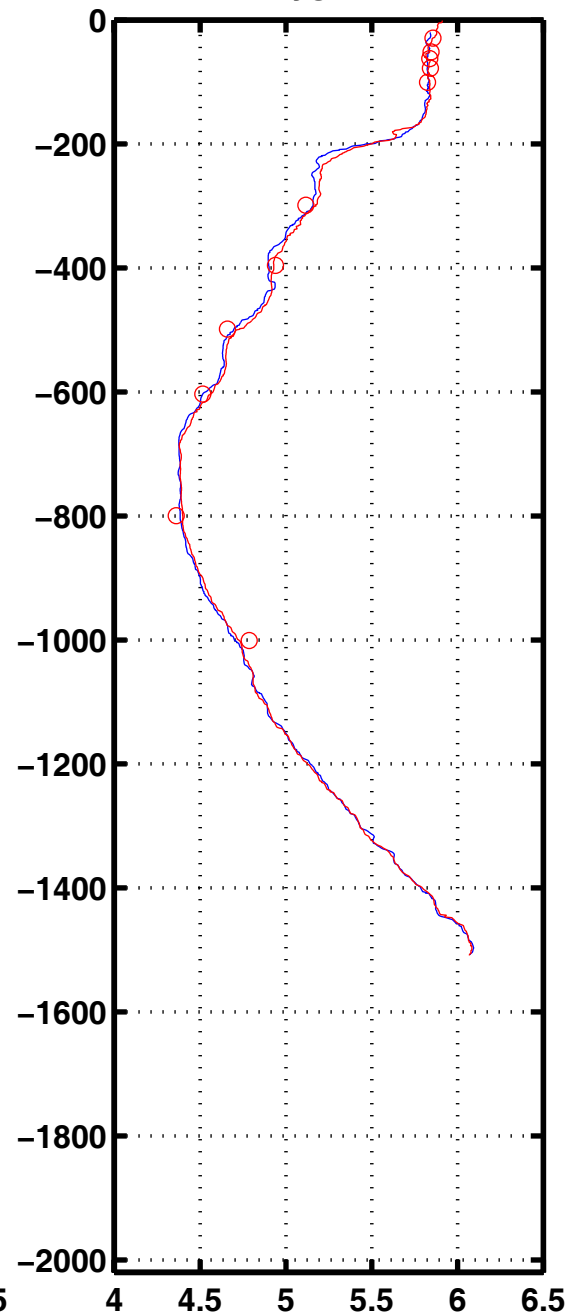
Oxyg 1139
