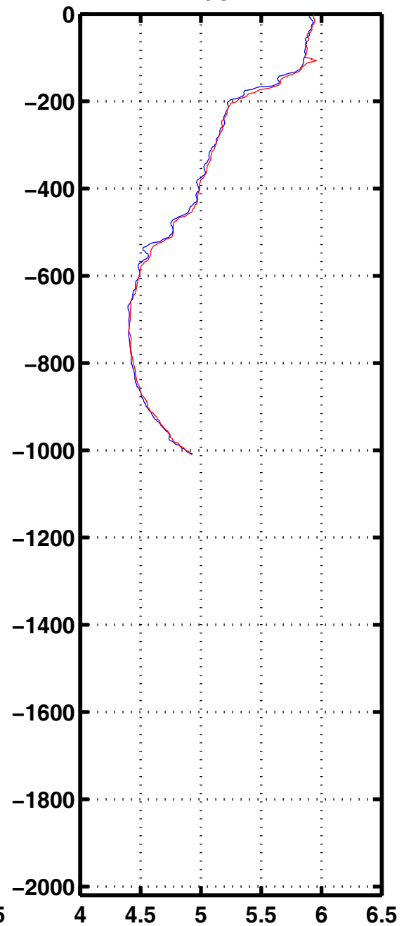
Oxyg 1135
