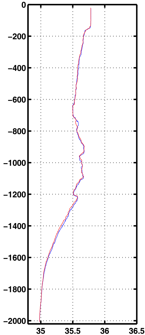
Sali 1007
