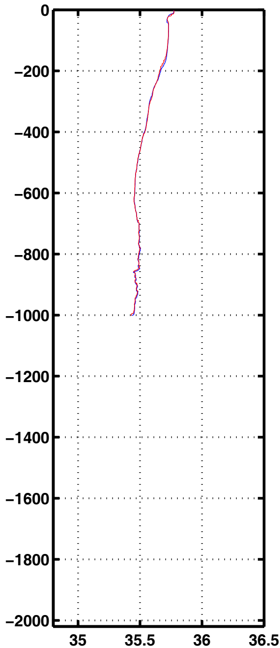
Sali 1105
