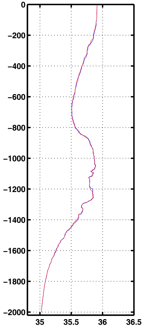
Sali 1054
