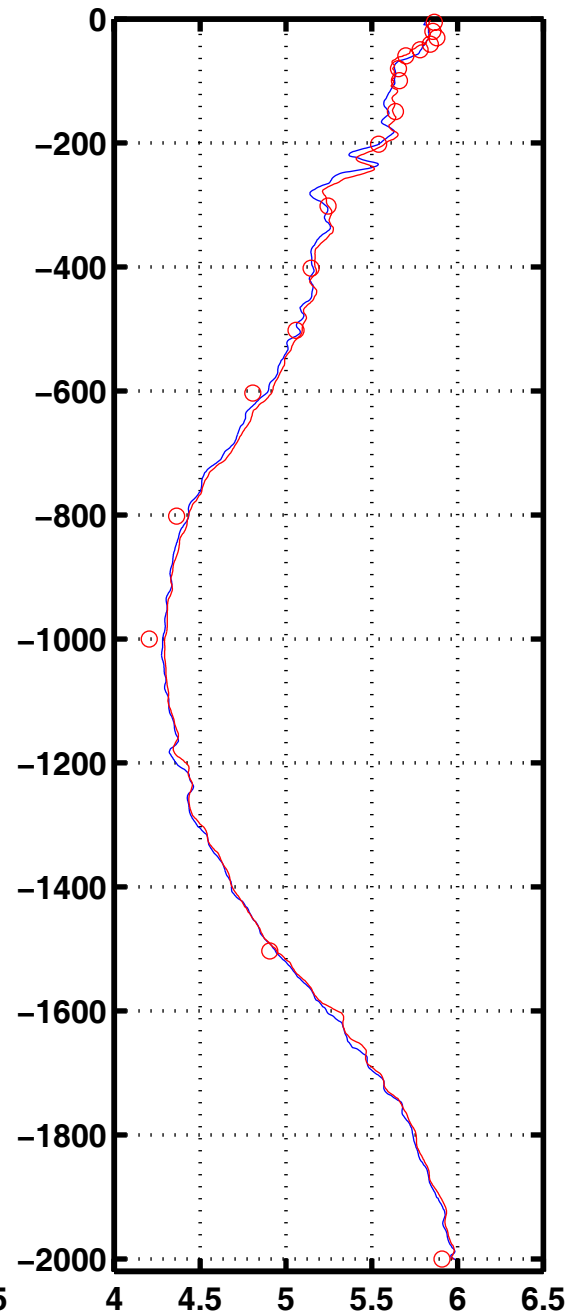
Oxyg 1053
