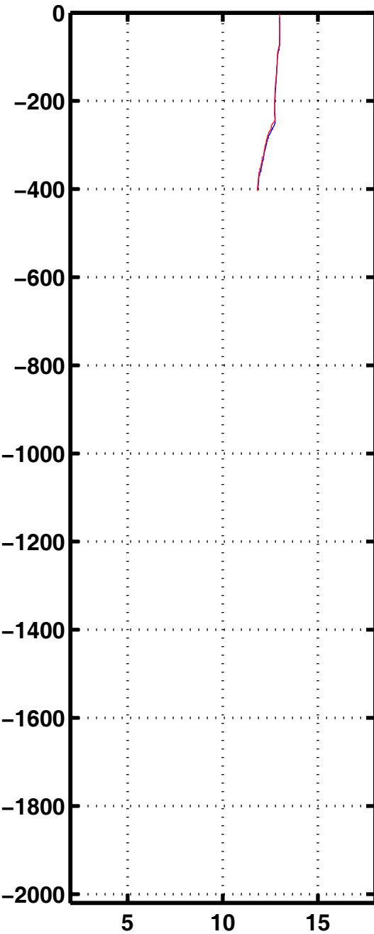
Tempe 1173
