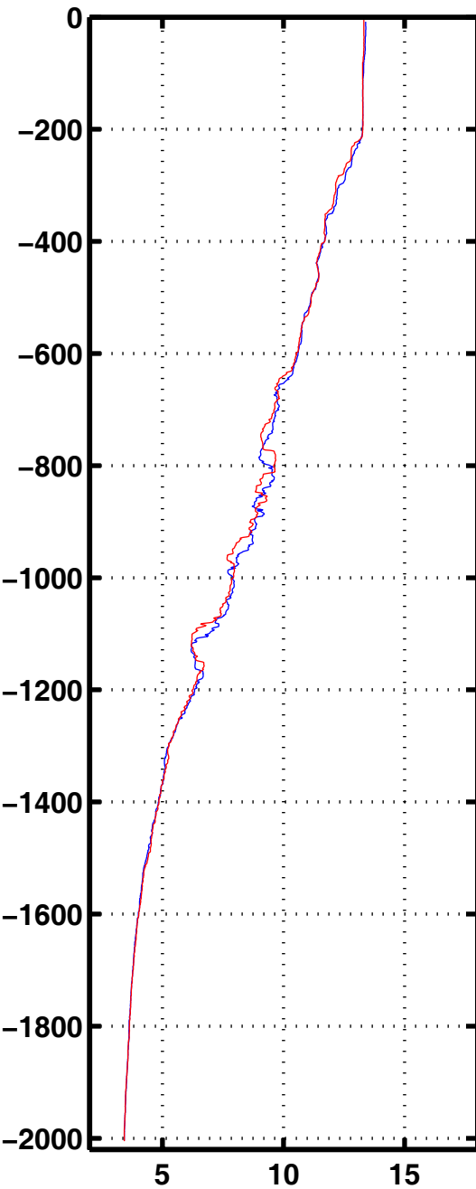
Tempe 1016
