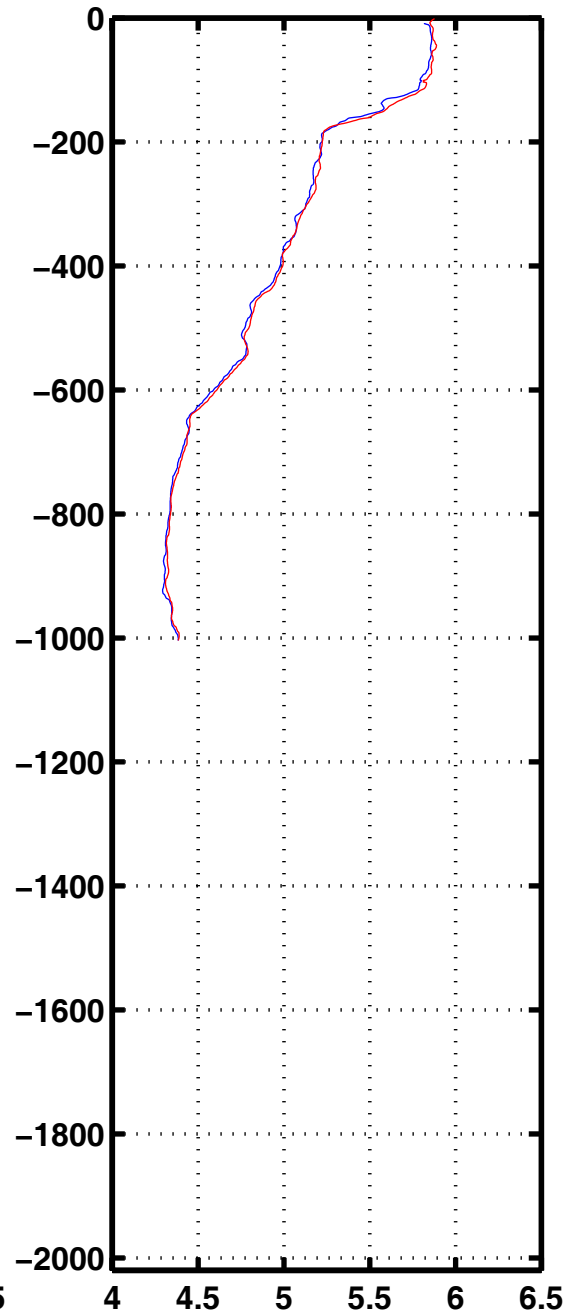
Oxyg 1202
