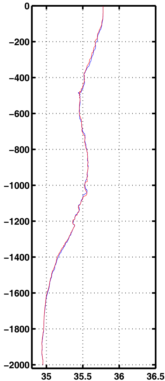
Sali 1050
