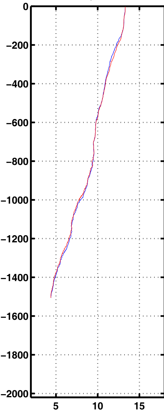
Tempe 1141
