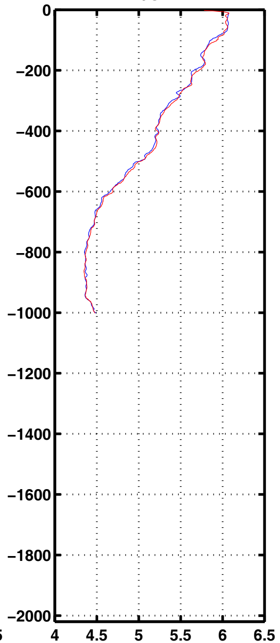
Oxyg 1193
