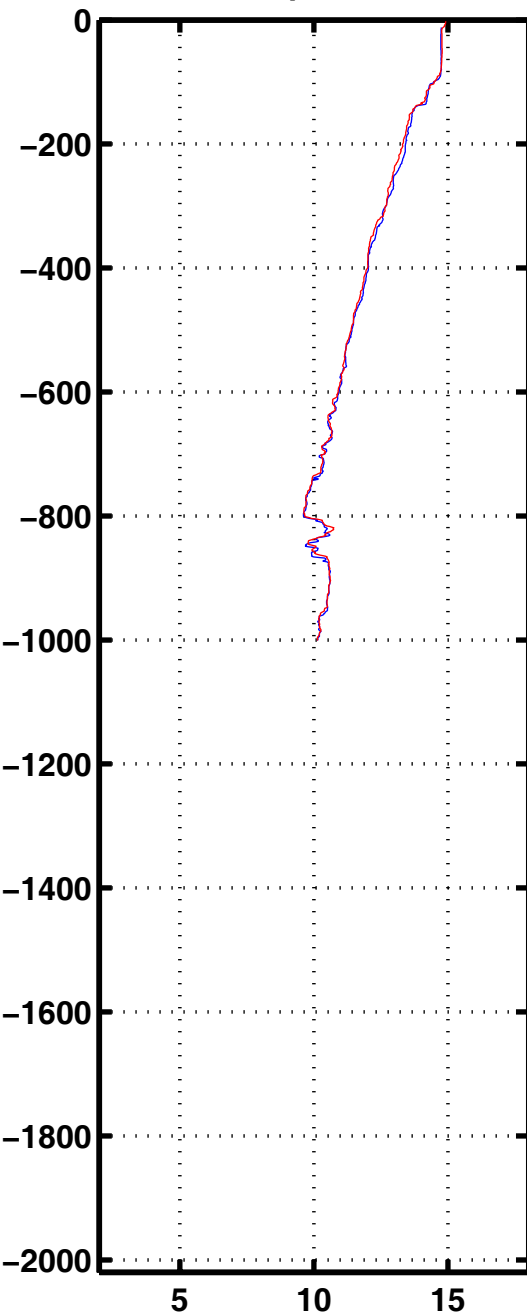
Tempe 1103
