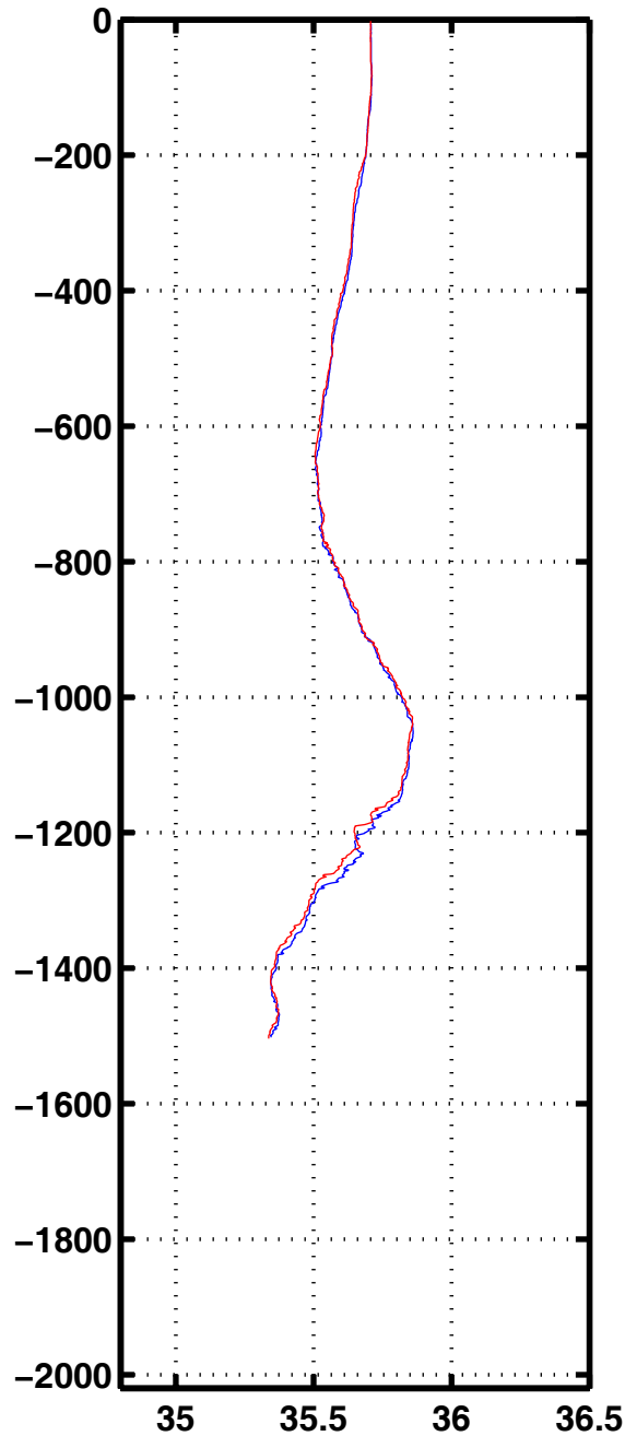
Sali 1167
