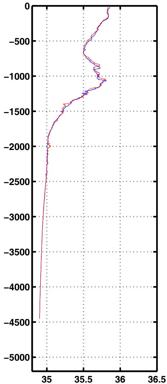
Sali 1032
