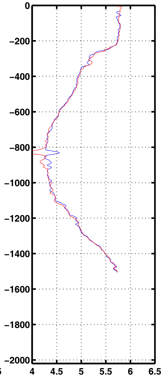
Oxyg 1114
