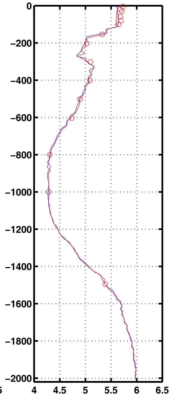
Oxyg 1060
