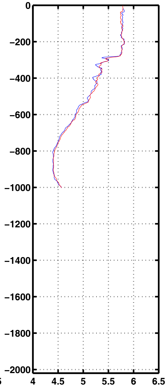
Oxyg 1125
