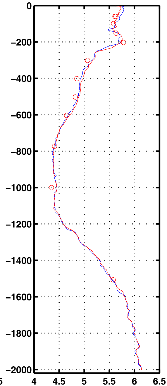
Oxyg 1036
