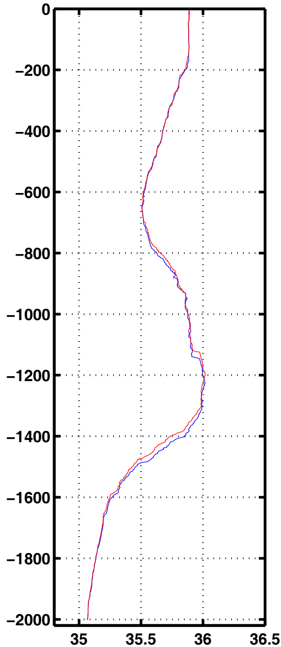
Sali 1059
