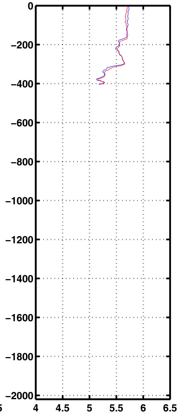
Oxyg 1090
