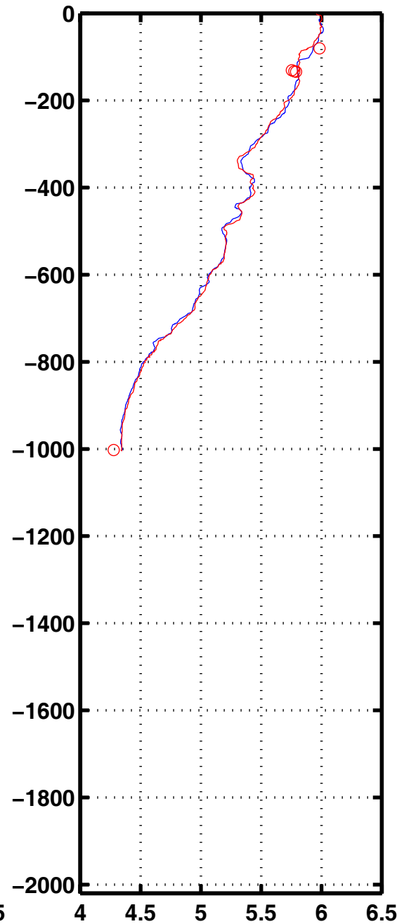
Oxyg 1169
