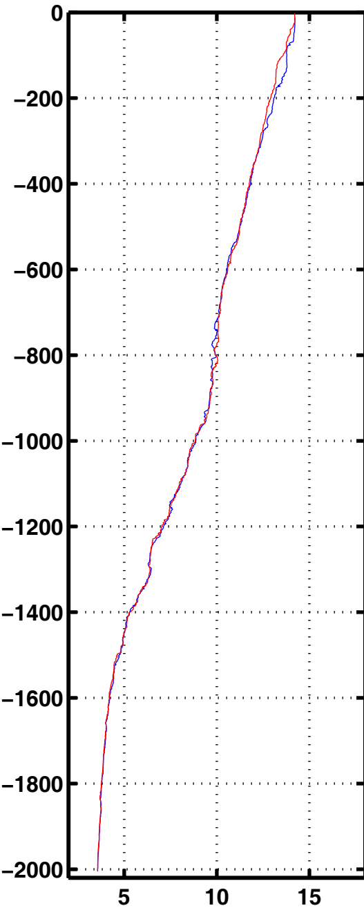
Tempe 1118
