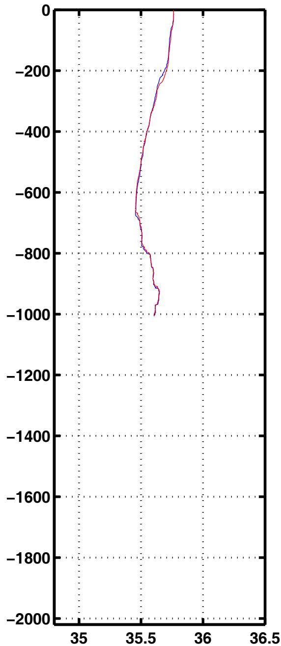
Sali 1128
