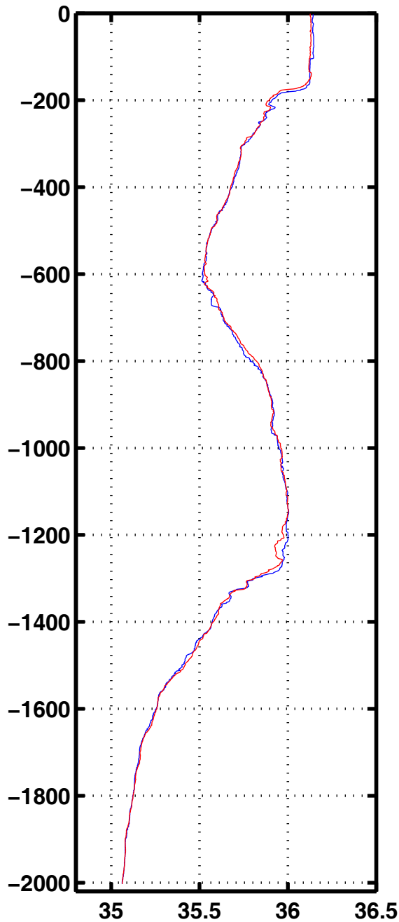
Sali 1077
