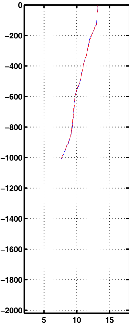
Tempe 1135
