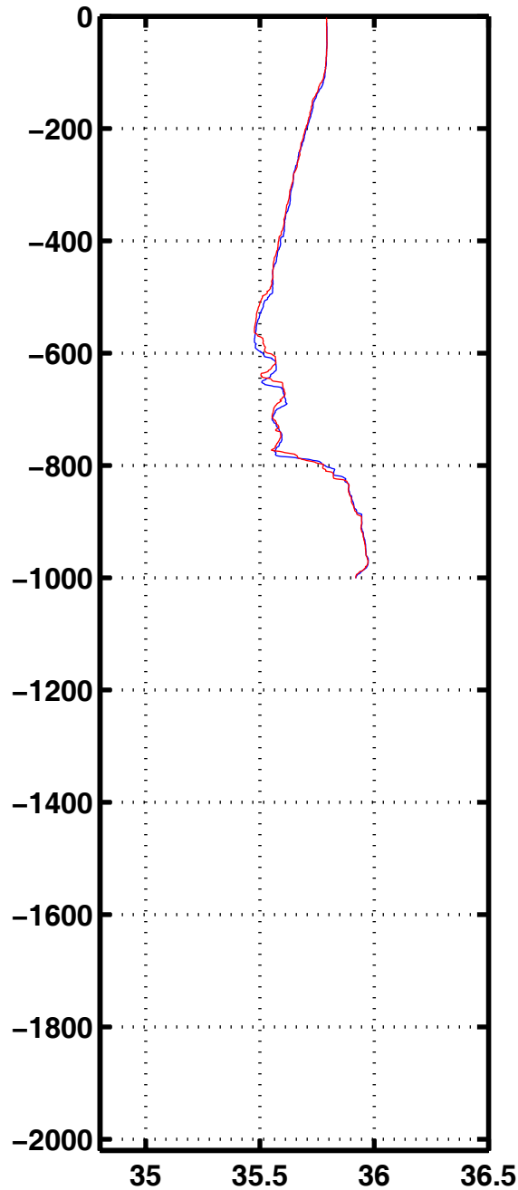
Sali 1200
