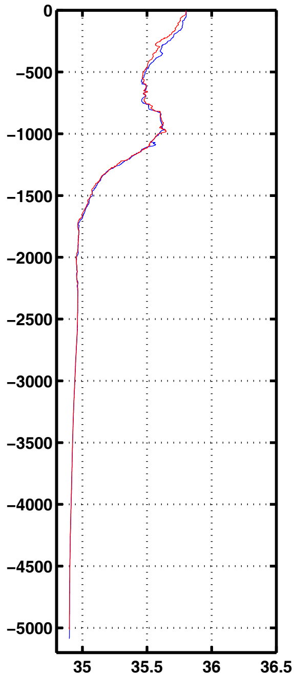
Sali 1051
