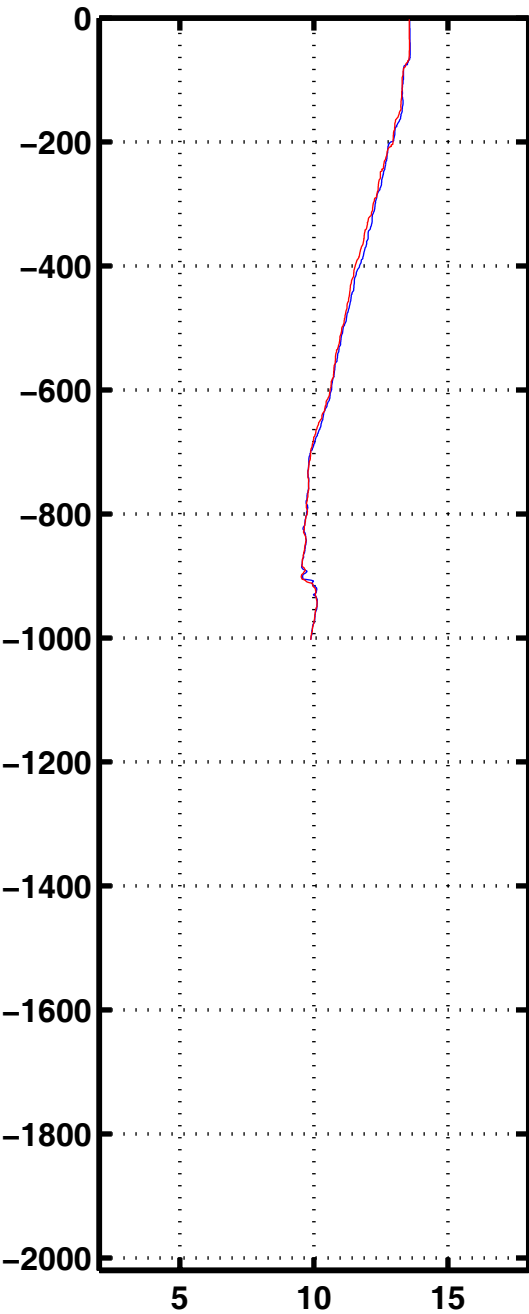
Tempe 1157
