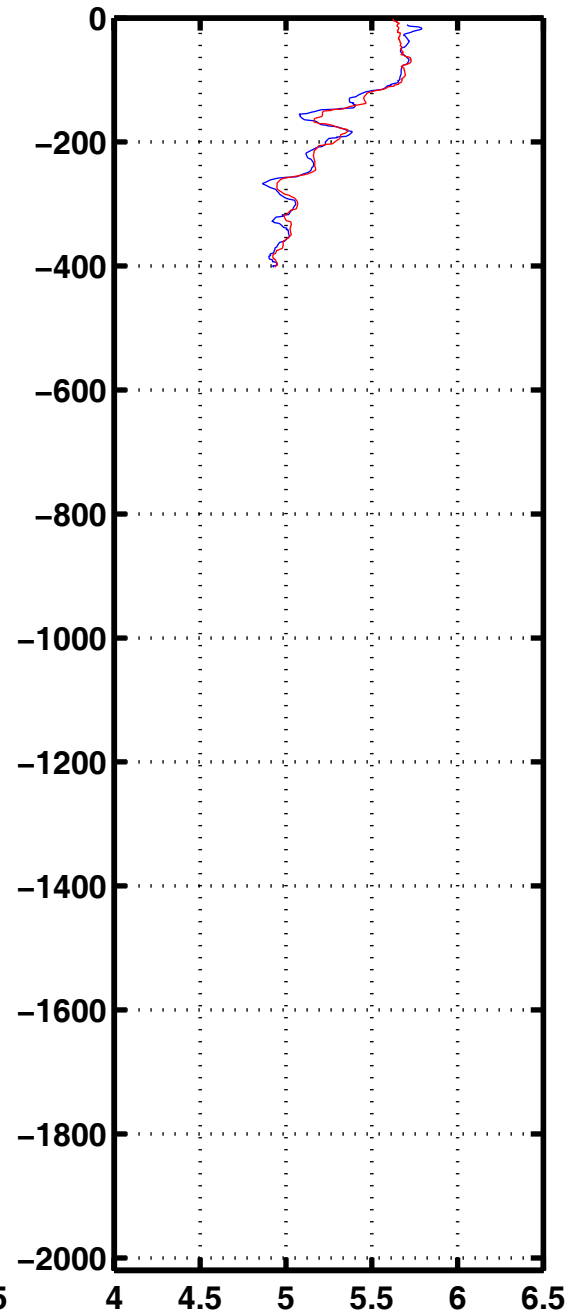
Oxyg 1117
