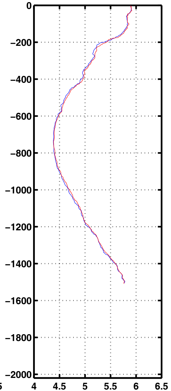
Oxyg 1140
