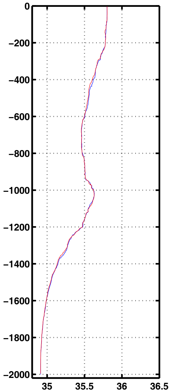
Sali 1067
