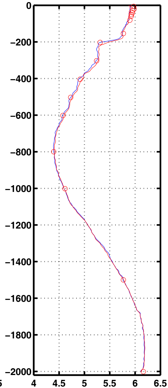
Oxyg 1047
