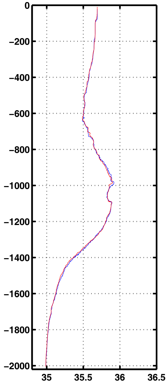
Sali 1008
