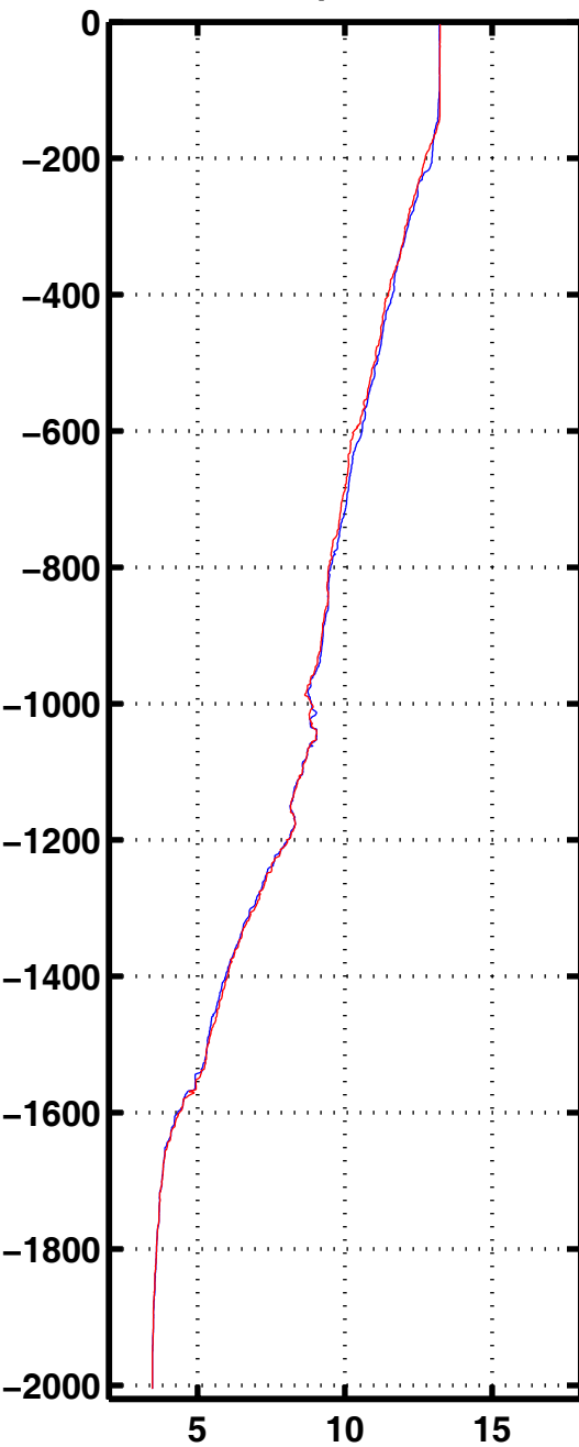
Tempe 1042
