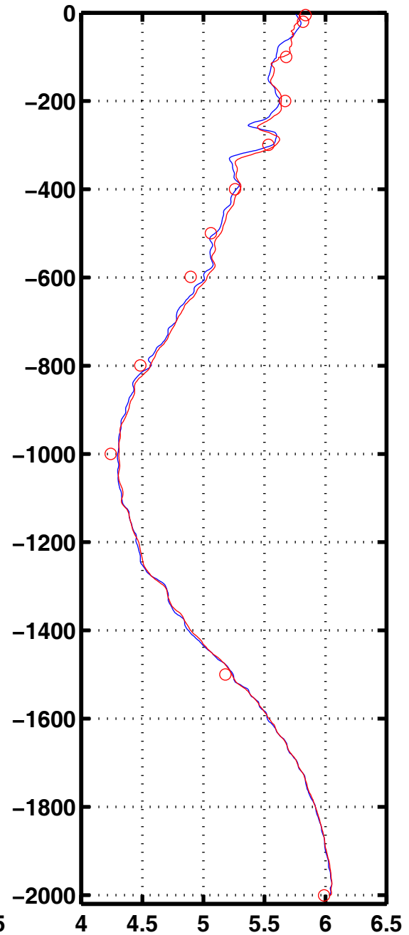
Oxyg 1054
