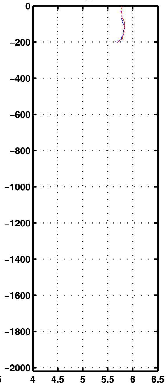
Oxyg 1112
