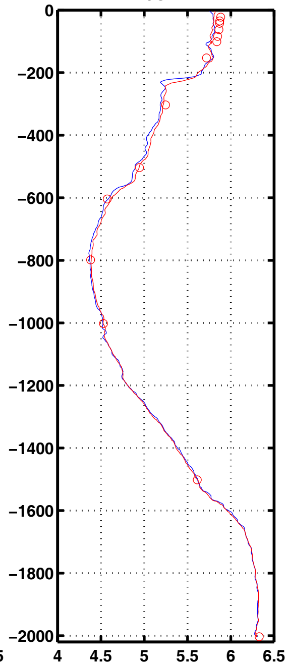
Oxyg 1042
