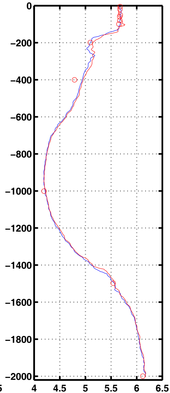
Oxyg 1073
