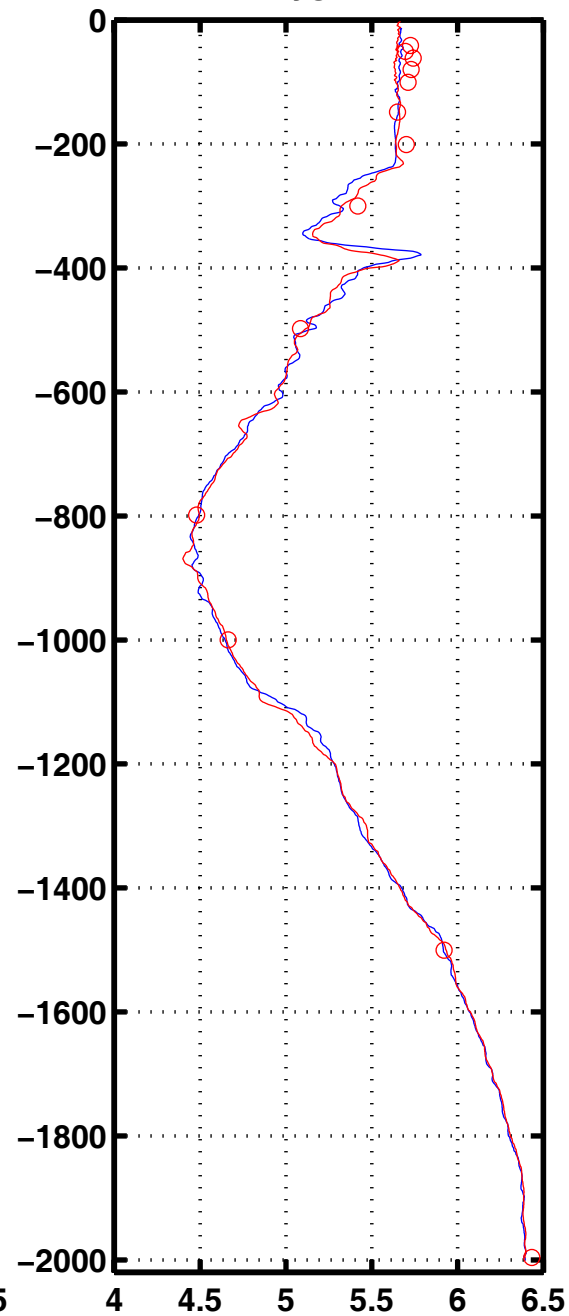
Oxyg 1017
