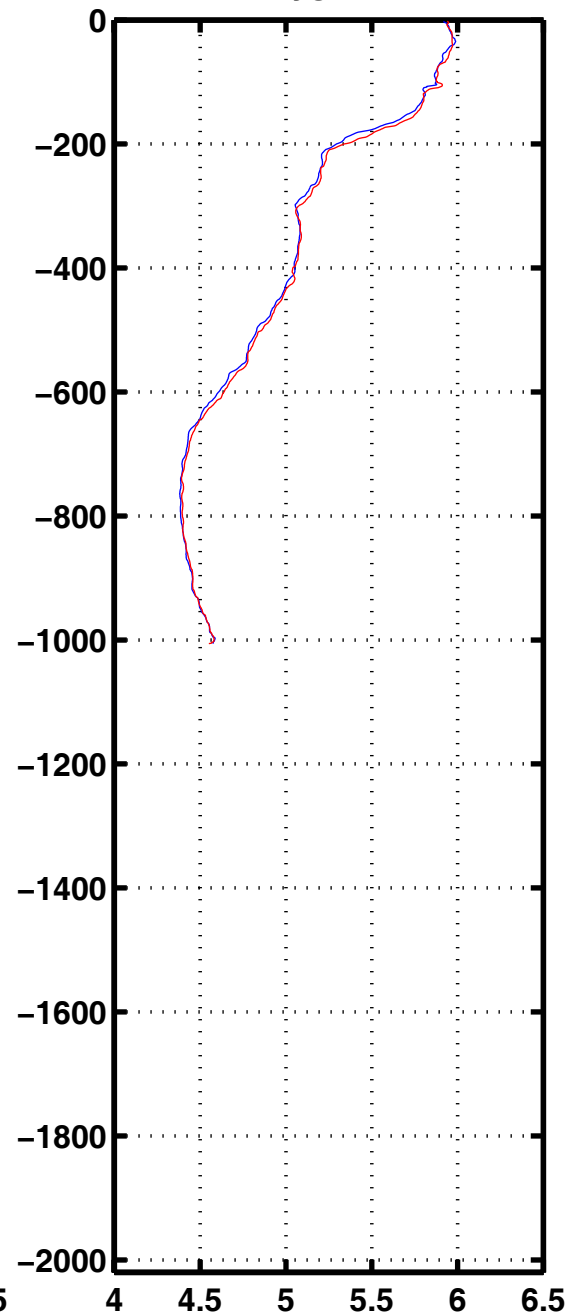
Oxyg 1106
