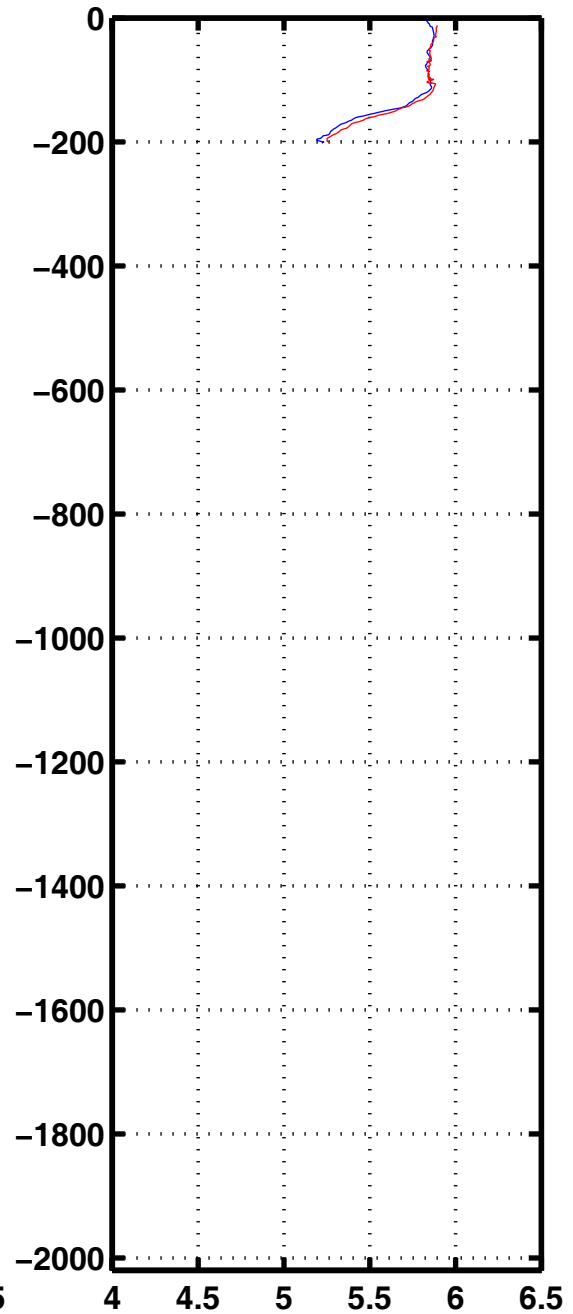
Oxyg 1137
