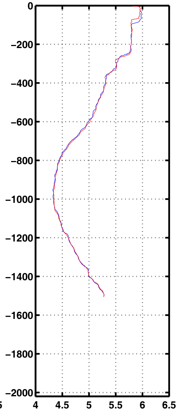
Oxyg 1176
