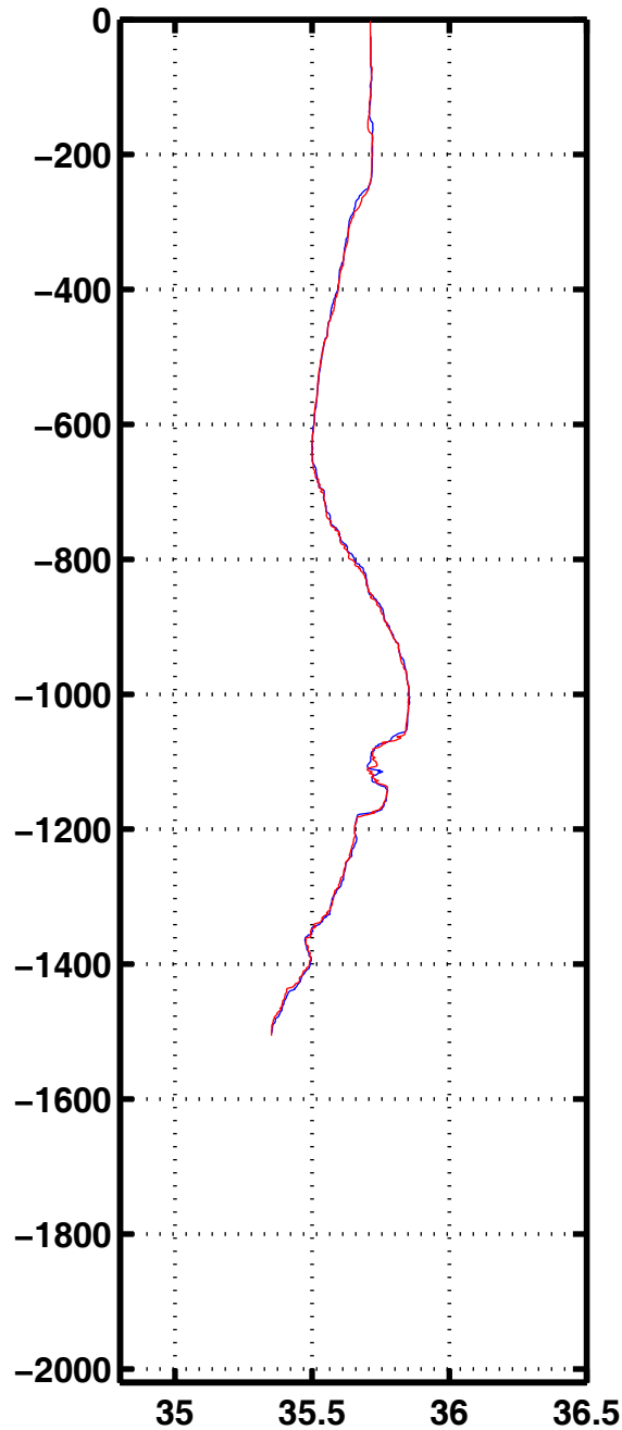
Sali 1176
