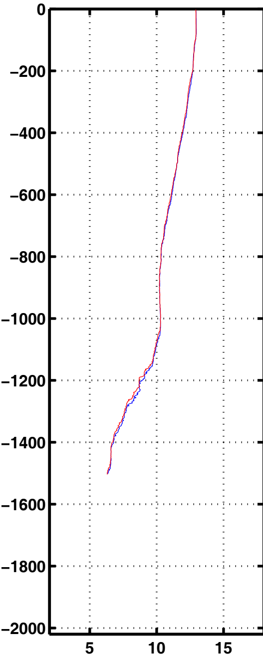
Tempe 1167
