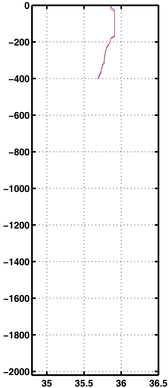
Sali 1090
