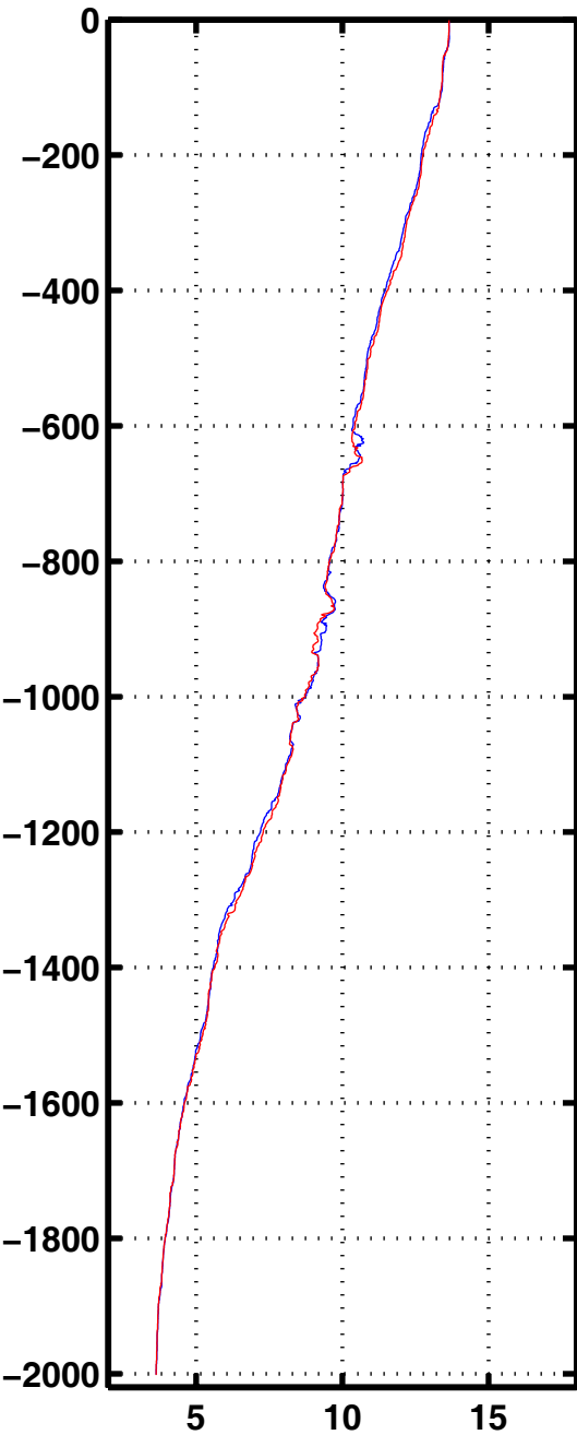
Tempe 1038
