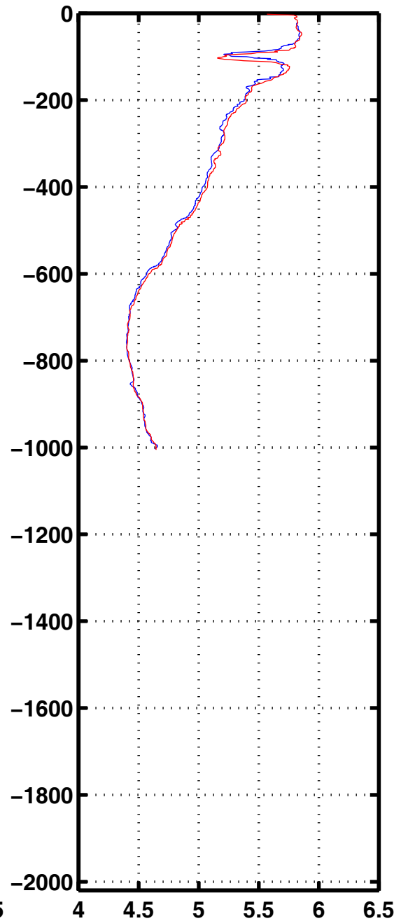
Oxyg 1153
