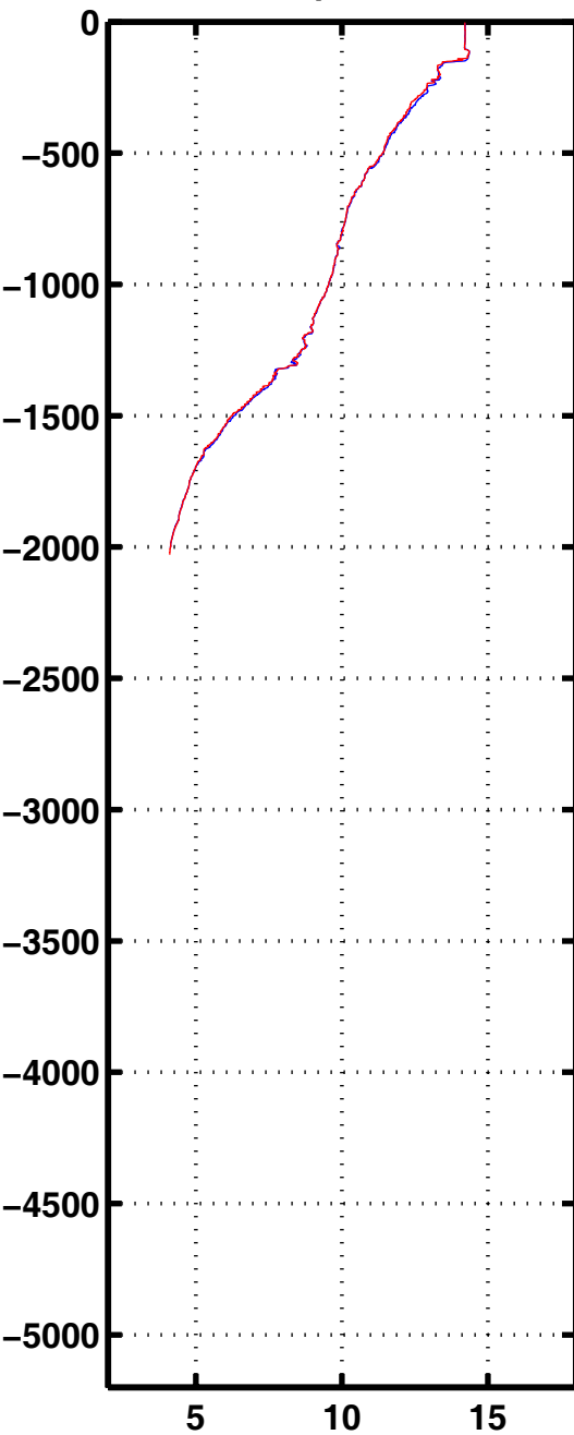
Tempe 1002
