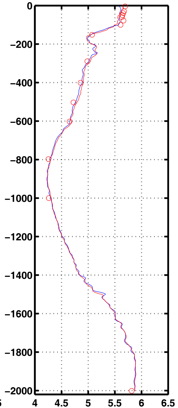
Oxyg 1057
