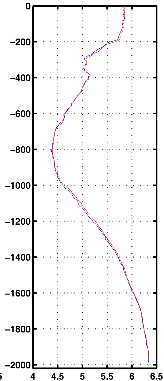
Oxyg 1065
