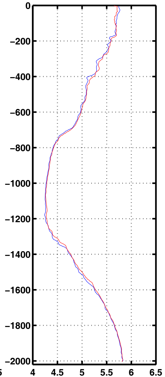
Oxyg 1093
