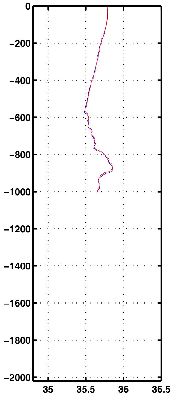
Sali 1196
