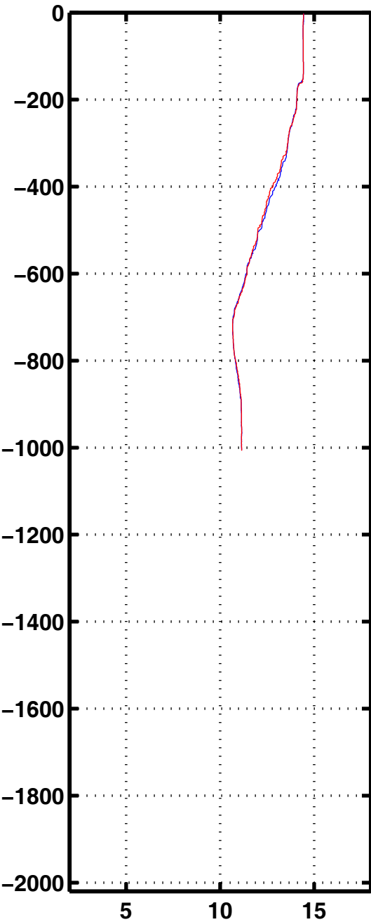
Tempe 1086
