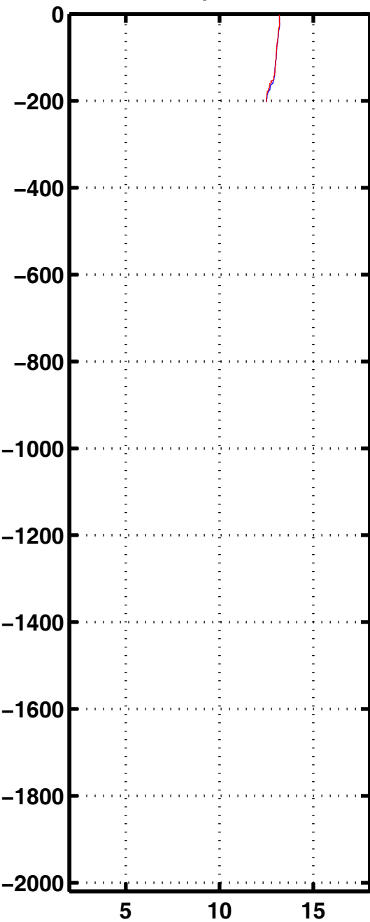
Tempe 1144
