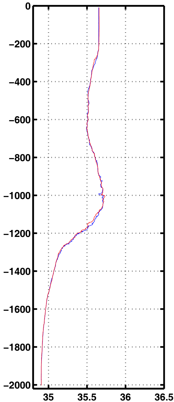
Sali 1012
