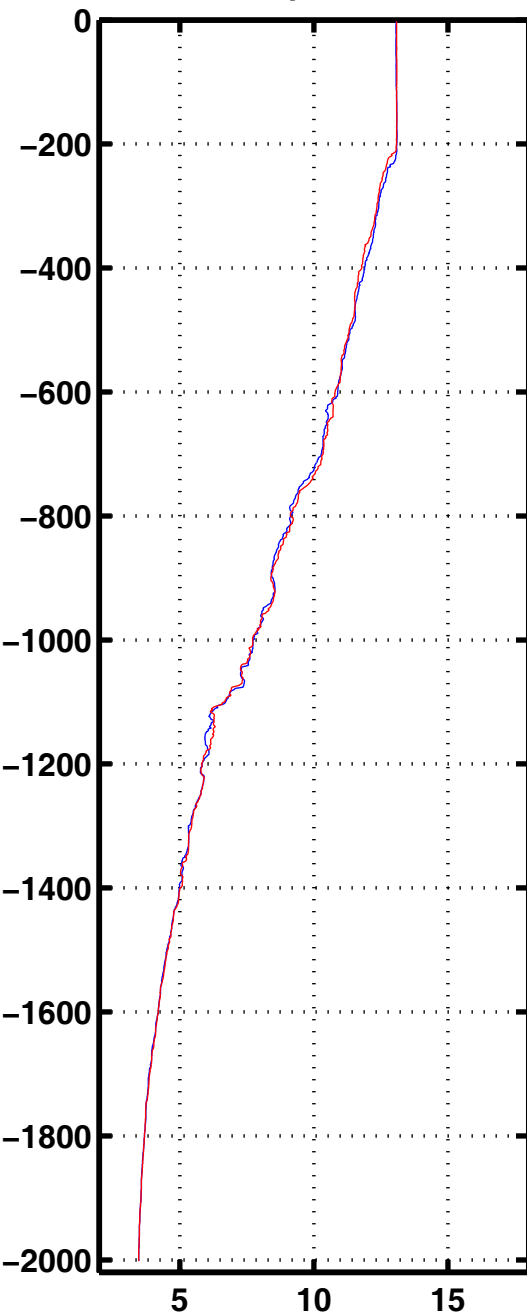
Tempe 1018
