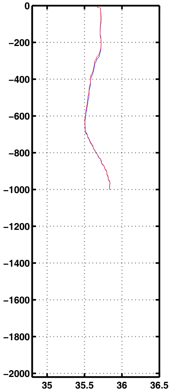
Sali 1178
