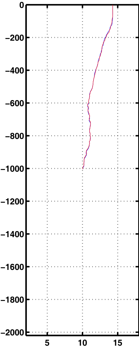
Tempe 1202
