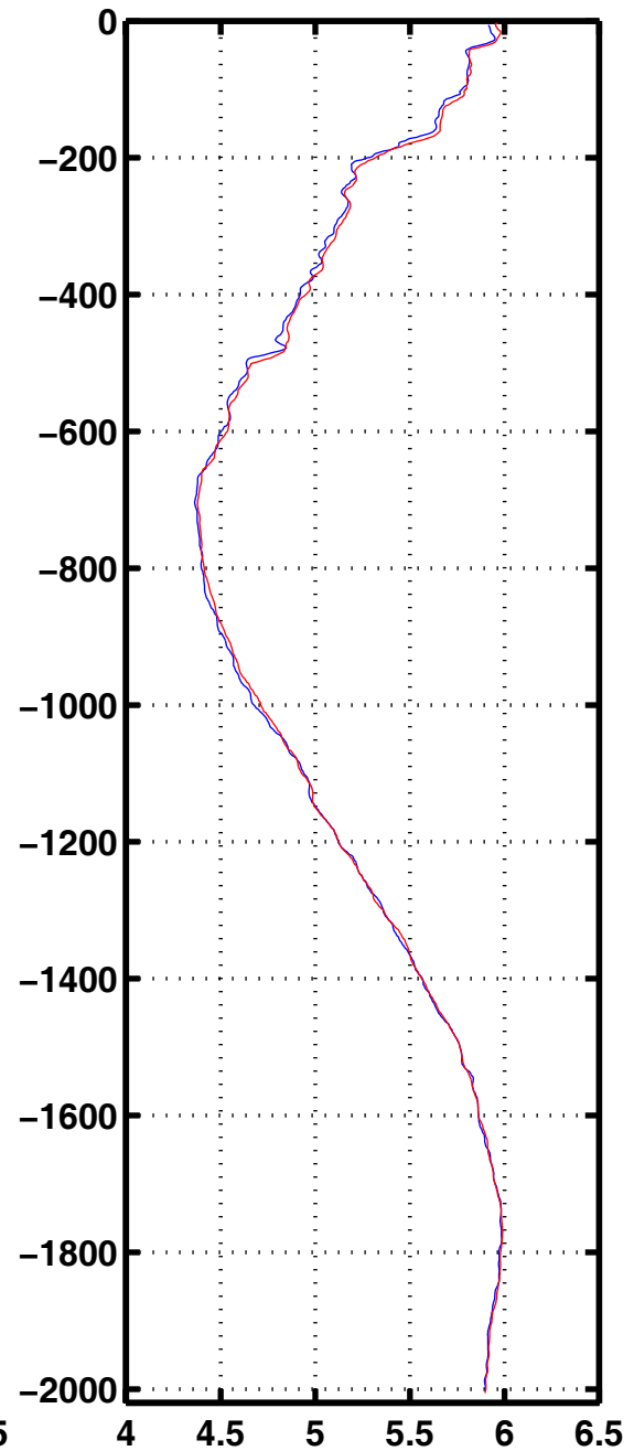
Oxyg 1149
