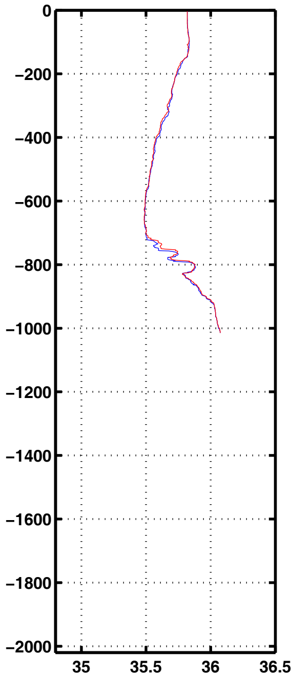
Sali 1204
