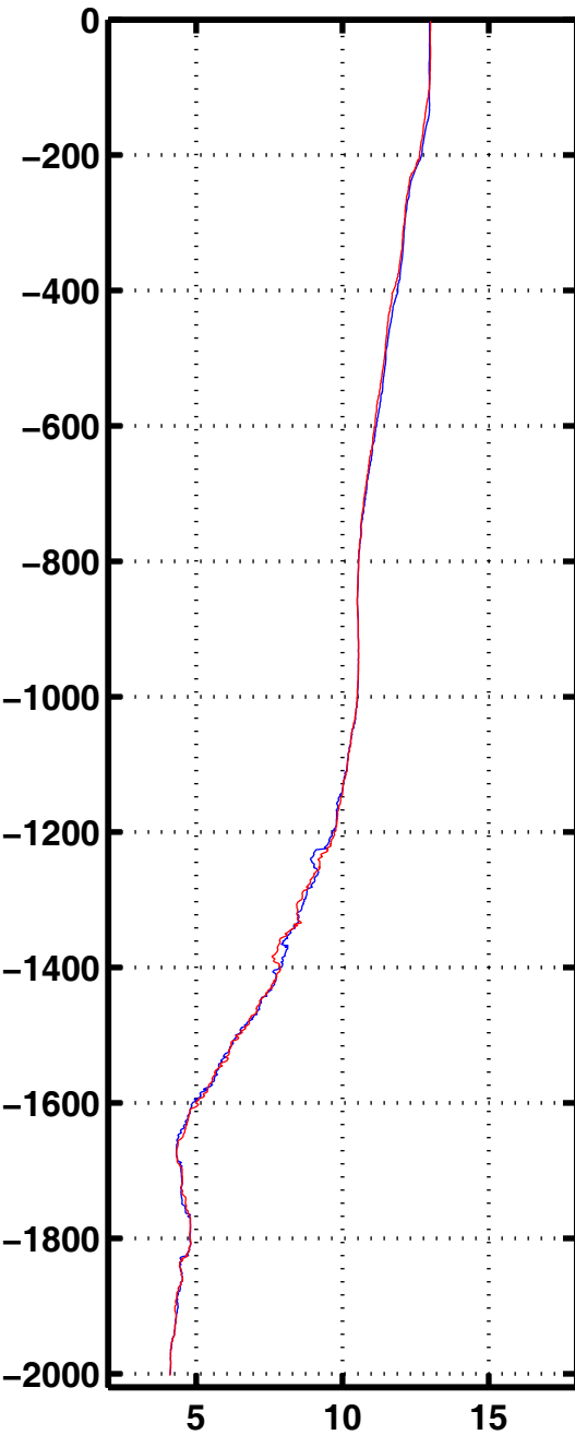
Tempe 1023
