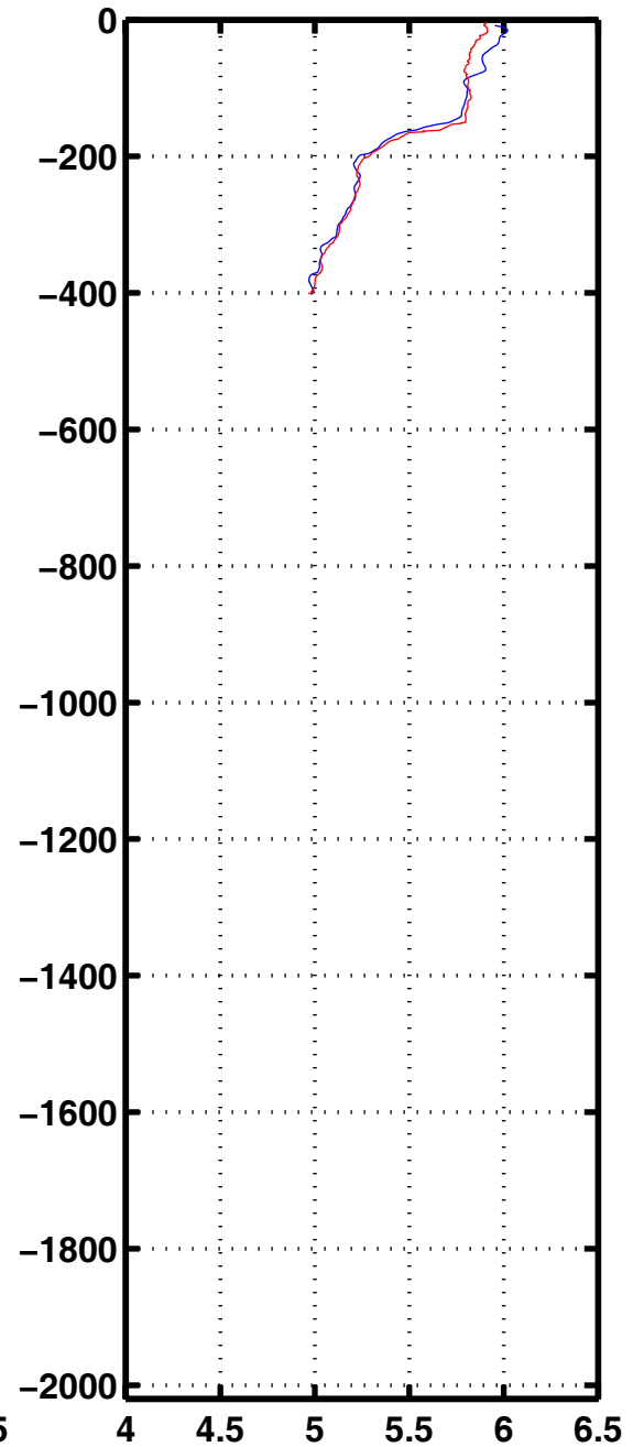
Oxyg 1146
