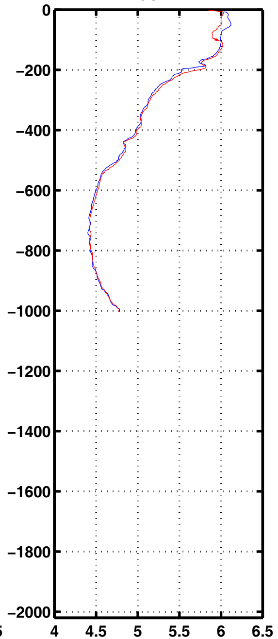
Oxyg 1151
