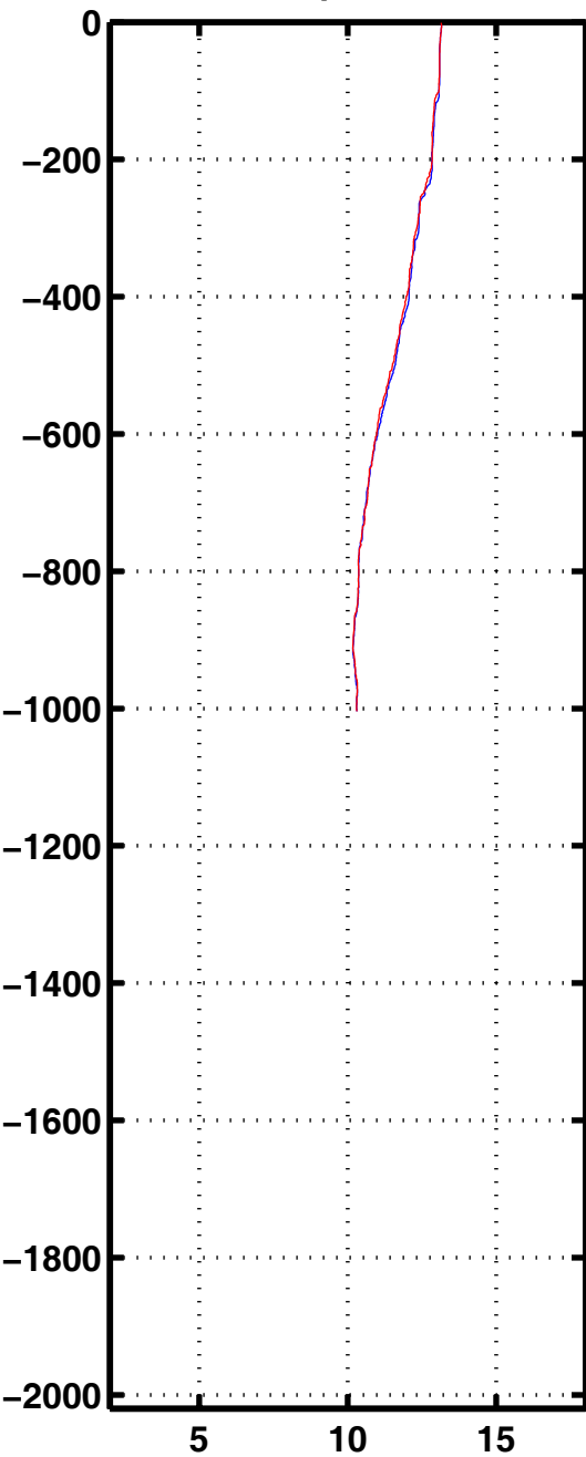
Tempe 1162
