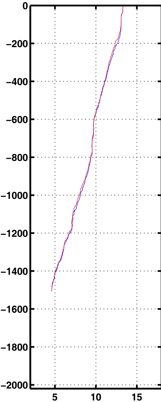
Tempe 1140
