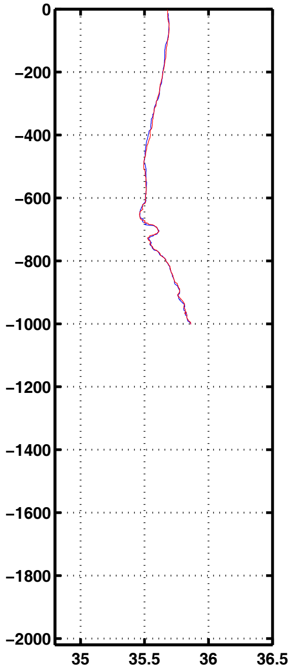
Sali 1187
