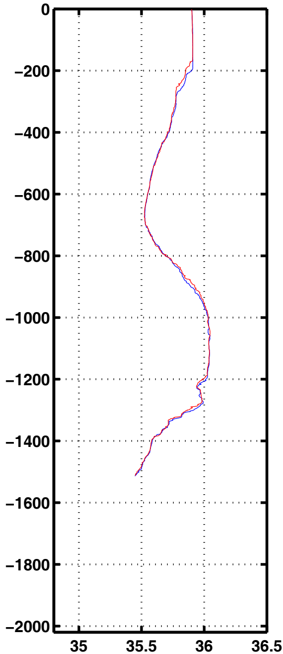
Sali 1082
