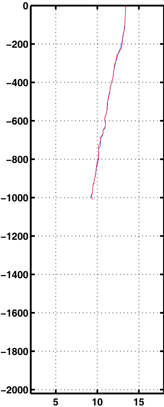
Tempe 1197
