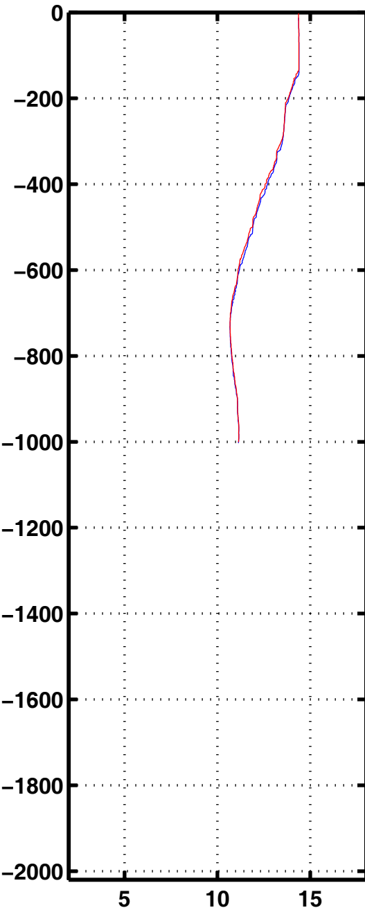
Tempe 1099
