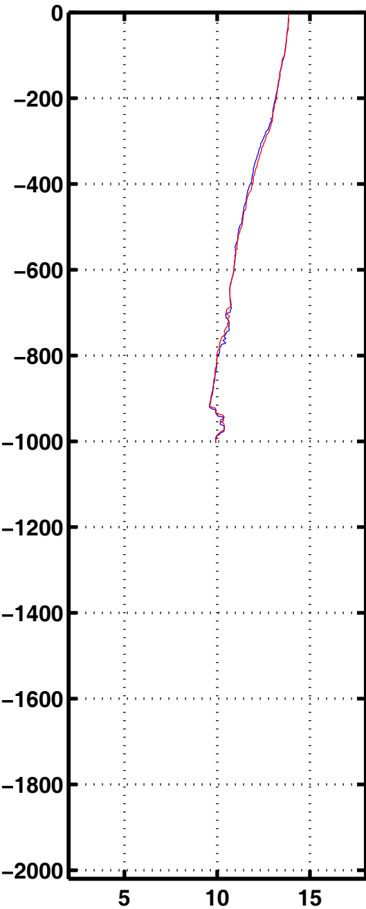
Tempe 1199
