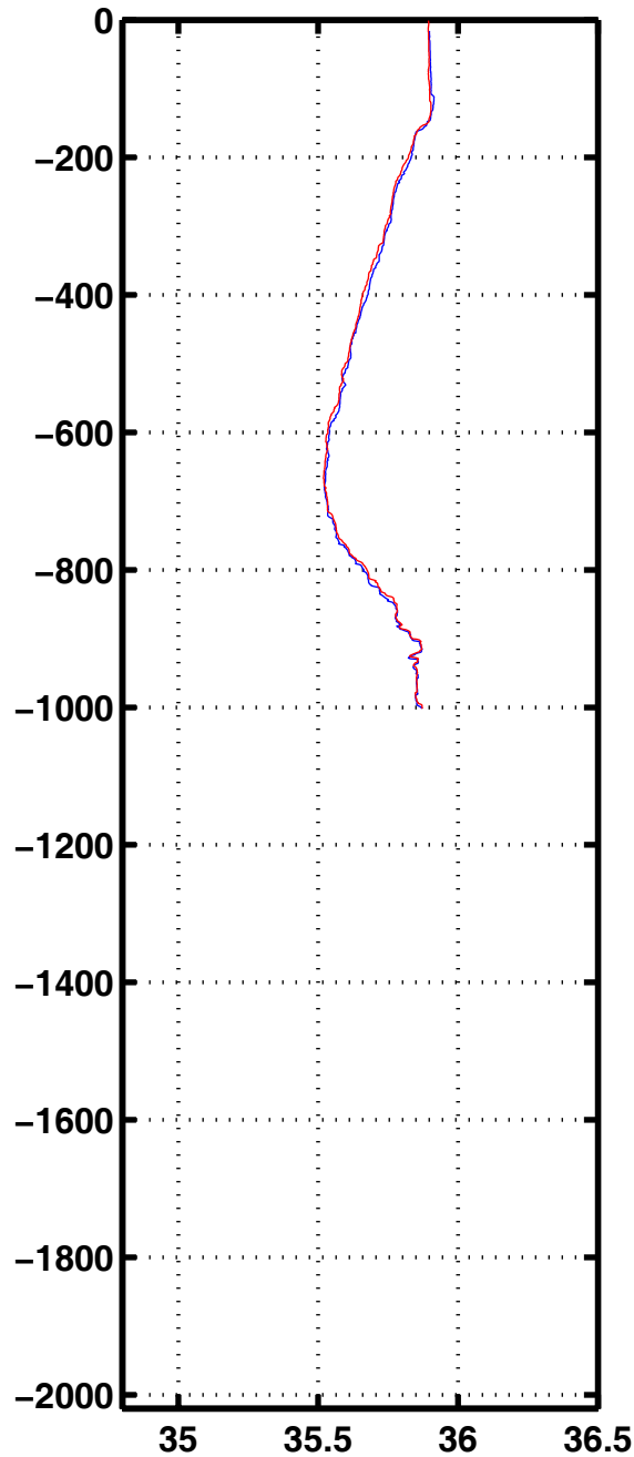
Sali 1100
