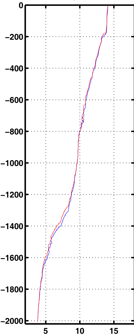
Tempe 1004
